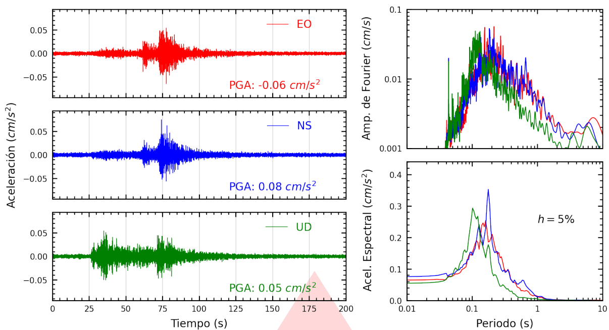
Figura A.1: Registros tiempo-historia, espectros de Fourier y de respuesta en las direcciones EO, NS y vertical de la estación UNIA. Sismo de Yurimaguas, Alto Amazonas - Loreto del 2026-01-04, 17:17:28 (Hora local)
