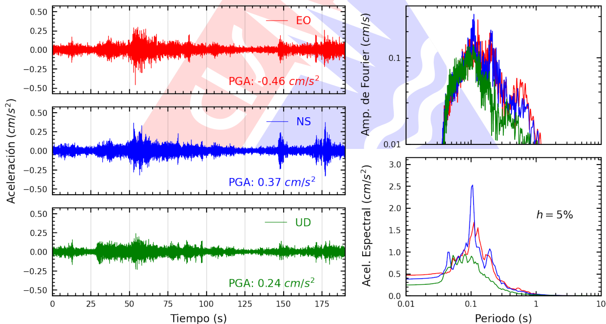
Figura A.12: Registros tiempo-historia, espectros de Fourier y de respuesta en las direcciones EO, NS y vertical de la estación SCCHO. Sismo de Pisco, Pisco - Ica del 2026-01-15, 22:46:47 (Hora local)
