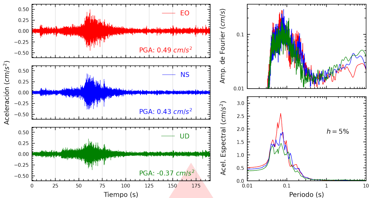
Figura A.11: Registros tiempo-historia, espectros de Fourier y de respuesta en las direcciones EO, NS y vertical de la estación INDEP. Sismo de Pisco, Pisco - Ica del 2026-01-15, 22:46:47 (Hora local)
