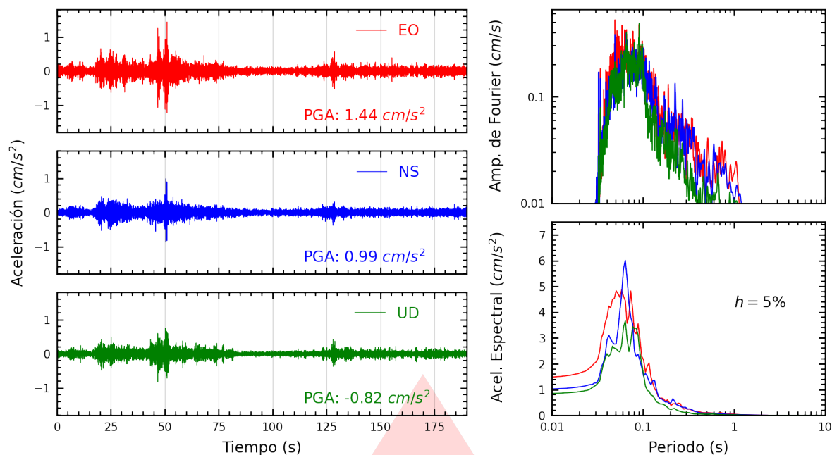
Figura A.3: Registros tiempo-historia, espectros de Fourier y de respuesta en las direcciones EO, NS y vertical de la estación SOBAR. Sismo de Pisco, Pisco - Ica del 2026-01-15, 22:46:47 (Hora local)
