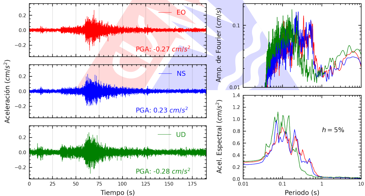
Figura A.20: Registros tiempo-historia, espectros de Fourier y de respuesta en las direcciones EO, NS y vertical de la estación MDPP. Sismo de Pisco, Pisco - Ica del 2026-01-15, 22:46:47 (Hora local)
