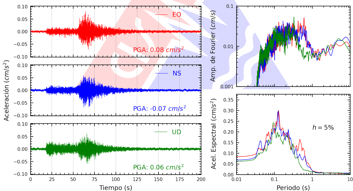
Figura A.34: Registros tiempo-historia, espectros de Fourier y de respuesta en las direcciones EO, NS y vertical de la estación CARAL. Sismo de Pisco, Pisco - Ica del 2026-01-15, 22:46:47 (Hora local)
