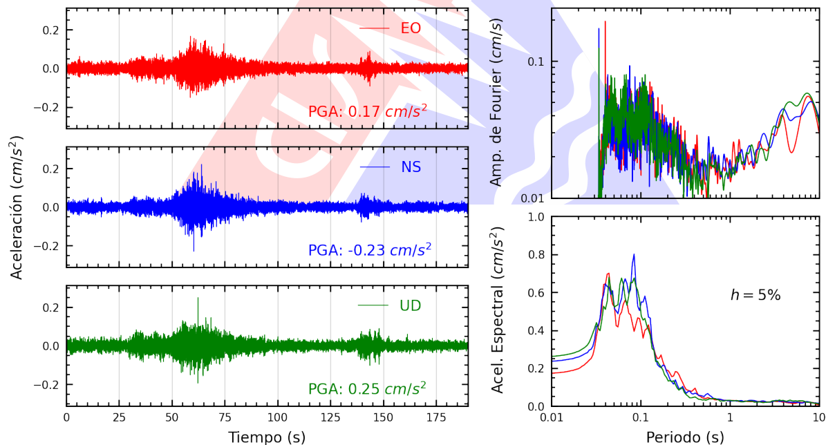
Figura A.22: Registros tiempo-historia, espectros de Fourier y de respuesta en las direcciones EO, NS y vertical de la estación USMP. Sismo de Pisco, Pisco - Ica del 2026-01-15, 22:46:47 (Hora local)
