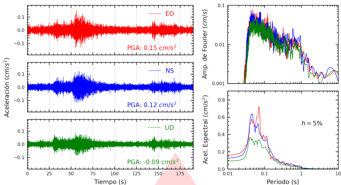
Figura A.31: Registros tiempo-historia, espectros de Fourier y de respuesta en las direcciones EO, NS y vertical de la estación BORJA. Sismo de Pisco, Pisco - Ica del 2026-01-15, 22:46:47 (Hora local)
