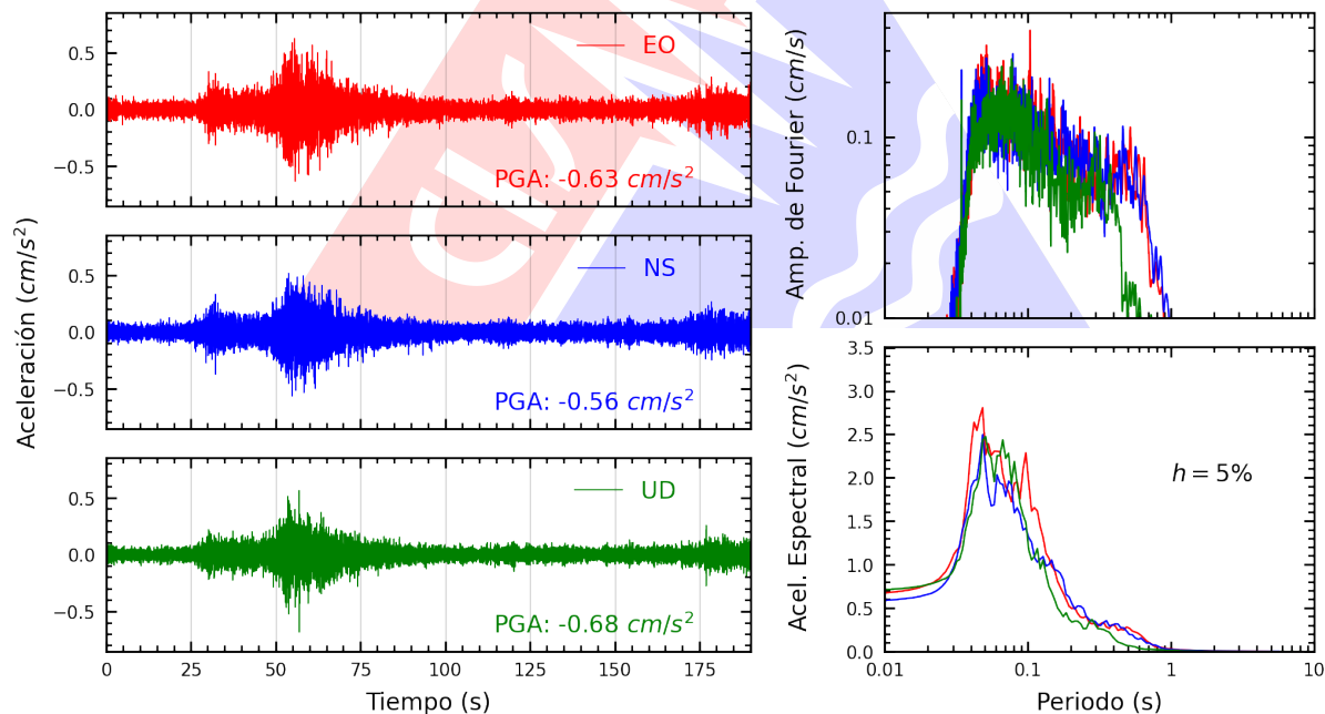
Figura A.8: Registros tiempo-historia, espectros de Fourier y de respuesta en las direcciones EO, NS y vertical de la estación UNTEL. Sismo de Pisco, Pisco - Ica del 2026-01-15, 22:46:47 (Hora local)
