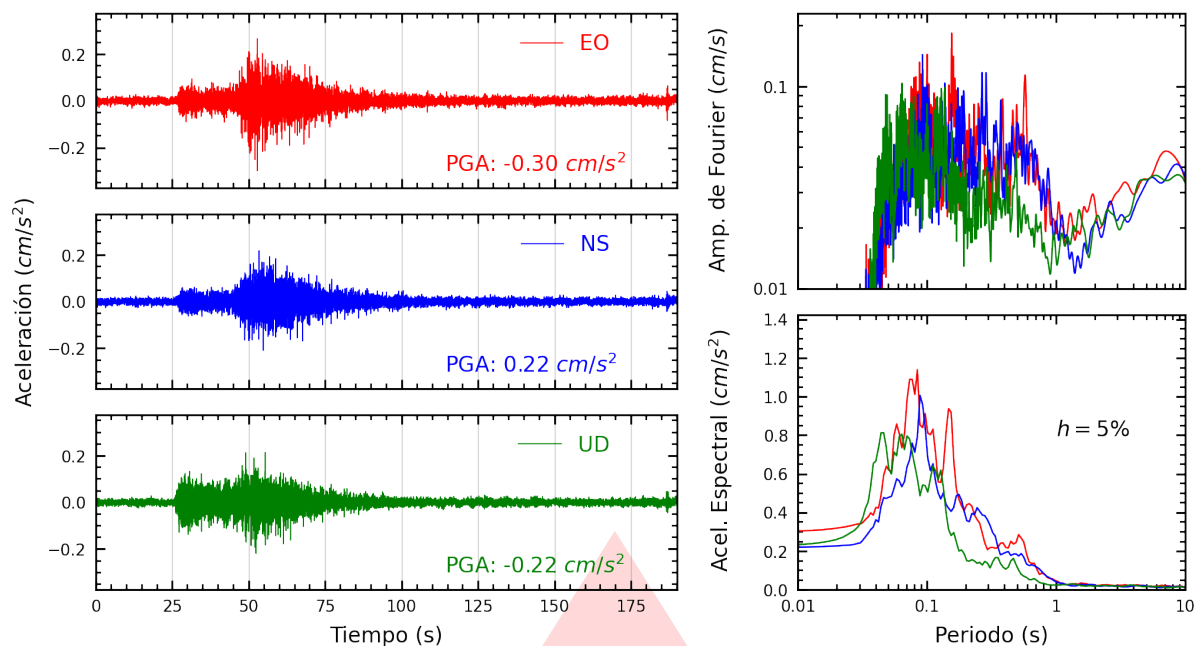
Figura A.19: Registros tiempo-historia, espectros de Fourier y de respuesta en las direcciones EO, NS y vertical de la estación USILP. Sismo de Pisco, Pisco - Ica del 2026-01-15, 22:46:47 (Hora local)
