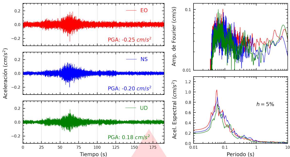
Figura A.25: Registros tiempo-historia, espectros de Fourier y de respuesta en las direcciones EO, NS y vertical de la estación IMCA. Sismo de Pisco, Pisco - Ica del 2026-01-15, 22:46:47 (Hora local)
