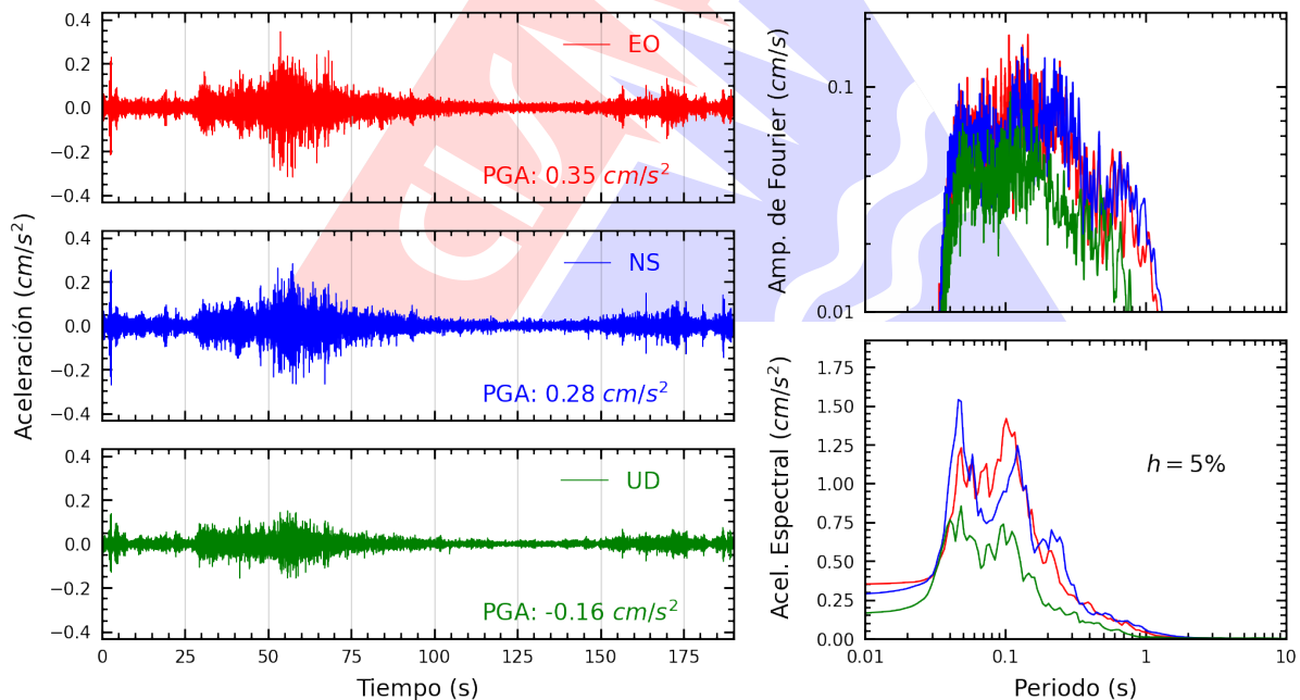
Figura A.16: Registros tiempo-historia, espectros de Fourier y de respuesta en las direcciones EO, NS y vertical de la estación BRISA. Sismo de Pisco, Pisco - Ica del 2026-01-15, 22:46:47 (Hora local)
