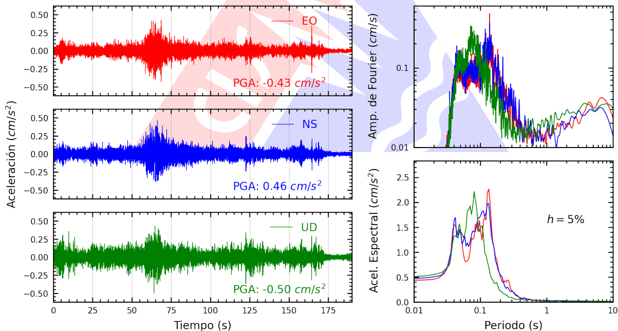
Figura A.10: Registros tiempo-historia, espectros de Fourier y de respuesta en las direcciones EO, NS y vertical de la estación CARAB. Sismo de Pisco, Pisco - Ica del 2026-01-15, 22:46:47 (Hora local)
