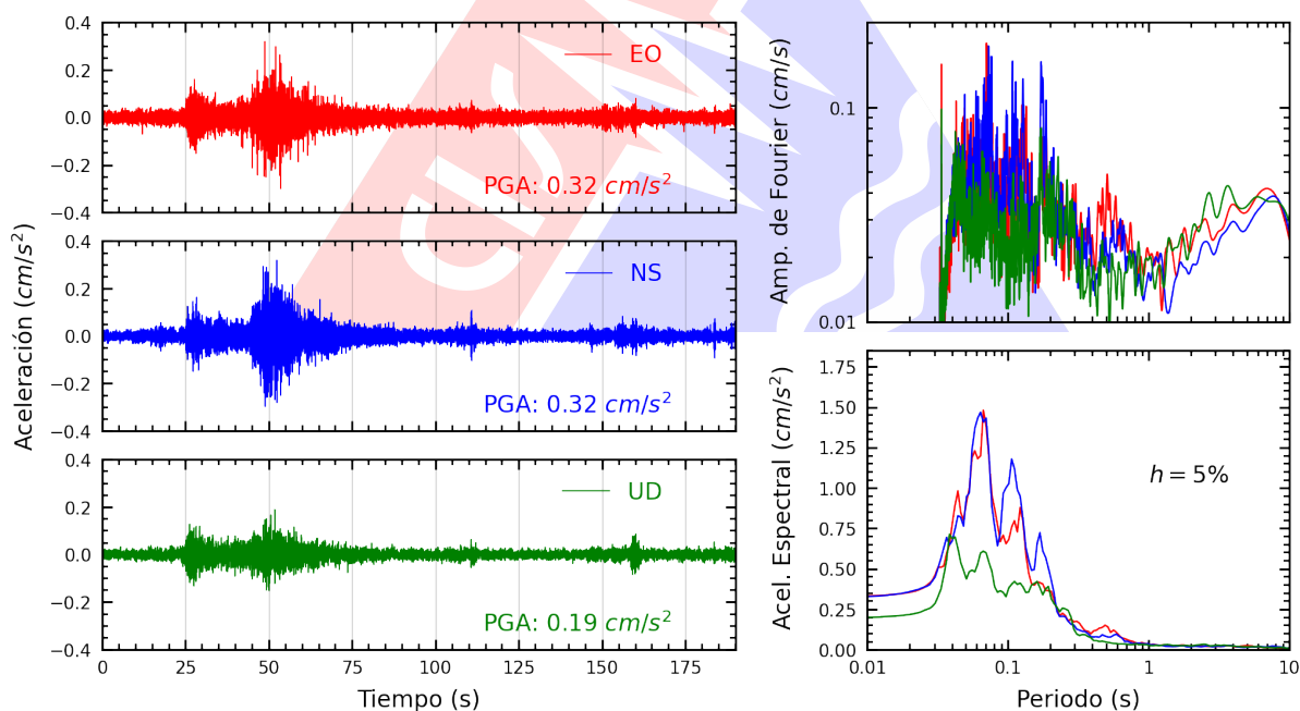
Figura A.18: Registros tiempo-historia, espectros de Fourier y de respuesta en las direcciones EO, NS y vertical de la estación UPCVI. Sismo de Pisco, Pisco - Ica del 2026-01-15, 22:46:47 (Hora local)
