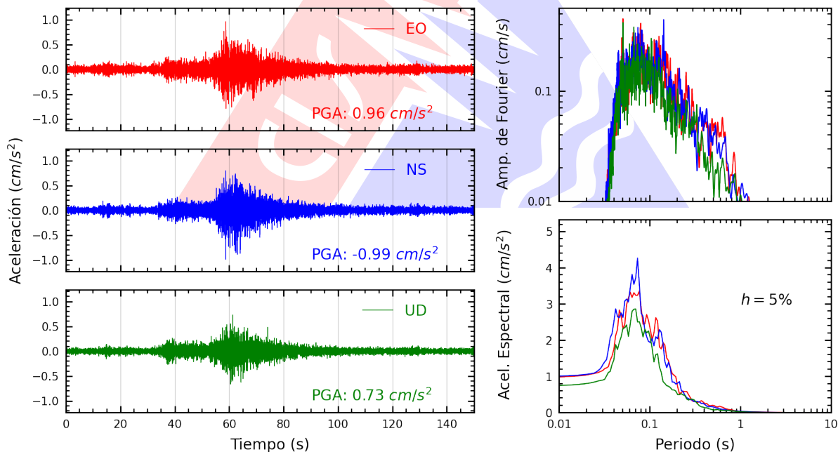
Figura A.4: Registros tiempo-historia, espectros de Fourier y de respuesta en las direcciones EO, NS y vertical de la estación PHERM. Sismo de Pisco, Pisco - Ica del 2026-01-15, 22:46:47 (Hora local)
