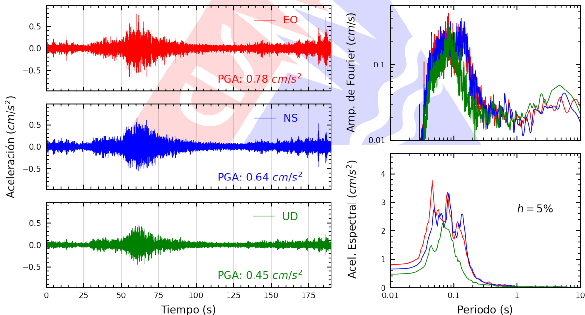
Figura A.6: Registros tiempo-historia, espectros de Fourier y de respuesta en las direcciones EO, NS y vertical de la estación USILM. Sismo de Pisco, Pisco - Ica del 2026-01-15, 22:46:47 (Hora local)
