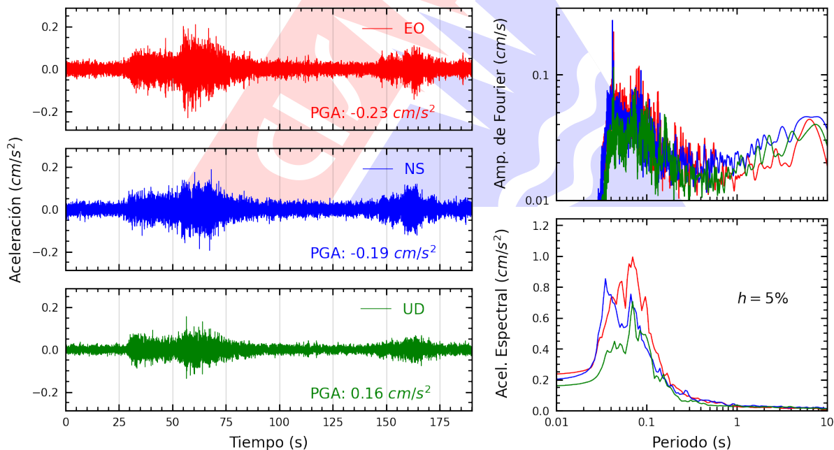
Figura A.26: Registros tiempo-historia, espectros de Fourier y de respuesta en las direcciones EO, NS y vertical de la estación CEPRE. Sismo de Pisco, Pisco - Ica del 2026-01-15, 22:46:47 (Hora local)
