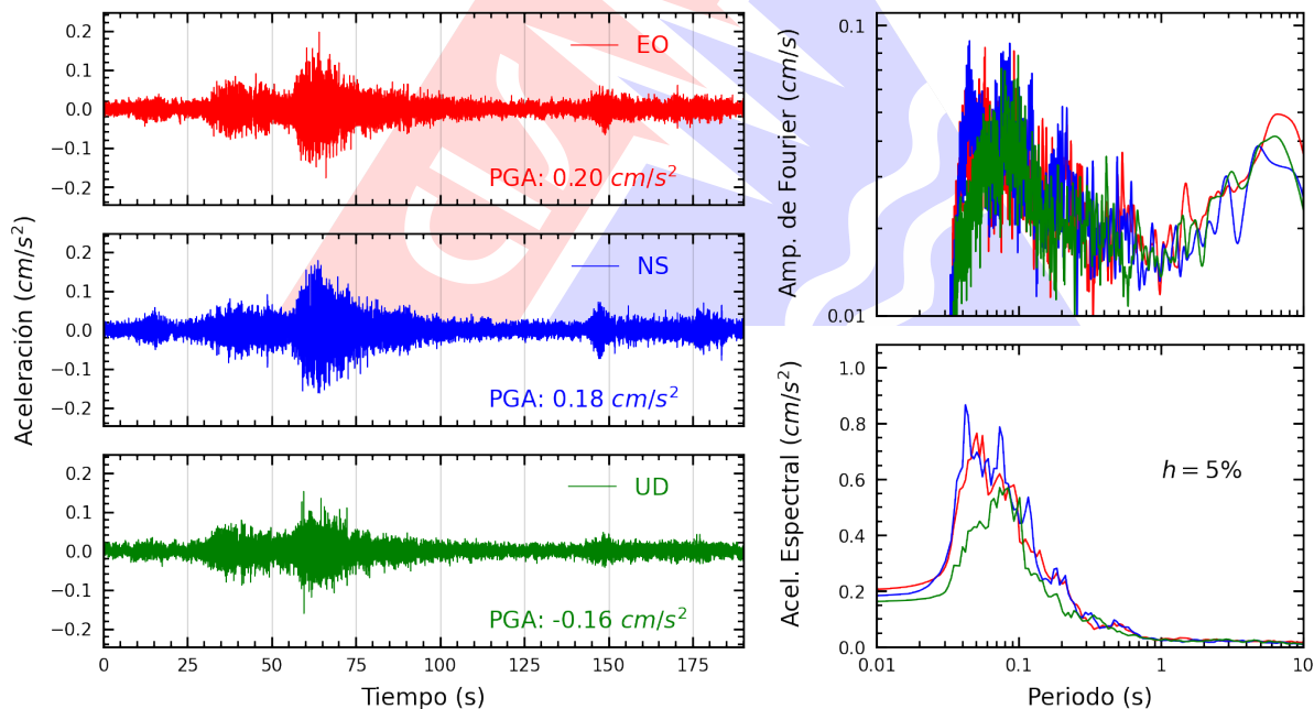
Figura A.28: Registros tiempo-historia, espectros de Fourier y de respuesta en las direcciones EO, NS y vertical de la estación COMAS. Sismo de Pisco, Pisco - Ica del 2026-01-15, 22:46:47 (Hora local)
