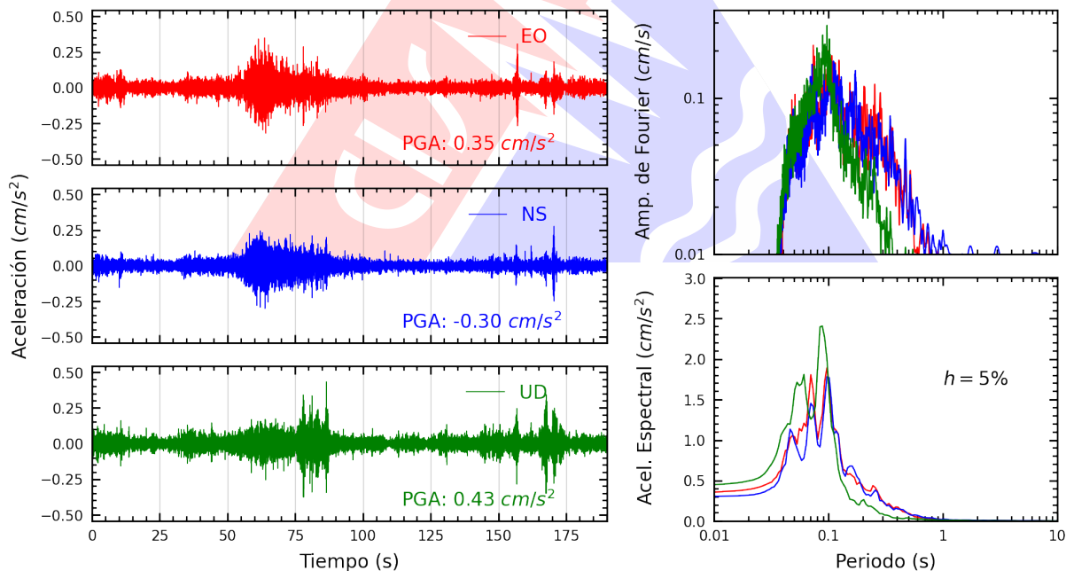
Figura A.14: Registros tiempo-historia, espectros de Fourier y de respuesta en las direcciones EO, NS y vertical de la estación SCOLI. Sismo de Pisco, Pisco - Ica del 2026-01-15, 22:46:47 (Hora local)
