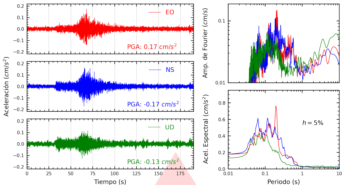
Figura A.29: Registros tiempo-historia, espectros de Fourier y de respuesta en las direcciones EO, NS y vertical de la estación VHAYA. Sismo de Pisco, Pisco - Ica del 2026-01-15, 22:46:47 (Hora local)
