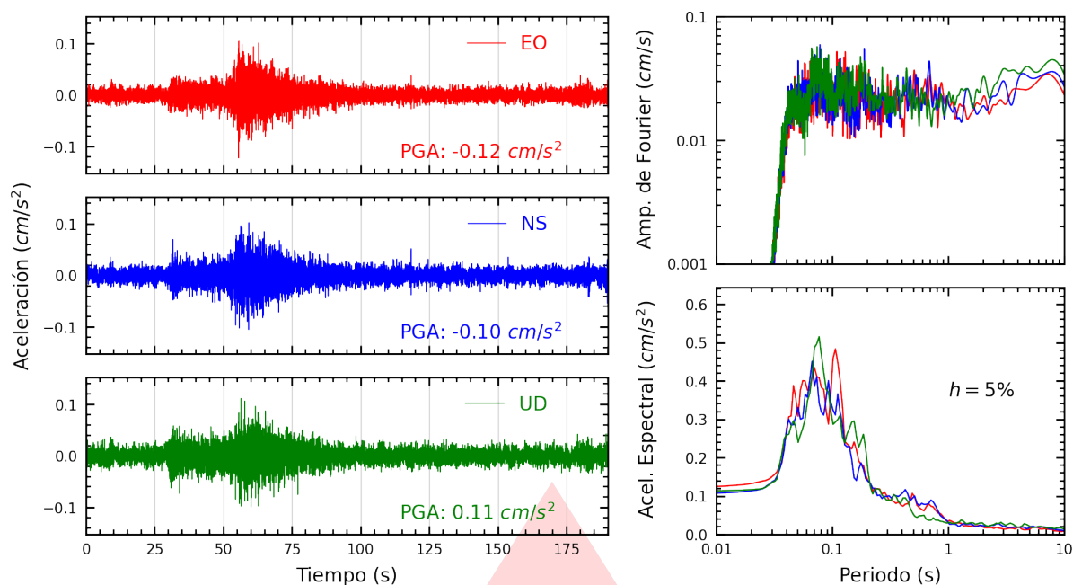
Figura A.33: Registros tiempo-historia, espectros de Fourier y de respuesta en las direcciones EO, NS y vertical de la estación UNFV. Sismo de Pisco, Pisco - Ica del 2026-01-15, 22:46:47 (Hora local)
