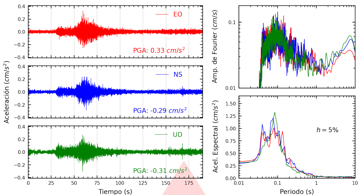
Figura A.17: Registros tiempo-historia, espectros de Fourier y de respuesta en las direcciones EO, NS y vertical de la estación UCVAT. Sismo de Pisco, Pisco - Ica del 2026-01-15, 22:46:47 (Hora local)
