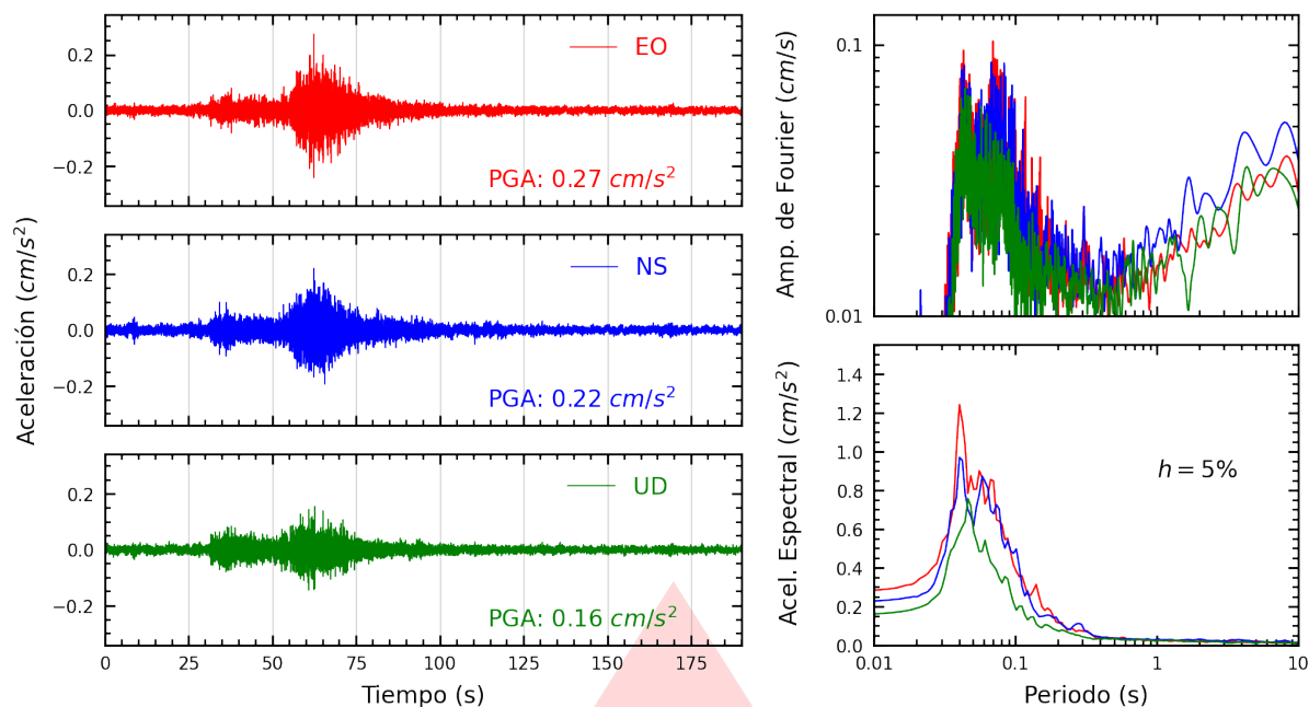
Figura A.21: Registros tiempo-historia, espectros de Fourier y de respuesta en las direcciones EO, NS y vertical de la estación SJLCE. Sismo de Pisco, Pisco - Ica del 2026-01-15, 22:46:47 (Hora local)
