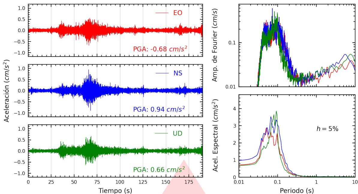
Figura A.5: Registros tiempo-historia, espectros de Fourier y de respuesta en las direcciones EO, NS y vertical de la estación SROSA. Sismo de Pisco, Pisco - Ica del 2026-01-15, 22:46:47 (Hora local)
