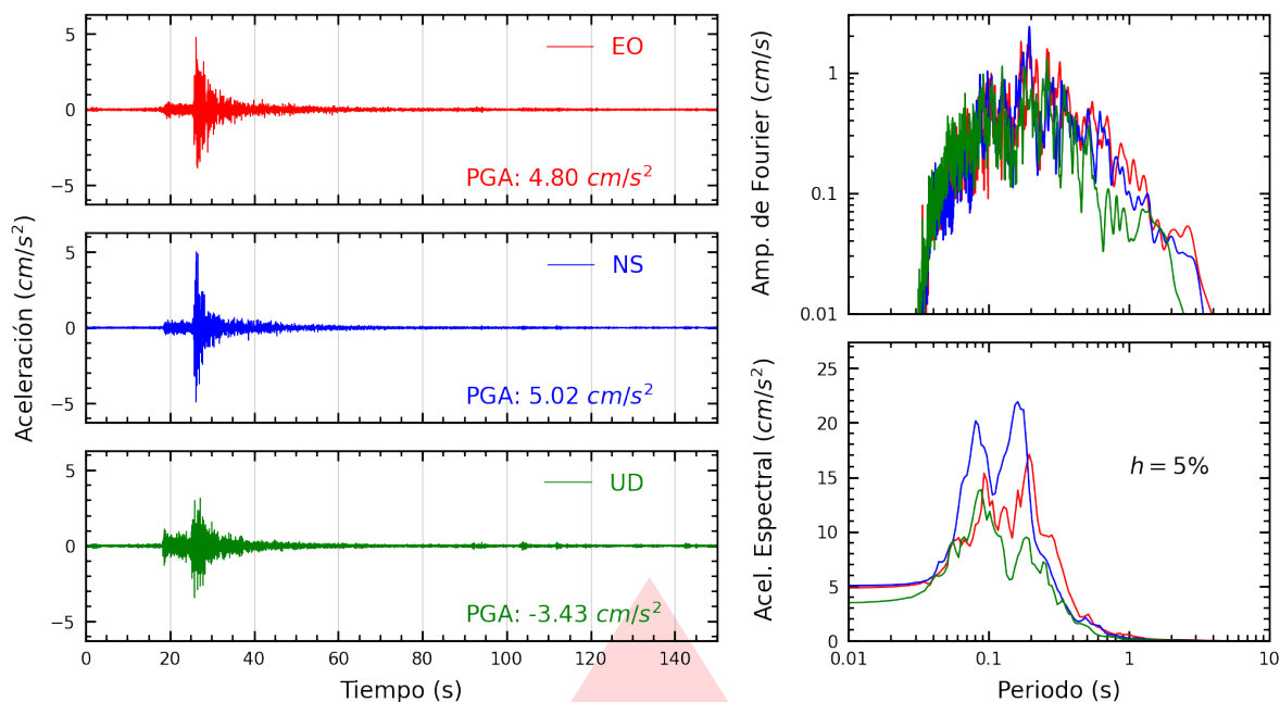
Figura A.1: Registros tiempo-historia, espectros de Fourier y de respuesta en las direcciones EO, NS y vertical de la estación SCICA. Sismo de Pisco, Pisco - Ica del 2026-01-15, 22:46:47 (Hora local)
