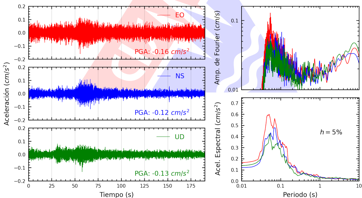
Figura A.30: Registros tiempo-historia, espectros de Fourier y de respuesta en las direcciones EO, NS y vertical de la estación INICT. Sismo de Pisco, Pisco - Ica del 2026-01-15, 22:46:47 (Hora local)
