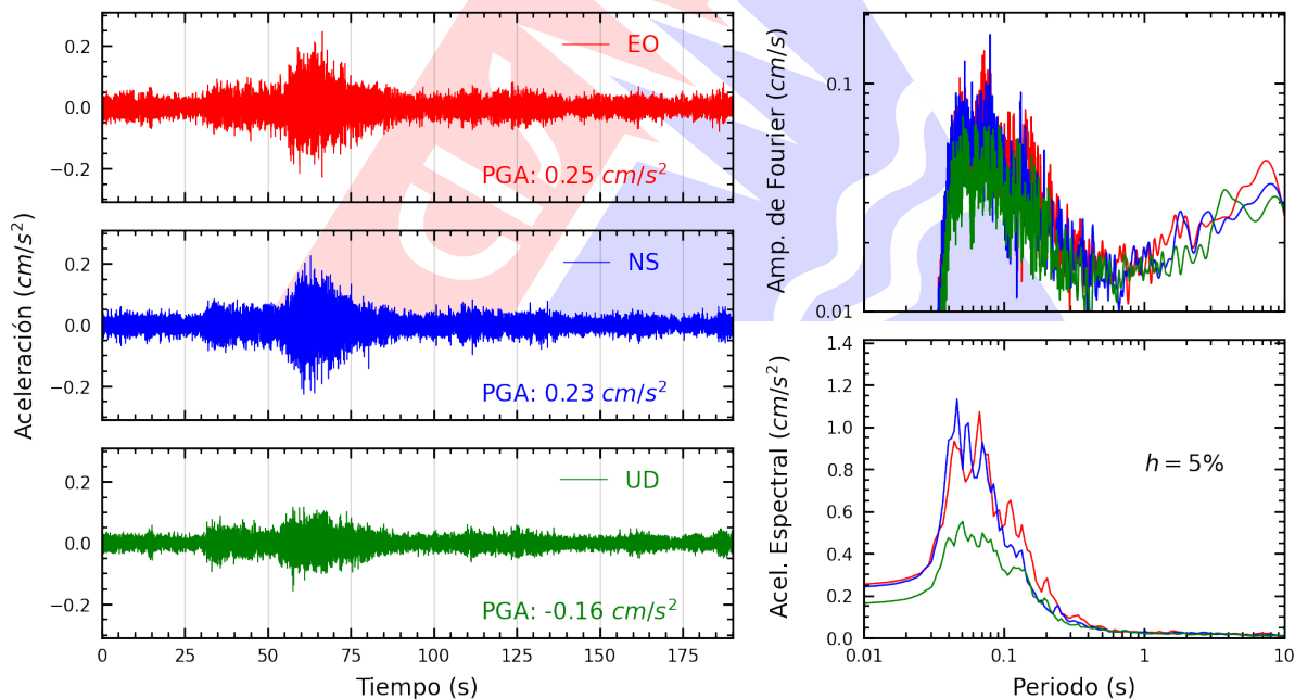
Figura A.24: Registros tiempo-historia, espectros de Fourier y de respuesta en las direcciones EO, NS y vertical de la estación FICPE. Sismo de Pisco, Pisco - Ica del 2026-01-15, 22:46:47 (Hora local)
