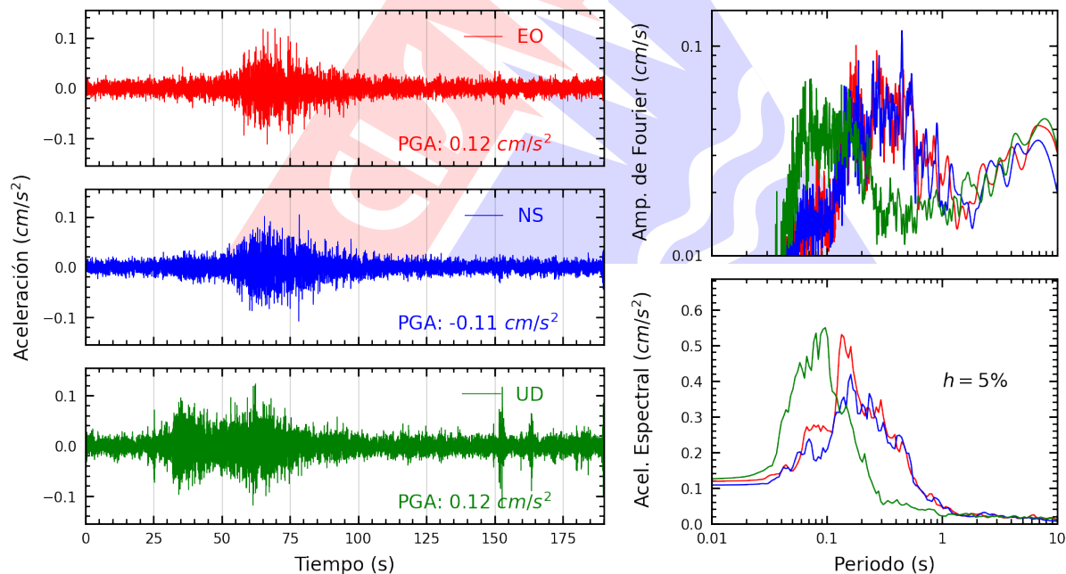
Figura A.32: Registros tiempo-historia, espectros de Fourier y de respuesta en las direcciones EO, NS y vertical de la estación ACAPU. Sismo de Pisco, Pisco - Ica del 2026-01-15, 22:46:47 (Hora local)
