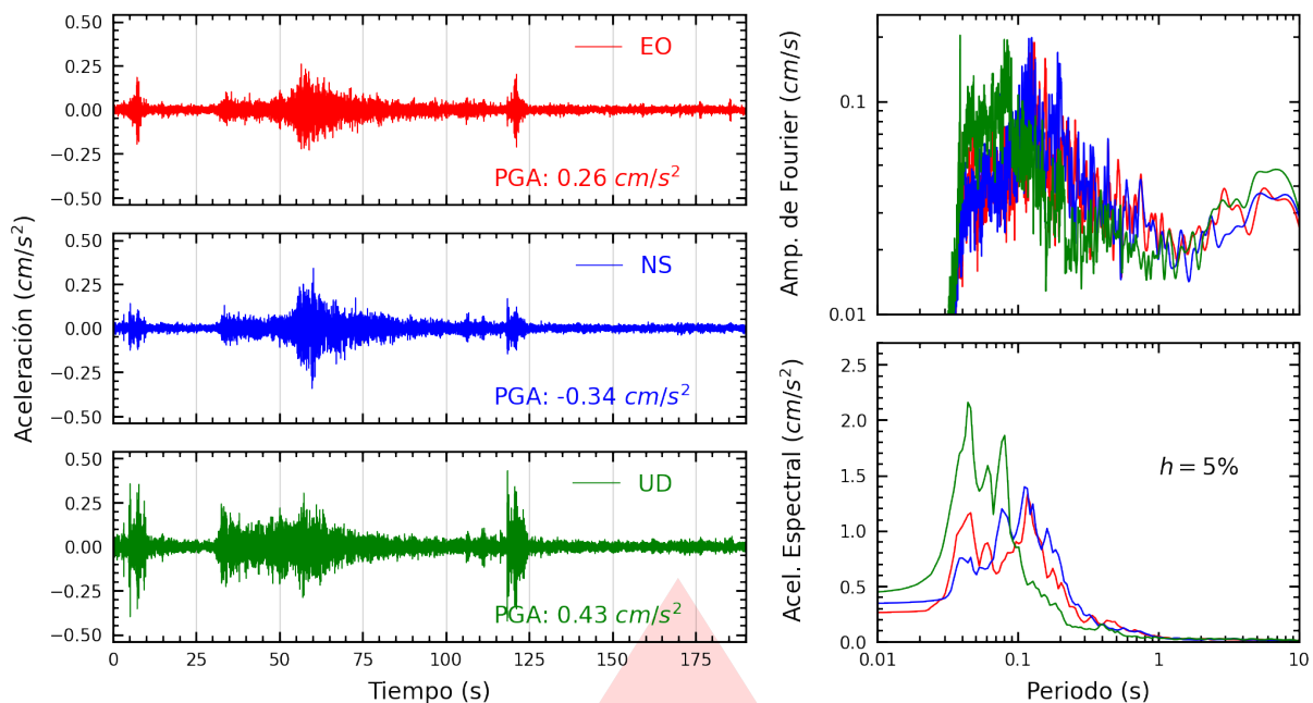
Figura A.15: Registros tiempo-historia, espectros de Fourier y de respuesta en las direcciones EO, NS y vertical de la estación SOCHO. Sismo de Pisco, Pisco - Ica del 2026-01-15, 22:46:47 (Hora local)
