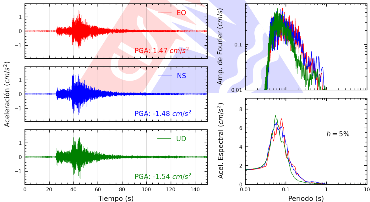
Figura A.2: Registros tiempo-historia, espectros de Fourier y de respuesta en las direcciones EO, NS y vertical de la estación ASIA. Sismo de Pisco, Pisco - Ica del 2026-01-15, 22:46:47 (Hora local)
