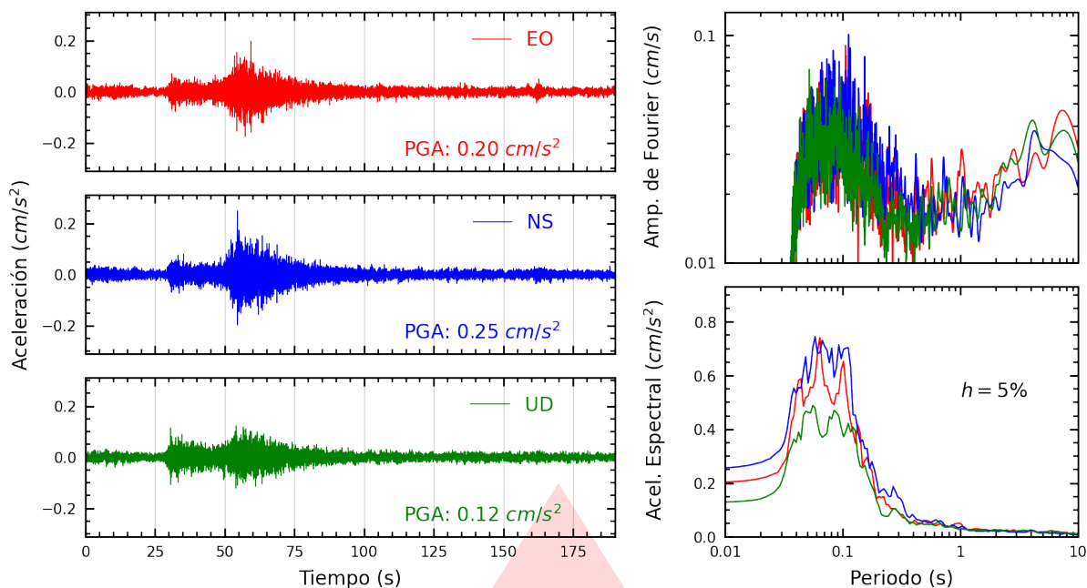
Figura A.23: Registros tiempo-historia, espectros de Fourier y de respuesta en las direcciones EO, NS y vertical de la estación SERVI. Sismo de Pisco, Pisco - Ica del 2026-01-15, 22:46:47 (Hora local)
