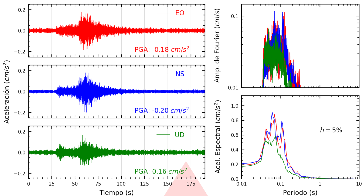
Figura A.27: Registros tiempo-historia, espectros de Fourier y de respuesta en las direcciones EO, NS y vertical de la estación ATARJ. Sismo de Pisco, Pisco - Ica del 2026-01-15, 22:46:47 (Hora local)
