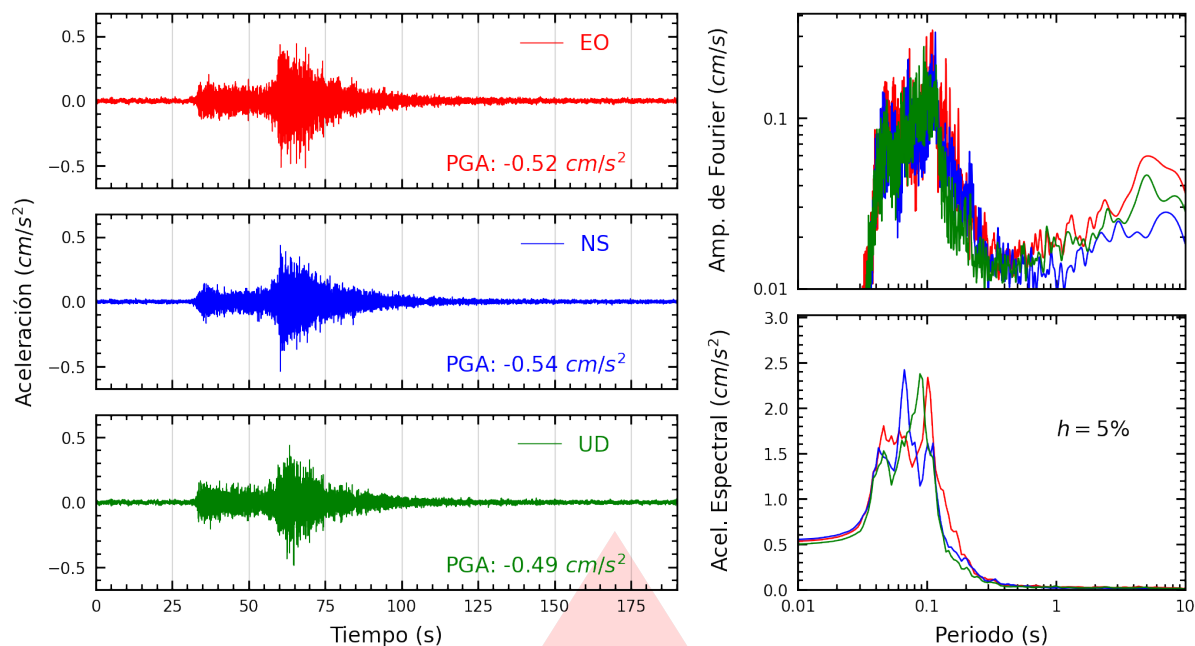
Figura A.9: Registros tiempo-historia, espectros de Fourier y de respuesta en las direcciones EO, NS y vertical de la estación AMORE. Sismo de Pisco, Pisco - Ica del 2026-01-15, 22:46:47 (Hora local)
