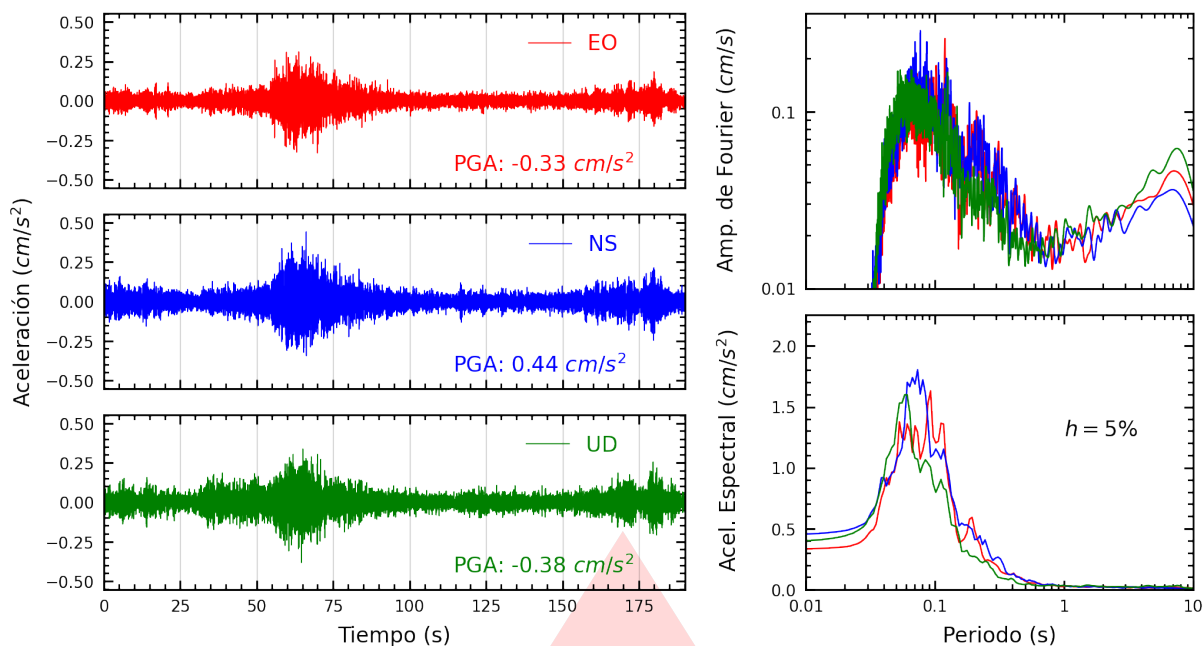
Figura A.13: Registros tiempo-historia, espectros de Fourier y de respuesta en las direcciones EO, NS y vertical de la estación SJLSC. Sismo de Pisco, Pisco - Ica del 2026-01-15, 22:46:47 (Hora local)
