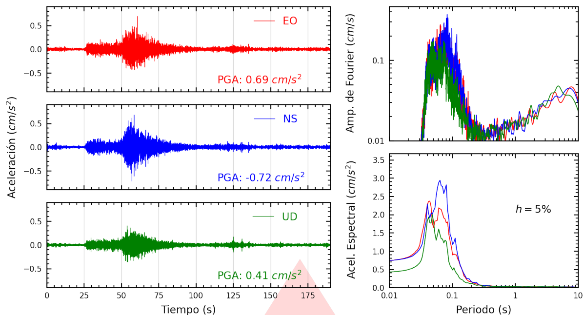
Figura A.7: Registros tiempo-historia, espectros de Fourier y de respuesta en las direcciones EO, NS y vertical de la estación JOSEO. Sismo de Pisco, Pisco - Ica del 2026-01-15, 22:46:47 (Hora local)
