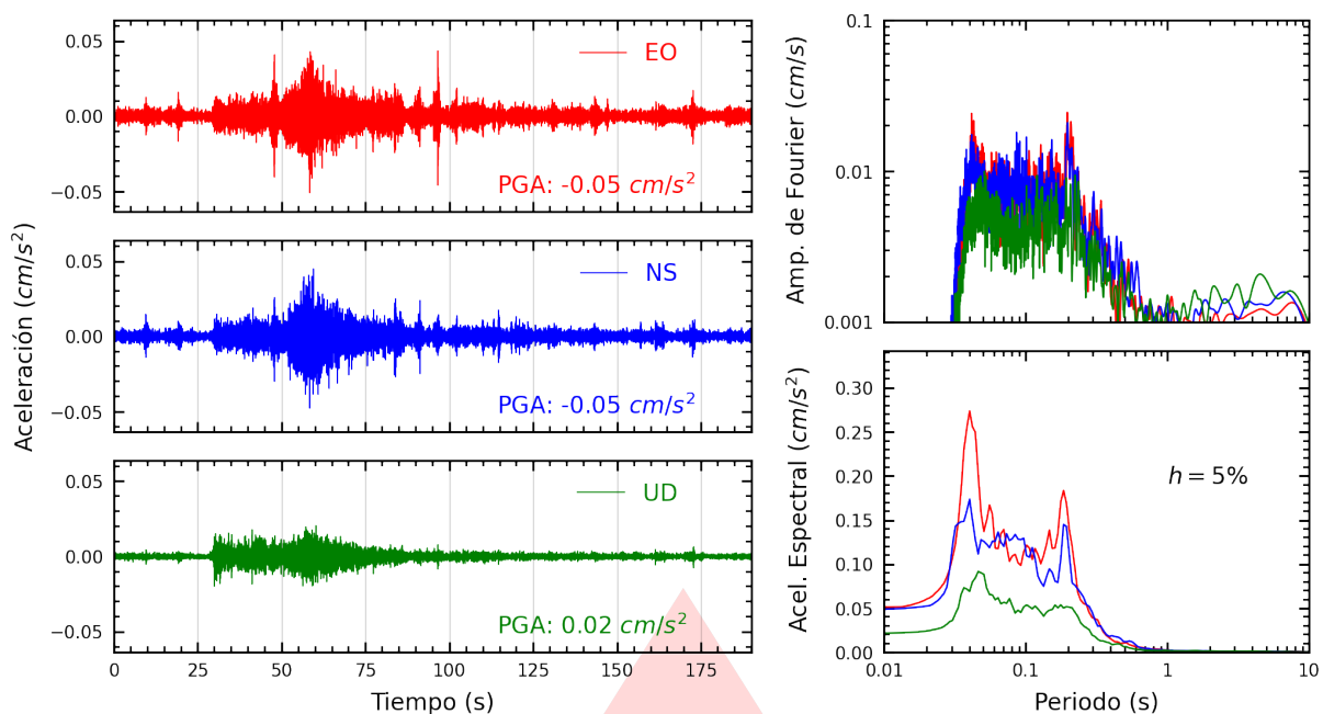
Figura A.1: Registros tiempo-historia, espectros de Fourier y de respuesta en las direcciones EO, NS y vertical de la estación UNSA2. Sismo de Chachas, Castilla - Arequipa del 2026-02-02, 08:04:26 (Hora local)
