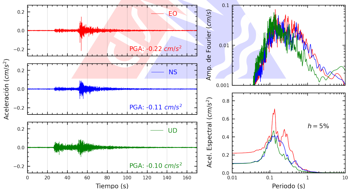
Figura A.2: Registros tiempo-historia, espectros de Fourier y de respuesta en las direcciones EO, NS y vertical de la estación UNIA. Sismo de Codo del Pozuzo, Puerto Inca - Huánuco del 2026-02-04, 19:20:04 (Hora local)
