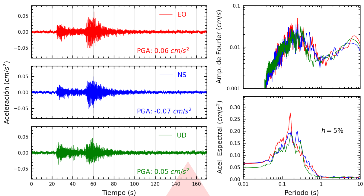
Figura A.3: Registros tiempo-historia, espectros de Fourier y de respuesta en las direcciones EO, NS y vertical de la estación CARAL. Sismo de Codo del Pozuzo, Puerto Inca - Huánuco del 2026-02-04, 19:20:04 (Hora local)
