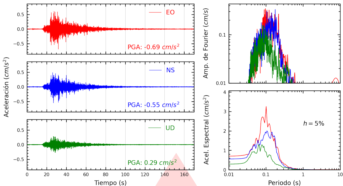
Figura A.1: Registros tiempo-historia, espectros de Fourier y de respuesta en las direcciones EO, NS y vertical de la estación UNAS. Sismo de Codo del Pozuzo, Puerto Inca - Huánuco del 2026-02-04, 19:20:04 (Hora local)
