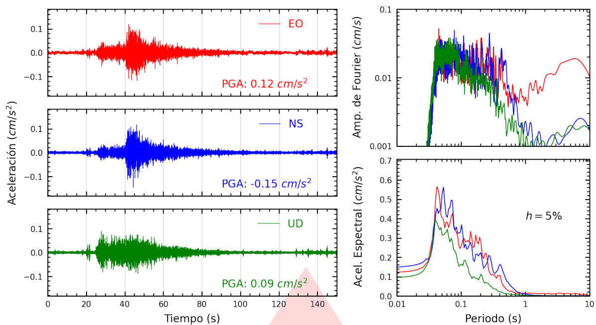
Figura A.3: Registros tiempo-historia, espectros de Fourier y de respuesta en las direcciones EO, NS y vertical de la estación SCCHI. Sismo de La Unión, Piura - Piura del 2026-02-05, 16:32:23 (Hora local)
