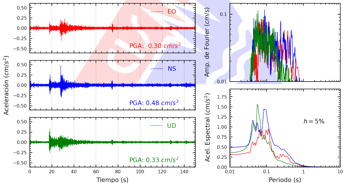
Figura A.2: Registros tiempo-historia, espectros de Fourier y de respuesta en las direcciones EO, NS y vertical de la estación UPAOP. Sismo de La Unión, Piura - Piura del 2026-02-05, 16:32:23 (Hora local)
