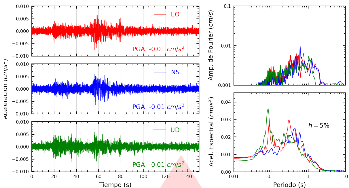
Figura A.1: Registros tiempo-historia, espectros de Fourier y de respuesta en las direcciones EO, NS y vertical de la estación UNCP. Sismo de Quillabamba, La Convención - Cusco del 2026-02-08, 23:02:29 (Hora local)
