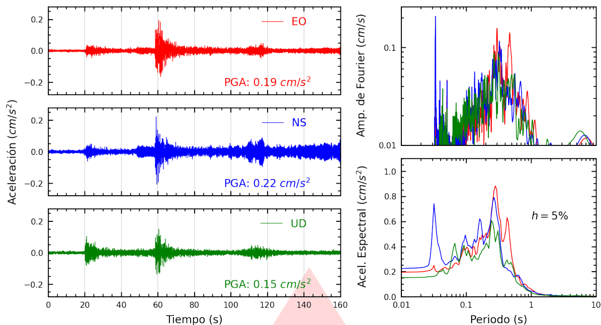
Figura A.1: Registros tiempo-historia, espectros de Fourier y de respuesta en las direcciones EO, NS y vertical de la estación UNJ. Sismo de Andoas, Datem del Marañón - Loreto del 2026-02-12, 16:52:54 (Hora local)
