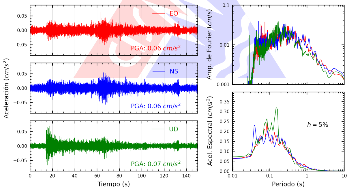
Figura A.2: Registros tiempo-historia, espectros de Fourier y de respuesta en las direcciones EO, NS y vertical de la estación UNF. Sismo de Andoas, Datem del Marañón - Loreto del 2026-02-12, 16:52:54 (Hora local)
