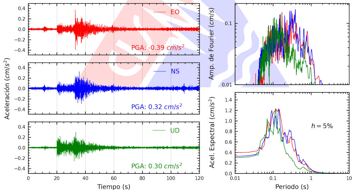
Figura A.2: Registros tiempo-historia, espectros de Fourier y de respuesta en las direcciones EO, NS y vertical de la estación UPAOP. Sismo de Talara, Talara - Piura del 2026-02-18, 08:27:52 (Hora local)
