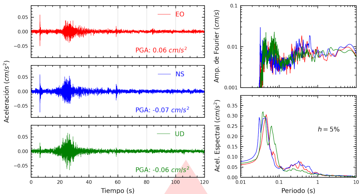
Figura A.3: Registros tiempo-historia, espectros de Fourier y de respuesta en las direcciones EO, NS y vertical de la estación UNJ. Sismo de Talara, Talara - Piura del 2026-02-18, 08:27:52 (Hora local)
