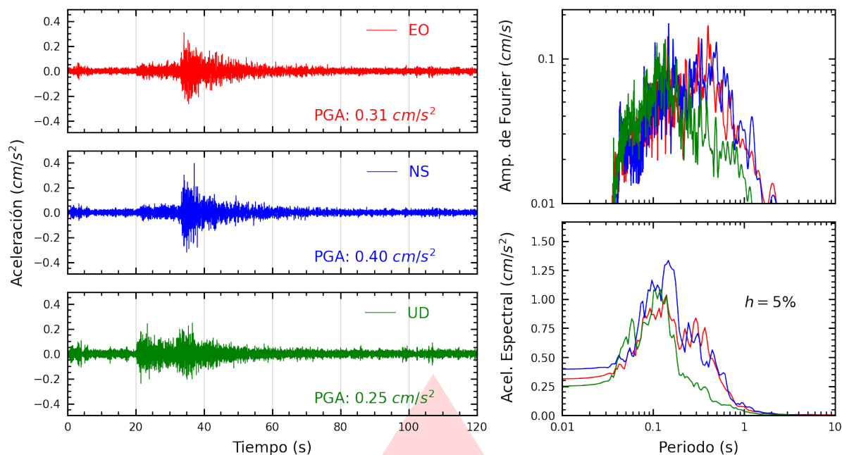
Figura A.1: Registros tiempo-historia, espectros de Fourier y de respuesta en las direcciones EO, NS y vertical de la estación SCPIU. Sismo de Talara, Talara - Piura del 2026-02-18, 08:27:52 (Hora local)
