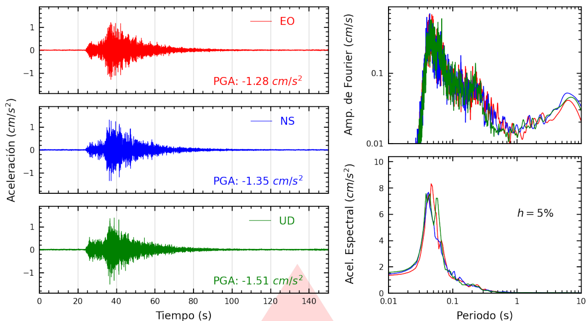
Figura A.35: Registros tiempo-historia, espectros de Fourier y de respuesta en las direcciones EO, NS y vertical de la estación USMP. Sismo de Mala, Cañete - Lima del 2026-02-19, 00:35:08 (Hora local)
