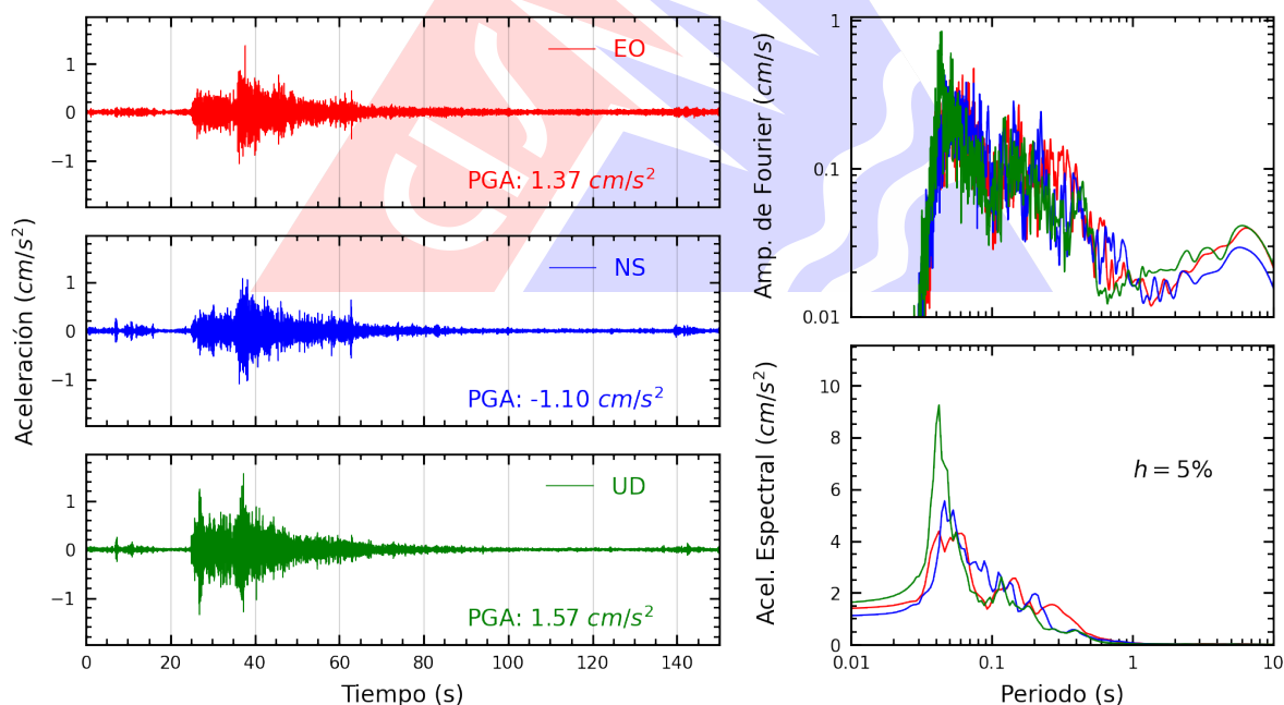
Figura A.30: Registros tiempo-historia, espectros de Fourier y de respuesta en las direcciones EO, NS y vertical de la estación UPCSM. Sismo de Mala, Cañete - Lima del 2026-02-19, 00:35:08 (Hora local)
