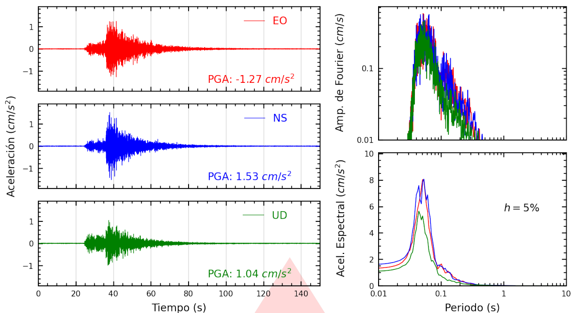
Figura A.33: Registros tiempo-historia, espectros de Fourier y de respuesta en las direcciones EO, NS y vertical de la estación ATARJ. Sismo de Mala, Cañete - Lima del 2026-02-19, 00:35:08 (Hora local)
