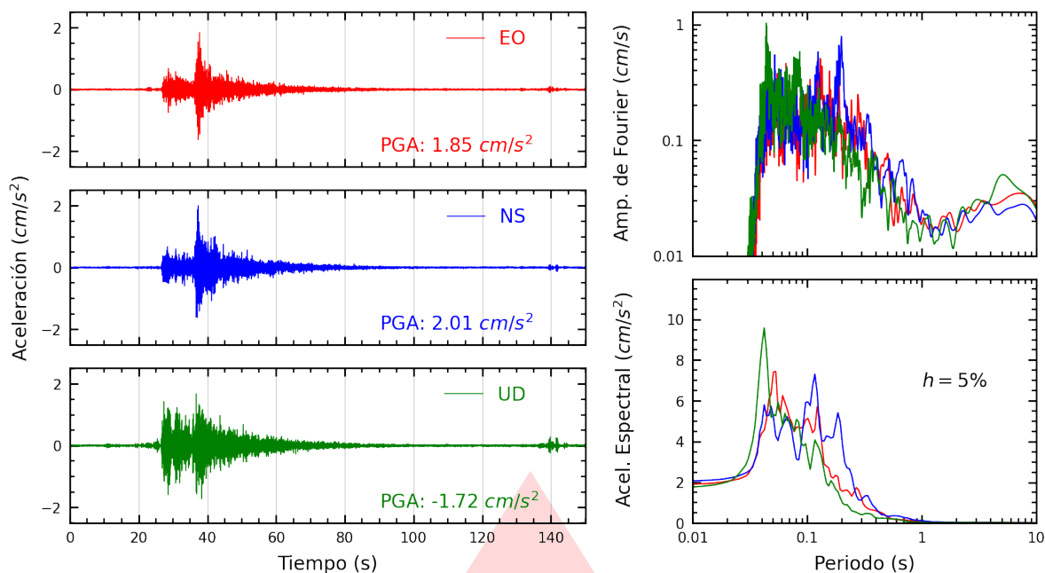
Figura A.25: Registros tiempo-historia, espectros de Fourier y de respuesta en las direcciones EO, NS y vertical de la estación SOCHO. Sismo de Mala, Cañete - Lima del 2026-02-19, 00:35:08 (Hora local)
