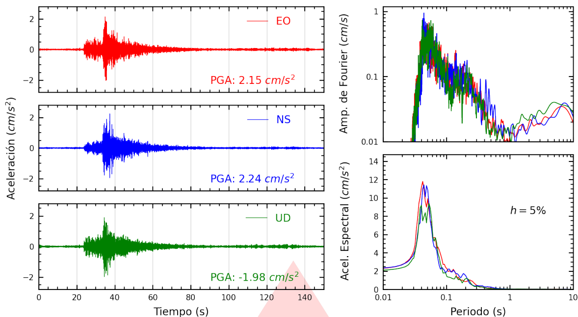
Figura A.21: Registros tiempo-historia, espectros de Fourier y de respuesta en las direcciones EO, NS y vertical de la estación URPPE. Sismo de Mala, Cañete - Lima del 2026-02-19, 00:35:08 (Hora local)
