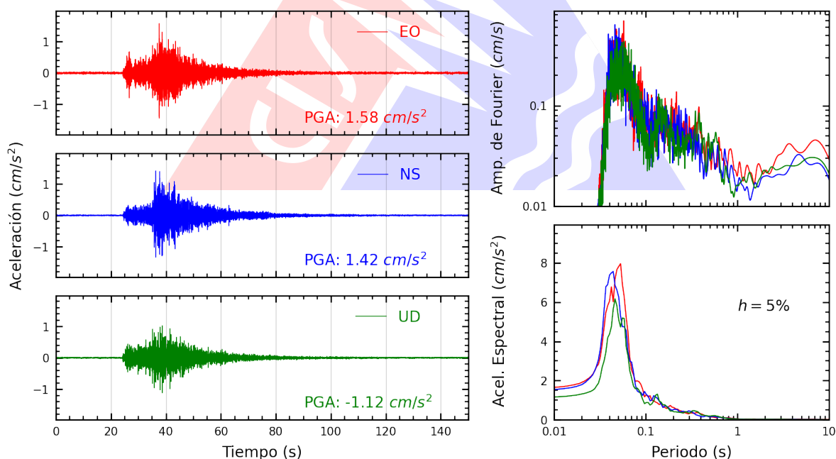
Figura A.28: Registros tiempo-historia, espectros de Fourier y de respuesta en las direcciones EO, NS y vertical de la estación IMCA. Sismo de Mala, Cañete - Lima del 2026-02-19, 00:35:08 (Hora local)
