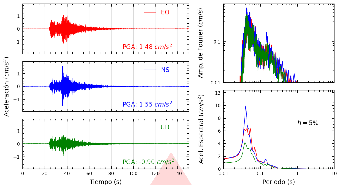
Figura A.31: Registros tiempo-historia, espectros de Fourier y de respuesta en las direcciones EO, NS y vertical de la estación BORJA. Sismo de Mala, Cañete - Lima del 2026-02-19, 00:35:08 (Hora local)
