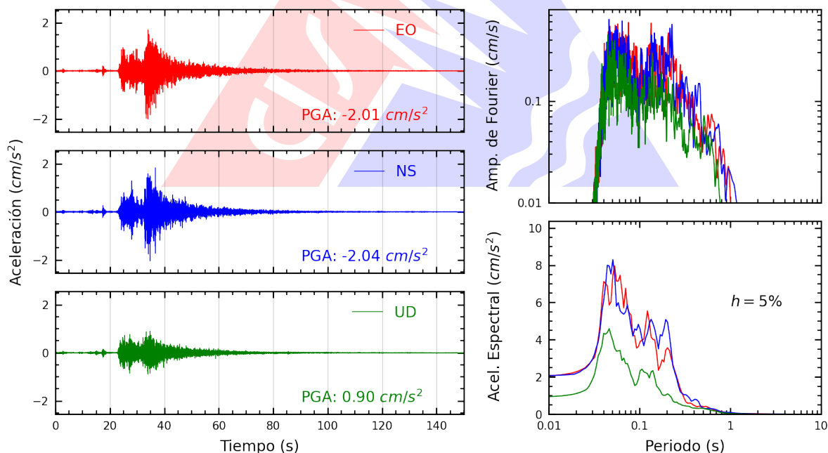
Figura A.24: Registros tiempo-historia, espectros de Fourier y de respuesta en las direcciones EO, NS y vertical de la estación BRIS2. Sismo de Mala, Cañete - Lima del 2026-02-19, 00:35:08 (Hora local)
