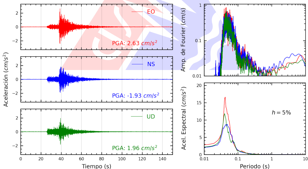
Figura A.18: Registros tiempo-historia, espectros de Fourier y de respuesta en las direcciones EO, NS y vertical de la estación SJLCE. Sismo de Mala, Cañete - Lima del 2026-02-19, 00:35:08 (Hora local)
