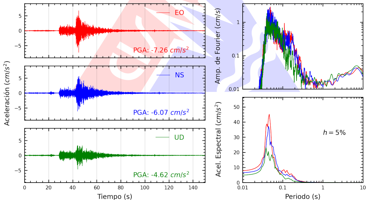
Figura A.4: Registros tiempo-historia, espectros de Fourier y de respuesta en las direcciones EO, NS y vertical de la estación SROSA. Sismo de Mala, Cañete - Lima del 2026-02-19, 00:35:08 (Hora local)
