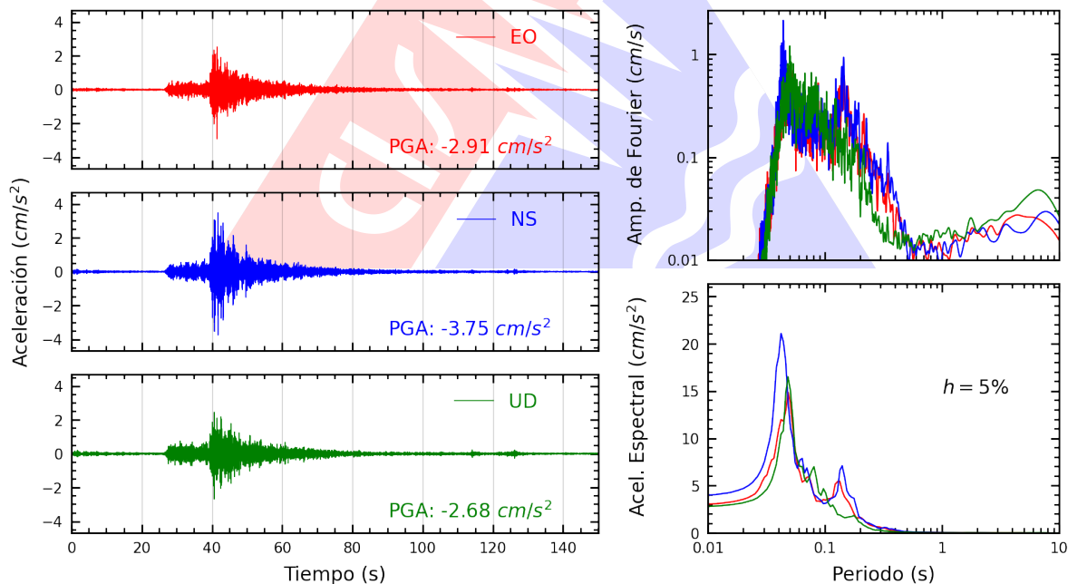
Figura A.10: Registros tiempo-historia, espectros de Fourier y de respuesta en las direcciones EO, NS y vertical de la estación CARAB. Sismo de Mala, Cañete - Lima del 2026-02-19, 00:35:08 (Hora local)
