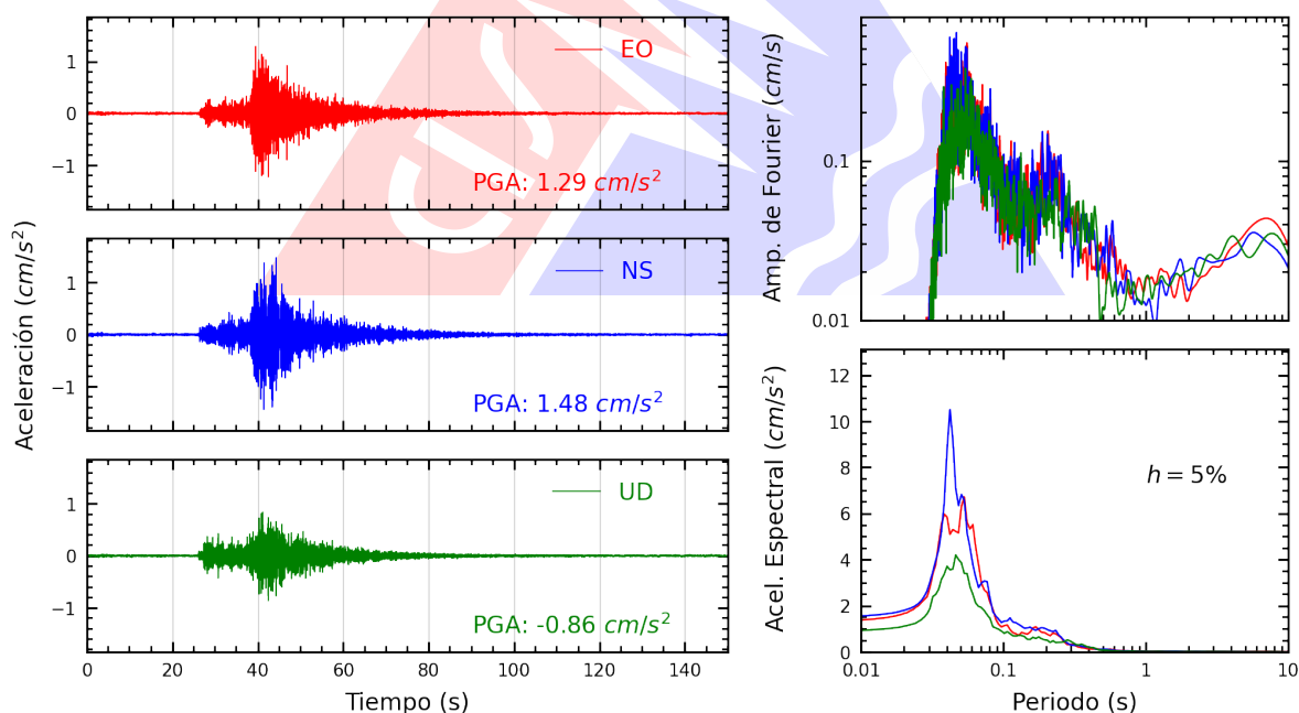
Figura A.38: Registros tiempo-historia, espectros de Fourier y de respuesta en las direcciones EO, NS y vertical de la estación COMAS. Sismo de Mala, Cañete - Lima del 2026-02-19, 00:35:08 (Hora local)
