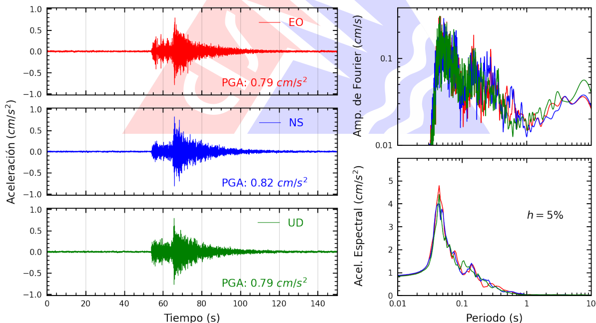
Figura A.42: Registros tiempo-historia, espectros de Fourier y de respuesta en las direcciones EO, NS y vertical de la estación UNMSM. Sismo de Mala, Cañete - Lima del 2026-02-19, 00:35:08 (Hora local)
