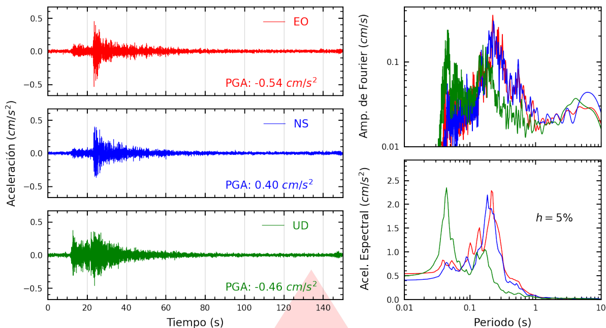
Figura A.45: Registros tiempo-historia, espectros de Fourier y de respuesta en las direcciones EO, NS y vertical de la estación DSML. Sismo de Mala, Cañete - Lima del 2026-02-19, 00:35:08 (Hora local)
