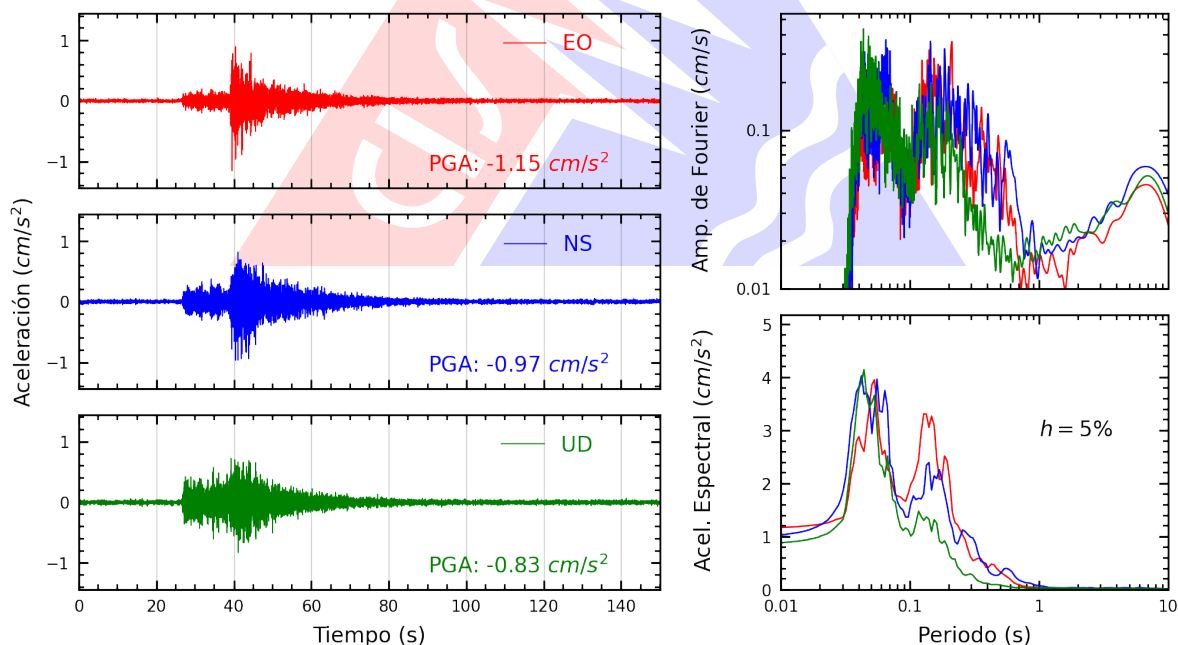
Figura A.40: Registros tiempo-historia, espectros de Fourier y de respuesta en las direcciones EO, NS y vertical de la estación VHAYA. Sismo de Mala, Cañete - Lima del 2026-02-19, 00:35:08 (Hora local)
