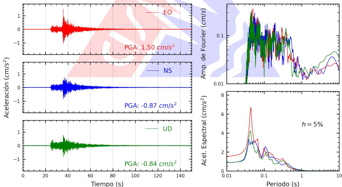
Figura A.36: Registros tiempo-historia, espectros de Fourier y de respuesta en las direcciones EO, NS y vertical de la estación UNFV. Sismo de Mala, Cañete - Lima del 2026-02-19, 00:35:08 (Hora local)
