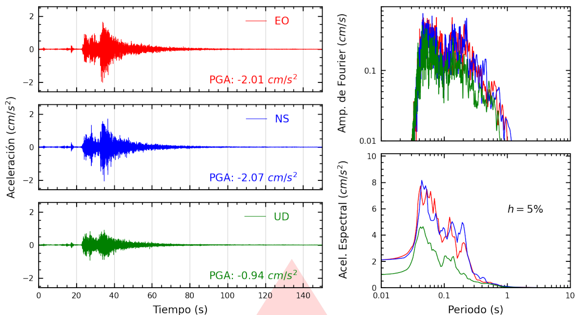
Figura A.23: Registros tiempo-historia, espectros de Fourier y de respuesta en las direcciones EO, NS y vertical de la estación BRISA. Sismo de Mala, Cañete - Lima del 2026-02-19, 00:35:08 (Hora local)
