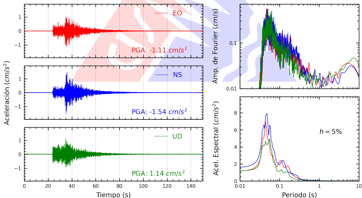
Figura A.32: Registros tiempo-historia, espectros de Fourier y de respuesta en las direcciones EO, NS y vertical de la estación SERVI. Sismo de Mala, Cañete - Lima del 2026-02-19, 00:35:08 (Hora local)
