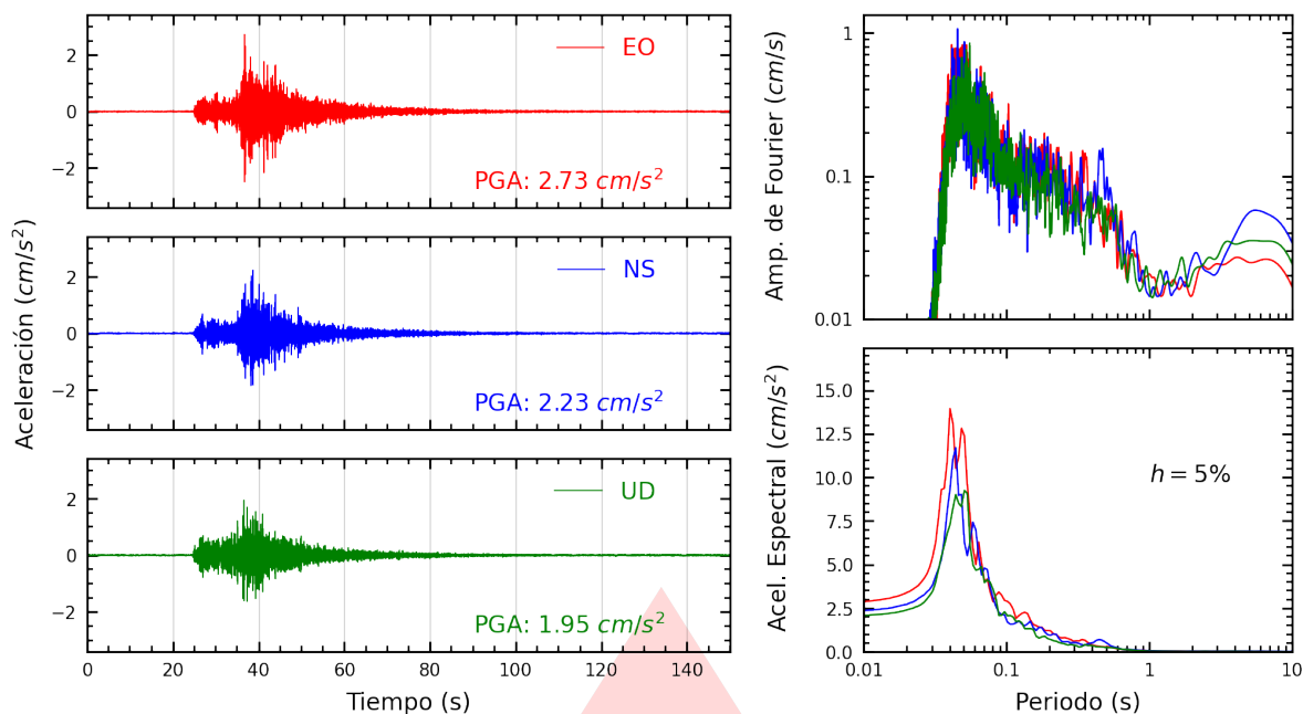
Figura A.15: Registros tiempo-historia, espectros de Fourier y de respuesta en las direcciones EO, NS y vertical de la estación UCVAT. Sismo de Mala, Cañete - Lima del 2026-02-19, 00:35:08 (Hora local)
