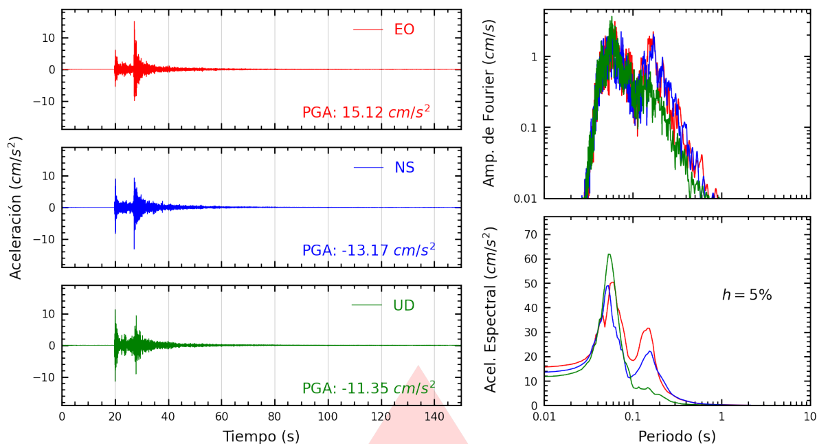
Figura A.1: Registros tiempo-historia, espectros de Fourier y de respuesta en las direcciones EO, NS y vertical de la estación ASIA. Sismo de Mala, Cañete - Lima del 2026-02-19, 00:35:08 (Hora local)
