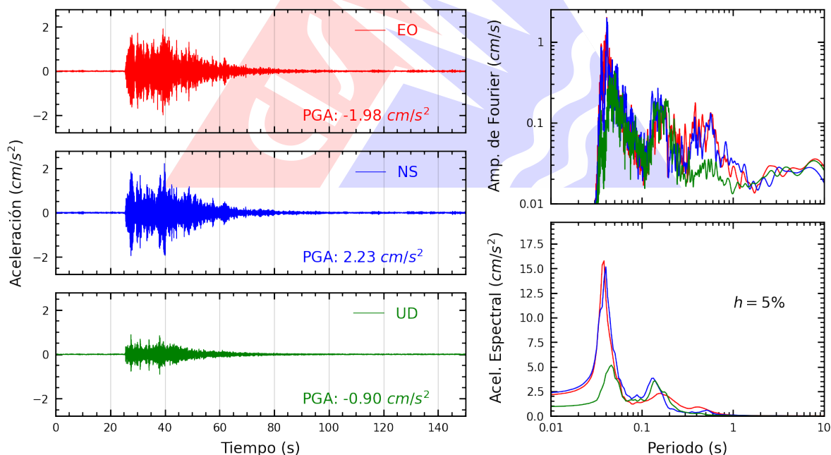
Figura A.22: Registros tiempo-historia, espectros de Fourier y de respuesta en las direcciones EO, NS y vertical de la estación DHNPE. Sismo de Mala, Cañete - Lima del 2026-02-19, 00:35:08 (Hora local)
