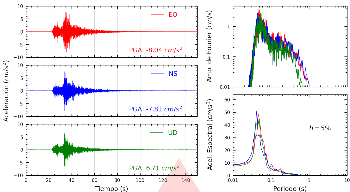
Figura A.3: Registros tiempo-historia, espectros de Fourier y de respuesta en las direcciones EO, NS y vertical de la estación UNTEL. Sismo de Mala, Cañete - Lima del 2026-02-19, 00:35:08 (Hora local)
