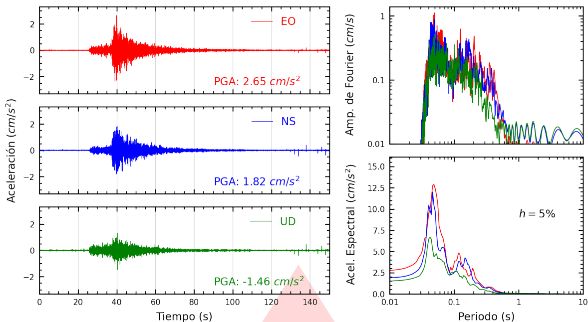
Figura A.17: Registros tiempo-historia, espectros de Fourier y de respuesta en las direcciones EO, NS y vertical de la estación SCOLI. Sismo de Mala, Cañete - Lima del 2026-02-19, 00:35:08 (Hora local)
