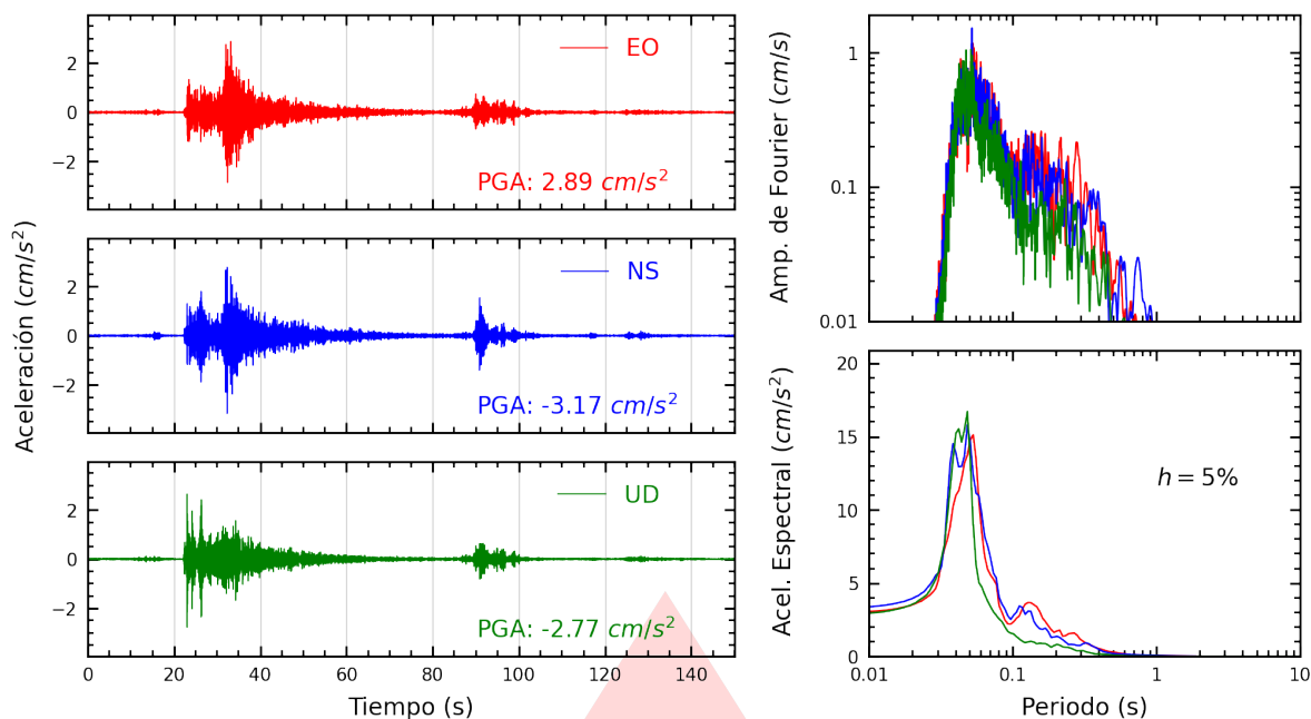
Figura A.13: Registros tiempo-historia, espectros de Fourier y de respuesta en las direcciones EO, NS y vertical de la estación PACHA. Sismo de Mala, Cañete - Lima del 2026-02-19, 00:35:08 (Hora local)
