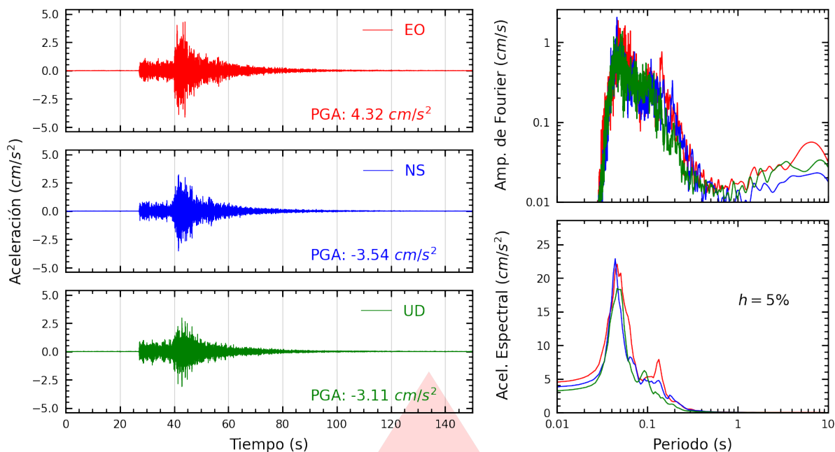
Figura A.7: Registros tiempo-historia, espectros de Fourier y de respuesta en las direcciones EO, NS y vertical de la estación AMORE. Sismo de Mala, Cañete - Lima del 2026-02-19, 00:35:08 (Hora local)
