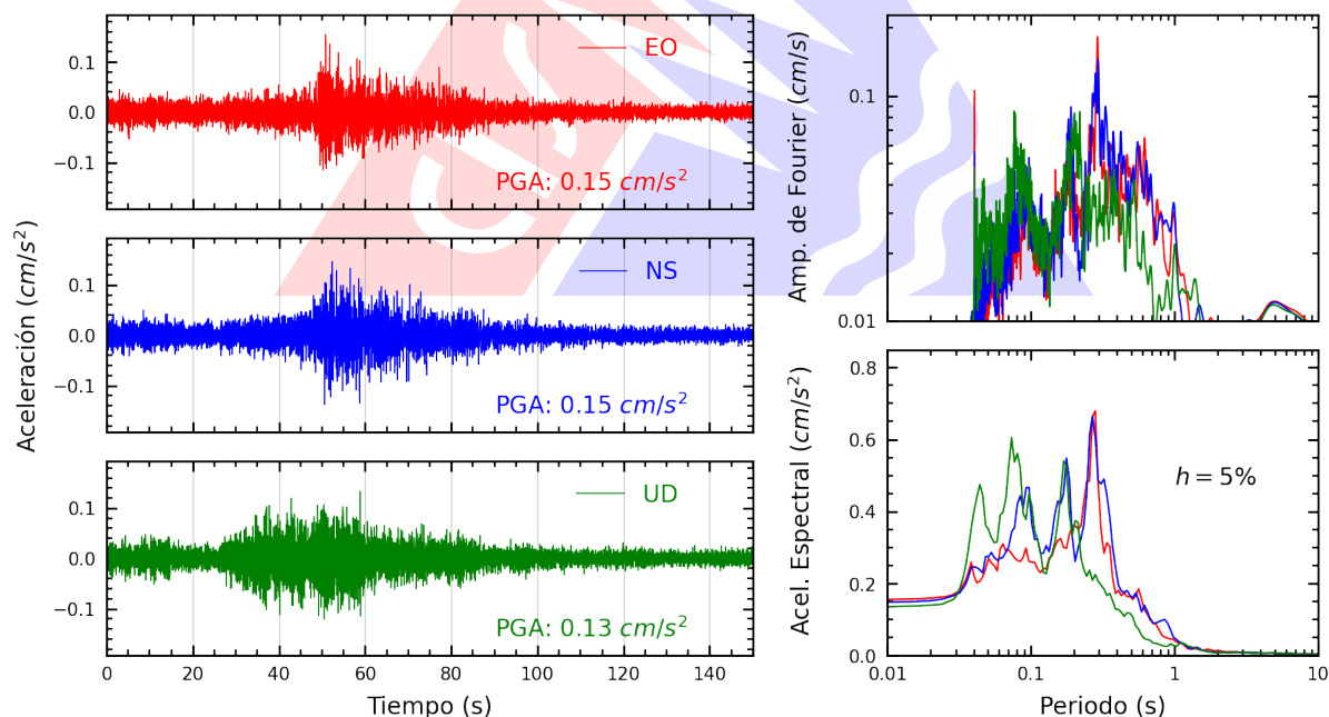
Figura A.48: Registros tiempo-historia, espectros de Fourier y de respuesta en las direcciones EO, NS y vertical de la estación UNICA. Sismo de Mala, Cañete - Lima del 2026-02-19, 00:35:08 (Hora local)
