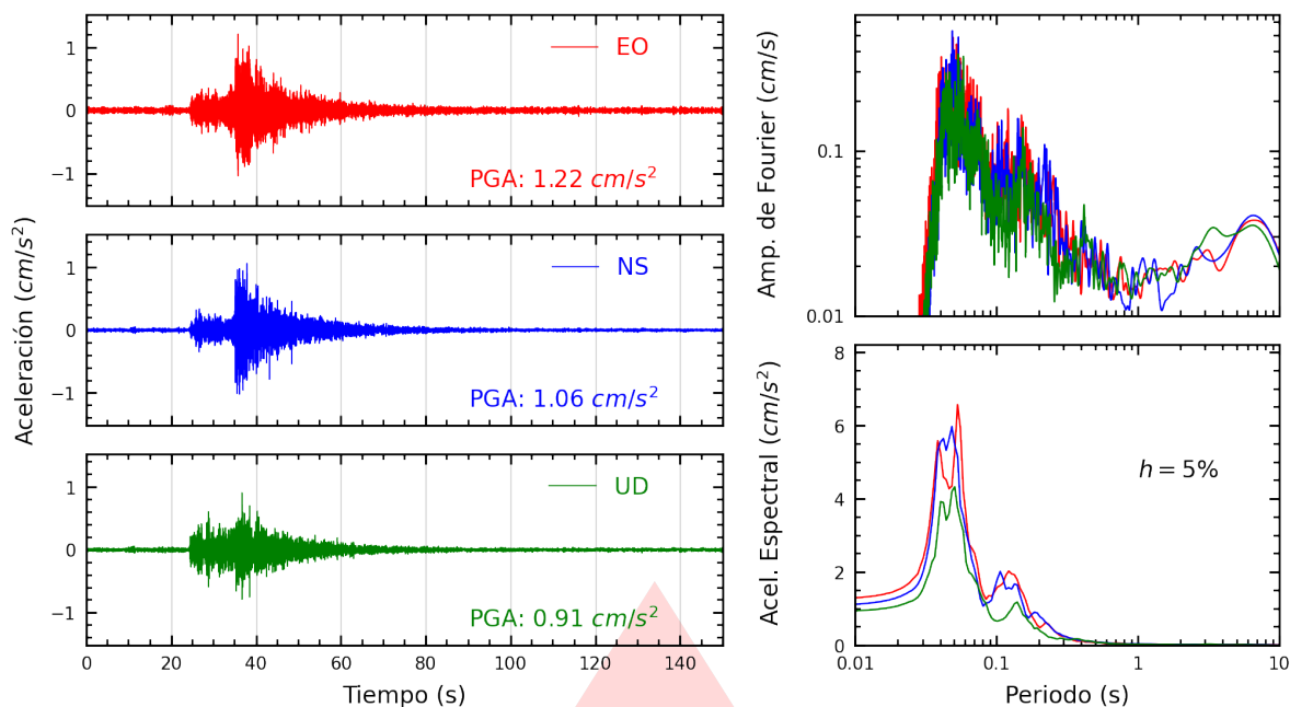
Figura A.39: Registros tiempo-historia, espectros de Fourier y de respuesta en las direcciones EO, NS y vertical de la estación INICT. Sismo de Mala, Cañete - Lima del 2026-02-19, 00:35:08 (Hora local)
