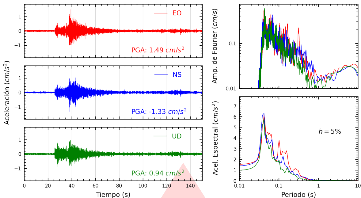
Figura A.37: Registros tiempo-historia, espectros de Fourier y de respuesta en las direcciones EO, NS y vertical de la estación MADRE. Sismo de Mala, Cañete - Lima del 2026-02-19, 00:35:08 (Hora local)
