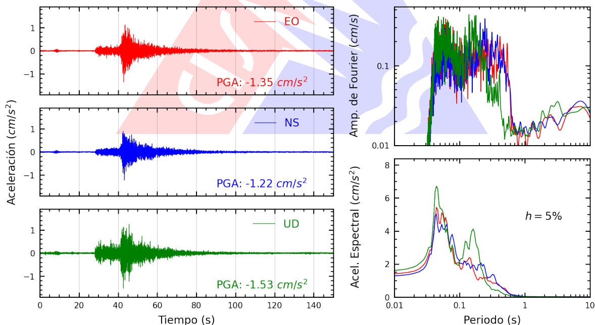
Figura A.34: Registros tiempo-historia, espectros de Fourier y de respuesta en las direcciones EO, NS y vertical de la estación MDPP. Sismo de Mala, Cañete - Lima del 2026-02-19, 00:35:08 (Hora local)
