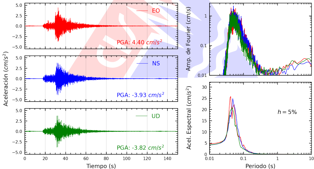
Figura A.6: Registros tiempo-historia, espectros de Fourier y de respuesta en las direcciones EO, NS y vertical de la estación JOSEO. Sismo de Mala, Cañete - Lima del 2026-02-19, 00:35:08 (Hora local)
