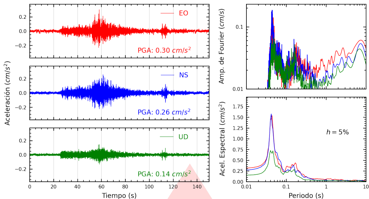
Figura A.47: Registros tiempo-historia, espectros de Fourier y de respuesta en las direcciones EO, NS y vertical de la estación UNAB. Sismo de Mala, Cañete - Lima del 2026-02-19, 00:35:08 (Hora local)
