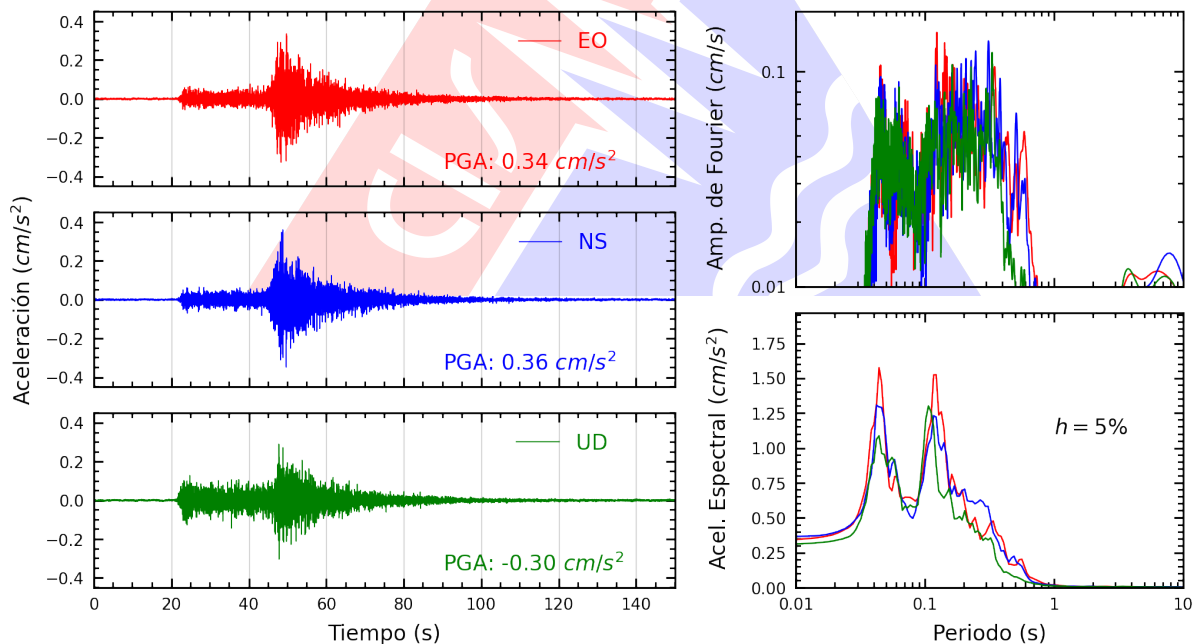
Figura A.46: Registros tiempo-historia, espectros de Fourier y de respuesta en las direcciones EO, NS y vertical de la estación CARAL. Sismo de Mala, Cañete - Lima del 2026-02-19, 00:35:08 (Hora local)
