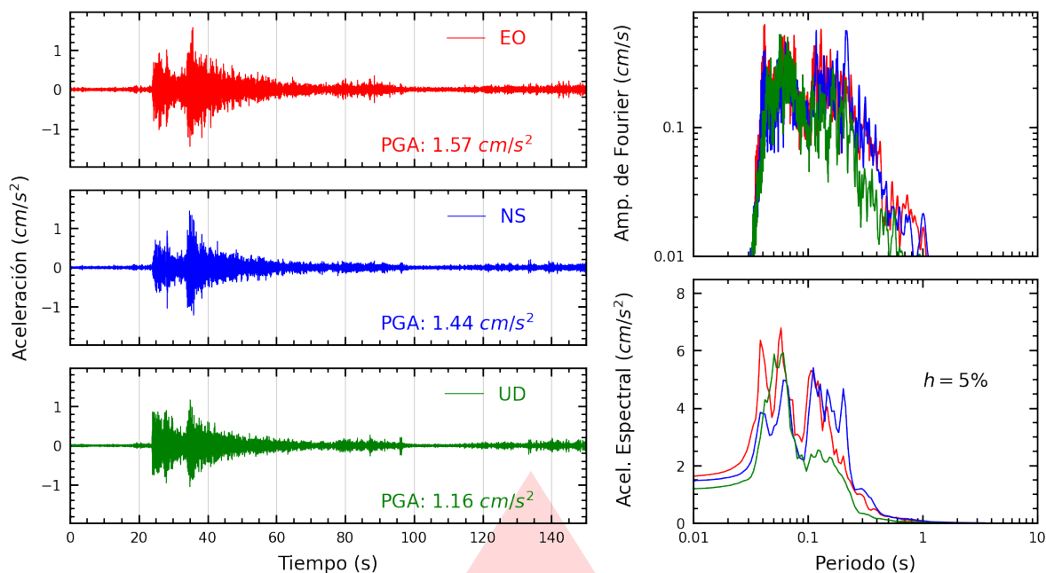
Figura A.29: Registros tiempo-historia, espectros de Fourier y de respuesta en las direcciones EO, NS y vertical de la estación SOBAR. Sismo de Mala, Cañete - Lima del 2026-02-19, 00:35:08 (Hora local)
