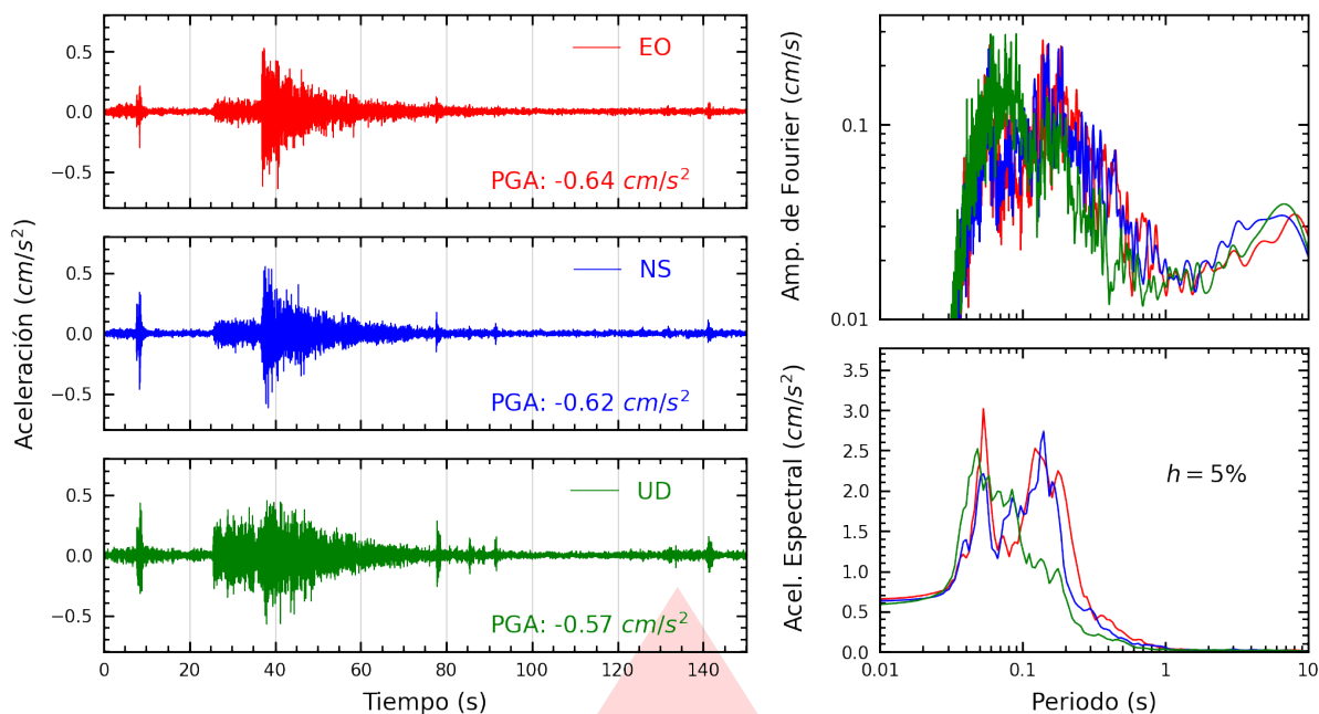
Figura A.43: Registros tiempo-historia, espectros de Fourier y de respuesta en las direcciones EO, NS y vertical de la estación RAMON. Sismo de Mala, Cañete - Lima del 2026-02-19, 00:35:08 (Hora local)
