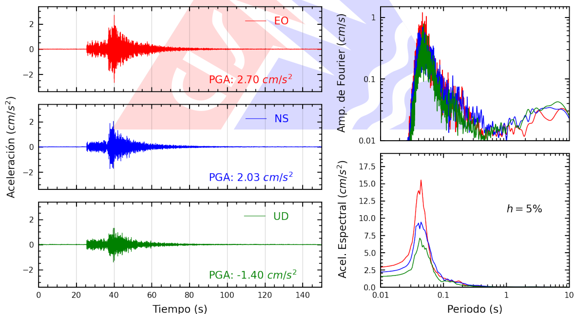
Figura A.16: Registros tiempo-historia, espectros de Fourier y de respuesta en las direcciones EO, NS y vertical de la estación UCSS. Sismo de Mala, Cañete - Lima del 2026-02-19, 00:35:08 (Hora local)
