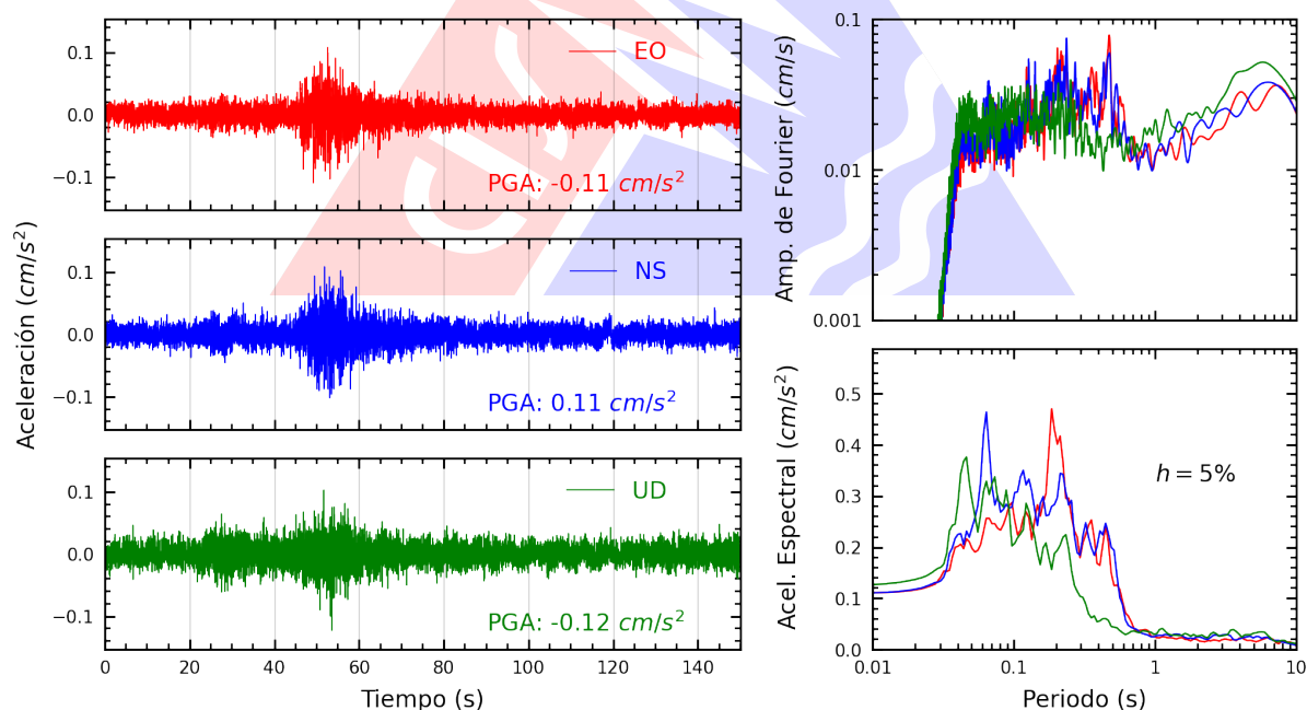
Figura A.14: Registros tiempo-historia, espectros de Fourier y de respuesta en las direcciones EO, NS y vertical de la estación VHAYA. Sismo de Huasichanca, Huancayo - Junín del 2026-02-20, 17:28:52 (Hora local)
