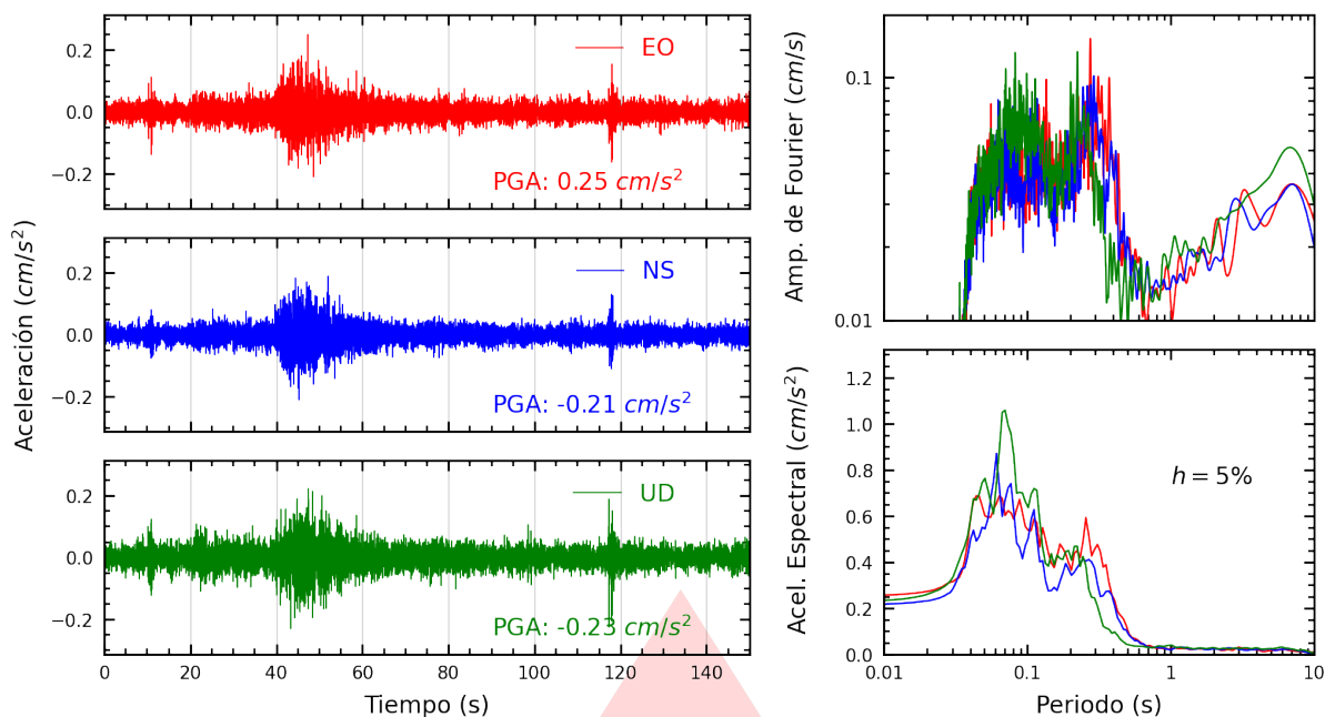
Figura A.7: Registros tiempo-historia, espectros de Fourier y de respuesta en las direcciones EO, NS y vertical de la estación SOVES. Sismo de Huasichanca, Huancayo - Junín del 2026-02-20, 17:28:52 (Hora local)
