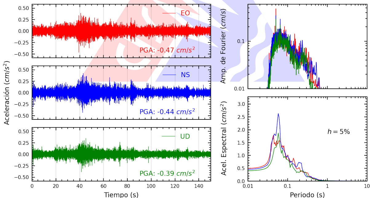
Figura A.2: Registros tiempo-historia, espectros de Fourier y de respuesta en las direcciones EO, NS y vertical de la estación PHERM. Sismo de Huasichanca, Huancayo - Junín del 2026-02-20, 17:28:52 (Hora local)
