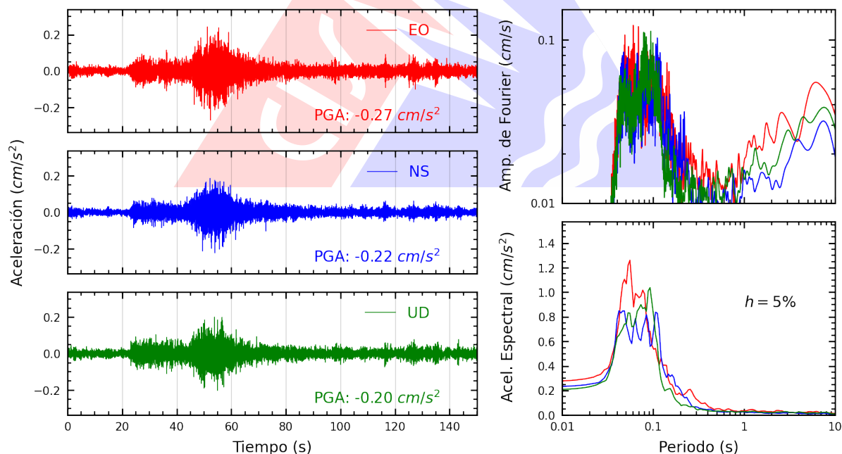
Figura A.6: Registros tiempo-historia, espectros de Fourier y de respuesta en las direcciones EO, NS y vertical de la estación AMORE. Sismo de Huasichanca, Huancayo - Junín del 2026-02-20, 17:28:52 (Hora local)
