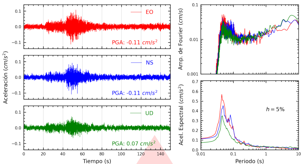
Figura A.17: Registros tiempo-historia, espectros de Fourier y de respuesta en las direcciones EO, NS y vertical de la estación UCSS. Sismo de Huasichanca, Huancayo - Junín del 2026-02-20, 17:28:52 (Hora local)
