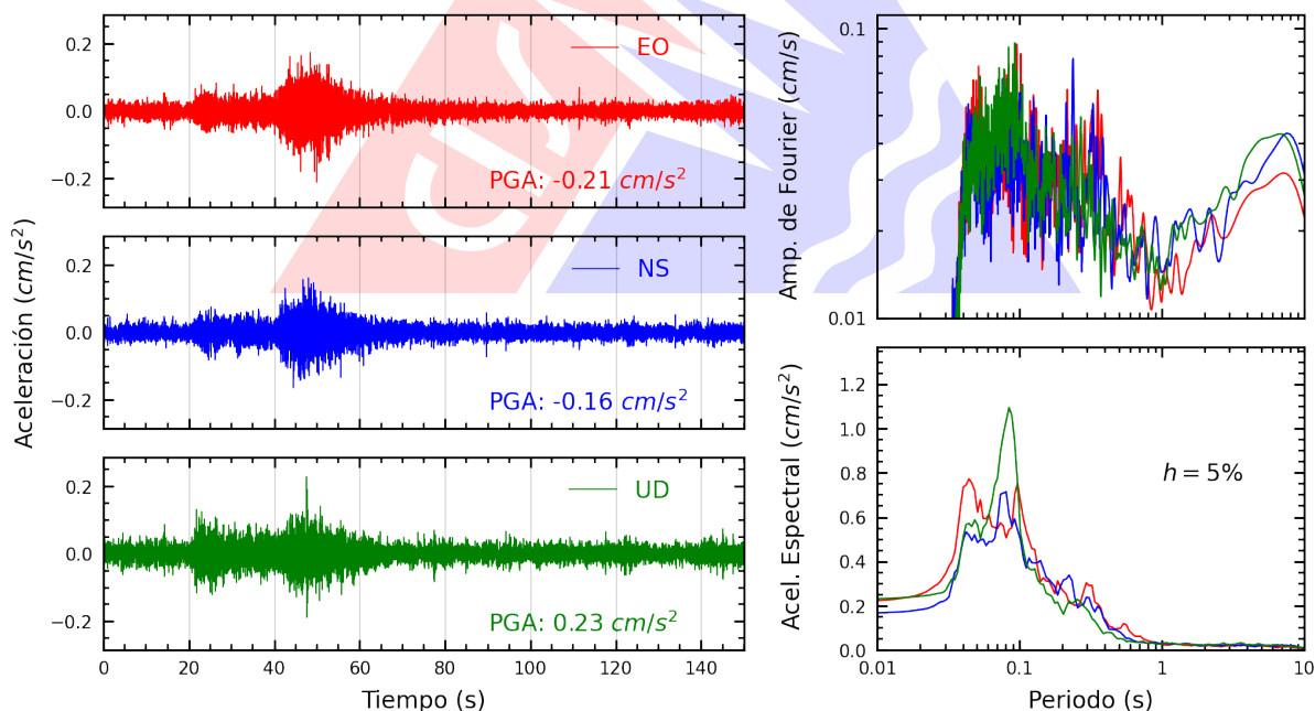
Figura A.8: Registros tiempo-historia, espectros de Fourier y de respuesta en las direcciones EO, NS y vertical de la estación UCVAT. Sismo de Huasichanca, Huancayo - Junín del 2026-02-20, 17:28:52 (Hora local)
