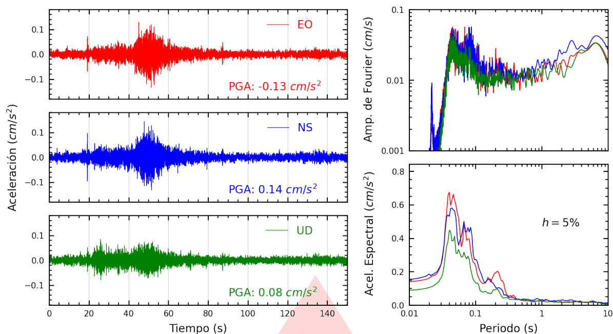
Figura A.13: Registros tiempo-historia, espectros de Fourier y de respuesta en las direcciones EO, NS y vertical de la estación SJLCE. Sismo de Huasichanca, Huancayo - Junín del 2026-02-20, 17:28:52 (Hora local)
