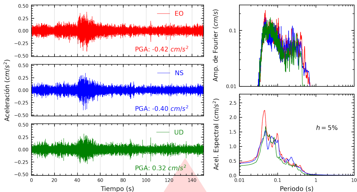
Figura A.3: Registros tiempo-historia, espectros de Fourier y de respuesta en las direcciones EO, NS y vertical de la estación UNTEL. Sismo de Huasichanca, Huancayo - Junín del 2026-02-20, 17:28:52 (Hora local)
