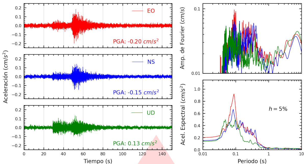
Figura A.9: Registros tiempo-historia, espectros de Fourier y de respuesta en las direcciones EO, NS y vertical de la estación USILP. Sismo de Huasicancha, Huancayo - Junín del 2026-02-20, 17:28:52 (Hora local)
