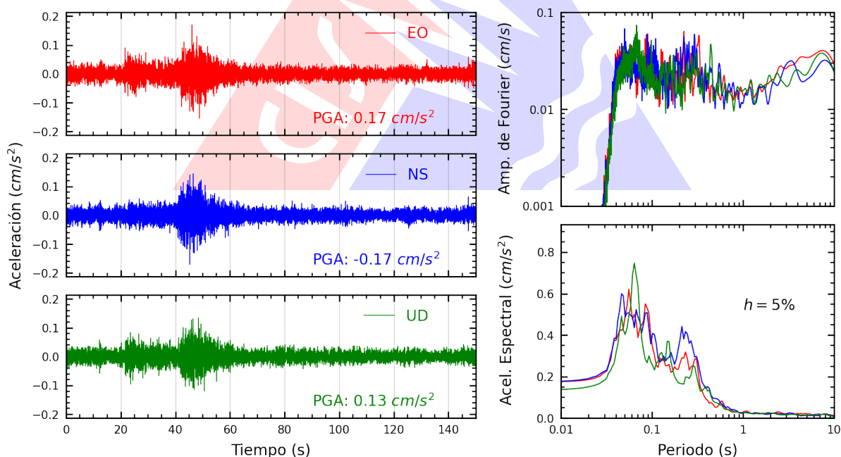
Figura A.10: Registros tiempo-historia, espectros de Fourier y de respuesta en las direcciones EO, NS y vertical de la estación IMCA. Sismo de Huasicancha, Huancayo - Junín del 2026-02-20, 17:28:52 (Hora local)
