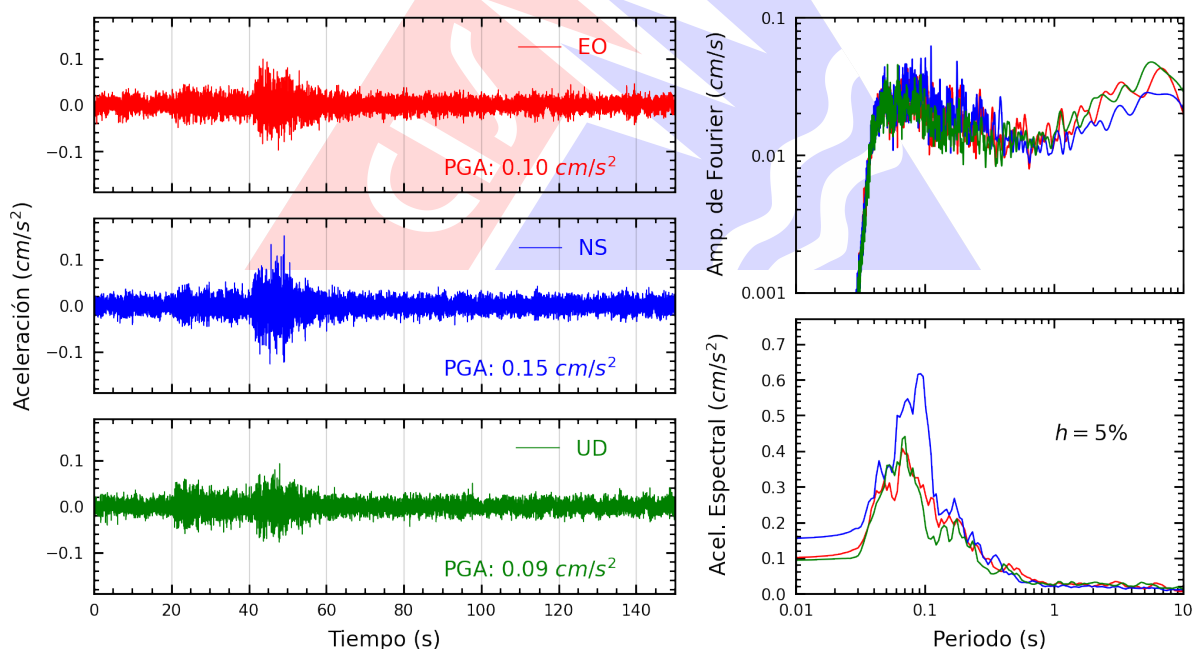
Figura A.12: Registros tiempo-historia, espectros de Fourier y de respuesta en las direcciones EO, NS y vertical de la estación SERVI. Sismo de Huasichanca, Huancayo - Junín del 2026-02-20, 17:28:52 (Hora local)
