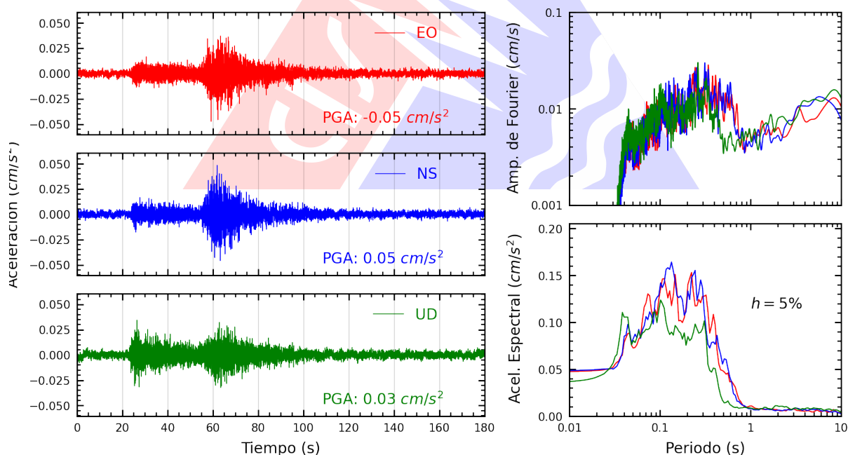
Figura A.18: Registros tiempo-historia, espectros de Fourier y de respuesta en las direcciones EO, NS y vertical de la estación CARAL. Sismo de Huasichanca, Huancayo - Junín del 2026-02-20, 17:28:52 (Hora local)
