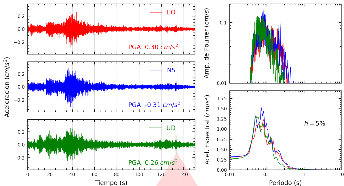
Figura A.5: Registros tiempo-historia, espectros de Fourier y de respuesta en las direcciones EO, NS y vertical de la estación ASIA. Sismo de Huasichanca, Huancayo - Junín del 2026-02-20, 17:28:52 (Hora local)
