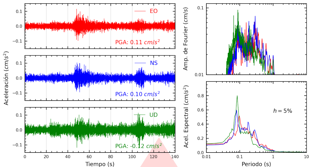
Figura A.15: Registros tiempo-historia, espectros de Fourier y de respuesta en las direcciones EO, NS y vertical de la estación UNICA. Sismo de Huasichanca, Huancayo - Junín del 2026-02-20, 17:28:52 (Hora local)
