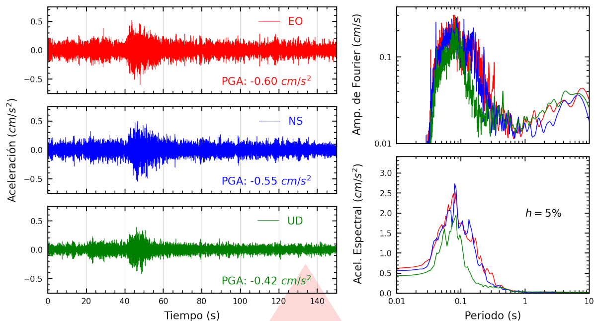
Figura A.1: Registros tiempo-historia, espectros de Fourier y de respuesta en las direcciones EO, NS y vertical de la estación USILM. Sismo de Huasichanca, Huancayo - Junín del 2026-02-20, 17:28:52 (Hora local)
