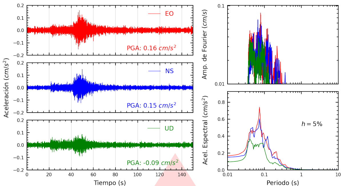
Figura A.11: Registros tiempo-historia, espectros de Fourier y de respuesta en las direcciones EO, NS y vertical de la estación ATARJ. Sismo de Huasichanca, Huancayo - Junín del 2026-02-20, 17:28:52 (Hora local)
