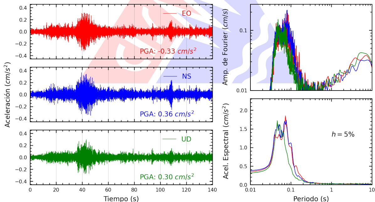
Figura A.4: Registros tiempo-historia, espectros de Fourier y de respuesta en las direcciones EO, NS y vertical de la estación JOSEO. Sismo de Huasichanca, Huancayo - Junín del 2026-02-20, 17:28:52 (Hora local)
