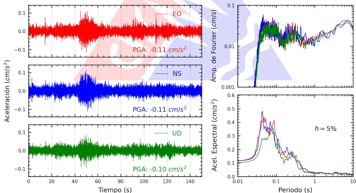
Figura A.16: Registros tiempo-historia, espectros de Fourier y de respuesta en las direcciones EO, NS y vertical de la estación COMAS. Sismo de Huasichanca, Huancayo - Junín del 2026-02-20, 17:28:52 (Hora local)
