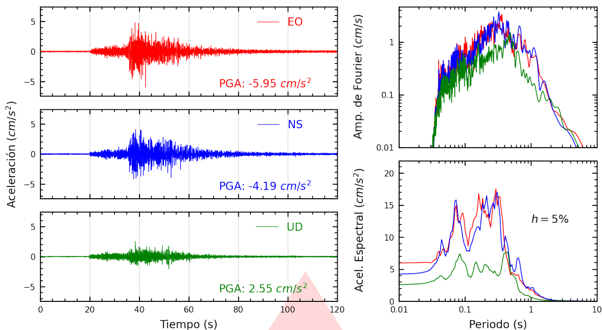
Figura A.17: Registros tiempo-historia, espectros de Fourier y de respuesta en las direcciones EO, NS y vertical de la estación BRIS2. Sismo de Pisco, Pisco - Ica del 2026-02-22, 17:36:14 (Hora local)
