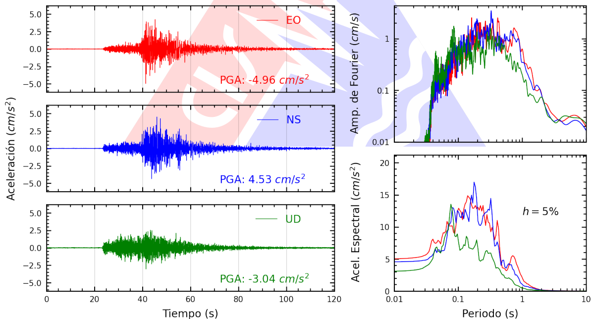
Figura A.20: Registros tiempo-historia, espectros de Fourier y de respuesta en las direcciones EO, NS y vertical de la estación SOCHO. Sismo de Pisco, Pisco - Ica del 2026-02-22, 17:36:14 (Hora local)
