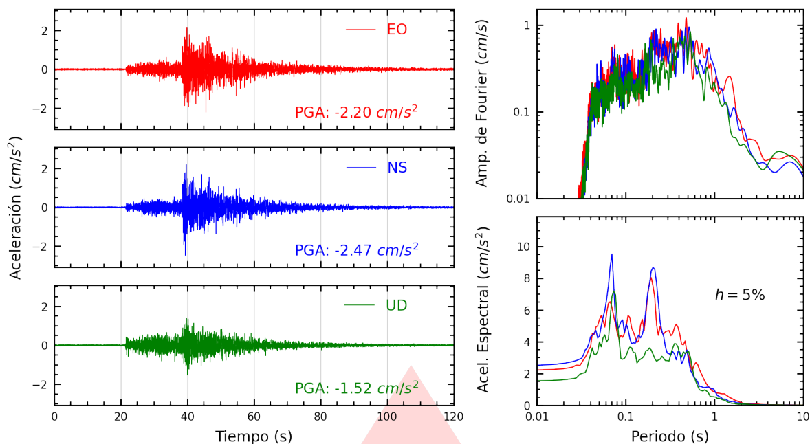
Figura A.39: Registros tiempo-historia, espectros de Fourier y de respuesta en las direcciones EO, NS y vertical de la estación INICT. Sismo de Pisco, Pisco - Ica del 2026-02-22, 17:36:14 (Hora local)
