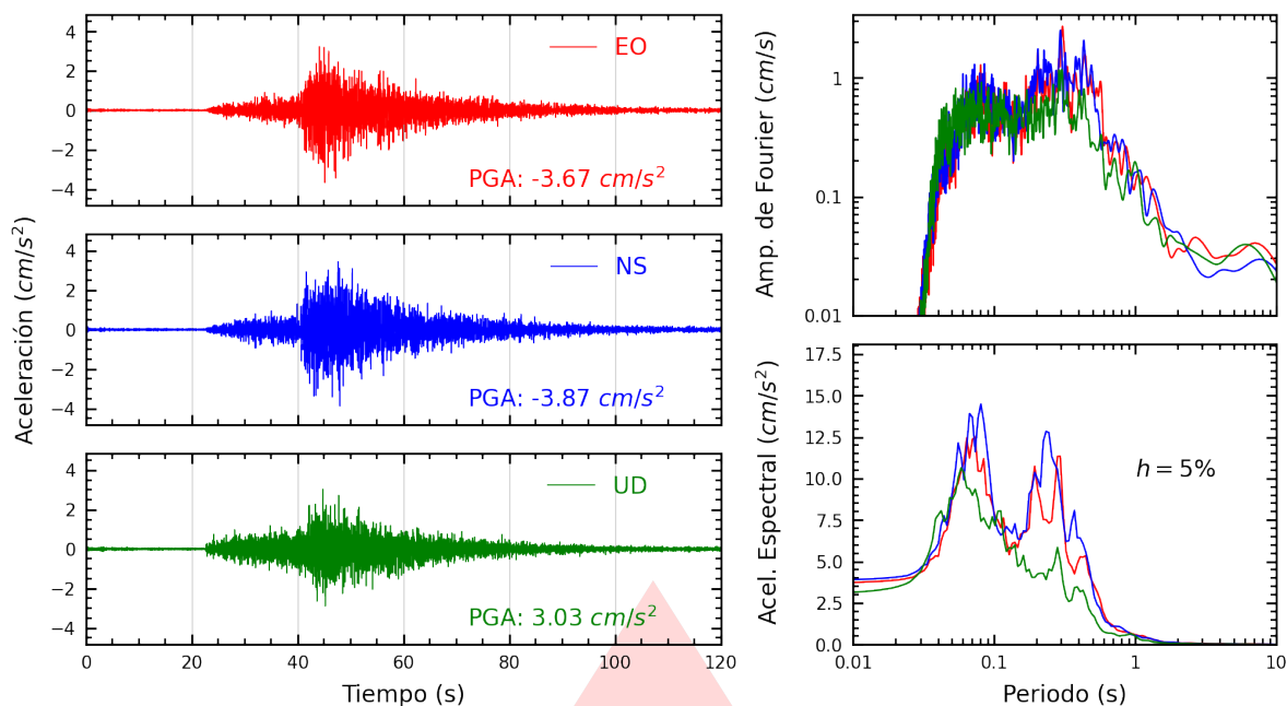
Figura A.27: Registros tiempo-historia, espectros de Fourier y de respuesta en las direcciones EO, NS y vertical de la estación SJLSC. Sismo de Pisco, Pisco - Ica del 2026-02-22, 17:36:14 (Hora local)
