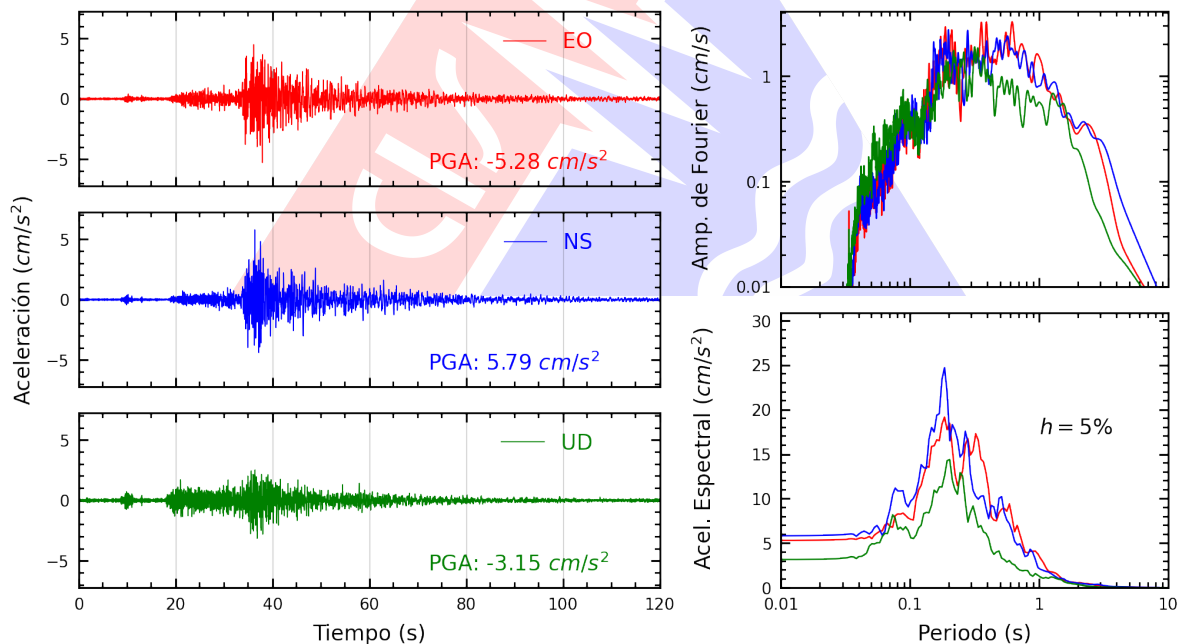
Figura A.18: Registros tiempo-historia, espectros de Fourier y de respuesta en las direcciones EO, NS y vertical de la estación SCICA. Sismo de Pisco, Pisco - Ica del 2026-02-22, 17:36:14 (Hora local)
