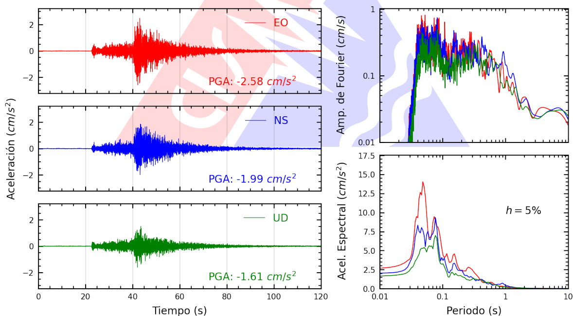
Figura A.38: Registros tiempo-historia, espectros de Fourier y de respuesta en las direcciones EO, NS y vertical de la estación UCSS. Sismo de Pisco, Pisco - Ica del 2026-02-22, 17:36:14 (Hora local)
