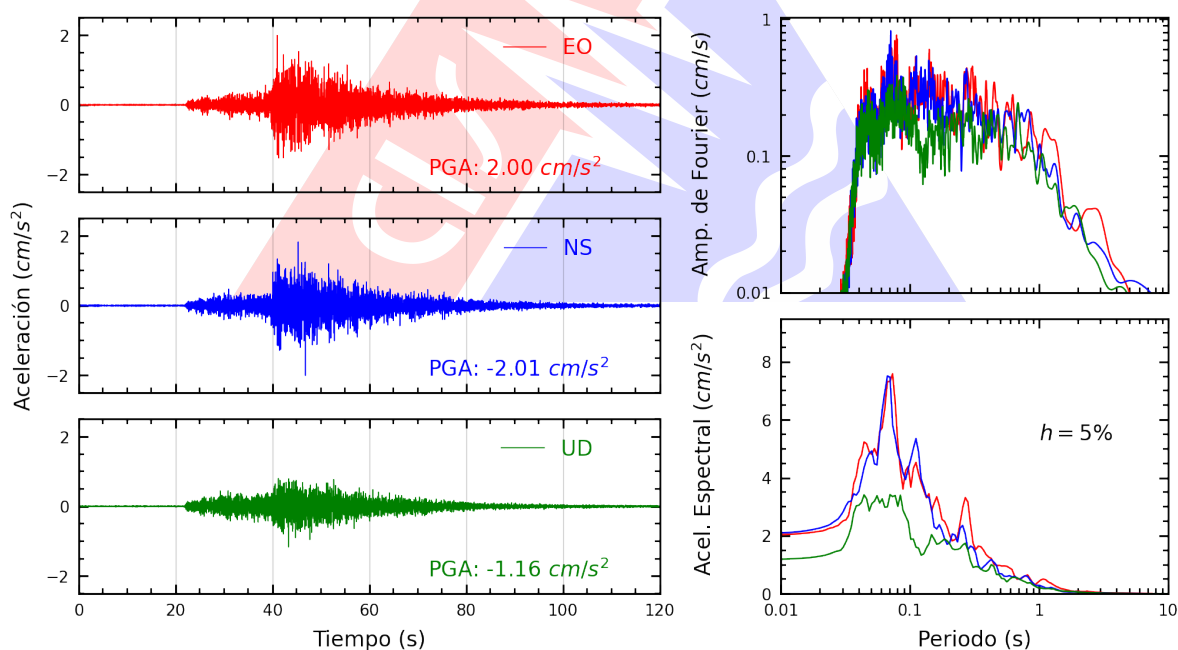
Figura A.42: Registros tiempo-historia, espectros de Fourier y de respuesta en las direcciones EO, NS y vertical de la estación ATARJ. Sismo de Pisco, Pisco - Ica del 2026-02-22, 17:36:14 (Hora local)
