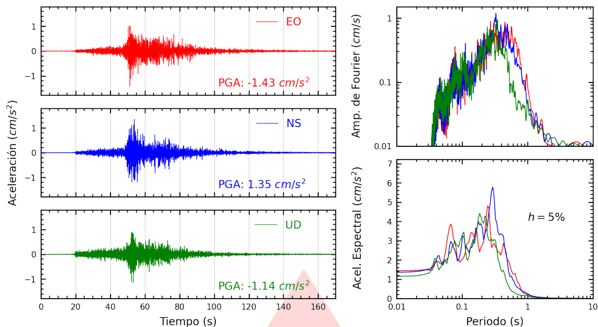
Figura A.45: Registros tiempo-historia, espectros de Fourier y de respuesta en las direcciones EO, NS y vertical de la estación CARAL. Sismo de Pisco, Pisco - Ica del 2026-02-22, 17:36:14 (Hora local)
