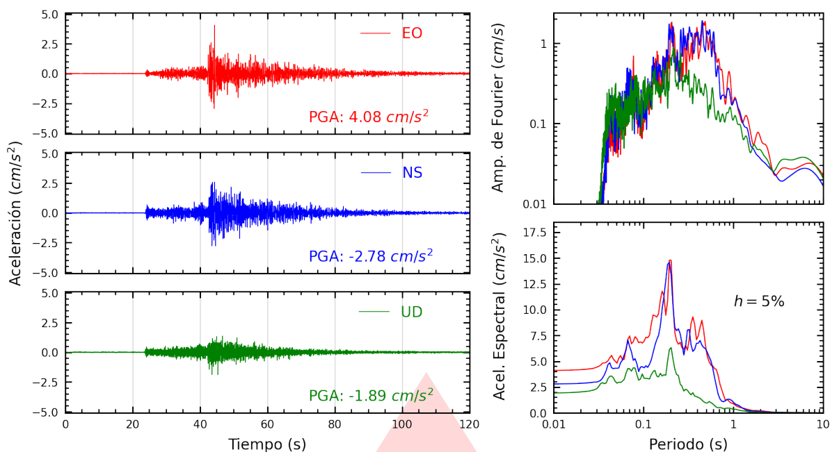
Figura A.25: Registros tiempo-historia, espectros de Fourier y de respuesta en las direcciones EO, NS y vertical de la estación VHAYA. Sismo de Pisco, Pisco - Ica del 2026-02-22, 17:36:14 (Hora local)
