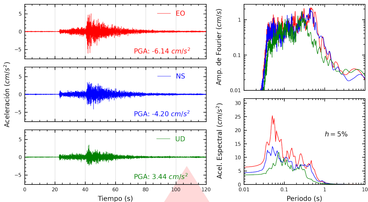
Figura A.15: Registros tiempo-historia, espectros de Fourier y de respuesta en las direcciones EO, NS y vertical de la estación OLIVO. Sismo de Pisco, Pisco - Ica del 2026-02-22, 17:36:14 (Hora local)
