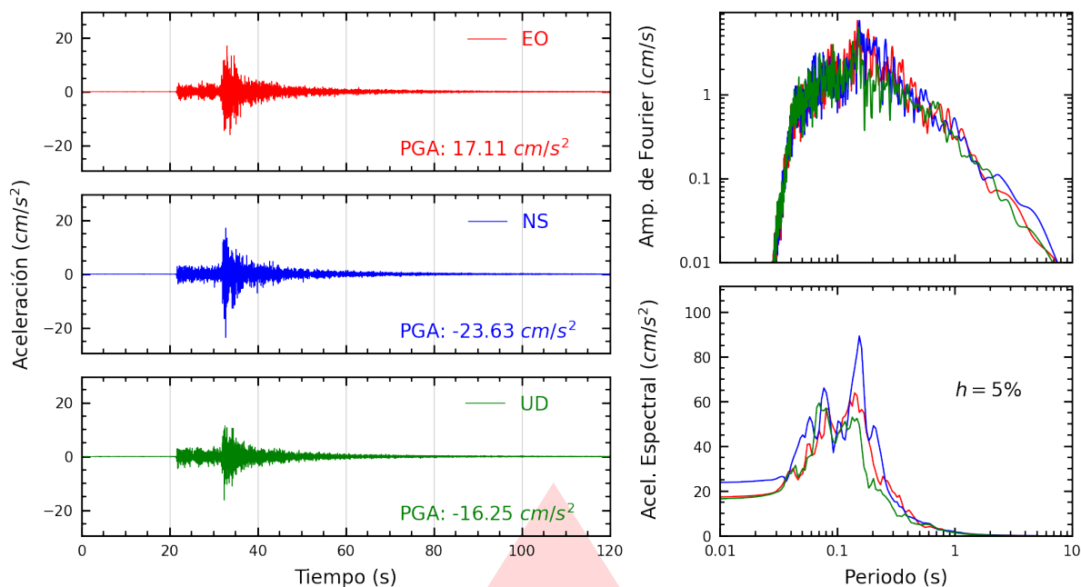
Figura A.1: Registros tiempo-historia, espectros de Fourier y de respuesta en las direcciones EO, NS y vertical de la estación ASIA. Sismo de Pisco, Pisco - Ica del 2026-02-22, 17:36:14 (Hora local)
