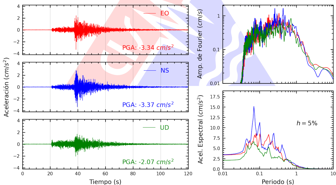
Figura A.30: Registros tiempo-historia, espectros de Fourier y de respuesta en las direcciones EO, NS y vertical de la estación SERVI. Sismo de Pisco, Pisco - Ica del 2026-02-22, 17:36:14 (Hora local)
