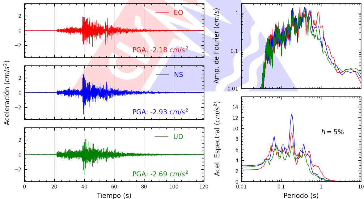
Figura A.34: Registros tiempo-historia, espectros de Fourier y de respuesta en las direcciones EO, NS y vertical de la estación UNFV. Sismo de Pisco, Pisco - Ica del 2026-02-22, 17:36:14 (Hora local)
