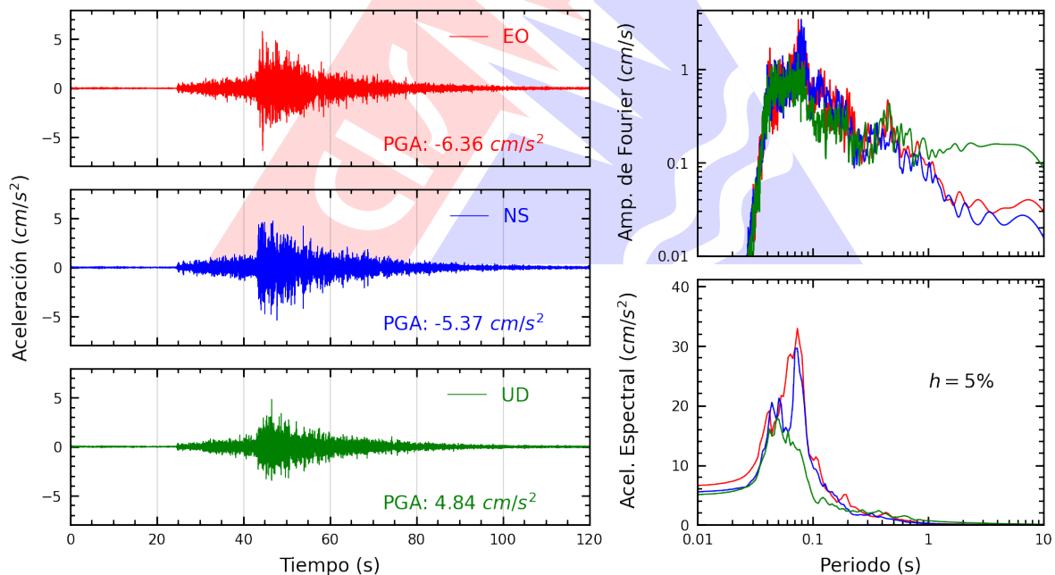
Figura A.12: Registros tiempo-historia, espectros de Fourier y de respuesta en las direcciones EO, NS y vertical de la estación JOSEO. Sismo de Pisco, Pisco - Ica del 2026-02-22, 17:36:14 (Hora local)
