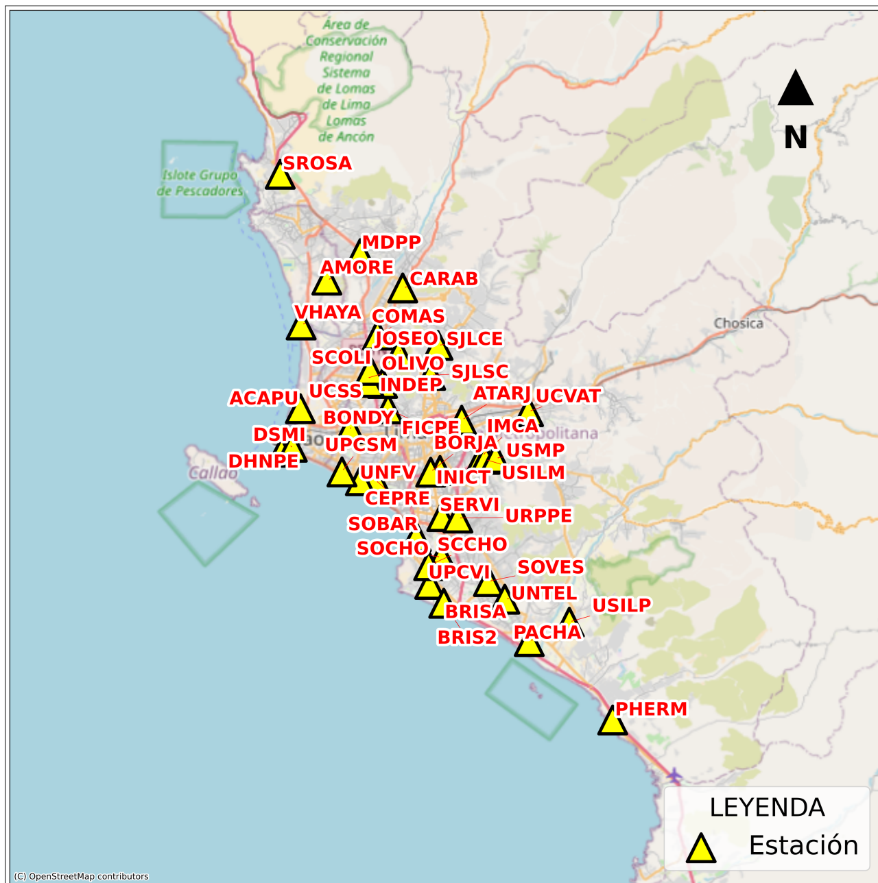
Figura 3: Mapa de ubicación de la(s) estación(es) acelerográfica(s) en Lima Metropolitana correspondiente(s) al Sismo de Pisco, Pisco - Ica del 22 de febrero de 2026 a las 17:36:14 (hora local)
