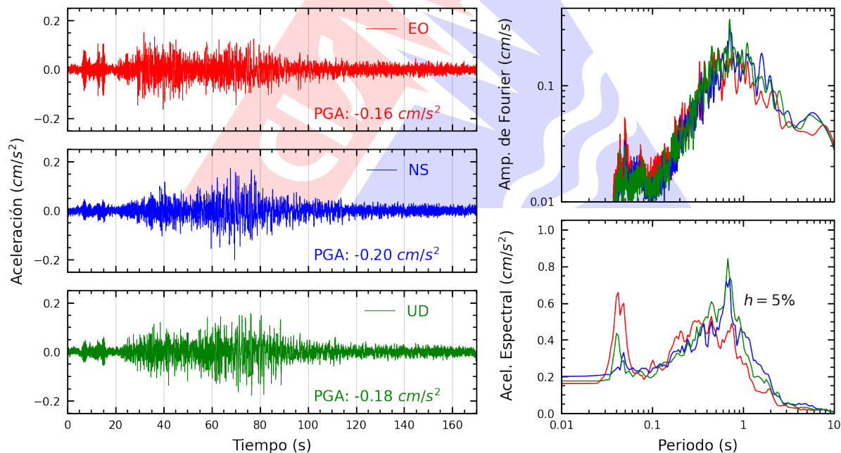
Figura A.46: Registros tiempo-historia, espectros de Fourier y de respuesta en las direcciones EO, NS y vertical de la estación UNSCH. Sismo de Pisco, Pisco - Ica del 2026-02-22, 17:36:14 (Hora local)
