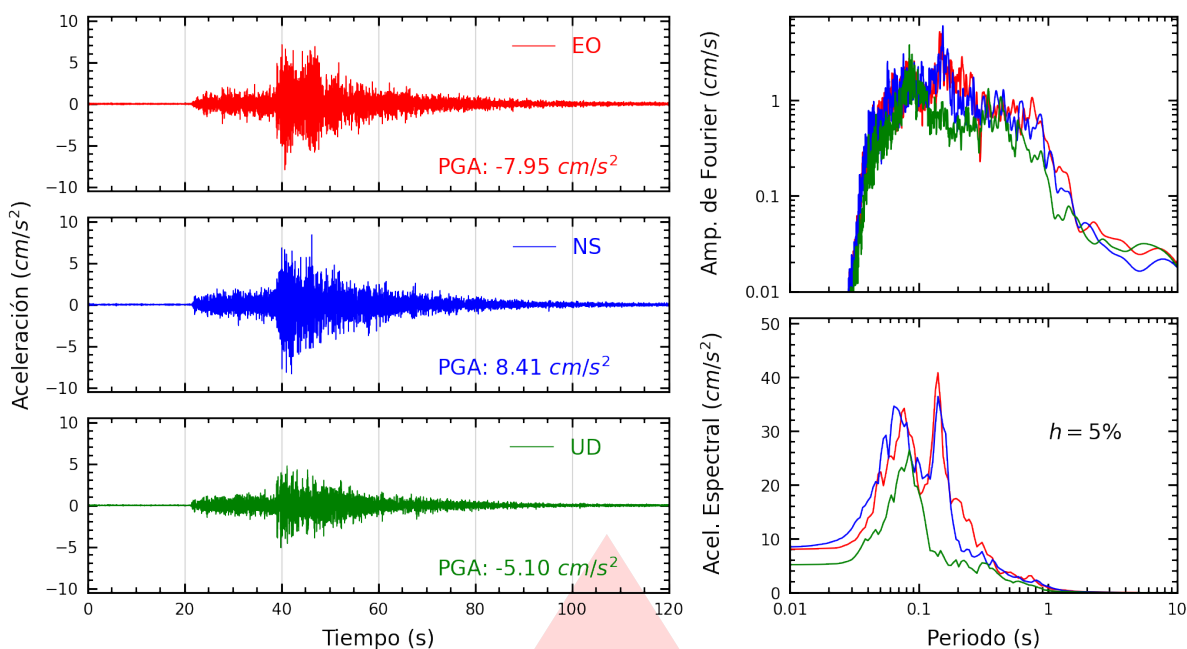
Figura A.5: Registros tiempo-historia, espectros de Fourier y de respuesta en las direcciones EO, NS y vertical de la estación USILM. Sismo de Pisco, Pisco - Ica del 2026-02-22, 17:36:14 (Hora local)
