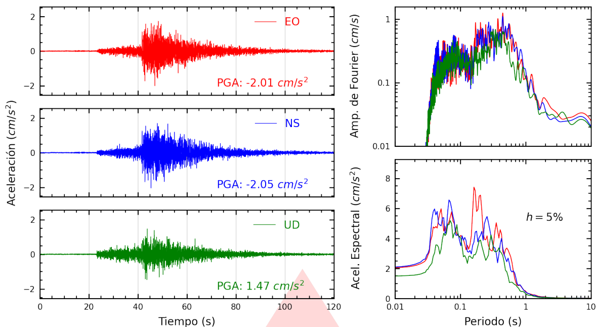
Figura A.41: Registros tiempo-historia, espectros de Fourier y de respuesta en las direcciones EO, NS y vertical de la estación COMAS. Sismo de Pisco, Pisco - Ica del 2026-02-22, 17:36:14 (Hora local)
