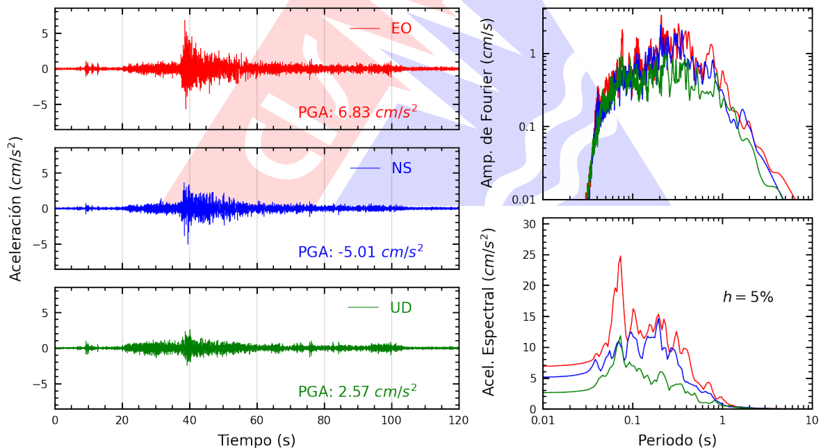
Figura A.8: Registros tiempo-historia, espectros de Fourier y de respuesta en las direcciones EO, NS y vertical de la estación SOBAR. Sismo de Pisco, Pisco - Ica del 2026-02-22, 17:36:14 (Hora local)
