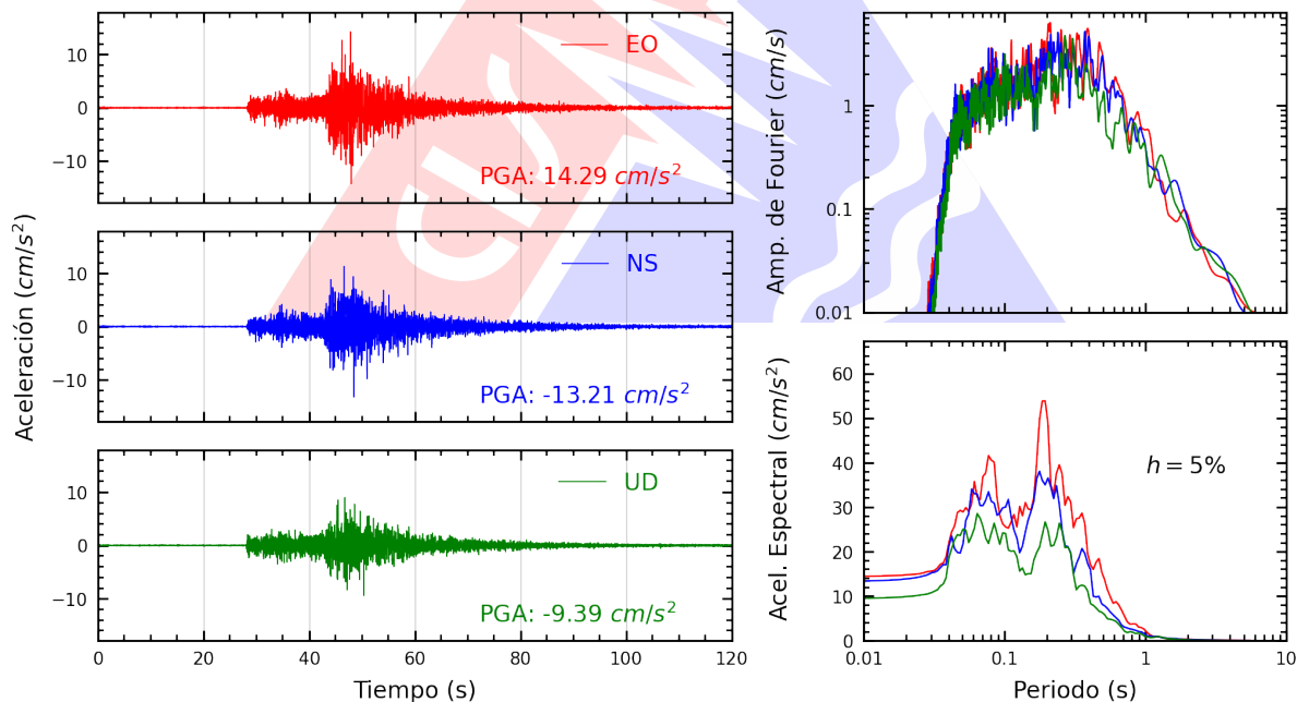
Figura A.2: Registros tiempo-historia, espectros de Fourier y de respuesta en las direcciones EO, NS y vertical de la estación PHERM. Sismo de Pisco, Pisco - Ica del 2026-02-22, 17:36:14 (Hora local)
