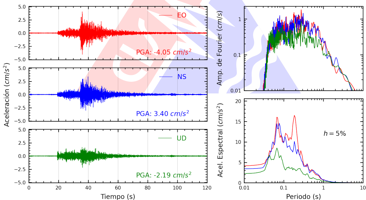
Figura A.26: Registros tiempo-historia, espectros de Fourier y de respuesta en las direcciones EO, NS y vertical de la estación PACHA. Sismo de Pisco, Pisco - Ica del 2026-02-22, 17:36:14 (Hora local)
