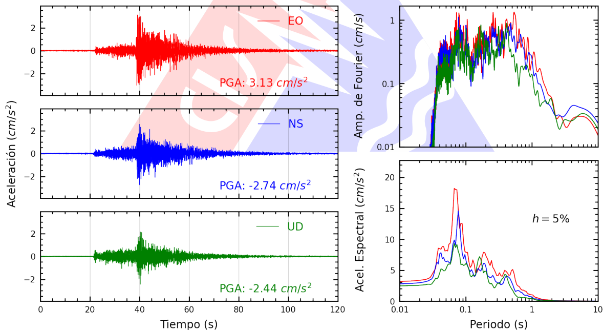
Figura A.32: Registros tiempo-historia, espectros de Fourier y de respuesta en las direcciones EO, NS y vertical de la estación CEPRE. Sismo de Pisco, Pisco - Ica del 2026-02-22, 17:36:14 (Hora local)
