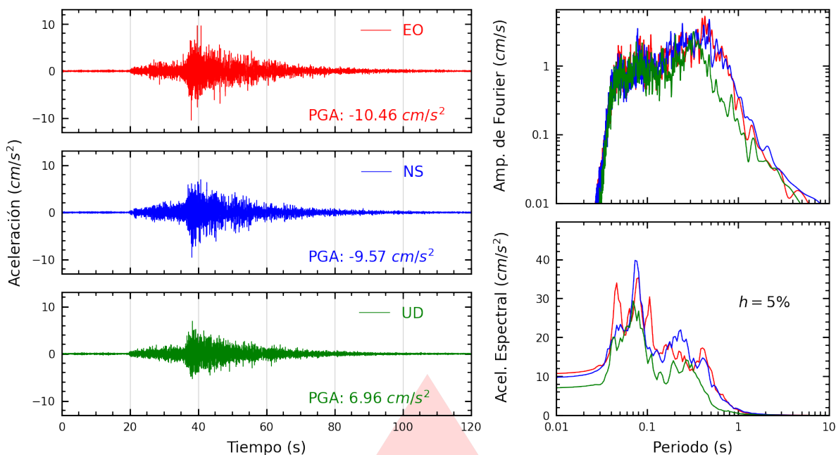
Figura A.3: Registros tiempo-historia, espectros de Fourier y de respuesta en las direcciones EO, NS y vertical de la estación UNTEL. Sismo de Pisco, Pisco - Ica del 2026-02-22, 17:36:14 (Hora local)
