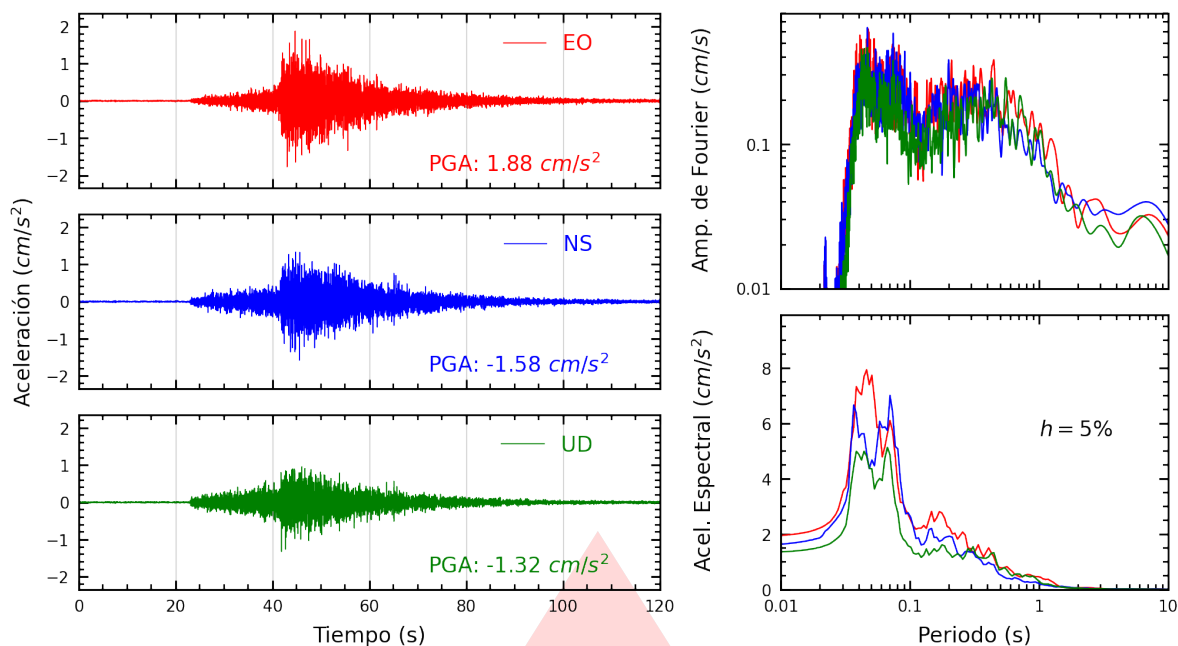
Figura A.43: Registros tiempo-historia, espectros de Fourier y de respuesta en las direcciones EO, NS y vertical de la estación SJLCE. Sismo de Pisco, Pisco - Ica del 2026-02-22, 17:36:14 (Hora local)
