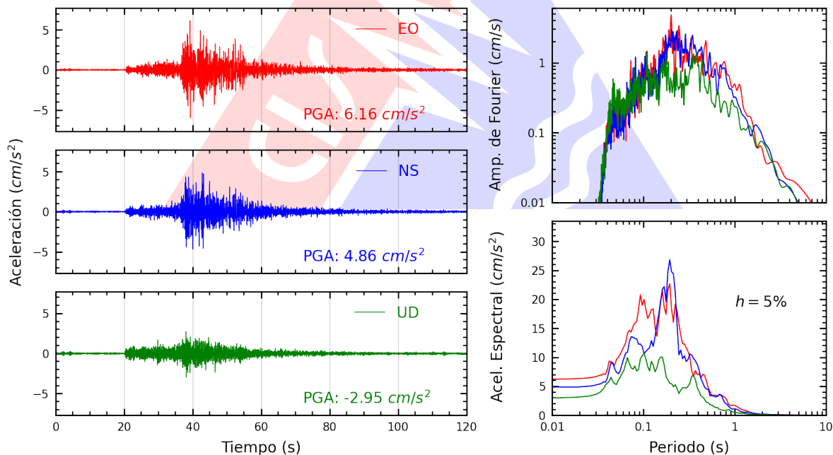
Figura A.14: Registros tiempo-historia, espectros de Fourier y de respuesta en las direcciones EO, NS y vertical de la estación SCCHO. Sismo de Pisco, Pisco - Ica del 2026-02-22, 17:36:14 (Hora local)
