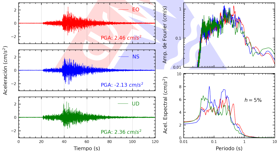
Figura A.40: Registros tiempo-historia, espectros de Fourier y de respuesta en las direcciones EO, NS y vertical de la estación USMP. Sismo de Pisco, Pisco - Ica del 2026-02-22, 17:36:14 (Hora local)
