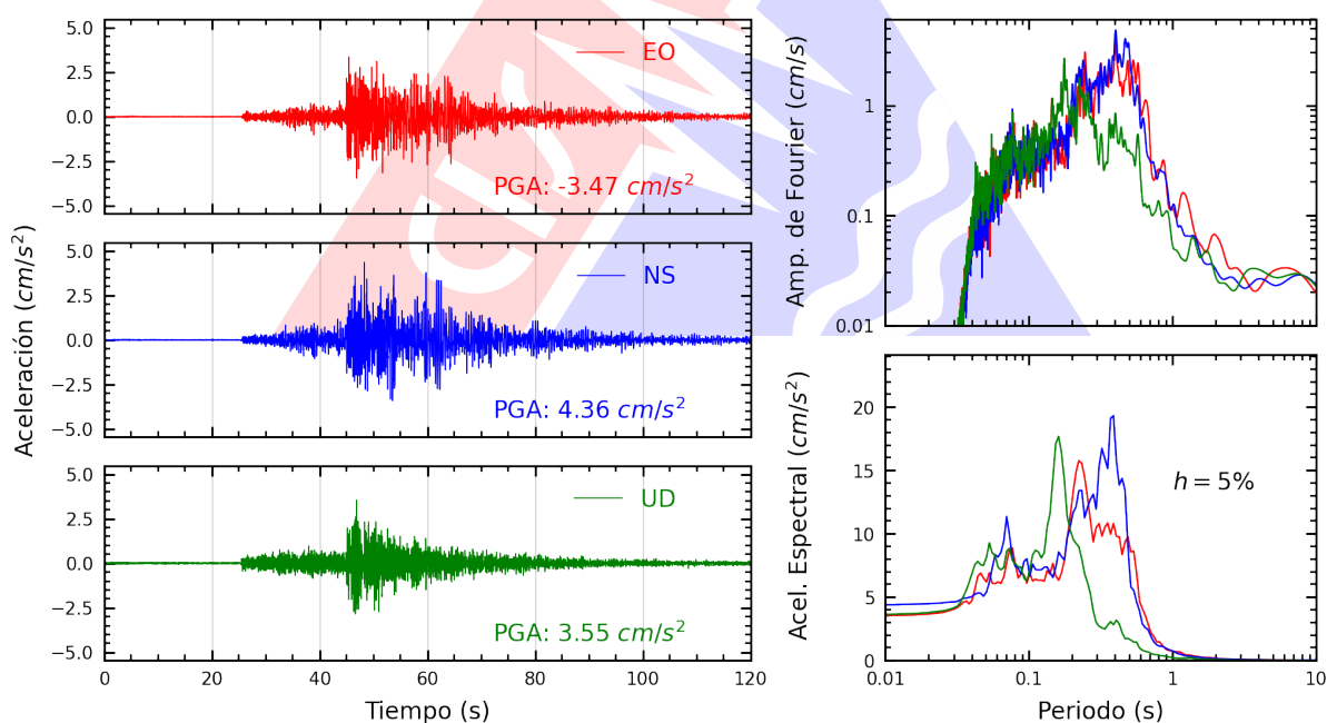
Figura A.24: Registros tiempo-historia, espectros de Fourier y de respuesta en las direcciones EO, NS y vertical de la estación MDPP. Sismo de Pisco, Pisco - Ica del 2026-02-22, 17:36:14 (Hora local)
