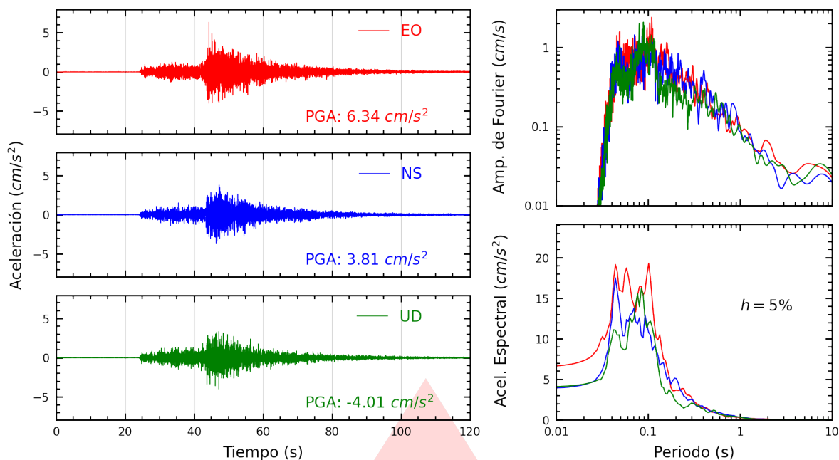
Figura A.13: Registros tiempo-historia, espectros de Fourier y de respuesta en las direcciones EO, NS y vertical de la estación AMORE. Sismo de Pisco, Pisco - Ica del 2026-02-22, 17:36:14 (Hora local)
