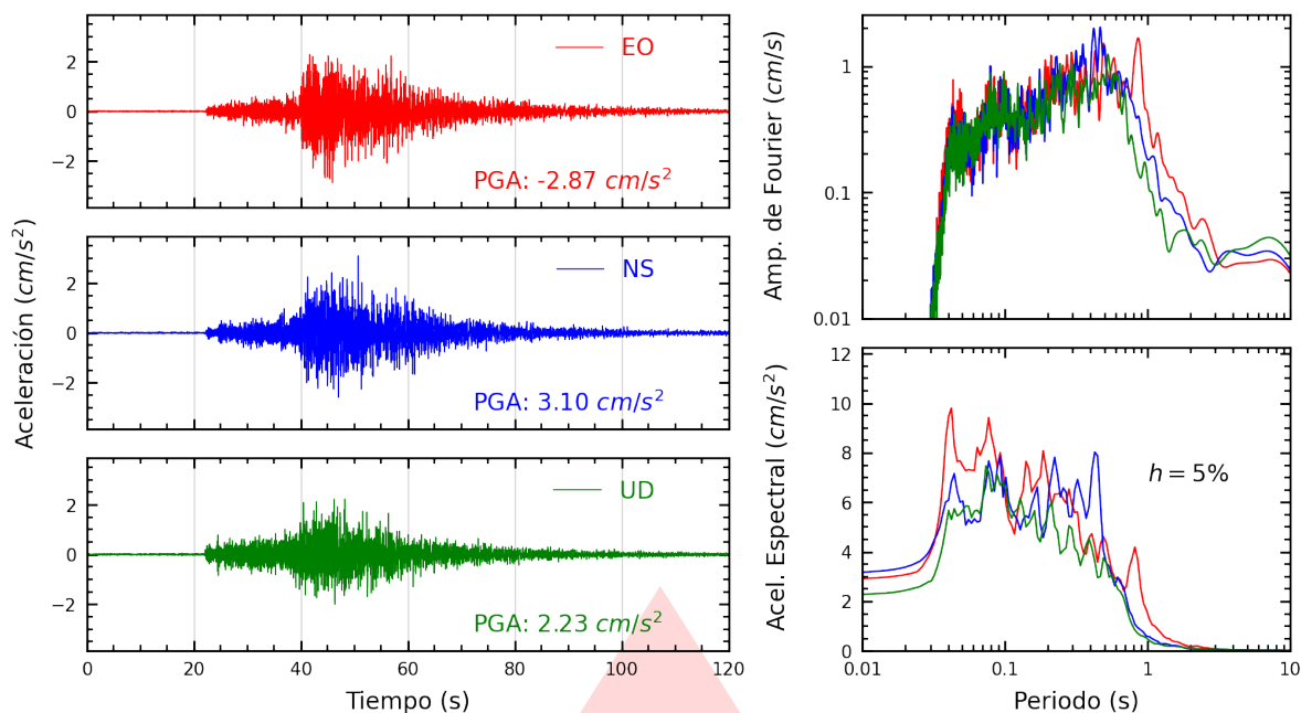
Figura A.33: Registros tiempo-historia, espectros de Fourier y de respuesta en las direcciones EO, NS y vertical de la estación UCVAT. Sismo de Pisco, Pisco - Ica del 2026-02-22, 17:36:14 (Hora local)
