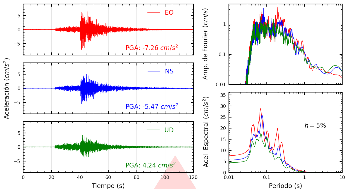
Figura A.7: Registros tiempo-historia, espectros de Fourier y de respuesta en las direcciones EO, NS y vertical de la estación INDEP. Sismo de Pisco, Pisco - Ica del 2026-02-22, 17:36:14 (Hora local)
