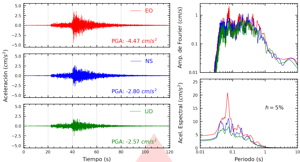
Figura A.23: Registros tiempo-historia, espectros de Fourier y de respuesta en las direcciones EO, NS y vertical de la estación FICPE. Sismo de Pisco, Pisco - Ica del 2026-02-22, 17:36:14 (Hora local)
