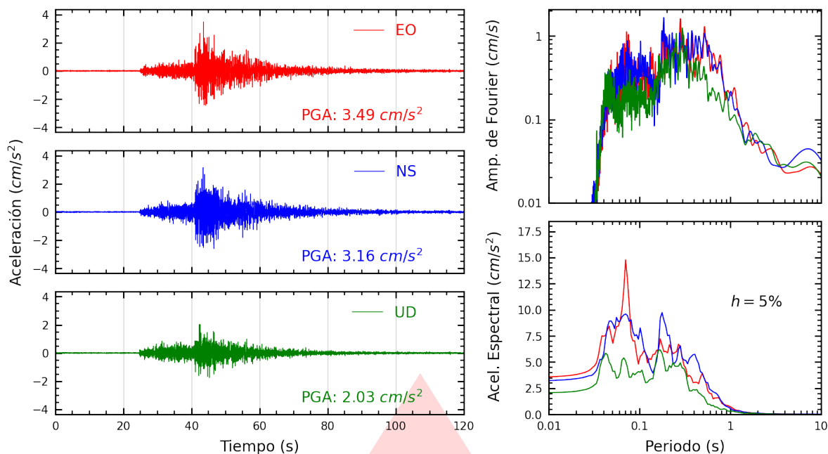
Figura A.29: Registros tiempo-historia, espectros de Fourier y de respuesta en las direcciones EO, NS y vertical de la estación UPCVI. Sismo de Pisco, Pisco - Ica del 2026-02-22, 17:36:14 (Hora local)
