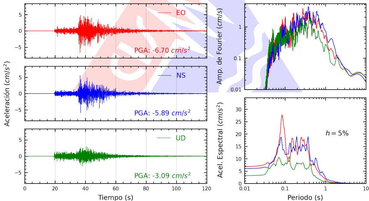
Figura A.10: Registros tiempo-historia, espectros de Fourier y de respuesta en las direcciones EO, NS y vertical de la estación USILP. Sismo de Pisco, Pisco - Ica del 2026-02-22, 17:36:14 (Hora local)
