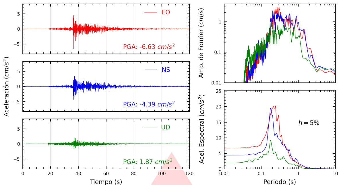
Figura A.11: Registros tiempo-historia, espectros de Fourier y de respuesta en las direcciones EO, NS y vertical de la estación DSMI. Sismo de Pisco, Pisco - Ica del 2026-02-22, 17:36:14 (Hora local)
