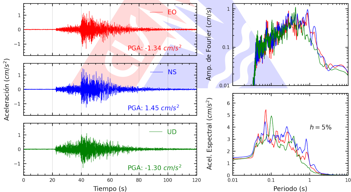
Figura A.44: Registros tiempo-historia, espectros de Fourier y de respuesta en las direcciones EO, NS y vertical de la estación BONDY. Sismo de Pisco, Pisco - Ica del 2026-02-22, 17:36:14 (Hora local)
