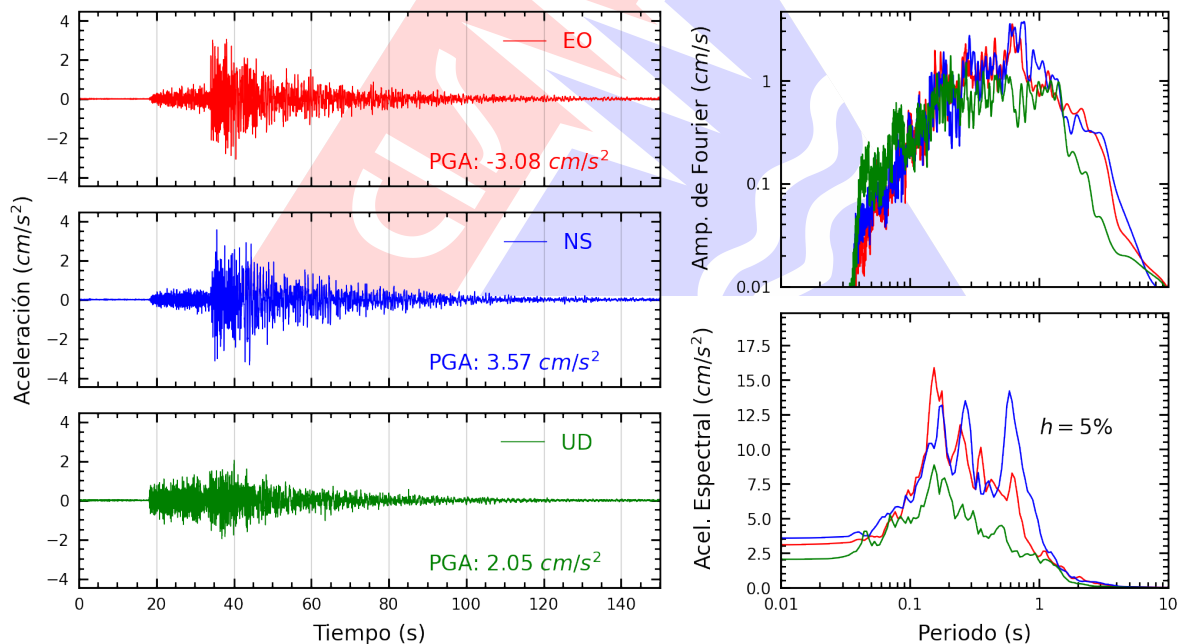
Figura A.28: Registros tiempo-historia, espectros de Fourier y de respuesta en las direcciones EO, NS y vertical de la estación UNICA. Sismo de Pisco, Pisco - Ica del 2026-02-22, 17:36:14 (Hora local)
