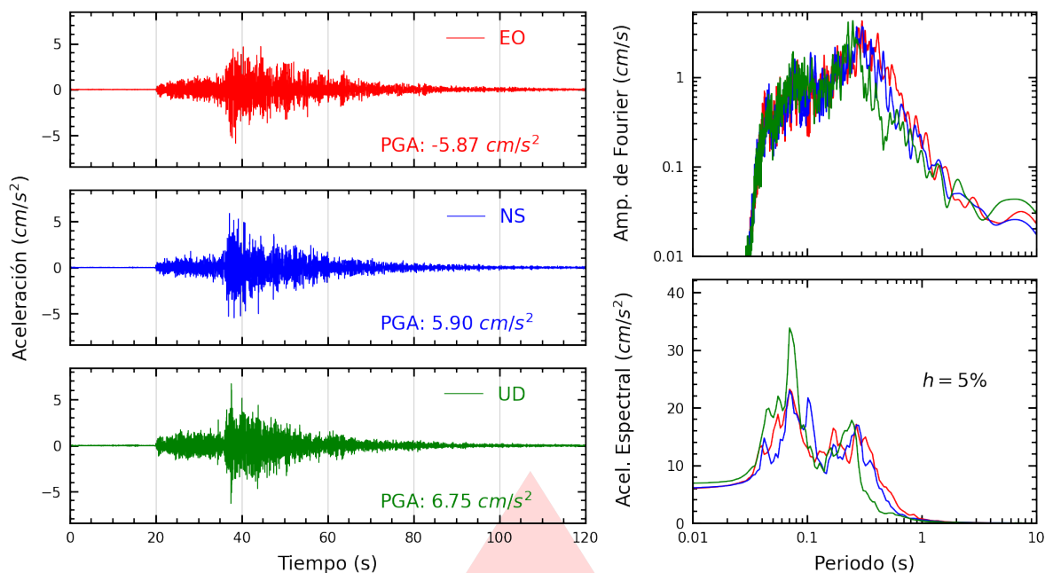
Figura A.9: Registros tiempo-historia, espectros de Fourier y de respuesta en las direcciones EO, NS y vertical de la estación SOVES. Sismo de Pisco, Pisco - Ica del 2026-02-22, 17:36:14 (Hora local)
