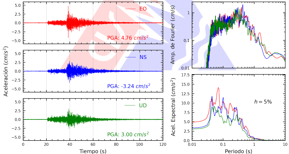
Figura A.22: Registros tiempo-historia, espectros de Fourier y de respuesta en las direcciones EO, NS y vertical de la estación URPE. Sismo de Pisco, Pisco - Ica del 2026-02-22, 17:36:14 (Hora local)
