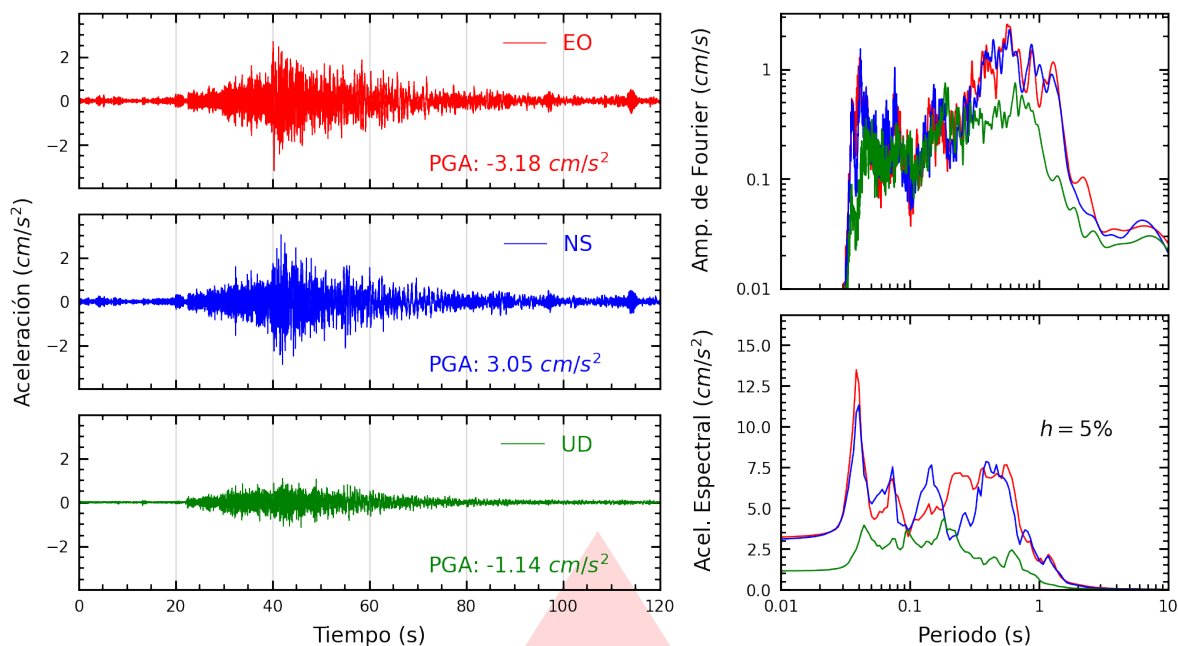
Figura A.31: Registros tiempo-historia, espectros de Fourier y de respuesta en las direcciones EO, NS y vertical de la estación DHNPE. Sismo de Pisco, Pisco - Ica del 2026-02-22, 17:36:14 (Hora local)
