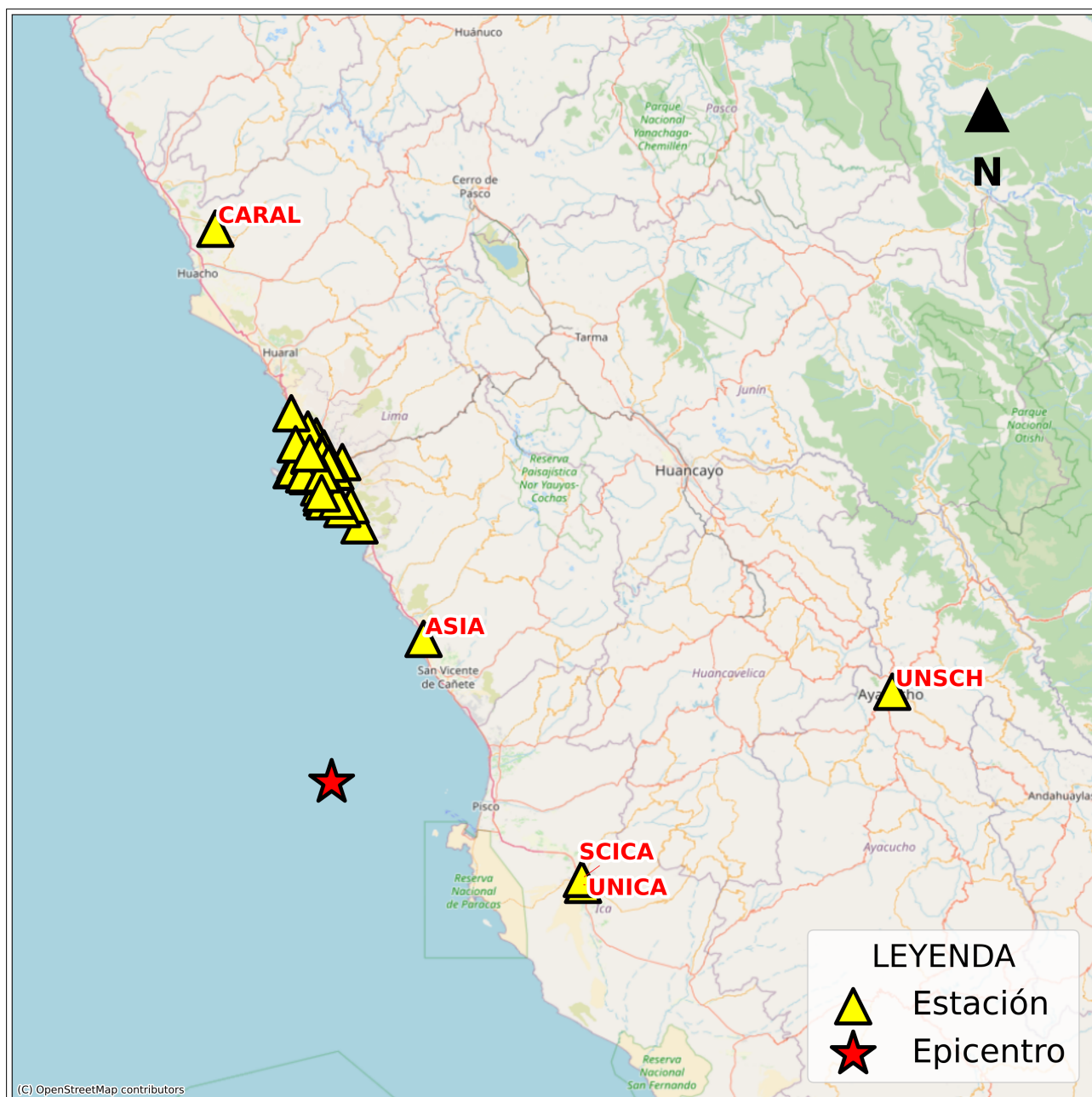
Figura 2: Mapa de ubicación de la(s) estación(es) acelerográfica(s) a nivel nacional correspondiente(s) al Sismo de Pisco, Pisco - Ica del 22 de febrero de 2026 a las 17:36:14 (hora local)
