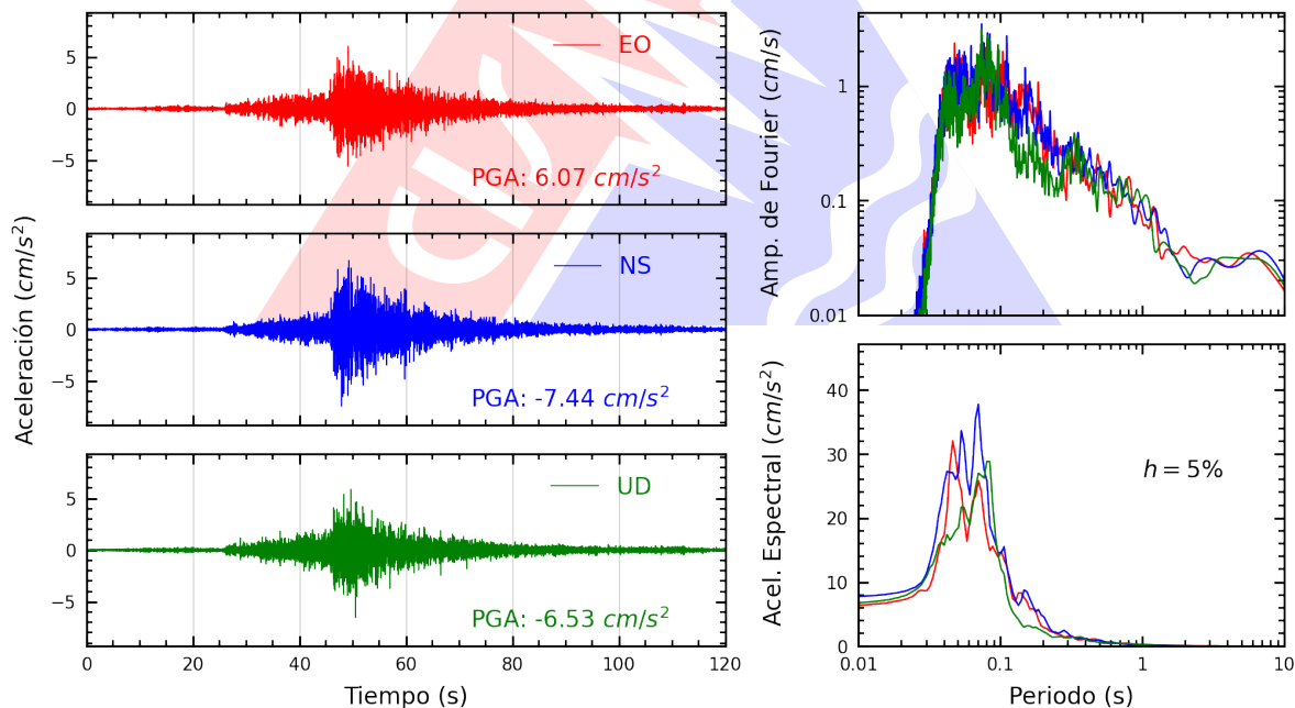
Figura A.6: Registros tiempo-historia, espectros de Fourier y de respuesta en las direcciones EO, NS y vertical de la estación SROSA. Sismo de Pisco, Pisco - Ica del 2026-02-22, 17:36:14 (Hora local)
