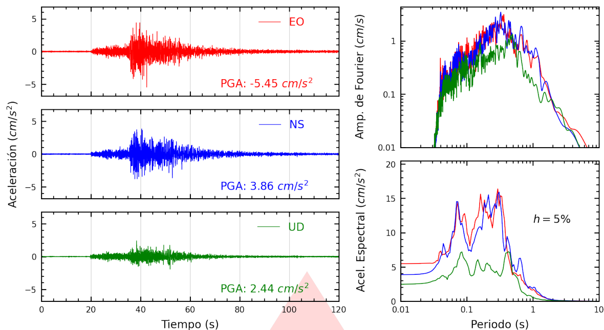
Figura A.19: Registros tiempo-historia, espectros de Fourier y de respuesta en las direcciones EO, NS y vertical de la estación BRISA. Sismo de Pisco, Pisco - Ica del 2026-02-22, 17:36:14 (Hora local)
