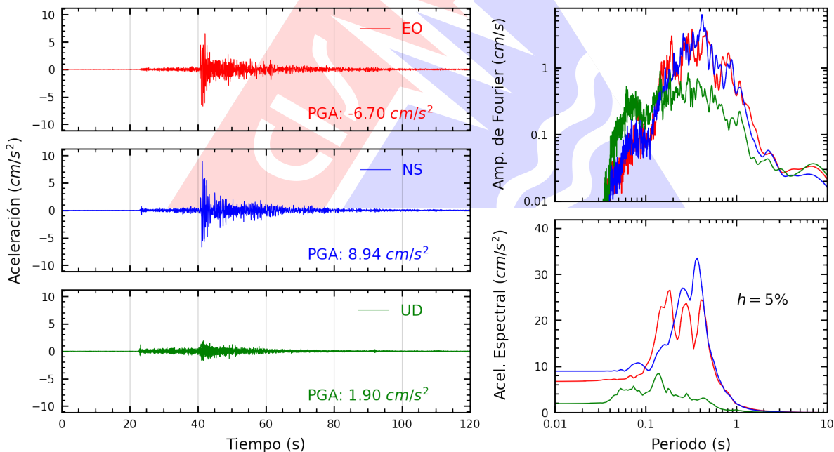
Figura A.4: Registros tiempo-historia, espectros de Fourier y de respuesta en las direcciones EO, NS y vertical de la estación ACAPU. Sismo de Pisco, Pisco - Ica del 2026-02-22, 17:36:14 (Hora local)
