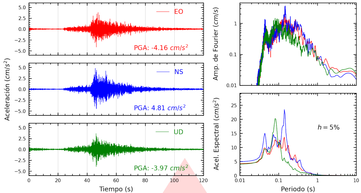
Figura A.21: Registros tiempo-historia, espectros de Fourier y de respuesta en las direcciones EO, NS y vertical de la estación CARAB. Sismo de Pisco, Pisco - Ica del 2026-02-22, 17:36:14 (Hora local)
