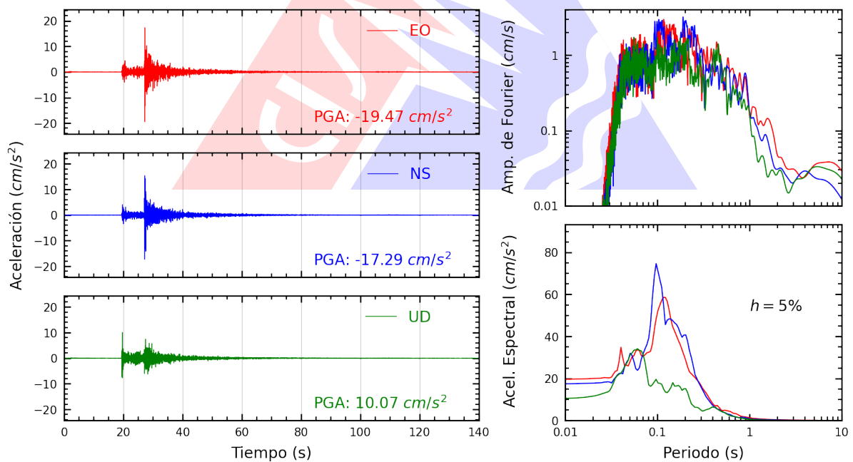
Figura A.24: Registros tiempo-historia, espectros de Fourier y de respuesta en las direcciones EO, NS y vertical de la estación INICT. Sismo de Chilca, Cañete - Lima del 2026-02-26, 18:21:08 (Hora local)
