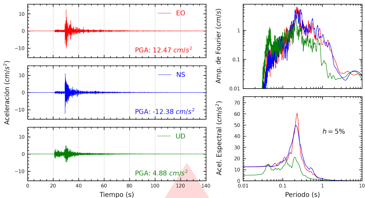
Figura A.35: Registros tiempo-historia, espectros de Fourier y de respuesta en las direcciones EO, NS y vertical de la estación DSMI. Sismo de Chilca, Cañete - Lima del 2026-02-26, 18:21:08 (Hora local)
