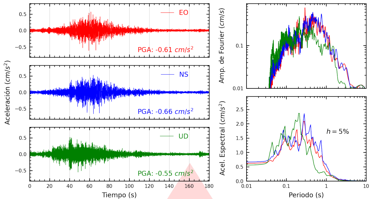
Figura A.45: Registros tiempo-historia, espectros de Fourier y de respuesta en las direcciones EO, NS y vertical de la estación UNICA. Sismo de Chilca, Cañete - Lima del 2026-02-26, 18:21:08 (Hora local)
