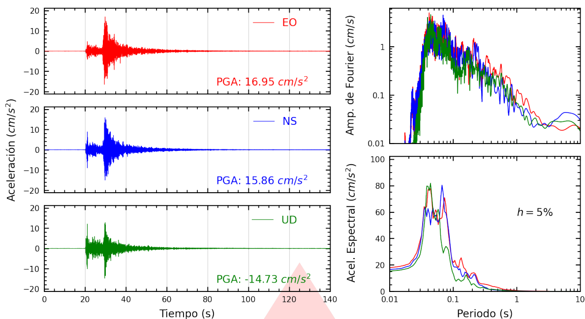
Figura A.27: Registros tiempo-historia, espectros de Fourier y de respuesta en las direcciones EO, NS y vertical de la estación SJLCE. Sismo de Chilca, Cañete - Lima del 2026-02-26, 18:21:08 (Hora local)
