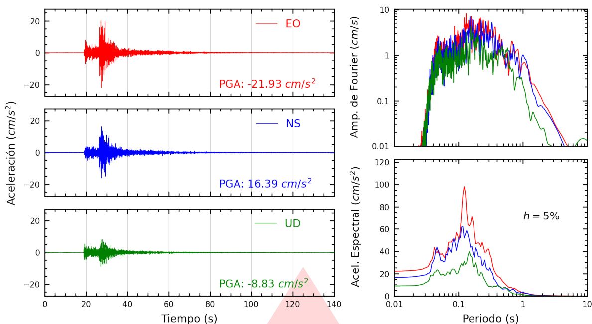
Figura A.21: Registros tiempo-historia, espectros de Fourier y de respuesta en las direcciones EO, NS y vertical de la estación BRISA. Sismo de Chilca, Cañete - Lima del 2026-02-26, 18:21:08 (Hora local)
