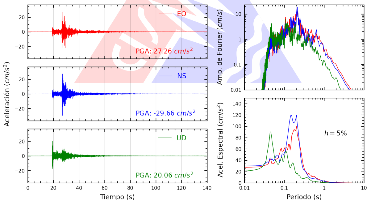
Figura A.12: Registros tiempo-historia, espectros de Fourier y de respuesta en las direcciones EO, NS y vertical de la estación SCCHO. Sismo de Chilca, Cañete - Lima del 2026-02-26, 18:21:08 (Hora local)
