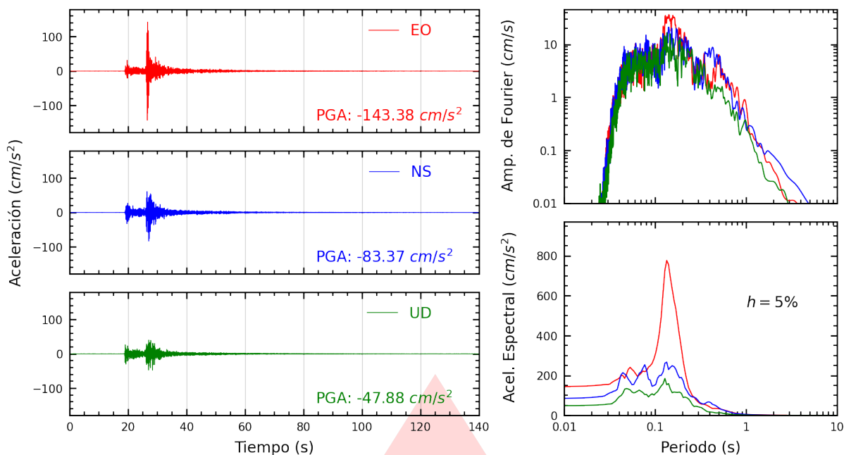
Figura A.1: Registros tiempo-historia, espectros de Fourier y de respuesta en las direcciones EO, NS y vertical de la estación PHERM. Sismo de Chilca, Cañete - Lima del 2026-02-26, 18:21:08 (Hora local)
