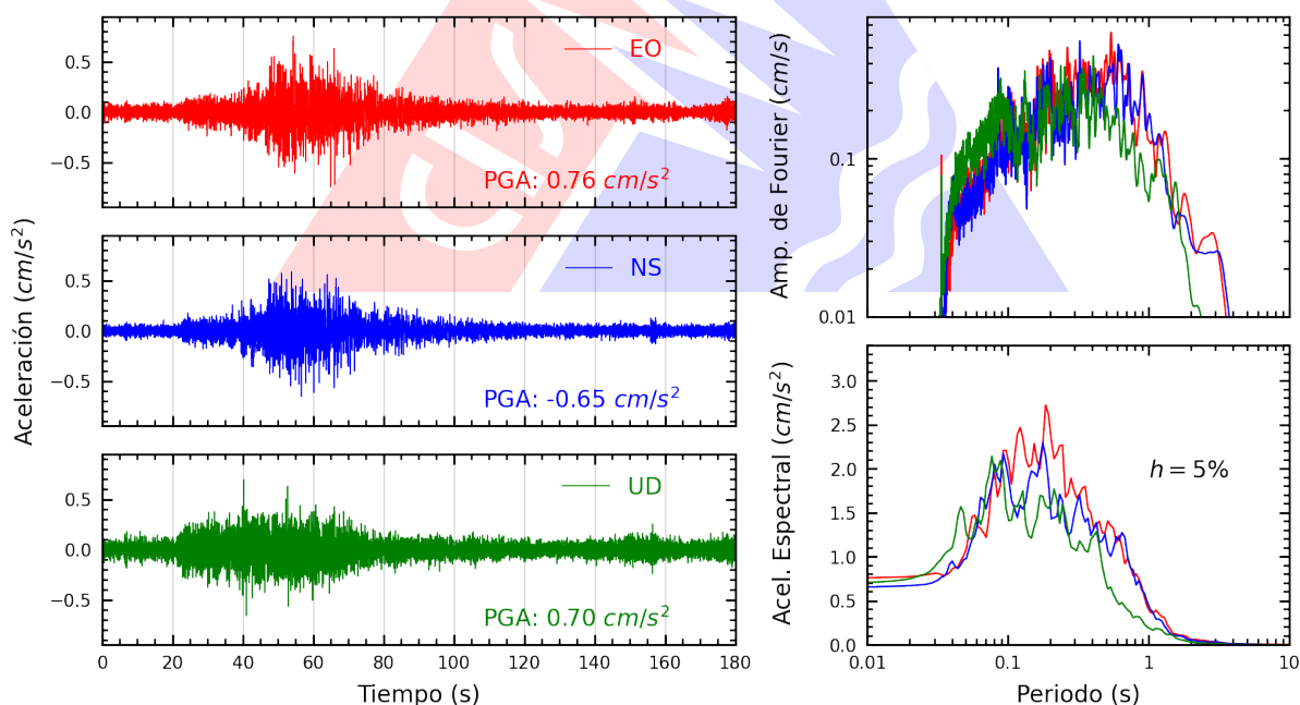
Figura A.44: Registros tiempo-historia, espectros de Fourier y de respuesta en las direcciones EO, NS y vertical de la estación SCICA. Sismo de Chilca, Cañete - Lima del 2026-02-26, 18:21:08 (Hora local)
