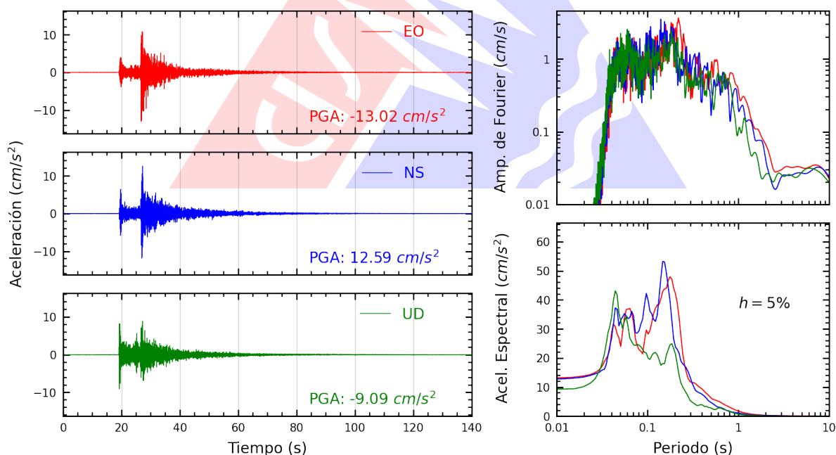
Figura A.34: Registros tiempo-historia, espectros de Fourier y de respuesta en las direcciones EO, NS y vertical de la estación SERVI. Sismo de Chilca, Cañete - Lima del 2026-02-26, 18:21:08 (Hora local)
