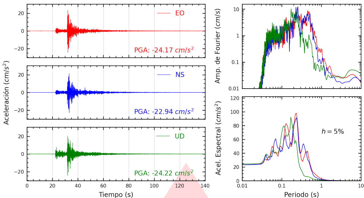
Figura A.19: Registros tiempo-historia, espectros de Fourier y de respuesta en las direcciones EO, NS y vertical de la estación MDPP. Sismo de Chilca, Cañete - Lima del 2026-02-26, 18:21:08 (Hora local)
