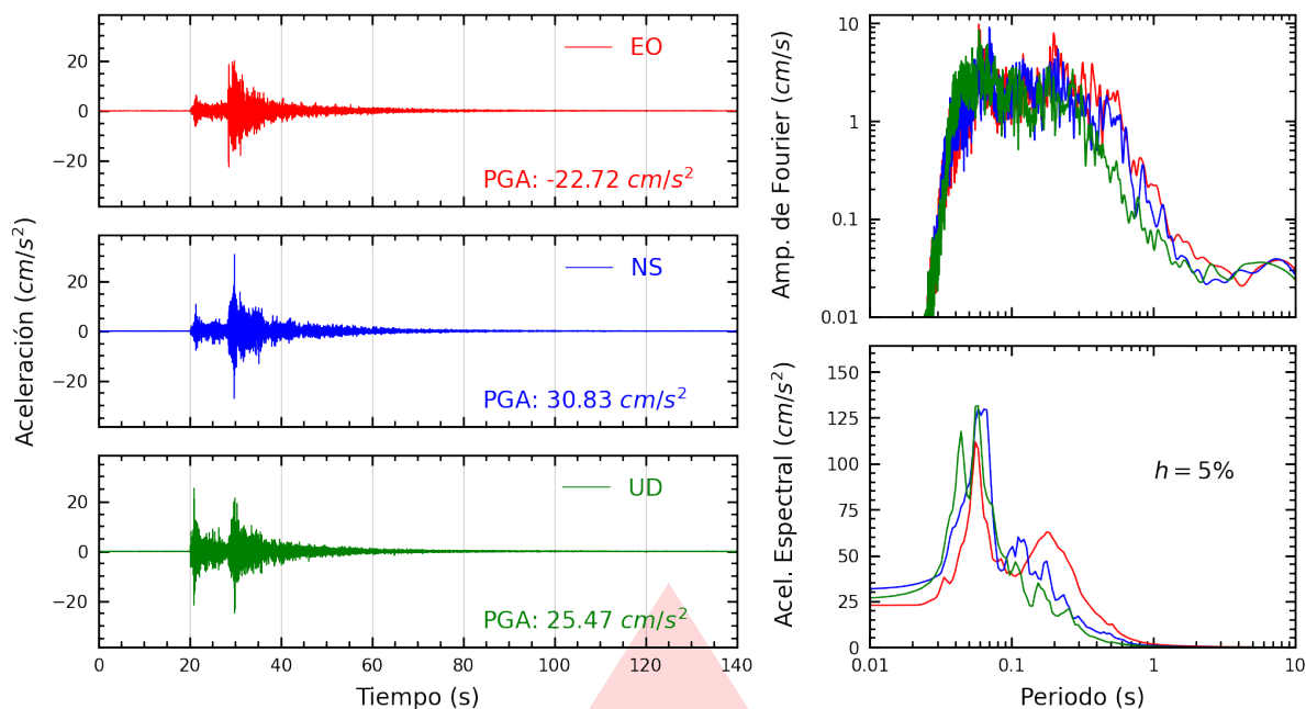
Figura A.11: Registros tiempo-historia, espectros de Fourier y de respuesta en las direcciones EO, NS y vertical de la estación SJLSC. Sismo de Chilca, Cañete - Lima del 2026-02-26, 18:21:08 (Hora local)
