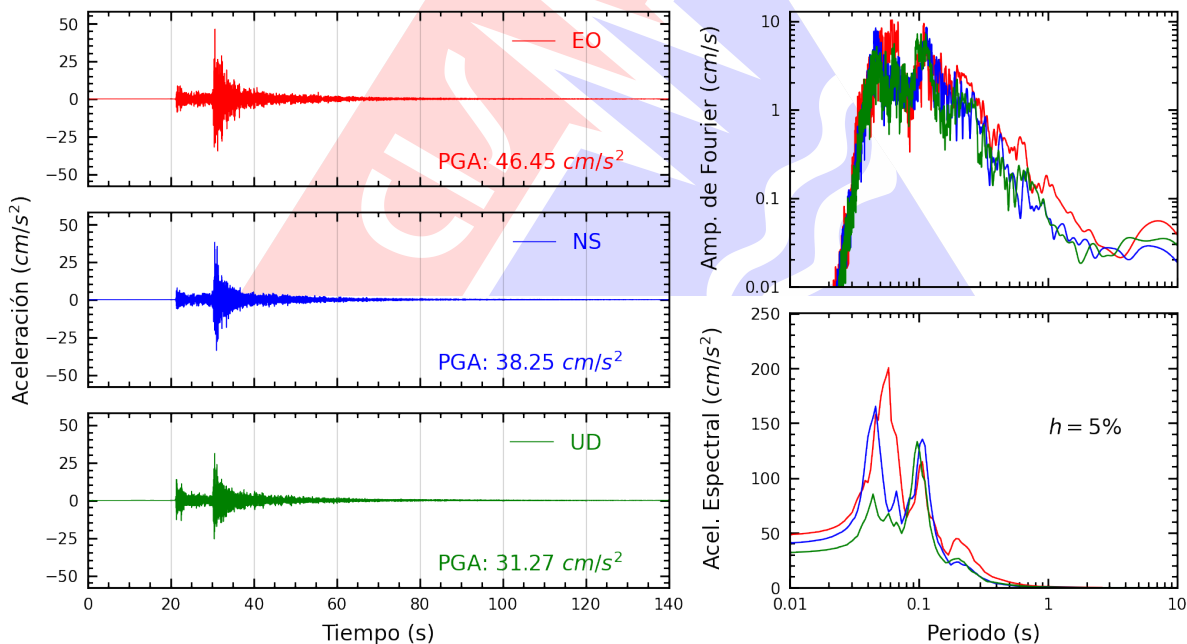
Figura A.2: Registros tiempo-historia, espectros de Fourier y de respuesta en las direcciones EO, NS y vertical de la estación AMORE. Sismo de Chilca, Cañete - Lima del 2026-02-26, 18:21:08 (Hora local)
