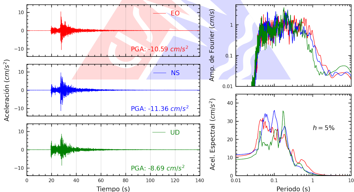
Figura A.38: Registros tiempo-historia, espectros de Fourier y de respuesta en las direcciones EO, NS y vertical de la estación UNFV. Sismo de Chilca, Cañete - Lima del 2026-02-26, 18:21:08 (Hora local)
