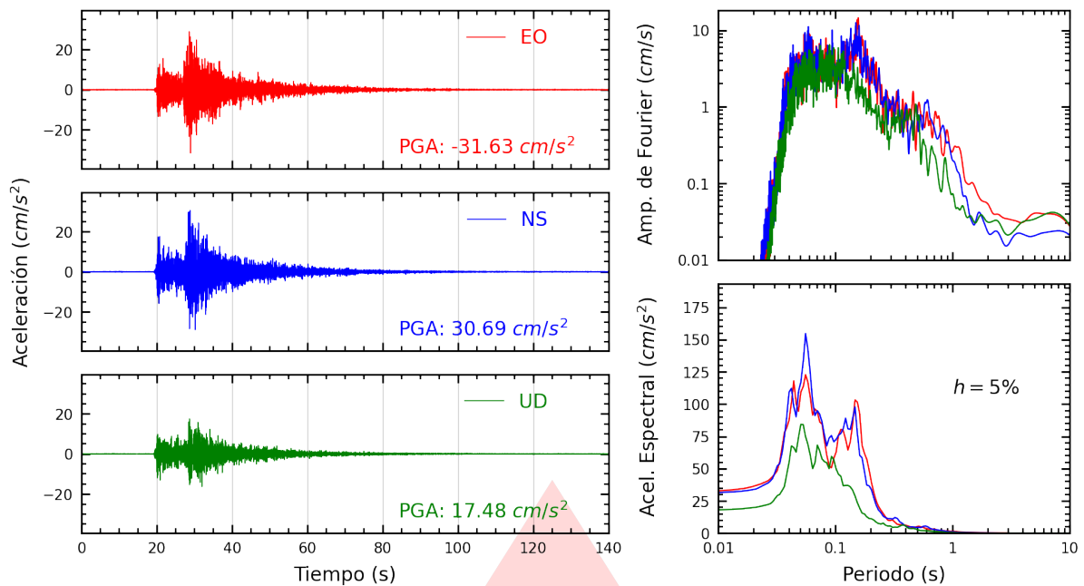
Figura A.9: Registros tiempo-historia, espectros de Fourier y de respuesta en las direcciones EO, NS y vertical de la estación USILM. Sismo de Chilca, Cañete - Lima del 2026-02-26, 18:21:08 (Hora local)
