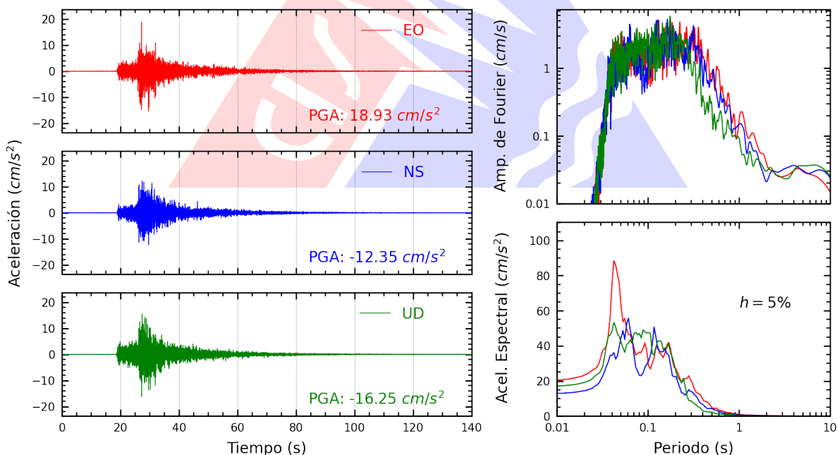
Figura A.26: Registros tiempo-historia, espectros de Fourier y de respuesta en las direcciones EO, NS y vertical de la estación SOVES. Sismo de Chilca, Cañete - Lima del 2026-02-26, 18:21:08 (Hora local)
