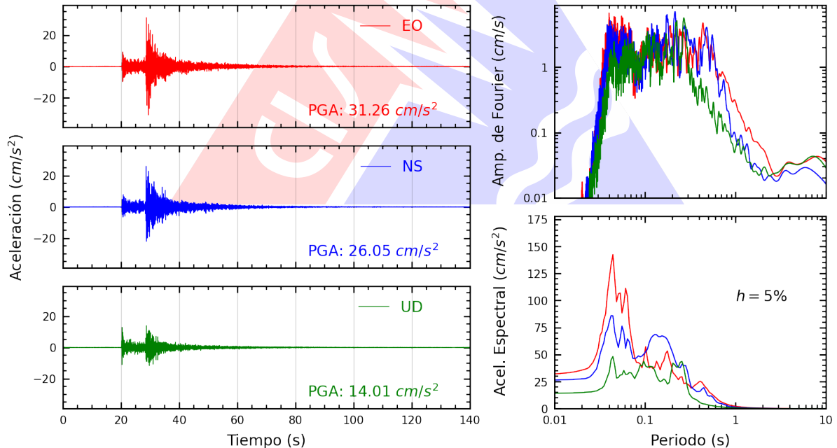
Figura A.10: Registros tiempo-historia, espectros de Fourier y de respuesta en las direcciones EO, NS y vertical de la estación OLIVO. Sismo de Chilca, Cañete - Lima del 2026-02-26, 18:21:08 (Hora local)
