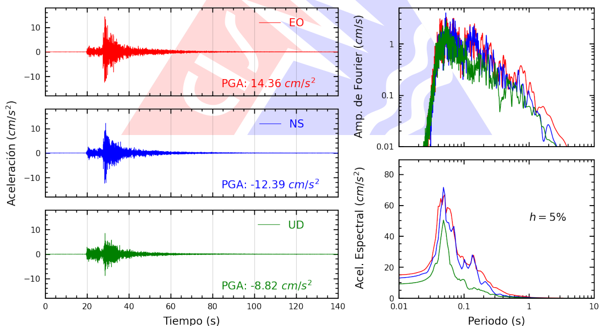
Figura A.32: Registros tiempo-historia, espectros de Fourier y de respuesta en las direcciones EO, NS y vertical de la estación ATARJ. Sismo de Chilca, Cañete - Lima del 2026-02-26, 18:21:08 (Hora local)
