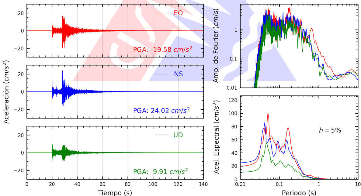
Figura A.20: Registros tiempo-historia, espectros de Fourier y de respuesta en las direcciones EO, NS y vertical de la estación FICPE. Sismo de Chilca, Cañete - Lima del 2026-02-26, 18:21:08 (Hora local)
