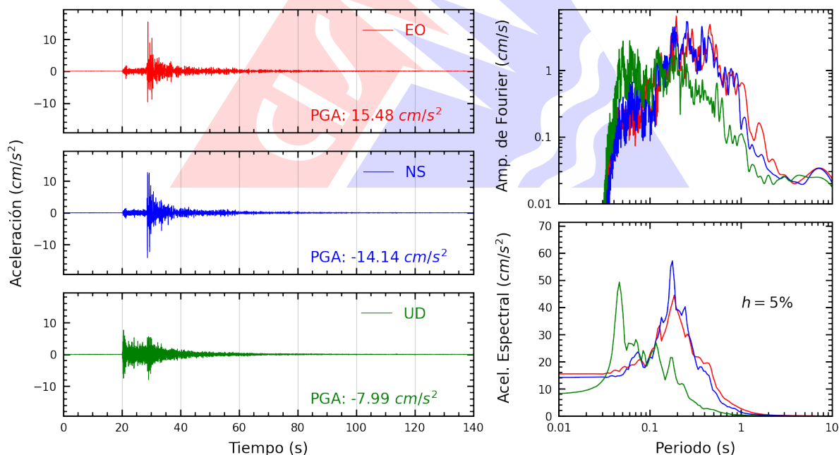
Figura A.30: Registros tiempo-historia, espectros de Fourier y de respuesta en las direcciones EO, NS y vertical de la estación ACAPU. Sismo de Chilca, Cañete - Lima del 2026-02-26, 18:21:08 (Hora local)
