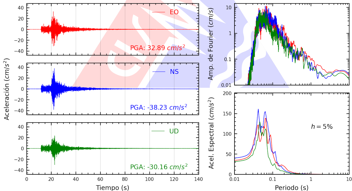
Figura A.8: Registros tiempo-historia, espectros de Fourier y de respuesta en las direcciones EO, NS y vertical de la estación JOSEO. Sismo de Chilca, Cañete - Lima del 2026-02-26, 18:21:08 (Hora local)
