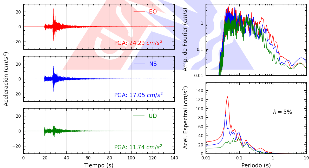
Figura A.18: Registros tiempo-historia, espectros de Fourier y de respuesta en las direcciones EO, NS y vertical de la estación CEPRE. Sismo de Chilca, Cañete - Lima del 2026-02-26, 18:21:08 (Hora local)
