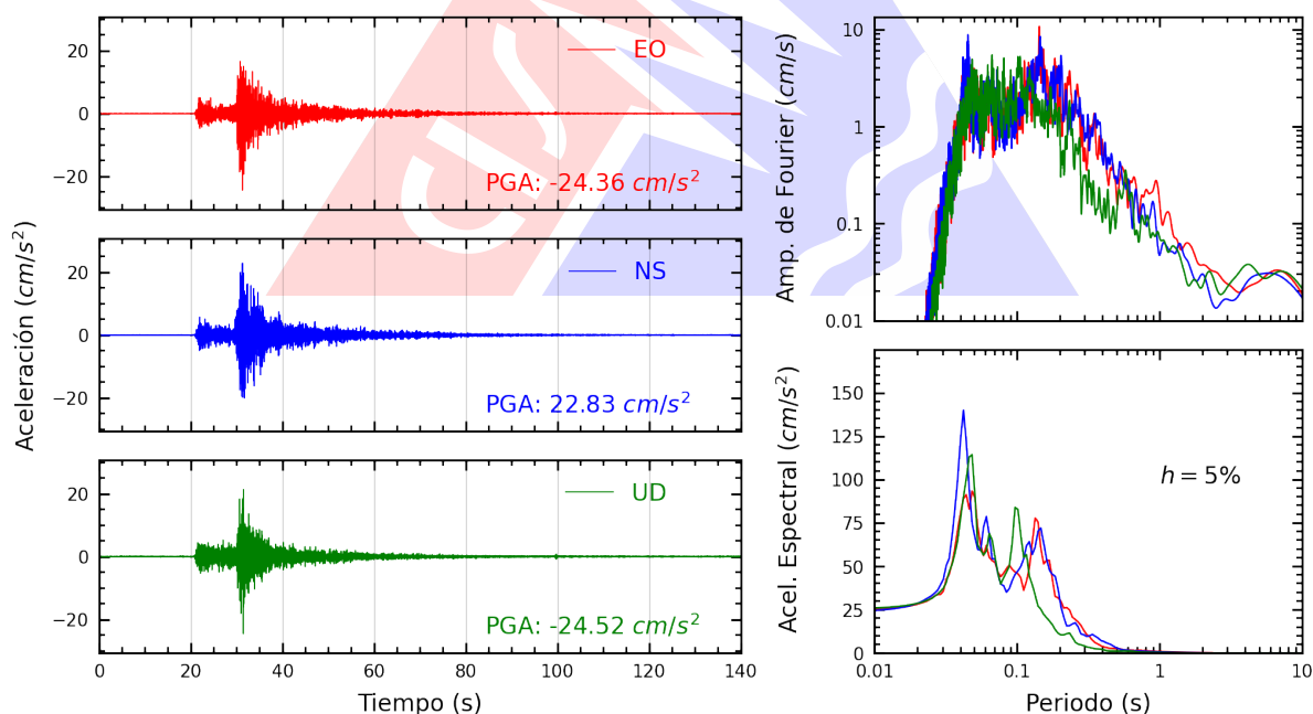
Figura A.16: Registros tiempo-historia, espectros de Fourier y de respuesta en las direcciones EO, NS y vertical de la estación CARAB. Sismo de Chilca, Cañete - Lima del 2026-02-26, 18:21:08 (Hora local)
