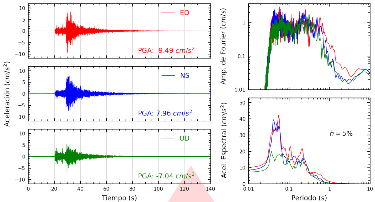
Figura A.41: Registros tiempo-historia, espectros de Fourier y de respuesta en las direcciones EO, NS y vertical de la estación COMAS. Sismo de Chilca, Cañete - Lima del 2026-02-26, 18:21:08 (Hora local)
