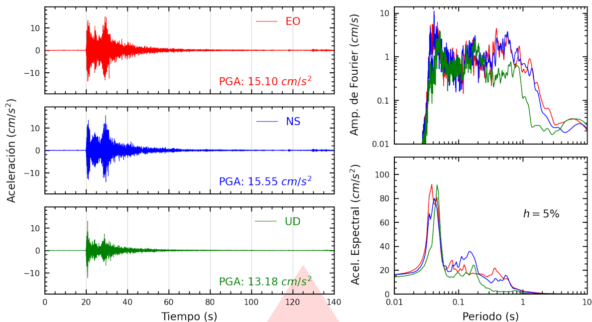
Figura A.29: Registros tiempo-historia, espectros de Fourier y de respuesta en las direcciones EO, NS y vertical de la estación DHNPE. Sismo de Chilca, Cañete - Lima del 2026-02-26, 18:21:08 (Hora local)
