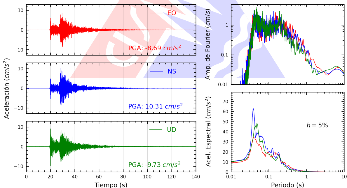
Figura A.40: Registros tiempo-historia, espectros de Fourier y de respuesta en las direcciones EO, NS y vertical de la estación USMP. Sismo de Chilca, Cañete - Lima del 2026-02-26, 18:21:08 (Hora local)
