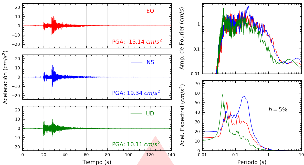
Figura A.25: Registros tiempo-historia, espectros de Fourier y de respuesta en las direcciones EO, NS y vertical de la estación UPCSM. Sismo de Chilca, Cañete - Lima del 2026-02-26, 18:21:08 (Hora local)
