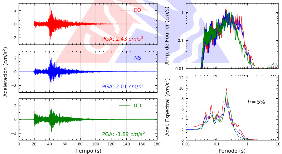
Figura A.42: Registros tiempo-historia, espectros de Fourier y de respuesta en las direcciones EO, NS y vertical de la estación CARAL. Sismo de Chilca, Cañete - Lima del 2026-02-26, 18:21:08 (Hora local)
