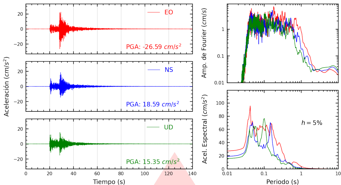
Figura A.15: Registros tiempo-historia, espectros de Fourier y de respuesta en las direcciones EO, NS y vertical de la estación UCVAT. Sismo de Chilca, Cañete - Lima del 2026-02-26, 18:21:08 (Hora local)
