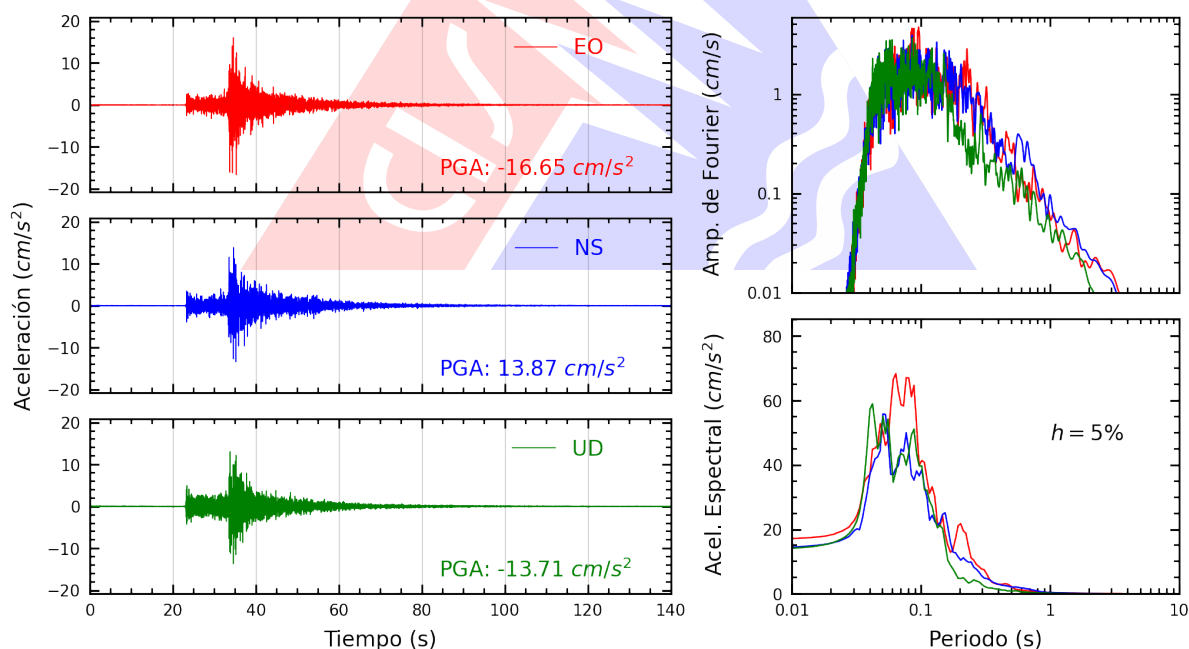
Figura A.28: Registros tiempo-historia, espectros de Fourier y de respuesta en las direcciones EO, NS y vertical de la estación ASIA. Sismo de Chilca, Cañete - Lima del 2026-02-26, 18:21:08 (Hora local)
