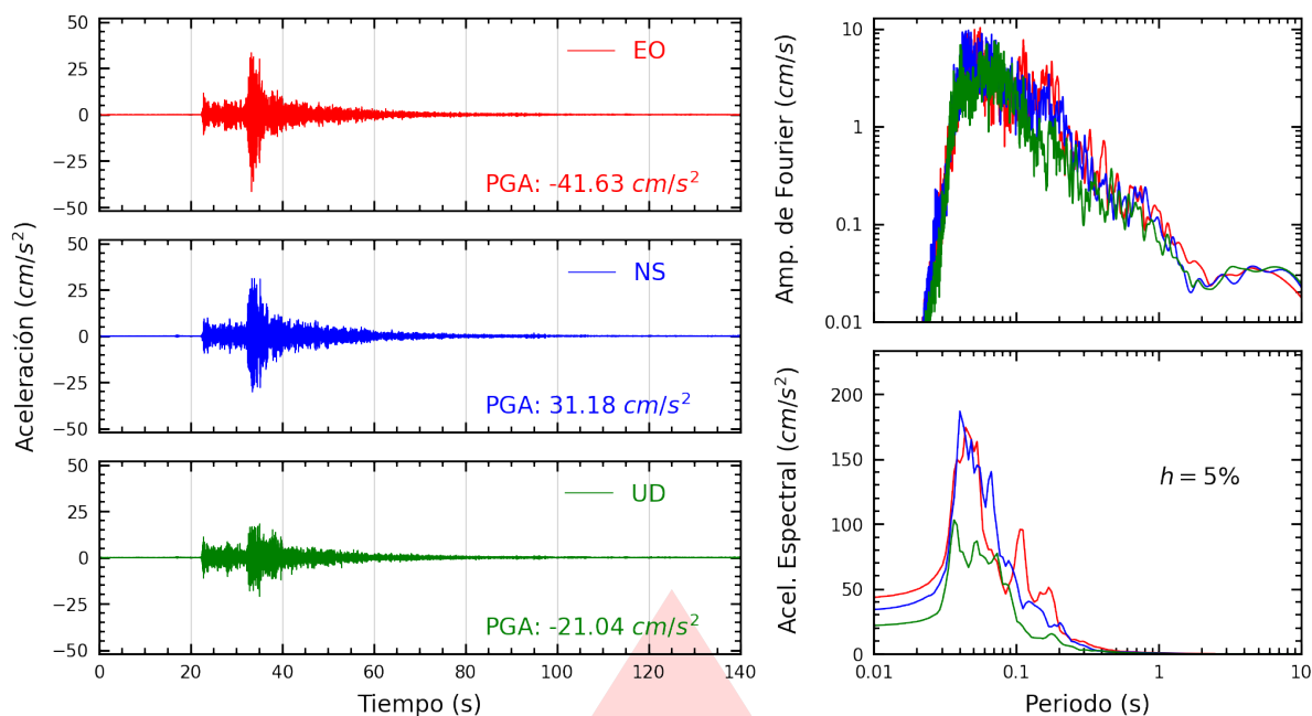
Figura A.5: Registros tiempo-historia, espectros de Fourier y de respuesta en las direcciones EO, NS y vertical de la estación SROSA. Sismo de Chilca, Cañete - Lima del 2026-02-26, 18:21:08 (Hora local)
