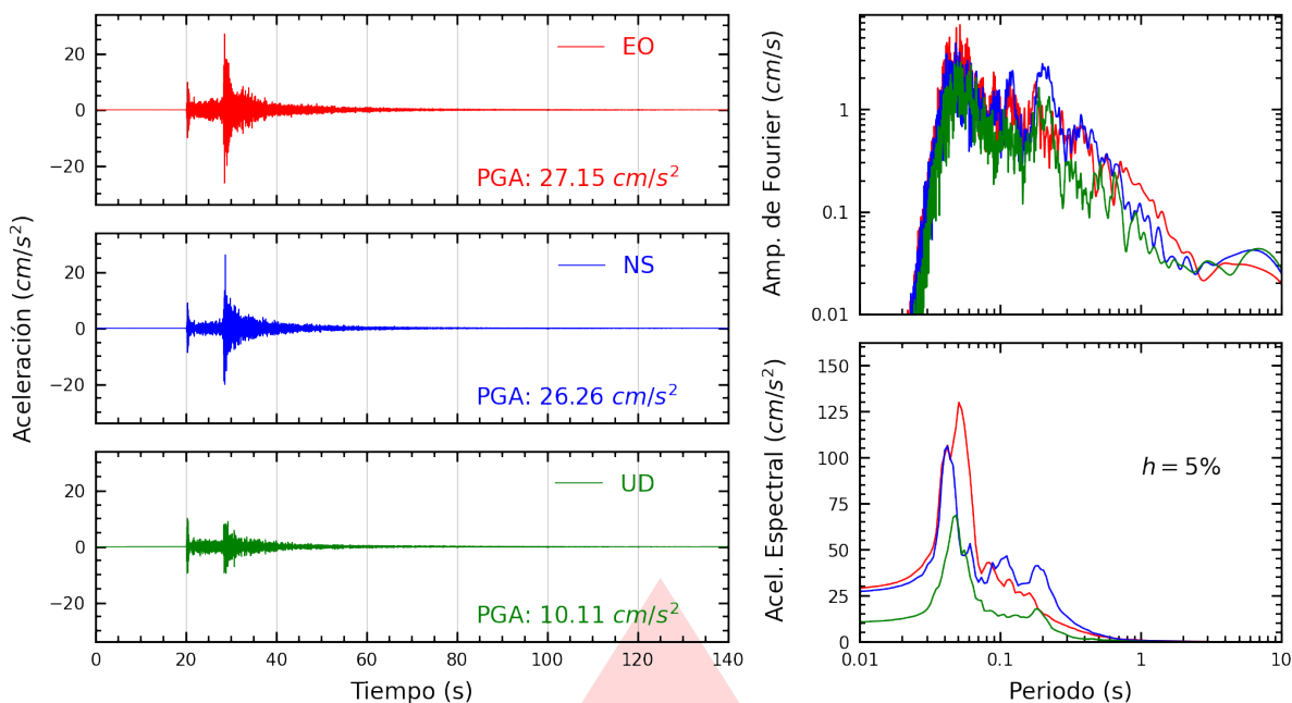
Figura A.13: Registros tiempo-historia, espectros de Fourier y de respuesta en las direcciones EO, NS y vertical de la estación UCSS. Sismo de Chilca, Cañete - Lima del 2026-02-26, 18:21:08 (Hora local)
