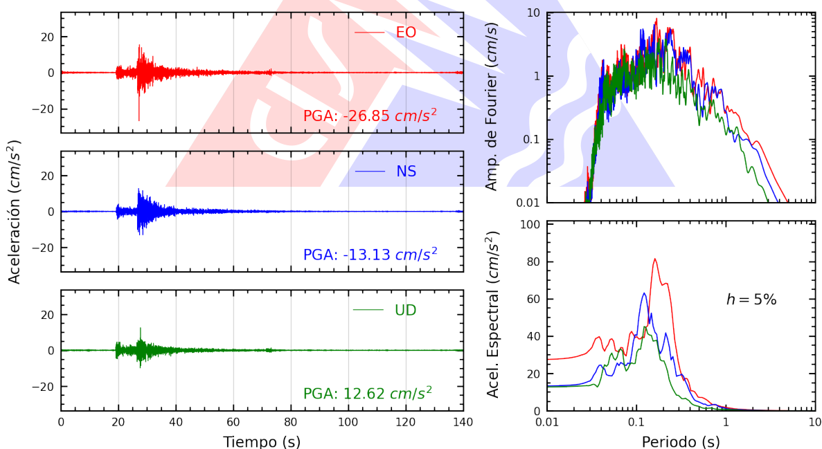
Figura A.14: Registros tiempo-historia, espectros de Fourier y de respuesta en las direcciones EO, NS y vertical de la estación SOBAR. Sismo de Chilca, Cañete - Lima del 2026-02-26, 18:21:08 (Hora local)
