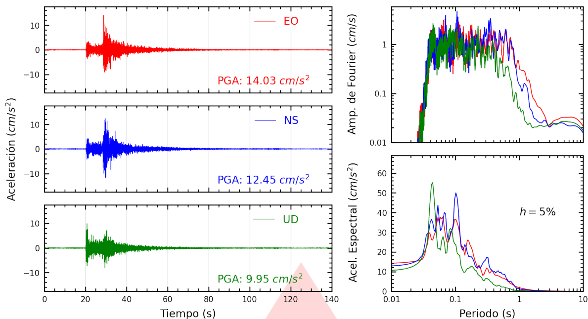
Figura A.33: Registros tiempo-historia, espectros de Fourier y de respuesta en las direcciones EO, NS y vertical de la estación MADRE. Sismo de Chilca, Cañete - Lima del 2026-02-26, 18:21:08 (Hora local)
