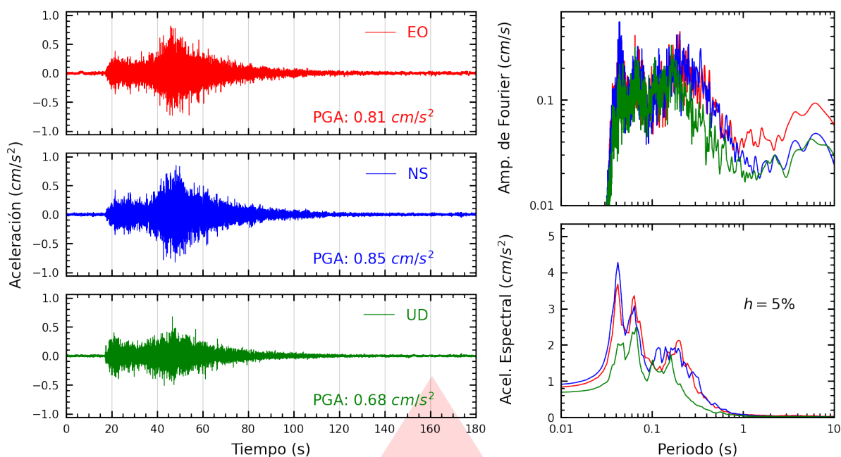
Figura A.43: Registros tiempo-historia, espectros de Fourier y de respuesta en las direcciones EO, NS y vertical de la estación UNAB. Sismo de Chilca, Cañete - Lima del 2026-02-26, 18:21:08 (Hora local)
