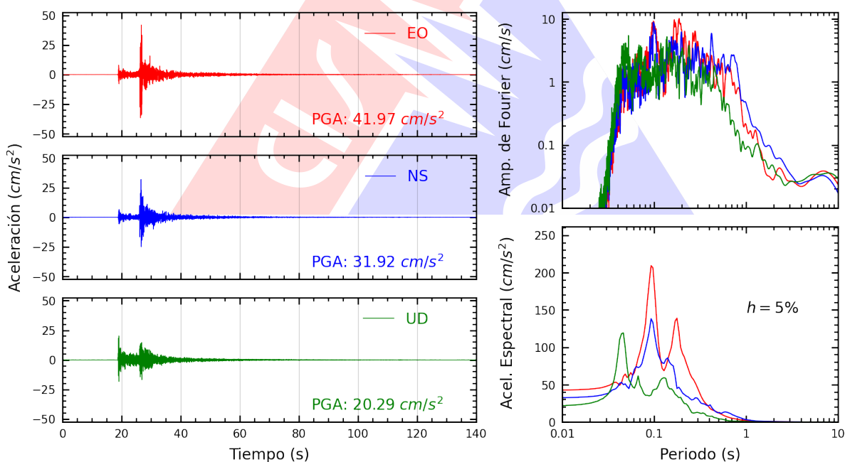
Figura A.4: Registros tiempo-historia, espectros de Fourier y de respuesta en las direcciones EO, NS y vertical de la estación USILP. Sismo de Chilca, Cañete - Lima del 2026-02-26, 18:21:08 (Hora local)
