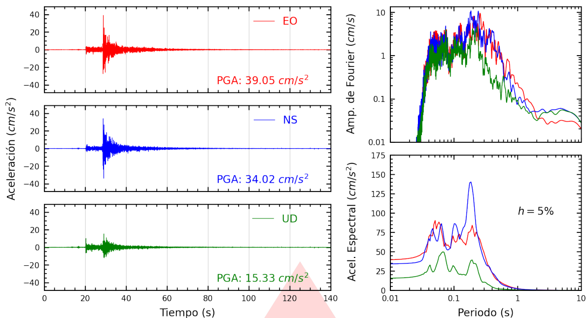
Figura A.7: Registros tiempo-historia, espectros de Fourier y de respuesta en las direcciones EO, NS y vertical de la estación SCOLI. Sismo de Chilca, Cañete - Lima del 2026-02-26, 18:21:08 (Hora local)
