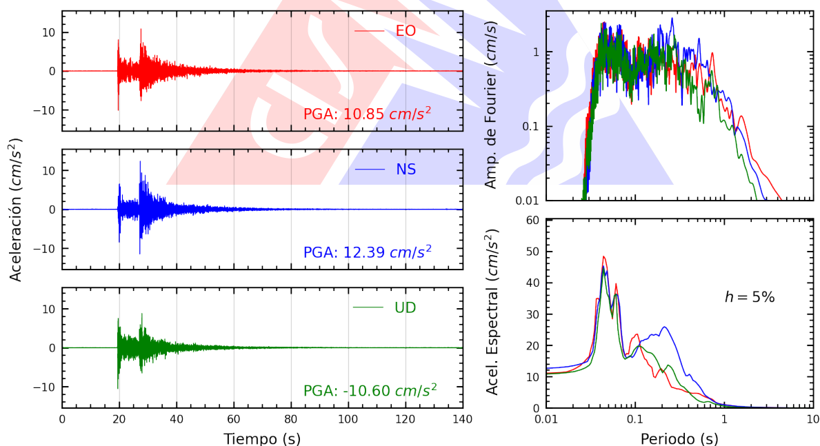
Figura A.36: Registros tiempo-historia, espectros de Fourier y de respuesta en las direcciones EO, NS y vertical de la estación BORJA. Sismo de Chilca, Cañete - Lima del 2026-02-26, 18:21:08 (Hora local)
