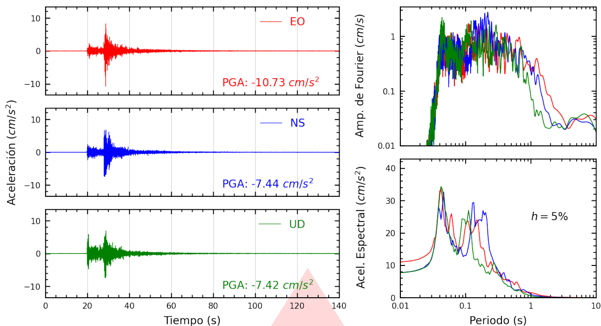
Figura A.39: Registros tiempo-historia, espectros de Fourier y de respuesta en las direcciones EO, NS y vertical de la estación BONDY. Sismo de Chilca, Cañete - Lima del 2026-02-26, 18:21:08 (Hora local)
