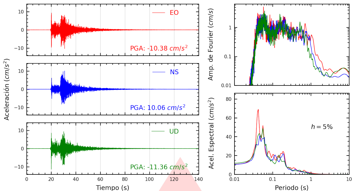
Figura A.37: Registros tiempo-historia, espectros de Fourier y de respuesta en las direcciones EO, NS y vertical de la estación IMCA. Sismo de Chilca, Cañete - Lima del 2026-02-26, 18:21:08 (Hora local)
