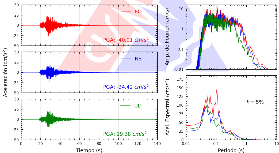
Figura A.6: Registros tiempo-historia, espectros de Fourier y de respuesta en las direcciones EO, NS y vertical de la estación UNTEL. Sismo de Chilca, Cañete - Lima del 2026-02-26, 18:21:08 (Hora local)
