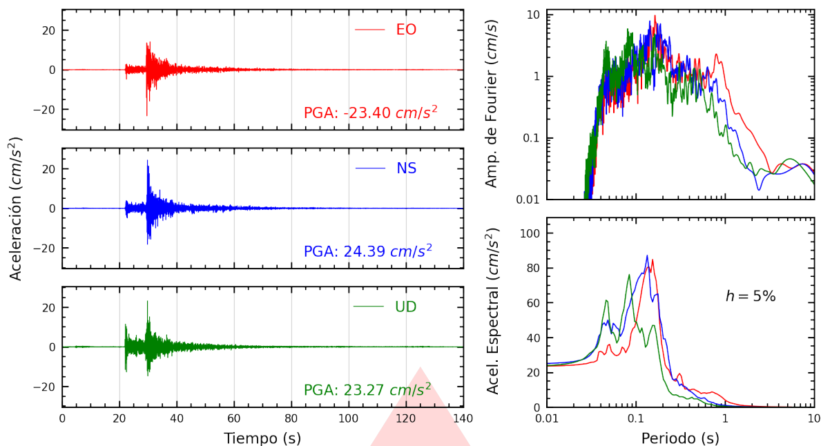
Figura A.17: Registros tiempo-historia, espectros de Fourier y de respuesta en las direcciones EO, NS y vertical de la estación SOCHO. Sismo de Chilca, Cañete - Lima del 2026-02-26, 18:21:08 (Hora local)
