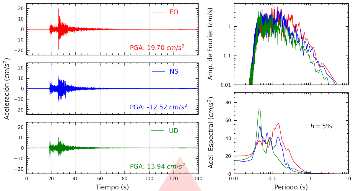
Figura A.23: Registros tiempo-historia, espectros de Fourier y de respuesta en las direcciones EO, NS y vertical de la estación PACHA. Sismo de Chilca, Cañete - Lima del 2026-02-26, 18:21:08 (Hora local)
