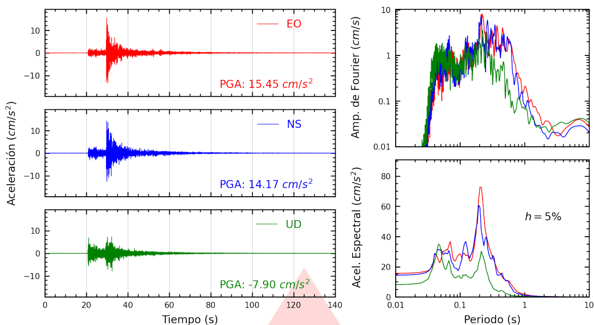
Figura A.31: Registros tiempo-historia, espectros de Fourier y de respuesta en las direcciones EO, NS y vertical de la estación VHAYA. Sismo de Chilca, Cañete - Lima del 2026-02-26, 18:21:08 (Hora local)
