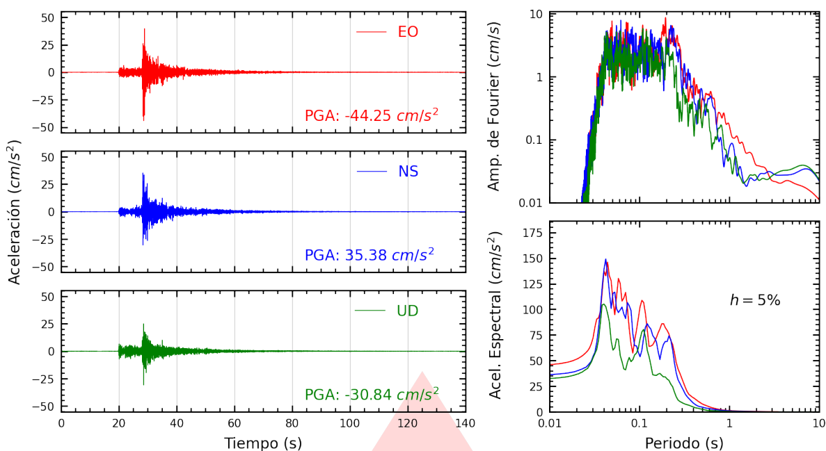
Figura A.3: Registros tiempo-historia, espectros de Fourier y de respuesta en las direcciones EO, NS y vertical de la estación INDEP. Sismo de Chilca, Cañete - Lima del 2026-02-26, 18:21:08 (Hora local)
