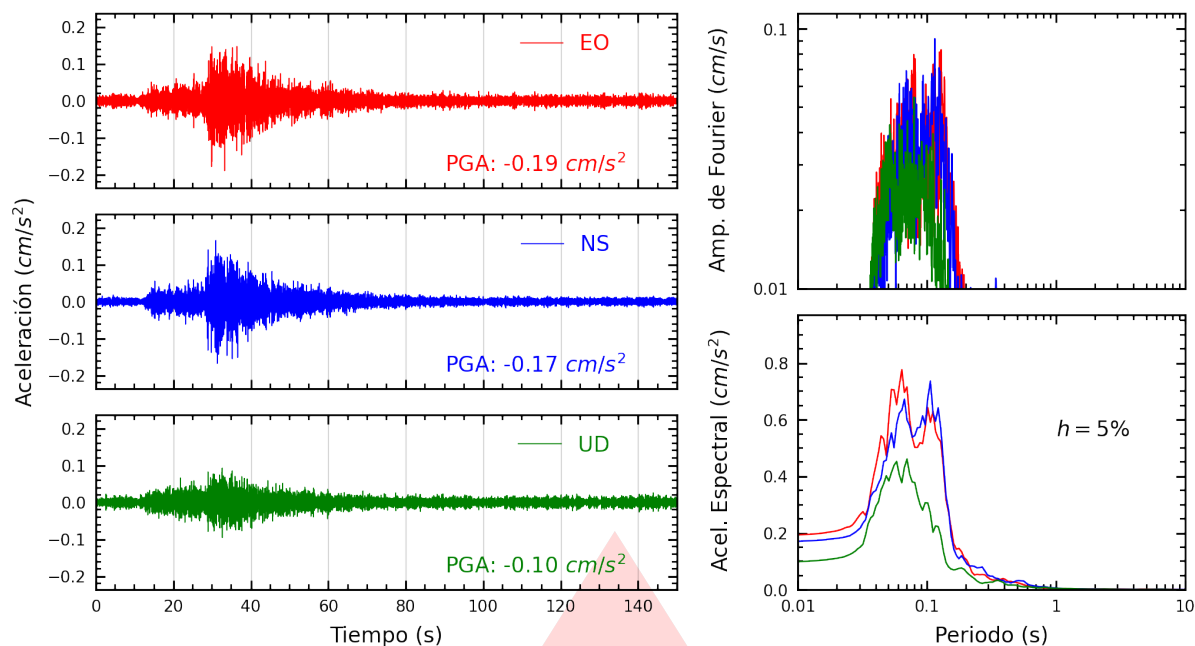
Figura A.21: Registros tiempo-historia, espectros de Fourier y de respuesta en las direcciones EO, NS y vertical de la estación ATARJ. Sismo de Huacho, Huaura - Lima del 2026-02-27, 03:30:39 (Hora local)
