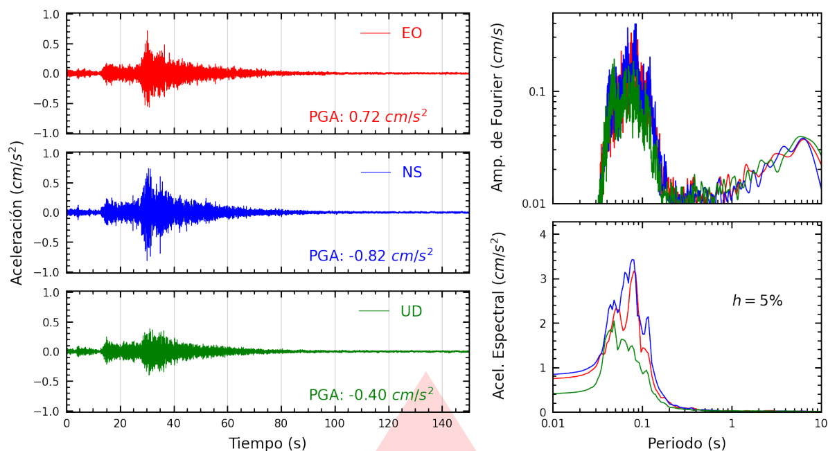
Figura A.3: Registros tiempo-historia, espectros de Fourier y de respuesta en las direcciones EO, NS y vertical de la estación JOSEO. Sismo de Huacho, Huaura - Lima del 2026-02-27, 03:30:39 (Hora local)
