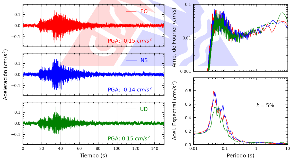
Figura A.24: Registros tiempo-historia, espectros de Fourier y de respuesta en las direcciones EO, NS y vertical de la estación UCSS. Sismo de Huacho, Huaura - Lima del 2026-02-27, 03:30:39 (Hora local)
