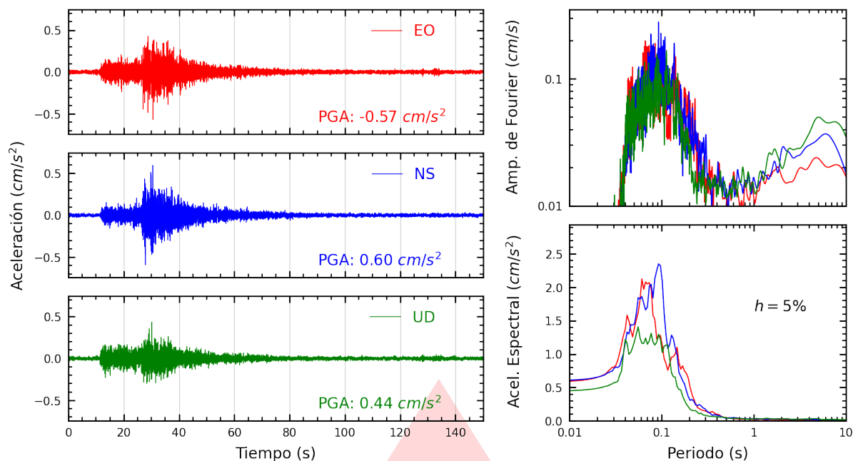
Figura A.7: Registros tiempo-historia, espectros de Fourier y de respuesta en las direcciones EO, NS y vertical de la estación INDEP. Sismo de Huacho, Huaura - Lima del 2026-02-27, 03:30:39 (Hora local)
