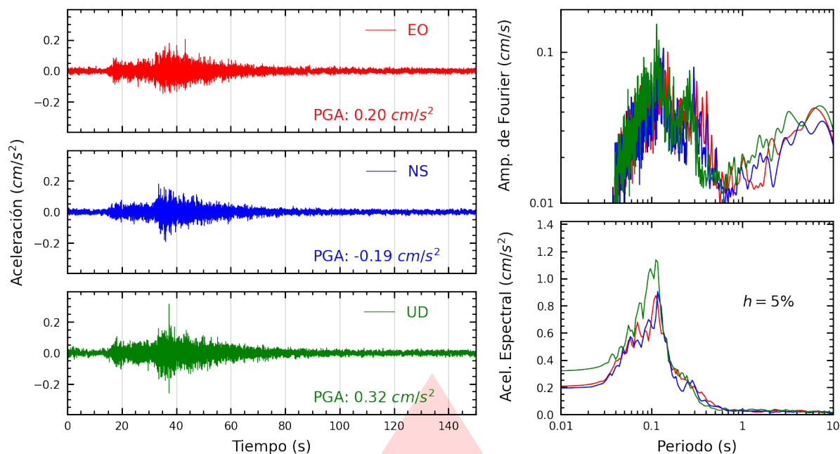
Figura A.15: Registros tiempo-historia, espectros de Fourier y de respuesta en las direcciones EO, NS y vertical de la estación SOVES. Sismo de Huacho, Huaura - Lima del 2026-02-27, 03:30:39 (Hora local)
