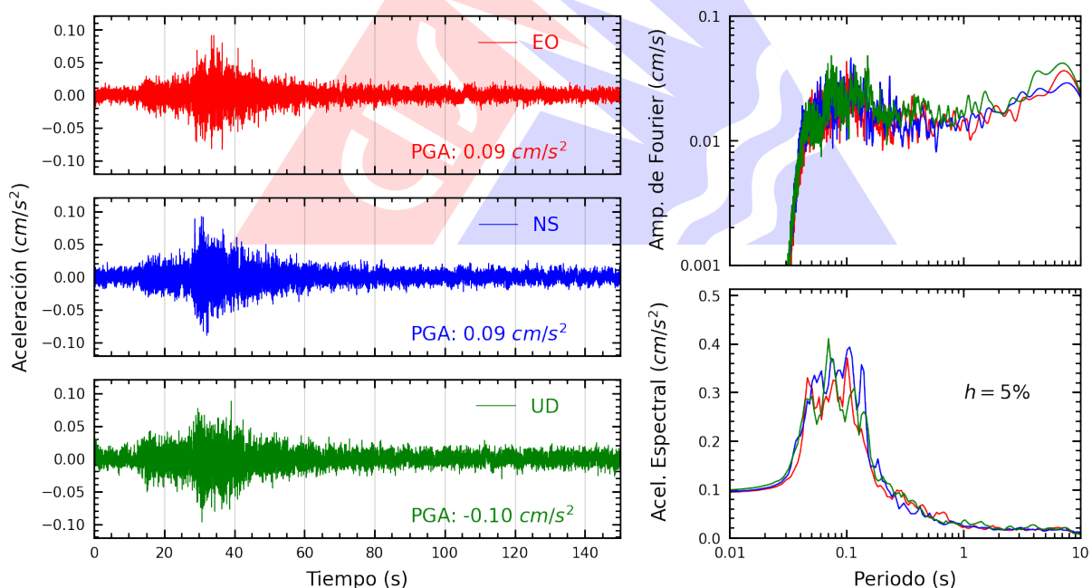
Figura A.28: Registros tiempo-historia, espectros de Fourier y de respuesta en las direcciones EO, NS y vertical de la estación UNFV. Sismo de Huacho, Huaura - Lima del 2026-02-27, 03:30:39 (Hora local)
