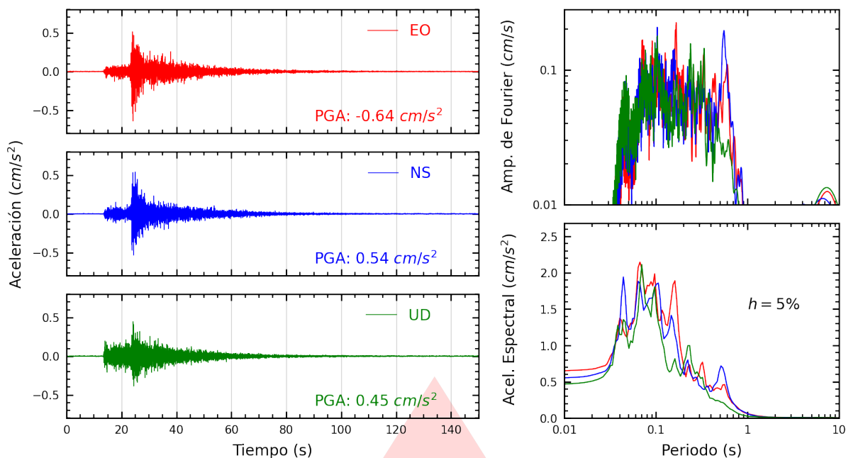
Figura A.5: Registros tiempo-historia, espectros de Fourier y de respuesta en las direcciones EO, NS y vertical de la estación CARAL. Sismo de Huacho, Huaura - Lima del 2026-02-27, 03:30:39 (Hora local)
