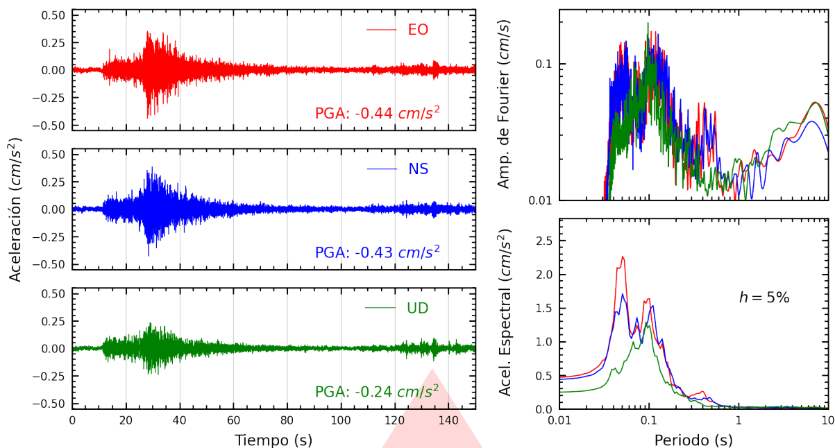
Figura A.9: Registros tiempo-historia, espectros de Fourier y de respuesta en las direcciones EO, NS y vertical de la estación OLIVO. Sismo de Huacho, Huaura - Lima del 2026-02-27, 03:30:39 (Hora local)
