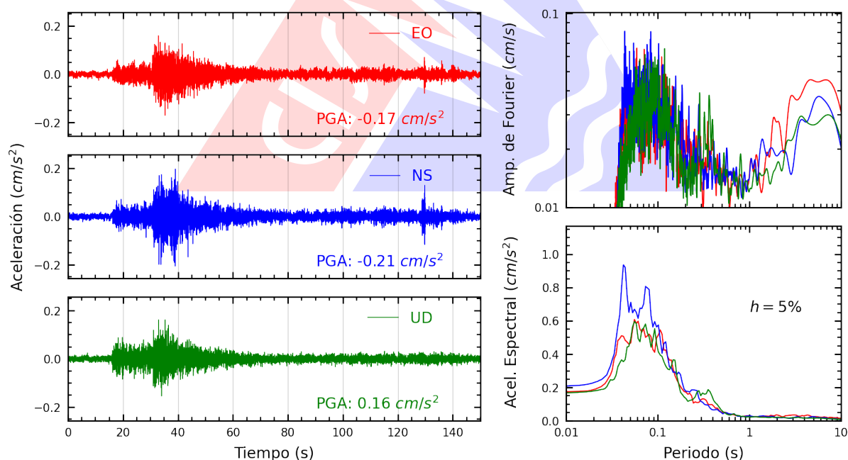
Figura A.20: Registros tiempo-historia, espectros de Fourier y de respuesta en las direcciones EO, NS y vertical de la estación COMAS. Sismo de Huacho, Huaura - Lima del 2026-02-27, 03:30:39 (Hora local)
