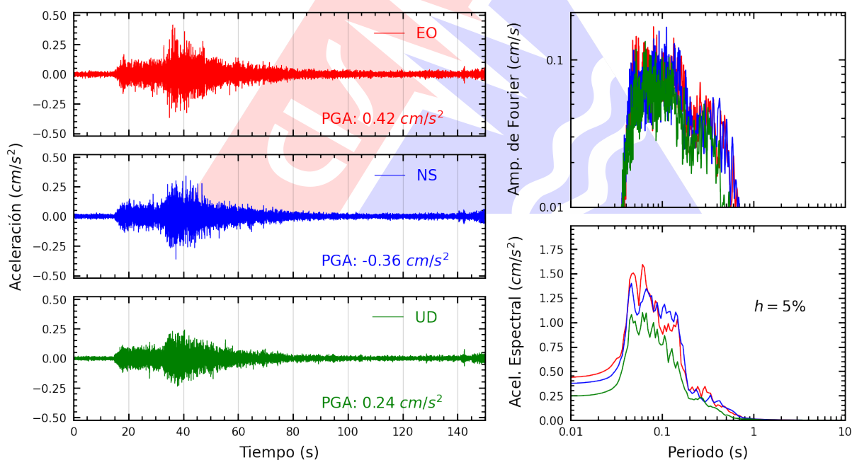
Figura A.10: Registros tiempo-historia, espectros de Fourier y de respuesta en las direcciones EO, NS y vertical de la estación UNTEL. Sismo de Huacho, Huaura - Lima del 2026-02-27, 03:30:39 (Hora local)
