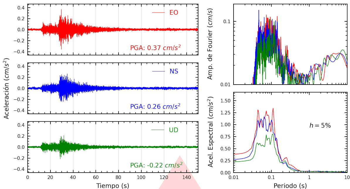
Figura A.13: Registros tiempo-historia, espectros de Fourier y de respuesta en las direcciones EO, NS y vertical de la estación FICPE. Sismo de Huacho, Huaura - Lima del 2026-02-27, 03:30:39 (Hora local)
