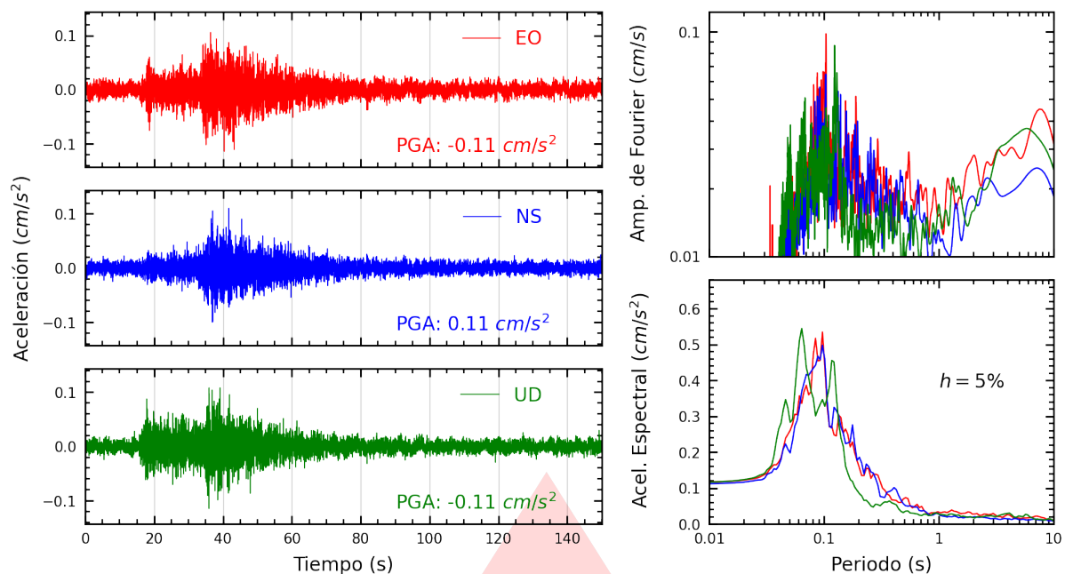
Figura A.27: Registros tiempo-historia, espectros de Fourier y de respuesta en las direcciones EO, NS y vertical de la estación USILP. Sismo de Huacho, Huaura - Lima del 2026-02-27, 03:30:39 (Hora local)
