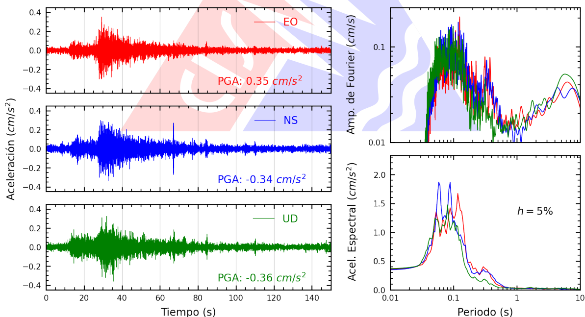
Figura A.14: Registros tiempo-historia, espectros de Fourier y de respuesta en las direcciones EO, NS y vertical de la estación SJLSC. Sismo de Huacho, Huaura - Lima del 2026-02-27, 03:30:39 (Hora local)
