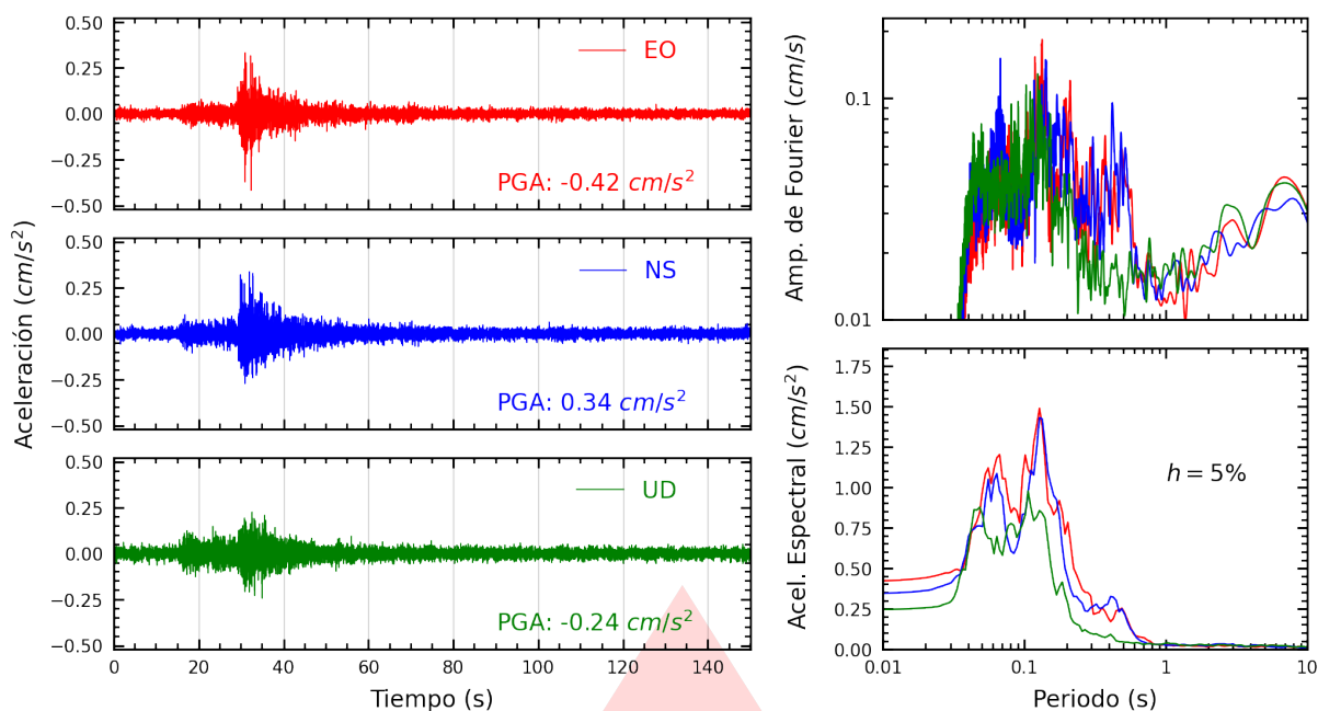
Figura A.11: Registros tiempo-historia, espectros de Fourier y de respuesta en las direcciones EO, NS y vertical de la estación VHAYA. Sismo de Huacho, Huaura - Lima del 2026-02-27, 03:30:39 (Hora local)
