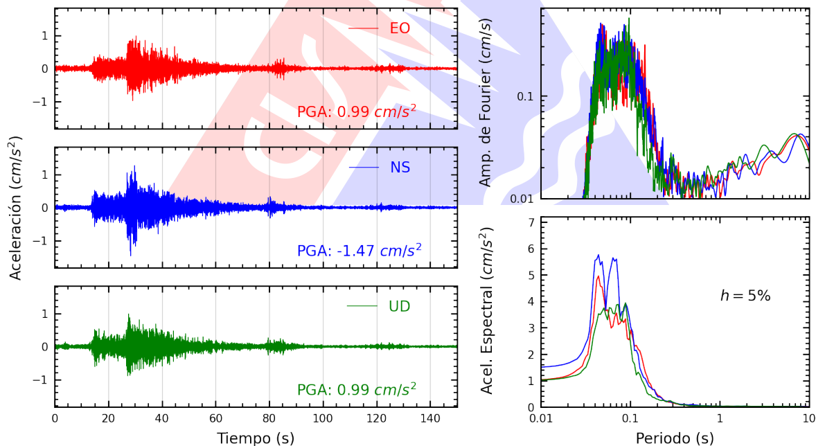
Figura A.2: Registros tiempo-historia, espectros de Fourier y de respuesta en las direcciones EO, NS y vertical de la estación SROSA. Sismo de Huacho, Huaura - Lima del 2026-02-27, 03:30:39 (Hora local)
