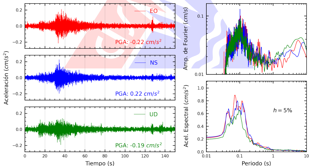
Figura A.16: Registros tiempo-historia, espectros de Fourier y de respuesta en las direcciones EO, NS y vertical de la estación UCVAT. Sismo de Huacho, Huaura - Lima del 2026-02-27, 03:30:39 (Hora local)
