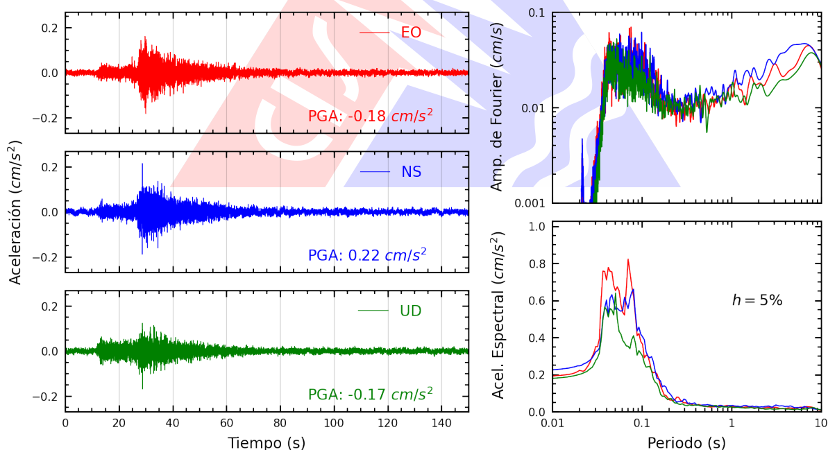
Figura A.18: Registros tiempo-historia, espectros de Fourier y de respuesta en las direcciones EO, NS y vertical de la estación SJLCE. Sismo de Huacho, Huaura - Lima del 2026-02-27, 03:30:39 (Hora local)
