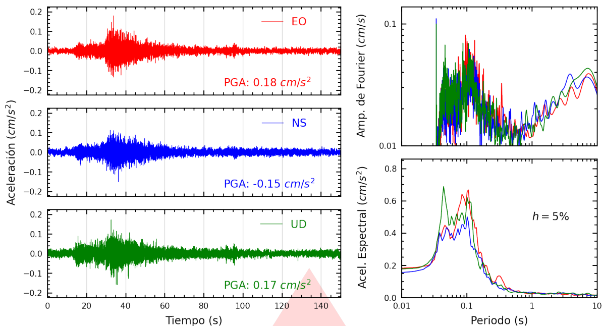
Figura A.23: Registros tiempo-historia, espectros de Fourier y de respuesta en las direcciones EO, NS y vertical de la estación USMP. Sismo de Huacho, Huaura - Lima del 2026-02-27, 03:30:39 (Hora local)
