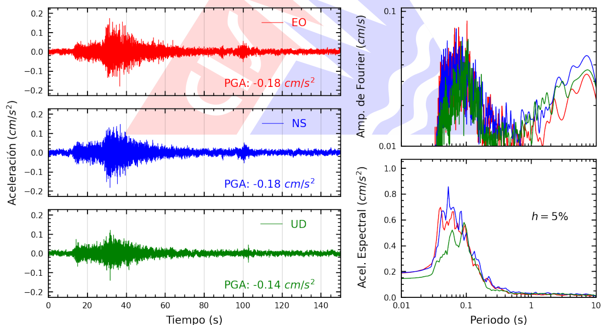
Figura A.22: Registros tiempo-historia, espectros de Fourier y de respuesta en las direcciones EO, NS y vertical de la estación CEPRE. Sismo de Huacho, Huaura - Lima del 2026-02-27, 03:30:39 (Hora local)
