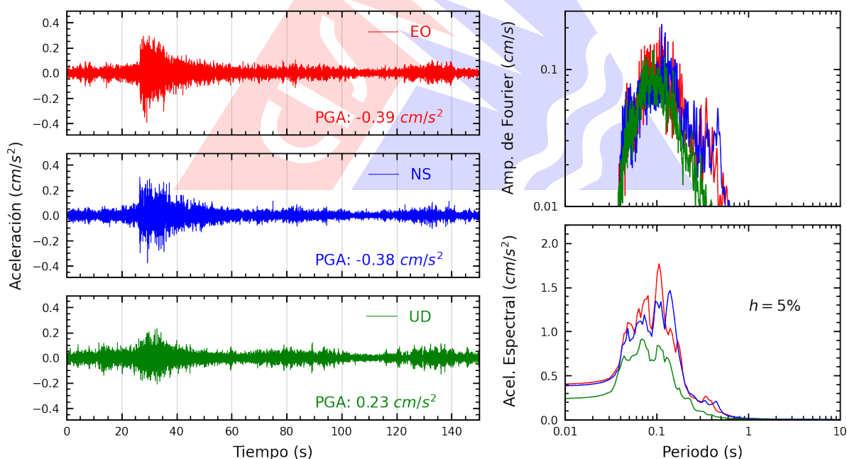
Figura A.12: Registros tiempo-historia, espectros de Fourier y de respuesta en las direcciones EO, NS y vertical de la estación SCOLI. Sismo de Huacho, Huaura - Lima del 2026-02-27, 03:30:39 (Hora local)
