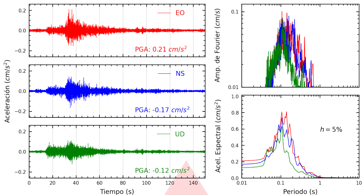
Figura A.19: Registros tiempo-historia, espectros de Fourier y de respuesta en las direcciones EO, NS y vertical de la estación SCCHO. Sismo de Huacho, Huaura - Lima del 2026-02-27, 03:30:39 (Hora local)
