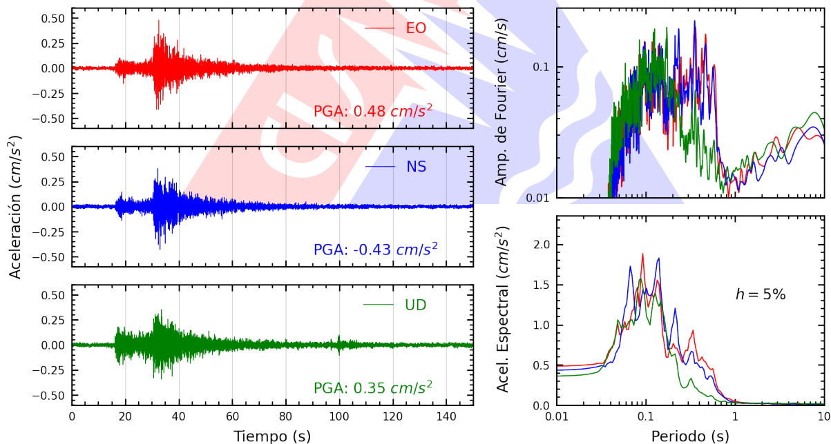
Figura A.8: Registros tiempo-historia, espectros de Fourier y de respuesta en las direcciones EO, NS y vertical de la estación MDPP. Sismo de Huacho, Huaura - Lima del 2026-02-27, 03:30:39 (Hora local)
