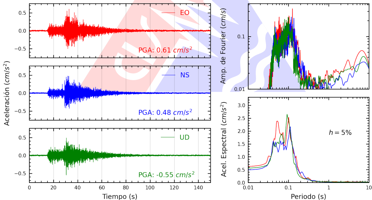
Figura A.6: Registros tiempo-historia, espectros de Fourier y de respuesta en las direcciones EO, NS y vertical de la estación AMORE. Sismo de Huacho, Huaura - Lima del 2026-02-27, 03:30:39 (Hora local)
