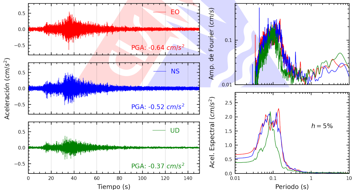
Figura A.4: Registros tiempo-historia, espectros de Fourier y de respuesta en las direcciones EO, NS y vertical de la estación USILM. Sismo de Huacho, Huaura - Lima del 2026-02-27, 03:30:39 (Hora local)
