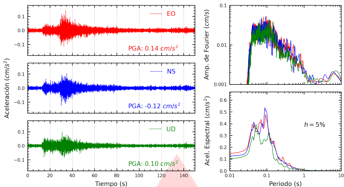
Figura A.25: Registros tiempo-historia, espectros de Fourier y de respuesta en las direcciones EO, NS y vertical de la estación BORJA. Sismo de Huacho, Huaura - Lima del 2026-02-27, 03:30:39 (Hora local)
