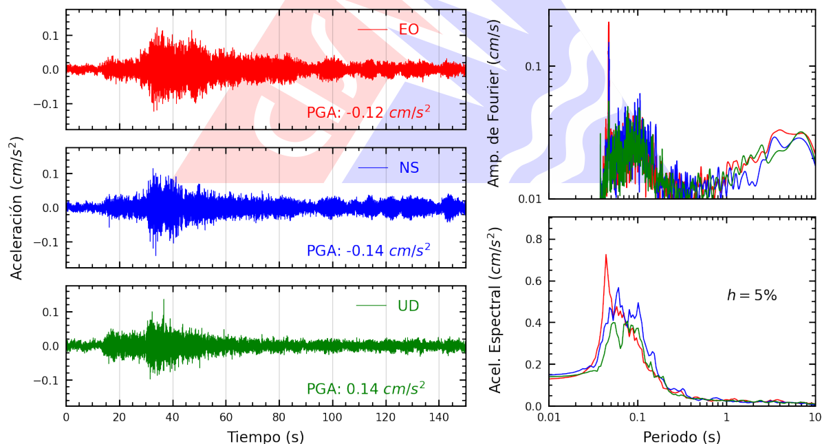
Figura A.26: Registros tiempo-historia, espectros de Fourier y de respuesta en las direcciones EO, NS y vertical de la estación SERVI. Sismo de Huacho, Huaura - Lima del 2026-02-27, 03:30:39 (Hora local)
