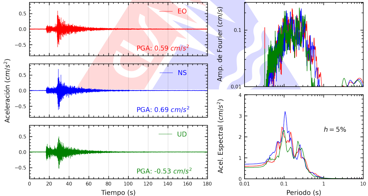
Figura A.6: Registros tiempo-historia, espectros de Fourier y de respuesta en las direcciones EO, NS y vertical de la estación CARAL. Sismo de Huacho, Huaura - Lima del 2026-01-31, 16:28:11 (Hora local)
