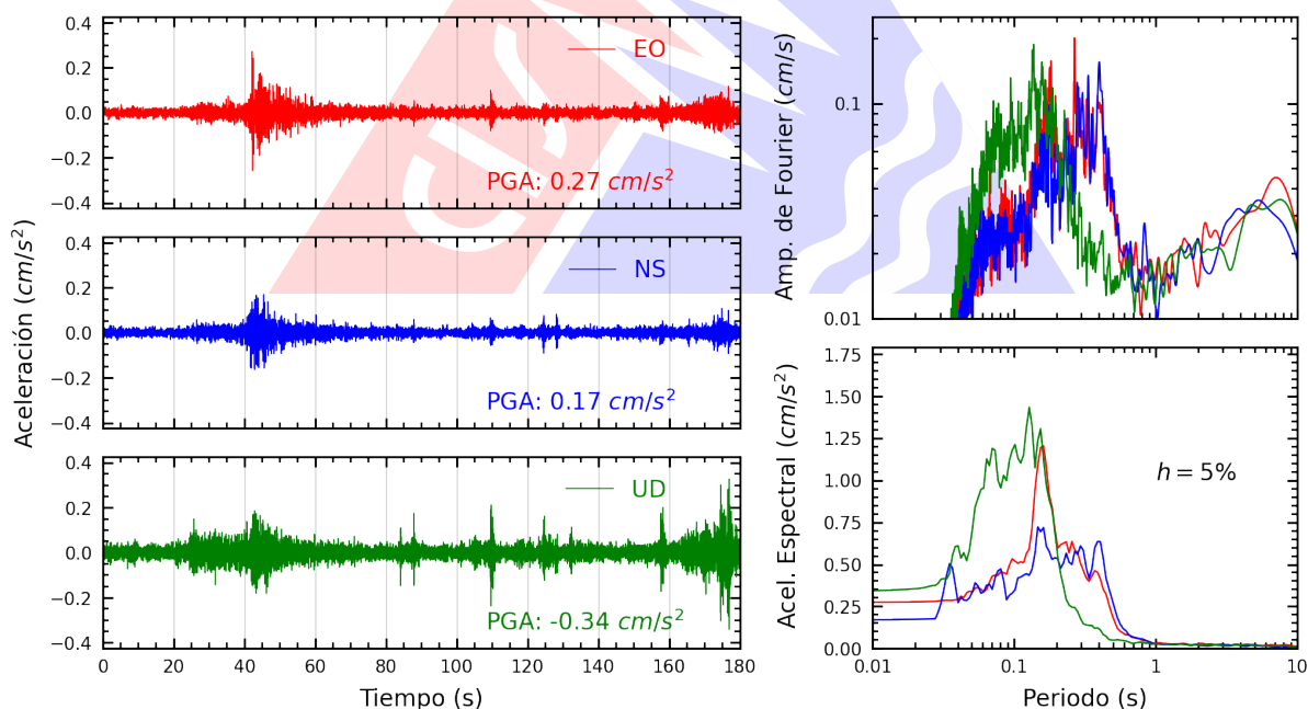
Figura A.12: Registros tiempo-historia, espectros de Fourier y de respuesta en las direcciones EO, NS y vertical de la estación ACAPU. Sismo de Huacho, Huaura - Lima del 2026-01-31, 16:28:11 (Hora local)
