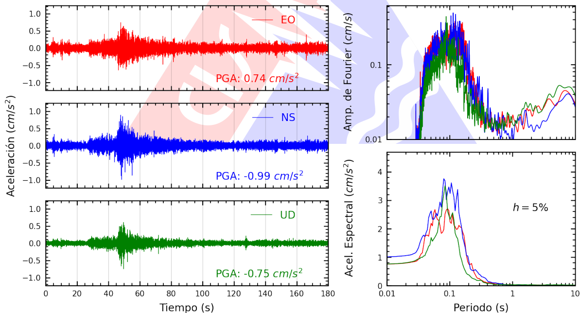
Figura A.4: Registros tiempo-historia, espectros de Fourier y de respuesta en las direcciones EO, NS y vertical de la estación USILM. Sismo de Huacho, Huaura - Lima del 2026-01-31, 16:28:11 (Hora local)
