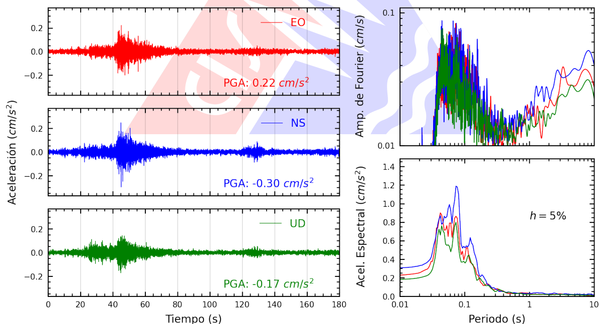
Figura A.14: Registros tiempo-historia, espectros de Fourier y de respuesta en las direcciones EO, NS y vertical de la estación SJLCE. Sismo de Huacho, Huaura - Lima del 2026-01-31, 16:28:11 (Hora local)
