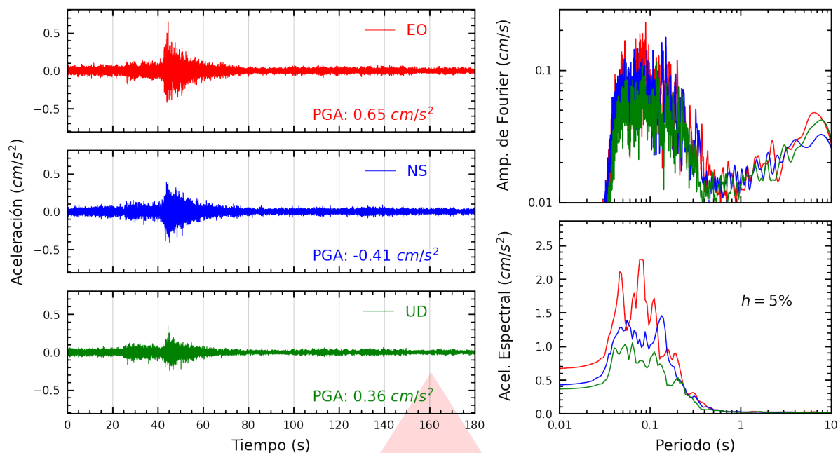
Figura A.7: Registros tiempo-historia, espectros de Fourier y de respuesta en las direcciones EO, NS y vertical de la estación FICPE. Sismo de Huacho, Huaura - Lima del 2026-01-31, 16:28:11 (Hora local)
