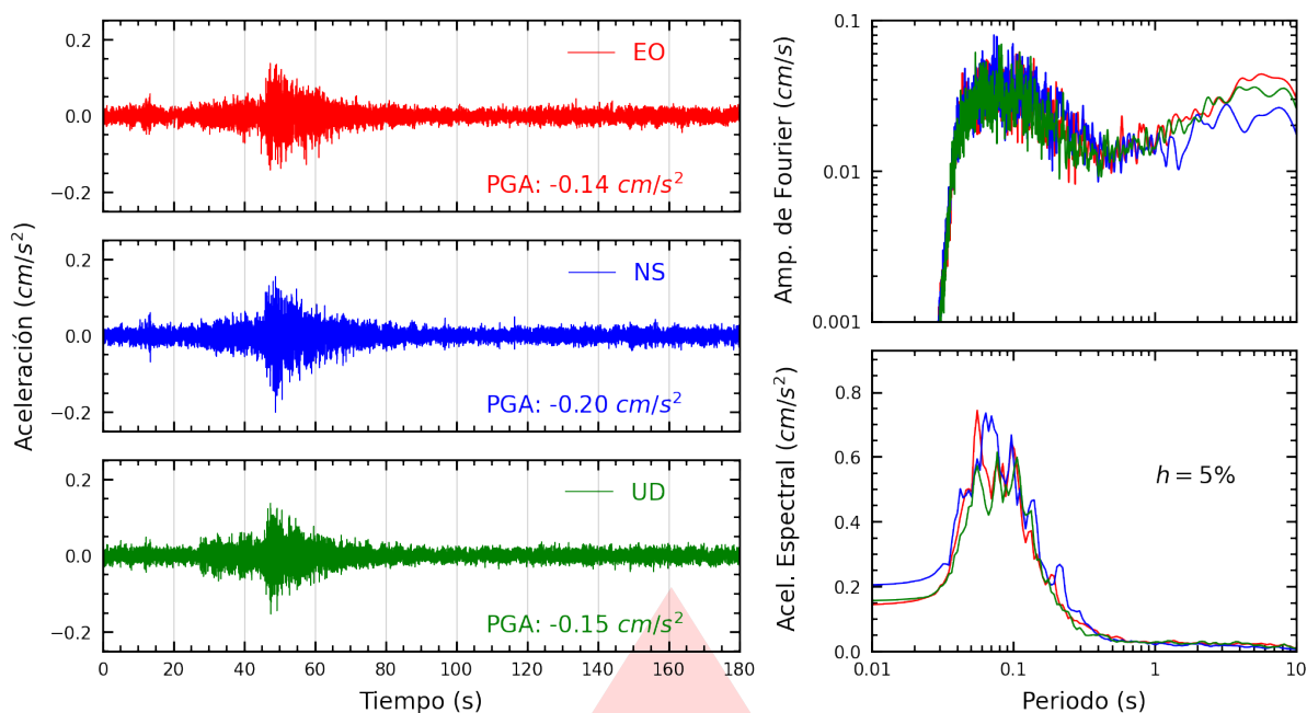
Figura A.19: Registros tiempo-historia, espectros de Fourier y de respuesta en las direcciones EO, NS y vertical de la estación SERVI. Sismo de Huacho, Huaura - Lima del 2026-01-31, 16:28:11 (Hora local)
