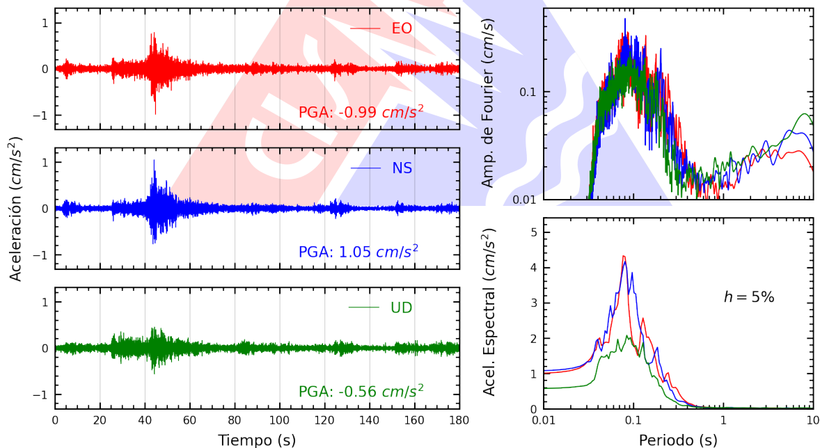
Figura A.2: Registros tiempo-historia, espectros de Fourier y de respuesta en las direcciones EO, NS y vertical de la estación INDEP. Sismo de Huacho, Huaura - Lima del 2026-01-31, 16:28:11 (Hora local)
