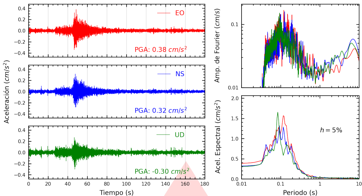
Figura A.11: Registros tiempo-historia, espectros de Fourier y de respuesta en las direcciones EO, NS y vertical de la estación UCVAT. Sismo de Huacho, Huaura - Lima del 2026-01-31, 16:28:11 (Hora local)
