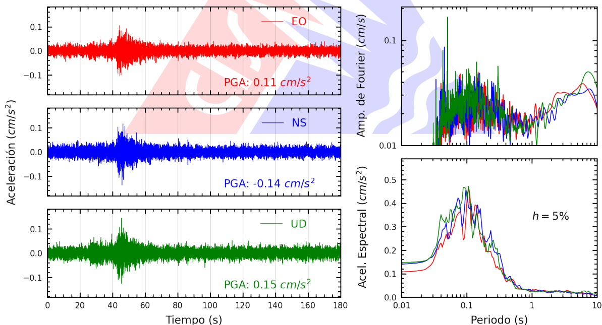
Figura A.22: Registros tiempo-historia, espectros de Fourier y de respuesta en las direcciones EO, NS y vertical de la estación BONDY. Sismo de Huacho, Huaura - Lima del 2026-01-31, 16:28:11 (Hora local)
