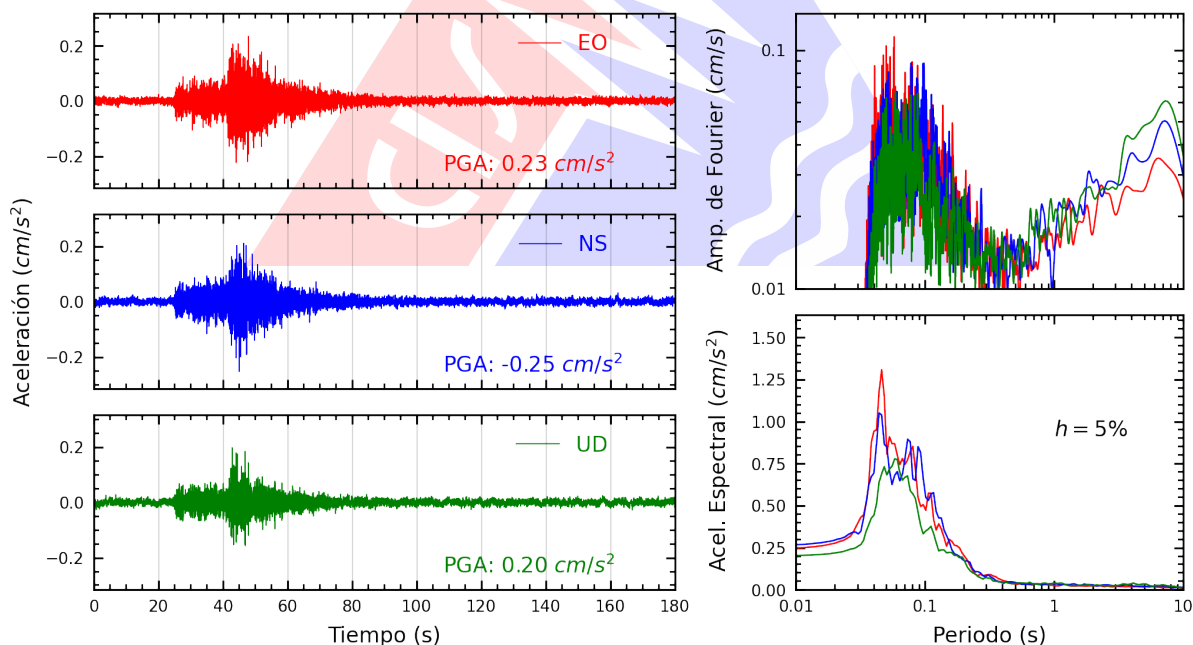
Figura A.16: Registros tiempo-historia, espectros de Fourier y de respuesta en las direcciones EO, NS y vertical de la estación UCSS. Sismo de Huacho, Huaura - Lima del 2026-01-31, 16:28:11 (Hora local)
