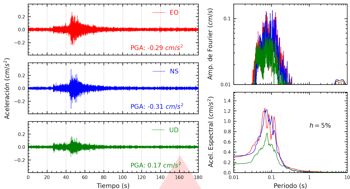
Figura A.13: Registros tiempo-historia, espectros de Fourier y de respuesta en las direcciones EO, NS y vertical de la estación ATARJ. Sismo de Huacho, Huaura - Lima del 2026-01-31, 16:28:11 (Hora local)
