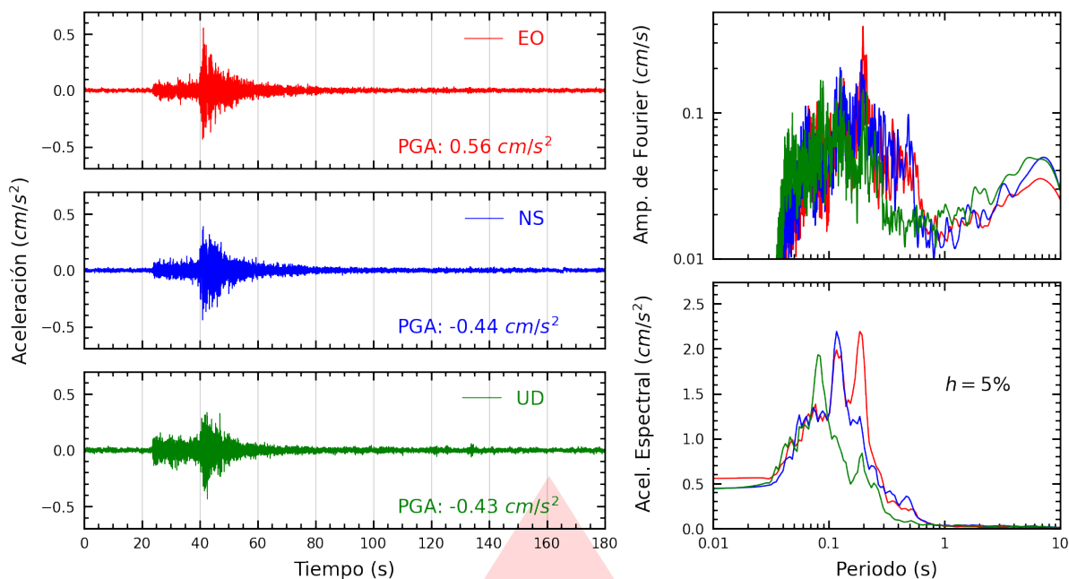
Figura A.9: Registros tiempo-historia, espectros de Fourier y de respuesta en las direcciones EO, NS y vertical de la estación VHAYA. Sismo de Huacho, Huaura - Lima del 2026-01-31, 16:28:11 (Hora local)
