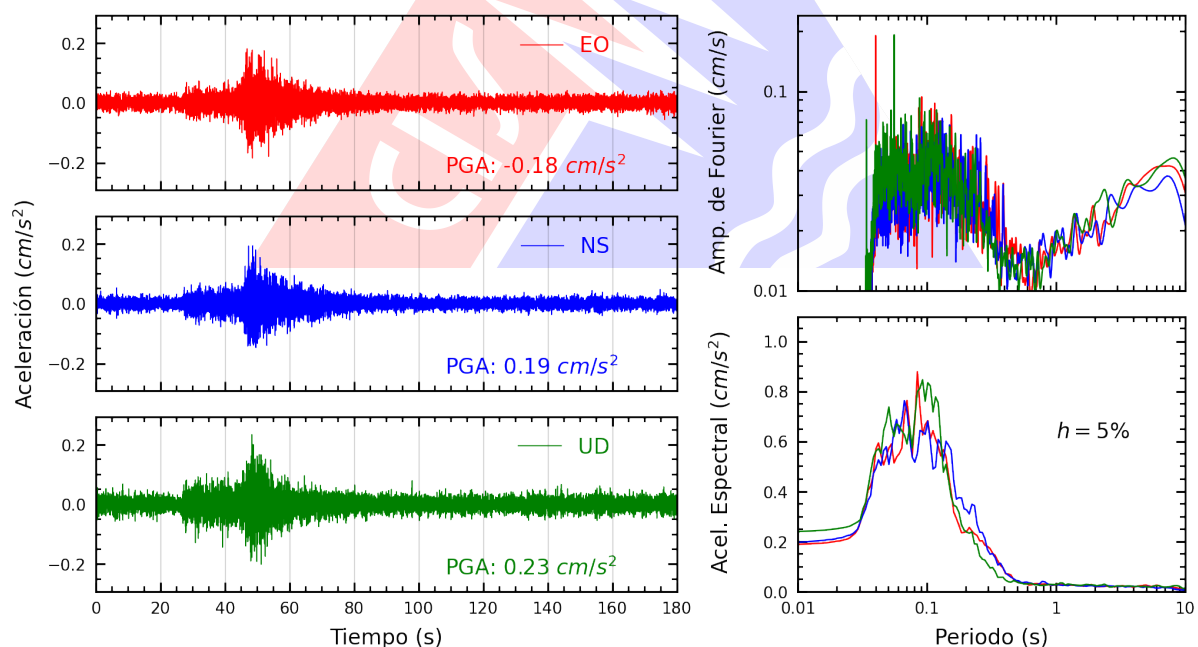
Figura A.18: Registros tiempo-historia, espectros de Fourier y de respuesta en las direcciones EO, NS y vertical de la estación USMP. Sismo de Huacho, Huaura - Lima del 2026-01-31, 16:28:11 (Hora local)
