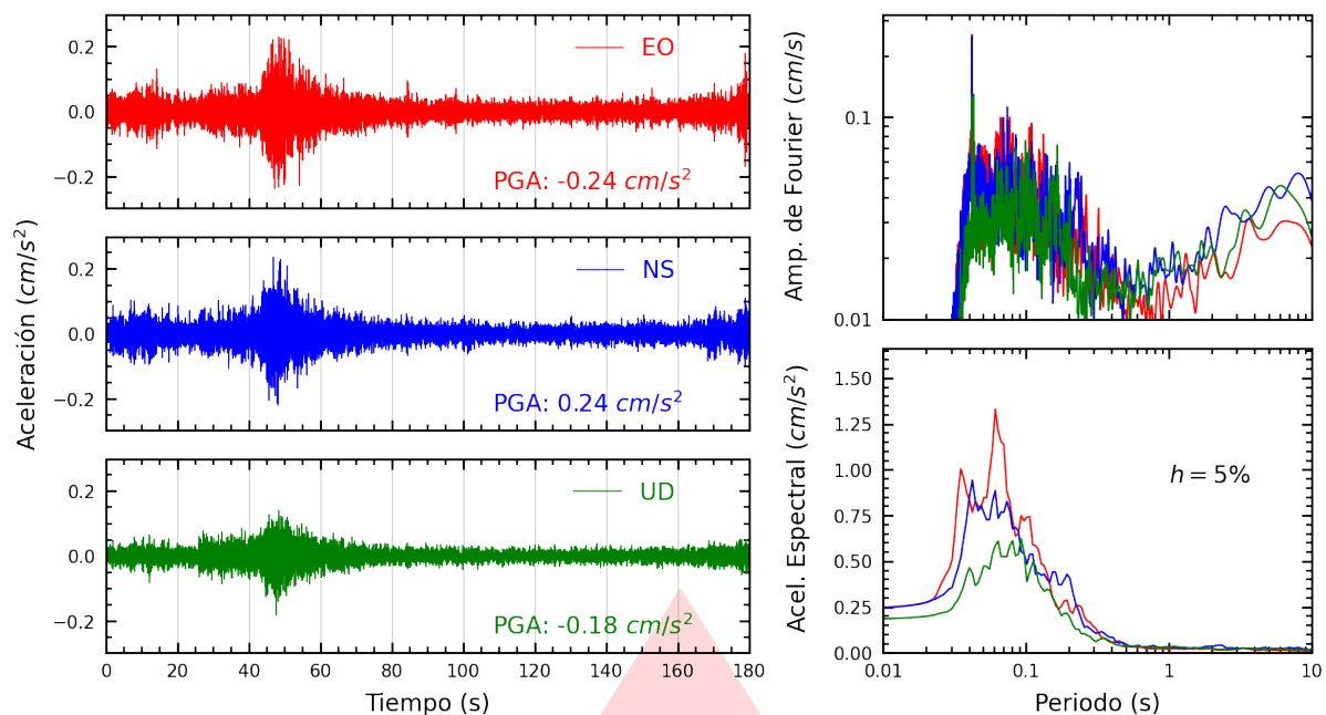
Figura A.17: Registros tiempo-historia, espectros de Fourier y de respuesta en las direcciones EO, NS y vertical de la estación CEPRE. Sismo de Huacho, Huaura - Lima del 2026-01-31, 16:28:11 (Hora local)
