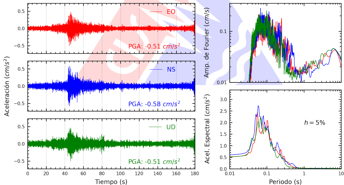
Figura A.8: Registros tiempo-historia, espectros de Fourier y de respuesta en las direcciones EO, NS y vertical de la estación SJLSC. Sismo de Huacho, Huaura - Lima del 2026-01-31, 16:28:11 (Hora local)
