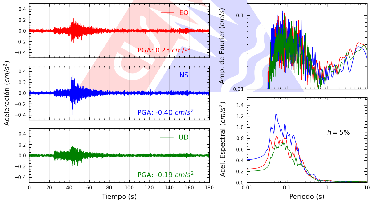
Figura A.10: Registros tiempo-historia, espectros de Fourier y de respuesta en las direcciones EO, NS y vertical de la estación COMAS. Sismo de Huacho, Huaura - Lima del 2026-01-31, 16:28:11 (Hora local)
