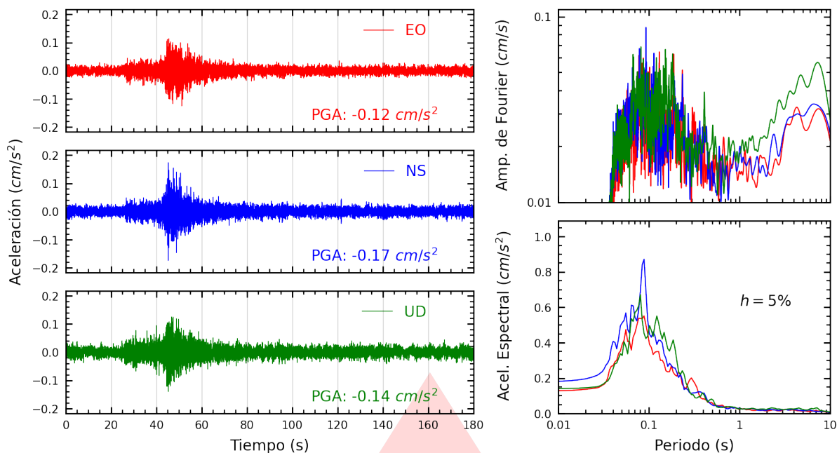
Figura A.21: Registros tiempo-historia, espectros de Fourier y de respuesta en las direcciones EO, NS y vertical de la estación UNFV. Sismo de Huacho, Huaura - Lima del 2026-01-31, 16:28:11 (Hora local)
