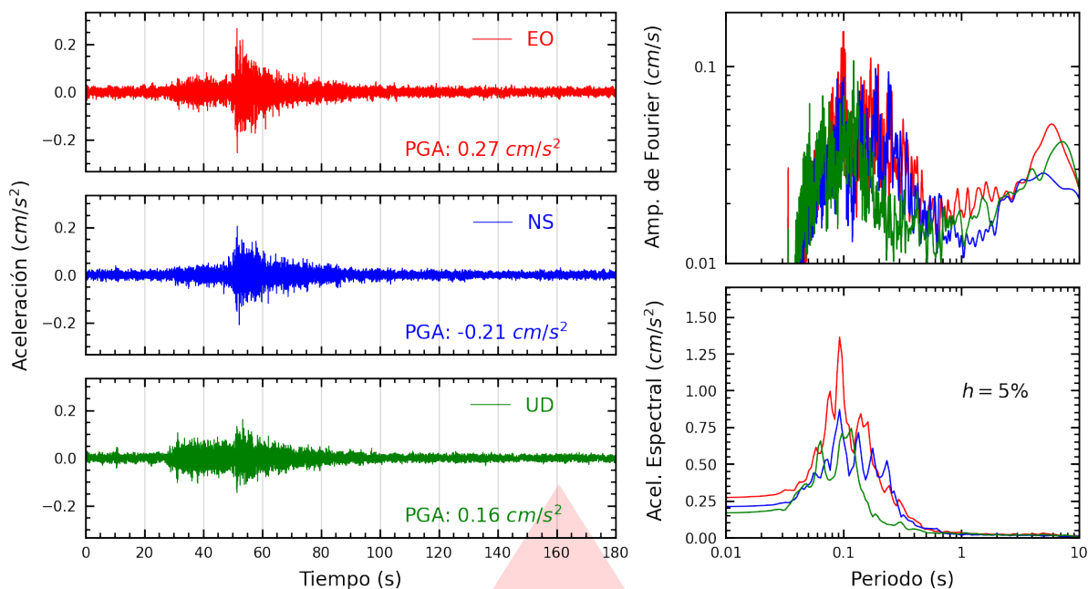
Figura A.15: Registros tiempo-historia, espectros de Fourier y de respuesta en las direcciones EO, NS y vertical de la estación USILP. Sismo de Huacho, Huaura - Lima del 2026-01-31, 16:28:11 (Hora local)
