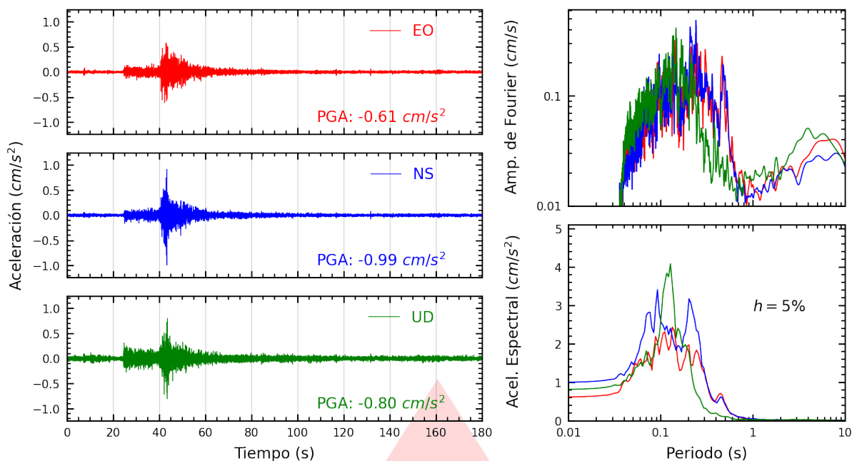
Figura A.3: Registros tiempo-historia, espectros de Fourier y de respuesta en las direcciones EO, NS y vertical de la estación MDPP. Sismo de Huacho, Huaura - Lima del 2026-01-31, 16:28:11 (Hora local)
