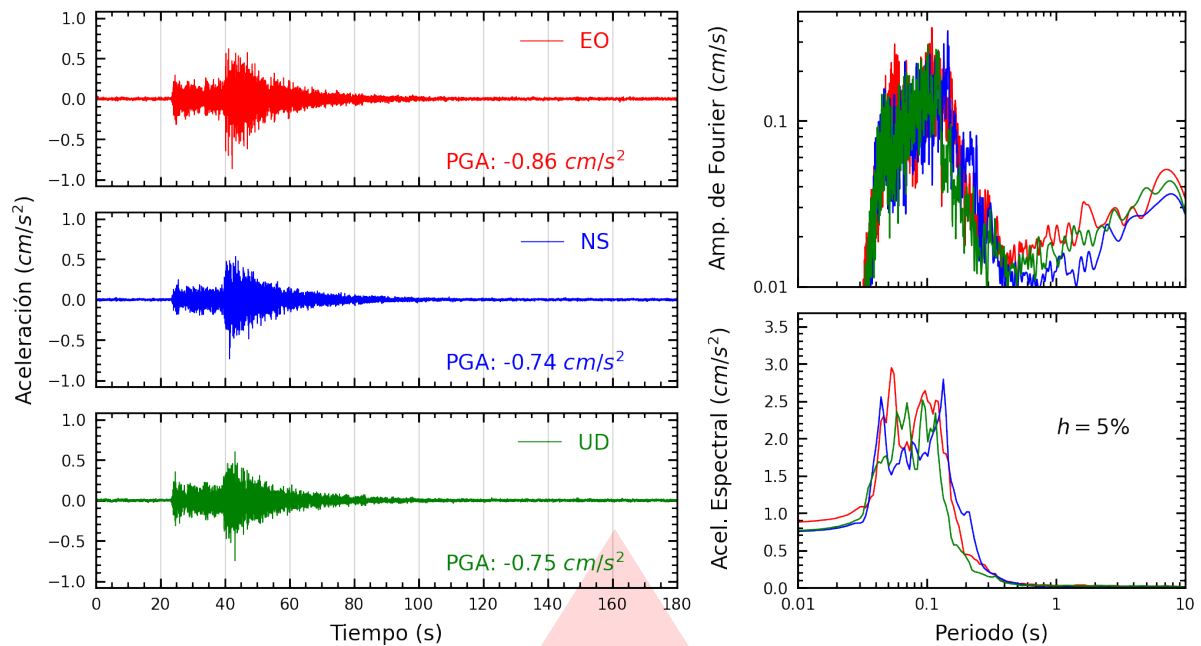
Figura A.5: Registros tiempo-historia, espectros de Fourier y de respuesta en las direcciones EO, NS y vertical de la estación AMORE. Sismo de Huacho, Huaura - Lima del 2026-01-31, 16:28:11 (Hora local)
