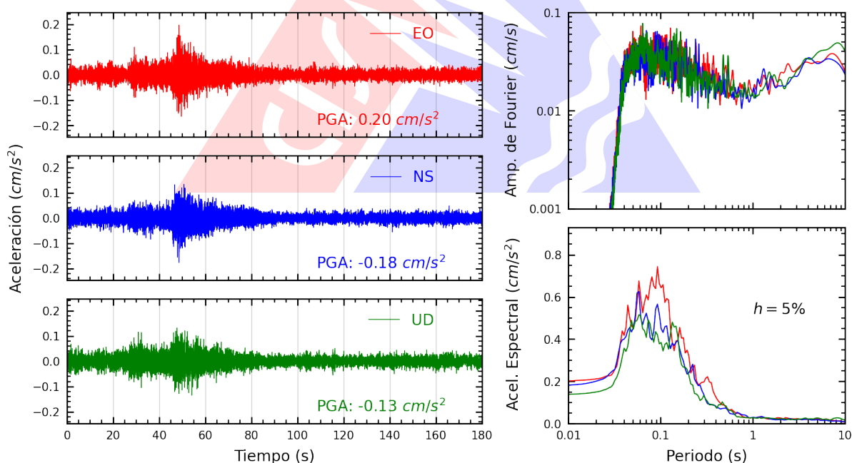
Figura A.20: Registros tiempo-historia, espectros de Fourier y de respuesta en las direcciones EO, NS y vertical de la estación IMCA. Sismo de Huacho, Huaura - Lima del 2026-01-31, 16:28:11 (Hora local)
