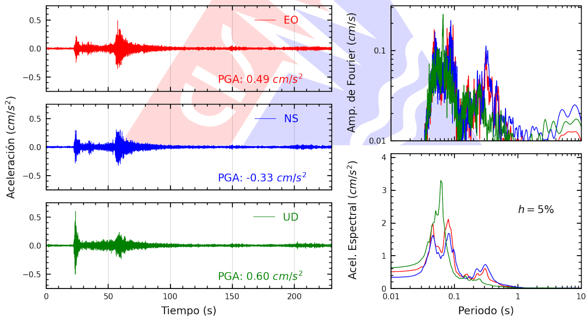
Figura A.2: Registros tiempo-historia, espectros de Fourier y de respuesta en las direcciones EO, NS y vertical de la estación CREY. Sismo de Santa Lucía, Lampa - Puno del 2026-02-02, 21:08:16 (Hora local)
