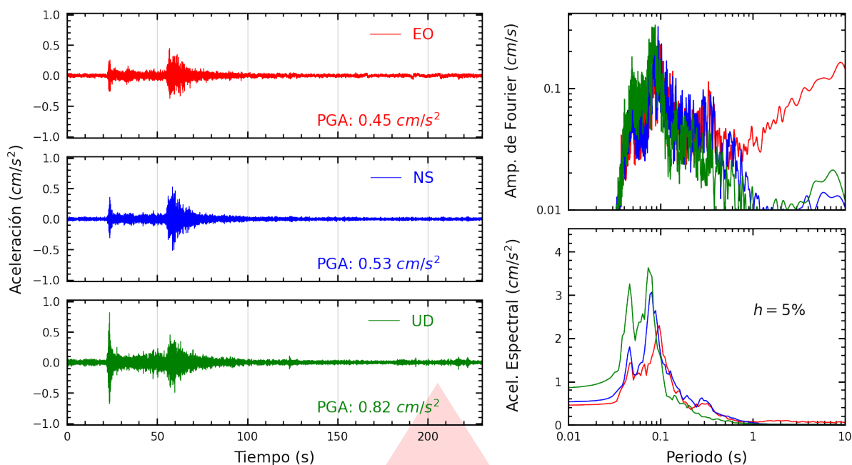
Figura A.1: Registros tiempo-historia, espectros de Fourier y de respuesta en las direcciones EO, NS y vertical de la estación UJBG3. Sismo de Santa Lucía, Lampa - Puno del 2026-02-02, 21:08:16 (Hora local)
