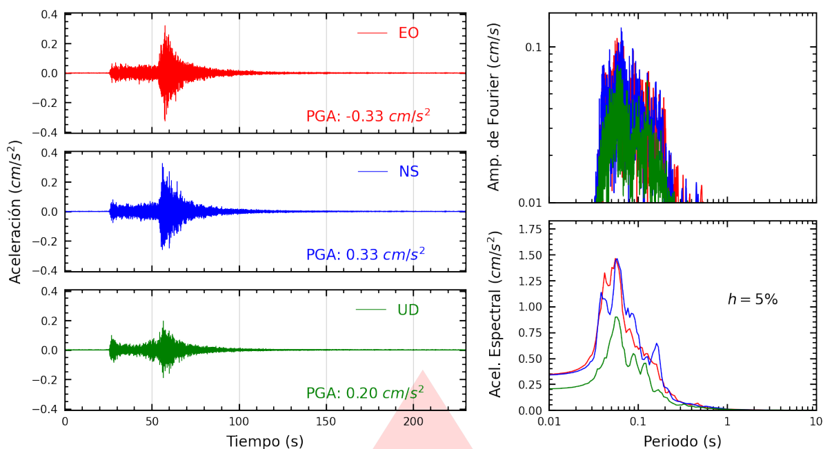
Figura A.5: Registros tiempo-historia, espectros de Fourier y de respuesta en las direcciones EO, NS y vertical de la estación UNSA2. Sismo de Santa Lucía, Lampa - Puno del 2026-02-02, 21:08:16 (Hora local)
