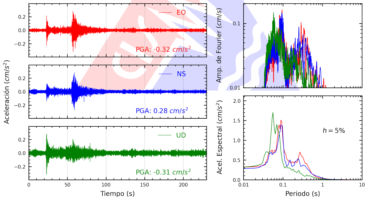
Figura A.6: Registros tiempo-historia, espectros de Fourier y de respuesta en las direcciones EO, NS y vertical de la estación UJBG2. Sismo de Santa Lucía, Lampa - Puno del 2026-02-02, 21:08:16 (Hora local)
