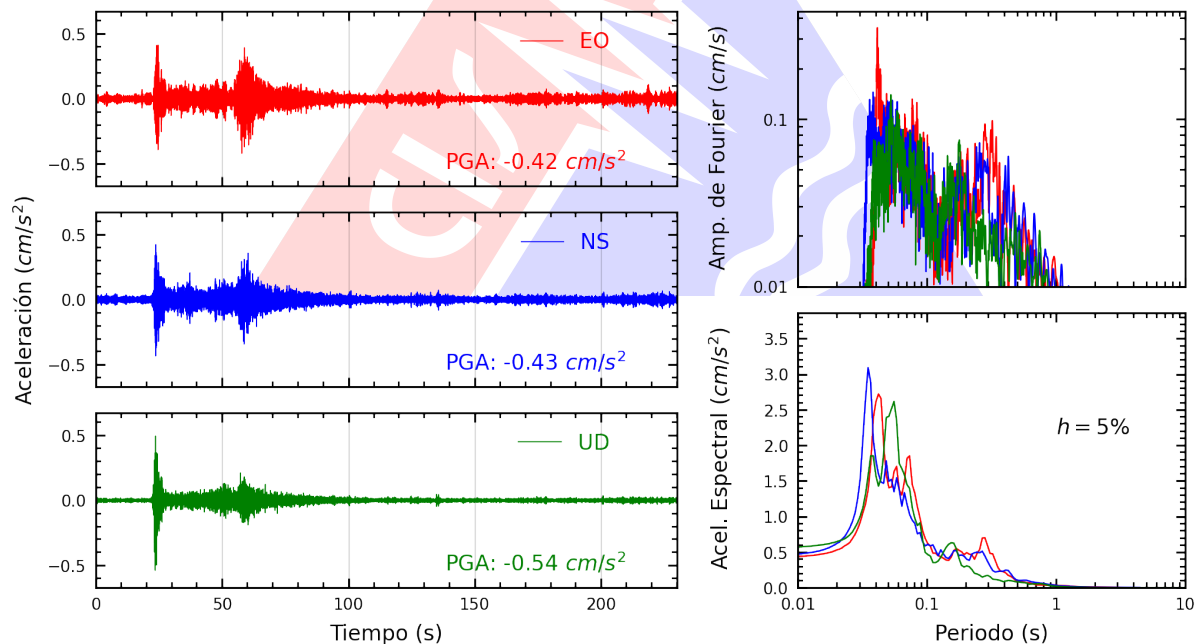
Figura A.4: Registros tiempo-historia, espectros de Fourier y de respuesta en las direcciones EO, NS y vertical de la estación UPTAC. Sismo de Santa Lucía, Lampa - Puno del 2026-02-02, 21:08:16 (Hora local)
