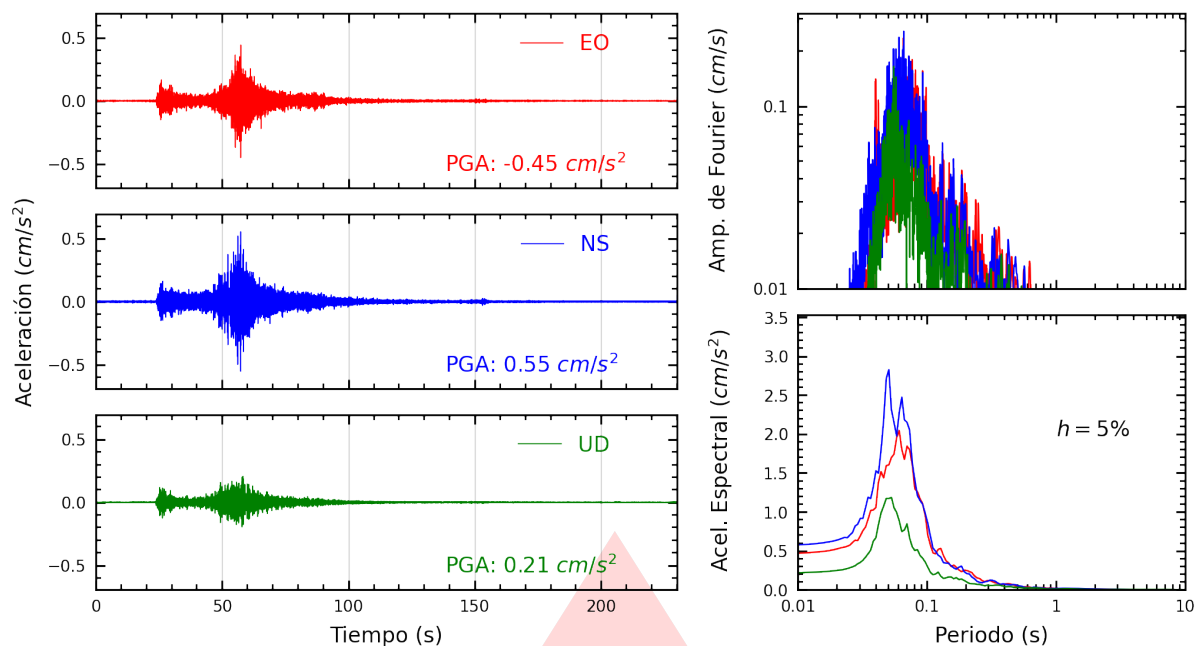
Figura A.3: Registros tiempo-historia, espectros de Fourier y de respuesta en las direcciones EO, NS y vertical de la estación UNAM. Sismo de Santa Lucía, Lampa - Puno del 2026-02-02, 21:08:16 (Hora local)
