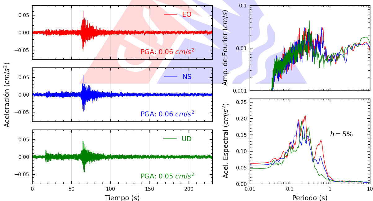
Figura A.2: Registros tiempo-historia, espectros de Fourier y de respuesta en las direcciones EO, NS y vertical de la estación CARAL. Sismo de Pucallpa, Coronel Portillo - Ucayali del 2026-02-26, 01:54:13 (Hora local)
