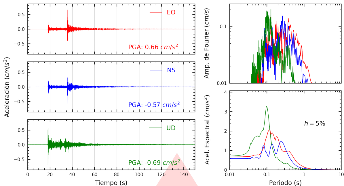
Figura A.1: Registros tiempo-historia, espectros de Fourier y de respuesta en las direcciones EO, NS y vertical de la estación UNIA. Sismo de Pucallpa, Coronel Portillo - Ucayali del 2026-02-26, 01:54:13 (Hora local)
