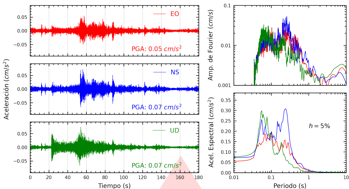
Figura A.1: Registros tiempo-historia, espectros de Fourier y de respuesta en las direcciones EO, NS y vertical de la estación UNAAA. Sismo de Andoas, Datem del Marañón - Loreto del 2026-02-27, 23:28:12 (Hora local)
