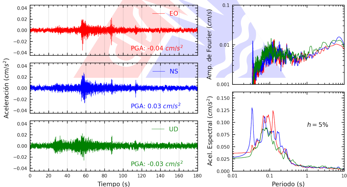
Figura A.2: Registros tiempo-historia, espectros de Fourier y de respuesta en las direcciones EO, NS y vertical de la estación UNJ. Sismo de Andoas, Datem del Marañón - Loreto del 2026-02-27, 23:28:12 (Hora local)
