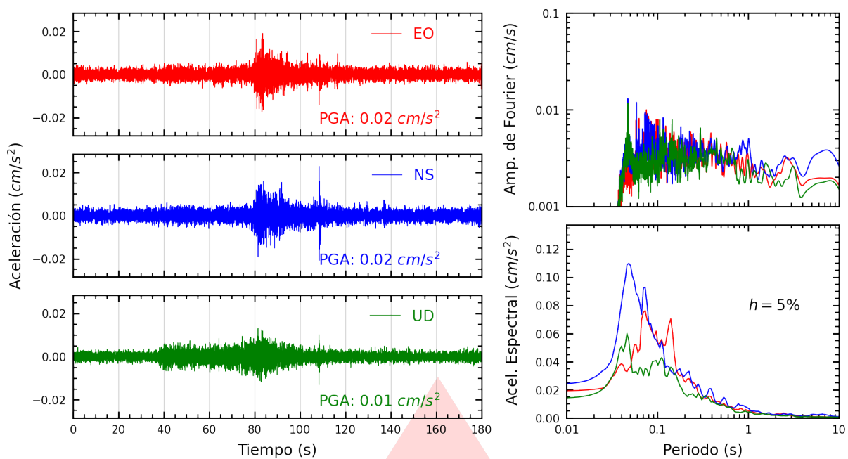
Figura A.3: Registros tiempo-historia, espectros de Fourier y de respuesta en las direcciones EO, NS y vertical de la estación UNF. Sismo de Andoas, Datem del Maraón - Loreto del 2026-02-27, 23:28:12 (Hora local)
