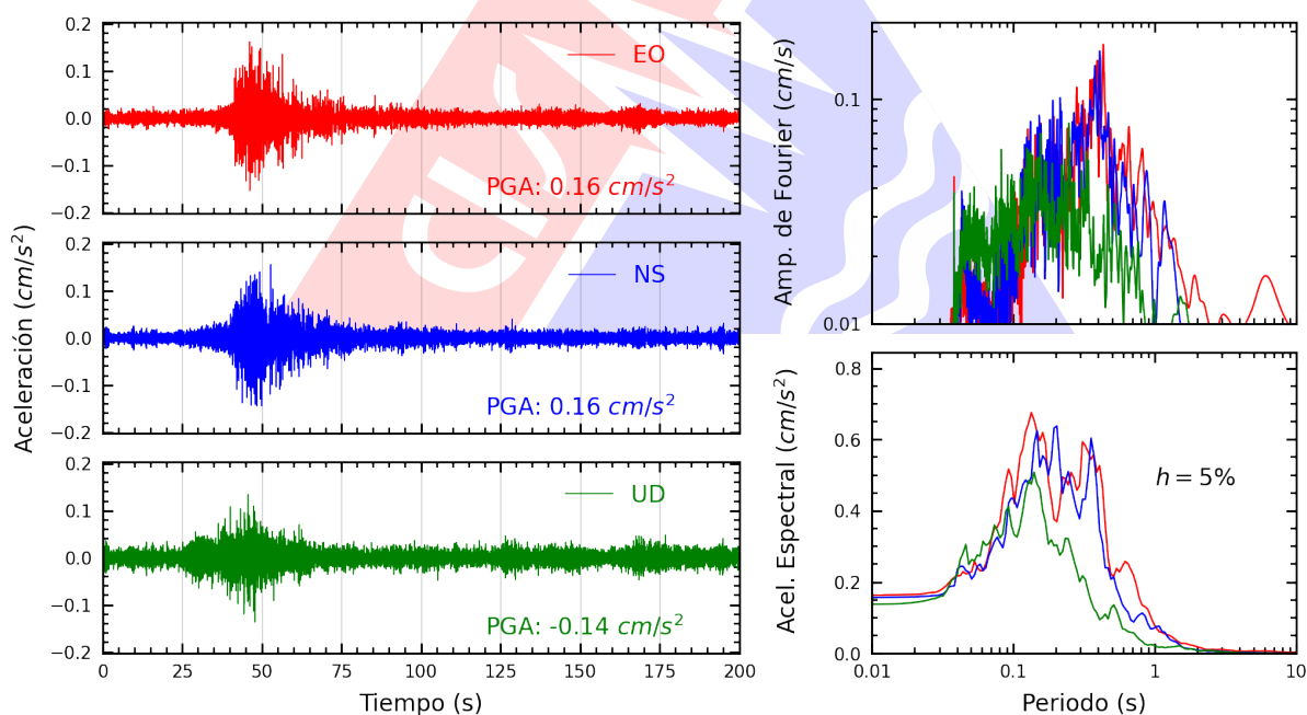
Figura A.2: Registros tiempo-historia, espectros de Fourier y de respuesta en las direcciones EO, NS y vertical de la estación SCPIU. Sismo de Máncora, Talara - Piura del 2026-03-03, 23:14:22 (Hora local)
