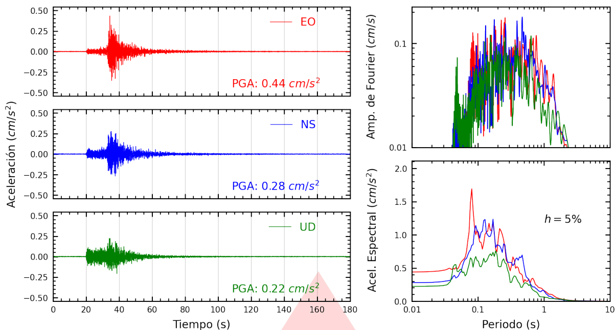
Figura A.1: Registros tiempo-historia, espectros de Fourier y de respuesta en las direcciones EO, NS y vertical de la estación UNF. Sismo de Máncora, Talara - Piura del 2026-03-03, 23:14:22 (Hora local)
