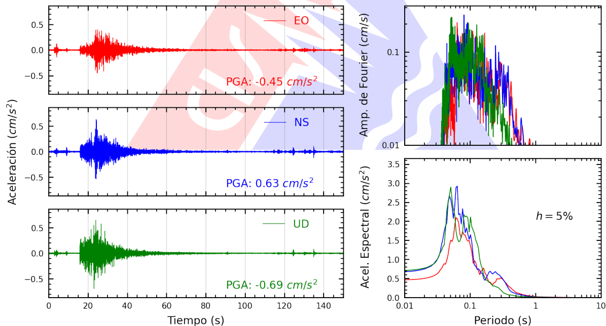
Figura A.2: Registros tiempo-historia, espectros de Fourier y de respuesta en las direcciones EO, NS y vertical de la estación UPAOP. Sismo de Sechura, Sechura - Piura del 2026-03-08, 06:55:11 (Hora local)
