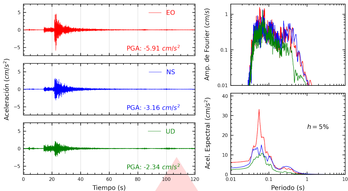
Figura A.15: Registros tiempo-historia, espectros de Fourier y de respuesta en las direcciones EO, NS y vertical de la estación SCOLI. Sismo de Chilca, Cañete - Lima del 2026-03-08, 14:11:41 (Hora local)
