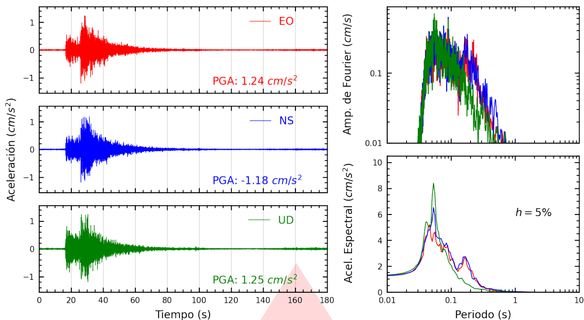
Figura A.37: Registros tiempo-historia, espectros de Fourier y de respuesta en las direcciones EO, NS y vertical de la estación ASIA. Sismo de Chilca, Cañete - Lima del 2026-03-08, 14:11:41 (Hora local)
