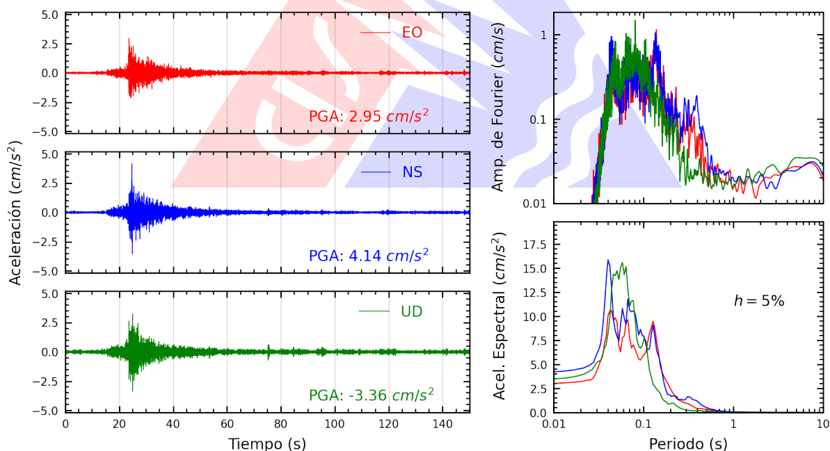
Figura A.22: Registros tiempo-historia, espectros de Fourier y de respuesta en las direcciones EO, NS y vertical de la estación CARAB. Sismo de Chilca, Cañete - Lima del 2026-03-08, 14:11:41 (Hora local)
