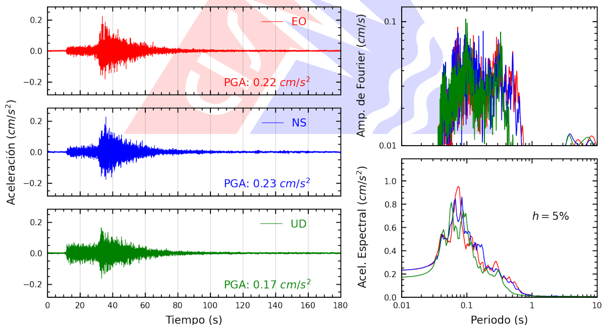
Figura A.38: Registros tiempo-historia, espectros de Fourier y de respuesta en las direcciones EO, NS y vertical de la estación CARAL. Sismo de Chilca, Cañete - Lima del 2026-03-08, 14:11:41 (Hora local)
