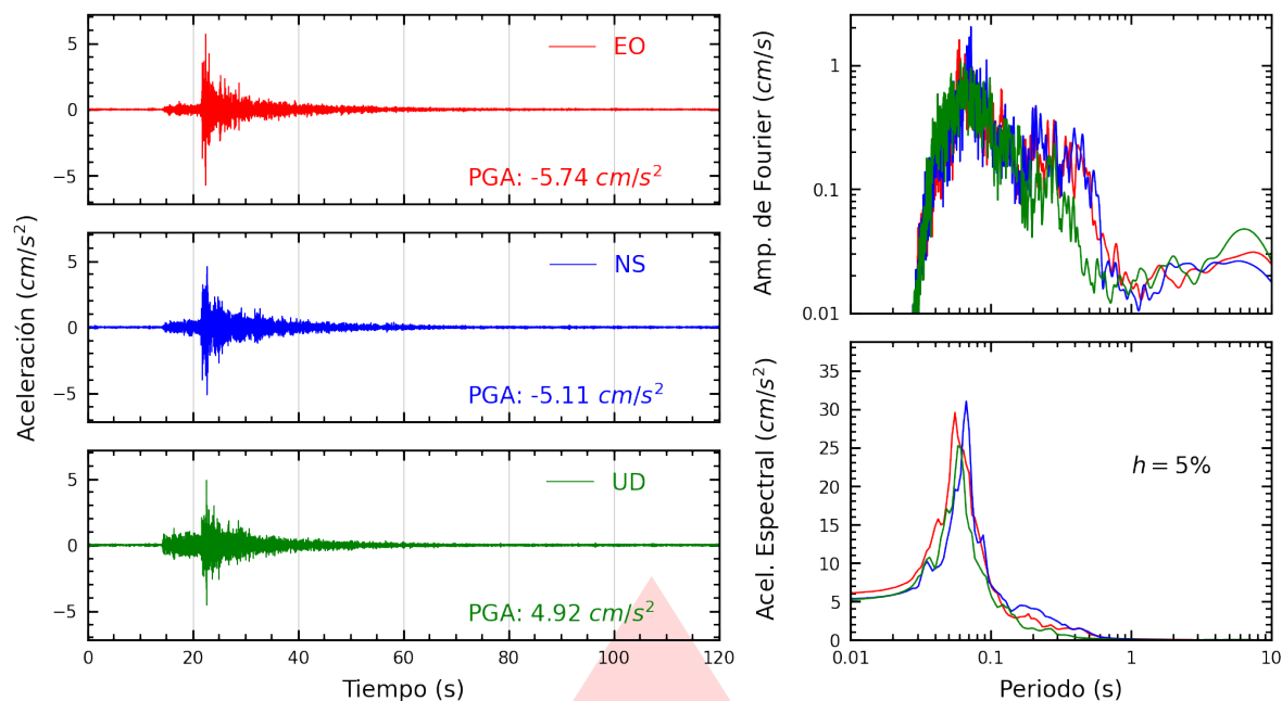
Figura A.17: Registros tiempo-historia, espectros de Fourier y de respuesta en las direcciones EO, NS y vertical de la estación SJLSC. Sismo de Chilca, Cañete - Lima del 2026-03-08, 14:11:41 (Hora local)
