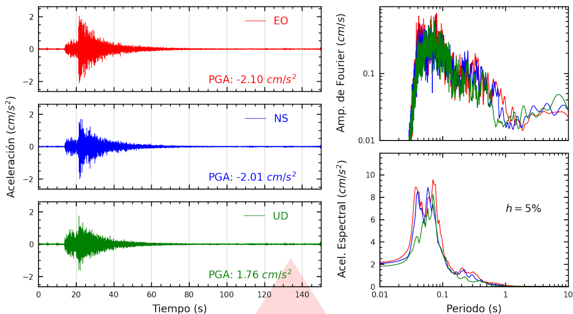
Figura A.33: Registros tiempo-historia, espectros de Fourier y de respuesta en las direcciones EO, NS y vertical de la estación UCVAT. Sismo de Chilca, Cañete - Lima del 2026-03-08, 14:11:41 (Hora local)
