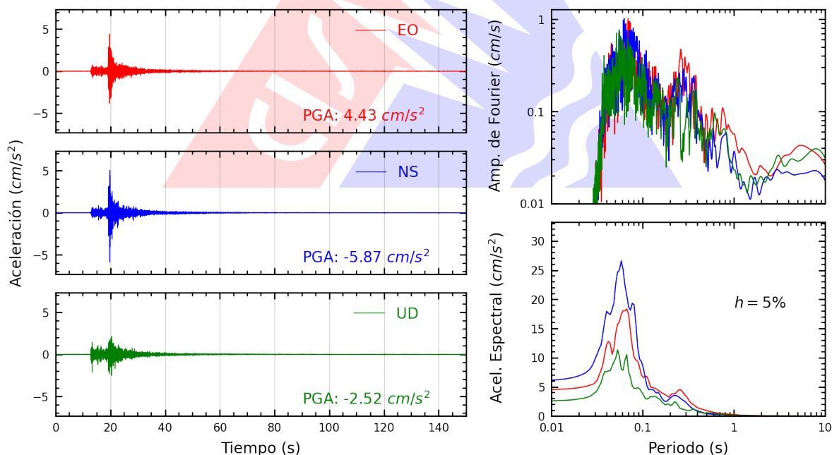
Figura A.16: Registros tiempo-historia, espectros de Fourier y de respuesta en las direcciones EO, NS y vertical de la estación SERVI. Sismo de Chilca, Cañete - Lima del 2026-03-08, 14:11:41 (Hora local)
