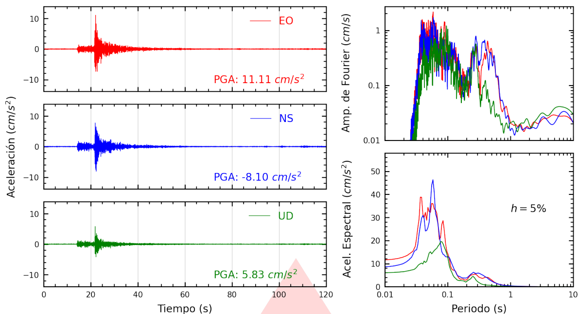
Figura A.5: Registros tiempo-historia, espectros de Fourier y de respuesta en las direcciones EO, NS y vertical de la estación OLIVO. Sismo de Chilca, Cañete - Lima del 2026-03-08, 14:11:41 (Hora local)
