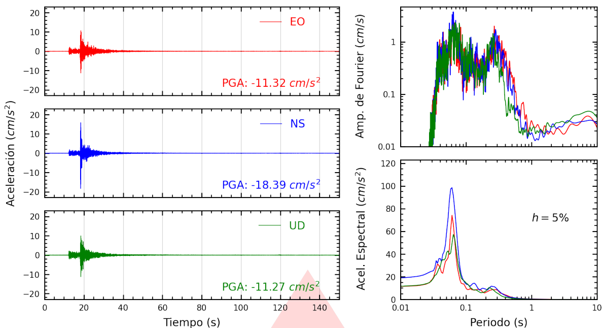
Figura A.1: Registros tiempo-historia, espectros de Fourier y de respuesta en las direcciones EO, NS y vertical de la estación SOVES. Sismo de Chilca, Cañete - Lima del 2026-03-08, 14:11:41 (Hora local)
