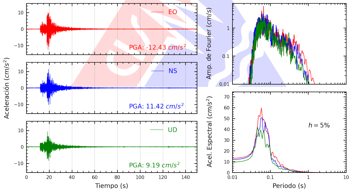
Figura A.4: Registros tiempo-historia, espectros de Fourier y de respuesta en las direcciones EO, NS y vertical de la estación PHERM. Sismo de Chilca, Cañete - Lima del 2026-03-08, 14:11:41 (Hora local)
