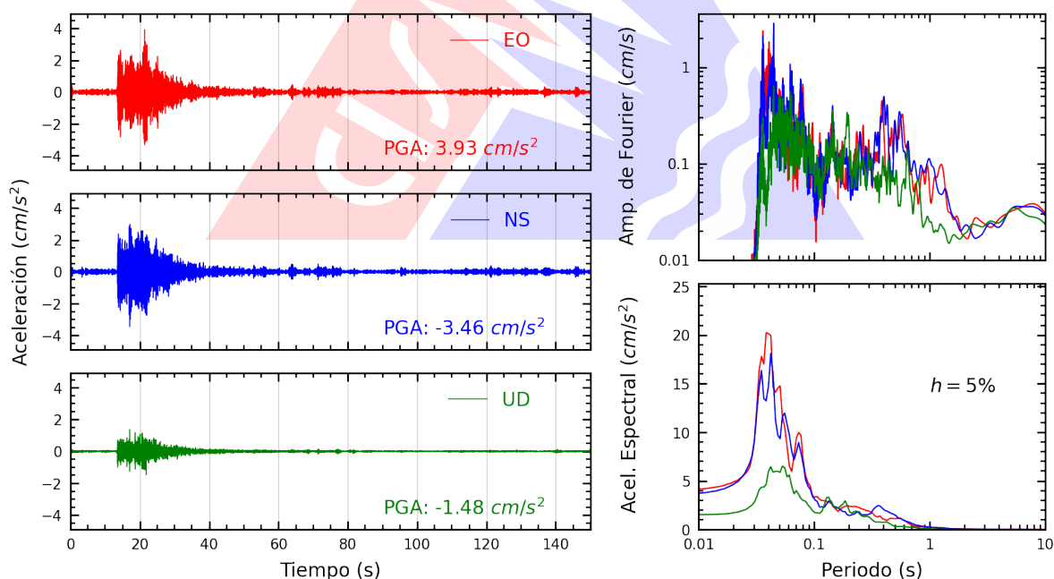
Figura A.24: Registros tiempo-historia, espectros de Fourier y de respuesta en las direcciones EO, NS y vertical de la estación DHNPE. Sismo de Chilca, Cañete - Lima del 2026-03-08, 14:11:41 (Hora local)
