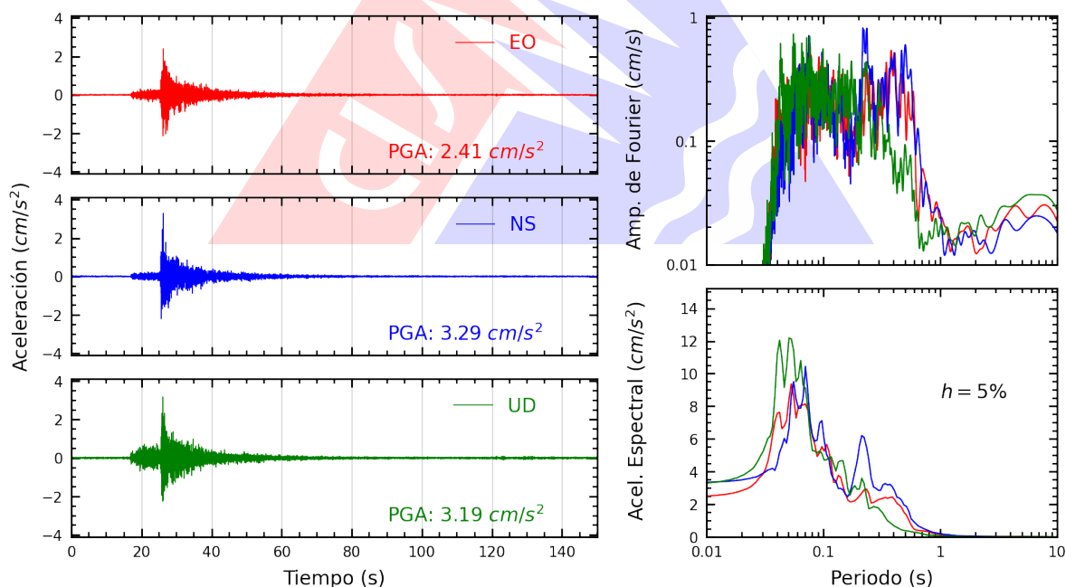
Figura A.28: Registros tiempo-historia, espectros de Fourier y de respuesta en las direcciones EO, NS y vertical de la estación MDPP. Sismo de Chilca, Cañete - Lima del 2026-03-08, 14:11:41 (Hora local)
