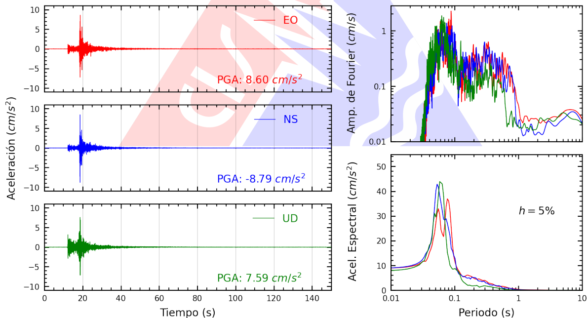
Figura A.8: Registros tiempo-historia, espectros de Fourier y de respuesta en las direcciones EO, NS y vertical de la estación USILP. Sismo de Chilca, Cañete - Lima del 2026-03-08, 14:11:41 (Hora local)
