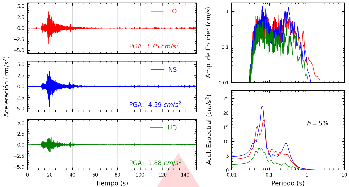
Figura A.19: Registros tiempo-historia, espectros de Fourier y de respuesta en las direcciones EO, NS y vertical de la estación BRIS2. Sismo de Chilca, Cañete - Lima del 2026-03-08, 14:11:41 (Hora local)
