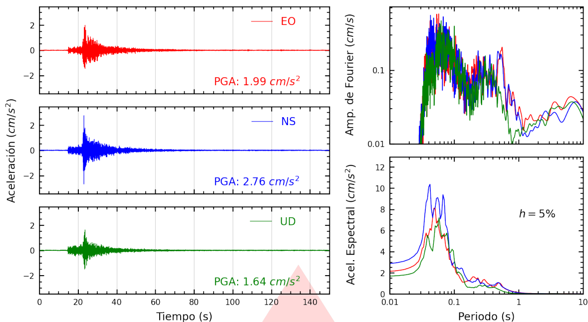
Figura A.29: Registros tiempo-historia, espectros de Fourier y de respuesta en las direcciones EO, NS y vertical de la estación COMAS. Sismo de Chilca, Cañete - Lima del 2026-03-08, 14:11:41 (Hora local)
