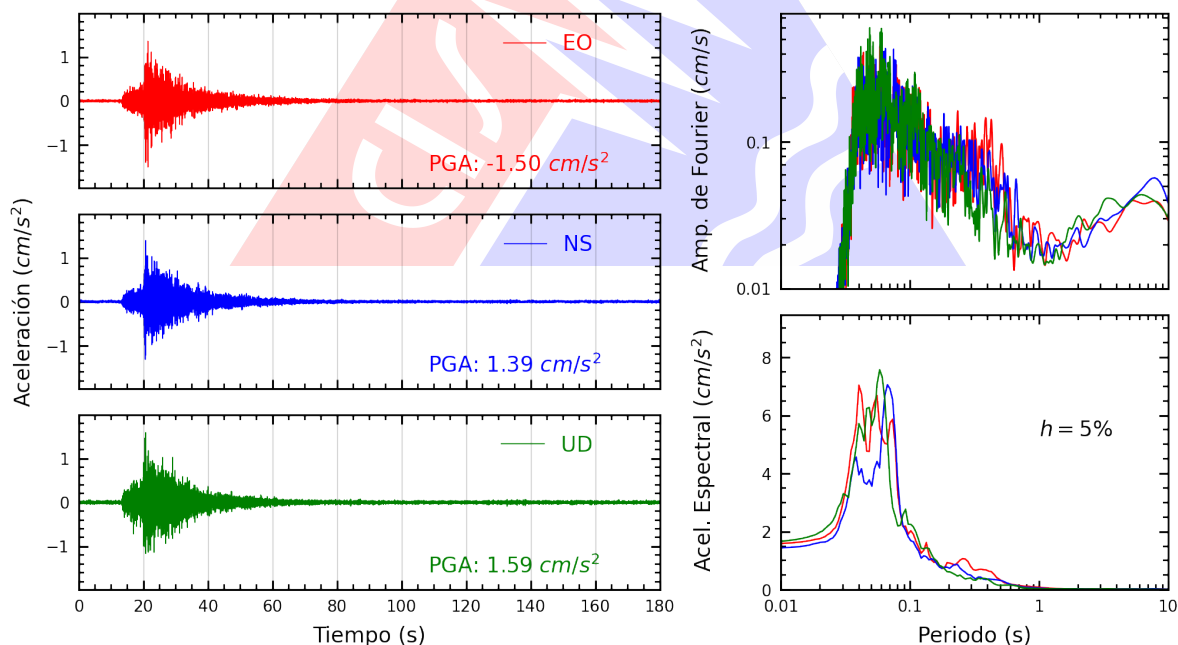
Figura A.36: Registros tiempo-historia, espectros de Fourier y de respuesta en las direcciones EO, NS y vertical de la estación USMP. Sismo de Chilca, Cañete - Lima del 2026-03-08, 14:11:41 (Hora local)
