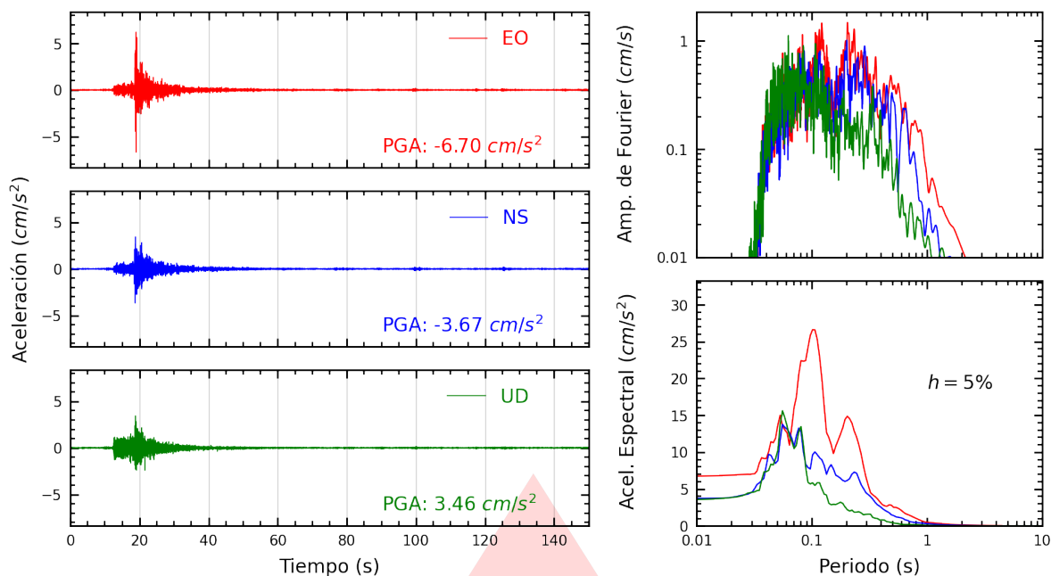
Figura A.13: Registros tiempo-historia, espectros de Fourier y de respuesta en las direcciones EO, NS y vertical de la estación SCCHO. Sismo de Chilca, Cañete - Lima del 2026-03-08, 14:11:41 (Hora local)
