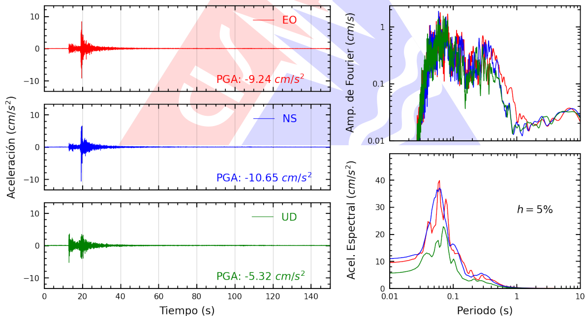
Figura A.6: Registros tiempo-historia, espectros de Fourier y de respuesta en las direcciones EO, NS y vertical de la estación URPE. Sismo de Chilca, Cañete - Lima del 2026-03-08, 14:11:41 (Hora local)
