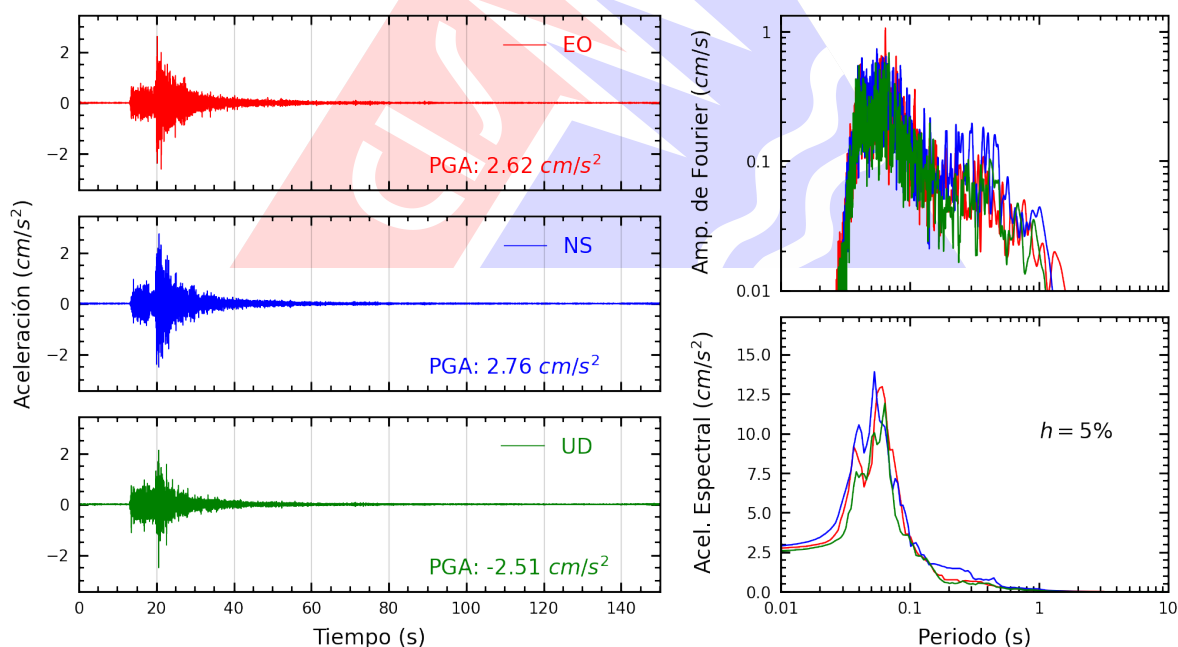
Figura A.30: Registros tiempo-historia, espectros de Fourier y de respuesta en las direcciones EO, NS y vertical de la estación BORJA. Sismo de Chilca, Cañete - Lima del 2026-03-08, 14:11:41 (Hora local)
