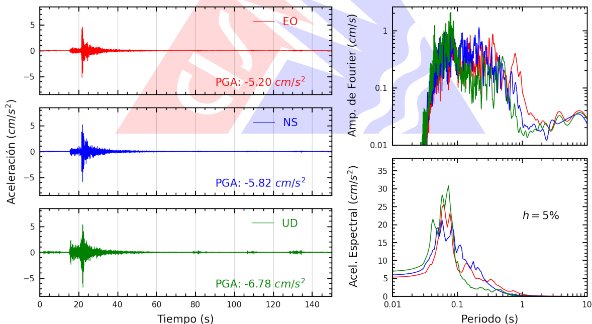
Figura A.12: Registros tiempo-historia, espectros de Fourier y de respuesta en las direcciones EO, NS y vertical de la estación SOCHO. Sismo de Chilca, Cañete - Lima del 2026-03-08, 14:11:41 (Hora local)
