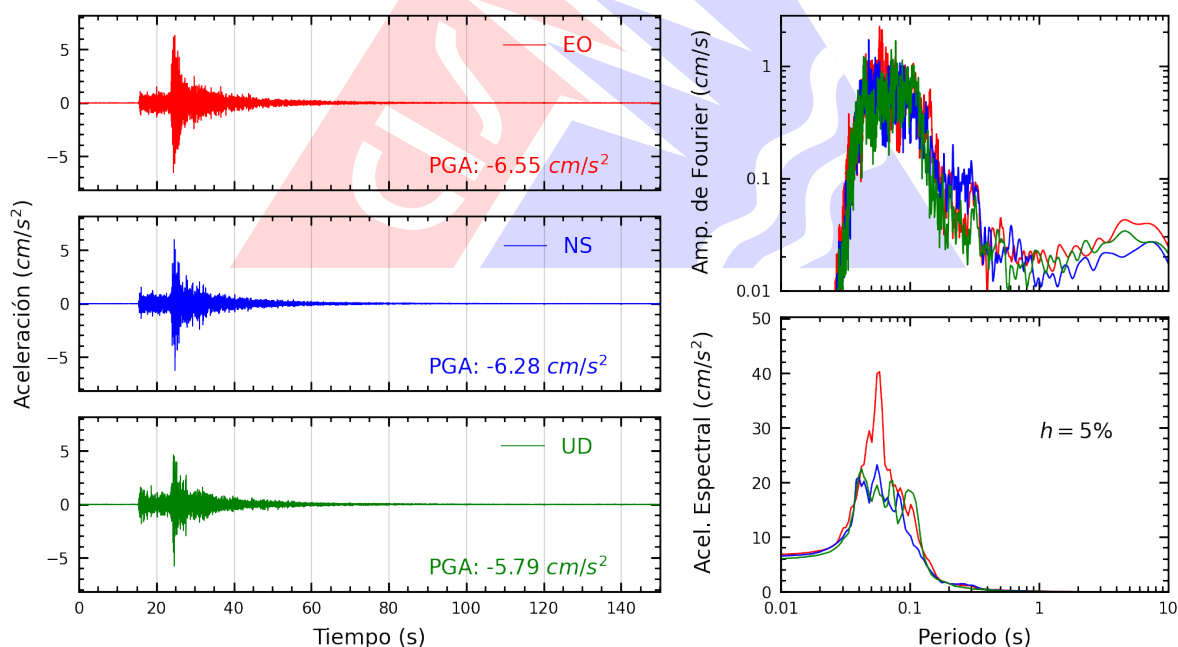
Figura A.14: Registros tiempo-historia, espectros de Fourier y de respuesta en las direcciones EO, NS y vertical de la estación AMORE. Sismo de Chilca, Cañete - Lima del 2026-03-08, 14:11:41 (Hora local)
