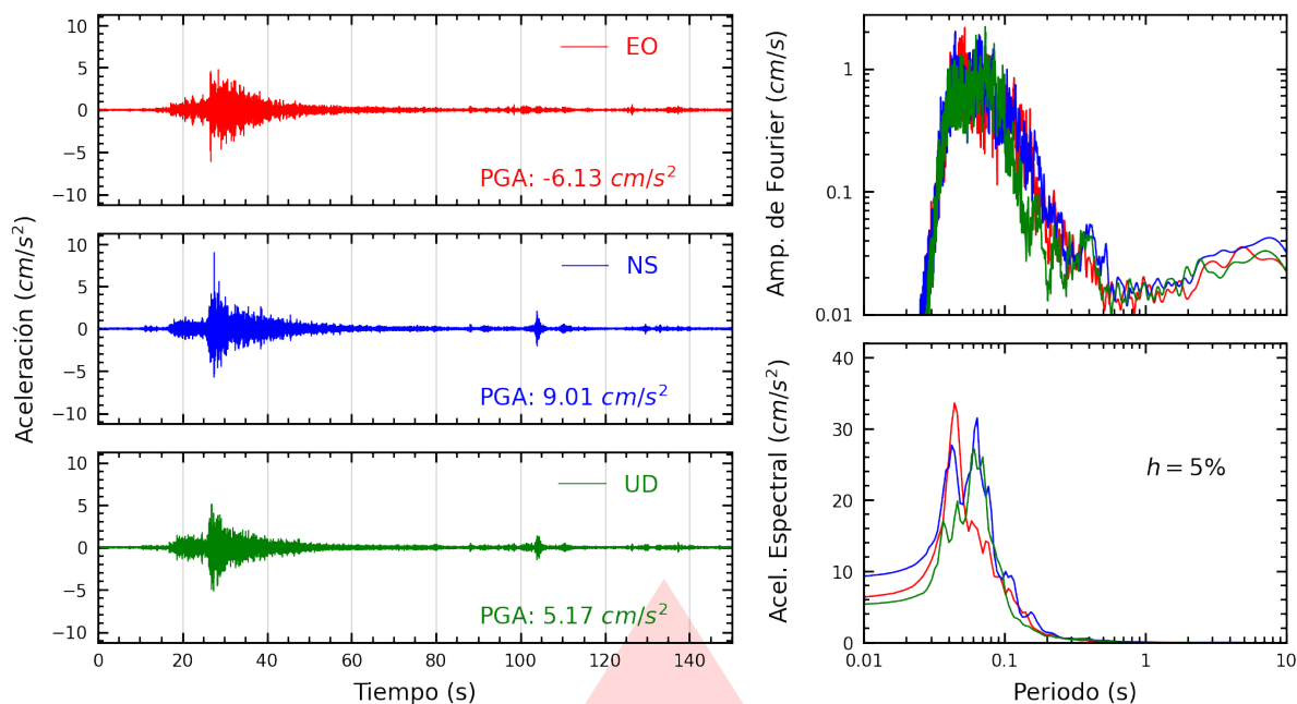
Figura A.7: Registros tiempo-historia, espectros de Fourier y de respuesta en las direcciones EO, NS y vertical de la estación SROSA. Sismo de Chilca, Cañete - Lima del 2026-03-08, 14:11:41 (Hora local)
