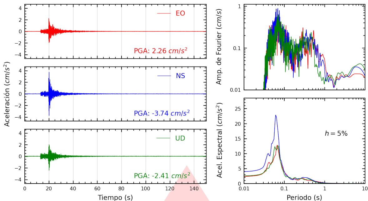
Figura A.25: Registros tiempo-historia, espectros de Fourier y de respuesta en las direcciones EO, NS y vertical de la estación UNFV. Sismo de Chilca, Cañete - Lima del 2026-03-08, 14:11:41 (Hora local)
