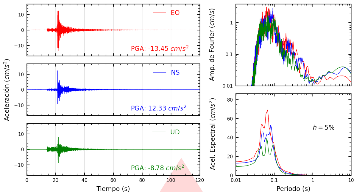
Figura A.3: Registros tiempo-historia, espectros de Fourier y de respuesta en las direcciones EO, NS y vertical de la estación INDEP. Sismo de Chilca, Cañete - Lima del 2026-03-08, 14:11:41 (Hora local)
