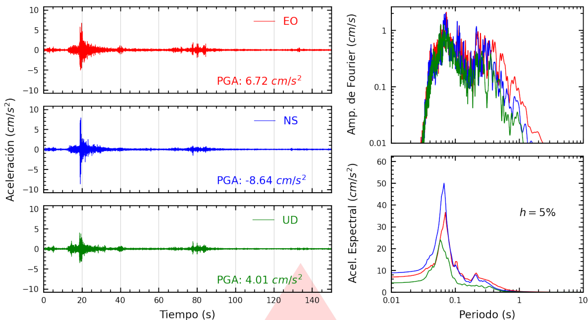
Figura A.9: Registros tiempo-historia, espectros de Fourier y de respuesta en las direcciones EO, NS y vertical de la estación SOBAR. Sismo de Chilca, Cañete - Lima del 2026-03-08, 14:11:41 (Hora local)
