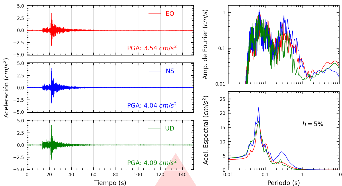
Figura A.23: Registros tiempo-historia, espectros de Fourier y de respuesta en las direcciones EO, NS y vertical de la estación MADRE. Sismo de Chilca, Cañete - Lima del 2026-03-08, 14:11:41 (Hora local)
