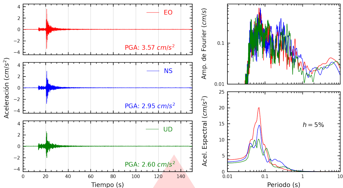
Figura A.27: Registros tiempo-historia, espectros de Fourier y de respuesta en las direcciones EO, NS y vertical de la estación BONDY. Sismo de Chilca, Cañete - Lima del 2026-03-08, 14:11:41 (Hora local)
