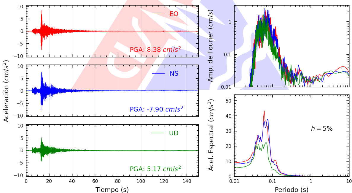
Figura A.10: Registros tiempo-historia, espectros de Fourier y de respuesta en las direcciones EO, NS y vertical de la estación JOSEO. Sismo de Chilca, Cañete - Lima del 2026-03-08, 14:11:41 (Hora local)
