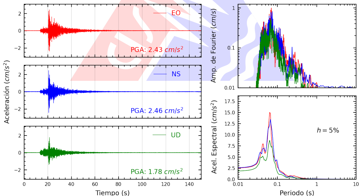
Figura A.32: Registros tiempo-historia, espectros de Fourier y de respuesta en las direcciones EO, NS y vertical de la estación ATARJ. Sismo de Chilca, Cañete - Lima del 2026-03-08, 14:11:41 (Hora local)
