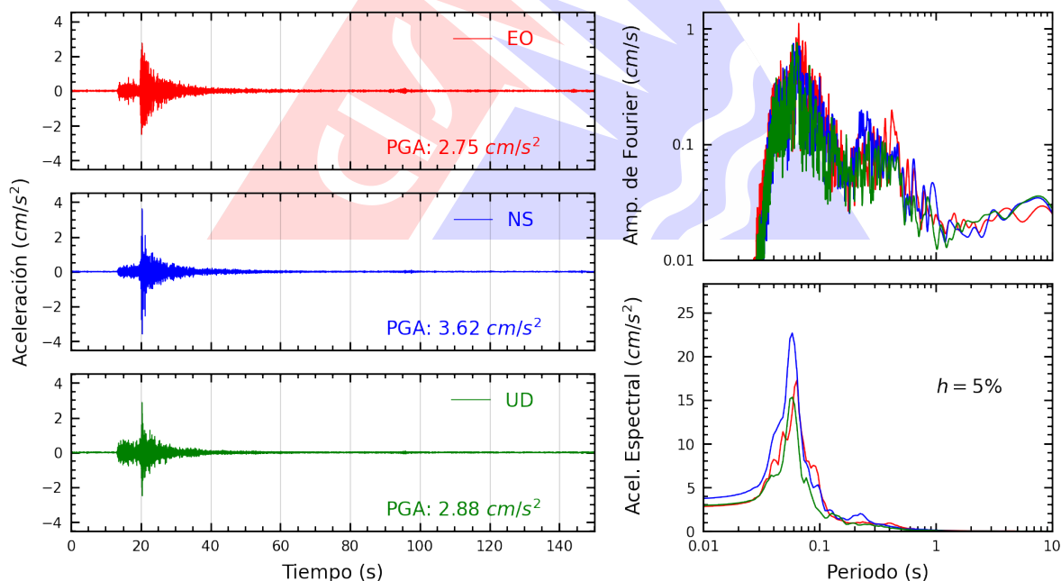
Figura A.26: Registros tiempo-historia, espectros de Fourier y de respuesta en las direcciones EO, NS y vertical de la estación INICT. Sismo de Chilca, Cañete - Lima del 2026-03-08, 14:11:41 (Hora local)
