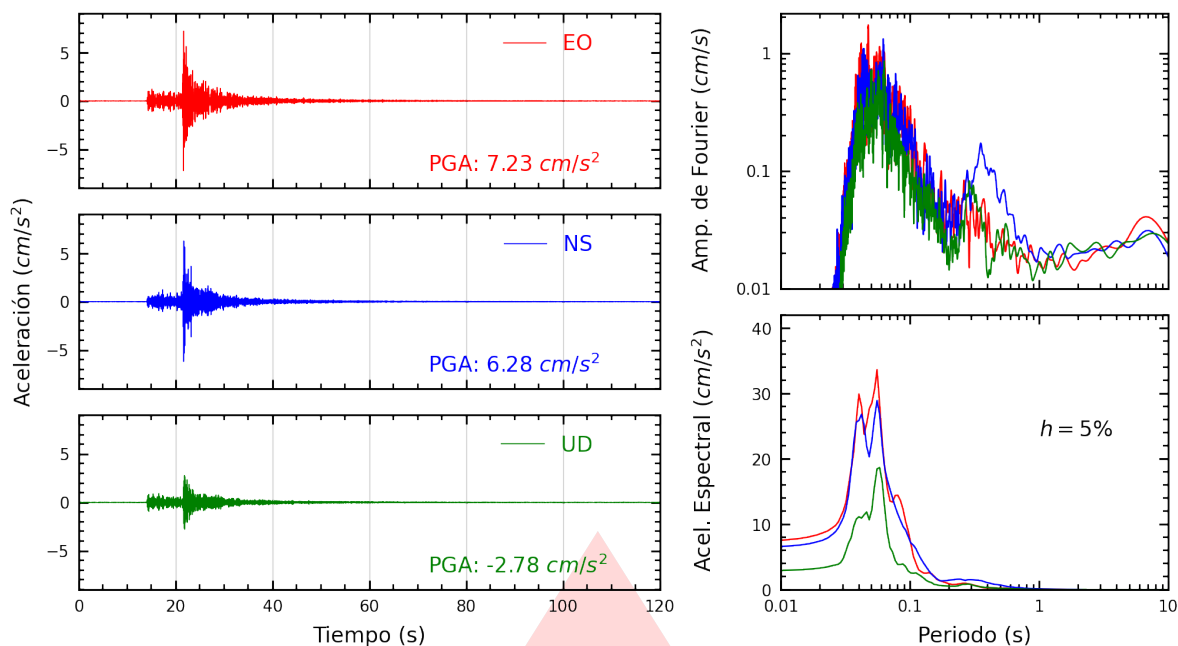
Figura A.11: Registros tiempo-historia, espectros de Fourier y de respuesta en las direcciones EO, NS y vertical de la estación UCSS. Sismo de Chilca, Cañete - Lima del 2026-03-08, 14:11:41 (Hora local)
