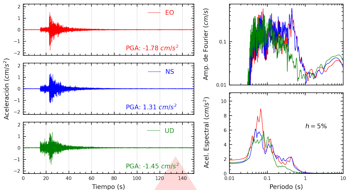
Figura A.35: Registros tiempo-historia, espectros de Fourier y de respuesta en las direcciones EO, NS y vertical de la estación VHAYA. Sismo de Chilca, Cañete - Lima del 2026-03-08, 14:11:41 (Hora local)
