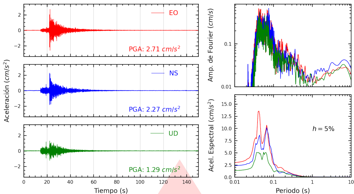
Figura A.31: Registros tiempo-historia, espectros de Fourier y de respuesta en las direcciones EO, NS y vertical de la estación SJLCE. Sismo de Chilca, Cañete - Lima del 2026-03-08, 14:11:41 (Hora local)
