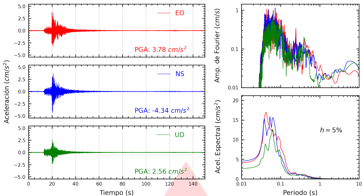
Figura A.21: Registros tiempo-historia, espectros de Fourier y de respuesta en las direcciones EO, NS y vertical de la estación CEPRE. Sismo de Chilca, Cañete - Lima del 2026-03-08, 14:11:41 (Hora local)
