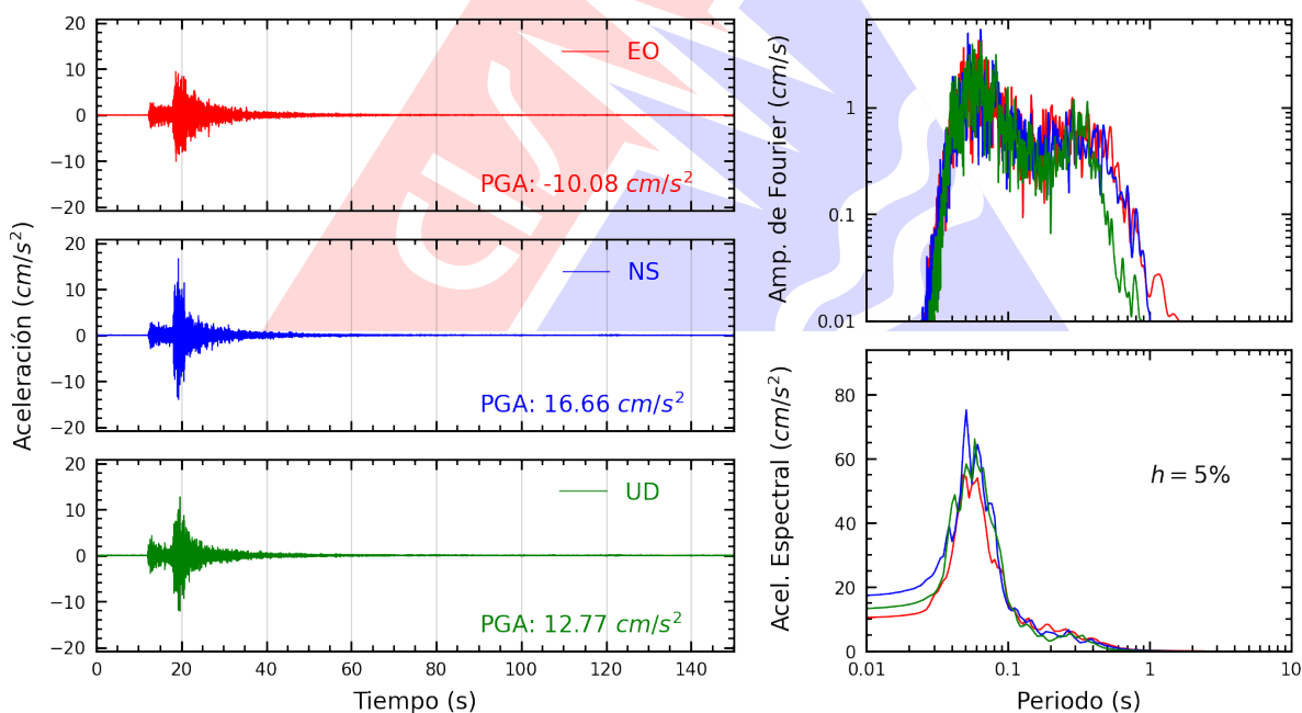
Figura A.2: Registros tiempo-historia, espectros de Fourier y de respuesta en las direcciones EO, NS y vertical de la estación UNTEL. Sismo de Chilca, Cañete - Lima del 2026-03-08, 14:11:41 (Hora local)
