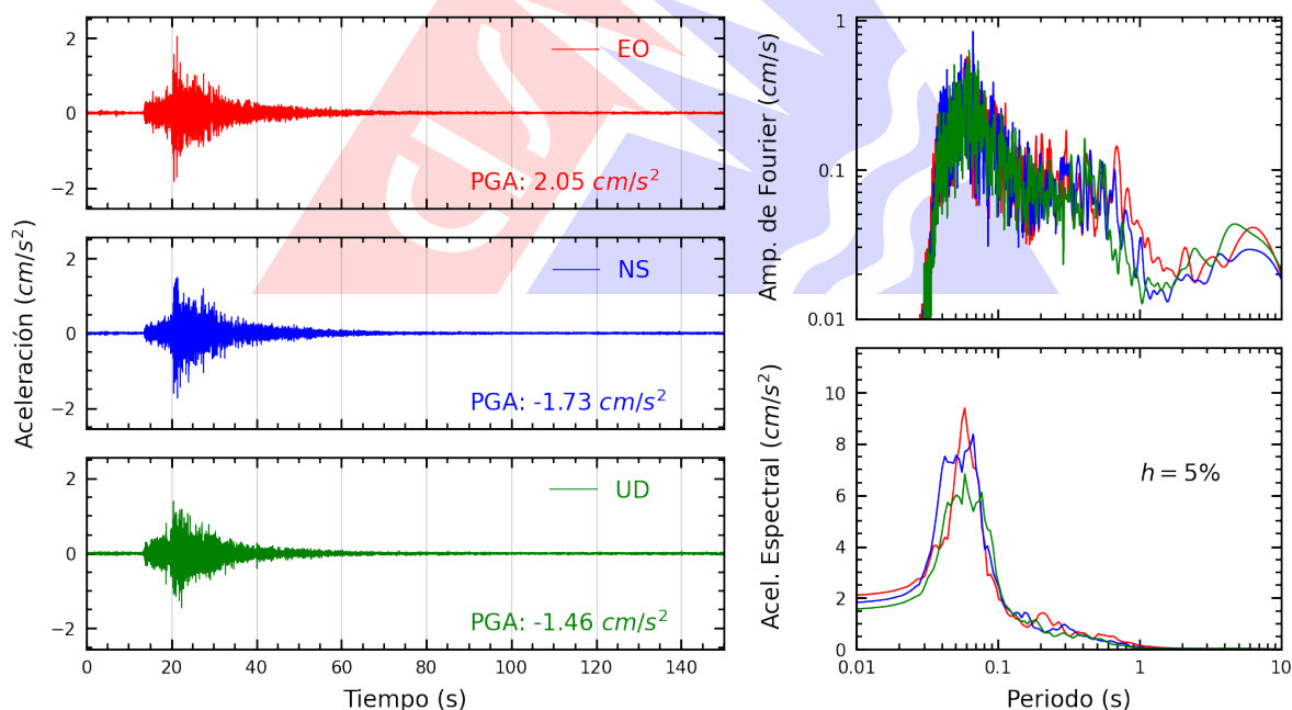
Figura A.34: Registros tiempo-historia, espectros de Fourier y de respuesta en las direcciones EO, NS y vertical de la estación IMCA. Sismo de Chilca, Cañete - Lima del 2026-03-08, 14:11:41 (Hora local)
