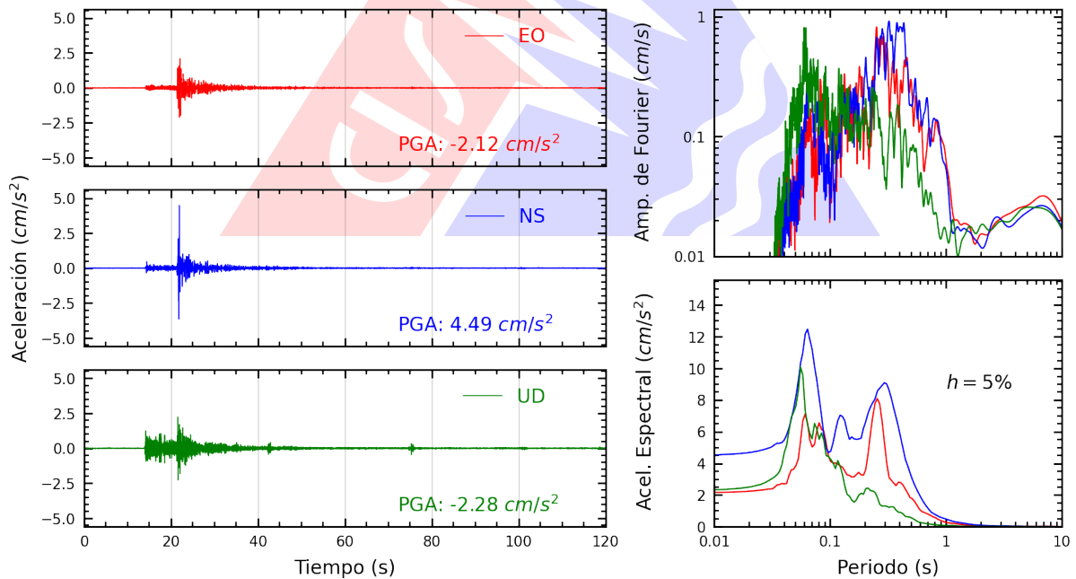
Figura A.20: Registros tiempo-historia, espectros de Fourier y de respuesta en las direcciones EO, NS y vertical de la estación ACAPU. Sismo de Chilca, Cañete - Lima del 2026-03-08, 14:11:41 (Hora local)
