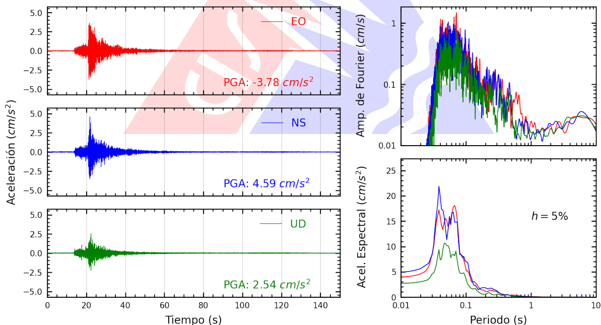
Figura A.18: Registros tiempo-historia, espectros de Fourier y de respuesta en las direcciones EO, NS y vertical de la estación FICPE. Sismo de Chilca, Cañete - Lima del 2026-03-08, 14:11:41 (Hora local)
