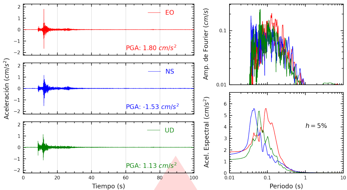
Figura A.1: Registros tiempo-historia, espectros de Fourier y de respuesta en las direcciones EO, NS y vertical de la estación UNJ. Sismo de Jaén, Jaén - Cajamarca del 2026-03-10, 15:50:54 (Hora local)
