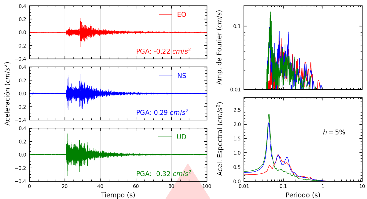
Figura A.1: Registros tiempo-historia, espectros de Fourier y de respuesta en las direcciones EO, NS y vertical de la estación UNF. Sismo de Lancones, Sullana - Piura del 2026-03-11, 05:27:28 (Hora local)
