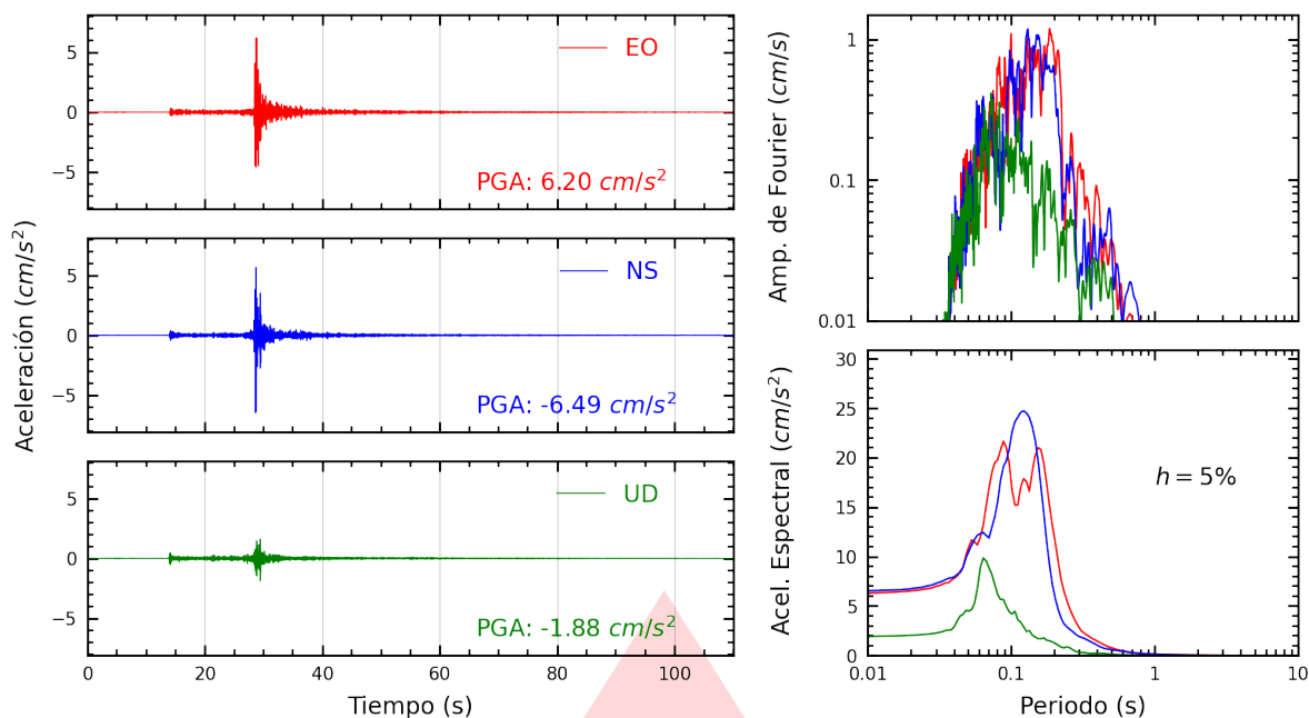
Figura A.1: Registros tiempo-historia, espectros de Fourier y de respuesta en las direcciones EO, NS y vertical de la estación UNAS. Sismo de Aucayacu, Leoncio Prado - Huánuco del 2026-03-13, 06:12:42 (Hora local)
