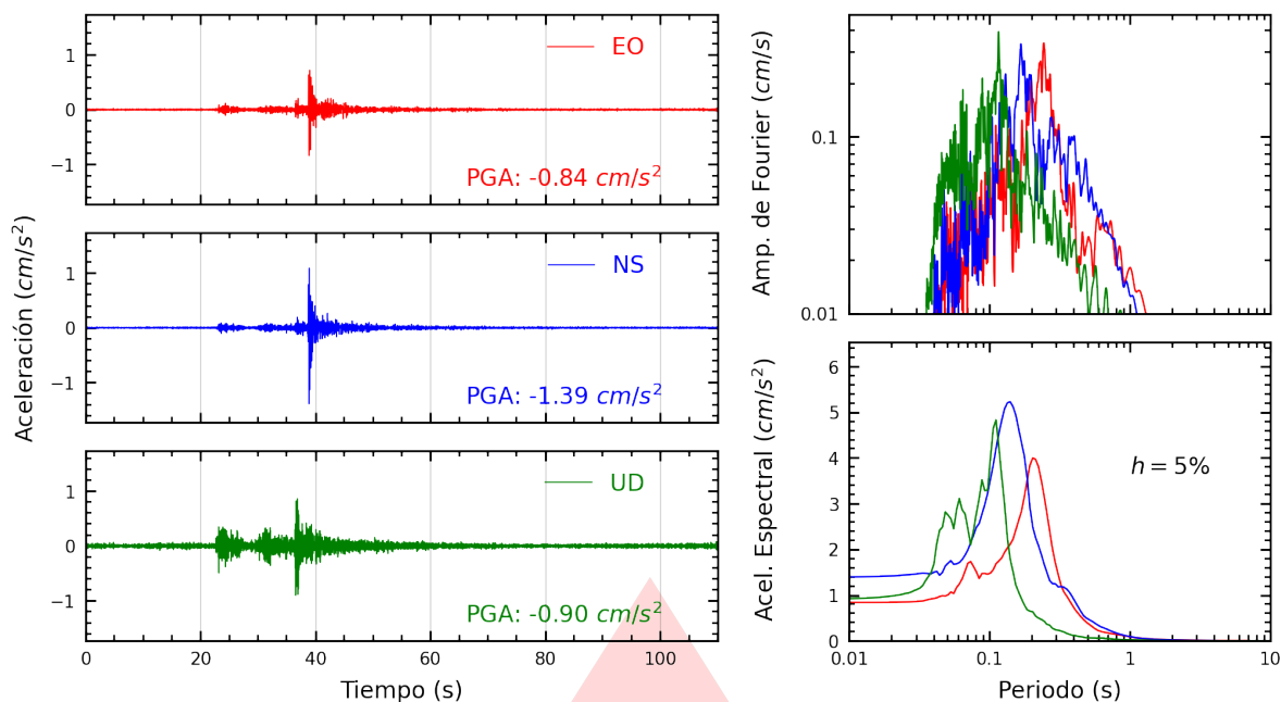
Figura A.1: Registros tiempo-historia, espectros de Fourier y de respuesta en las direcciones EO, NS y vertical de la estación SCPUC. Sismo de Pucallpa, Coronel Portillo - Ucayali del 2026-03-13, 09:22:30 (Hora local)
