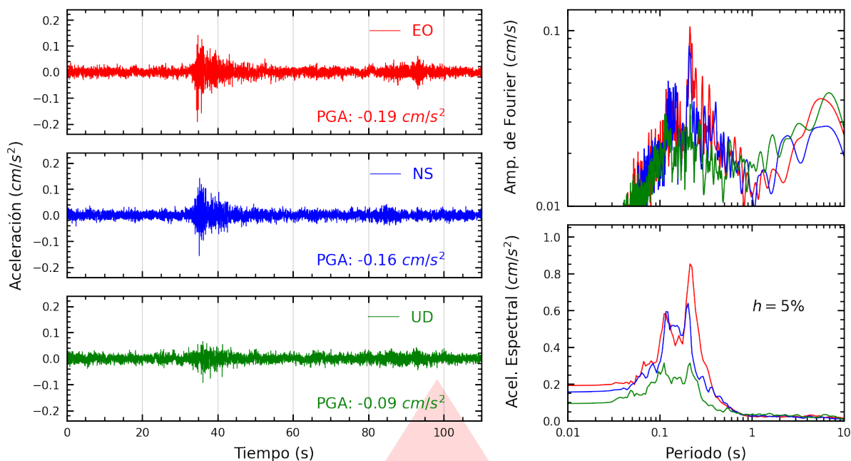
Figura A.3: Registros tiempo-historia, espectros de Fourier y de respuesta en las direcciones EO, NS y vertical de la estación UNTRM. Sismo de Pucallpa, Coronel Portillo - Ucayali del 2026-03-13, 09:22:30 (Hora local)
