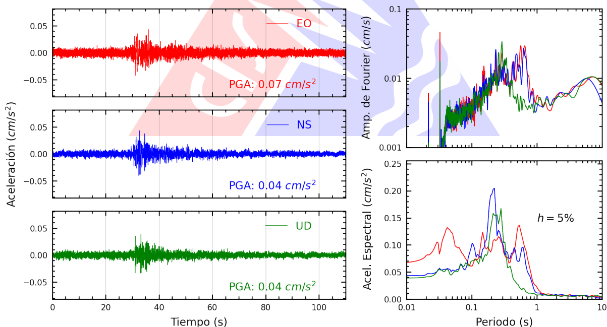
Figura A.4: Registros tiempo-historia, espectros de Fourier y de respuesta en las direcciones EO, NS y vertical de la estación CARAL. Sismo de Pucallpa, Coronel Portillo - Ucayali del 2026-03-13, 09:22:30 (Hora local)
