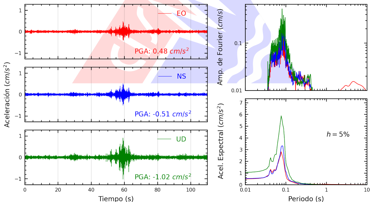
Figura A.2: Registros tiempo-historia, espectros de Fourier y de respuesta en las direcciones EO, NS y vertical de la estación SCICU. Sismo de Pucallpa, Coronel Portillo - Ucayali del 2026-03-13, 09:22:30 (Hora local)
