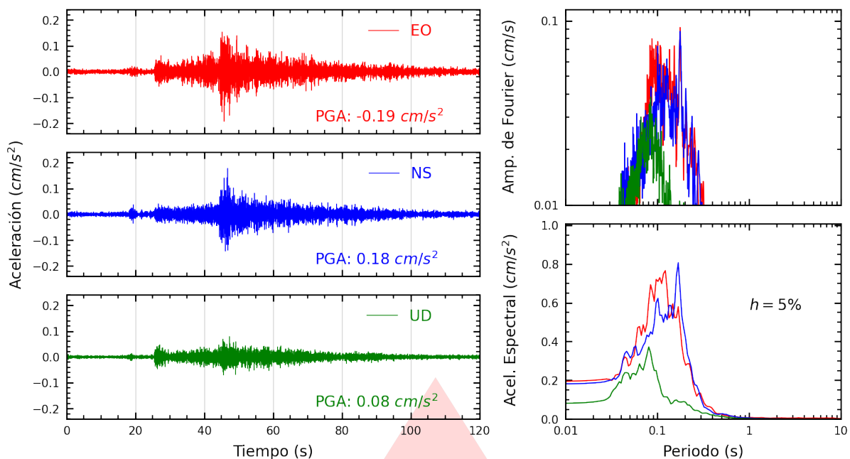
Figura A.3: Registros tiempo-historia, espectros de Fourier y de respuesta en las direcciones EO, NS y vertical de la estación UNAS. Sismo de Pucallpa, Coronel Portillo - Ucayali del 2026-03-16, 11:49:49 (Hora local)
