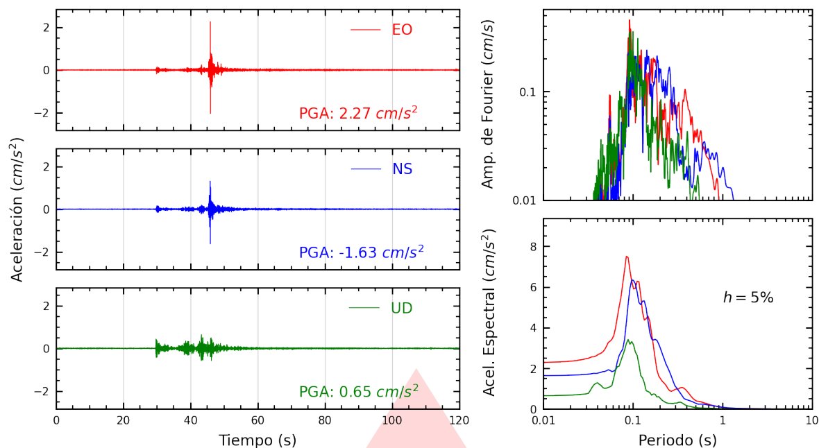
Figura A.1: Registros tiempo-historia, espectros de Fourier y de respuesta en las direcciones EO, NS y vertical de la estación UNIA. Sismo de Pucallpa, Coronel Portillo - Ucayali del 2026-03-16, 11:49:49 (Hora local)
