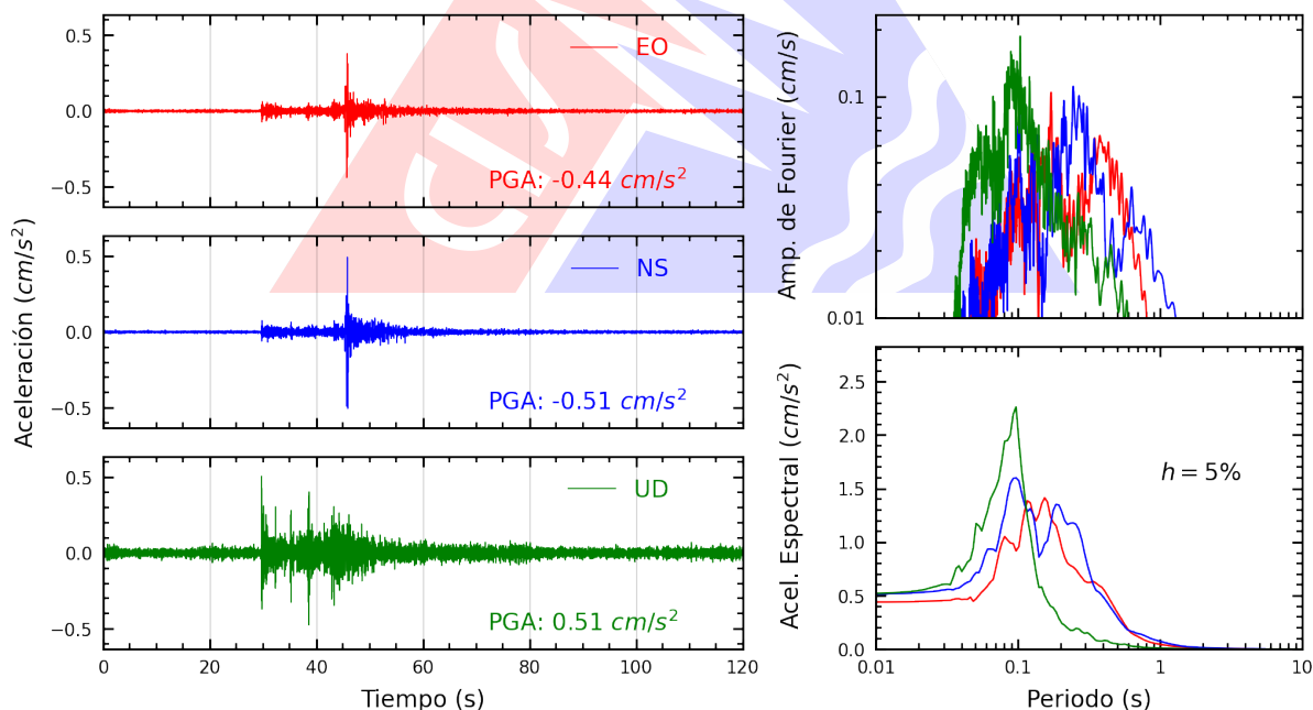
Figura A.2: Registros tiempo-historia, espectros de Fourier y de respuesta en las direcciones EO, NS y vertical de la estación SCPUC. Sismo de Pucallpa, Coronel Portillo - Ucayali del 2026-03-16, 11:49:49 (Hora local)
