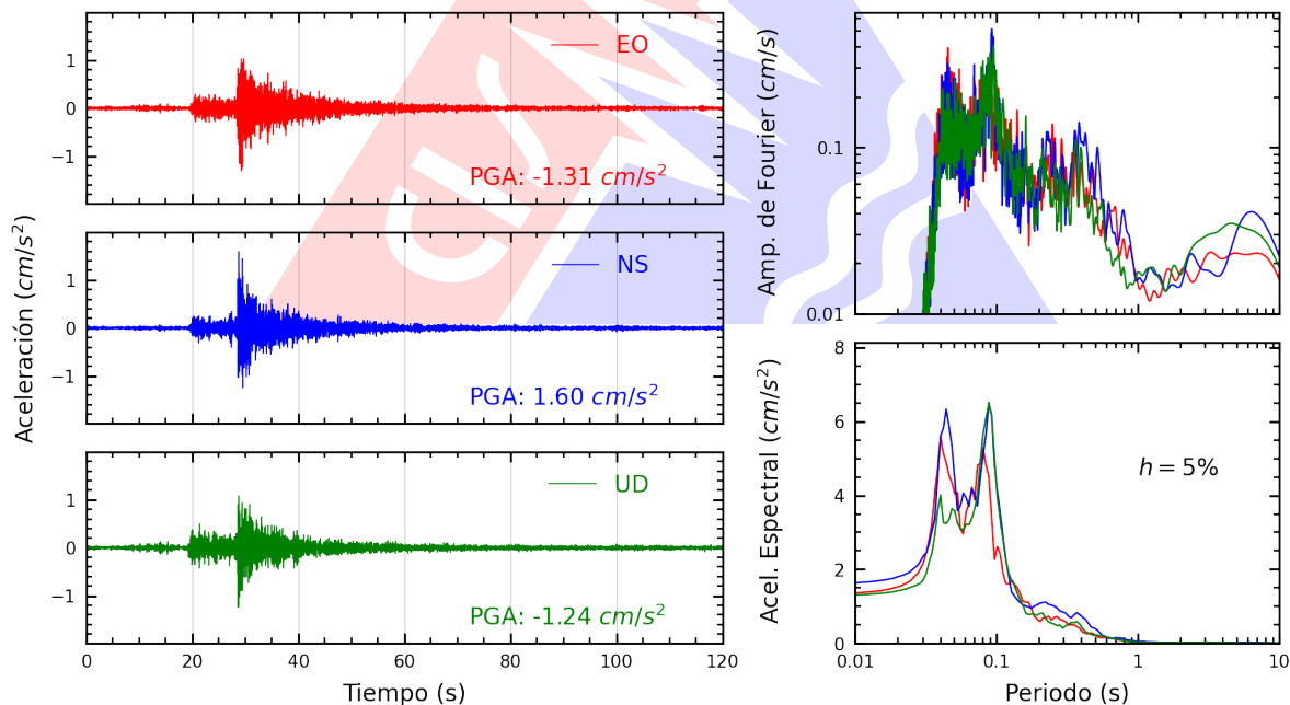
Figura A.8: Registros tiempo-historia, espectros de Fourier y de respuesta en las direcciones EO, NS y vertical de la estación UCVAT. Sismo de Chilca, Cañete - Lima del 2026-03-18, 07:20:06 (Hora local)
