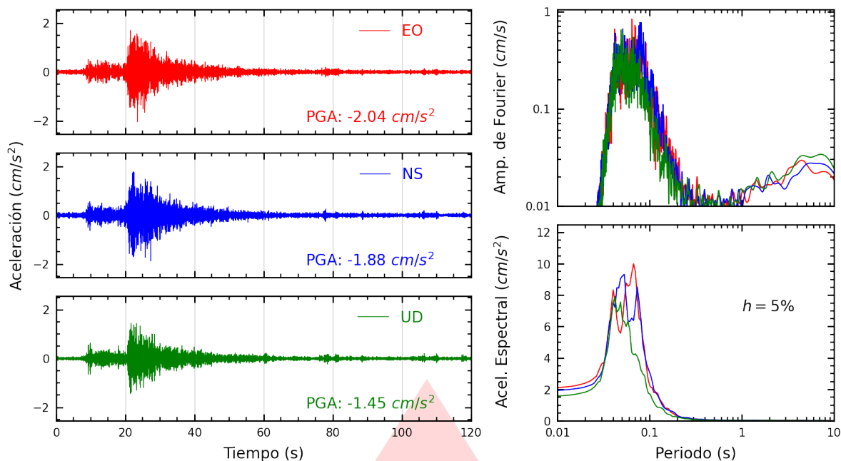
Figura A.5: Registros tiempo-historia, espectros de Fourier y de respuesta en las direcciones EO, NS y vertical de la estación JOSEO. Sismo de Chilca, Cañete - Lima del 2026-03-18, 07:20:06 (Hora local)
