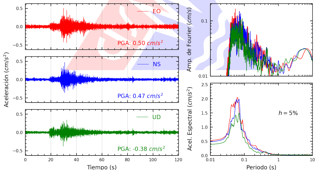
Figura A.26: Registros tiempo-historia, espectros de Fourier y de respuesta en las direcciones EO, NS y vertical de la estación INICT. Sismo de Chilca, Cañete - Lima del 2026-03-18, 07:20:06 (Hora local)
