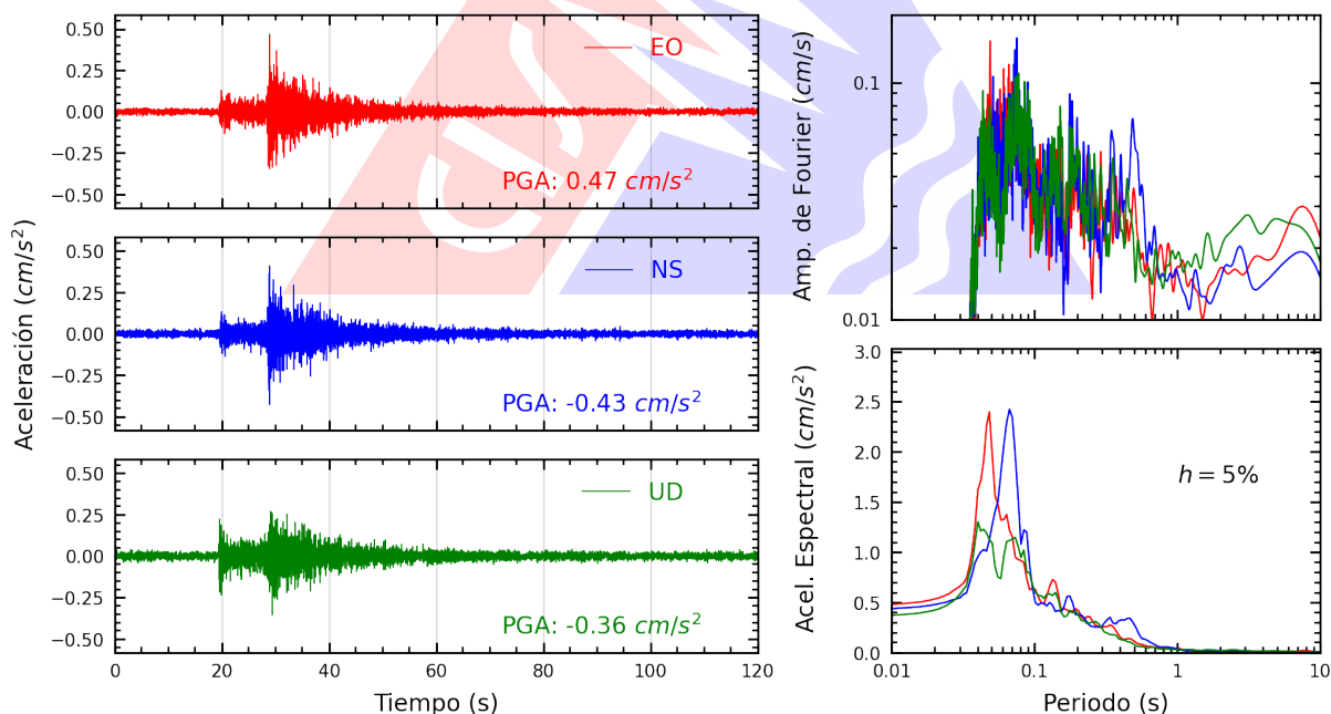
Figura A.28: Registros tiempo-historia, espectros de Fourier y de respuesta en las direcciones EO, NS y vertical de la estación UNFV. Sismo de Chilca, Cañete - Lima del 2026-03-18, 07:20:06 (Hora local)
