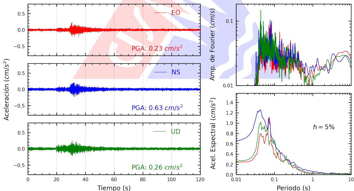
Figura A.24: Registros tiempo-historia, espectros de Fourier y de respuesta en las direcciones EO, NS y vertical de la estación BONDY. Sismo de Chilca, Cañete - Lima del 2026-03-18, 07:20:06 (Hora local)
