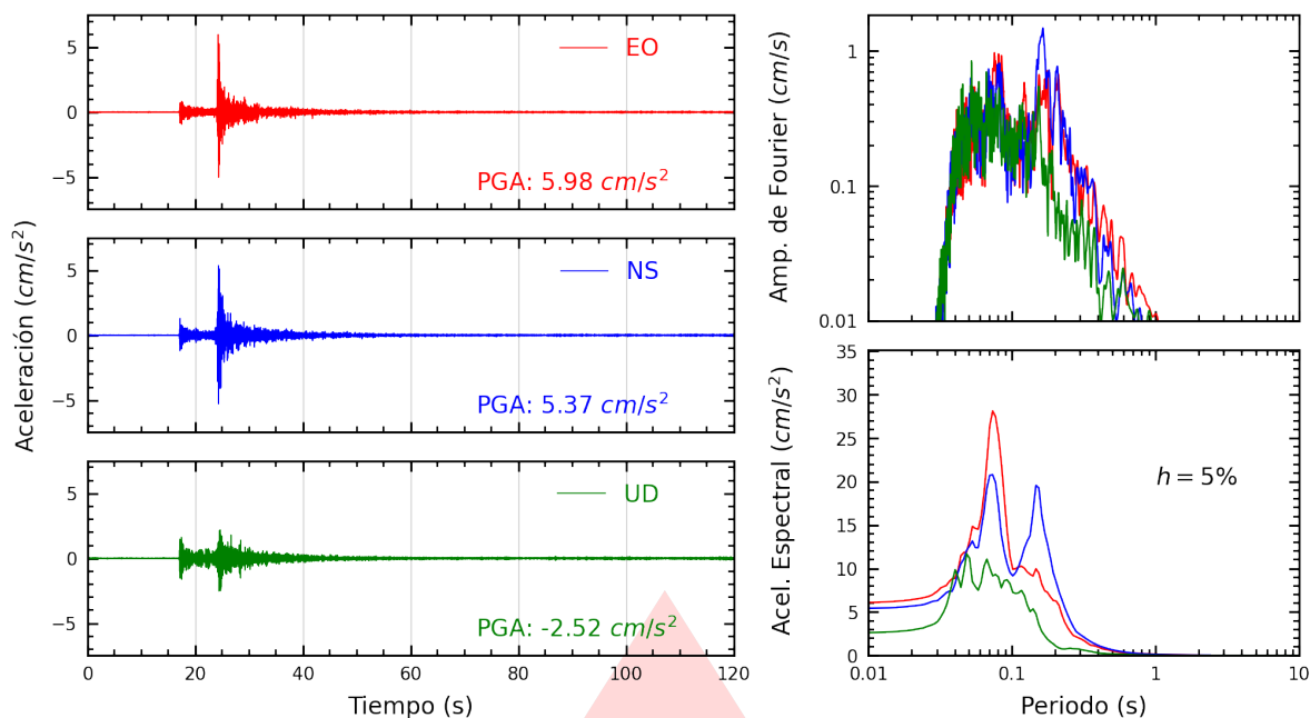
Figura A.1: Registros tiempo-historia, espectros de Fourier y de respuesta en las direcciones EO, NS y vertical de la estación ASIA. Sismo de Chilca, Cañete - Lima del 2026-03-18, 07:20:06 (Hora local)
