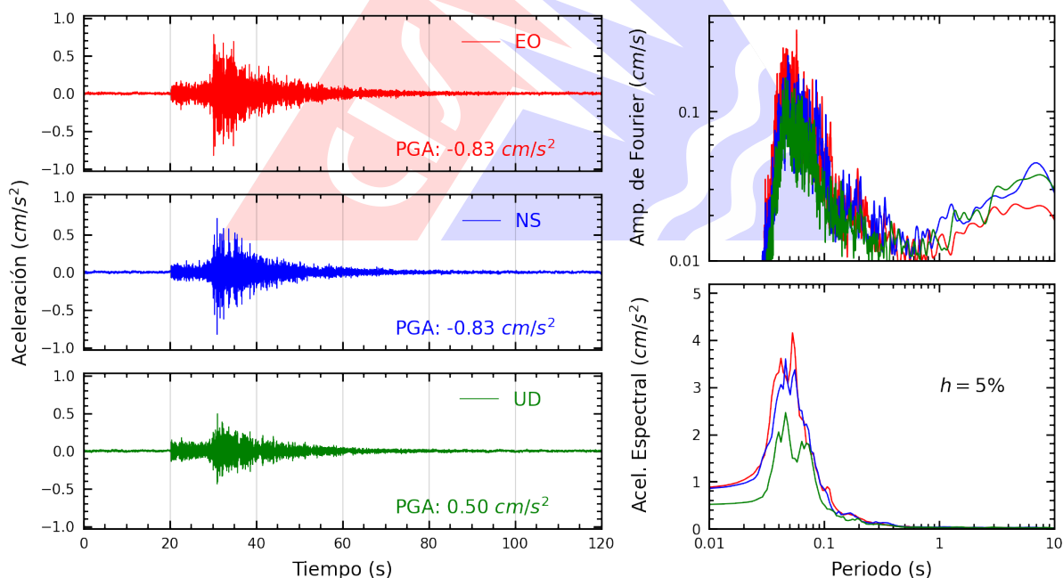
Figura A.18: Registros tiempo-historia, espectros de Fourier y de respuesta en las direcciones EO, NS y vertical de la estación UCSS. Sismo de Chilca, Cañete - Lima del 2026-03-18, 07:20:06 (Hora local)
