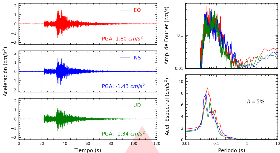
Figura A.7: Registros tiempo-historia, espectros de Fourier y de respuesta en las direcciones EO, NS y vertical de la estación AMORE. Sismo de Chilca, Cañete - Lima del 2026-03-18, 07:20:06 (Hora local)
