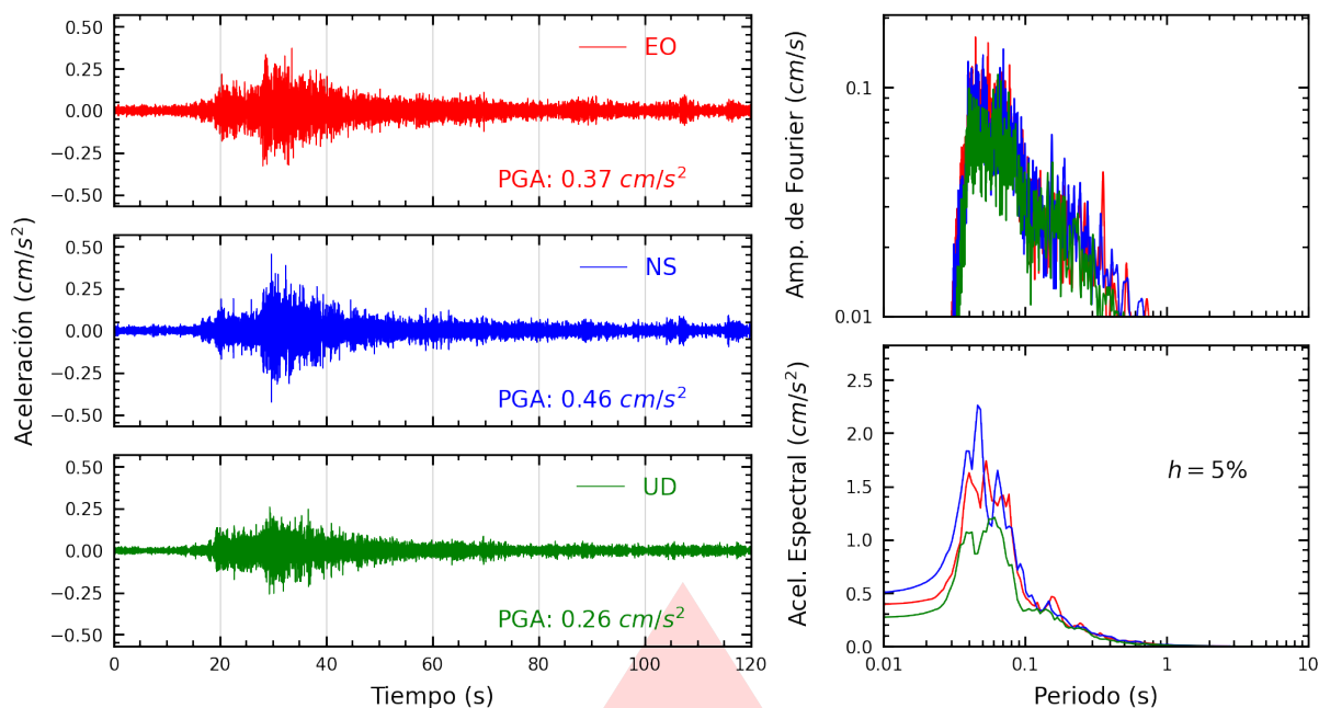
Figura A.29: Registros tiempo-historia, espectros de Fourier y de respuesta en las direcciones EO, NS y vertical de la estación BORJA. Sismo de Chilca, Cañete - Lima del 2026-03-18, 07:20:06 (Hora local)
