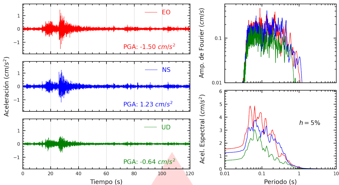
Figura A.9: Registros tiempo-historia, espectros de Fourier y de respuesta en las direcciones EO, NS y vertical de la estación BRISA. Sismo de Chilca, Cañete - Lima del 2026-03-18, 07:20:06 (Hora local)
