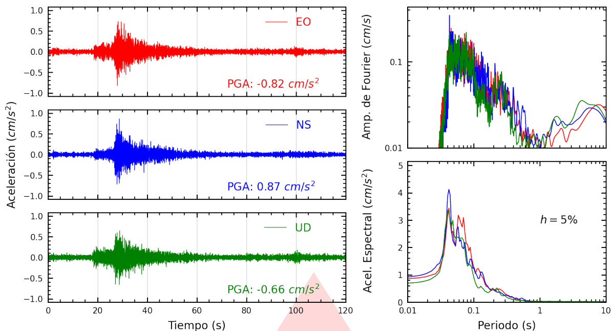
Figura A.17: Registros tiempo-historia, espectros de Fourier y de respuesta en las direcciones EO, NS y vertical de la estación URPPE. Sismo de Chilca, Cañete - Lima del 2026-03-18, 07:20:06 (Hora local)
