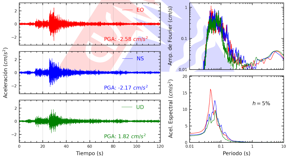
Figura A.4: Registros tiempo-historia, espectros de Fourier y de respuesta en las direcciones EO, NS y vertical de la estación SROSA. Sismo de Chilca, Cañete - Lima del 2026-03-18, 07:20:06 (Hora local)
