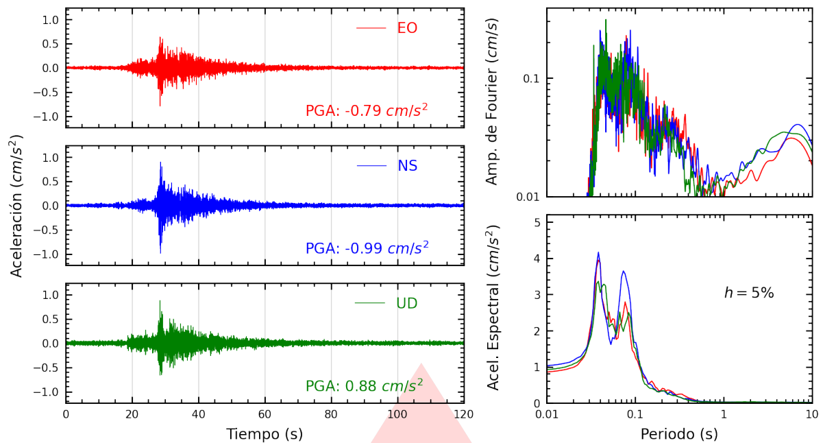
Figura A.15: Registros tiempo-historia, espectros de Fourier y de respuesta en las direcciones EO, NS y vertical de la estación USMP. Sismo de Chilca, Cañete - Lima del 2026-03-18, 07:20:06 (Hora local)
