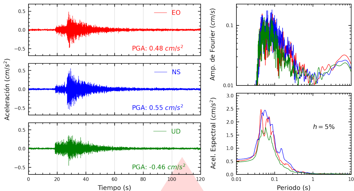
Figura A.25: Registros tiempo-historia, espectros de Fourier y de respuesta en las direcciones EO, NS y vertical de la estación SERVI. Sismo de Chilca, Cañete - Lima del 2026-03-18, 07:20:06 (Hora local)
