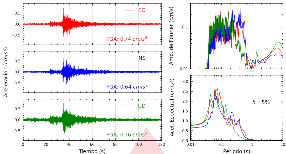
Figura A.19: Registros tiempo-historia, espectros de Fourier y de respuesta en las direcciones EO, NS y vertical de la estación MDPP. Sismo de Chilca, Cañete - Lima del 2026-03-18, 07:20:06 (Hora local)
