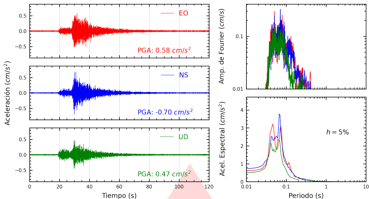
Figura A.21: Registros tiempo-historia, espectros de Fourier y de respuesta en las direcciones EO, NS y vertical de la estación ATARJ. Sismo de Chilca, Cañete - Lima del 2026-03-18, 07:20:06 (Hora local)
