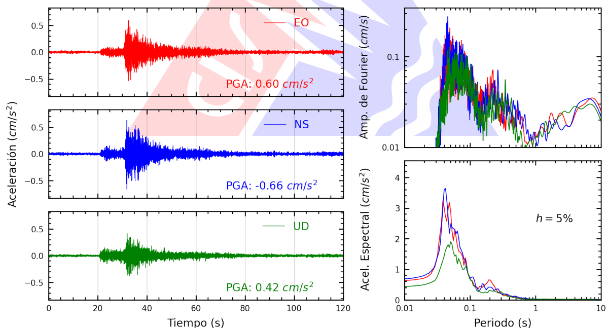
Figura A.22: Registros tiempo-historia, espectros de Fourier y de respuesta en las direcciones EO, NS y vertical de la estación COMAS. Sismo de Chilca, Cañete - Lima del 2026-03-18, 07:20:06 (Hora local)
