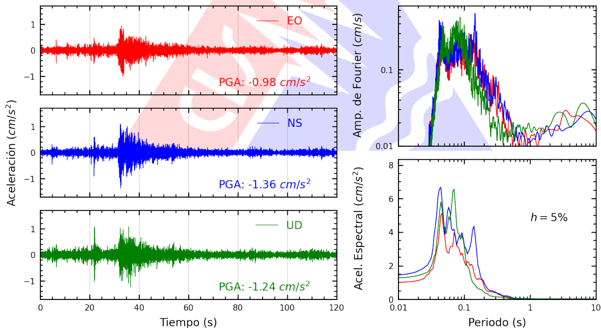
Figura A.10: Registros tiempo-historia, espectros de Fourier y de respuesta en las direcciones EO, NS y vertical de la estación CARAB. Sismo de Chilca, Cañete - Lima del 2026-03-18, 07:20:06 (Hora local)
