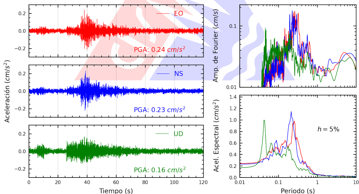
Figura A.30: Registros tiempo-historia, espectros de Fourier y de respuesta en las direcciones EO, NS y vertical de la estación DMSI. Sismo de Chilca, Cañete - Lima del 2026-03-18, 07:20:06 (Hora local)
