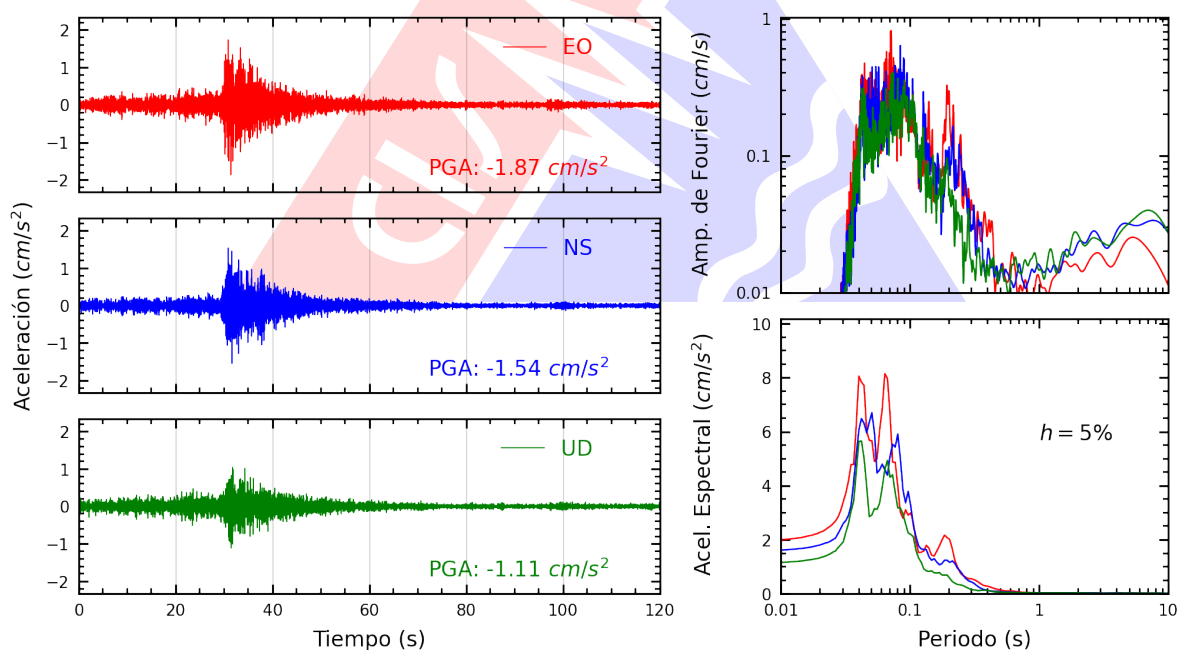
Figura A.6: Registros tiempo-historia, espectros de Fourier y de respuesta en las direcciones EO, NS y vertical de la estación INDEP. Sismo de Chilca, Cañete - Lima del 2026-03-18, 07:20:06 (Hora local)
