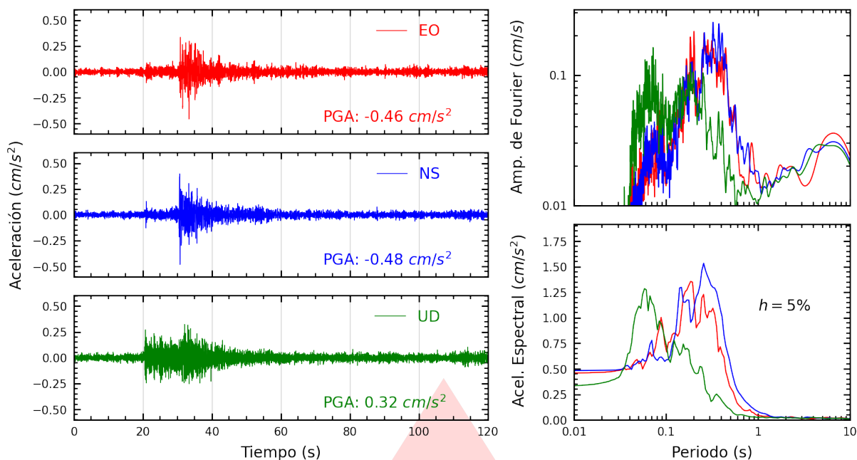
Figura A.27: Registros tiempo-historia, espectros de Fourier y de respuesta en las direcciones EO, NS y vertical de la estación ACAPU. Sismo de Chilca, Cañete - Lima del 2026-03-18, 07:20:06 (Hora local)
