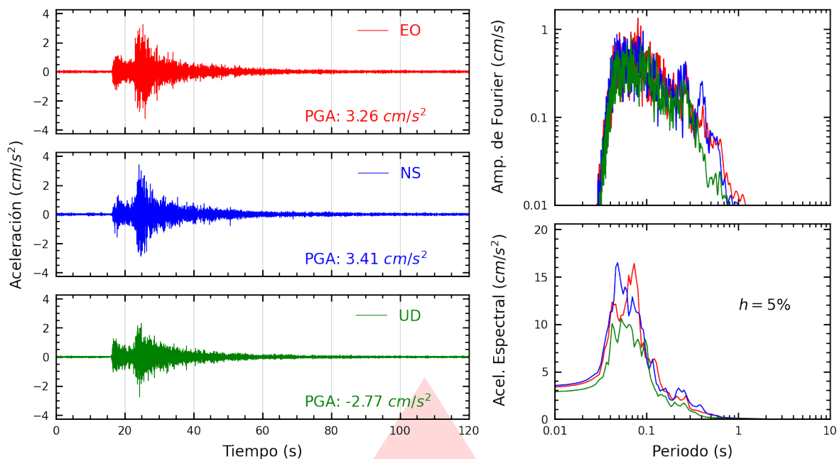
Figura A.3: Registros tiempo-historia, espectros de Fourier y de respuesta en las direcciones EO, NS y vertical de la estación PHERM. Sismo de Chilca, Cañete - Lima del 2026-03-18, 07:20:06 (Hora local)
