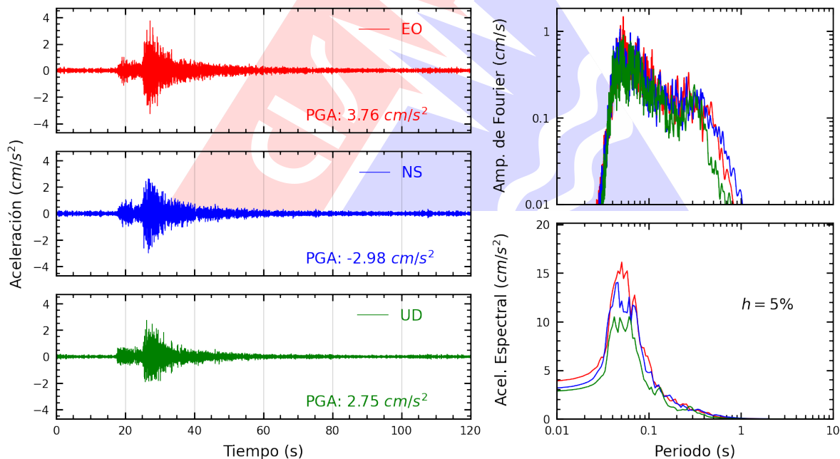
Figura A.2: Registros tiempo-historia, espectros de Fourier y de respuesta en las direcciones EO, NS y vertical de la estación UNTEL. Sismo de Chilca, Cañete - Lima del 2026-03-18, 07:20:06 (Hora local)
