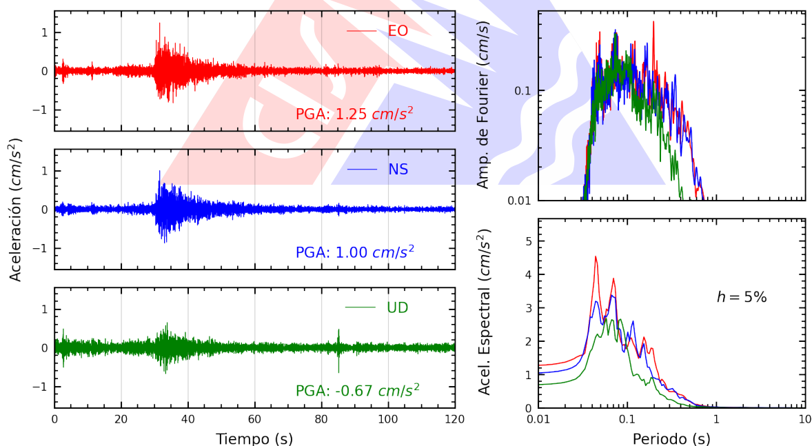
Figura A.12: Registros tiempo-historia, espectros de Fourier y de respuesta en las direcciones EO, NS y vertical de la estación SCOLI. Sismo de Chilca, Cañete - Lima del 2026-03-18, 07:20:06 (Hora local)
