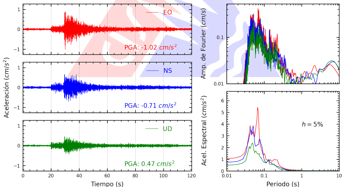
Figura A.14: Registros tiempo-historia, espectros de Fourier y de respuesta en las direcciones EO, NS y vertical de la estación FICPE. Sismo de Chilca, Cañete - Lima del 2026-03-18, 07:20:06 (Hora local)
