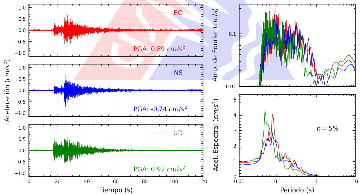
Figura A.16: Registros tiempo-historia, espectros de Fourier y de respuesta en las direcciones EO, NS y vertical de la estación USILP. Sismo de Chilca, Cañete - Lima del 2026-03-18, 07:20:06 (Hora local)
