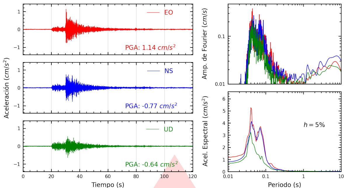
Figura A.13: Registros tiempo-historia, espectros de Fourier y de respuesta en las direcciones EO, NS y vertical de la estación SJLCE. Sismo de Chilca, Cañete - Lima del 2026-03-18, 07:20:06 (Hora local)
