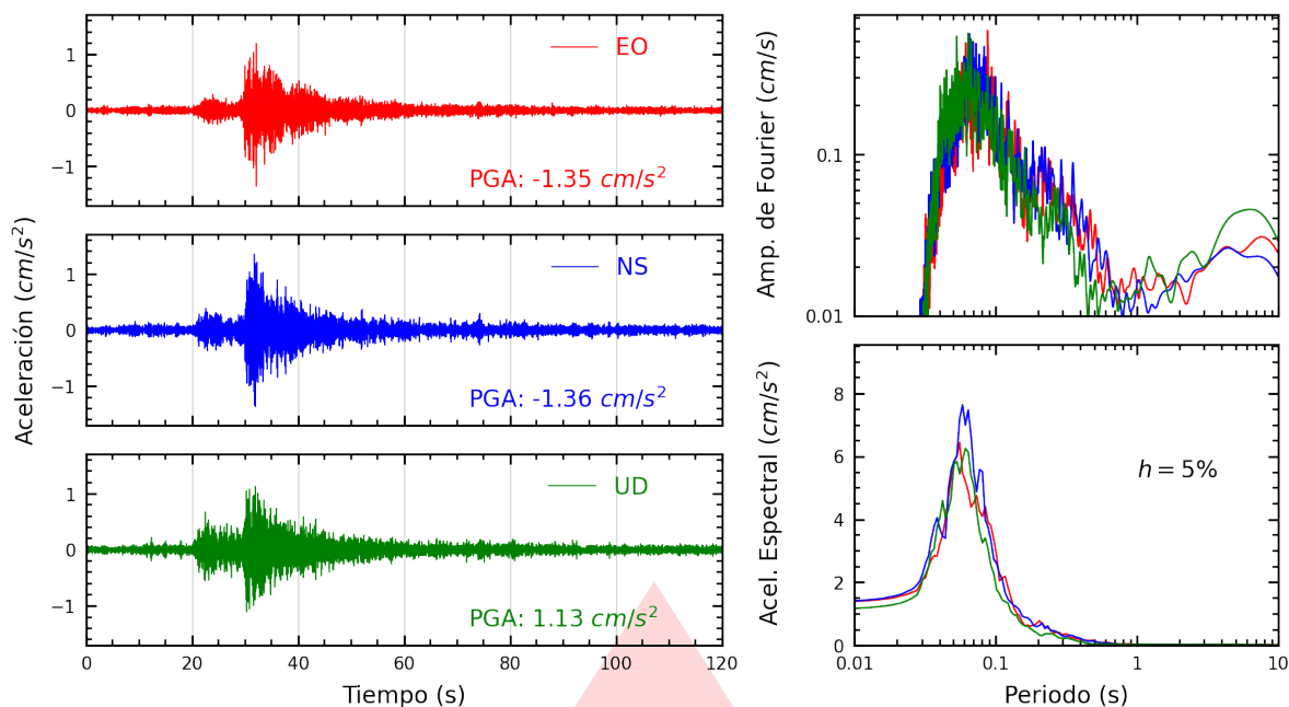
Figura A.11: Registros tiempo-historia, espectros de Fourier y de respuesta en las direcciones EO, NS y vertical de la estación SJLSC. Sismo de Chilca, Cañete - Lima del 2026-03-18, 07:20:06 (Hora local)
