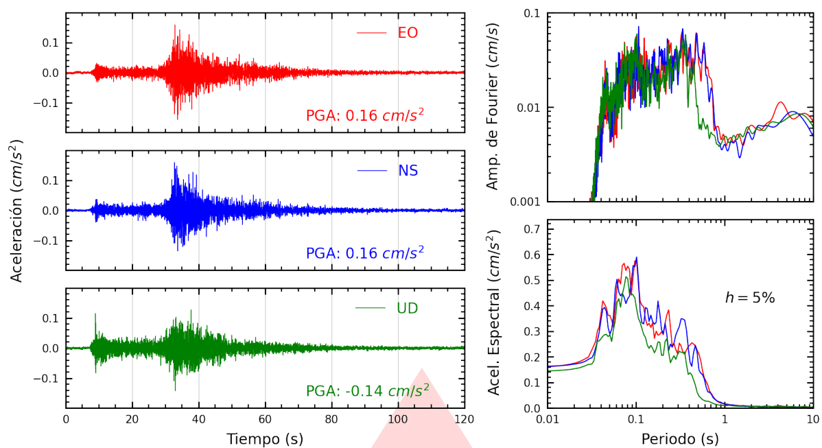
Figura A.31: Registros tiempo-historia, espectros de Fourier y de respuesta en las direcciones EO, NS y vertical de la estación CARAL. Sismo de Chilca, Cañete - Lima del 2026-03-18, 07:20:06 (Hora local)
