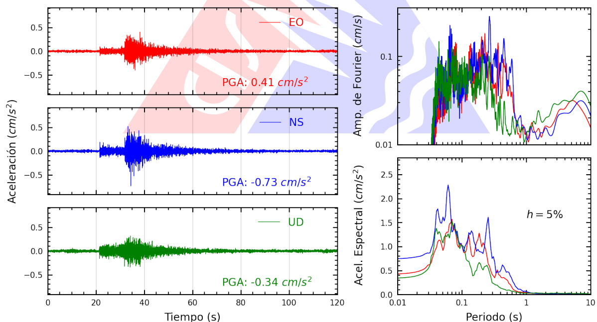
Figura A.20: Registros tiempo-historia, espectros de Fourier y de respuesta en las direcciones EO, NS y vertical de la estación VHAYA. Sismo de Chilca, Cañete - Lima del 2026-03-18, 07:20:06 (Hora local)
