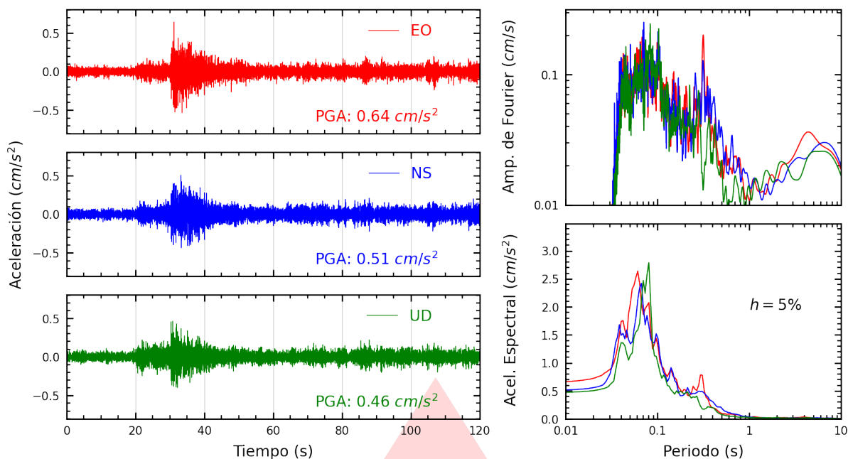
Figura A.23: Registros tiempo-historia, espectros de Fourier y de respuesta en las direcciones EO, NS y vertical de la estación MADRE. Sismo de Chilca, Cañete - Lima del 2026-03-18, 07:20:06 (Hora local)
