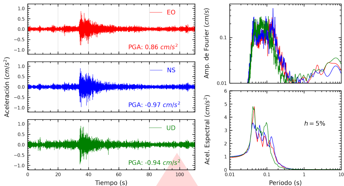
Figura A.13: Registros tiempo-historia, espectros de Fourier y de respuesta en las direcciones EO, NS y vertical de la estación CARAB. Sismo de Chilca, Cañete - Lima del 2026-03-18, 13:04:38 (Hora local)
