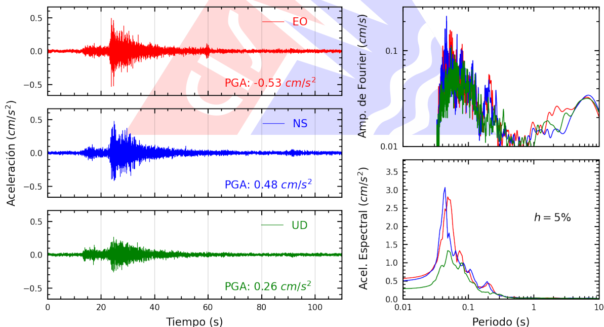
Figura A.20: Registros tiempo-historia, espectros de Fourier y de respuesta en las direcciones EO, NS y vertical de la estación COMAS. Sismo de Chilca, Cañete - Lima del 2026-03-18, 13:04:38 (Hora local)
