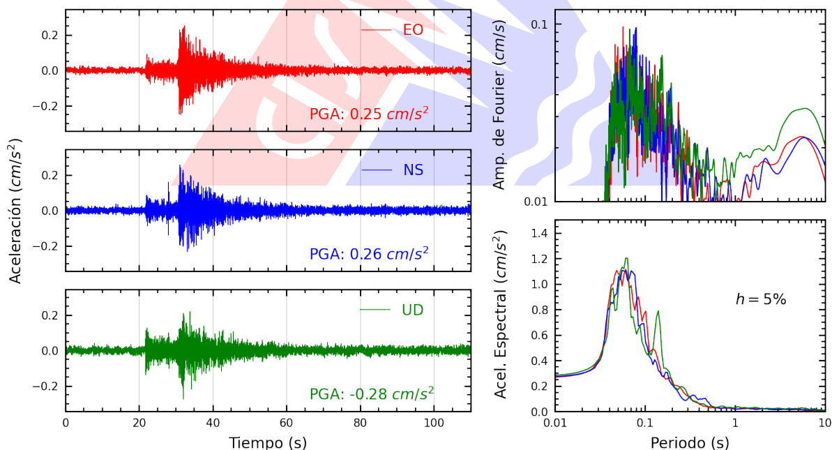
Figura A.26: Registros tiempo-historia, espectros de Fourier y de respuesta en las direcciones EO, NS y vertical de la estación UNFV. Sismo de Chilca, Cañete - Lima del 2026-03-18, 13:04:38 (Hora local)
