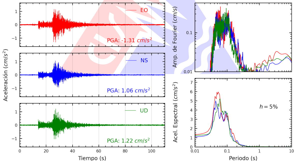
Figura A.8: Registros tiempo-historia, espectros de Fourier y de respuesta en las direcciones EO, NS y vertical de la estación AMORE. Sismo de Chilca, Cañete - Lima del 2026-03-18, 13:04:38 (Hora local)
