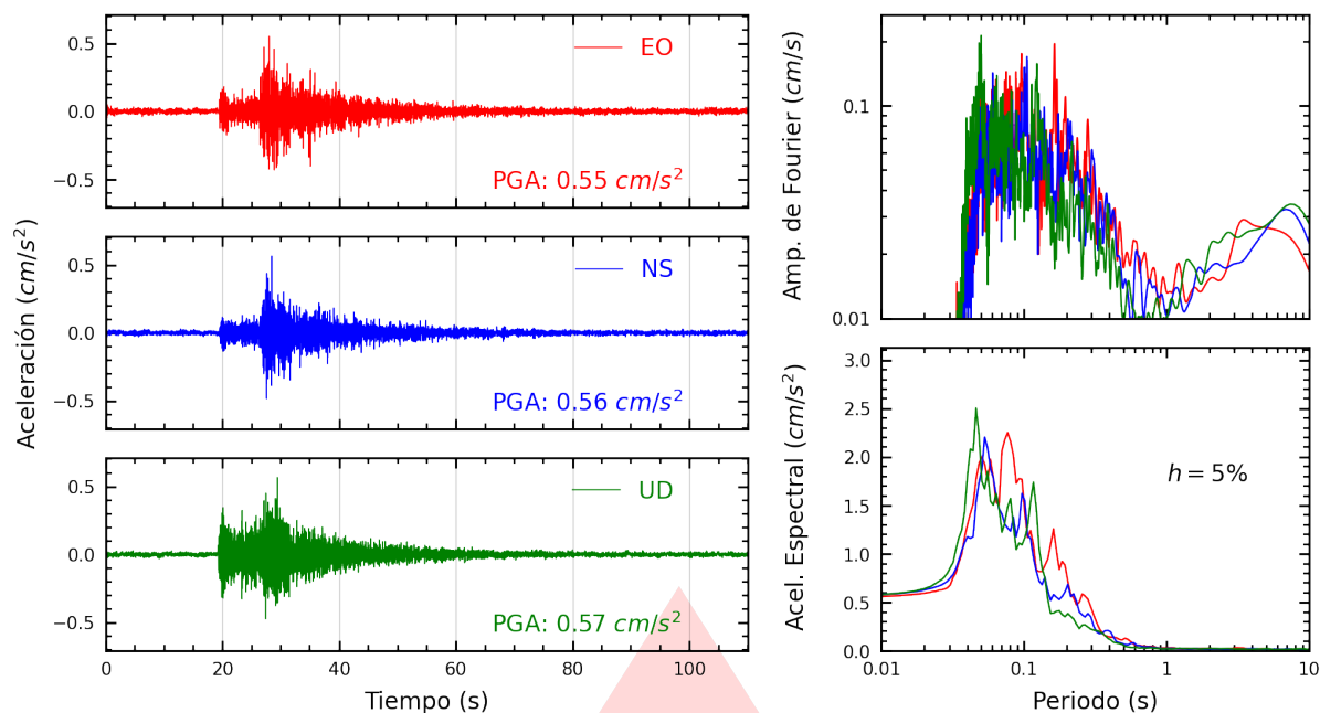
Figura A.17: Registros tiempo-historia, espectros de Fourier y de respuesta en las direcciones EO, NS y vertical de la estación USILP. Sismo de Chilca, Cañete - Lima del 2026-03-18, 13:04:38 (Hora local)
