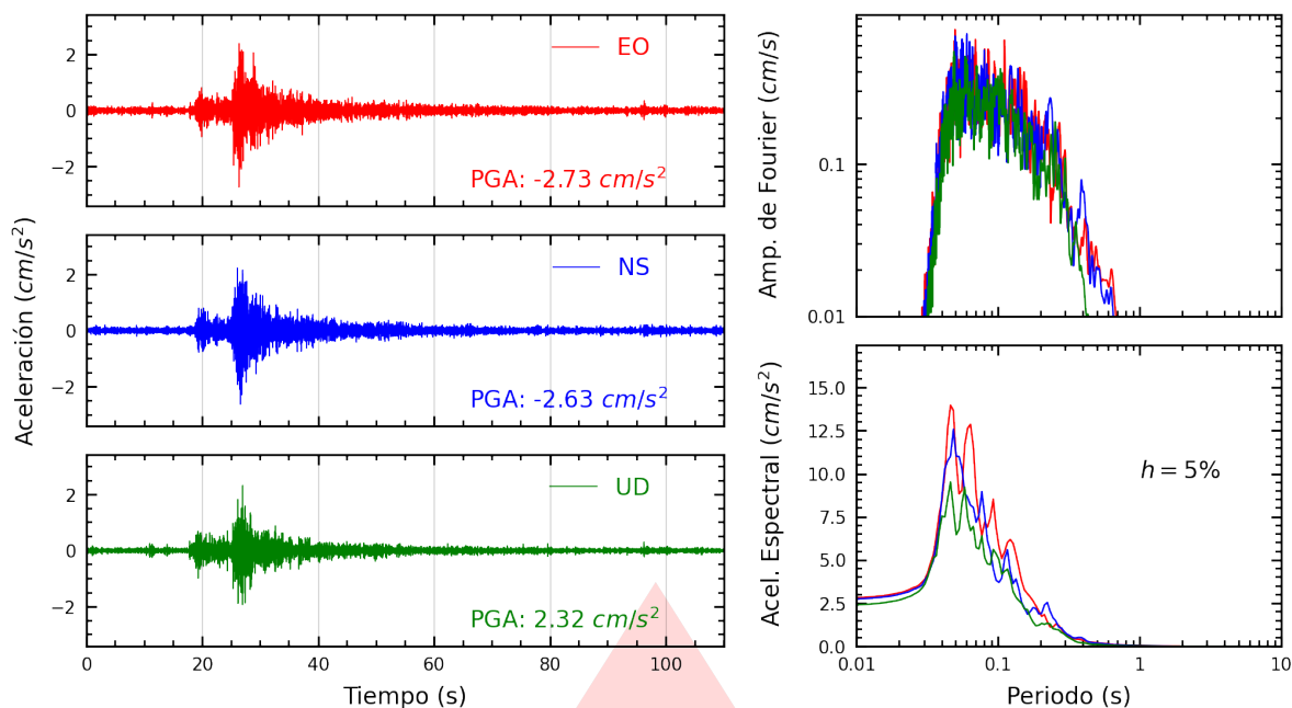
Figura A.1: Registros tiempo-historia, espectros de Fourier y de respuesta en las direcciones EO, NS y vertical de la estación PHERM. Sismo de Chilca, Cañete - Lima del 2026-03-18, 13:04:38 (Hora local)
