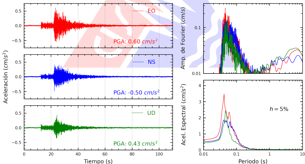
Figura A.16: Registros tiempo-historia, espectros de Fourier y de respuesta en las direcciones EO, NS y vertical de la estación UCSS. Sismo de Chilca, Cañete - Lima del 2026-03-18, 13:04:38 (Hora local)
