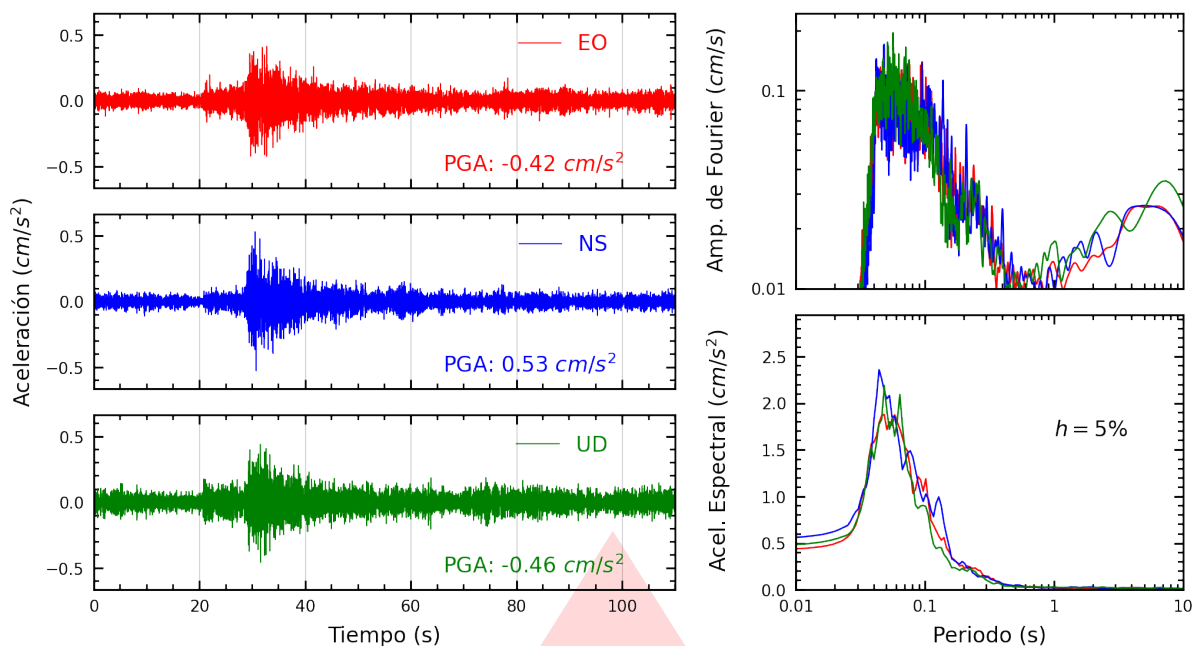
Figura A.19: Registros tiempo-historia, espectros de Fourier y de respuesta en las direcciones EO, NS y vertical de la estación URPPE. Sismo de Chilca, Cañete - Lima del 2026-03-18, 13:04:38 (Hora local)
