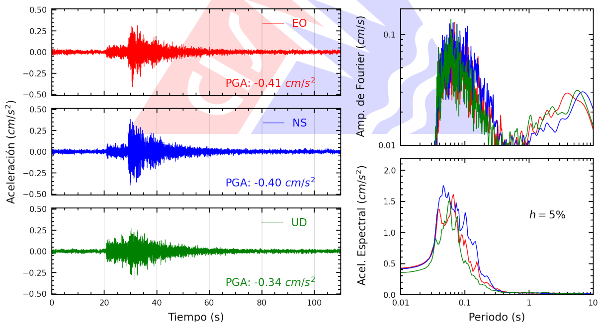
Figura A.22: Registros tiempo-historia, espectros de Fourier y de respuesta en las direcciones EO, NS y vertical de la estación SERVI. Sismo de Chilca, Cañete - Lima del 2026-03-18, 13:04:38 (Hora local)
