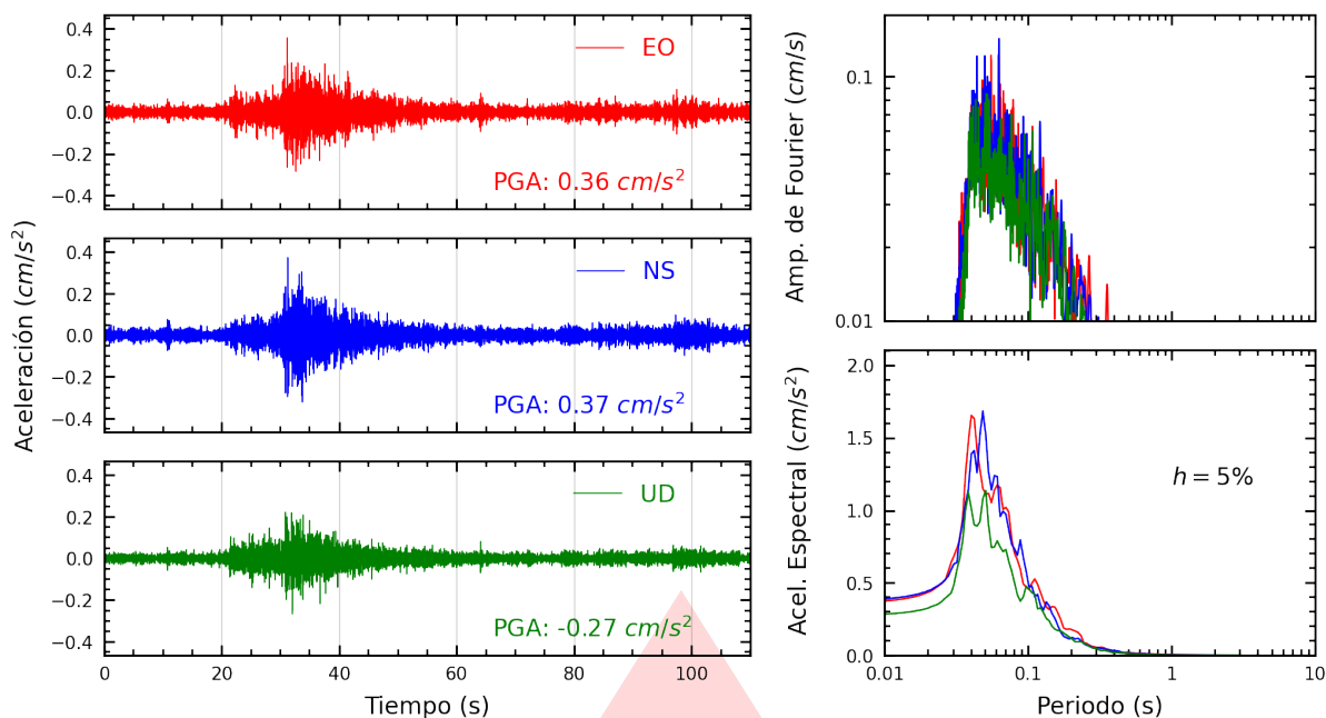
Figura A.23: Registros tiempo-historia, espectros de Fourier y de respuesta en las direcciones EO, NS y vertical de la estación BORJA. Sismo de Chilca, Cañete - Lima del 2026-03-18, 13:04:38 (Hora local)
