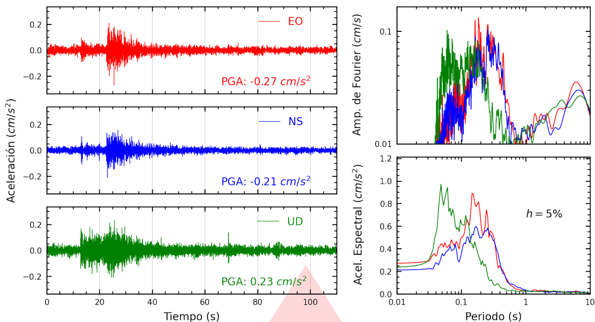
Figura A.27: Registros tiempo-historia, espectros de Fourier y de respuesta en las direcciones EO, NS y vertical de la estación ACAPU. Sismo de Chilca, Cañete - Lima del 2026-03-18, 13:04:38 (Hora local)
