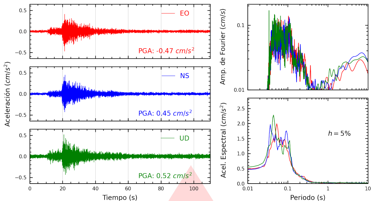
Figura A.21: Registros tiempo-historia, espectros de Fourier y de respuesta en las direcciones EO, NS y vertical de la estación USMP. Sismo de Chilca, Cañete - Lima del 2026-03-18, 13:04:38 (Hora local)
