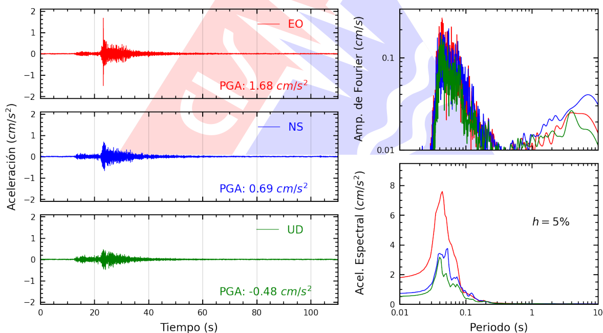
Figura A.6: Registros tiempo-historia, espectros de Fourier y de respuesta en las direcciones EO, NS y vertical de la estación SJLCE. Sismo de Chilca, Cañete - Lima del 2026-03-18, 13:04:38 (Hora local)
