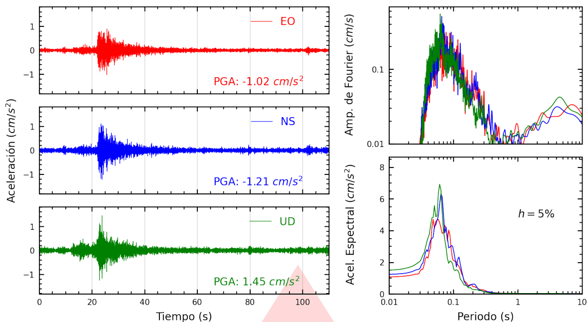
Figura A.7: Registros tiempo-historia, espectros de Fourier y de respuesta en las direcciones EO, NS y vertical de la estación SJLSC. Sismo de Chilca, Cañete - Lima del 2026-03-18, 13:04:38 (Hora local)
