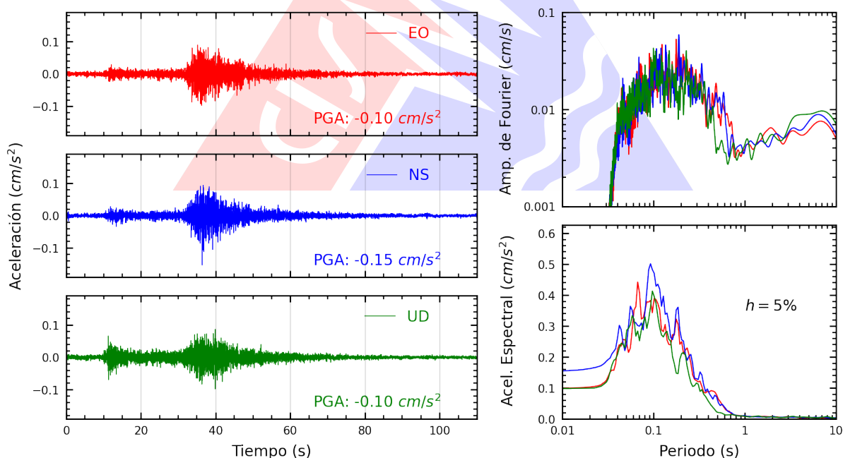
Figura A.28: Registros tiempo-historia, espectros de Fourier y de respuesta en las direcciones EO, NS y vertical de la estación CARAL. Sismo de Chilca, Cañete - Lima del 2026-03-18, 13:04:38 (Hora local)
