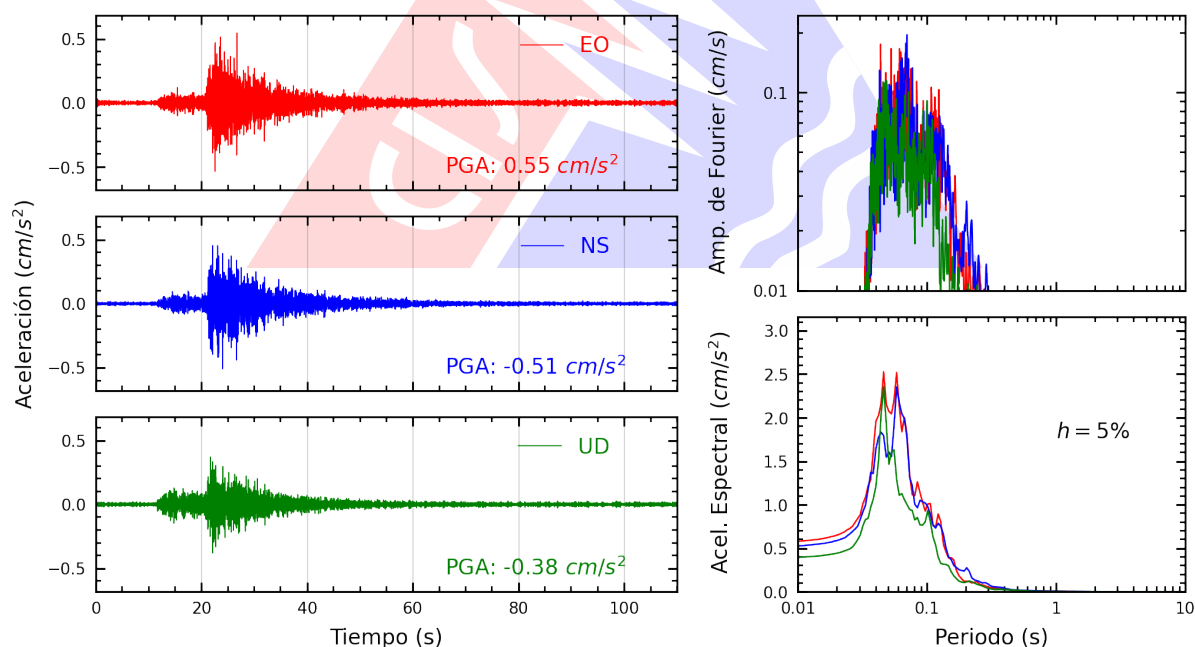
Figura A.18: Registros tiempo-historia, espectros de Fourier y de respuesta en las direcciones EO, NS y vertical de la estación ATARJ. Sismo de Chilca, Cañete - Lima del 2026-03-18, 13:04:38 (Hora local)
