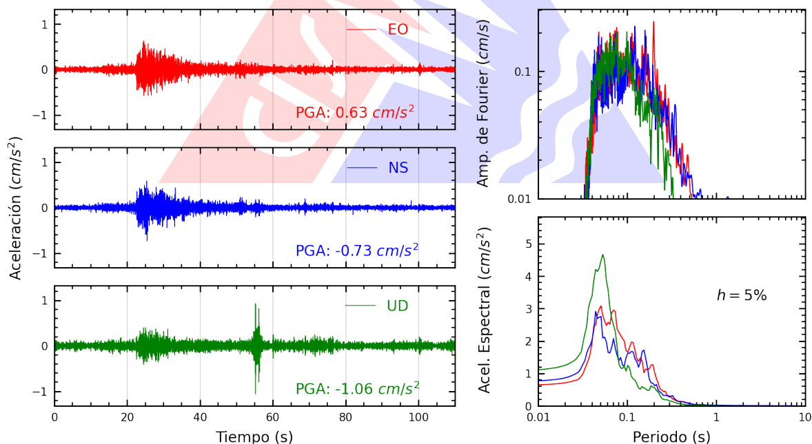
Figura A.12: Registros tiempo-historia, espectros de Fourier y de respuesta en las direcciones EO, NS y vertical de la estación SCOLI. Sismo de Chilca, Cañete - Lima del 2026-03-18, 13:04:38 (Hora local)
