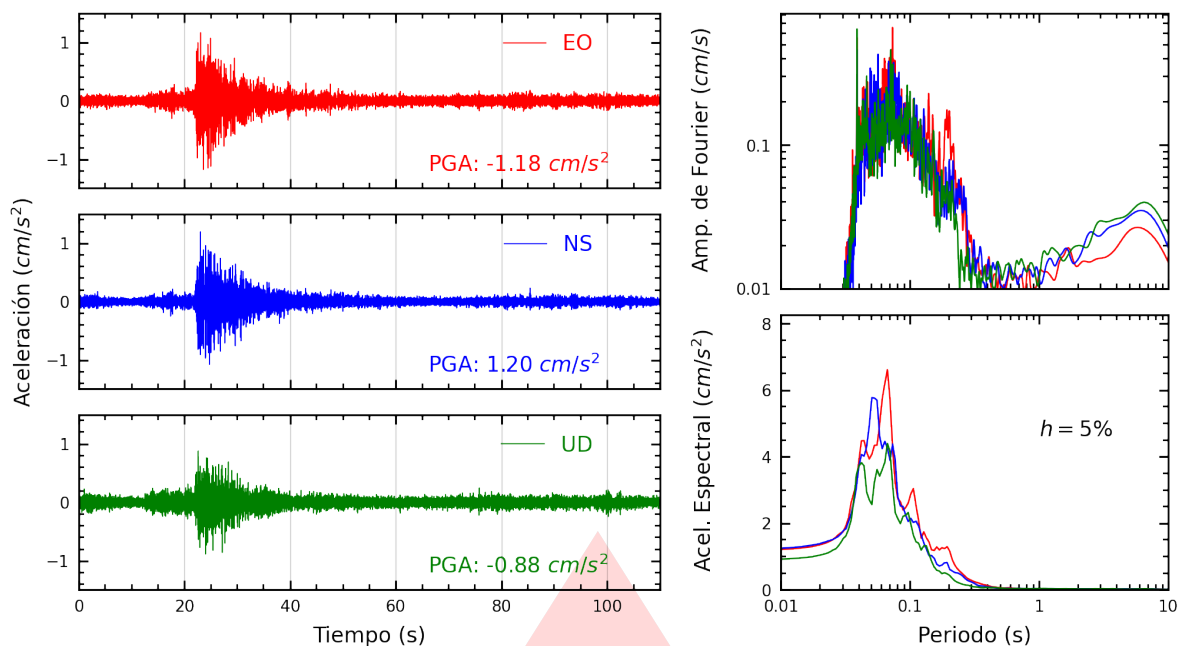
Figura A.9: Registros tiempo-historia, espectros de Fourier y de respuesta en las direcciones EO, NS y vertical de la estación INDEP. Sismo de Chilca, Cañete - Lima del 2026-03-18, 13:04:38 (Hora local)
