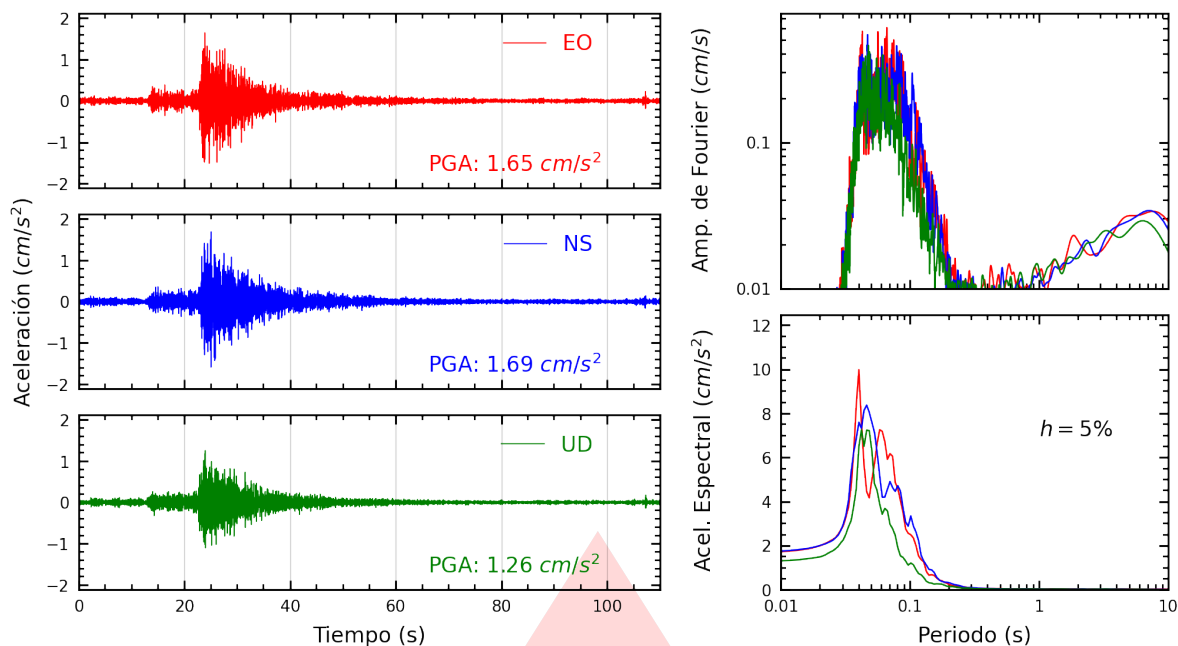
Figura A.5: Registros tiempo-historia, espectros de Fourier y de respuesta en las direcciones EO, NS y vertical de la estación JOSEO. Sismo de Chilca, Cañete - Lima del 2026-03-18, 13:04:38 (Hora local)
