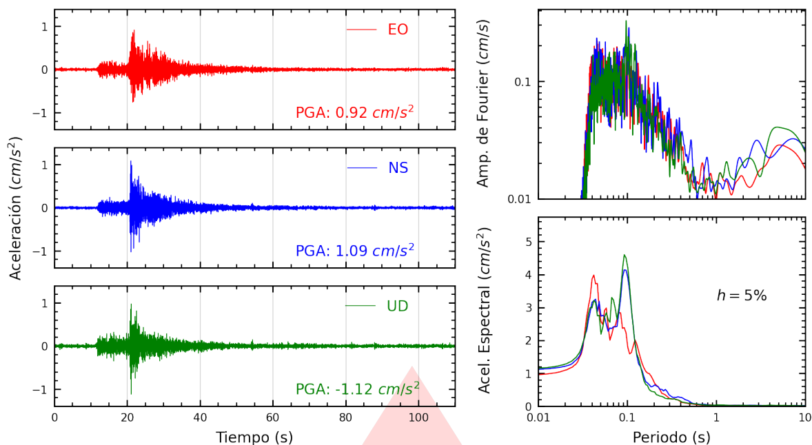
Figura A.11: Registros tiempo-historia, espectros de Fourier y de respuesta en las direcciones EO, NS y vertical de la estación UCVAT. Sismo de Chilca, Cañete - Lima del 2026-03-18, 13:04:38 (Hora local)
