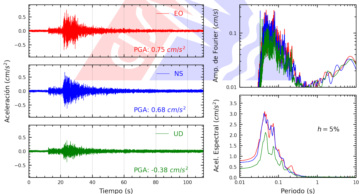
Figura A.14: Registros tiempo-historia, espectros de Fourier y de respuesta en las direcciones EO, NS y vertical de la estación FICPE. Sismo de Chilca, Cañete - Lima del 2026-03-18, 13:04:38 (Hora local)
