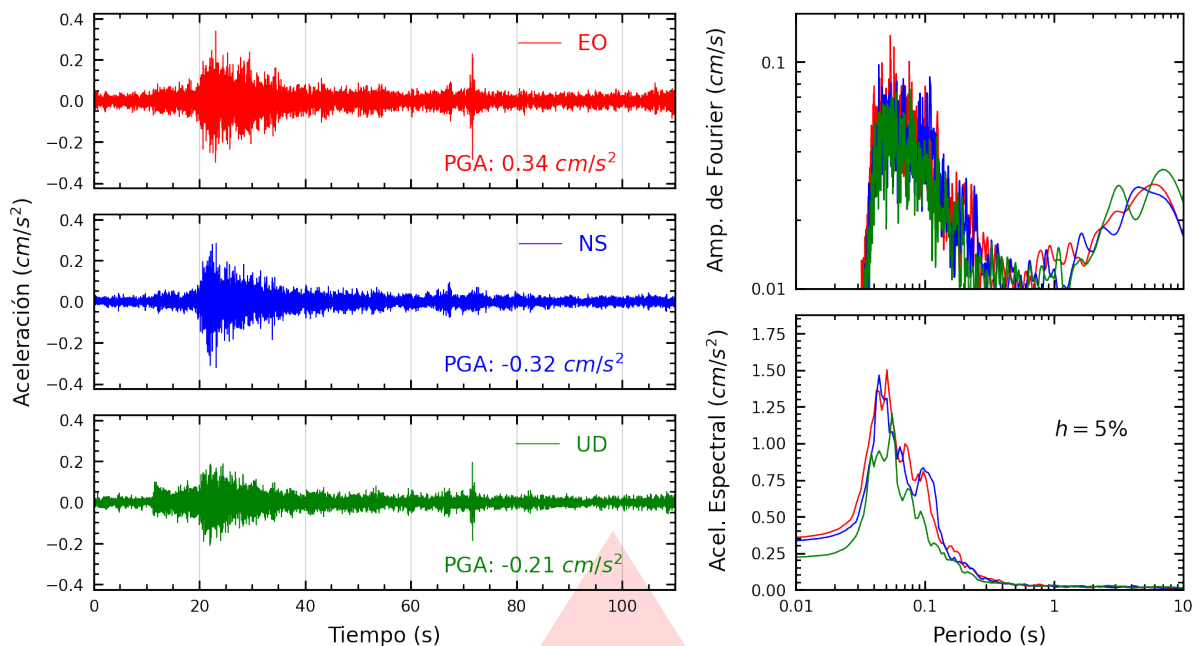
Figura A.25: Registros tiempo-historia, espectros de Fourier y de respuesta en las direcciones EO, NS y vertical de la estación INICT. Sismo de Chilca, Cañete - Lima del 2026-03-18, 13:04:38 (Hora local)
