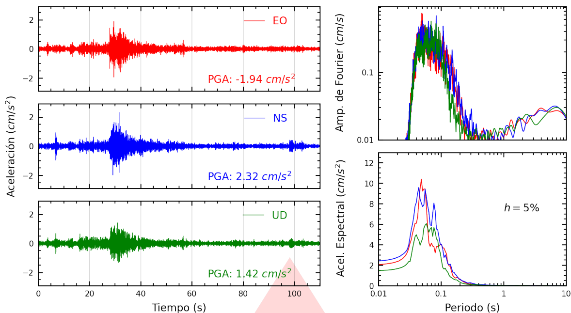
Figura A.3: Registros tiempo-historia, espectros de Fourier y de respuesta en las direcciones EO, NS y vertical de la estación SROSA. Sismo de Chilca, Cañete - Lima del 2026-03-18, 13:04:38 (Hora local)
