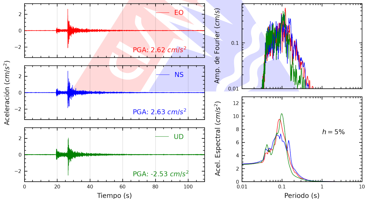
Figura A.2: Registros tiempo-historia, espectros de Fourier y de respuesta en las direcciones EO, NS y vertical de la estación ASIA. Sismo de Chilca, Cañete - Lima del 2026-03-18, 13:04:38 (Hora local)
