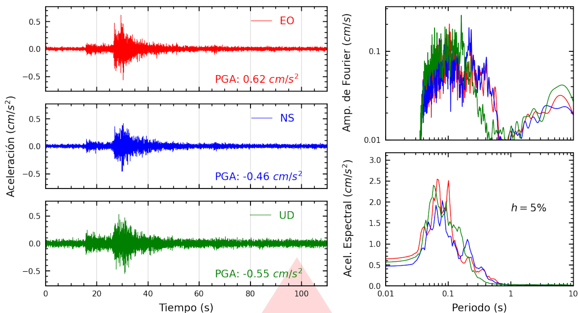
Figura A.15: Registros tiempo-historia, espectros de Fourier y de respuesta en las direcciones EO, NS y vertical de la estación MDPP. Sismo de Chilca, Cañete - Lima del 2026-03-18, 13:04:38 (Hora local)
