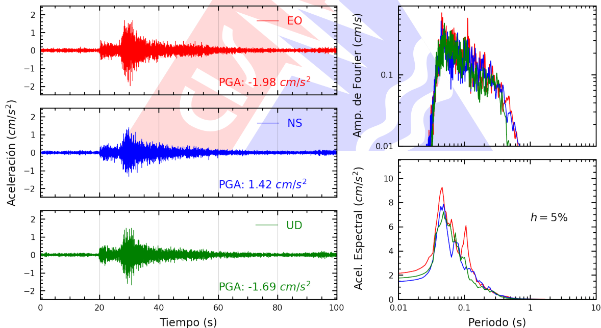
Figura A.4: Registros tiempo-historia, espectros de Fourier y de respuesta en las direcciones EO, NS y vertical de la estación UNTEL. Sismo de Chilca, Cañete - Lima del 2026-03-18, 13:04:38 (Hora local)
