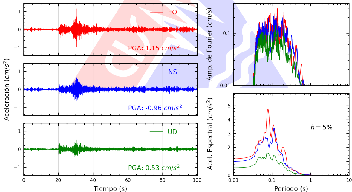
Figura A.10: Registros tiempo-historia, espectros de Fourier y de respuesta en las direcciones EO, NS y vertical de la estación BRISA. Sismo de Chilca, Cañete - Lima del 2026-03-18, 13:04:38 (Hora local)
