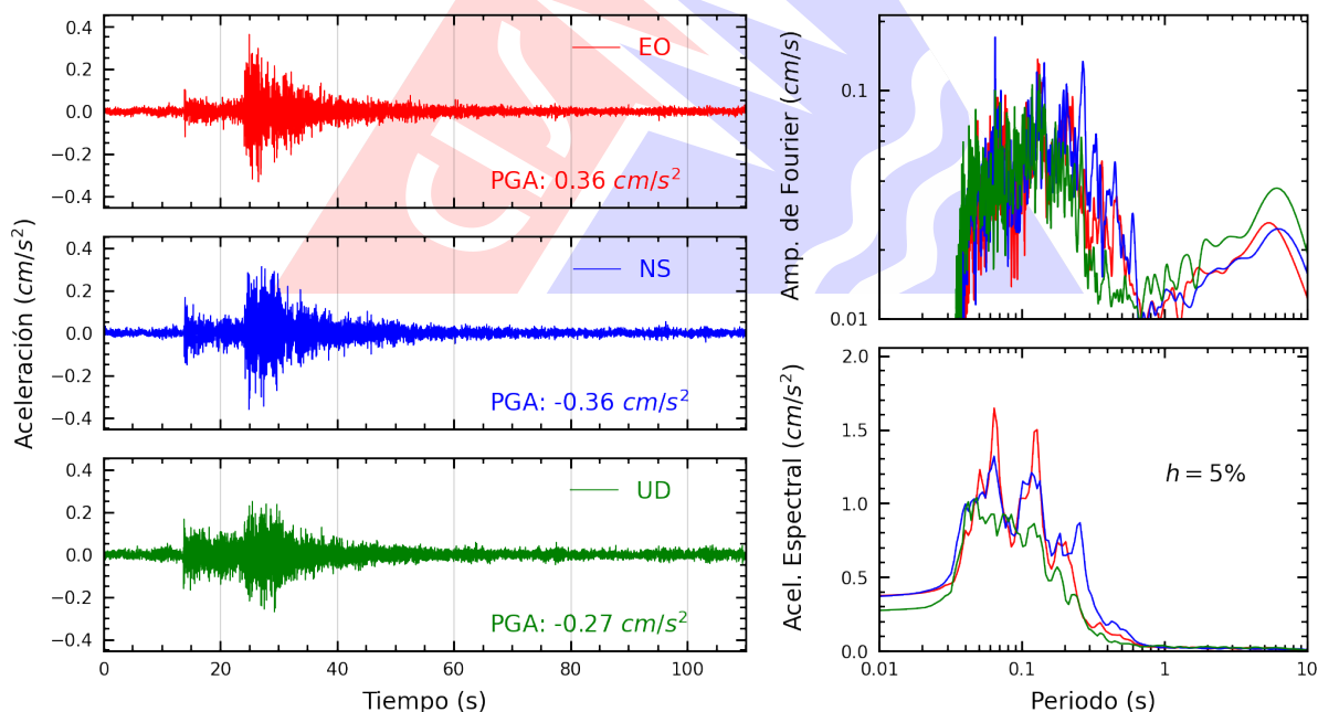
Figura A.24: Registros tiempo-historia, espectros de Fourier y de respuesta en las direcciones EO, NS y vertical de la estación VHAYA. Sismo de Chilca, Cañete - Lima del 2026-03-18, 13:04:38 (Hora local)
