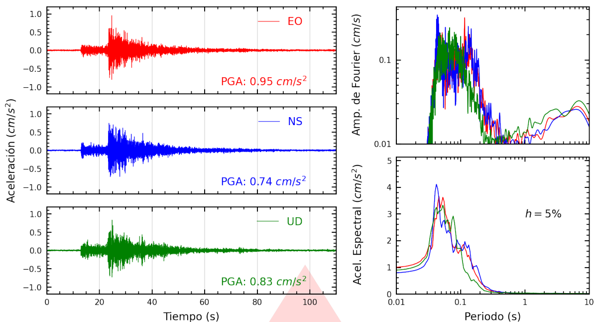
Figura A.13: Registros tiempo-historia, espectros de Fourier y de respuesta en las direcciones EO, NS y vertical de la estación CARAB. Sismo de Chilca, Cañete - Lima del 2026-03-19, 03:27:47 (Hora local)
