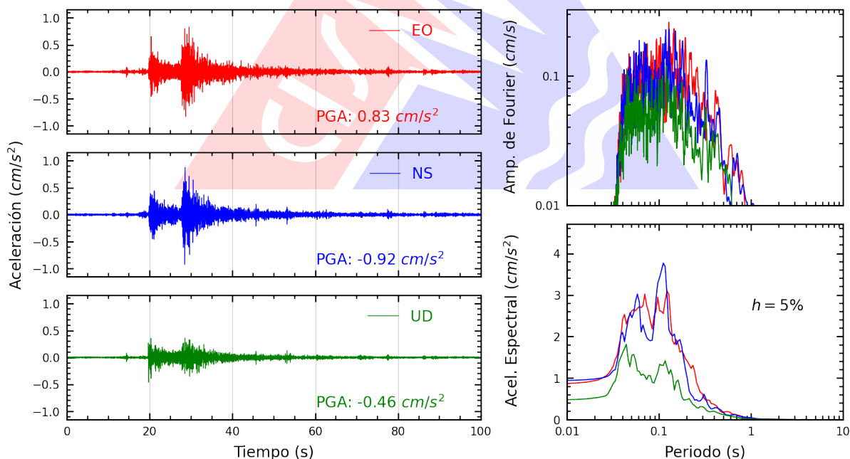
Figura A.14: Registros tiempo-historia, espectros de Fourier y de respuesta en las direcciones EO, NS y vertical de la estación BRISA. Sismo de Chilca, Cañete - Lima del 2026-03-19, 03:27:47 (Hora local)
