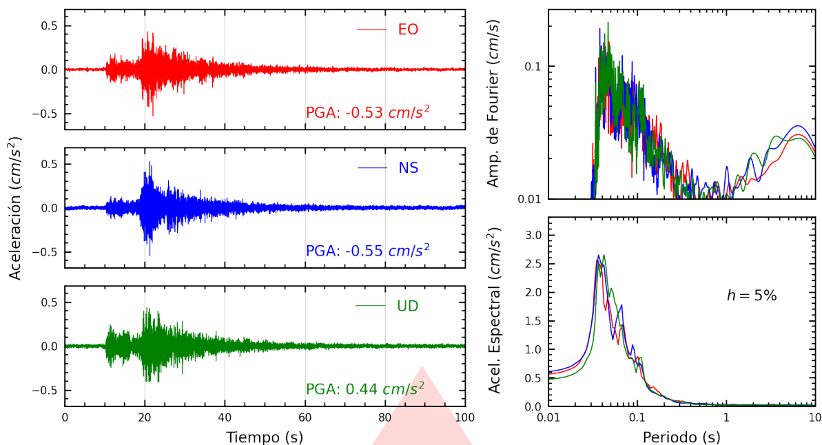
Figura A.23: Registros tiempo-historia, espectros de Fourier y de respuesta en las direcciones EO, NS y vertical de la estación USMP. Sismo de Chilca, Cañete - Lima del 2026-03-19, 03:27:47 (Hora local)
