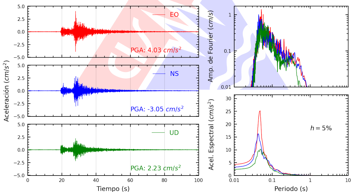
Figura A.2: Registros tiempo-historia, espectros de Fourier y de respuesta en las direcciones EO, NS y vertical de la estación UNTEL. Sismo de Chilca, Cañete - Lima del 2026-03-19, 03:27:47 (Hora local)
