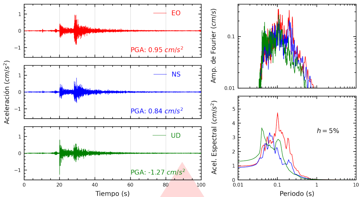
Figura A.9: Registros tiempo-historia, espectros de Fourier y de respuesta en las direcciones EO, NS y vertical de la estación SCCHO. Sismo de Chilca, Cañete - Lima del 2026-03-19, 03:27:47 (Hora local)
