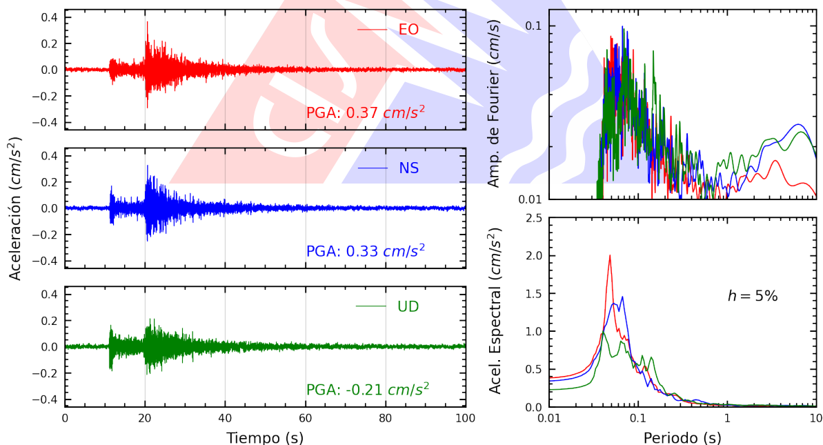
Figura A.30: Registros tiempo-historia, espectros de Fourier y de respuesta en las direcciones EO, NS y vertical de la estación UNFV. Sismo de Chilca, Cañete - Lima del 2026-03-19, 03:27:47 (Hora local)
