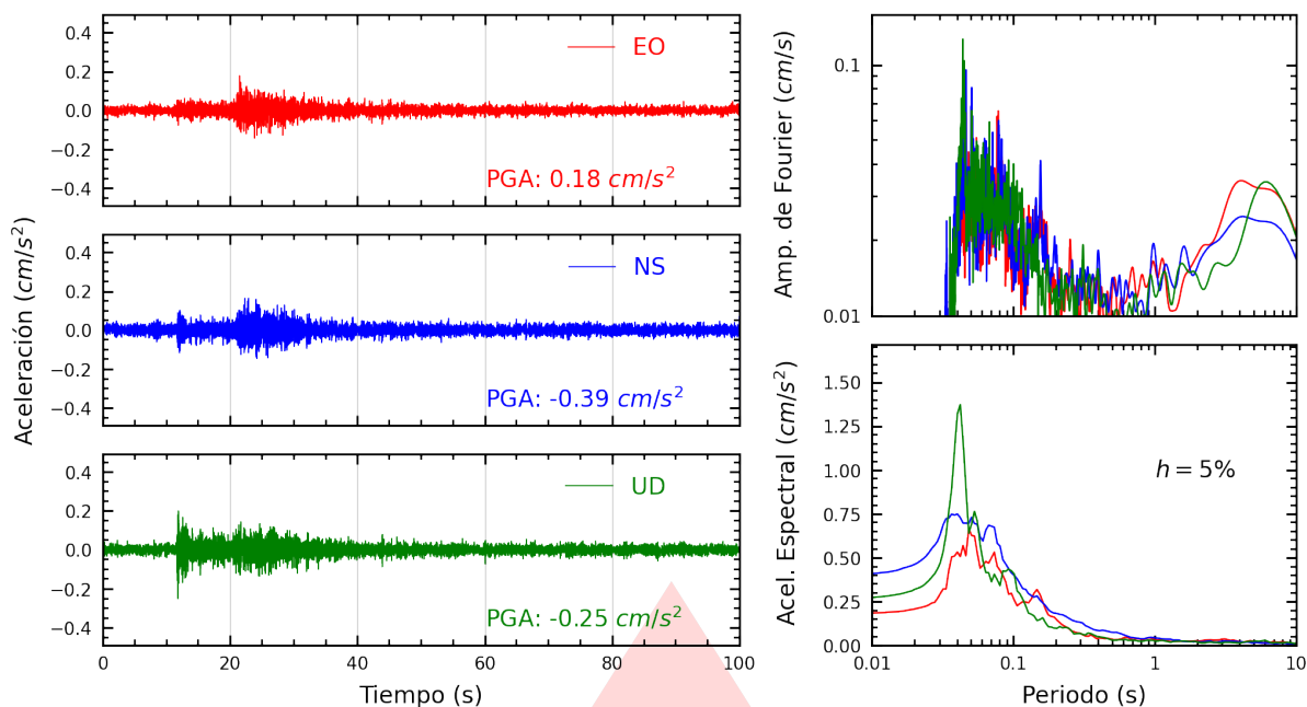
Figura A.29: Registros tiempo-historia, espectros de Fourier y de respuesta en las direcciones EO, NS y vertical de la estación BONDY. Sismo de Chilca, Cañete - Lima del 2026-03-19, 03:27:47 (Hora local)
