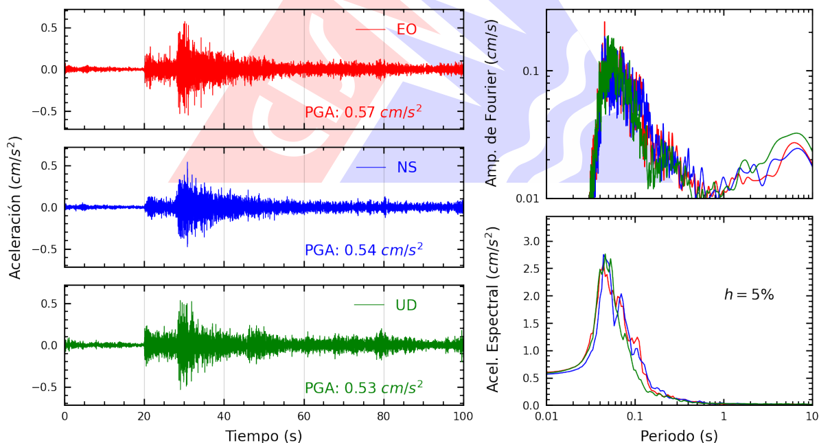
Figura A.22: Registros tiempo-historia, espectros de Fourier y de respuesta en las direcciones EO, NS y vertical de la estación URPPE. Sismo de Chilca, Cañete - Lima del 2026-03-19, 03:27:47 (Hora local)
