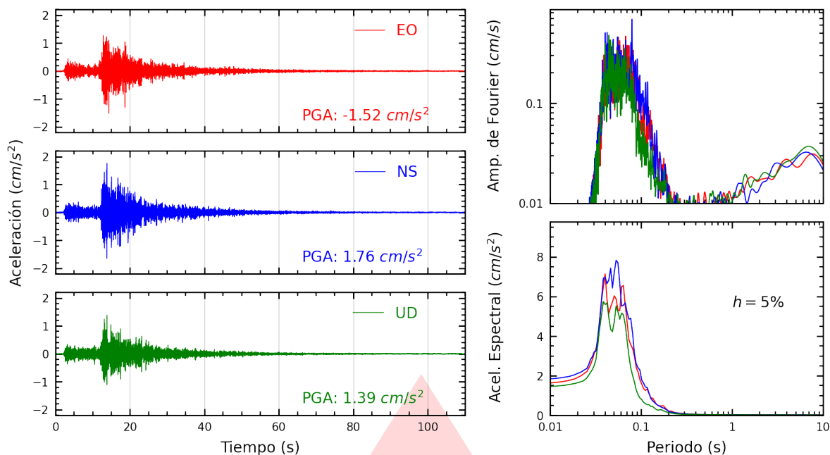
Figura A.5: Registros tiempo-historia, espectros de Fourier y de respuesta en las direcciones EO, NS y vertical de la estación JOSEO. Sismo de Chilca, Cañete - Lima del 2026-03-19, 03:27:47 (Hora local)
