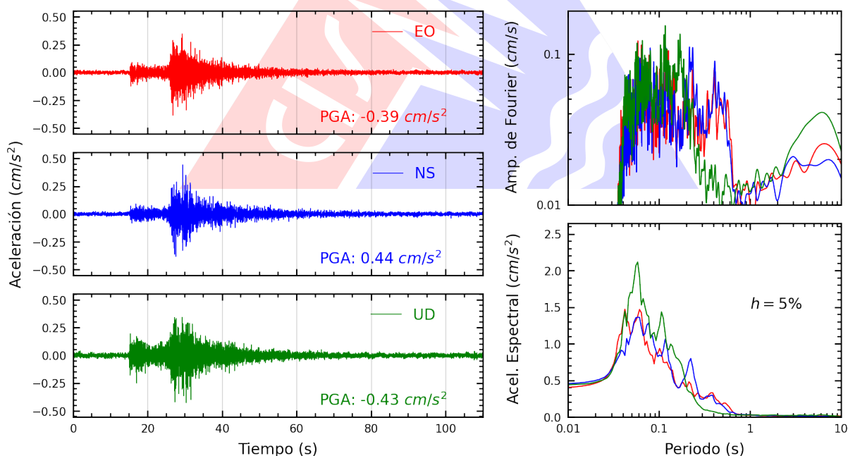
Figura A.26: Registros tiempo-historia, espectros de Fourier y de respuesta en las direcciones EO, NS y vertical de la estación MDPP. Sismo de Chilca, Cañete - Lima del 2026-03-19, 03:27:47 (Hora local)
