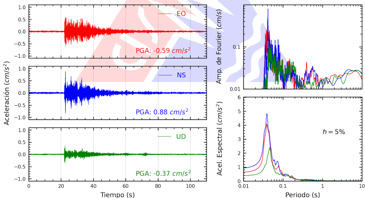
Figura A.16: Registros tiempo-historia, espectros de Fourier y de respuesta en las direcciones EO, NS y vertical de la estación DHNPE. Sismo de Chilca, Cañete - Lima del 2026-03-19, 03:27:47 (Hora local)
