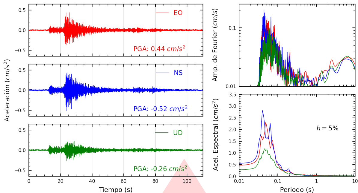
Figura A.25: Registros tiempo-historia, espectros de Fourier y de respuesta en las direcciones EO, NS y vertical de la estación COMAS. Sismo de Chilca, Cañete - Lima del 2026-03-19, 03:27:47 (Hora local)
