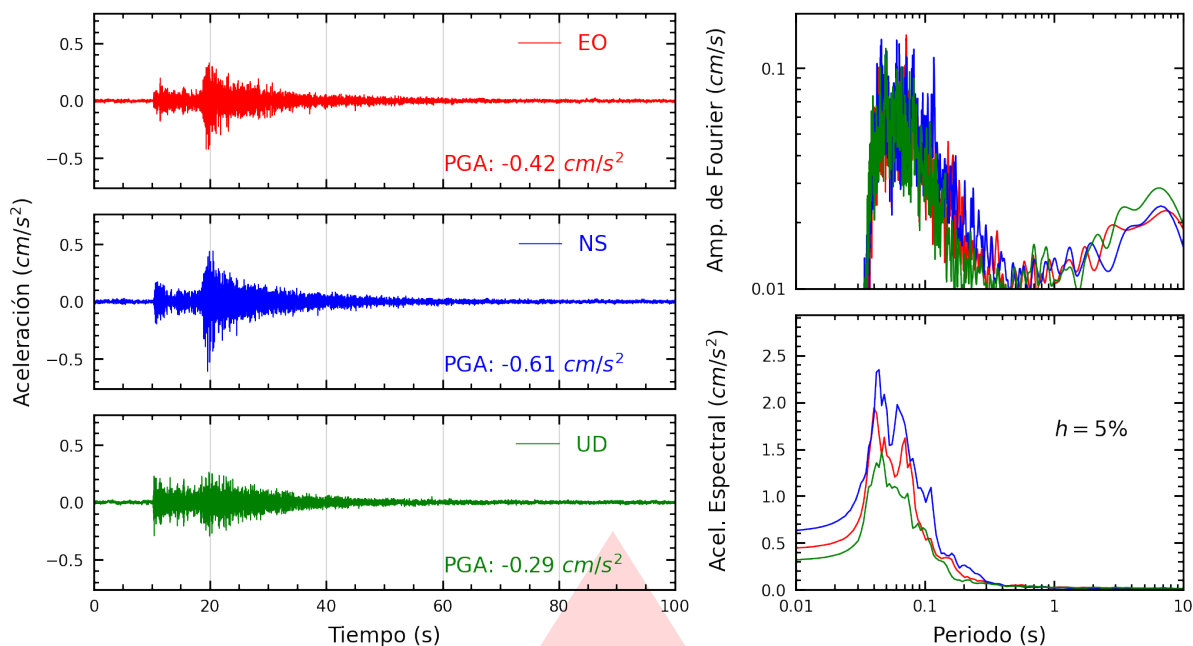
Figura A.21: Registros tiempo-historia, espectros de Fourier y de respuesta en las direcciones EO, NS y vertical de la estación SERVI. Sismo de Chilca, Cañete - Lima del 2026-03-19, 03:27:47 (Hora local)
