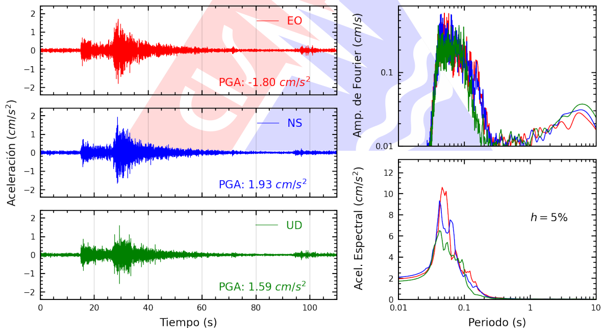
Figura A.4: Registros tiempo-historia, espectros de Fourier y de respuesta en las direcciones EO, NS y vertical de la estación SROSA. Sismo de Chilca, Cañete - Lima del 2026-03-19, 03:27:47 (Hora local)
