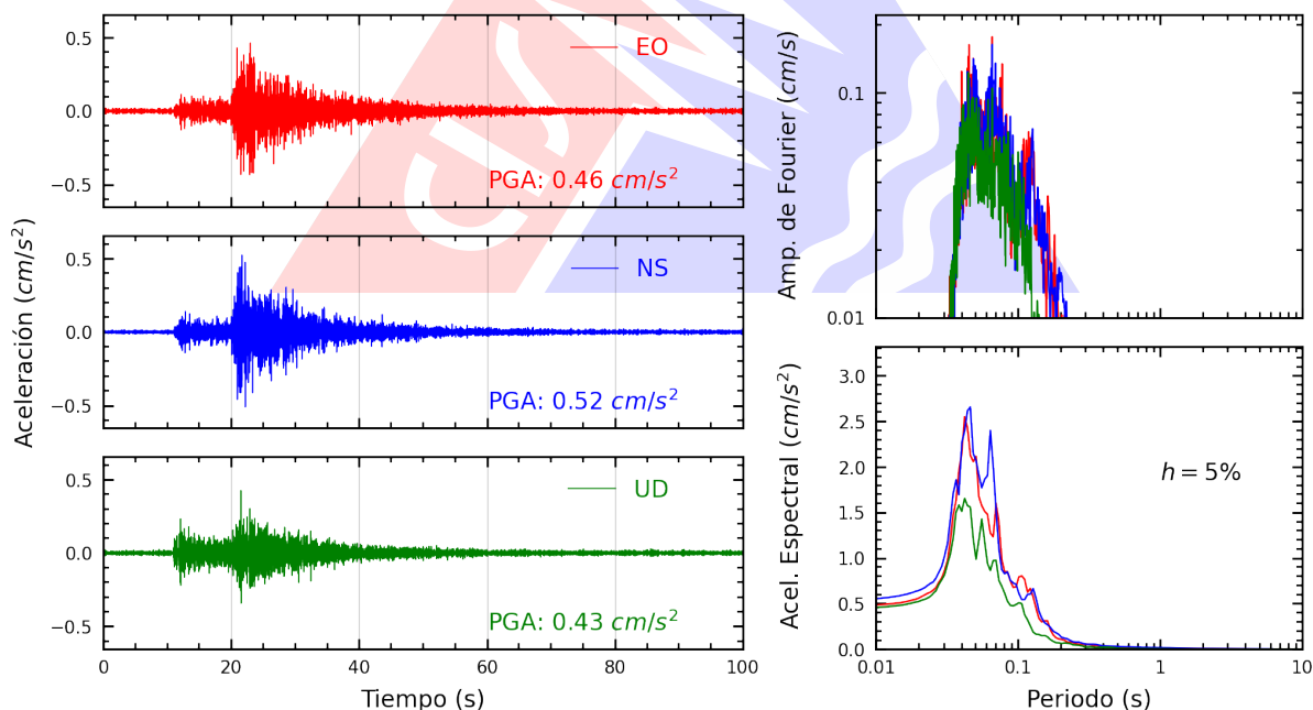
Figura A.24: Registros tiempo-historia, espectros de Fourier y de respuesta en las direcciones EO, NS y vertical de la estación ATARJ. Sismo de Chilca, Cañete - Lima del 2026-03-19, 03:27:47 (Hora local)
