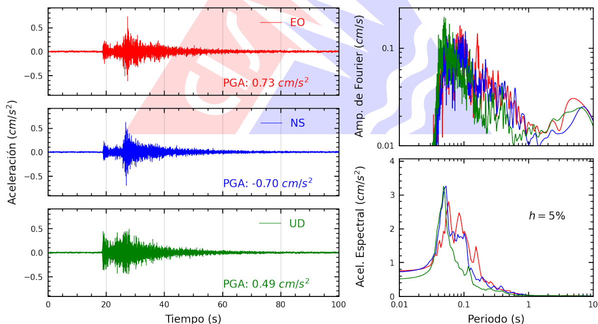
Figura A.18: Registros tiempo-historia, espectros de Fourier y de respuesta en las direcciones EO, NS y vertical de la estación USILP. Sismo de Chilca, Cañete - Lima del 2026-03-19, 03:27:47 (Hora local)
