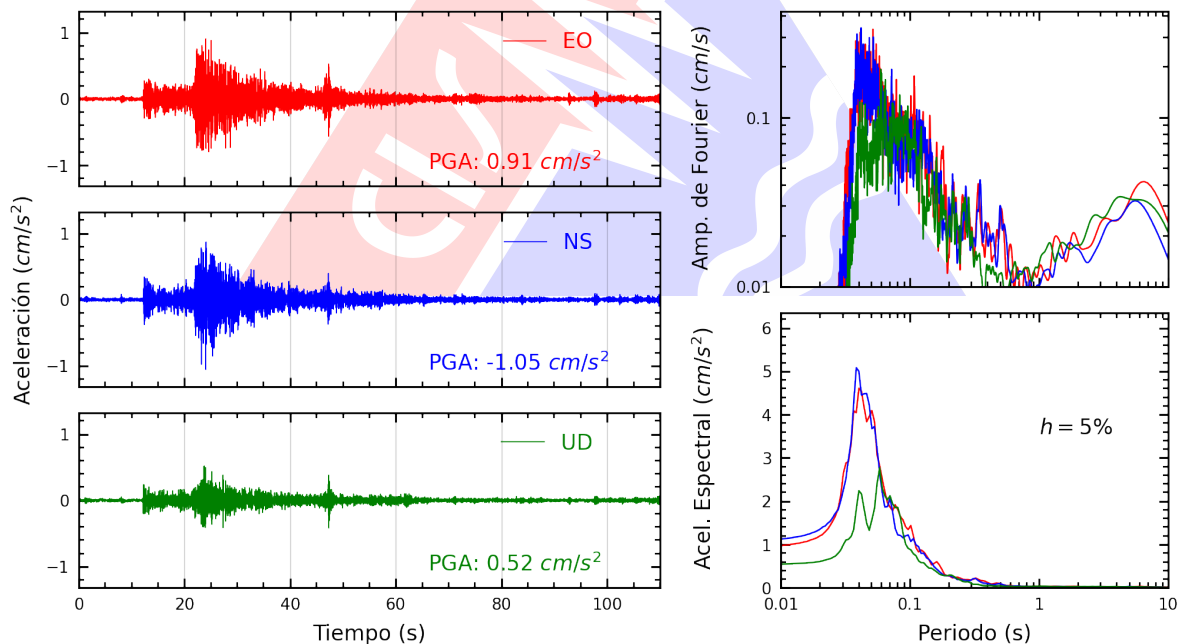
Figura A.10: Registros tiempo-historia, espectros de Fourier y de respuesta en las direcciones EO, NS y vertical de la estación OLIVO. Sismo de Chilca, Cañete - Lima del 2026-03-19, 03:27:47 (Hora local)
