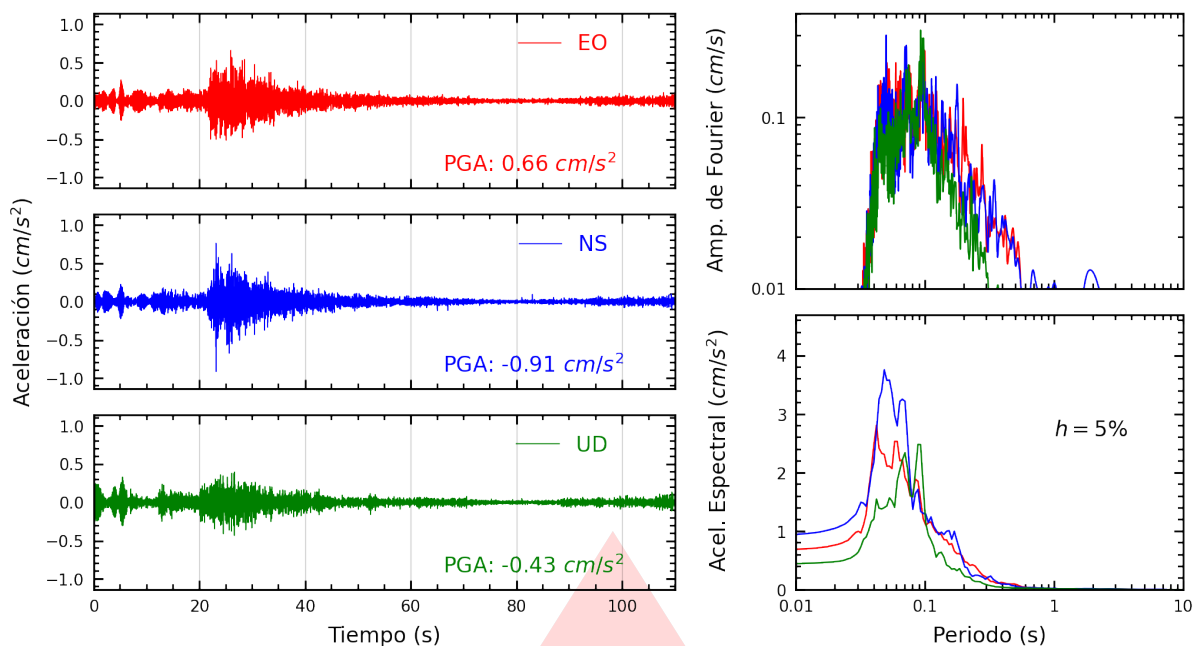
Figura A.15: Registros tiempo-historia, espectros de Fourier y de respuesta en las direcciones EO, NS y vertical de la estación SCOLI. Sismo de Chilca, Cañete - Lima del 2026-03-19, 03:27:47 (Hora local)
