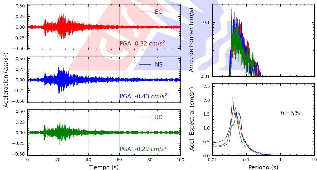
Figura A.28: Registros tiempo-historia, espectros de Fourier y de respuesta en las direcciones EO, NS y vertical de la estación BORJA. Sismo de Chilca, Cañete - Lima del 2026-03-19, 03:27:47 (Hora local)
