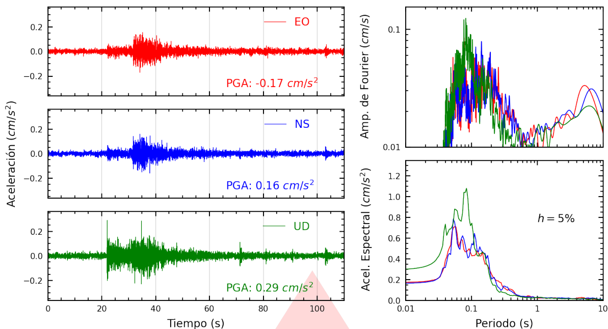
Figura A.33: Registros tiempo-historia, espectros de Fourier y de respuesta en las direcciones EO, NS y vertical de la estación RAMON. Sismo de Chilca, Cañete - Lima del 2026-03-19, 03:27:47 (Hora local)
