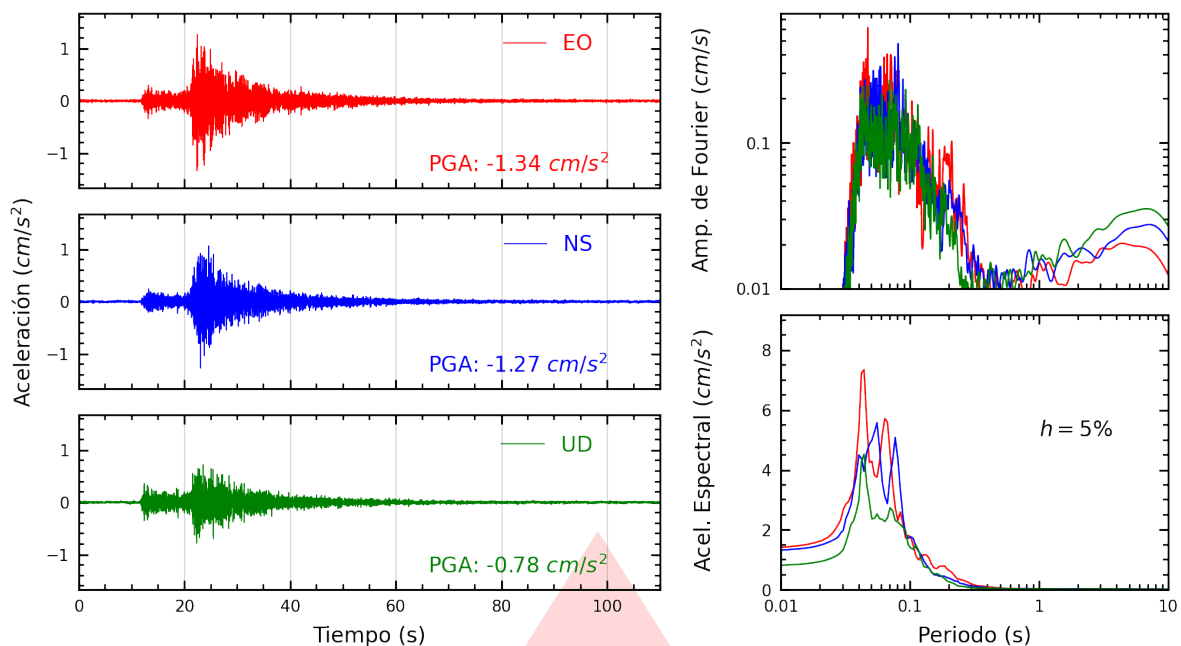
Figura A.7: Registros tiempo-historia, espectros de Fourier y de respuesta en las direcciones EO, NS y vertical de la estación INDEP. Sismo de Chilca, Cañete - Lima del 2026-03-19, 03:27:47 (Hora local)
