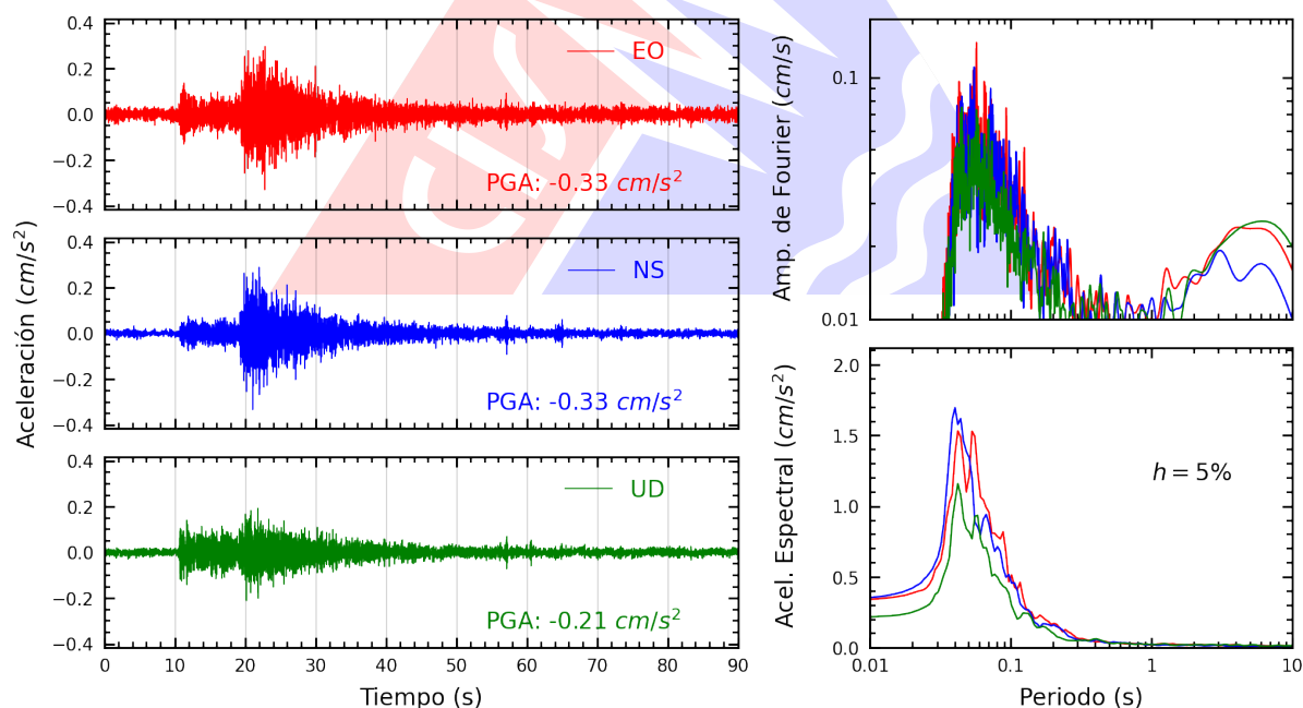
Figura A.32: Registros tiempo-historia, espectros de Fourier y de respuesta en las direcciones EO, NS y vertical de la estación INICT. Sismo de Chilca, Cañete - Lima del 2026-03-19, 03:27:47 (Hora local)
