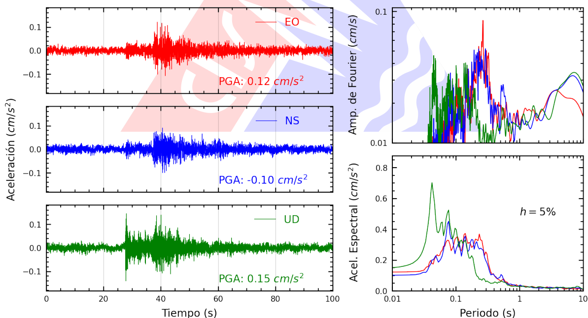
Figura A.34: Registros tiempo-historia, espectros de Fourier y de respuesta en las direcciones EO, NS y vertical de la estación DMSI. Sismo de Chilca, Cañete - Lima del 2026-03-19, 03:27:47 (Hora local)
