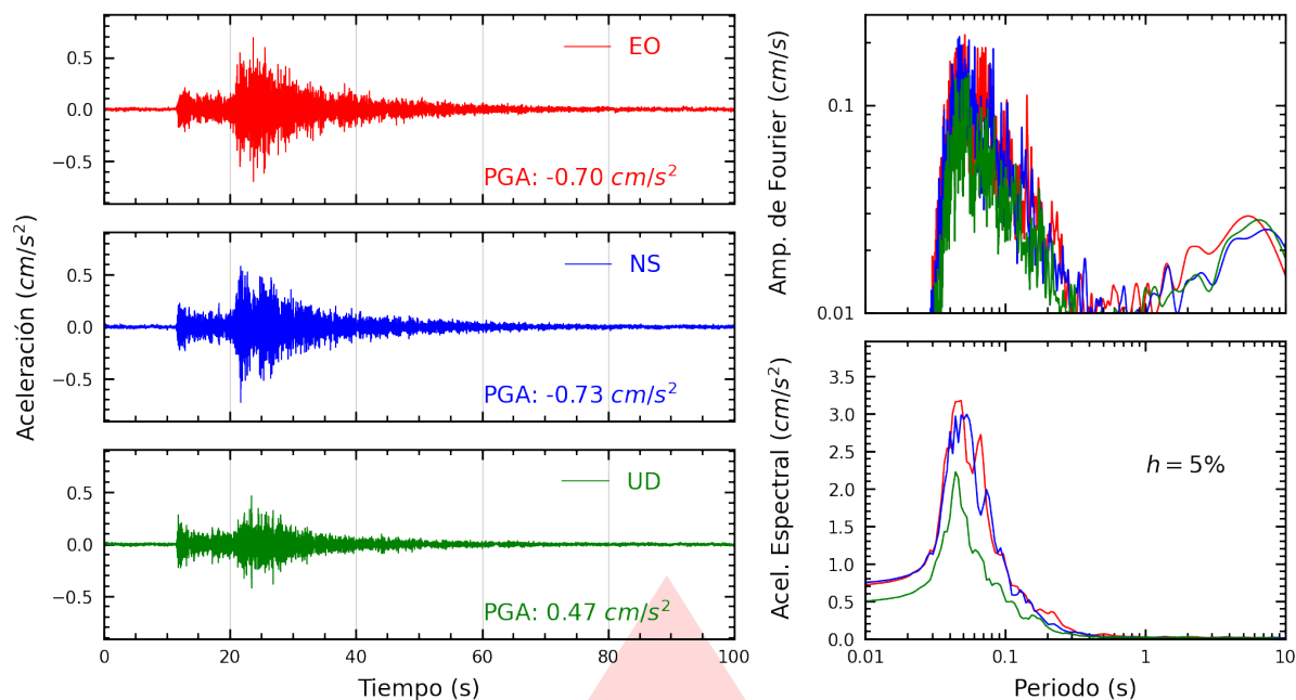
Figura A.19: Registros tiempo-historia, espectros de Fourier y de respuesta en las direcciones EO, NS y vertical de la estación FICPE. Sismo de Chilca, Cañete - Lima del 2026-03-19, 03:27:47 (Hora local)
