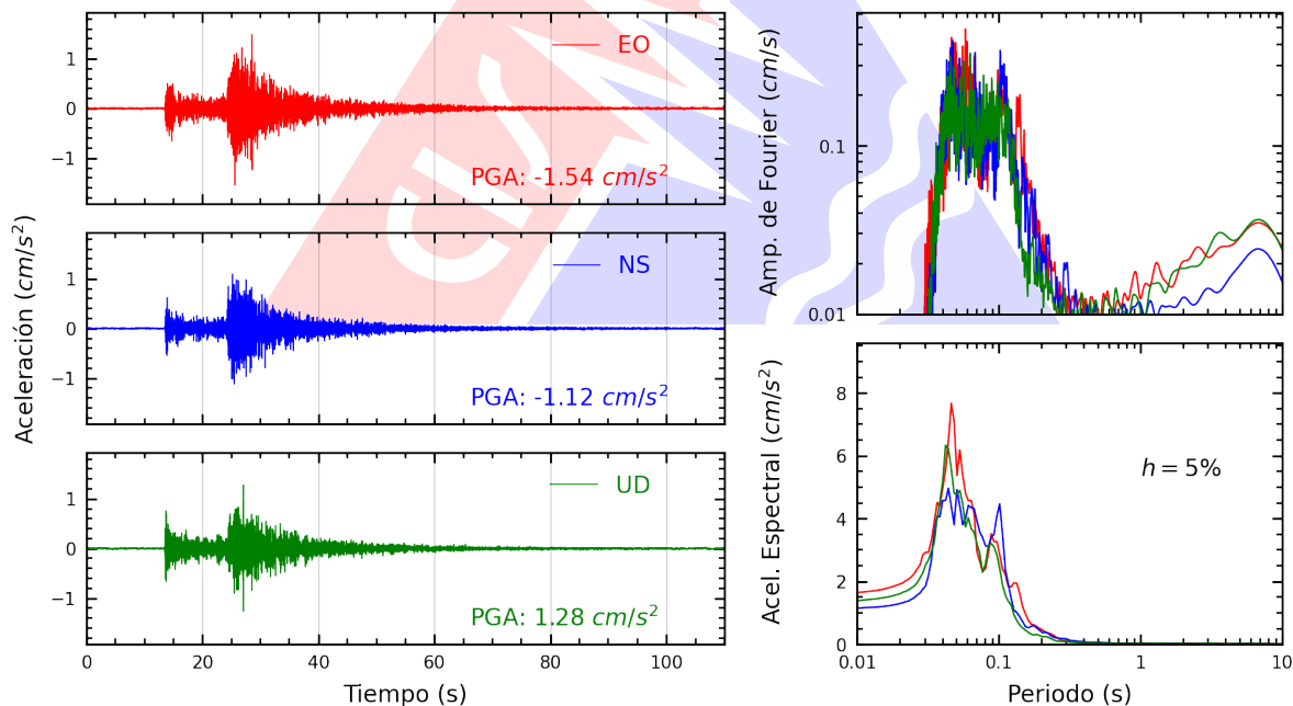
Figura A.6: Registros tiempo-historia, espectros de Fourier y de respuesta en las direcciones EO, NS y vertical de la estación AMORE. Sismo de Chilca, Cañete - Lima del 2026-03-19, 03:27:47 (Hora local)
