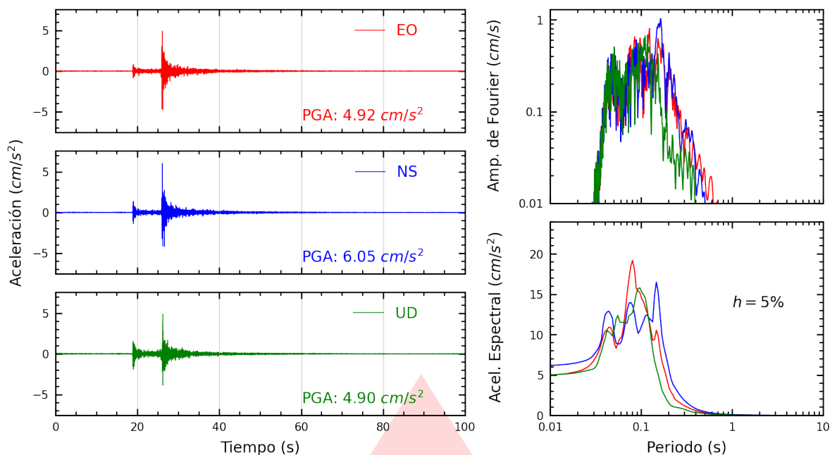
Figura A.1: Registros tiempo-historia, espectros de Fourier y de respuesta en las direcciones EO, NS y vertical de la estación ASIA. Sismo de Chilca, Cañete - Lima del 2026-03-19, 03:27:47 (Hora local)
