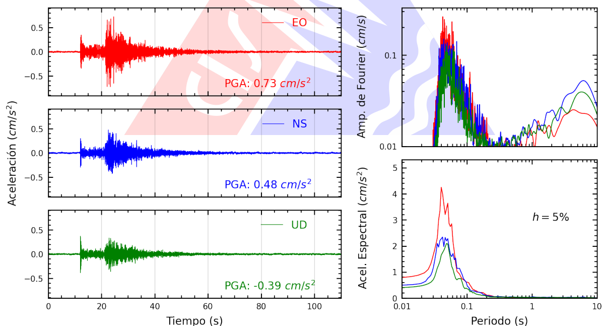
Figura A.20: Registros tiempo-historia, espectros de Fourier y de respuesta en las direcciones EO, NS y vertical de la estación UCSS. Sismo de Chilca, Cañete - Lima del 2026-03-19, 03:27:47 (Hora local)
