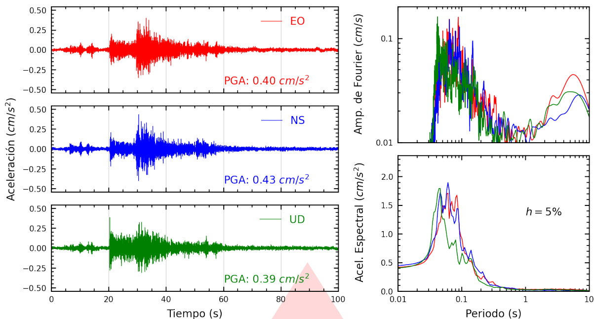
Figura A.27: Registros tiempo-historia, espectros de Fourier y de respuesta en las direcciones EO, NS y vertical de la estación UPCSM. Sismo de Chilca, Cañete - Lima del 2026-03-19, 03:27:47 (Hora local)
