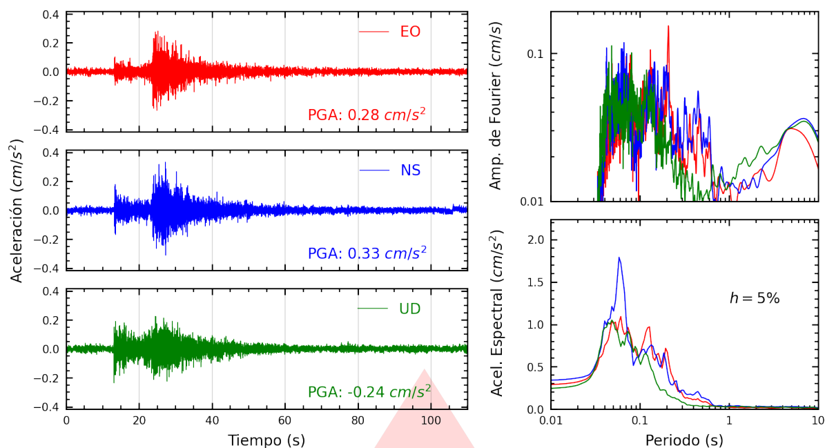
Figura A.31: Registros tiempo-historia, espectros de Fourier y de respuesta en las direcciones EO, NS y vertical de la estación VHAYA. Sismo de Chilca, Cañete - Lima del 2026-03-19, 03:27:47 (Hora local)
