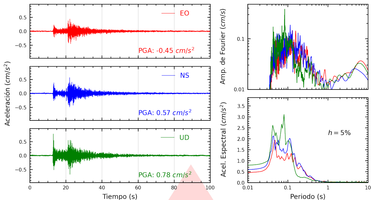
Figura A.17: Registros tiempo-historia, espectros de Fourier y de respuesta en las direcciones EO, NS y vertical de la estación SOCHO. Sismo de Chilca, Cañete - Lima del 2026-03-19, 03:27:47 (Hora local)
