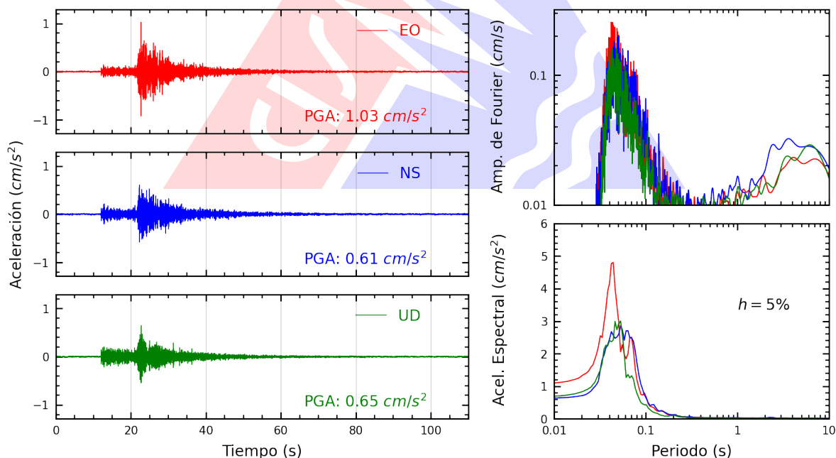
Figura A.12: Registros tiempo-historia, espectros de Fourier y de respuesta en las direcciones EO, NS y vertical de la estación SJLCE. Sismo de Chilca, Cañete - Lima del 2026-03-19, 03:27:47 (Hora local)
