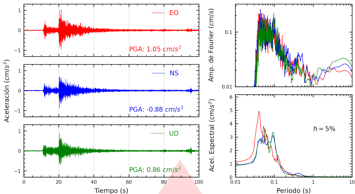
Figura A.11: Registros tiempo-historia, espectros de Fourier y de respuesta en las direcciones EO, NS y vertical de la estación UCVAT. Sismo de Chilca, Cañete - Lima del 2026-03-19, 03:27:47 (Hora local)
