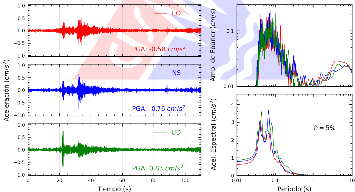
Figura A.22: Registros tiempo-historia, espectros de Fourier y de respuesta en las direcciones EO, NS y vertical de la estación MADRE. Sismo de Lima, Lima - Lima del 2026-03-19, 23:00:37 (Hora local)
