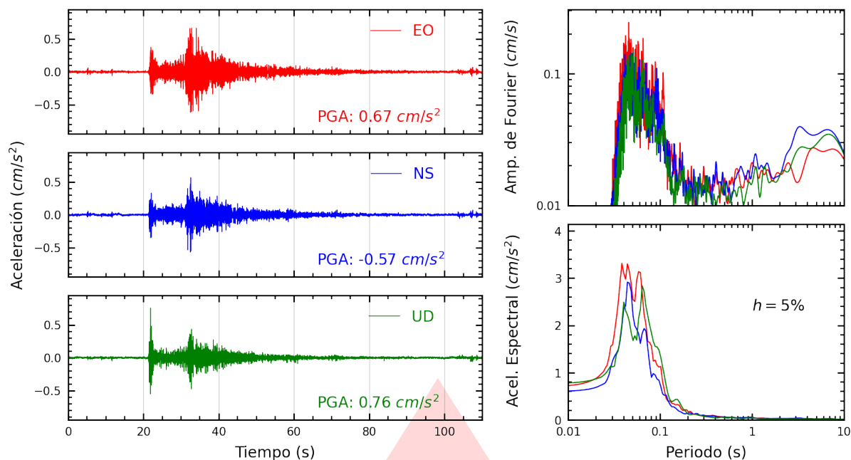
Figura A.25: Registros tiempo-historia, espectros de Fourier y de respuesta en las direcciones EO, NS y vertical de la estación UCSS. Sismo de Lima, Lima - Lima del 2026-03-19, 23:00:37 (Hora local)
