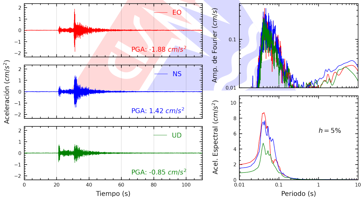
Figura A.8: Registros tiempo-historia, espectros de Fourier y de respuesta en las direcciones EO, NS y vertical de la estación SJLCE. Sismo de Lima, Lima - Lima del 2026-03-19, 23:00:37 (Hora local)
