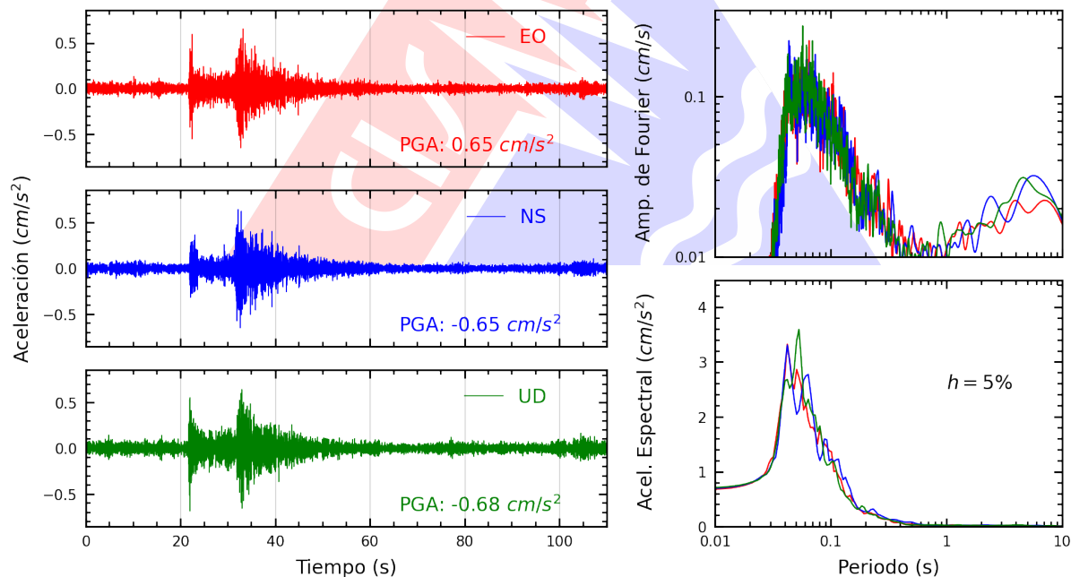
Figura A.26: Registros tiempo-historia, espectros de Fourier y de respuesta en las direcciones EO, NS y vertical de la estación URPE. Sismo de Lima, Lima - Lima del 2026-03-19, 23:00:37 (Hora local)
