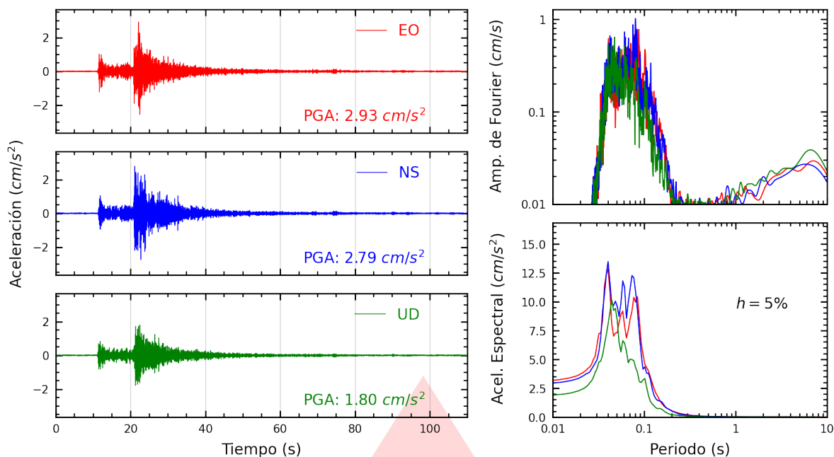
Figura A.5: Registros tiempo-historia, espectros de Fourier y de respuesta en las direcciones EO, NS y vertical de la estación JOSEO. Sismo de Lima, Lima - Lima del 2026-03-19, 23:00:37 (Hora local)
