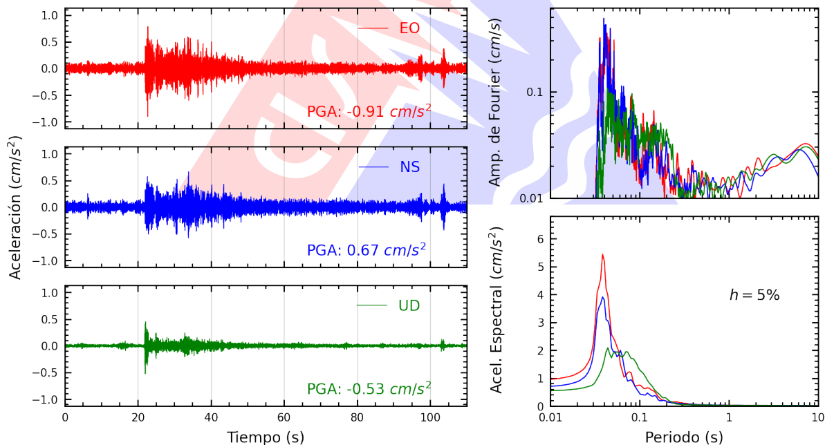
Figura A.18: Registros tiempo-historia, espectros de Fourier y de respuesta en las direcciones EO, NS y vertical de la estación DHNPE. Sismo de Lima, Lima - Lima del 2026-03-19, 23:00:37 (Hora local)
