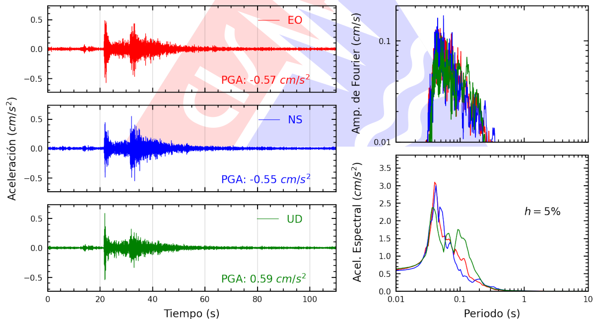
Figura A.30: Registros tiempo-historia, espectros de Fourier y de respuesta en las direcciones EO, NS y vertical de la estación BORJA. Sismo de Lima, Lima - Lima del 2026-03-19, 23:00:37 (Hora local)
