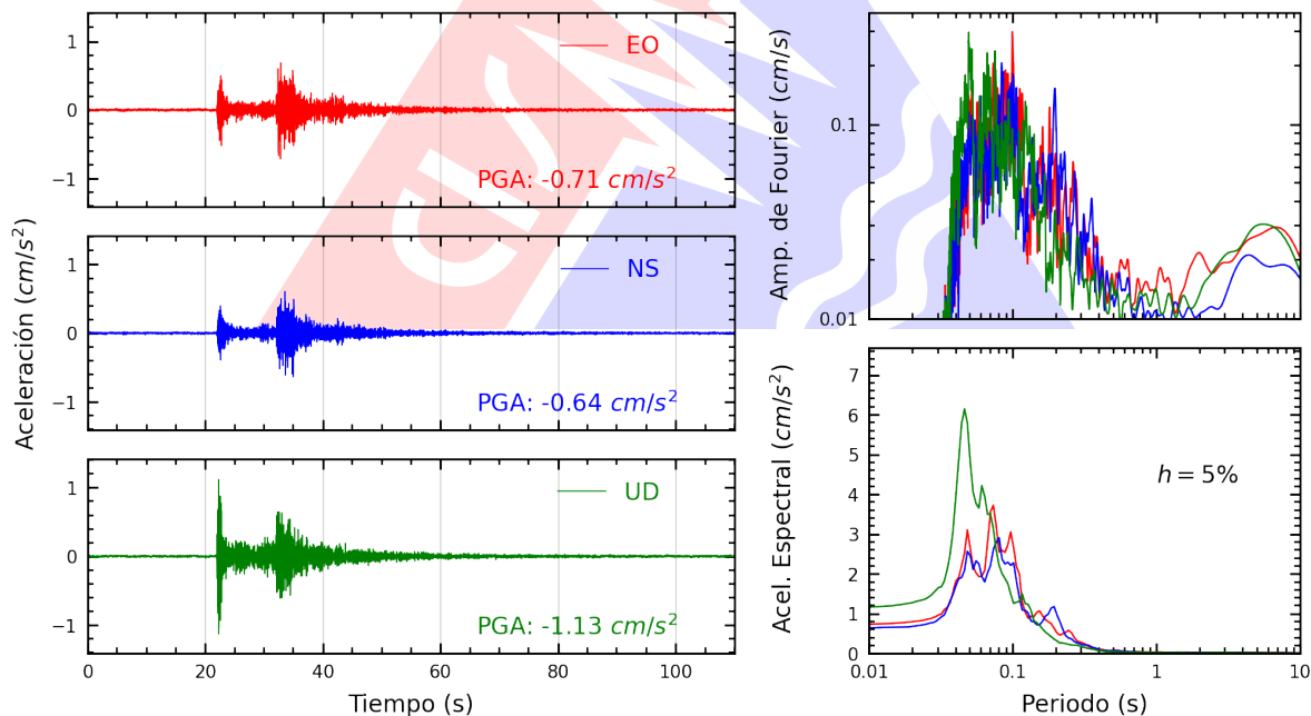
Figura A.16: Registros tiempo-historia, espectros de Fourier y de respuesta en las direcciones EO, NS y vertical de la estación USILP. Sismo de Lima, Lima - Lima del 2026-03-19, 23:00:37 (Hora local)
