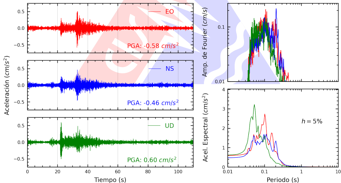
Figura A.28: Registros tiempo-historia, espectros de Fourier y de respuesta en las direcciones EO, NS y vertical de la estación SCCHO. Sismo de Lima, Lima - Lima del 2026-03-19, 23:00:37 (Hora local)
