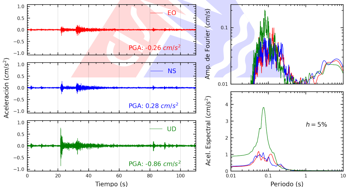
Figura A.20: Registros tiempo-historia, espectros de Fourier y de respuesta en las direcciones EO, NS y vertical de la estación RAMON. Sismo de Lima, Lima - Lima del 2026-03-19, 23:00:37 (Hora local)
