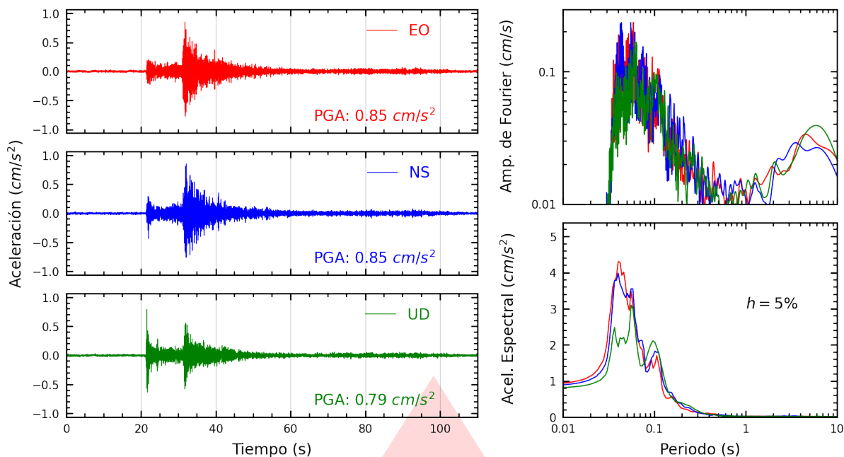
Figura A.21: Registros tiempo-historia, espectros de Fourier y de respuesta en las direcciones EO, NS y vertical de la estación COMAS. Sismo de Lima, Lima - Lima del 2026-03-19, 23:00:37 (Hora local)
