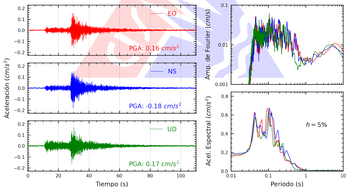
Figura A.32: Registros tiempo-historia, espectros de Fourier y de respuesta en las direcciones EO, NS y vertical de la estación CARAL. Sismo de Lima, Lima - Lima del 2026-03-19, 23:00:37 (Hora local)
