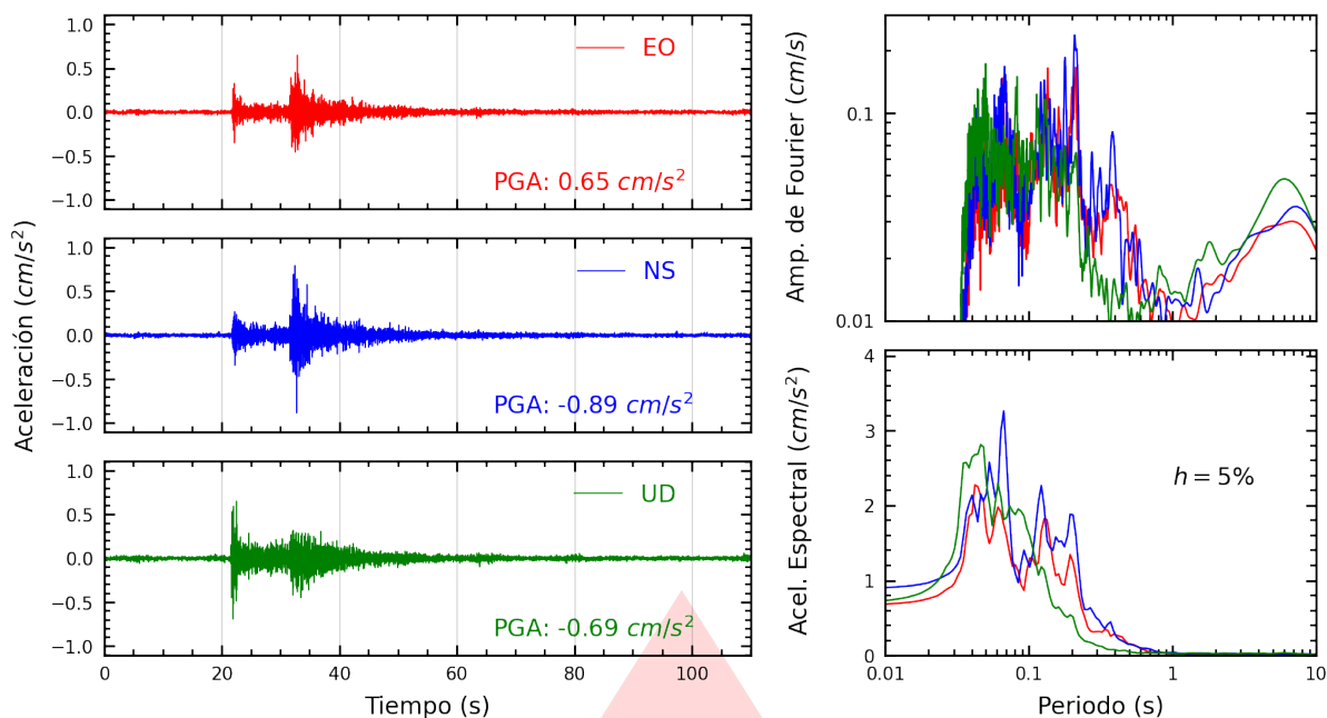
Figura A.19: Registros tiempo-historia, espectros de Fourier y de respuesta en las direcciones EO, NS y vertical de la estación VHAYA. Sismo de Lima, Lima - Lima del 2026-03-19, 23:00:37 (Hora local)
