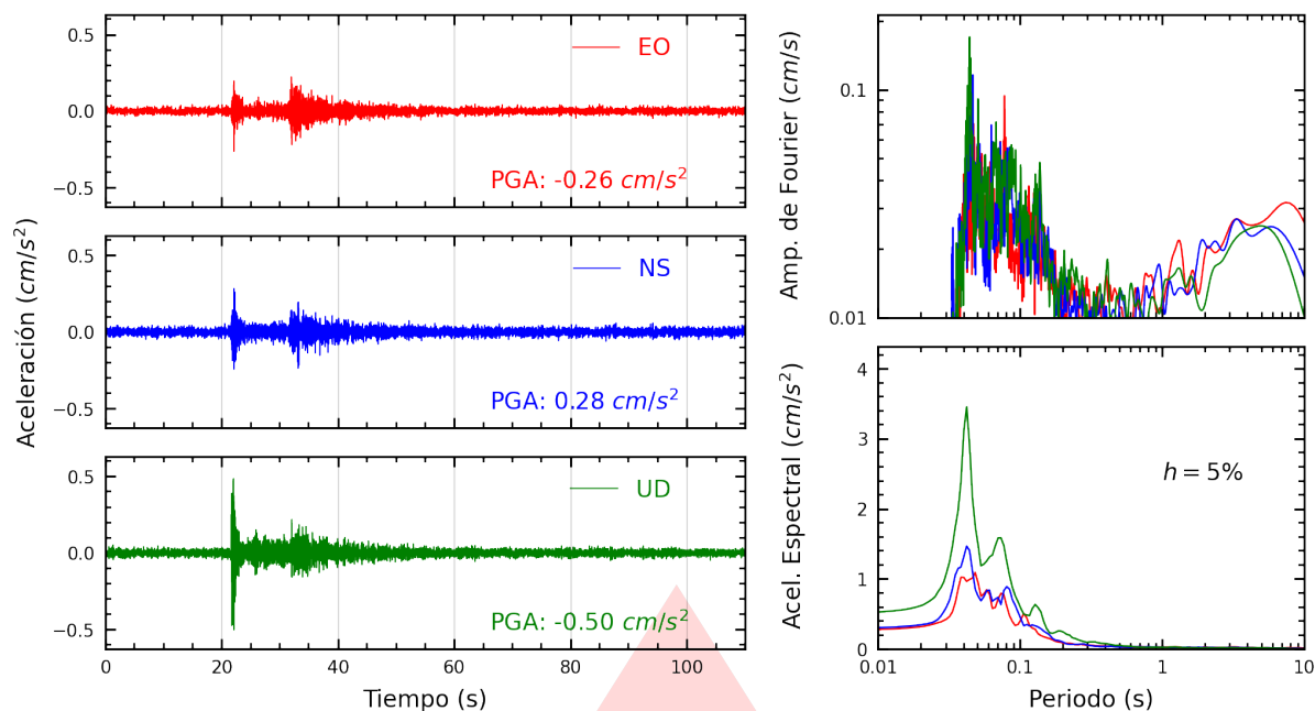
Figura A.31: Registros tiempo-historia, espectros de Fourier y de respuesta en las direcciones EO, NS y vertical de la estación BONDY. Sismo de Lima, Lima - Lima del 2026-03-19, 23:00:37 (Hora local)
