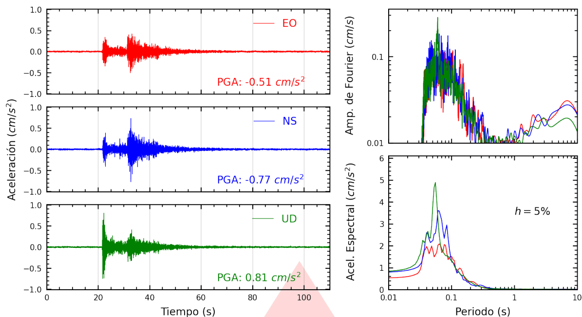
Figura A.23: Registros tiempo-historia, espectros de Fourier y de respuesta en las direcciones EO, NS y vertical de la estación SERVI. Sismo de Lima, Lima - Lima del 2026-03-19, 23:00:37 (Hora local)
