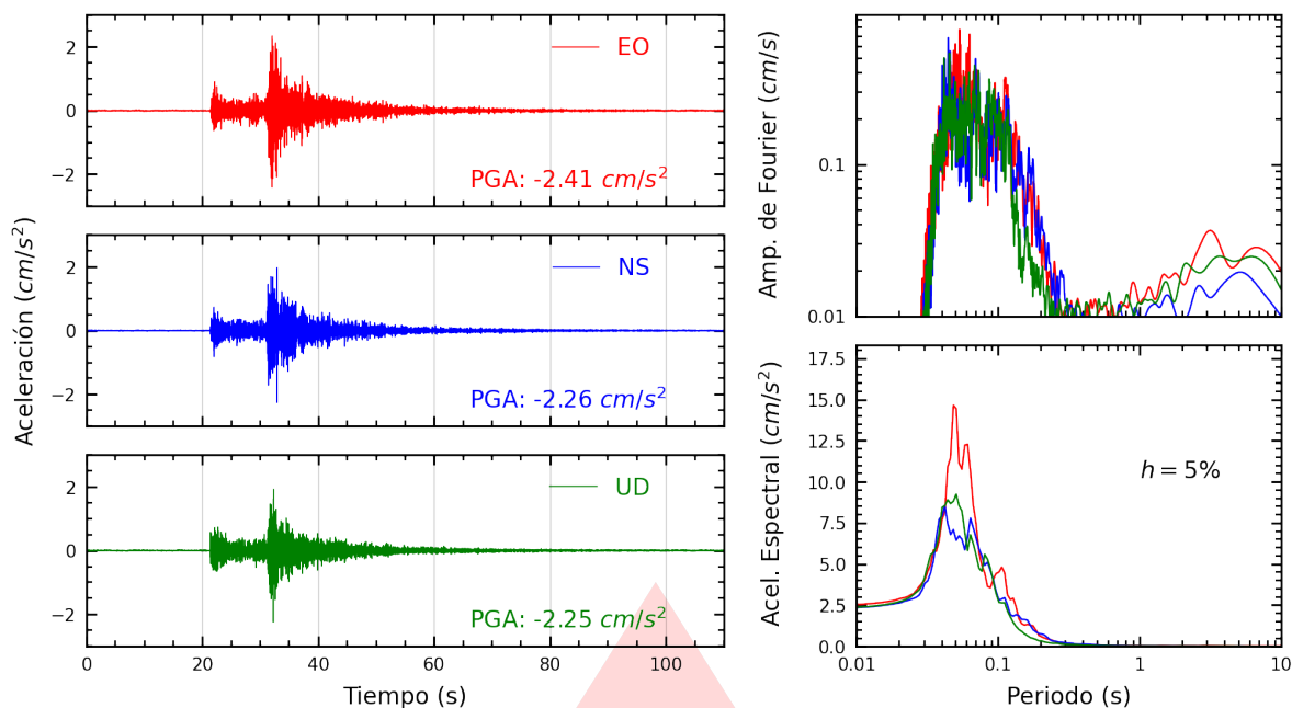
Figura A.7: Registros tiempo-historia, espectros de Fourier y de respuesta en las direcciones EO, NS y vertical de la estación AMORE. Sismo de Lima, Lima - Lima del 2026-03-19, 23:00:37 (Hora local)
