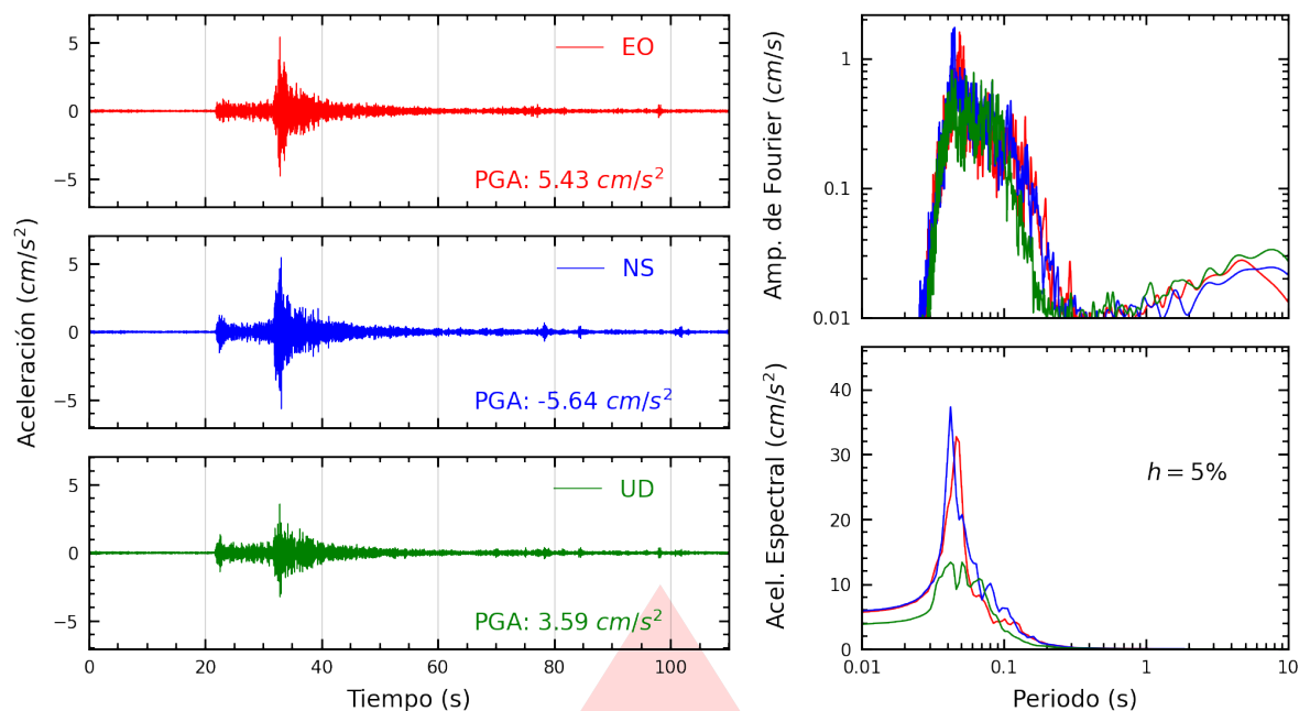
Figura A.1: Registros tiempo-historia, espectros de Fourier y de respuesta en las direcciones EO, NS y vertical de la estación SROSA. Sismo de Lima, Lima - Lima del 2026-03-19, 23:00:37 (Hora local)
