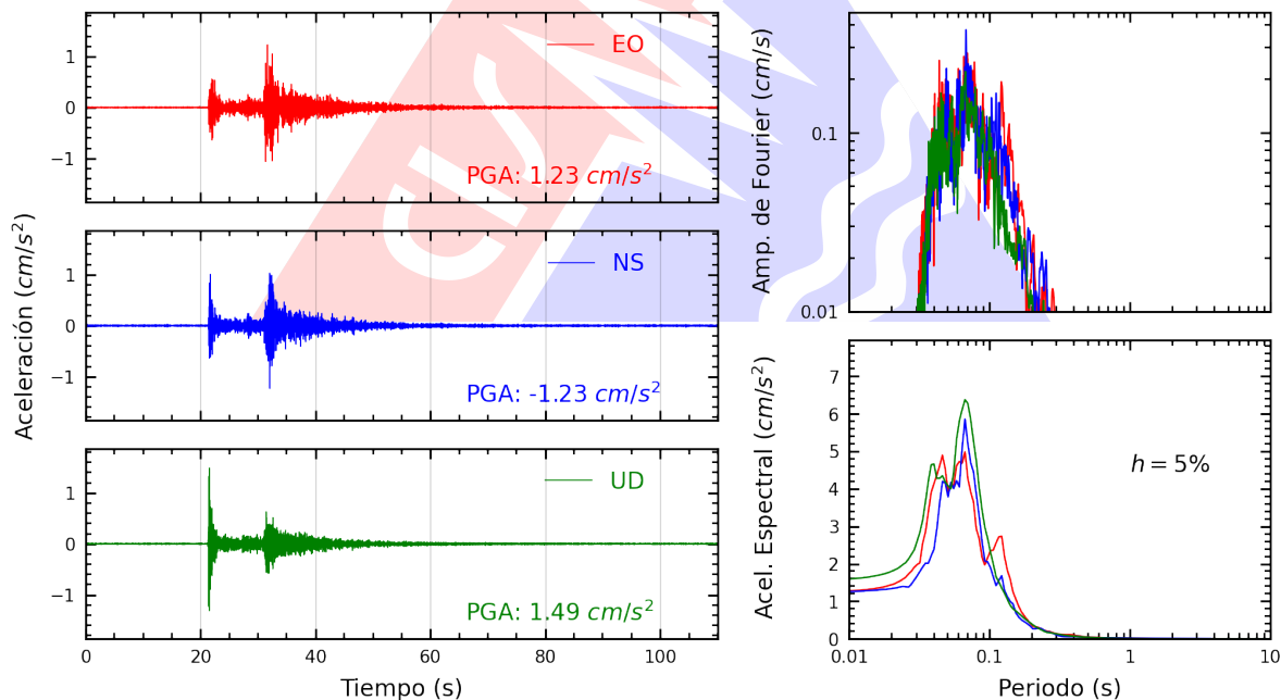
Figura A.12: Registros tiempo-historia, espectros de Fourier y de respuesta en las direcciones EO, NS y vertical de la estación ATARJ. Sismo de Lima, Lima - Lima del 2026-03-19, 23:00:37 (Hora local)
