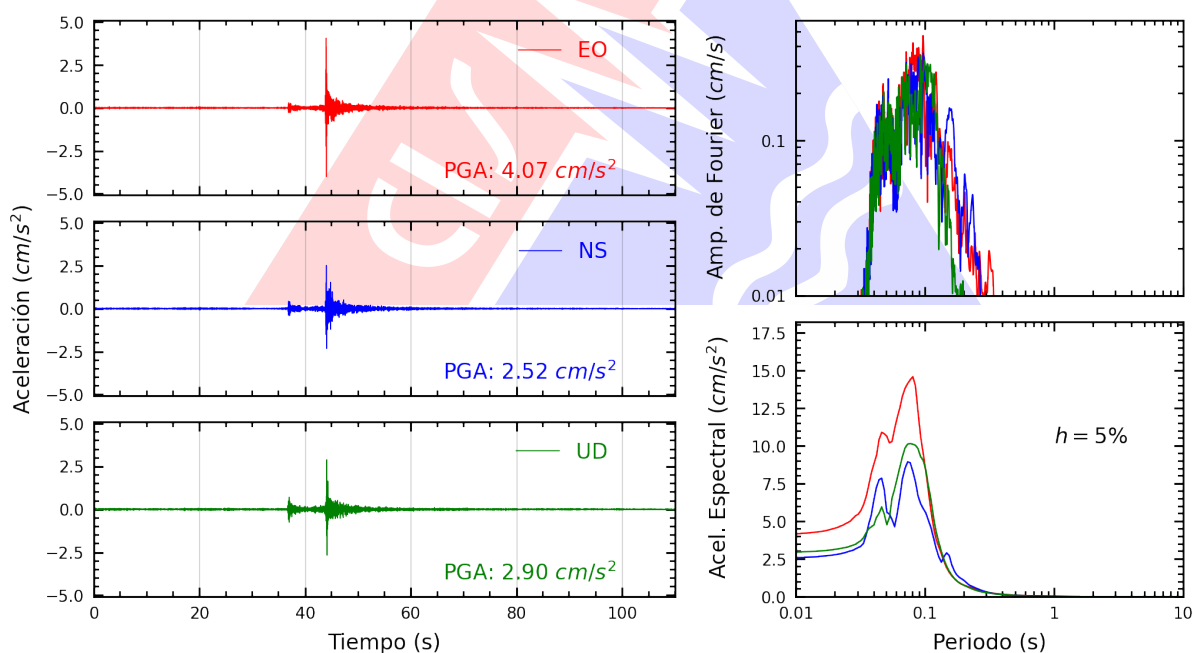
Figura A.2: Registros tiempo-historia, espectros de Fourier y de respuesta en las direcciones EO, NS y vertical de la estación ASIA. Sismo de Lima, Lima - Lima del 2026-03-19, 23:00:37 (Hora local)
