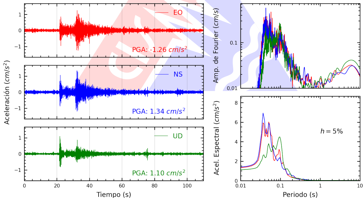
Figura A.14: Registros tiempo-historia, espectros de Fourier y de respuesta en las direcciones EO, NS y vertical de la estación OLIVO. Sismo de Lima, Lima - Lima del 2026-03-19, 23:00:37 (Hora local)
