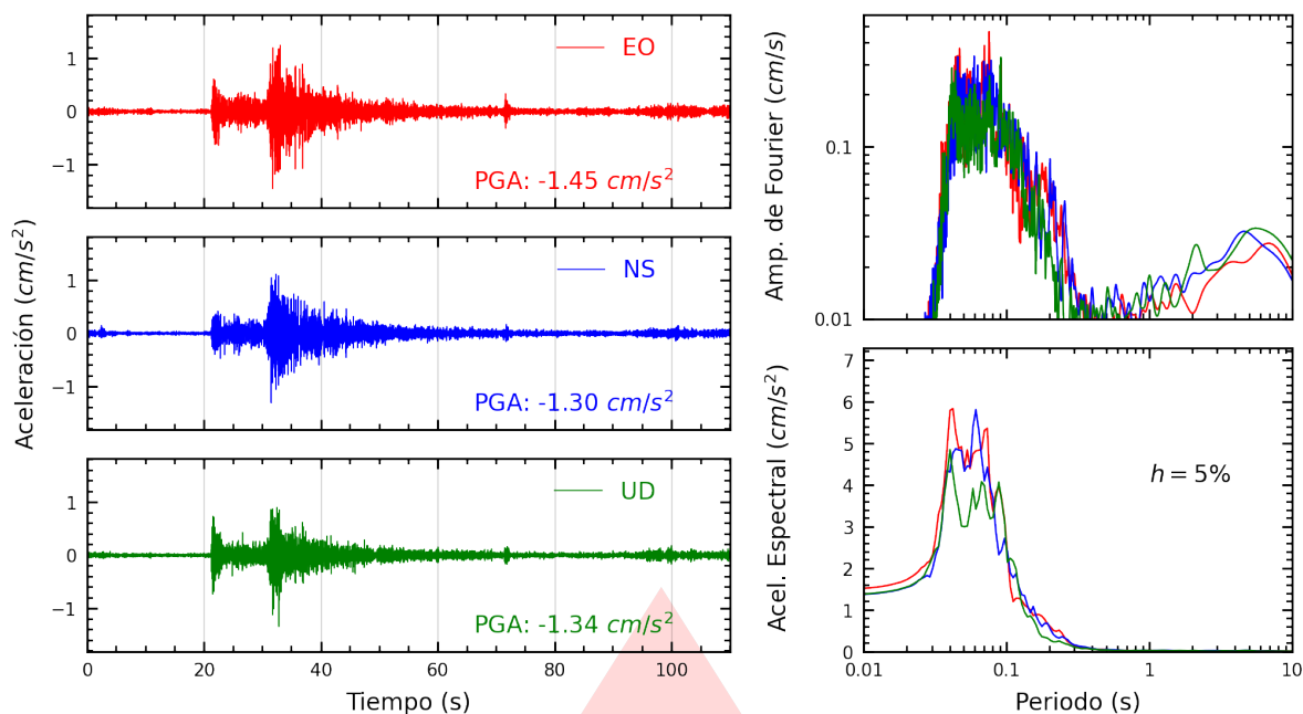
Figura A.13: Registros tiempo-historia, espectros de Fourier y de respuesta en las direcciones EO, NS y vertical de la estación INDEP. Sismo de Lima, Lima - Lima del 2026-03-19, 23:00:37 (Hora local)
