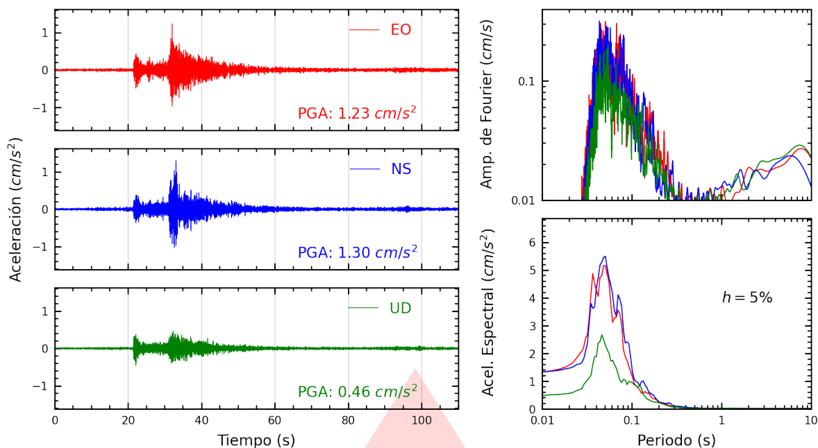
Figura A.15: Registros tiempo-historia, espectros de Fourier y de respuesta en las direcciones EO, NS y vertical de la estación FICPE. Sismo de Lima, Lima - Lima del 2026-03-19, 23:00:37 (Hora local)
