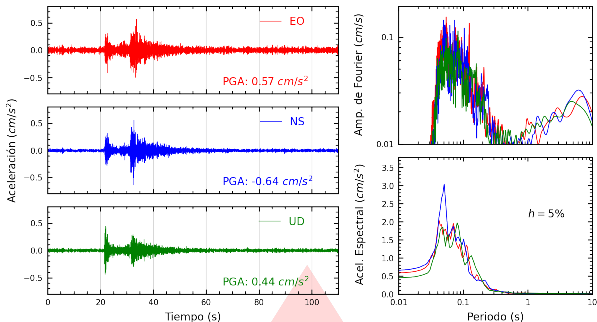
Figura A.27: Registros tiempo-historia, espectros de Fourier y de respuesta en las direcciones EO, NS y vertical de la estación INICT. Sismo de Lima, Lima - Lima del 2026-03-19, 23:00:37 (Hora local)
