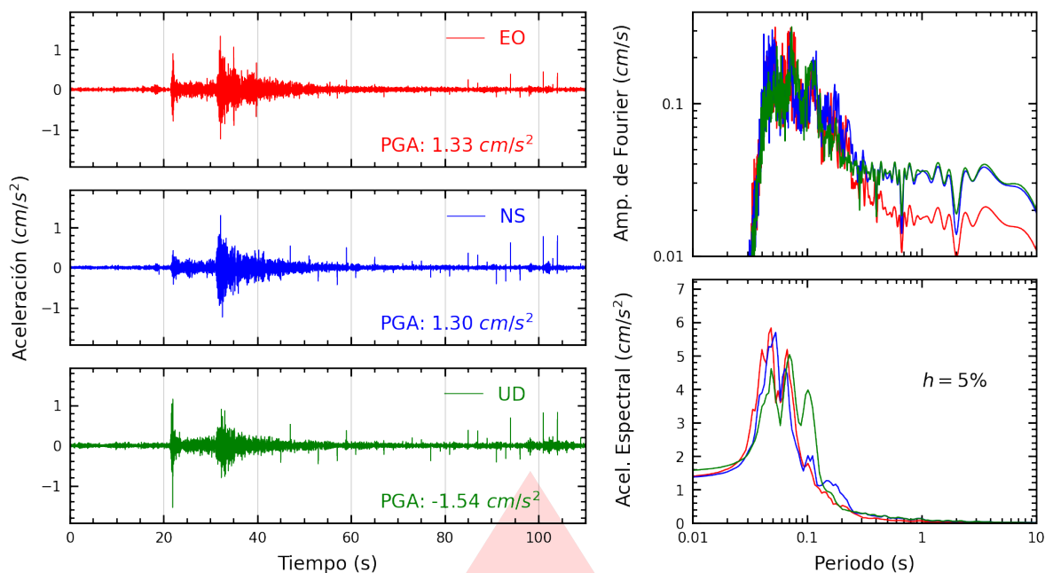
Figura A.11: Registros tiempo-historia, espectros de Fourier y de respuesta en las direcciones EO, NS y vertical de la estación SCOLI. Sismo de Lima, Lima - Lima del 2026-03-19, 23:00:37 (Hora local)
