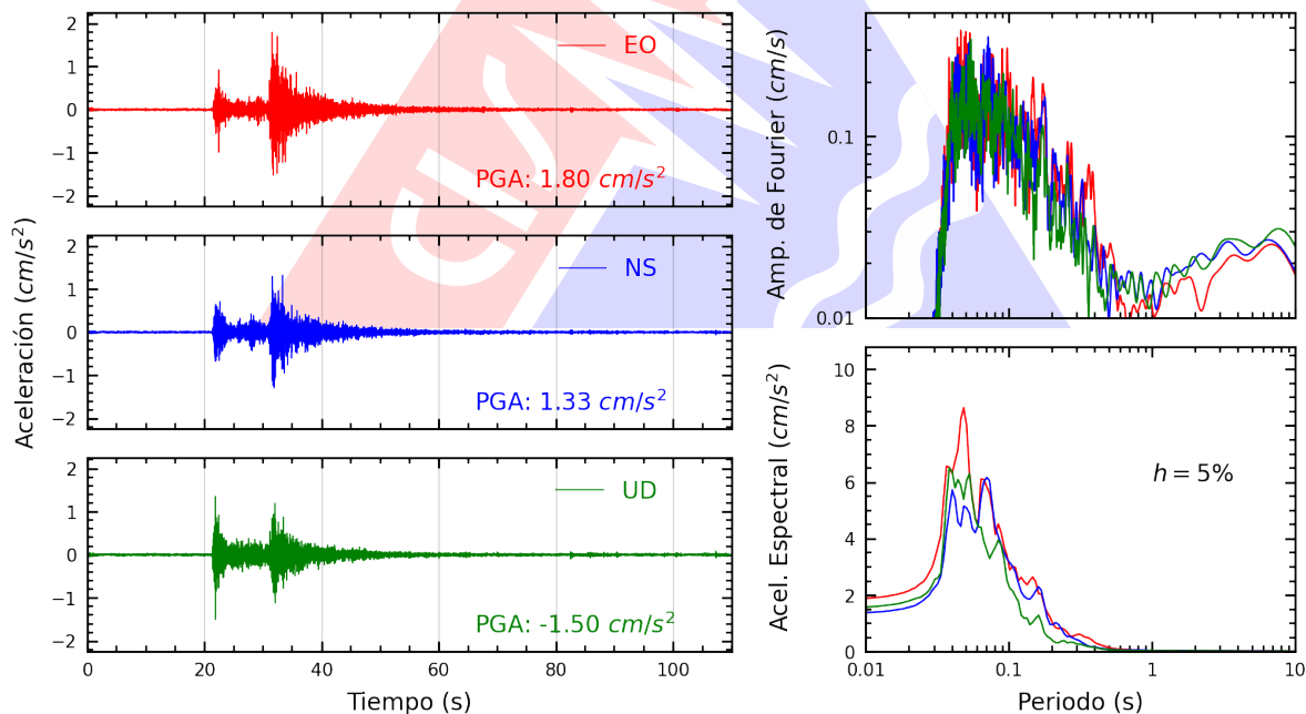
Figura A.10: Registros tiempo-historia, espectros de Fourier y de respuesta en las direcciones EO, NS y vertical de la estación UCVAT. Sismo de Lima, Lima - Lima del 2026-03-19, 23:00:37 (Hora local)
