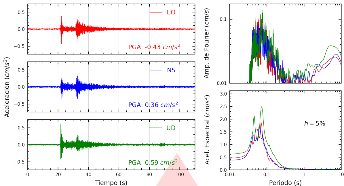
Figura A.29: Registros tiempo-historia, espectros de Fourier y de respuesta en las direcciones EO, NS y vertical de la estación UNFV. Sismo de Lima, Lima - Lima del 2026-03-19, 23:00:37 (Hora local)
