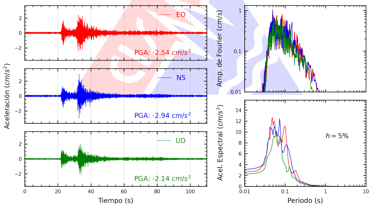
Figura A.4: Registros tiempo-historia, espectros de Fourier y de respuesta en las direcciones EO, NS y vertical de la estación UNTEL. Sismo de Lima, Lima - Lima del 2026-03-19, 23:00:37 (Hora local)
