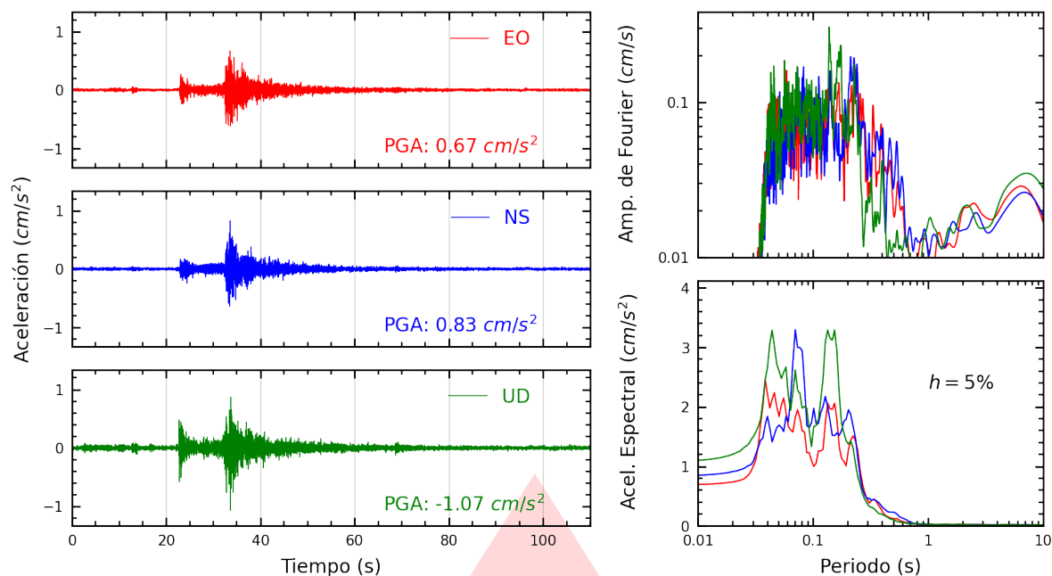
Figura A.17: Registros tiempo-historia, espectros de Fourier y de respuesta en las direcciones EO, NS y vertical de la estación MDPP. Sismo de Lima, Lima - Lima del 2026-03-19, 23:00:37 (Hora local)
