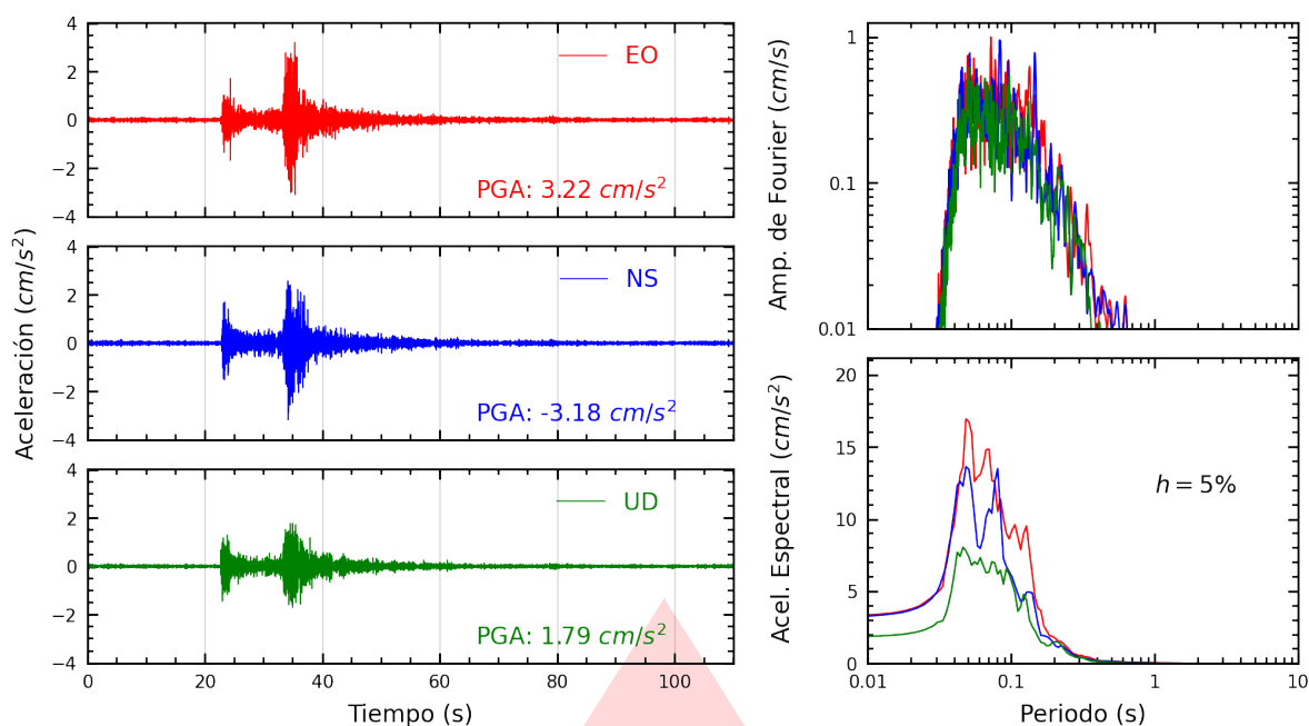
Figura A.3: Registros tiempo-historia, espectros de Fourier y de respuesta en las direcciones EO, NS y vertical de la estación PHERM. Sismo de Lima, Lima - Lima del 2026-03-19, 23:00:37 (Hora local)
