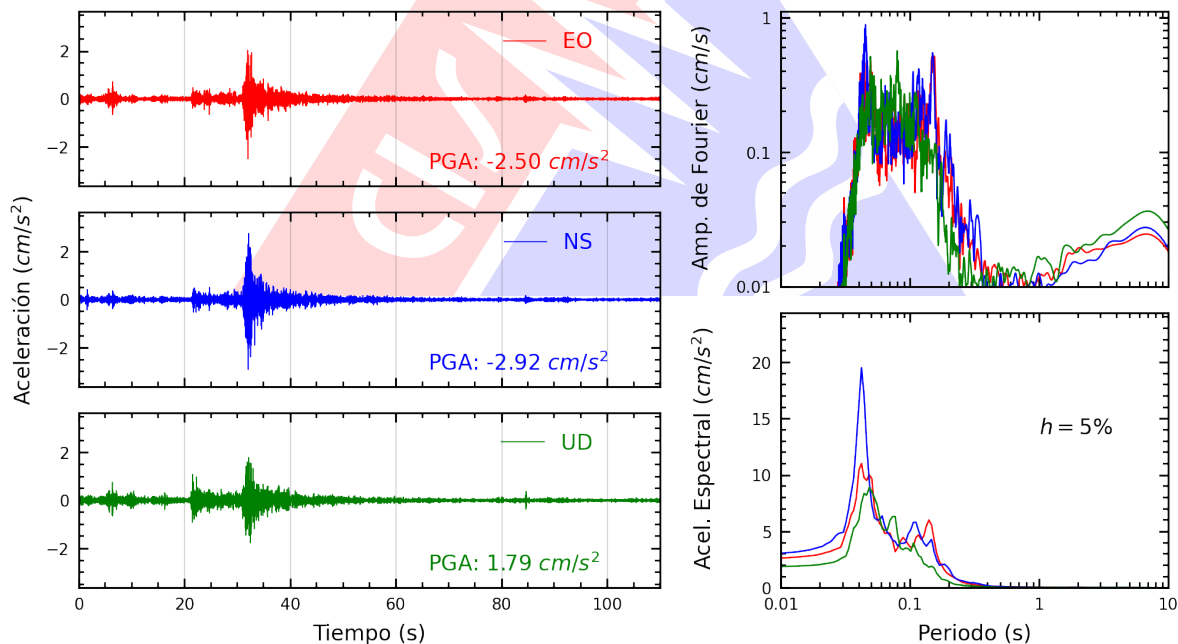
Figura A.6: Registros tiempo-historia, espectros de Fourier y de respuesta en las direcciones EO, NS y vertical de la estación CARAB. Sismo de Lima, Lima - Lima del 2026-03-19, 23:00:37 (Hora local)
