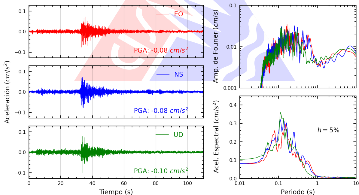
Figura A.2: Registros tiempo-historia, espectros de Fourier y de respuesta en las direcciones EO, NS y vertical de la estación CARAL. Sismo de Codo del Pozuzo, Puerto Inca - Huánuco del 2026-03-20, 11:59:56 (Hora local)
