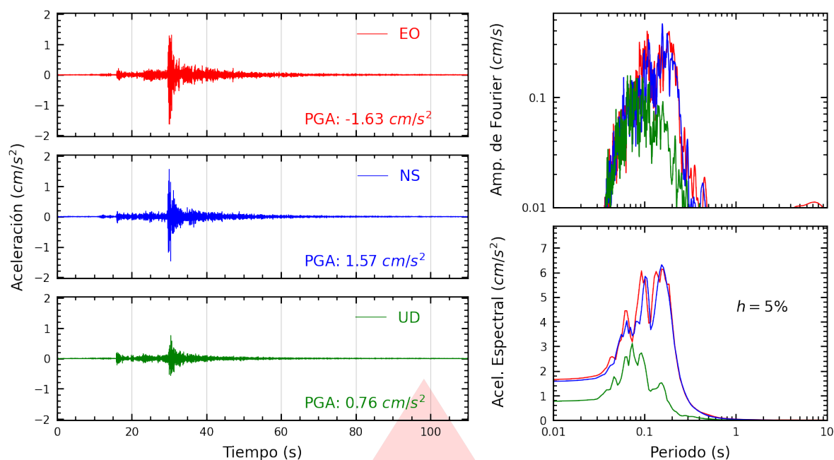
Figura A.1: Registros tiempo-historia, espectros de Fourier y de respuesta en las direcciones EO, NS y vertical de la estación UNAS. Sismo de Codo del Pozuzo, Puerto Inca - Huánuco del 2026-03-20, 11:59:56 (Hora local)
