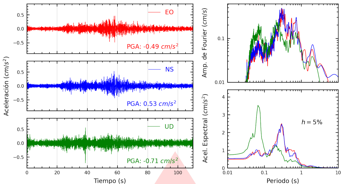
Figura A.1: Registros tiempo-historia, espectros de Fourier y de respuesta en las direcciones EO, NS y vertical de la estación SCTAC. Sismo de Tacna, Tacna - Tacna del 2026-03-20, 15:06:52 (Hora local)
