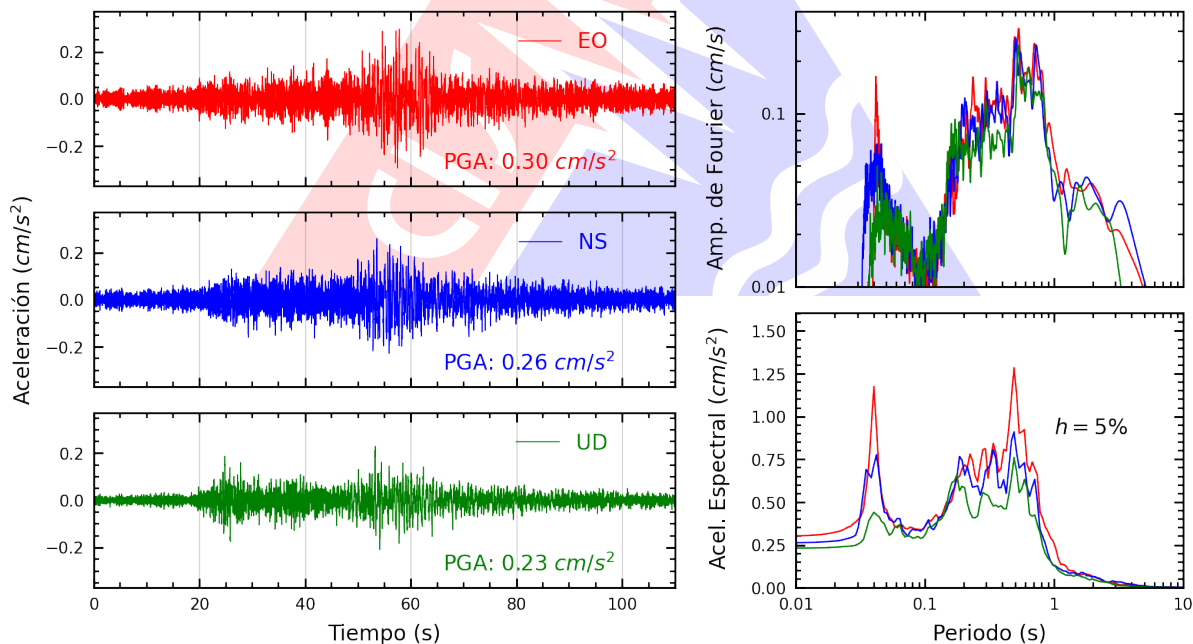
Figura A.2: Registros tiempo-historia, espectros de Fourier y de respuesta en las direcciones EO, NS y vertical de la estación UPTAC. Sismo de Tacna, Tacna - Tacna del 2026-03-20, 15:06:52 (Hora local)
