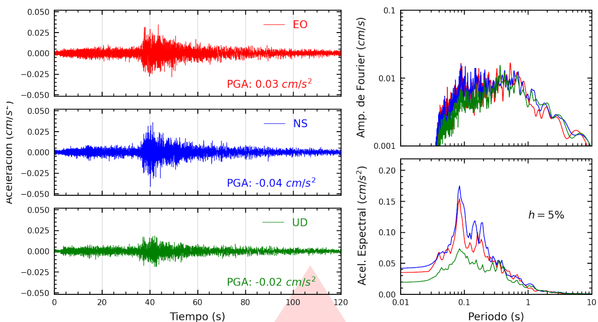
Figura A.3: Registros tiempo-historia, espectros de Fourier y de respuesta en las direcciones EO, NS y vertical de la estación UNSA2. Sismo de Tacna, Tacna - Tacna del 2026-03-20, 15:06:52 (Hora local)
