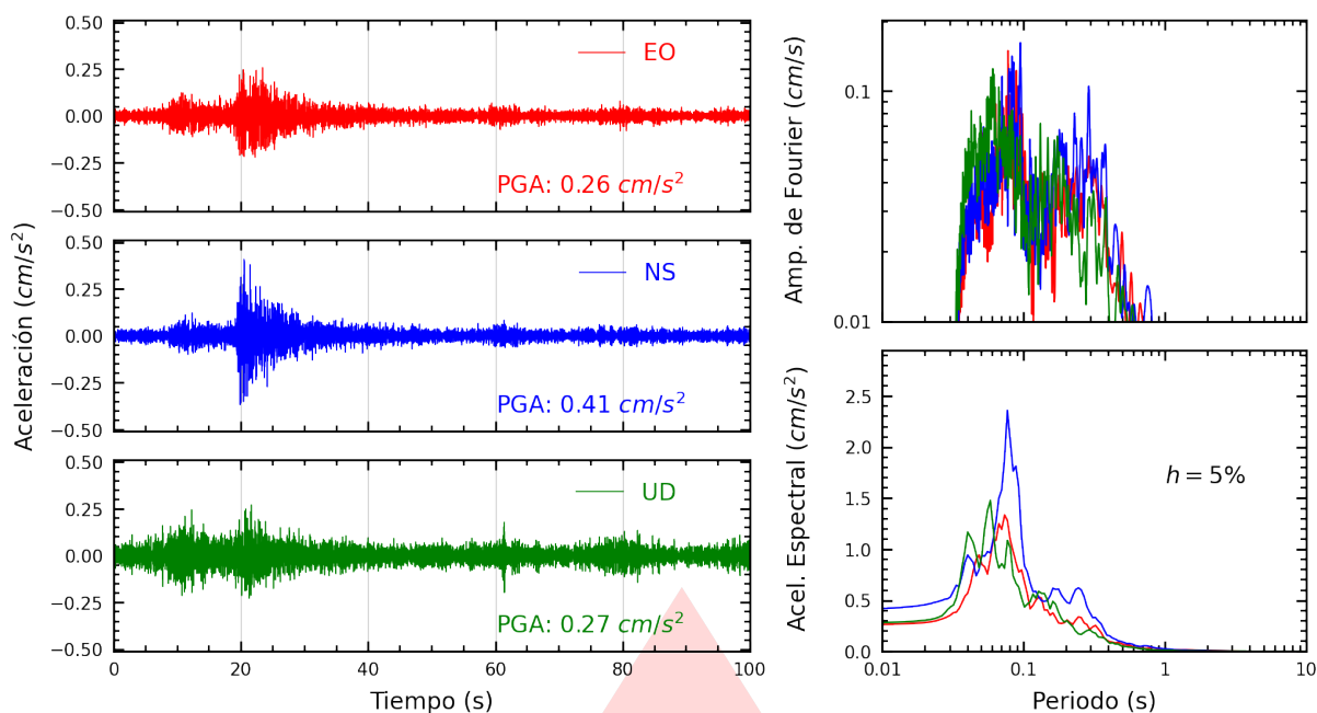
Figura A.3: Registros tiempo-historia, espectros de Fourier y de respuesta en las direcciones EO, NS y vertical de la estación UJBG2. Sismo de Tacna, Tacna - Tacna del 2026-03-20, 18:04:12 (Hora local)
