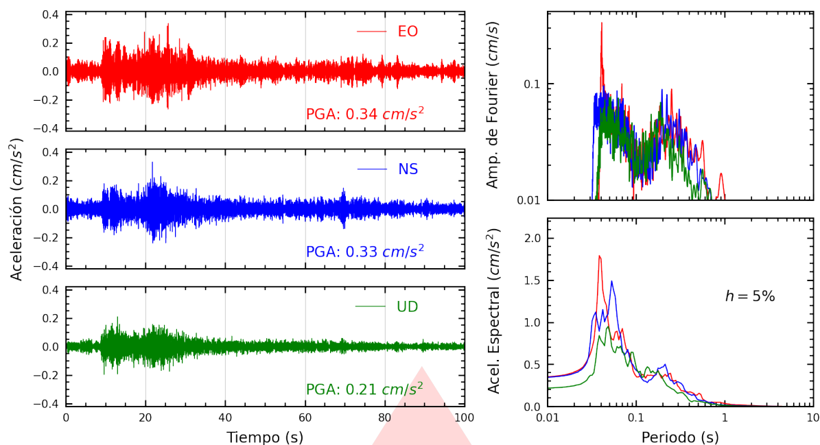
Figura A.5: Registros tiempo-historia, espectros de Fourier y de respuesta en las direcciones EO, NS y vertical de la estación UPTAC. Sismo de Tacna, Tacna - Tacna del 2026-03-20, 18:04:12 (Hora local)
