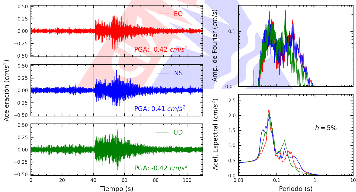
Figura A.2: Registros tiempo-historia, espectros de Fourier y de respuesta en las direcciones EO, NS y vertical de la estación UJBG4. Sismo de Tacna, Tacna - Tacna del 2026-03-20, 18:04:12 (Hora local)
