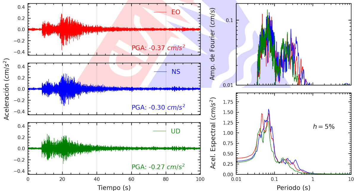
Figura A.4: Registros tiempo-historia, espectros de Fourier y de respuesta en las direcciones EO, NS y vertical de la estación CREY. Sismo de Tacna, Tacna - Tacna del 2026-03-20, 18:04:12 (Hora local)
