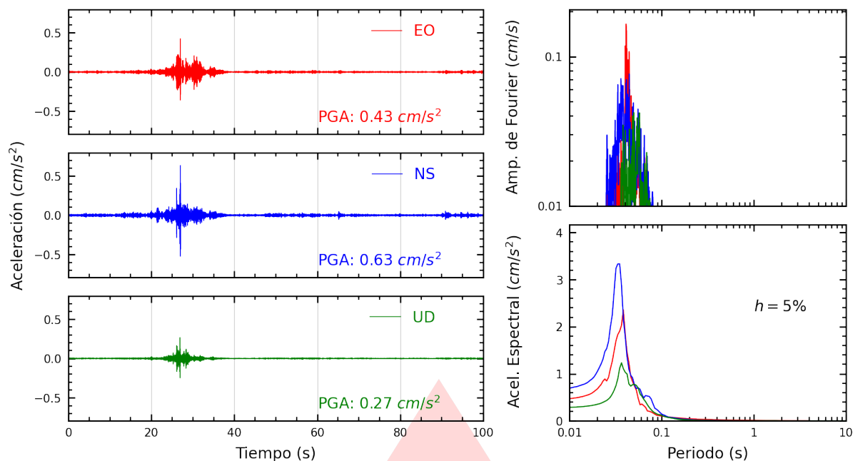
Figura A.1: Registros tiempo-historia, espectros de Fourier y de respuesta en las direcciones EO, NS y vertical de la estación UNAM. Sismo de Tacna, Tacna - Tacna del 2026-03-20, 18:04:12 (Hora local)
