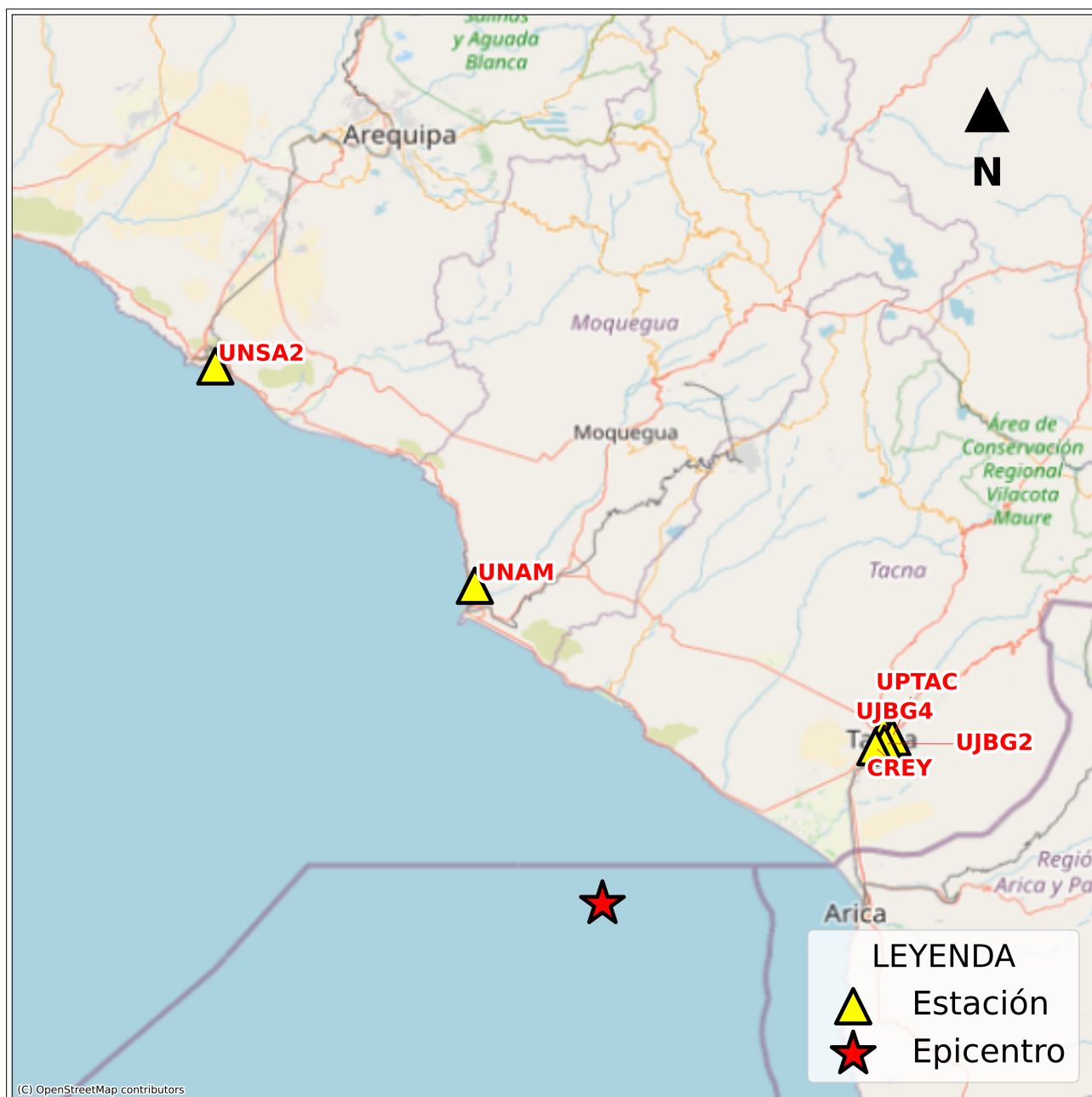
Figura 2: Mapa de ubicación de la(s) estación(es) acelerográfica(s) correspondiente(s) al Sismo de Tacna, Tacna - Tacna del 20 de marzo de 2026 a las 18:04:12 (hora local)
