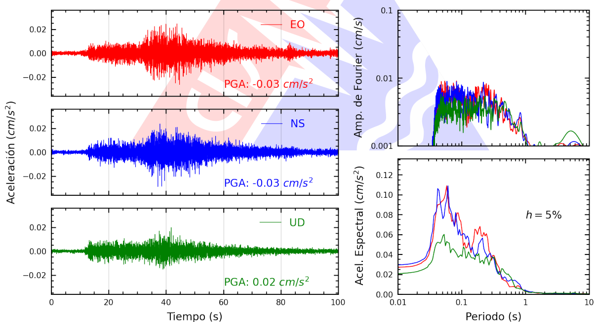
Figura A.6: Registros tiempo-historia, espectros de Fourier y de respuesta en las direcciones EO, NS y vertical de la estación UNSA2. Sismo de Tacna, Tacna - Tacna del 2026-03-20, 18:04:12 (Hora local)
