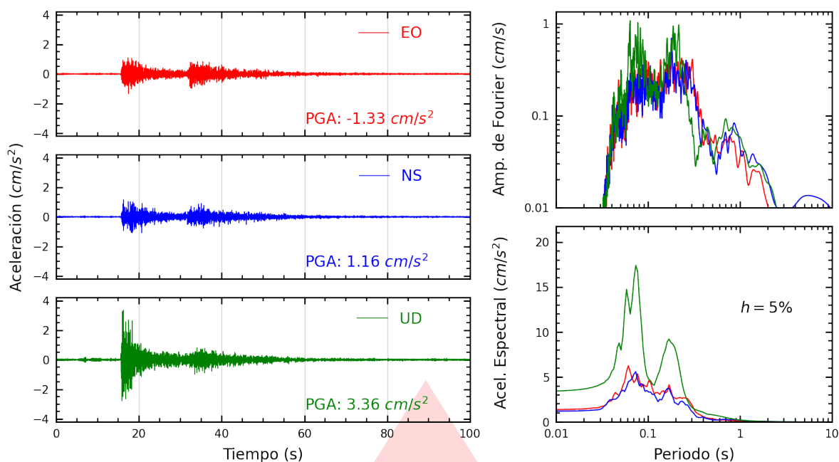
Figura A.1: Registros tiempo-historia, espectros de Fourier y de respuesta en las direcciones EO, NS y vertical de la estación SCTAC. Sismo de Calana, Tacna - Tacna del 2026-03-22, 03:02:54 (Hora local)
