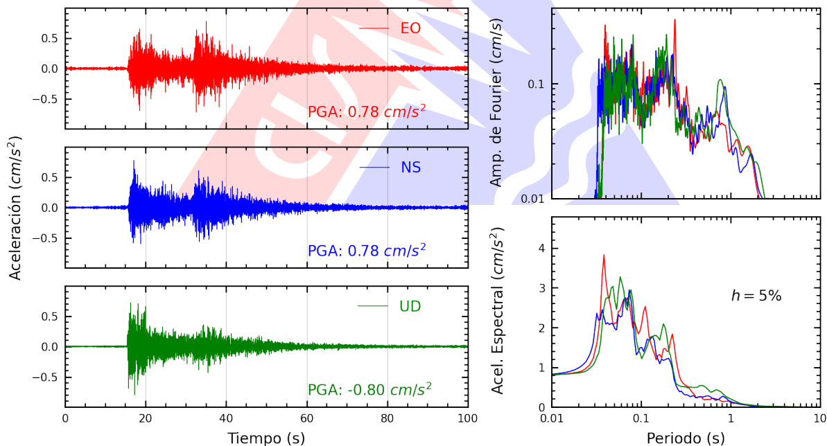
Figura A.4: Registros tiempo-historia, espectros de Fourier y de respuesta en las direcciones EO, NS y vertical de la estación UPTAC. Sismo de Calana, Tacna - Tacna del 2026-03-22, 03:02:54 (Hora local)
