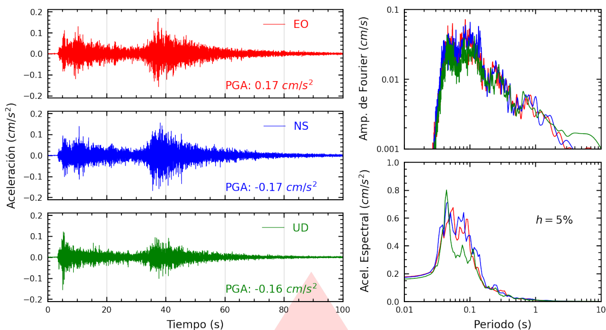
Figura A.5: Registros tiempo-historia, espectros de Fourier y de respuesta en las direcciones EO, NS y vertical de la estación UNSA2. Sismo de Calana, Tacna - Tacna del 2026-03-22, 03:02:54 (Hora local)
