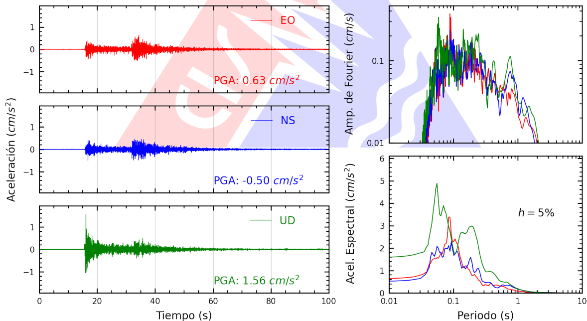
Figura A.2: Registros tiempo-historia, espectros de Fourier y de respuesta en las direcciones EO, NS y vertical de la estación UJBG2. Sismo de Calana, Tacna - Tacna del 2026-03-22, 03:02:54 (Hora local)
