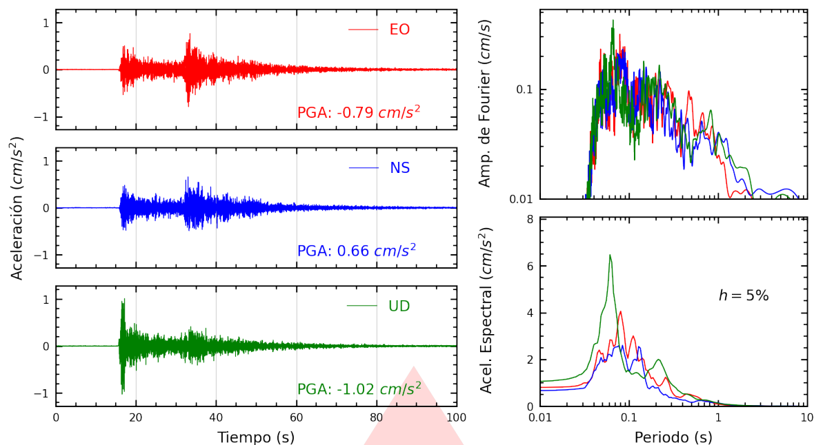
Figura A.3: Registros tiempo-historia, espectros de Fourier y de respuesta en las direcciones EO, NS y vertical de la estación CREY. Sismo de Calana, Tacna - Tacna del 2026-03-22, 03:02:54 (Hora local)
