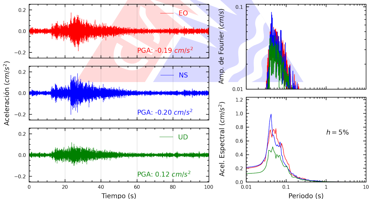
Figura A.26: Registros tiempo-historia, espectros de Fourier y de respuesta en las direcciones EO, NS y vertical de la estación BORJA. Sismo de Chilca, Cañete - Lima del 2026-03-22, 06:03:20 (Hora local)
