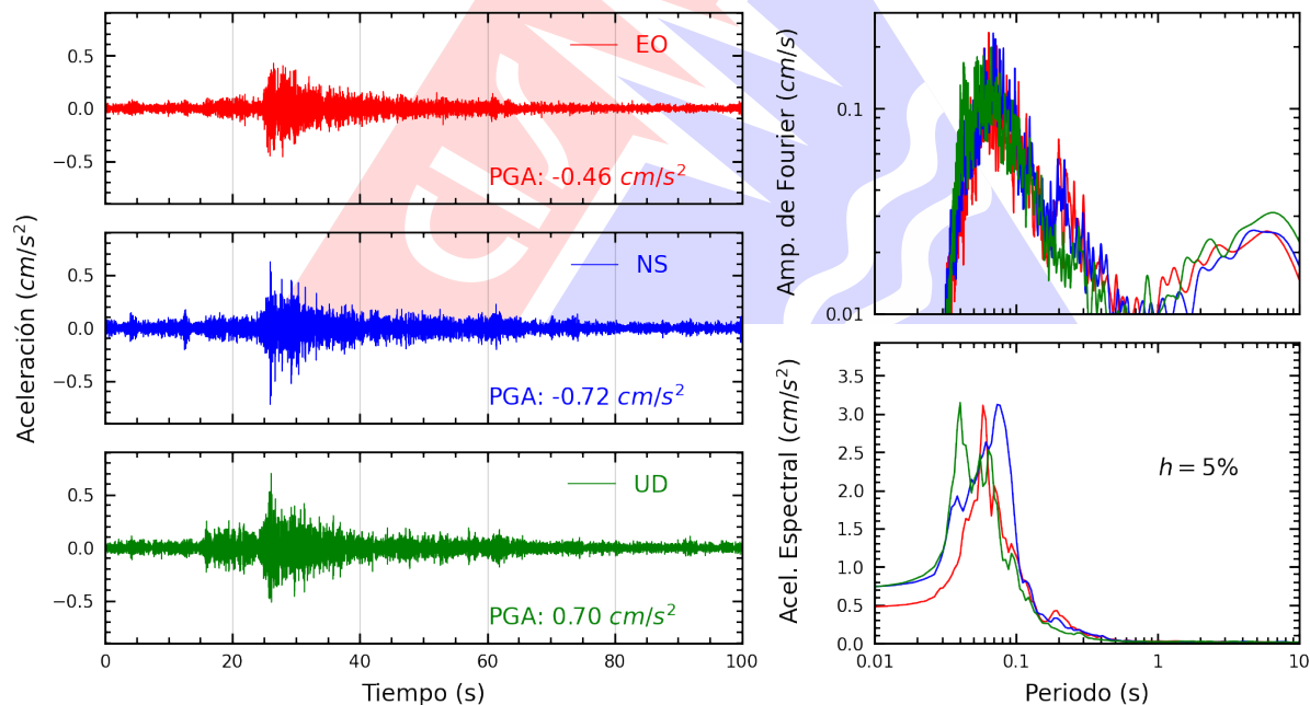
Figura A.6: Registros tiempo-historia, espectros de Fourier y de respuesta en las direcciones EO, NS y vertical de la estación SJLSC. Sismo de Chilca, Cañete - Lima del 2026-03-22, 06:03:20 (Hora local)
