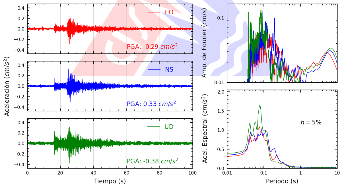
Figura A.14: Registros tiempo-historia, espectros de Fourier y de respuesta en las direcciones EO, NS y vertical de la estación SOCHO. Sismo de Chilca, Cañete - Lima del 2026-03-22, 06:03:20 (Hora local)
