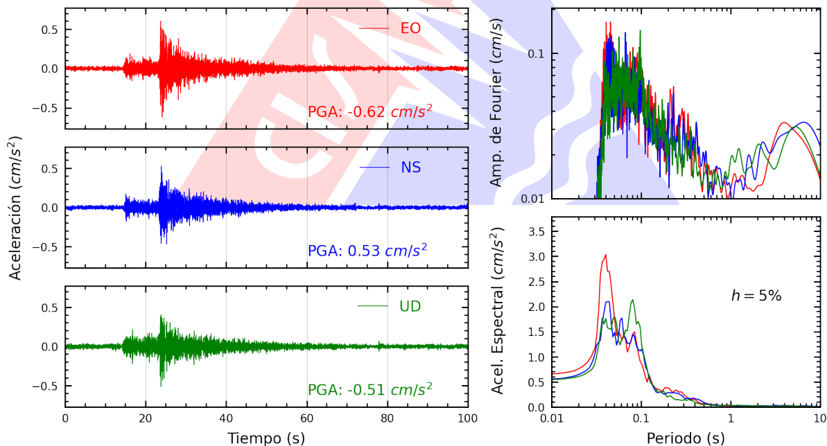
Figura A.10: Registros tiempo-historia, espectros de Fourier y de respuesta en las direcciones EO, NS y vertical de la estación UCVAT. Sismo de Chilca, Cañete - Lima del 2026-03-22, 06:03:20 (Hora local)
