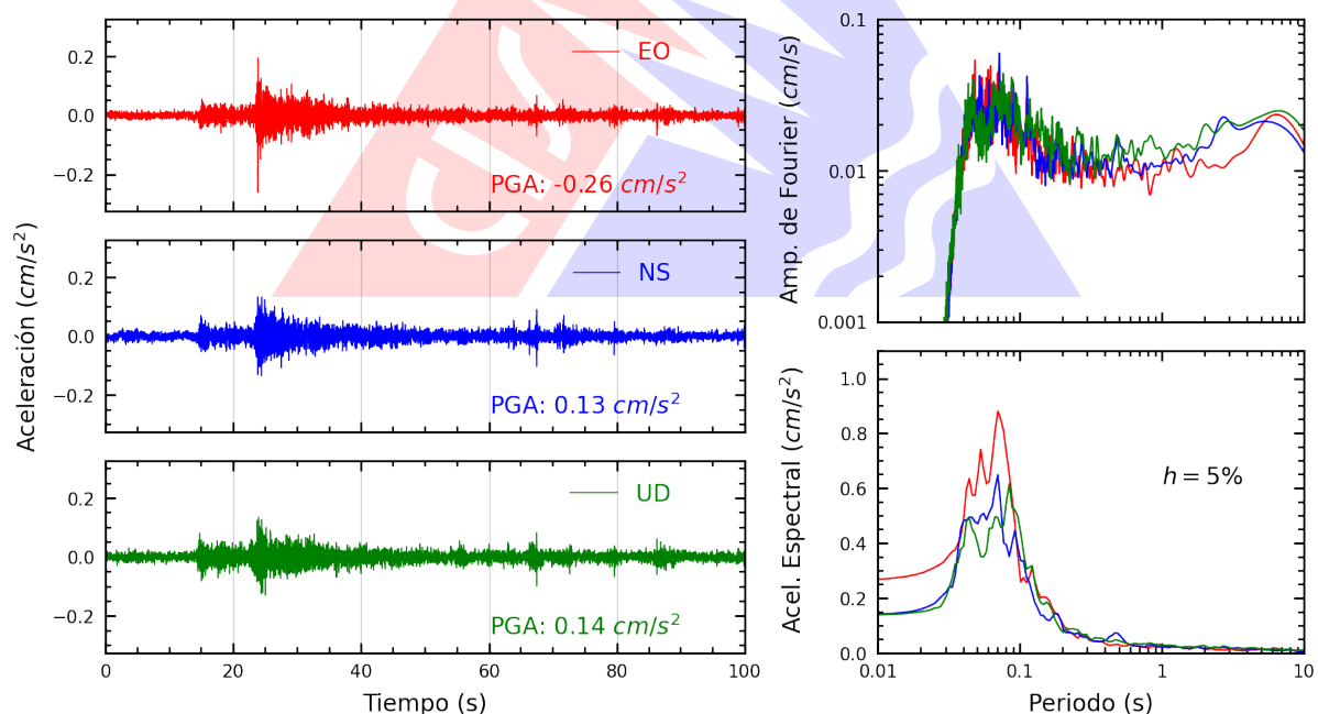
Figura A.24: Registros tiempo-historia, espectros de Fourier y de respuesta en las direcciones EO, NS y vertical de la estación UNFV. Sismo de Chilca, Cañete - Lima del 2026-03-22, 06:03:20 (Hora local)
