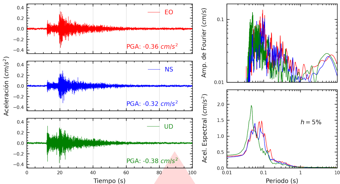
Figura A.15: Registros tiempo-historia, espectros de Fourier y de respuesta en las direcciones EO, NS y vertical de la estación USILP. Sismo de Chilca, Cañete - Lima del 2026-03-22, 06:03:20 (Hora local)
