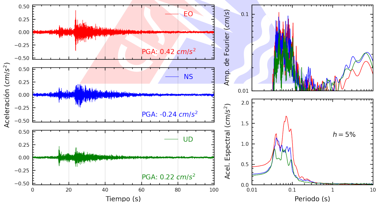
Figura A.12: Registros tiempo-historia, espectros de Fourier y de respuesta en las direcciones EO, NS y vertical de la estación CEPRE. Sismo de Chilca, Cañete - Lima del 2026-03-22, 06:03:20 (Hora local)
