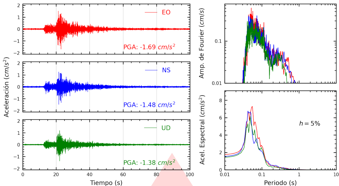
Figura A.3: Registros tiempo-historia, espectros de Fourier y de respuesta en las direcciones EO, NS y vertical de la estación UNTEL. Sismo de Chilca, Cañete - Lima del 2026-03-22, 06:03:20 (Hora local)
