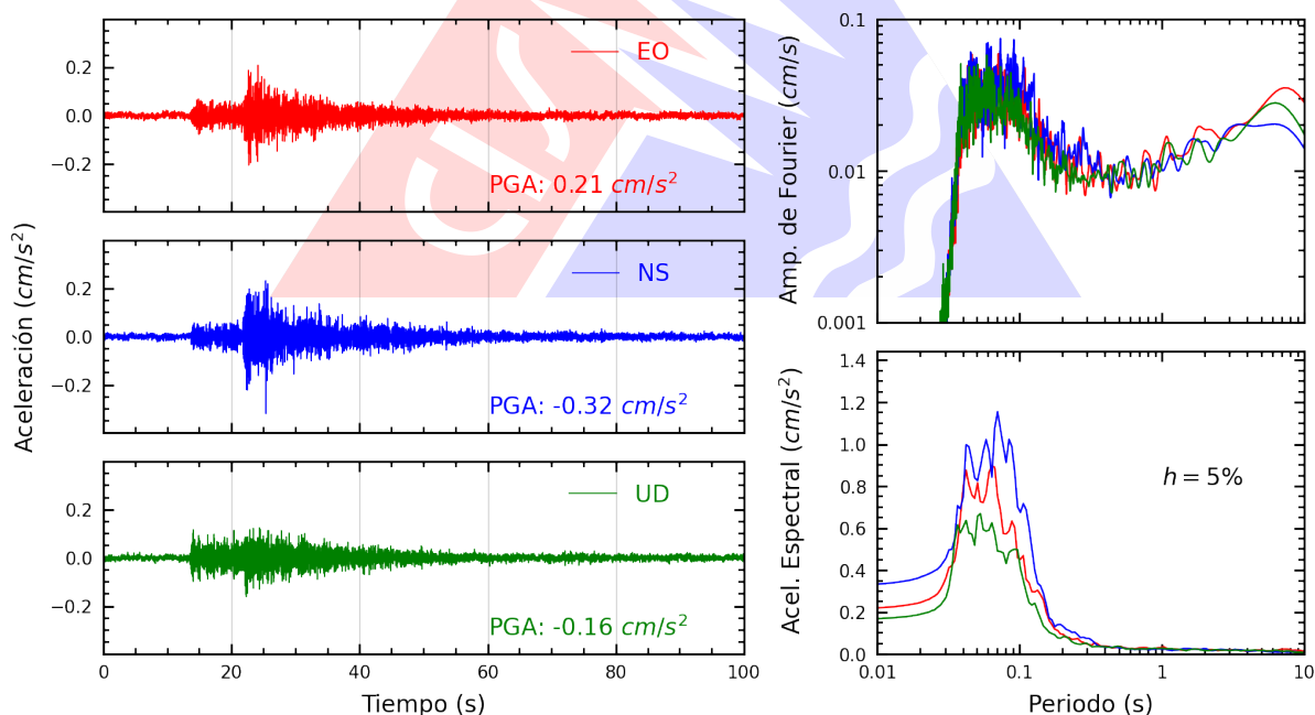
Figura A.20: Registros tiempo-historia, espectros de Fourier y de respuesta en las direcciones EO, NS y vertical de la estación SERVI. Sismo de Chilca, Cañete - Lima del 2026-03-22, 06:03:20 (Hora local)
