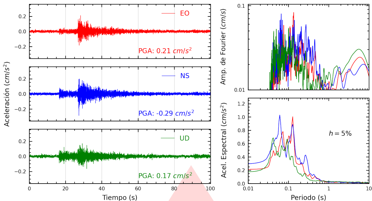
Figura A.21: Registros tiempo-historia, espectros de Fourier y de respuesta en las direcciones EO, NS y vertical de la estación VHAYA. Sismo de Chilca, Cañete - Lima del 2026-03-22, 06:03:20 (Hora local)
