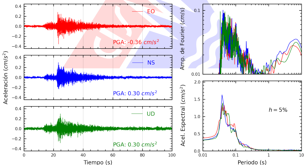
Figura A.16: Registros tiempo-historia, espectros de Fourier y de respuesta en las direcciones EO, NS y vertical de la estación USMP. Sismo de Chilca, Cañete - Lima del 2026-03-22, 06:03:20 (Hora local)
