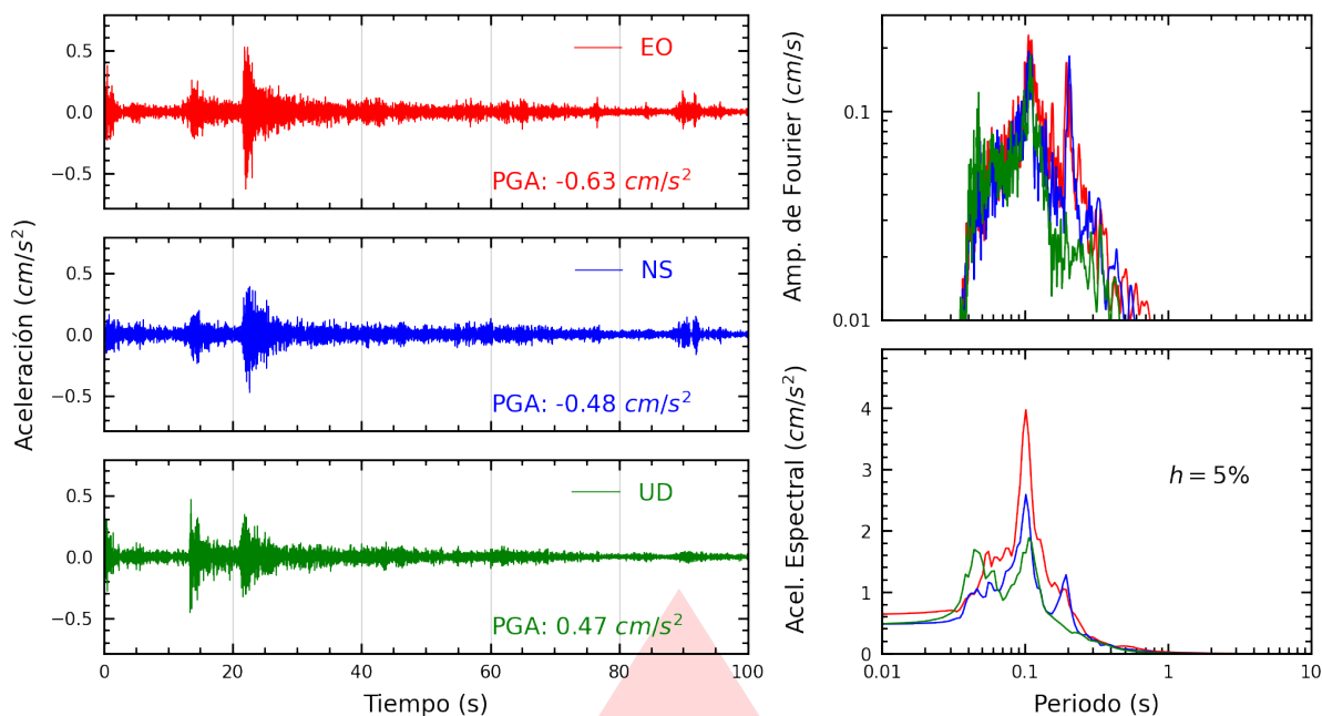
Figura A.9: Registros tiempo-historia, espectros de Fourier y de respuesta en las direcciones EO, NS y vertical de la estación SCCHO. Sismo de Chilca, Cañete - Lima del 2026-03-22, 06:03:20 (Hora local)
