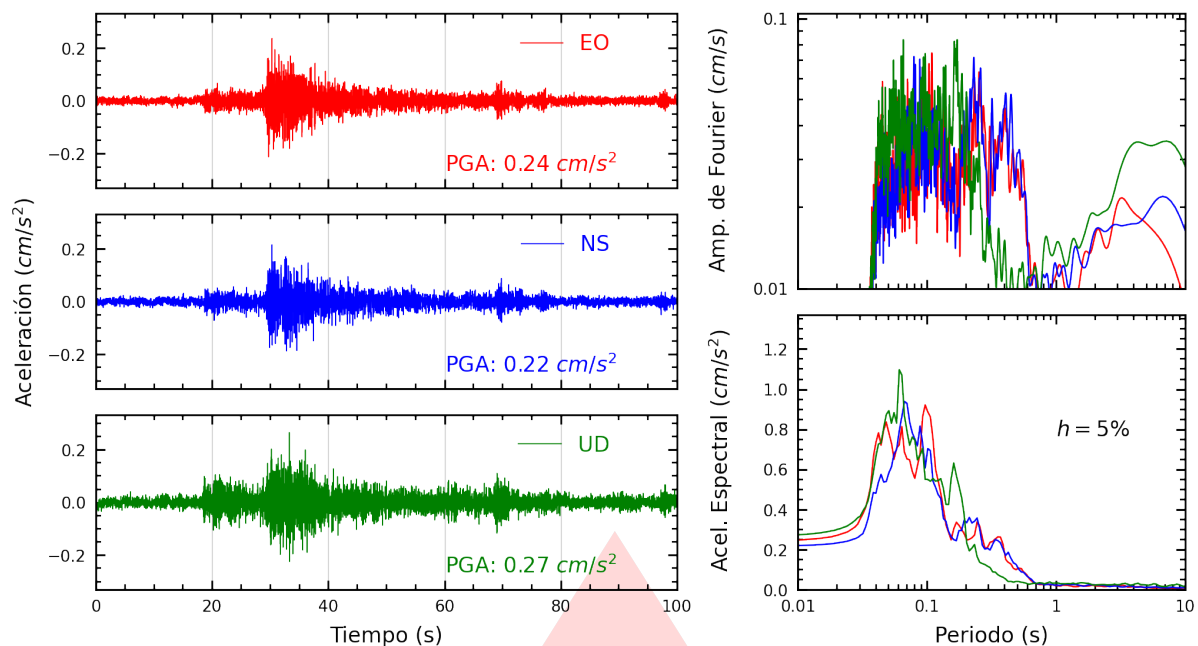
Figura A.23: Registros tiempo-historia, espectros de Fourier y de respuesta en las direcciones EO, NS y vertical de la estación MDPP. Sismo de Chilca, Cañete - Lima del 2026-03-22, 06:03:20 (Hora local)
