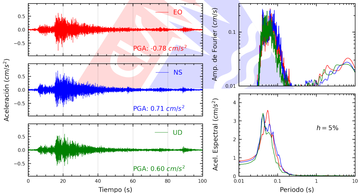
Figura A.4: Registros tiempo-historia, espectros de Fourier y de respuesta en las direcciones EO, NS y vertical de la estación JOSEO. Sismo de Chilca, Cañete - Lima del 2026-03-22, 06:03:20 (Hora local)
