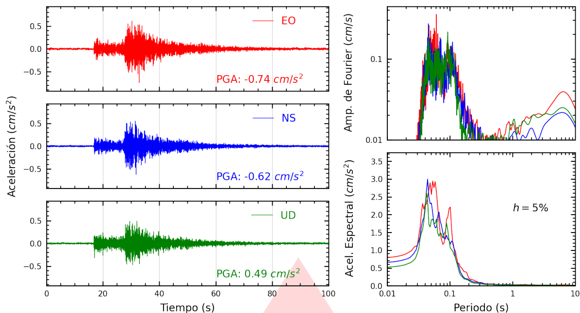
Figura A.5: Registros tiempo-historia, espectros de Fourier y de respuesta en las direcciones EO, NS y vertical de la estación AMORE. Sismo de Chilca, Cañete - Lima del 2026-03-22, 06:03:20 (Hora local)
