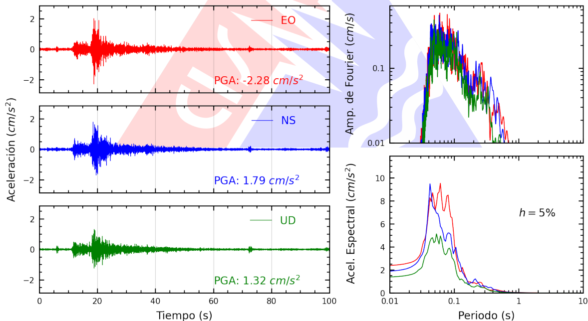
Figura A.2: Registros tiempo-historia, espectros de Fourier y de respuesta en las direcciones EO, NS y vertical de la estación PHERM. Sismo de Chilca, Cañete - Lima del 2026-03-22, 06:03:20 (Hora local)
