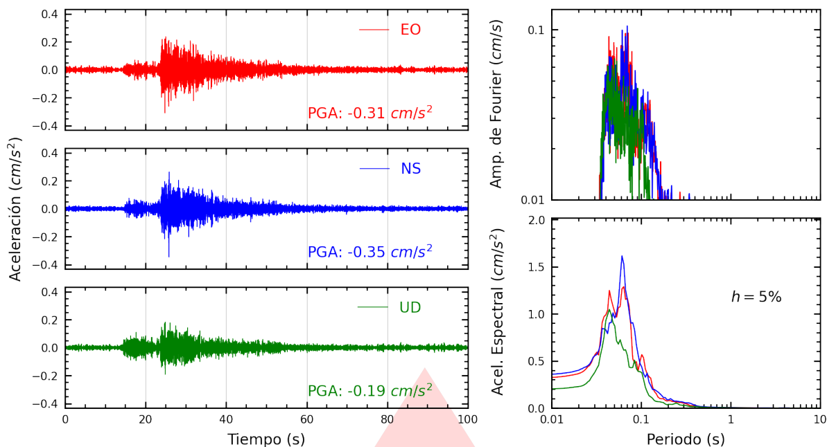
Figura A.17: Registros tiempo-historia, espectros de Fourier y de respuesta en las direcciones EO, NS y vertical de la estación ATARJ. Sismo de Chilca, Cañete - Lima del 2026-03-22, 06:03:20 (Hora local)
