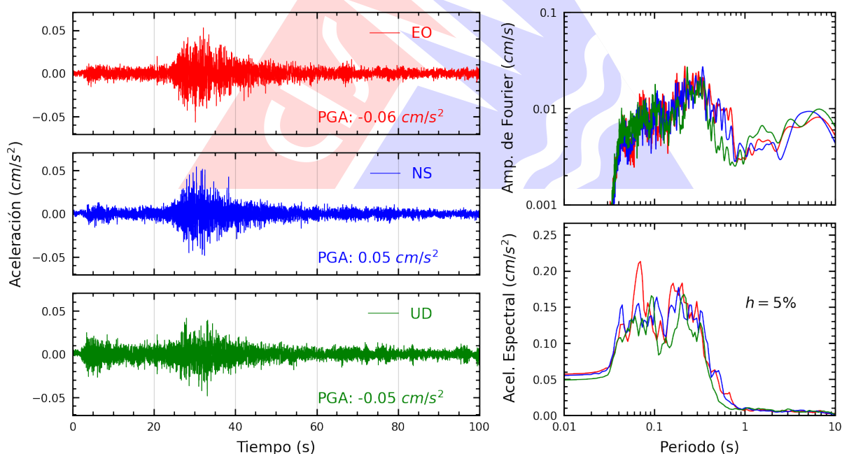
Figura A.28: Registros tiempo-historia, espectros de Fourier y de respuesta en las direcciones EO, NS y vertical de la estación CARAL. Sismo de Chilca, Cañete - Lima del 2026-03-22, 06:03:20 (Hora local)
