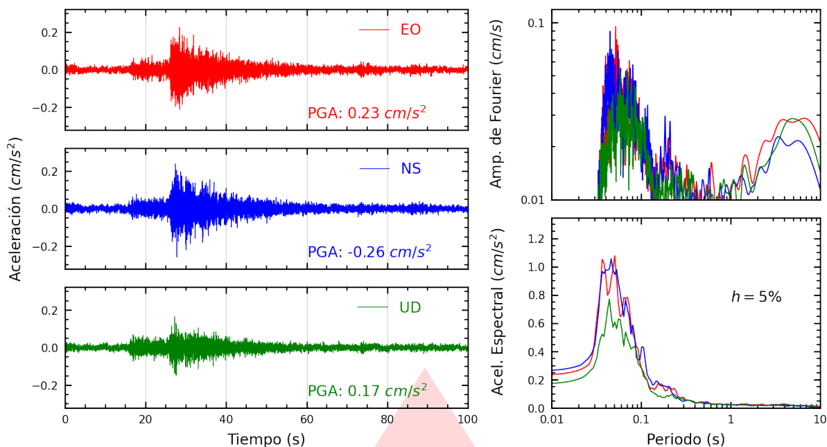
Figura A.25: Registros tiempo-historia, espectros de Fourier y de respuesta en las direcciones EO, NS y vertical de la estación COMAS. Sismo de Chilca, Cañete - Lima del 2026-03-22, 06:03:20 (Hora local)
