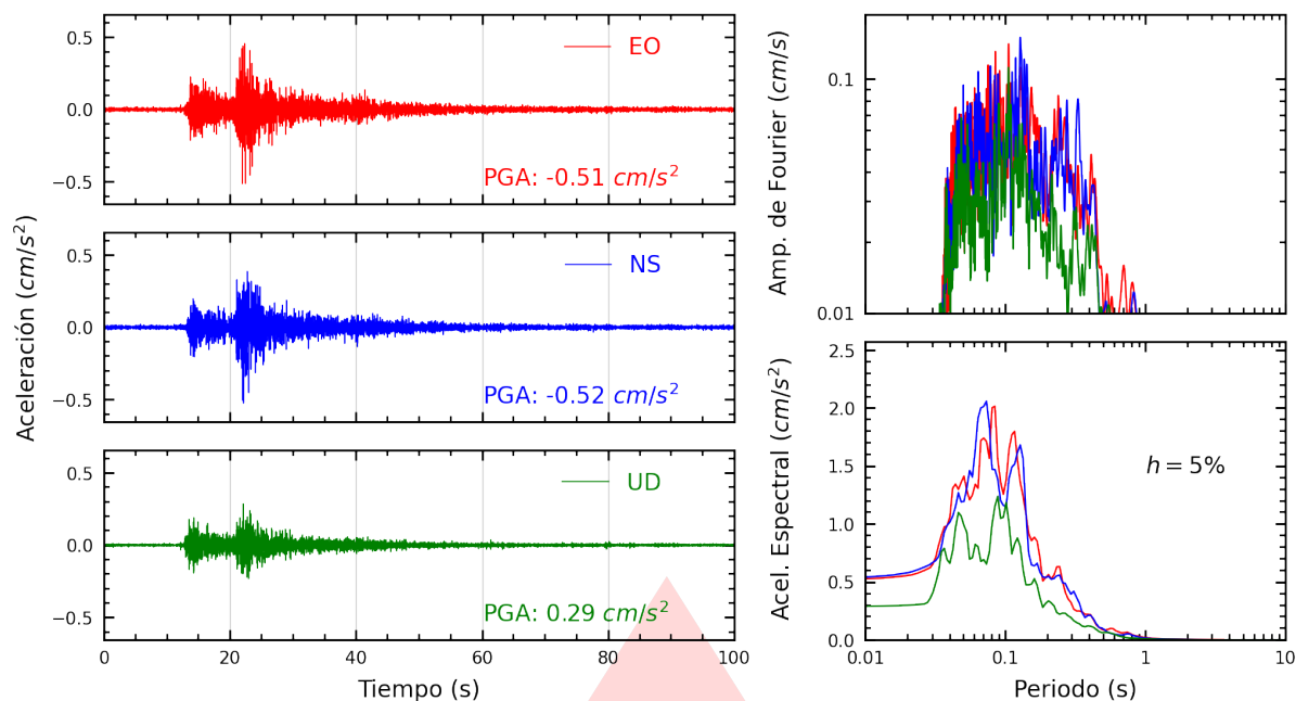
Figura A.11: Registros tiempo-historia, espectros de Fourier y de respuesta en las direcciones EO, NS y vertical de la estación BRISA. Sismo de Chilca, Cañete - Lima del 2026-03-22, 06:03:20 (Hora local)
