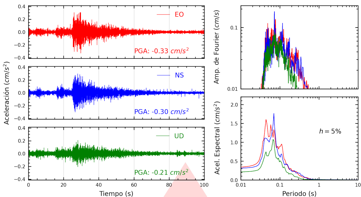
Figura A.19: Registros tiempo-historia, espectros de Fourier y de respuesta en las direcciones EO, NS y vertical de la estación SCOLI. Sismo de Chilca, Cañete - Lima del 2026-03-22, 06:03:20 (Hora local)
