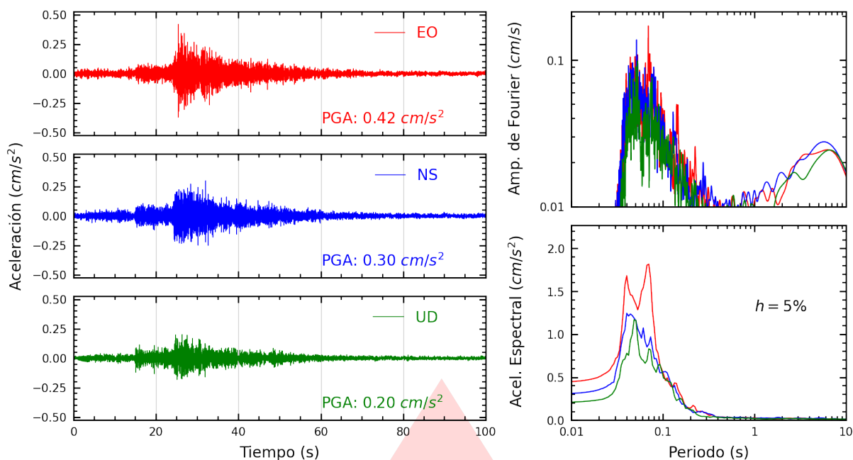
Figura A.13: Registros tiempo-historia, espectros de Fourier y de respuesta en las direcciones EO, NS y vertical de la estación FICPE. Sismo de Chilca, Cañete - Lima del 2026-03-22, 06:03:20 (Hora local)
