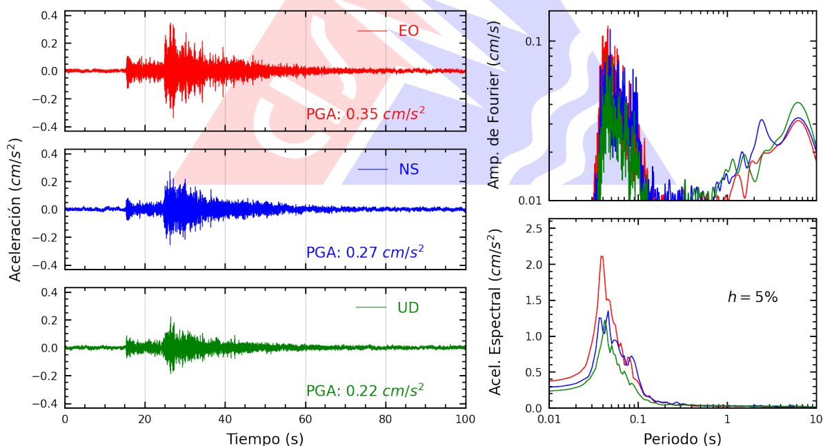
Figura A.18: Registros tiempo-historia, espectros de Fourier y de respuesta en las direcciones EO, NS y vertical de la estación UCSS. Sismo de Chilca, Cañete - Lima del 2026-03-22, 06:03:20 (Hora local)
