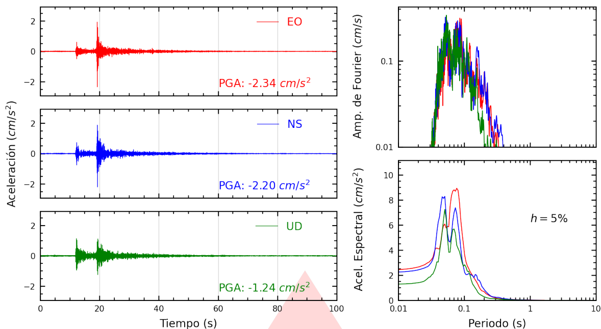
Figura A.1: Registros tiempo-historia, espectros de Fourier y de respuesta en las direcciones EO, NS y vertical de la estación ASIA. Sismo de Chilca, Cañete - Lima del 2026-03-22, 06:03:20 (Hora local)
