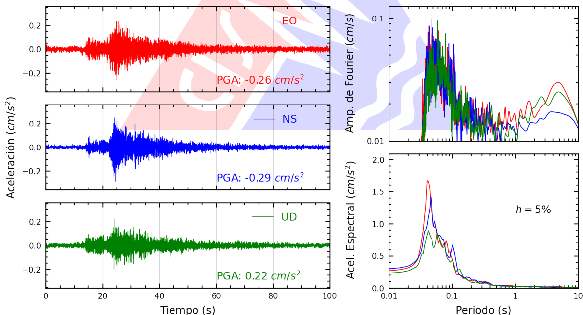
Figura A.22: Registros tiempo-historia, espectros de Fourier y de respuesta en las direcciones EO, NS y vertical de la estación IMCA. Sismo de Chilca, Cañete - Lima del 2026-03-22, 06:03:20 (Hora local)
