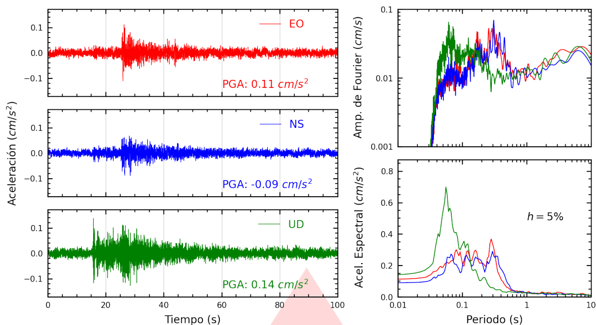
Figura A.27: Registros tiempo-historia, espectros de Fourier y de respuesta en las direcciones EO, NS y vertical de la estación ACAPU. Sismo de Chilca, Cañete - Lima del 2026-03-22, 06:03:20 (Hora local)
