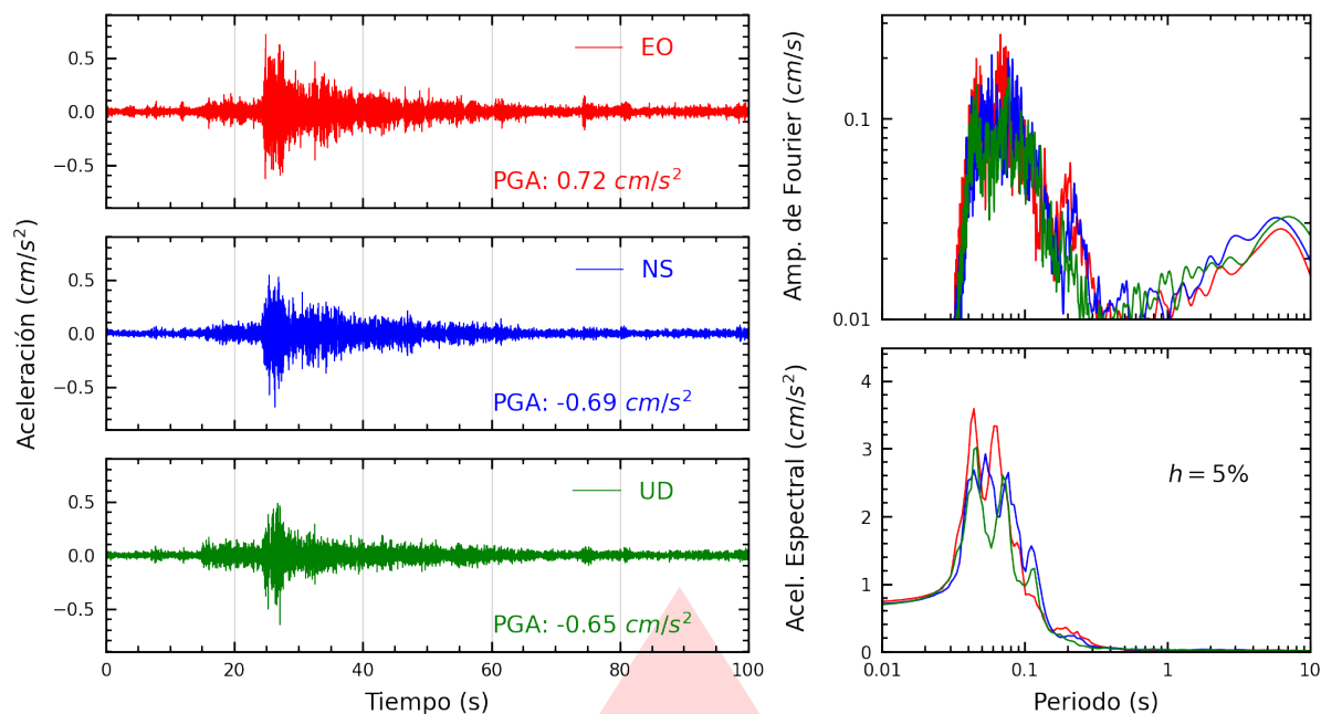
Figura A.7: Registros tiempo-historia, espectros de Fourier y de respuesta en las direcciones EO, NS y vertical de la estación INDEP. Sismo de Chilca, Cañete - Lima del 2026-03-22, 06:03:20 (Hora local)
