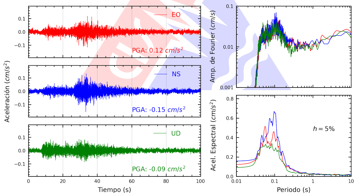
Figura A.6: Registros tiempo-historia, espectros de Fourier y de respuesta en las direcciones EO, NS y vertical de la estación SERVI. Sismo de Pisco, Pisco - Ica del 2026-03-22, 06:36:49 (Hora local)
