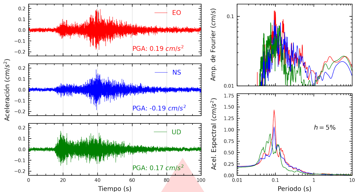
Figura A.5: Registros tiempo-historia, espectros de Fourier y de respuesta en las direcciones EO, NS y vertical de la estación USILP. Sismo de Pisco, Pisco - Ica del 2026-03-22, 06:36:49 (Hora local)
