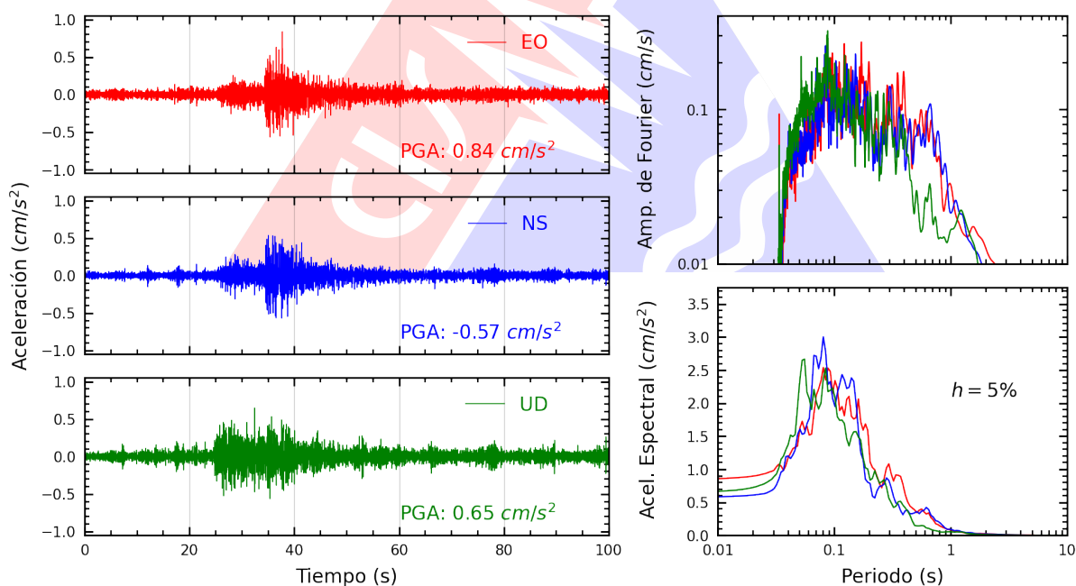
Figura A.2: Registros tiempo-historia, espectros de Fourier y de respuesta en las direcciones EO, NS y vertical de la estación SCICA. Sismo de Pisco, Pisco - Ica del 2026-03-22, 06:36:49 (Hora local)
