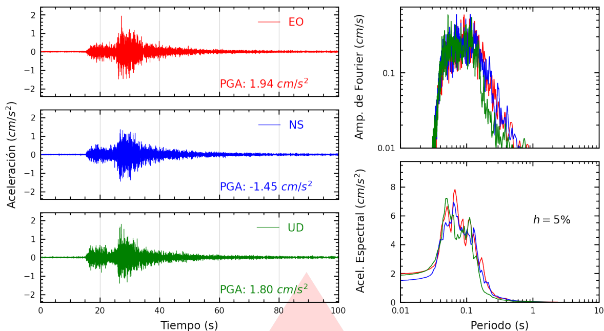
Figura A.1: Registros tiempo-historia, espectros de Fourier y de respuesta en las direcciones EO, NS y vertical de la estación ASIA. Sismo de Pisco, Pisco - Ica del 2026-03-22, 06:36:49 (Hora local)
