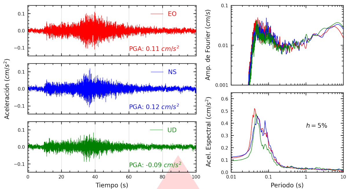
Figura A.7: Registros tiempo-historia, espectros de Fourier y de respuesta en las direcciones EO, NS y vertical de la estación UCSS. Sismo de Pisco, Pisco - Ica del 2026-03-22, 06:36:49 (Hora local)
