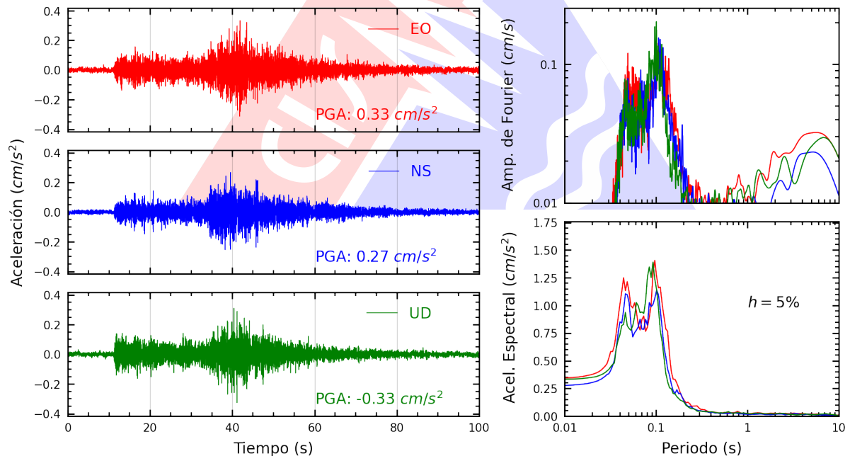
Figura A.4: Registros tiempo-historia, espectros de Fourier y de respuesta en las direcciones EO, NS y vertical de la estación AMORE. Sismo de Pisco, Pisco - Ica del 2026-03-22, 06:36:49 (Hora local)
