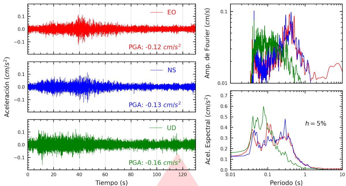
Figura A.1: Registros tiempo-historia, espectros de Fourier y de respuesta en las direcciones EO, NS y vertical de la estación SCPIU. Sismo de Zarumilla, Zarumilla - Tumbes del 2026-03-23, 12:46:03 (Hora local)
