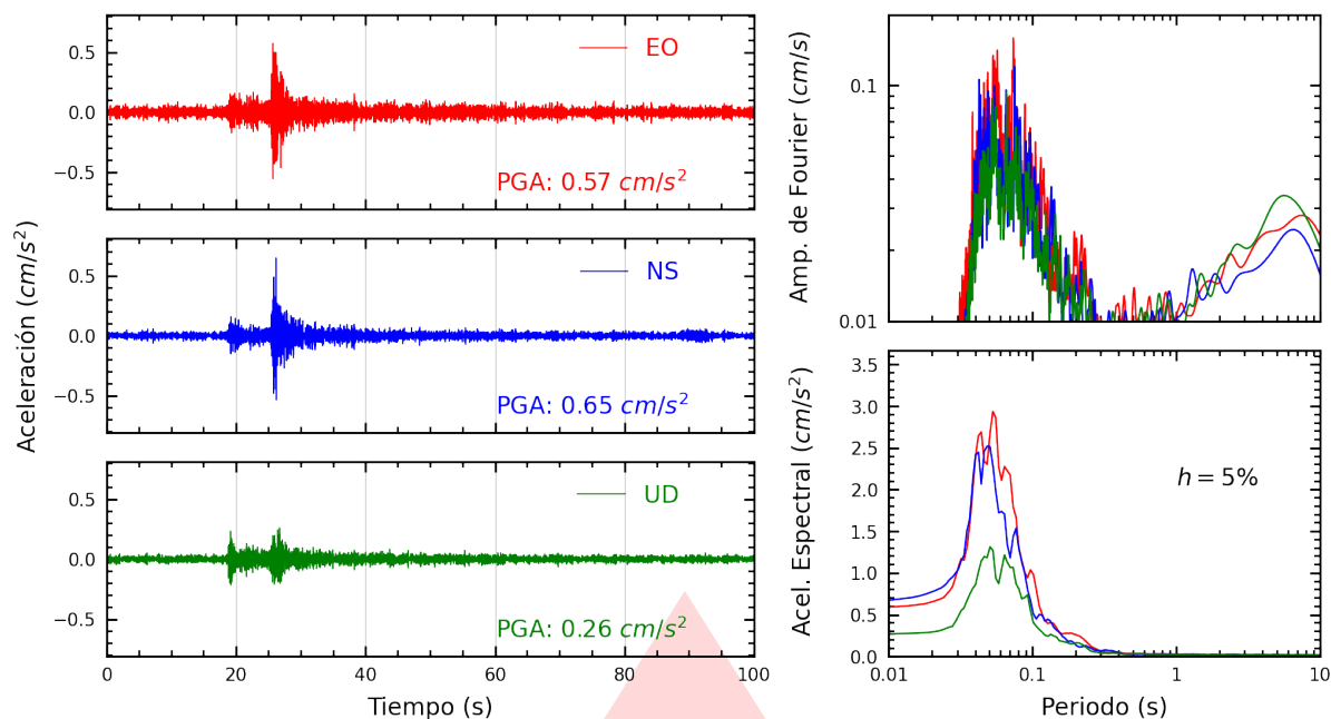
Figura A.25: Registros tiempo-historia, espectros de Fourier y de respuesta en las direcciones EO, NS y vertical de la estación INICT. Sismo de Callao, Provincia Constitucional del Callao del 2026-03-24, 21:21:08 (Hora local)
