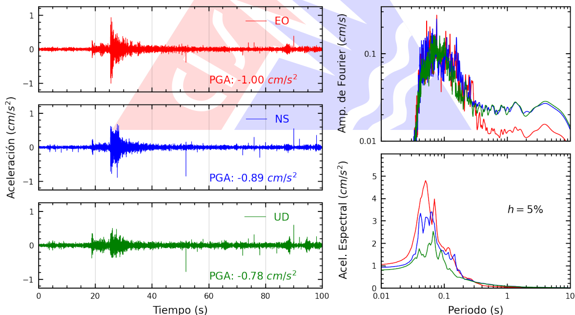
Figura A.12: Registros tiempo-historia, espectros de Fourier y de respuesta en las direcciones EO, NS y vertical de la estación SCOLI. Sismo de Callao, Provincia Constitucional del Callao del 2026-03-24, 21:21:08 (Hora local)
