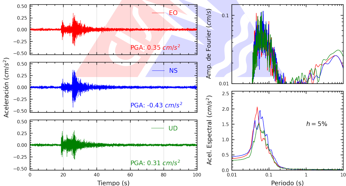
Figura A.26: Registros tiempo-historia, espectros de Fourier y de respuesta en las direcciones EO, NS y vertical de la estación SERVI. Sismo de Callao, Provincia Constitucional del Callao del 2026-03-24, 21:21:08 (Hora local)
