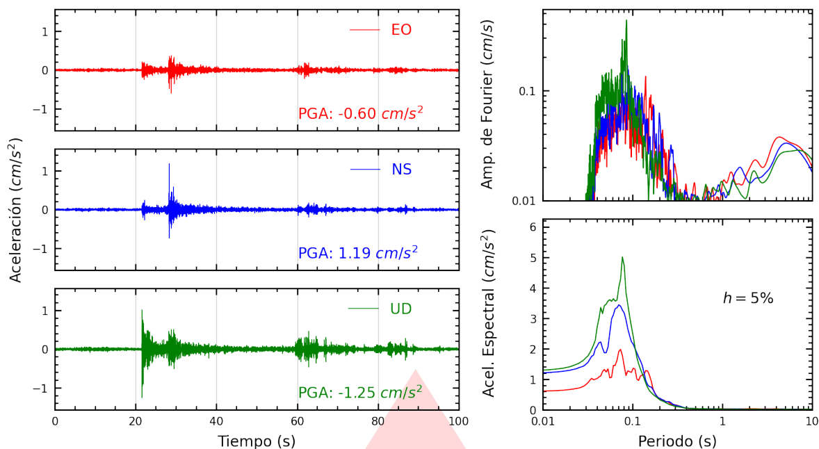
Figura A.9: Registros tiempo-historia, espectros de Fourier y de respuesta en las direcciones EO, NS y vertical de la estación SOCHO. Sismo de Callao, Provincia Constitucional del Callao del 2026-03-24, 21:21:08 (Hora local)
