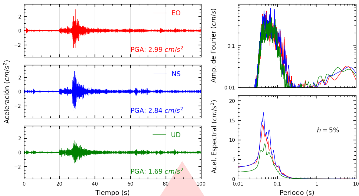
Figura A.1: Registros tiempo-historia, espectros de Fourier y de respuesta en las direcciones EO, NS y vertical de la estación SROSA. Sismo de Callao, Provincia Constitucional del Callao del 2026-03-24, 21:21:08 (Hora local)
