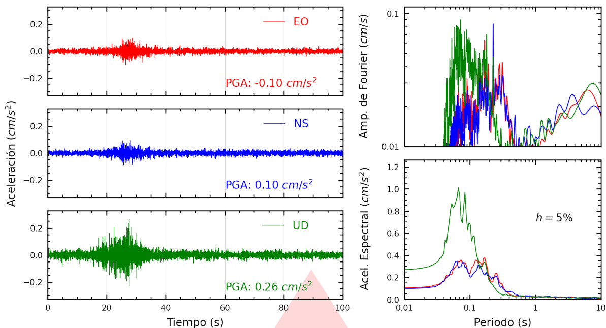
Figura A.31: Registros tiempo-historia, espectros de Fourier y de respuesta en las direcciones EO, NS y vertical de la estación ACAPU. Sismo de Callao, Provincia Constitucional del Callao del 2026-03-24, 21:21:08 (Hora local)
