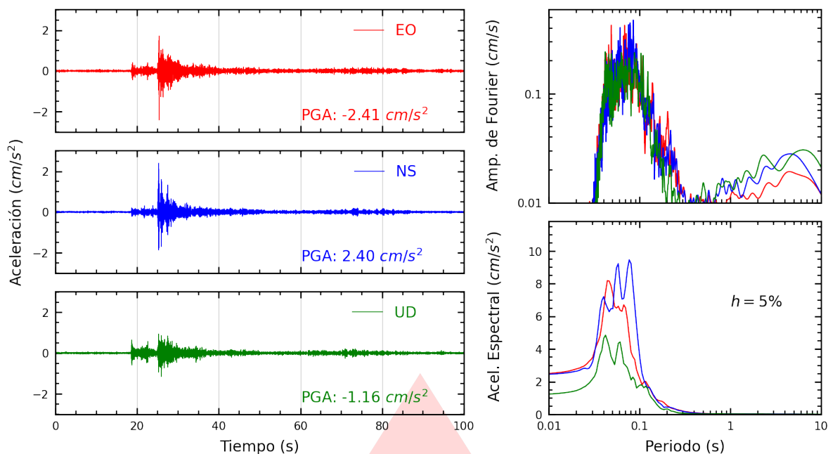
Figura A.3: Registros tiempo-historia, espectros de Fourier y de respuesta en las direcciones EO, NS y vertical de la estación INDEP. Sismo de Callao, Provincia Constitucional del Callao del 2026-03-24, 21:21:08 (Hora local)
