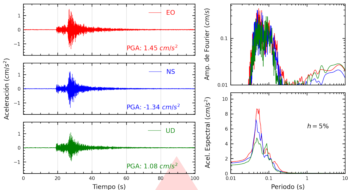
Figura A.7: Registros tiempo-historia, espectros de Fourier y de respuesta en las direcciones EO, NS y vertical de la estación AMORE. Sismo de Callao, Provincia Constitucional del Callao del 2026-03-24, 21:21:08 (Hora local)
