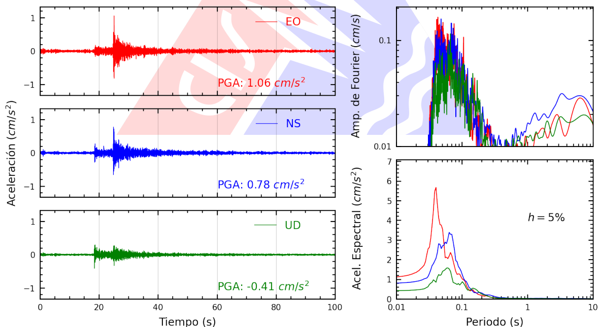
Figura A.10: Registros tiempo-historia, espectros de Fourier y de respuesta en las direcciones EO, NS y vertical de la estación CEPRE. Sismo de Callao, Provincia Constitucional del Callao del 2026-03-24, 21:21:08 (Hora local)
