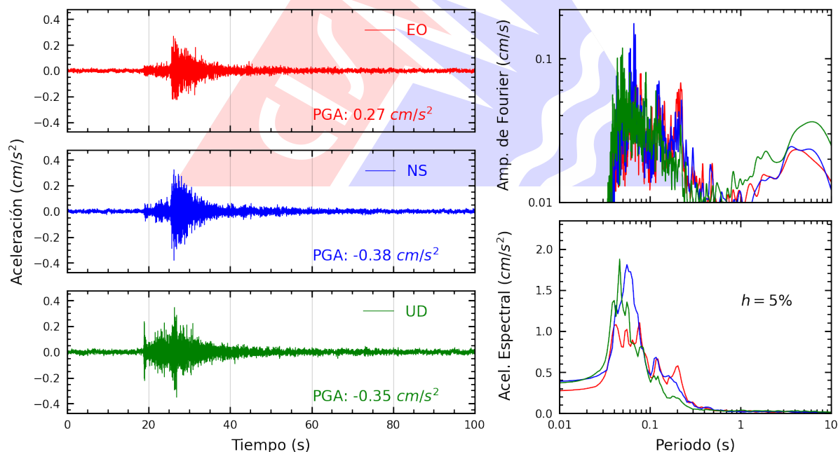
Figura A.28: Registros tiempo-historia, espectros de Fourier y de respuesta en las direcciones EO, NS y vertical de la estación VHAYA. Sismo de Callao, Provincia Constitucional del Callao del 2026-03-24, 21:21:08 (Hora local)
