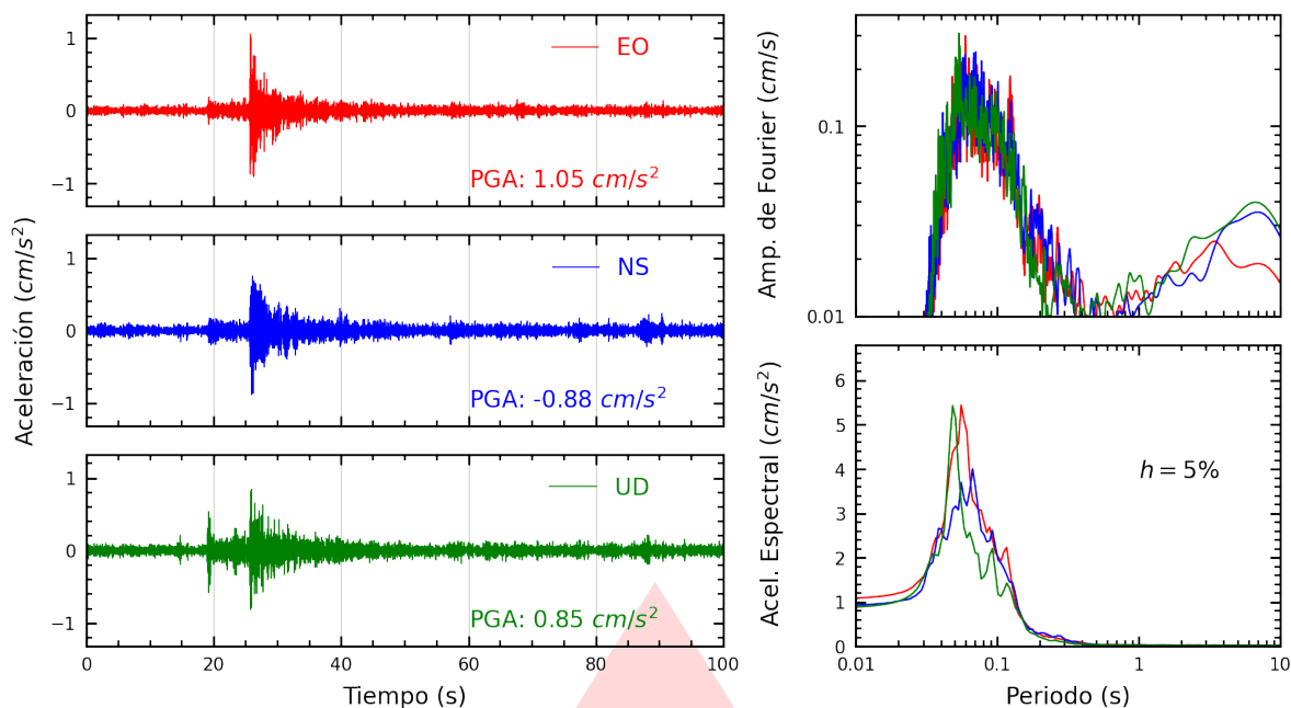
Figura A.11: Registros tiempo-historia, espectros de Fourier y de respuesta en las direcciones EO, NS y vertical de la estación SJLSC. Sismo de Callao, Provincia Constitucional del Callao del 2026-03-24, 21:21:08 (Hora local)
