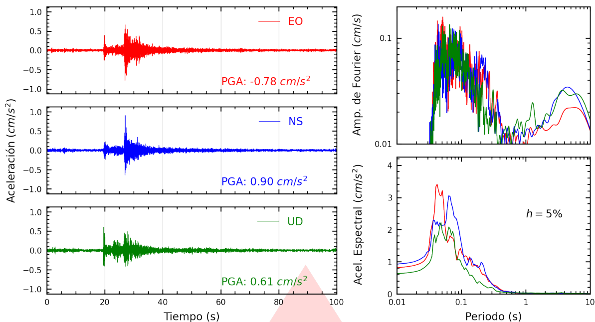
Figura A.17: Registros tiempo-historia, espectros de Fourier y de respuesta en las direcciones EO, NS y vertical de la estación UCVAT. Sismo de Callao, Provincia Constitucional del Callao del 2026-03-24, 21:21:08 (Hora local)
