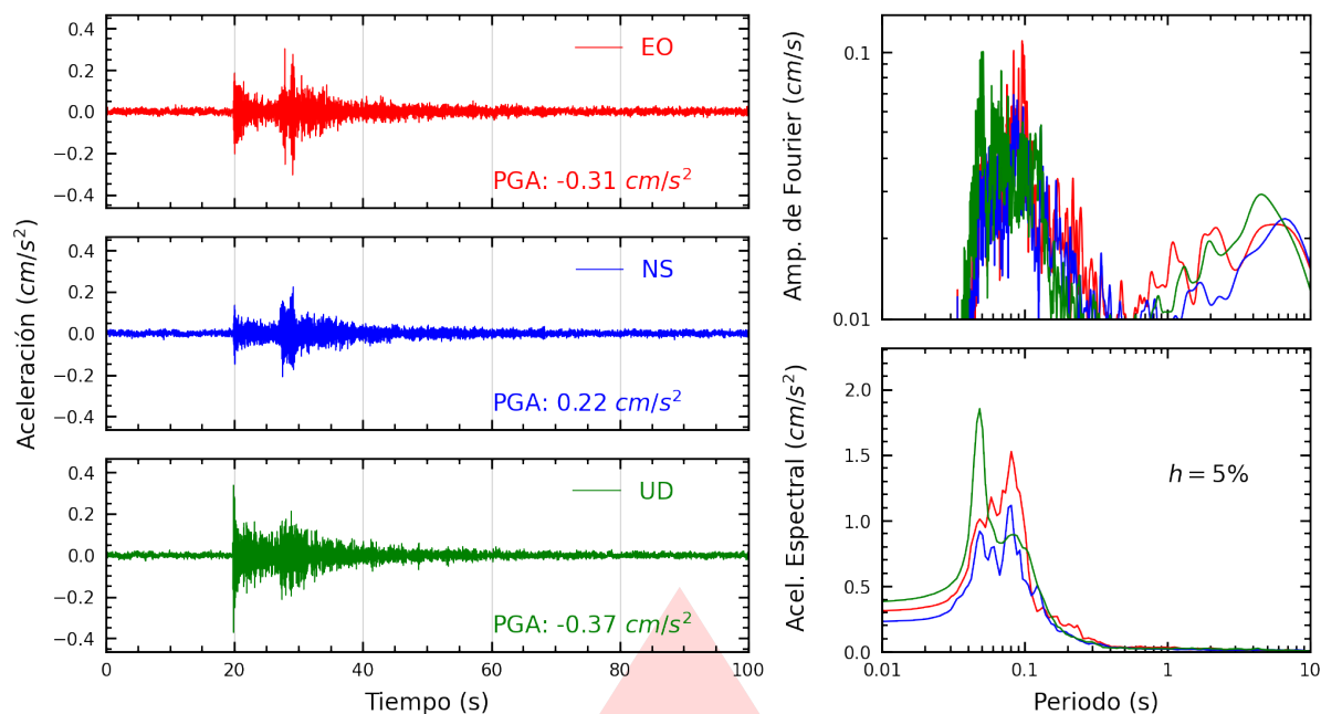
Figura A.29: Registros tiempo-historia, espectros de Fourier y de respuesta en las direcciones EO, NS y vertical de la estación USILP. Sismo de Callao, Provincia Constitucional del Callao del 2026-03-24, 21:21:08 (Hora local)
