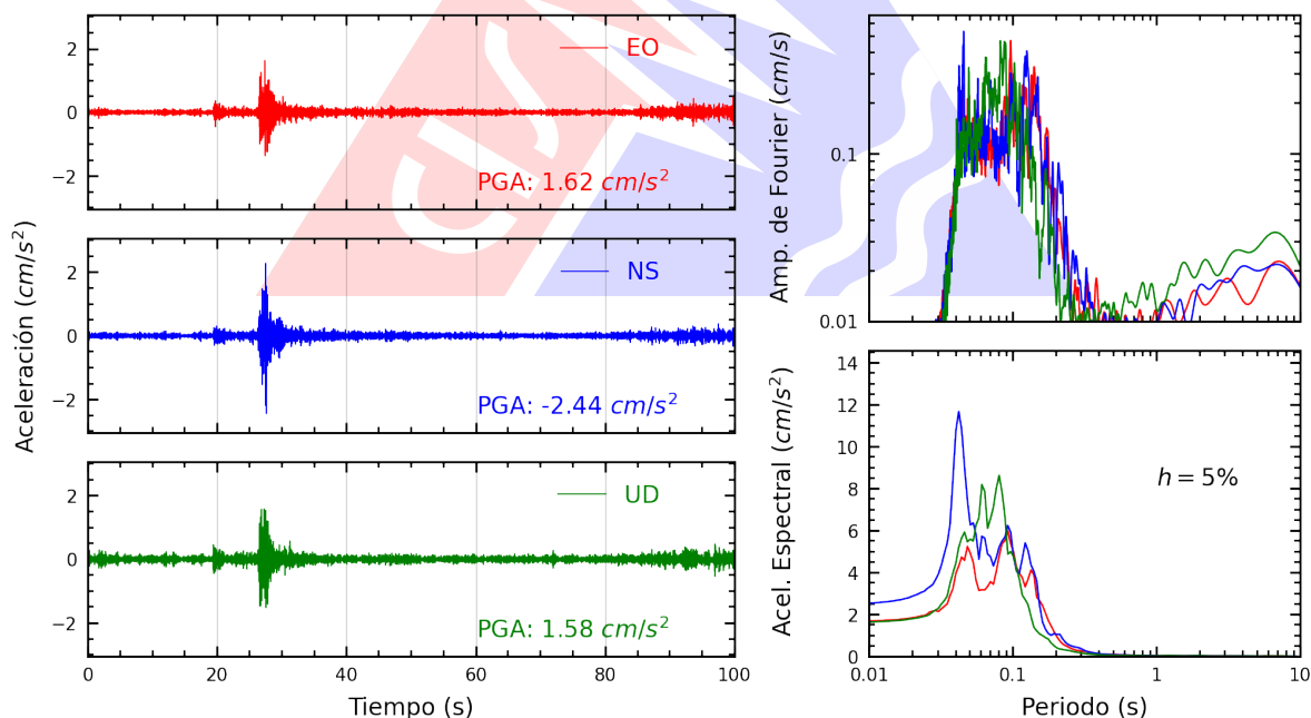
Figura A.2: Registros tiempo-historia, espectros de Fourier y de respuesta en las direcciones EO, NS y vertical de la estación CARAB. Sismo de Callao, Provincia Constitucional del Callao del 2026-03-24, 21:21:08 (Hora local)
