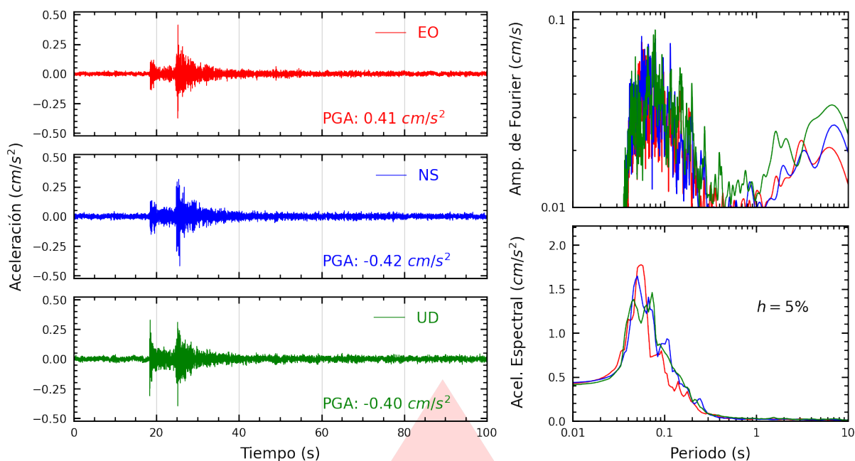
Figura A.27: Registros tiempo-historia, espectros de Fourier y de respuesta en las direcciones EO, NS y vertical de la estación UNFV. Sismo de Callao, Provincia Constitucional del Callao del 2026-03-24, 21:21:08 (Hora local)
