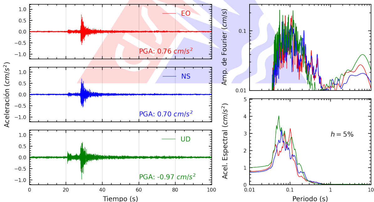
Figura A.14: Registros tiempo-historia, espectros de Fourier y de respuesta en las direcciones EO, NS y vertical de la estación MDPP. Sismo de Callao, Provincia Constitucional del Callao del 2026-03-24, 21:21:08 (Hora local)
