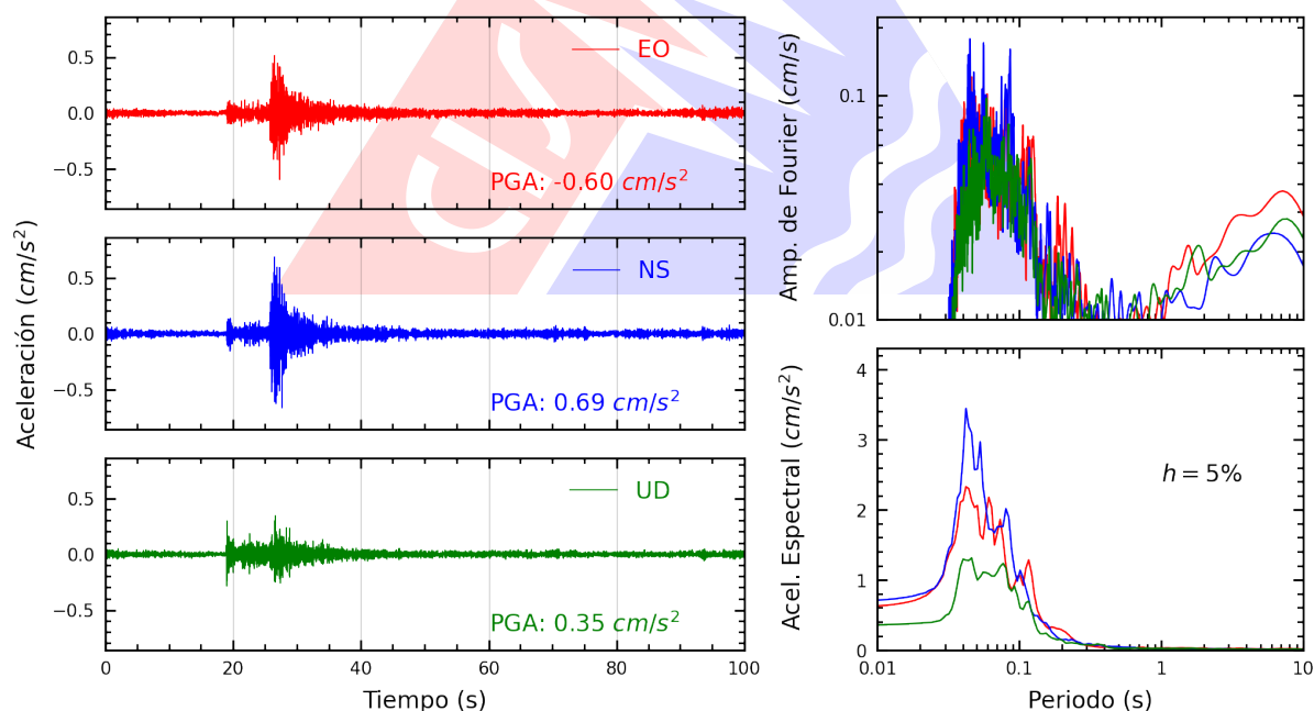
Figura A.22: Registros tiempo-historia, espectros de Fourier y de respuesta en las direcciones EO, NS y vertical de la estación COMAS. Sismo de Callao, Provincia Constitucional del Callao del 2026-03-24, 21:21:08 (Hora local)
