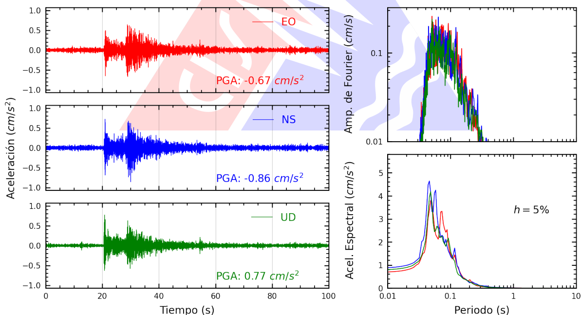
Figura A.18: Registros tiempo-historia, espectros de Fourier y de respuesta en las direcciones EO, NS y vertical de la estación PHERM. Sismo de Callao, Provincia Constitucional del Callao del 2026-03-24, 21:21:08 (Hora local)
