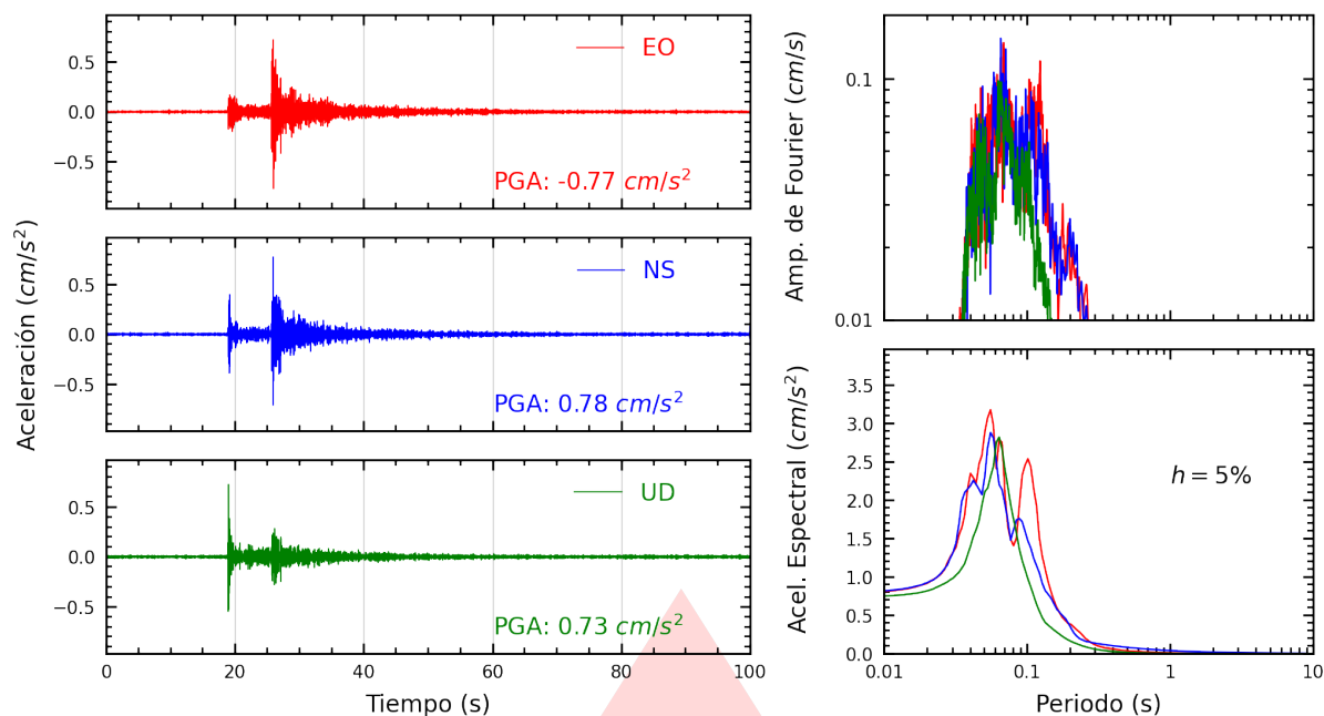
Figura A.19: Registros tiempo-historia, espectros de Fourier y de respuesta en las direcciones EO, NS y vertical de la estación ATARJ. Sismo de Callao, Provincia Constitucional del Callao del 2026-03-24, 21:21:08 (Hora local)
