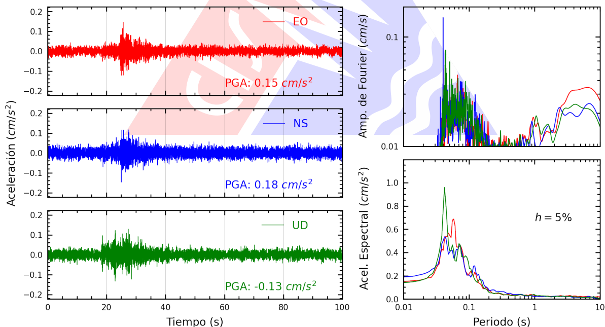
Figura A.32: Registros tiempo-historia, espectros de Fourier y de respuesta en las direcciones EO, NS y vertical de la estación BONDY. Sismo de Callao, Provincia Constitucional del Callao del 2026-03-24, 21:21:08 (Hora local)
