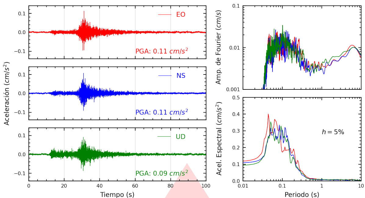
Figura A.33: Registros tiempo-historia, espectros de Fourier y de respuesta en las direcciones EO, NS y vertical de la estación CARAL. Sismo de Callao, Provincia Constitucional del Callao del 2026-03-24, 21:21:08 (Hora local)
