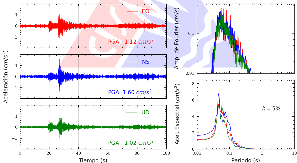
Figura A.6: Registros tiempo-historia, espectros de Fourier y de respuesta en las direcciones EO, NS y vertical de la estación UNTEL. Sismo de Callao, Provincia Constitucional del Callao del 2026-03-24, 21:21:08 (Hora local)
