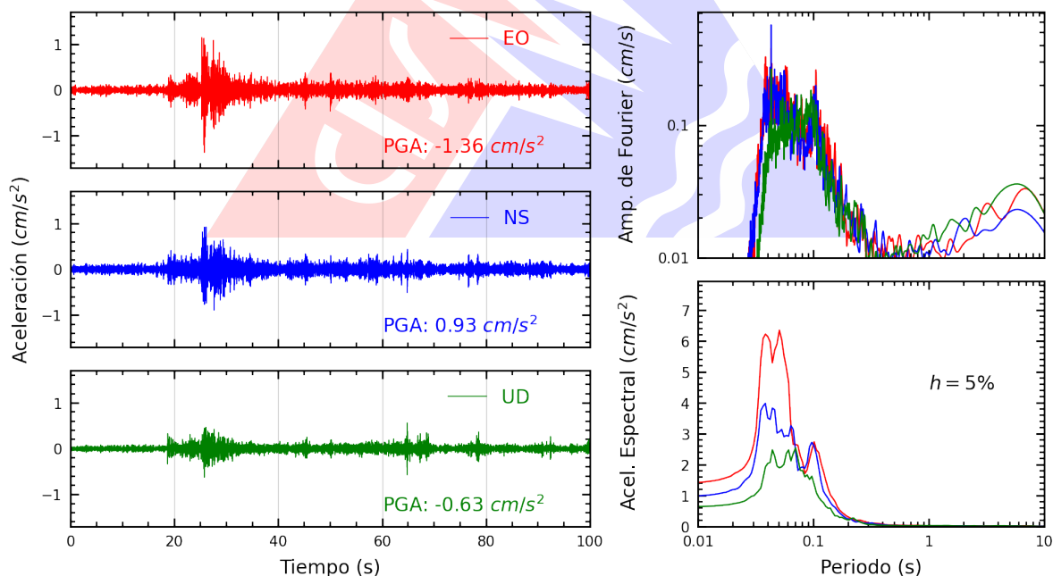
Figura A.8: Registros tiempo-historia, espectros de Fourier y de respuesta en las direcciones EO, NS y vertical de la estación OLIVO. Sismo de Callao, Provincia Constitucional del Callao del 2026-03-24, 21:21:08 (Hora local)
