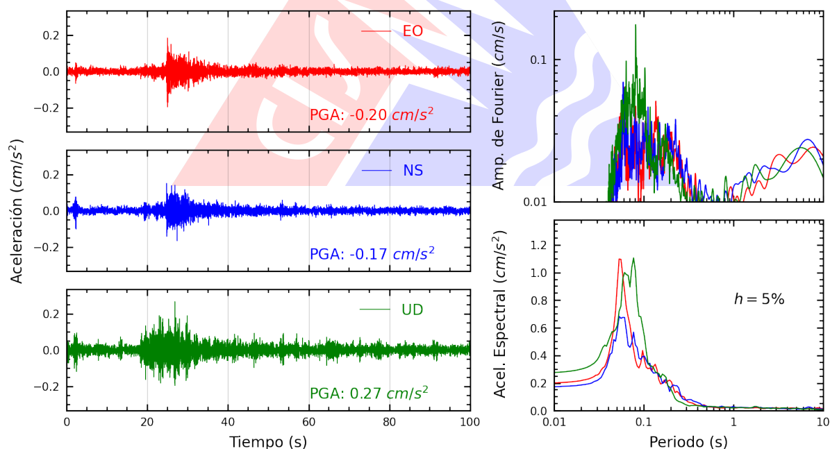
Figura A.30: Registros tiempo-historia, espectros de Fourier y de respuesta en las direcciones EO, NS y vertical de la estación RAMON. Sismo de Callao, Provincia Constitucional del Callao del 2026-03-24, 21:21:08 (Hora local)
