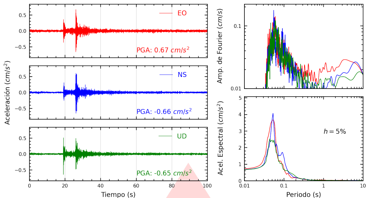
Figura A.23: Registros tiempo-historia, espectros de Fourier y de respuesta en las direcciones EO, NS y vertical de la estación IMCA. Sismo de Callao, Provincia Constitucional del Callao del 2026-03-24, 21:21:08 (Hora local)
