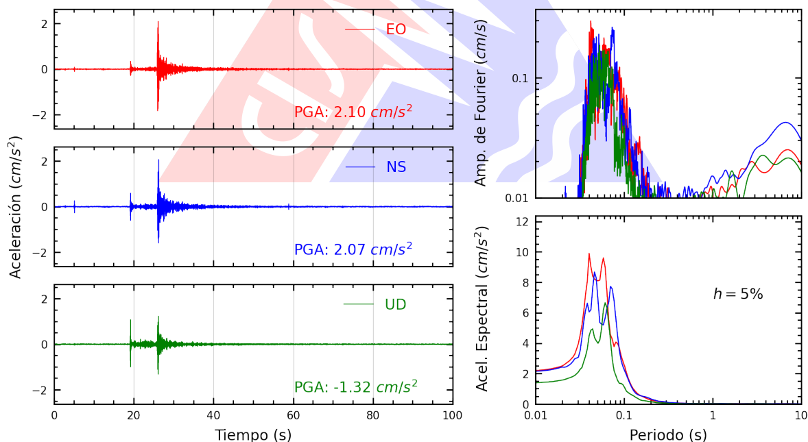
Figura A.4: Registros tiempo-historia, espectros de Fourier y de respuesta en las direcciones EO, NS y vertical de la estación SJLCE. Sismo de Callao, Provincia Constitucional del Callao del 2026-03-24, 21:21:08 (Hora local)
