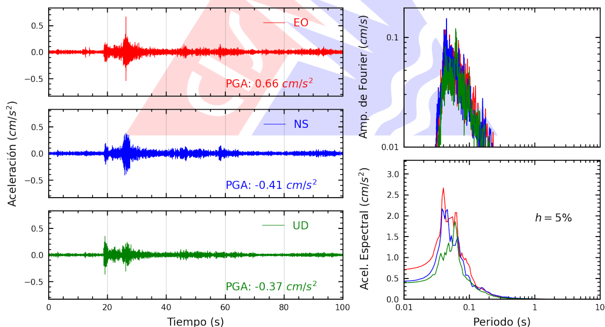
Figura A.24: Registros tiempo-historia, espectros de Fourier y de respuesta en las direcciones EO, NS y vertical de la estación BORJA. Sismo de Callao, Provincia Constitucional del Callao del 2026-03-24, 21:21:08 (Hora local)
