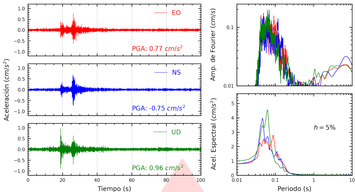
Figura A.15: Registros tiempo-historia, espectros de Fourier y de respuesta en las direcciones EO, NS y vertical de la estación URPE. Sismo de Callao, Provincia Constitucional del Callao del 2026-03-24, 21:21:08 (Hora local)
