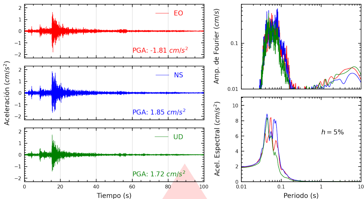
Figura A.5: Registros tiempo-historia, espectros de Fourier y de respuesta en las direcciones EO, NS y vertical de la estación JOSEO. Sismo de Callao, Provincia Constitucional del Callao del 2026-03-24, 21:21:08 (Hora local)
