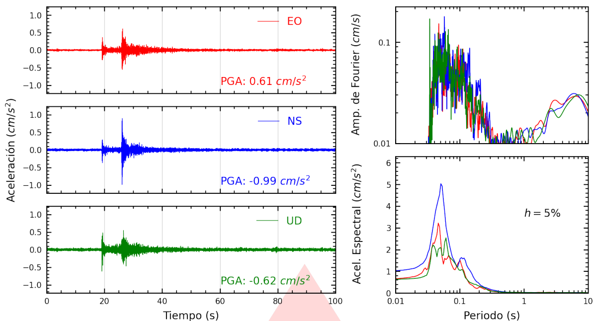
Figura A.13: Registros tiempo-historia, espectros de Fourier y de respuesta en las direcciones EO, NS y vertical de la estación USMP. Sismo de Callao, Provincia Constitucional del Callao del 2026-03-24, 21:21:08 (Hora local)
