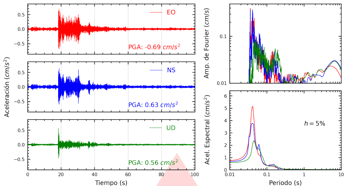
Figura A.21: Registros tiempo-historia, espectros de Fourier y de respuesta en las direcciones EO, NS y vertical de la estación DHNPE. Sismo de Callao, Provincia Constitucional del Callao del 2026-03-24, 21:21:08 (Hora local)
