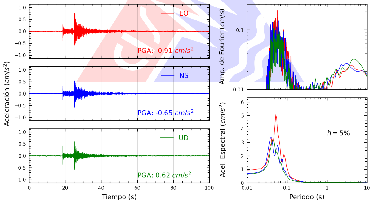
Figura A.16: Registros tiempo-historia, espectros de Fourier y de respuesta en las direcciones EO, NS y vertical de la estación UCSS. Sismo de Callao, Provincia Constitucional del Callao del 2026-03-24, 21:21:08 (Hora local)
