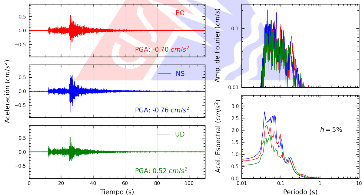
Figura A.20: Registros tiempo-historia, espectros de Fourier y de respuesta en las direcciones EO, NS y vertical de la estación BORJA. Sismo de Huacho, Huaura - Lima del 2026-03-26, 00:32:54 (Hora local)
