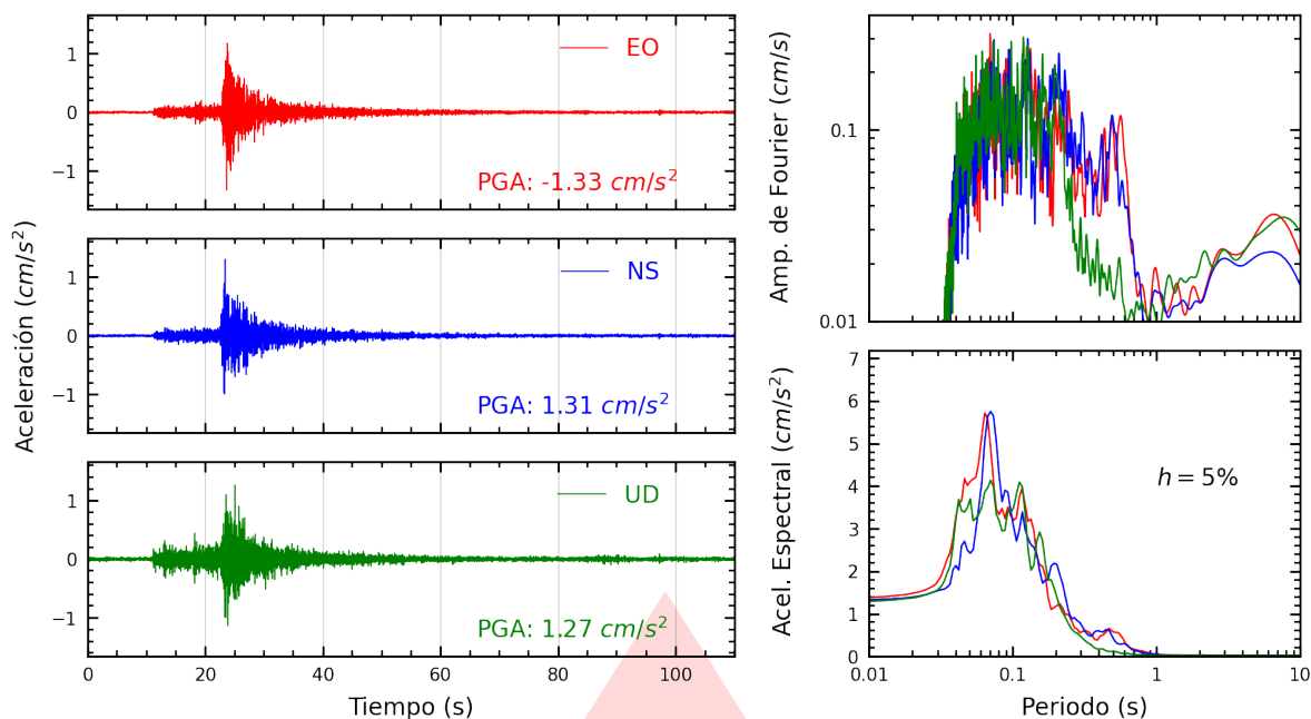
Figura A.9: Registros tiempo-historia, espectros de Fourier y de respuesta en las direcciones EO, NS y vertical de la estación MDPP. Sismo de Huacho, Huaura - Lima del 2026-03-26, 00:32:54 (Hora local)
