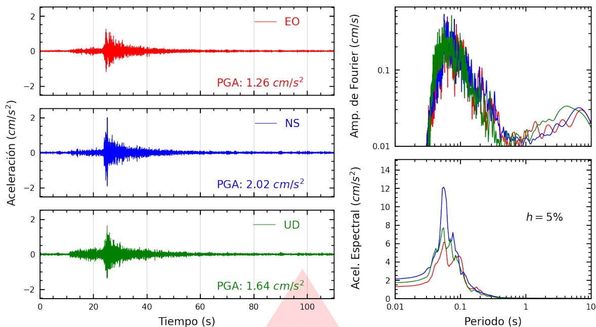
Figura A.5: Registros tiempo-historia, espectros de Fourier y de respuesta en las direcciones EO, NS y vertical de la estación SJLSC. Sismo de Huacho, Huaura - Lima del 2026-03-26, 00:32:54 (Hora local)
