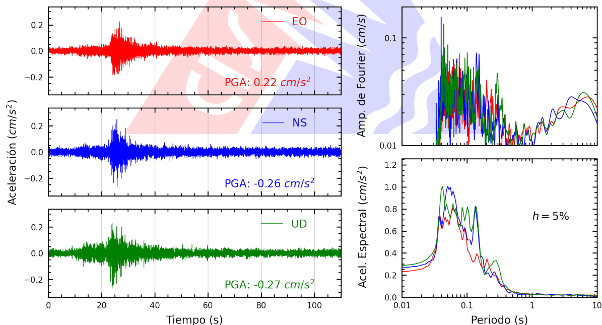
Figura A.32: Registros tiempo-historia, espectros de Fourier y de respuesta en las direcciones EO, NS y vertical de la estación BONDY. Sismo de Huacho, Huaura - Lima del 2026-03-26, 00:32:54 (Hora local)
