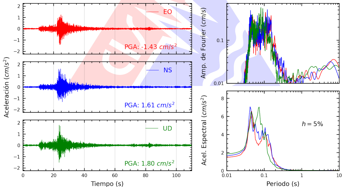
Figura A.6: Registros tiempo-historia, espectros de Fourier y de respuesta en las direcciones EO, NS y vertical de la estación CARAB. Sismo de Huacho, Huaura - Lima del 2026-03-26, 00:32:54 (Hora local)
