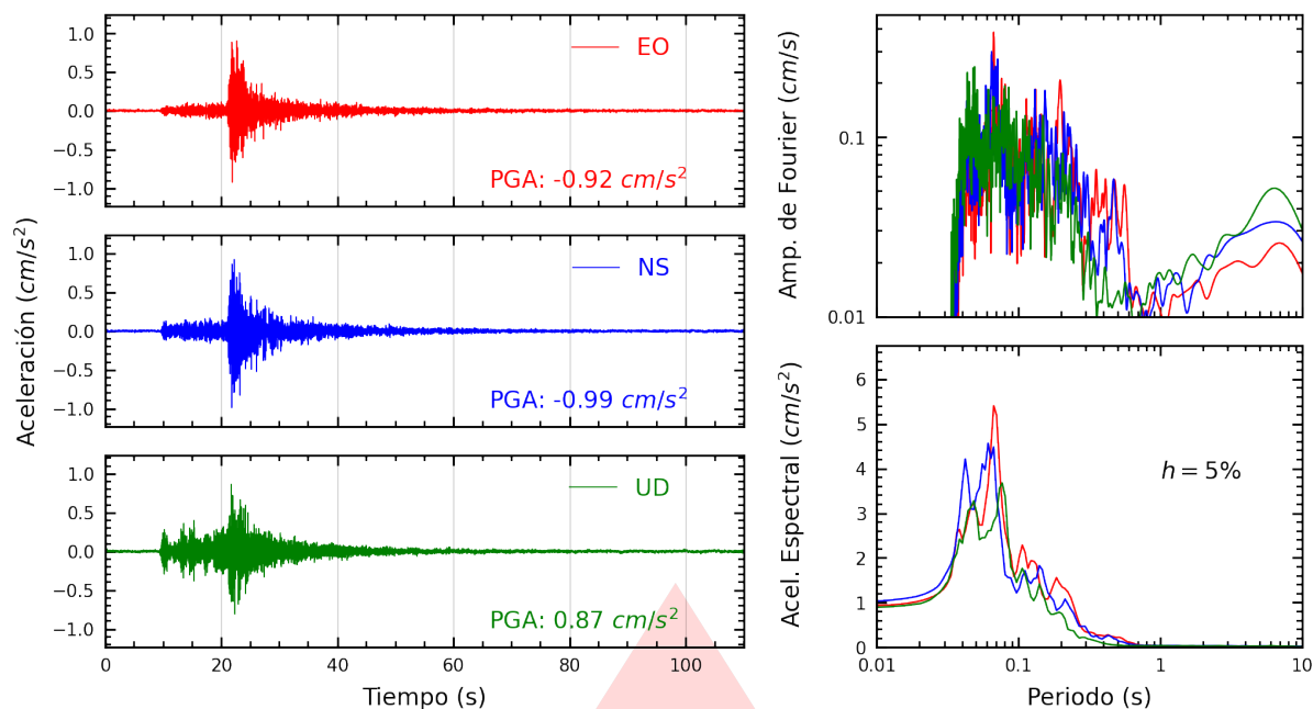
Figura A.15: Registros tiempo-historia, espectros de Fourier y de respuesta en las direcciones EO, NS y vertical de la estación VHAYA. Sismo de Huacho, Huaura - Lima del 2026-03-26, 00:32:54 (Hora local)
