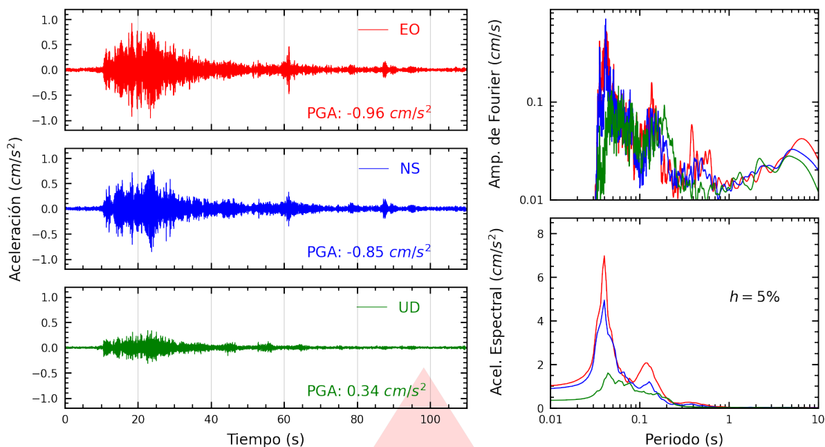
Figura A.17: Registros tiempo-historia, espectros de Fourier y de respuesta en las direcciones EO, NS y vertical de la estación DHNPE. Sismo de Huacho, Huaura - Lima del 2026-03-26, 00:32:54 (Hora local)
