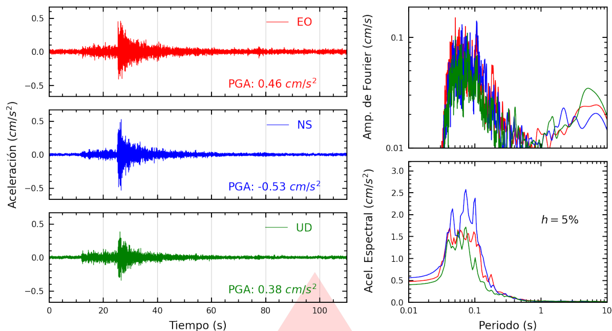
Figura A.27: Registros tiempo-historia, espectros de Fourier y de respuesta en las direcciones EO, NS y vertical de la estación INICT. Sismo de Huacho, Huaura - Lima del 2026-03-26, 00:32:54 (Hora local)
