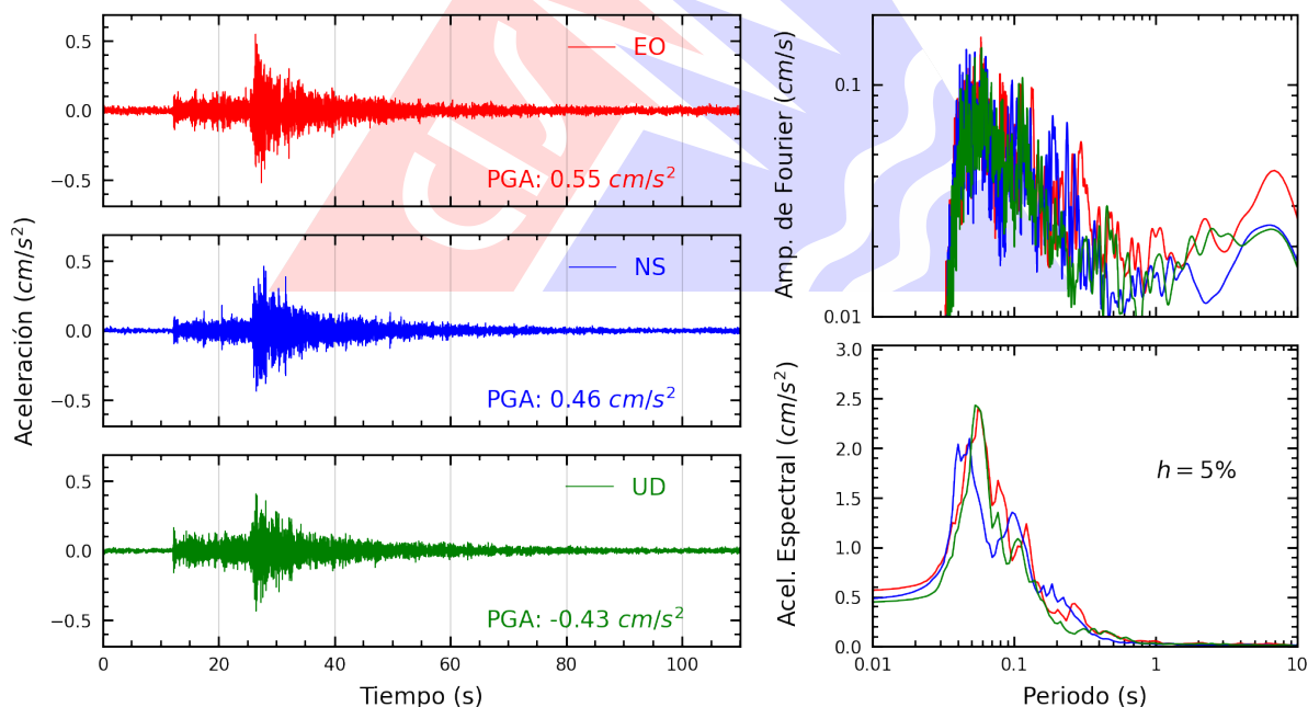
Figura A.26: Registros tiempo-historia, espectros de Fourier y de respuesta en las direcciones EO, NS y vertical de la estación IMCA. Sismo de Huacho, Huaura - Lima del 2026-03-26, 00:32:54 (Hora local)
