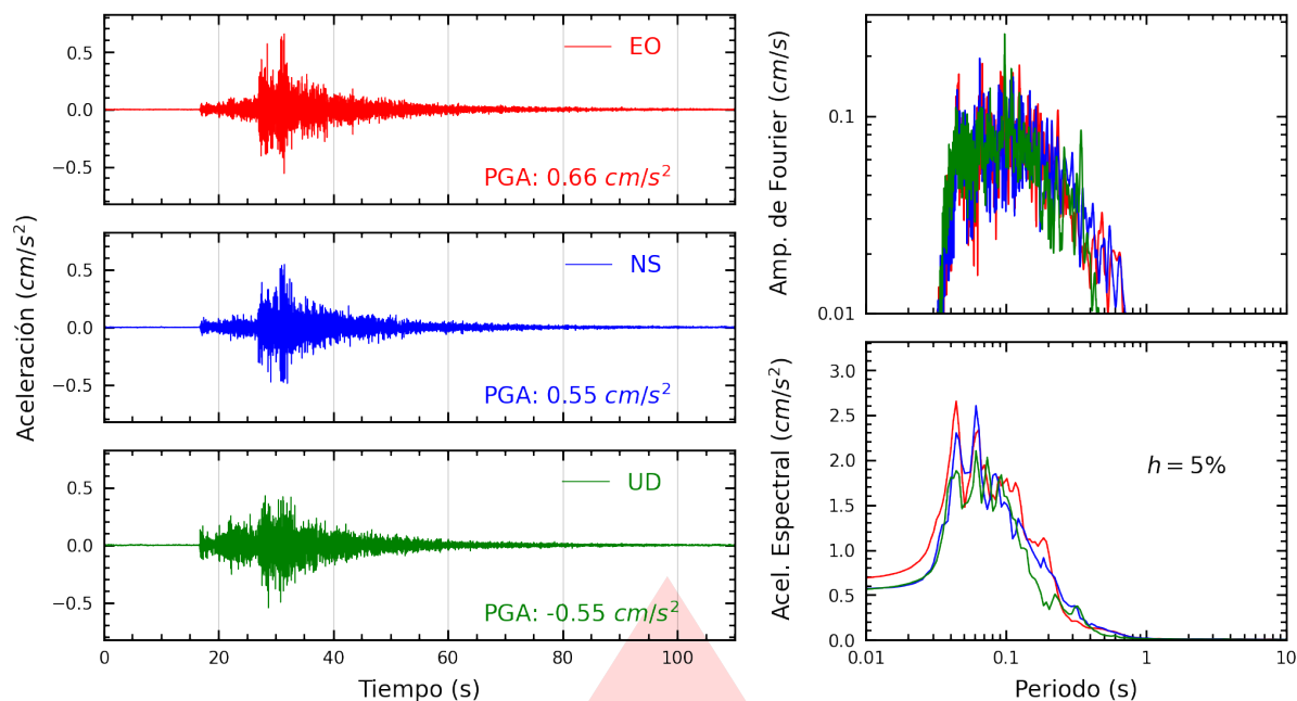
Figura A.21: Registros tiempo-historia, espectros de Fourier y de respuesta en las direcciones EO, NS y vertical de la estación CARAL. Sismo de Huacho, Huaura - Lima del 2026-03-26, 00:32:54 (Hora local)
