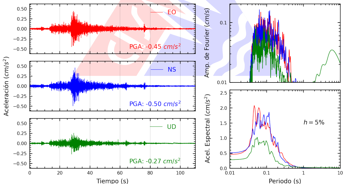
Figura A.28: Registros tiempo-historia, espectros de Fourier y de respuesta en las direcciones EO, NS y vertical de la estación BRISA. Sismo de Huacho, Huaura - Lima del 2026-03-26, 00:32:54 (Hora local)
