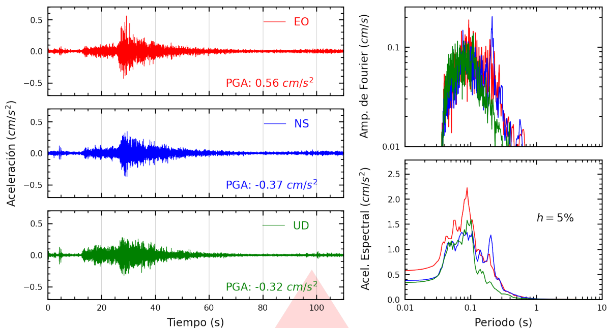
Figura A.25: Registros tiempo-historia, espectros de Fourier y de respuesta en las direcciones EO, NS y vertical de la estación SCCHO. Sismo de Huacho, Huaura - Lima del 2026-03-26, 00:32:54 (Hora local)
