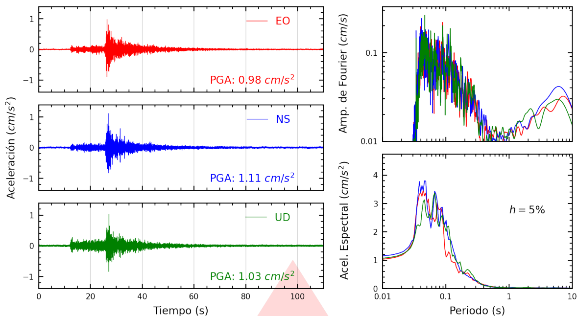
Figura A.13: Registros tiempo-historia, espectros de Fourier y de respuesta en las direcciones EO, NS y vertical de la estación USMP. Sismo de Huacho, Huaura - Lima del 2026-03-26, 00:32:54 (Hora local)
