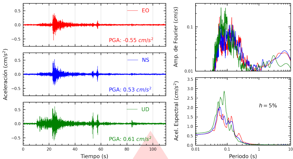
Figura A.23: Registros tiempo-historia, espectros de Fourier y de respuesta en las direcciones EO, NS y vertical de la estación RAMON. Sismo de Huacho, Huaura - Lima del 2026-03-26, 00:32:54 (Hora local)
