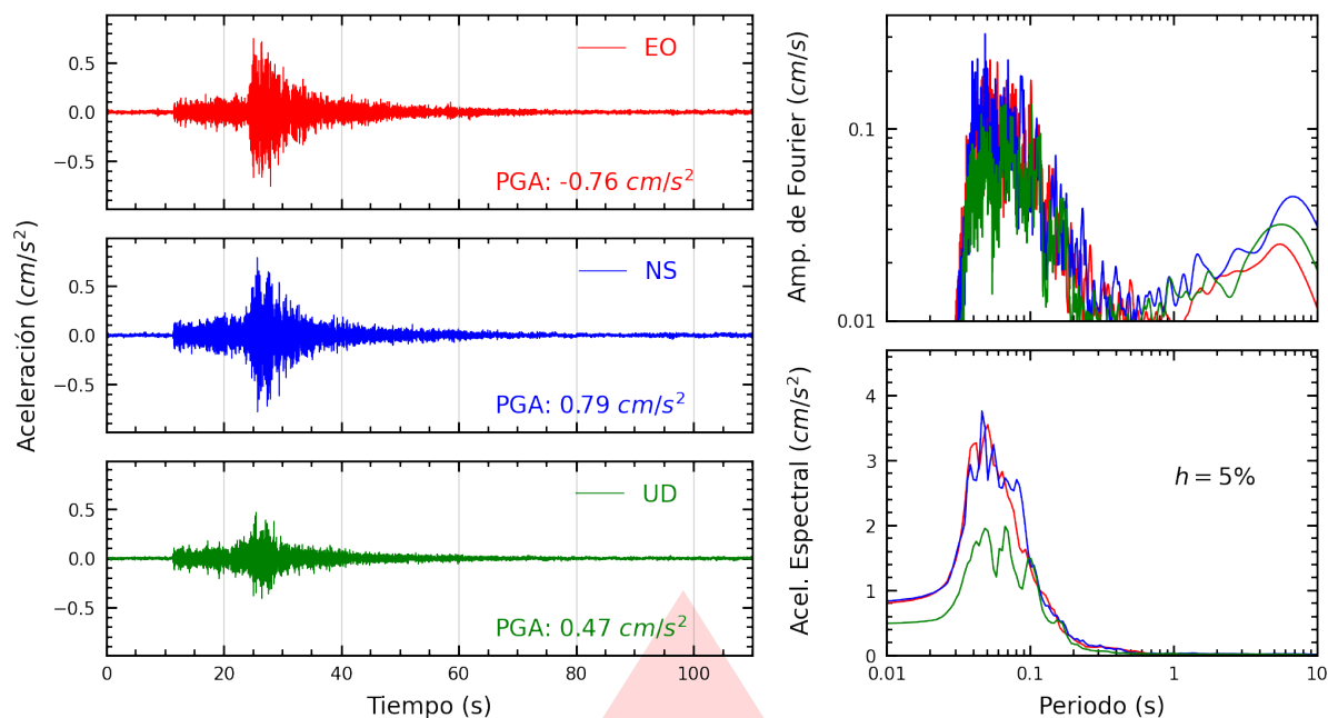
Figura A.19: Registros tiempo-historia, espectros de Fourier y de respuesta en las direcciones EO, NS y vertical de la estación CEPRE. Sismo de Huacho, Huaura - Lima del 2026-03-26, 00:32:54 (Hora local)
