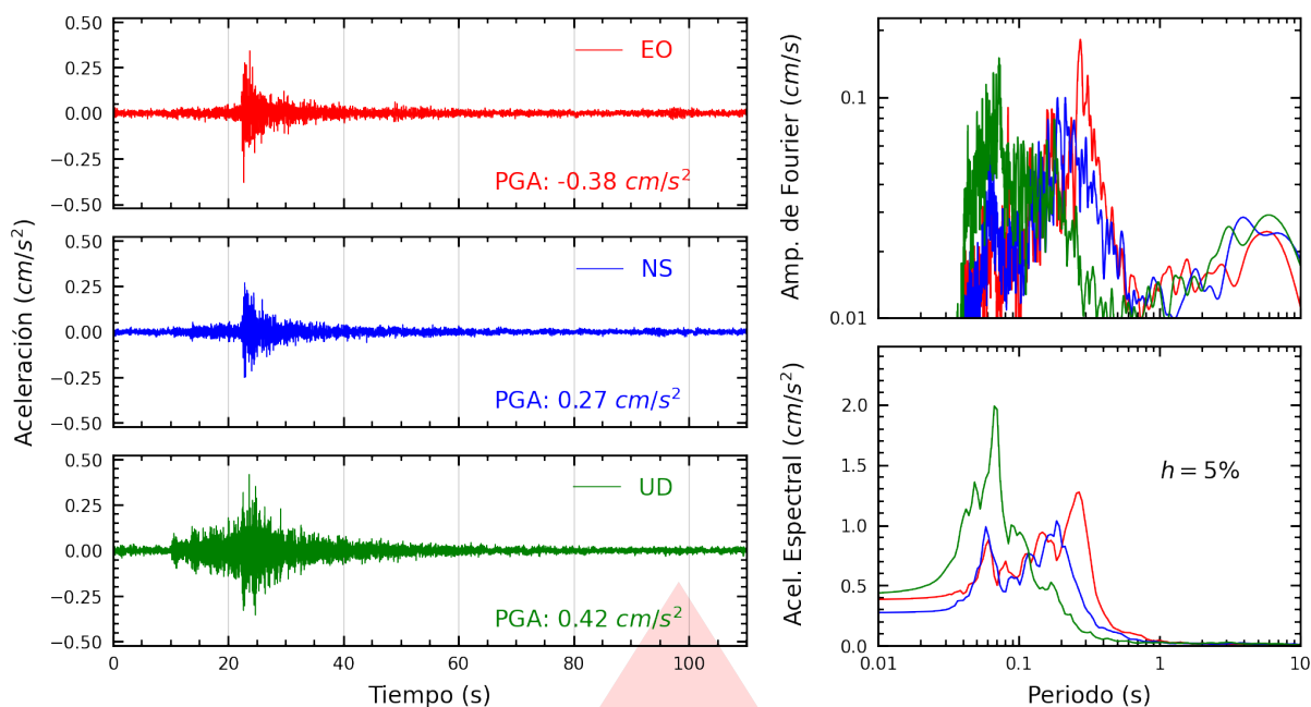
Figura A.29: Registros tiempo-historia, espectros de Fourier y de respuesta en las direcciones EO, NS y vertical de la estación ACAPU. Sismo de Huacho, Huaura - Lima del 2026-03-26, 00:32:54 (Hora local)
