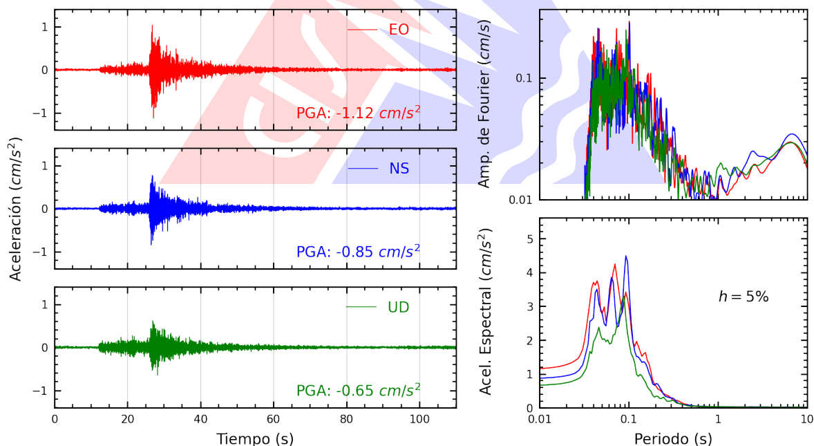
Figura A.12: Registros tiempo-historia, espectros de Fourier y de respuesta en las direcciones EO, NS y vertical de la estación UCVAT. Sismo de Huacho, Huaura - Lima del 2026-03-26, 00:32:54 (Hora local)
