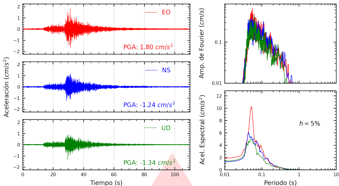
Figura A.7: Registros tiempo-historia, espectros de Fourier y de respuesta en las direcciones EO, NS y vertical de la estación UNTEL. Sismo de Huacho, Huaura - Lima del 2026-03-26, 00:32:54 (Hora local)
