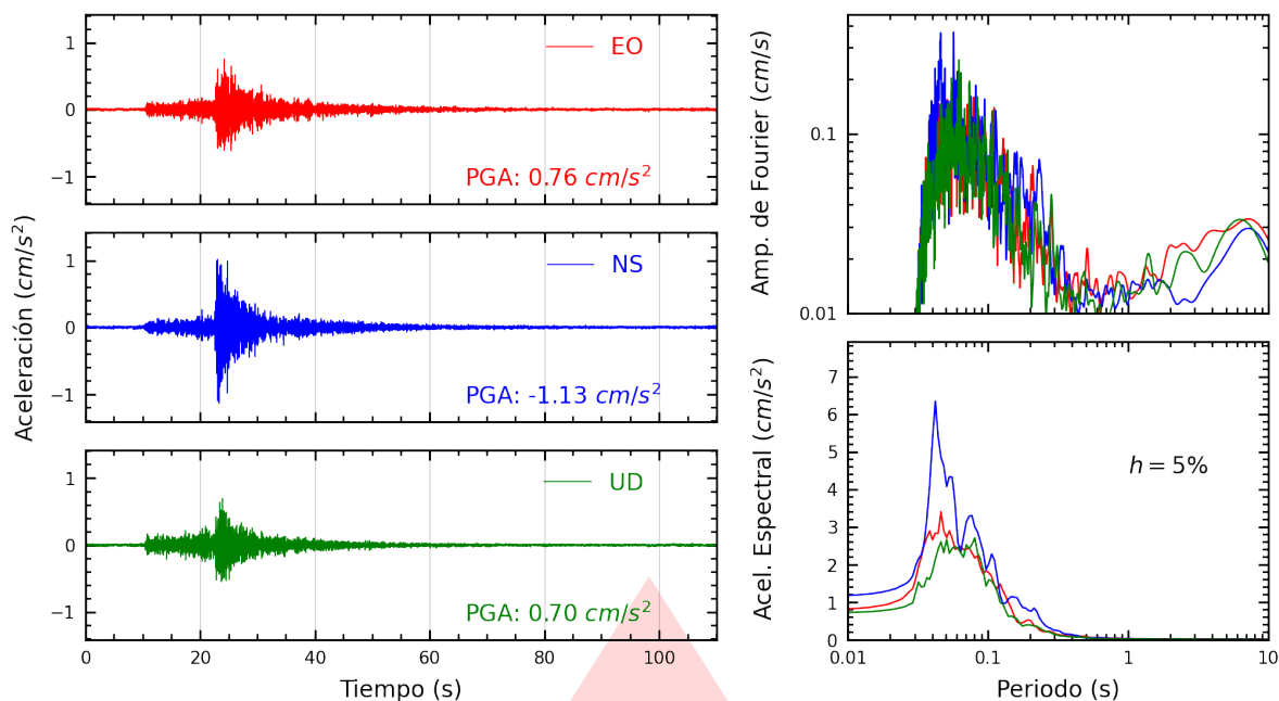
Figura A.11: Registros tiempo-historia, espectros de Fourier y de respuesta en las direcciones EO, NS y vertical de la estación COMAS. Sismo de Huacho, Huaura - Lima del 2026-03-26, 00:32:54 (Hora local)
