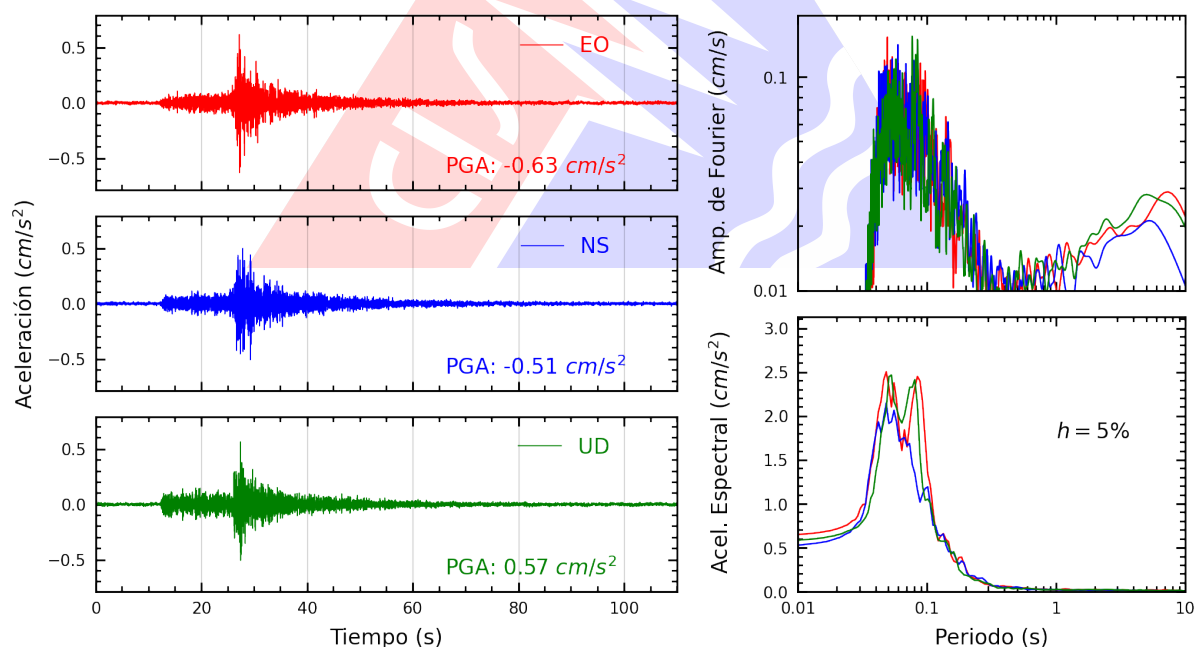
Figura A.22: Registros tiempo-historia, espectros de Fourier y de respuesta en las direcciones EO, NS y vertical de la estación SERVI. Sismo de Huacho, Huaura - Lima del 2026-03-26, 00:32:54 (Hora local)
