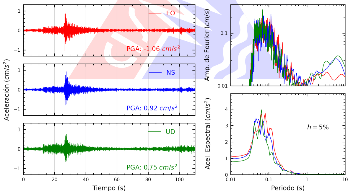
Figura A.14: Registros tiempo-historia, espectros de Fourier y de respuesta en las direcciones EO, NS y vertical de la estación URPE. Sismo de Huacho, Huaura - Lima del 2026-03-26, 00:32:54 (Hora local)
