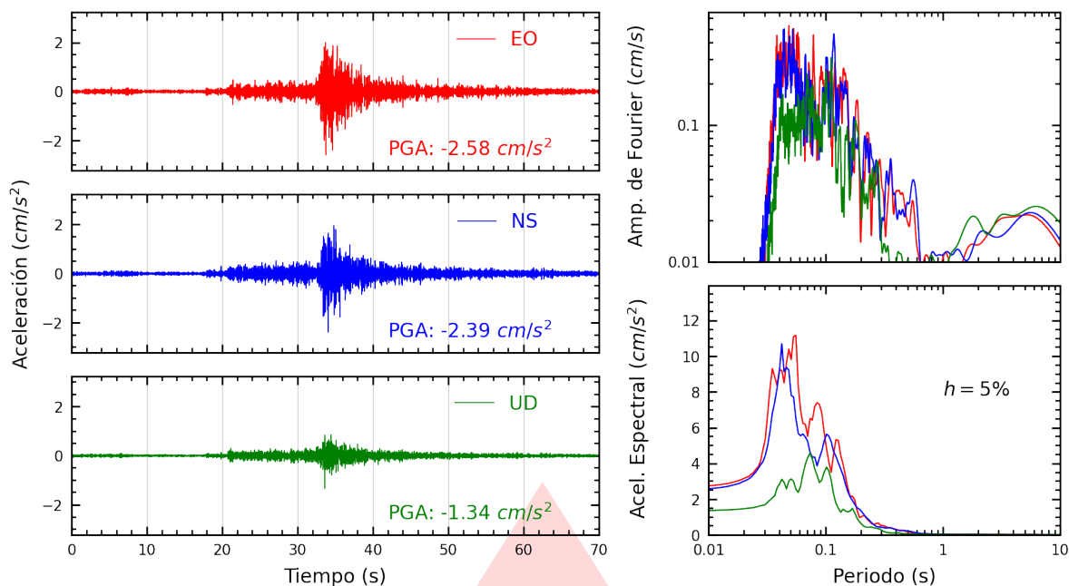
Figura A.3: Registros tiempo-historia, espectros de Fourier y de respuesta en las direcciones EO, NS y vertical de la estación OLIVO. Sismo de Huacho, Huaura - Lima del 2026-03-26, 00:32:54 (Hora local)
