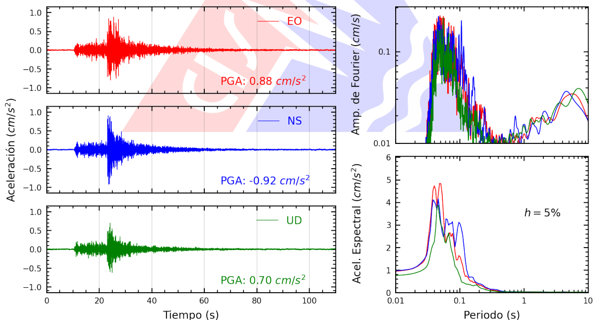
Figura A.18: Registros tiempo-historia, espectros de Fourier y de respuesta en las direcciones EO, NS y vertical de la estación UCSS. Sismo de Huacho, Huaura - Lima del 2026-03-26, 00:32:54 (Hora local)
