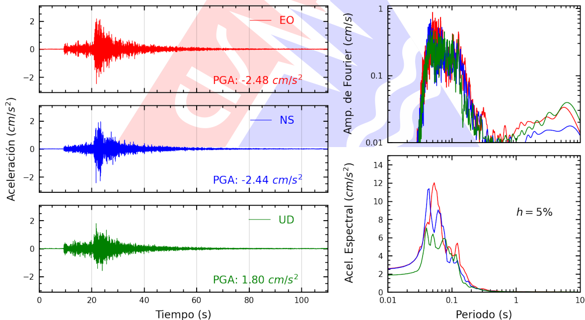
Figura A.4: Registros tiempo-historia, espectros de Fourier y de respuesta en las direcciones EO, NS y vertical de la estación AMORE. Sismo de Huacho, Huaura - Lima del 2026-03-26, 00:32:54 (Hora local)
