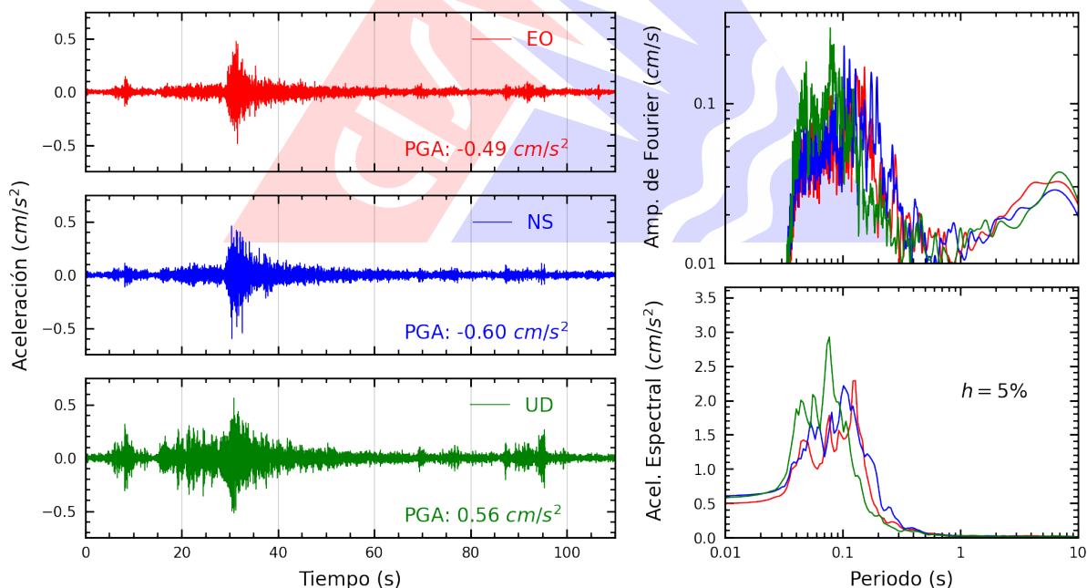
Figura A.24: Registros tiempo-historia, espectros de Fourier y de respuesta en las direcciones EO, NS y vertical de la estación SOCHO. Sismo de Huacho, Huaura - Lima del 2026-03-26, 00:32:54 (Hora local)
