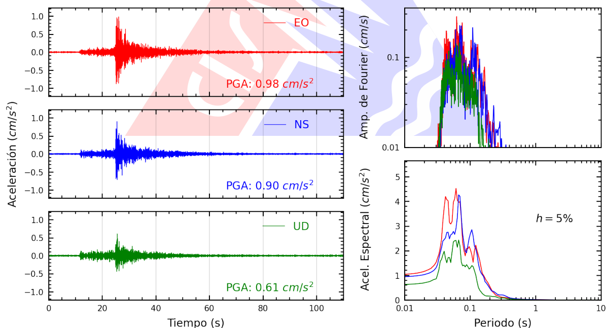
Figura A.16: Registros tiempo-historia, espectros de Fourier y de respuesta en las direcciones EO, NS y vertical de la estación ATARJ. Sismo de Huacho, Huaura - Lima del 2026-03-26, 00:32:54 (Hora local)
