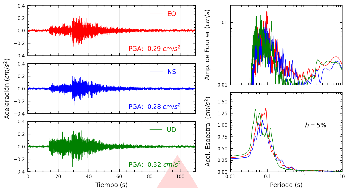
Figura A.31: Registros tiempo-historia, espectros de Fourier y de respuesta en las direcciones EO, NS y vertical de la estación USILP. Sismo de Huacho, Huaura - Lima del 2026-03-26, 00:32:54 (Hora local)
