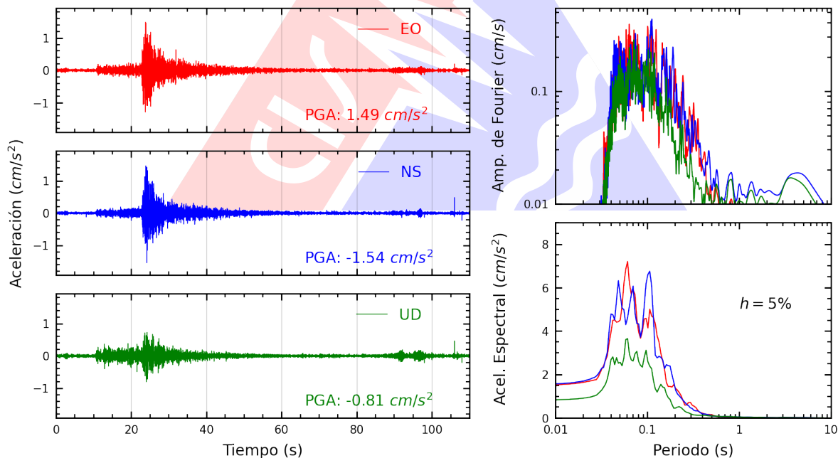
Figura A.8: Registros tiempo-historia, espectros de Fourier y de respuesta en las direcciones EO, NS y vertical de la estación SCOLI. Sismo de Huacho, Huaura - Lima del 2026-03-26, 00:32:54 (Hora local)
