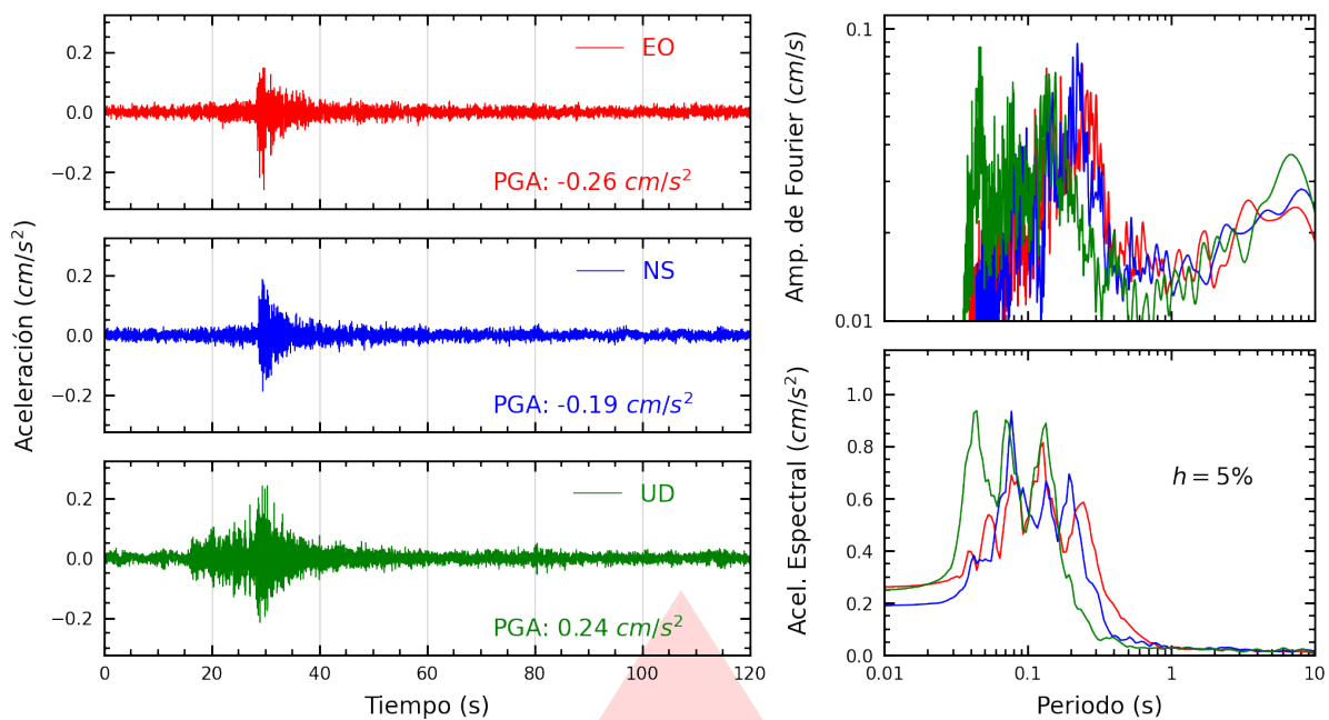
Figura A.33: Registros tiempo-historia, espectros de Fourier y de respuesta en las direcciones EO, NS y vertical de la estación DSML. Sismo de Huacho, Huaura - Lima del 2026-03-26, 00:32:54 (Hora local)
