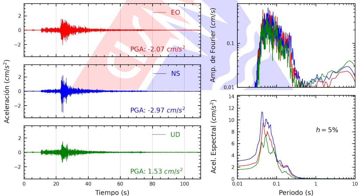
Figura A.2: Registros tiempo-historia, espectros de Fourier y de respuesta en las direcciones EO, NS y vertical de la estación INDEP. Sismo de Huacho, Huaura - Lima del 2026-03-26, 00:32:54 (Hora local)
