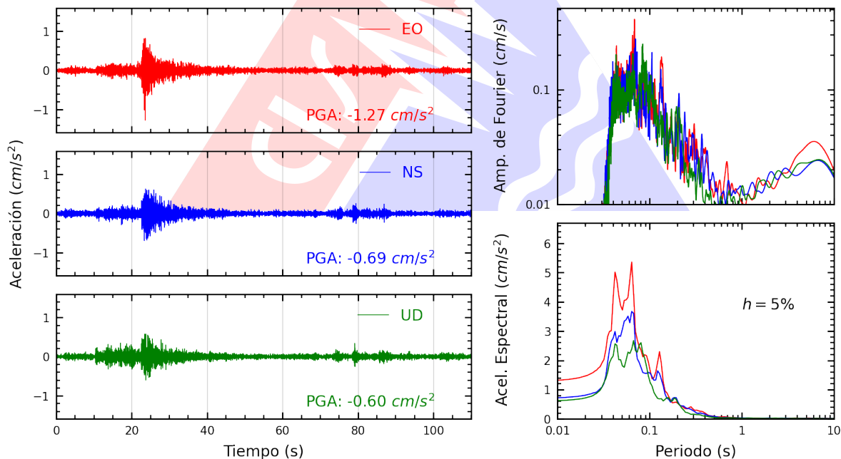
Figura A.10: Registros tiempo-historia, espectros de Fourier y de respuesta en las direcciones EO, NS y vertical de la estación MADRE. Sismo de Huacho, Huaura - Lima del 2026-03-26, 00:32:54 (Hora local)
