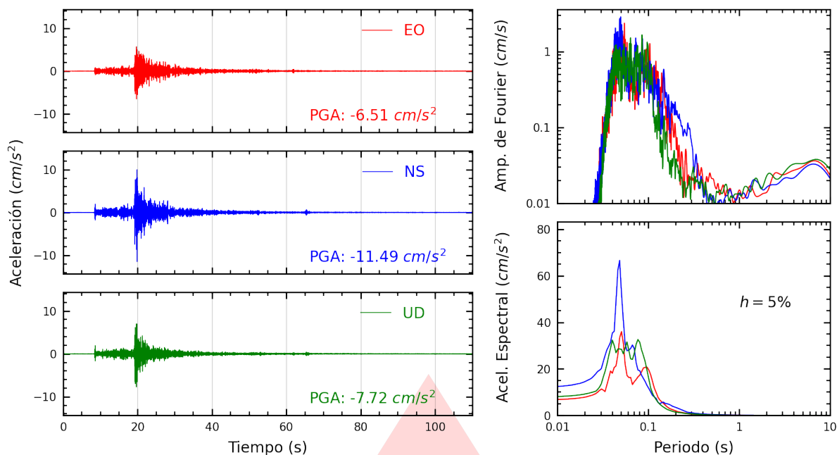
Figura A.1: Registros tiempo-historia, espectros de Fourier y de respuesta en las direcciones EO, NS y vertical de la estación SROSA. Sismo de Huacho, Huaura - Lima del 2026-03-26, 00:32:54 (Hora local)
