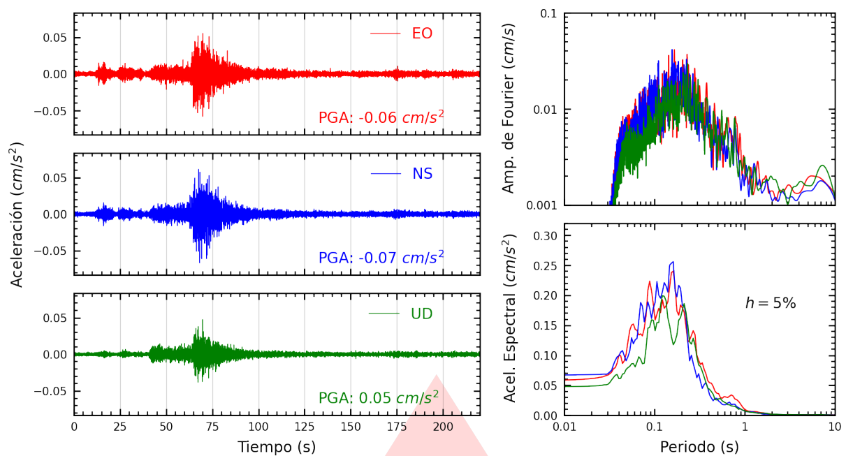
Figura A.1: Registros tiempo-historia, espectros de Fourier y de respuesta en las direcciones EO, NS y vertical de la estación UNSA2. Sismo de Atico, Caravelí - Arequipa del 2026-03-27, 10:41:36 (Hora local)
