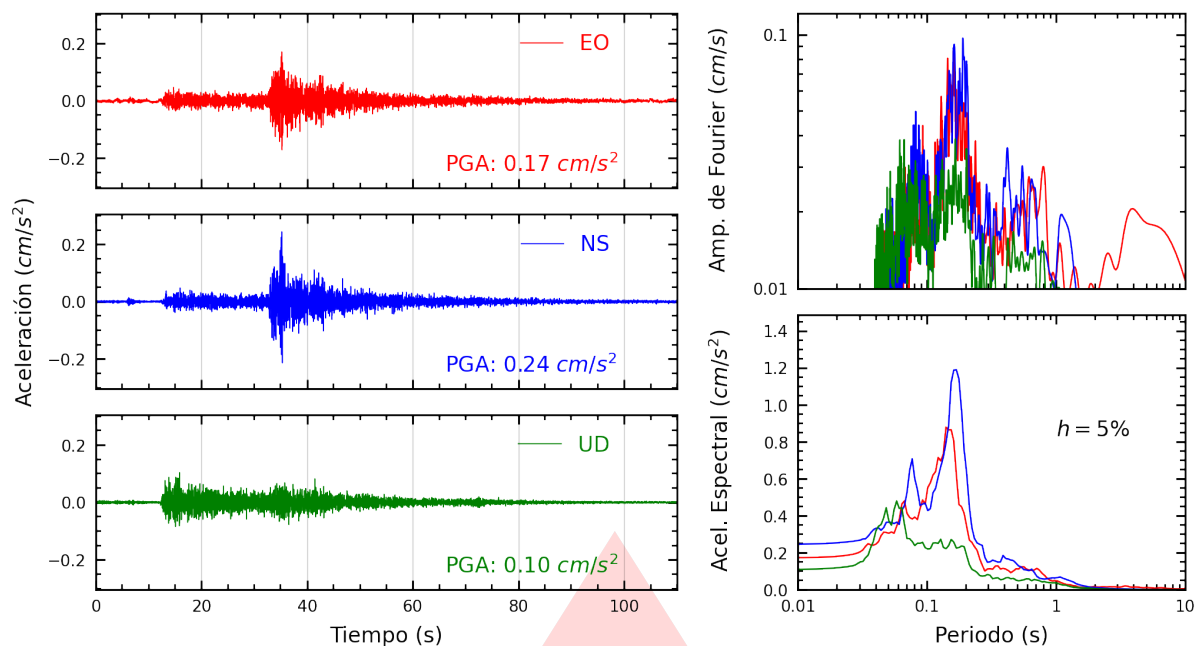
Figura A.5: Registros tiempo-historia, espectros de Fourier y de respuesta en las direcciones EO, NS y vertical de la estación SCCHI. Sismo de Jaén, Jaén - Cajamarca del 2026-03-28, 02:30:44 (Hora local)
