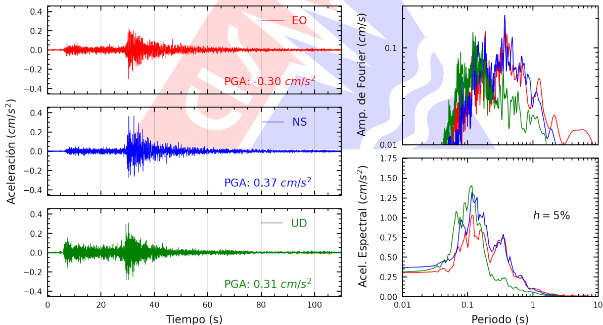
Figura A.4: Registros tiempo-historia, espectros de Fourier y de respuesta en las direcciones EO, NS y vertical de la estación SCPIU. Sismo de Jaén, Jaén - Cajamarca del 2026-03-28, 02:30:44 (Hora local)
