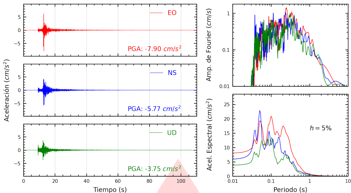
Figura A.1: Registros tiempo-historia, espectros de Fourier y de respuesta en las direcciones EO, NS y vertical de la estación UNJ. Sismo de Jaén, Jaén - Cajamarca del 2026-03-28, 02:30:44 (Hora local)
