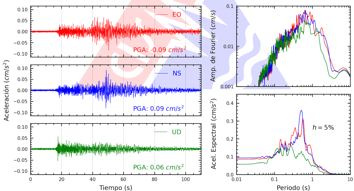
Figura A.6: Registros tiempo-historia, espectros de Fourier y de respuesta en las direcciones EO, NS y vertical de la estación UNC. Sismo de Jaén, Jaén - Cajamarca del 2026-03-28, 02:30:44 (Hora local)
