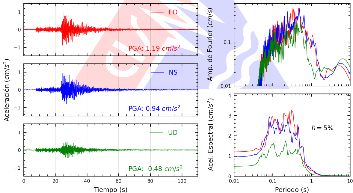
Figura A.2: Registros tiempo-historia, espectros de Fourier y de respuesta en las direcciones EO, NS y vertical de la estación UNTRM. Sismo de Jaén, Jaén - Cajamarca del 2026-03-28, 02:30:44 (Hora local)
