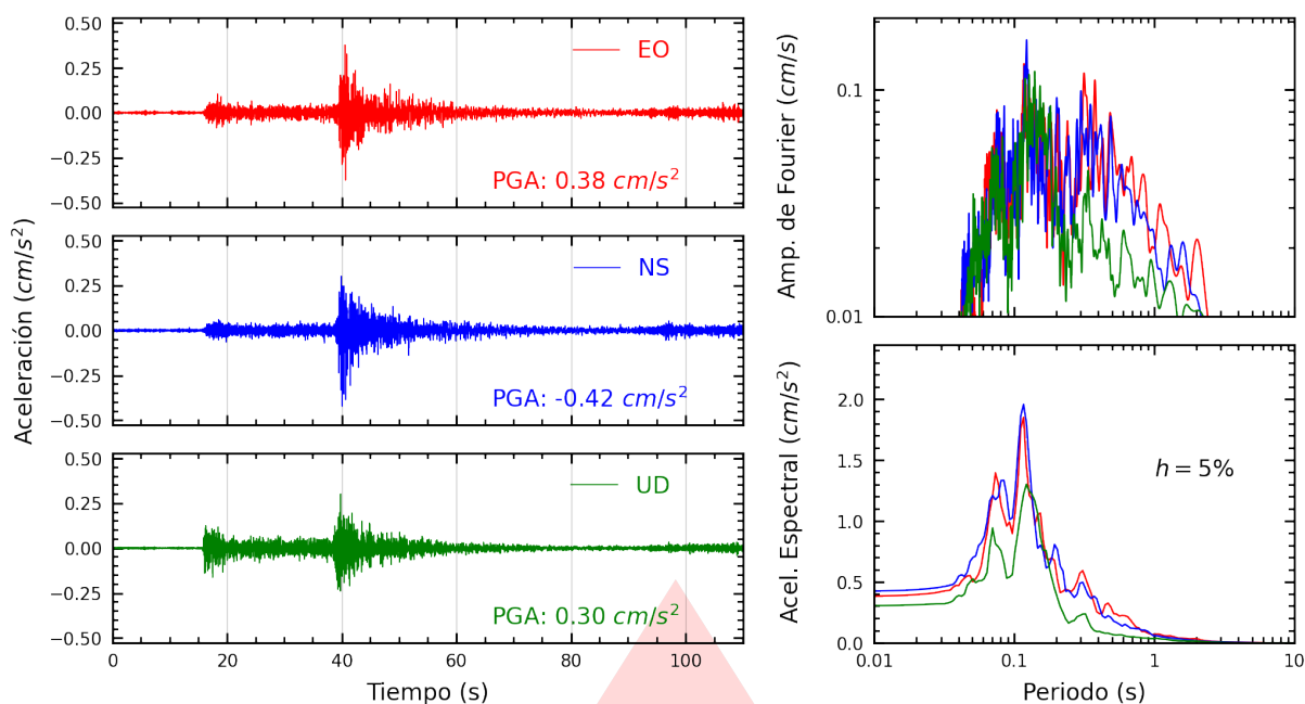
Figura A.3: Registros tiempo-historia, espectros de Fourier y de respuesta en las direcciones EO, NS y vertical de la estación UPAOP. Sismo de Jaén, Jaén - Cajamarca del 2026-03-28, 02:30:44 (Hora local)
