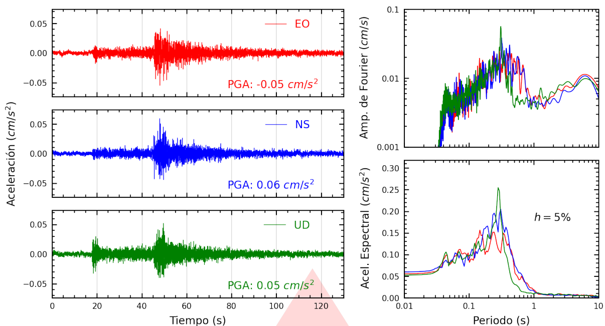
Figura A.3: Registros tiempo-historia, espectros de Fourier y de respuesta en las direcciones EO, NS y vertical de la estación CARAL. Sismo de Tingo María, Leoncio Prado - Huánuco del 2026-03-28, 23:05:11 (Hora local)
