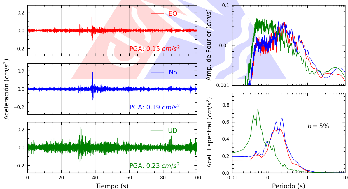
Figura A.2: Registros tiempo-historia, espectros de Fourier y de respuesta en las direcciones EO, NS y vertical de la estación SCPUC. Sismo de Tingo María, Leoncio Prado - Huánuco del 2026-03-28, 23:05:11 (Hora local)
