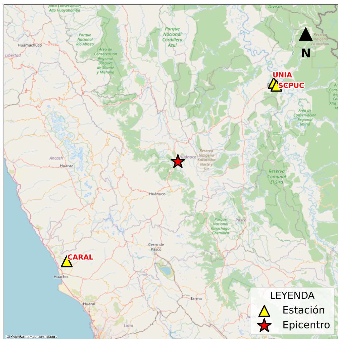
Figura 2: Mapa de ubicación de la(s) estación(es) acelerográfica(s) correspondiente(s) al Sismo de Tingo María, Leoncio Prado - Huánuco del 28 de marzo de 2026 a las 23:05:11 (hora local)
