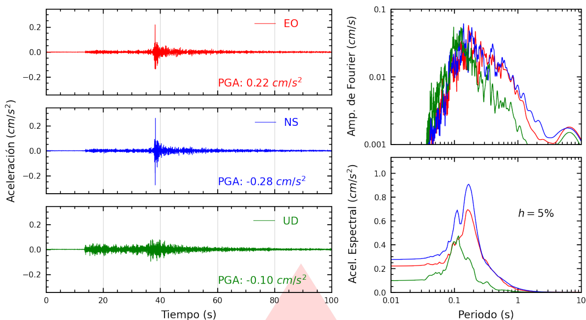
Figura A.1: Registros tiempo-historia, espectros de Fourier y de respuesta en las direcciones EO, NS y vertical de la estación UNIA. Sismo de Tingo María, Leoncio Prado - Huánuco del 2026-03-28, 23:05:11 (Hora local)
