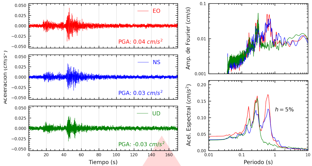
Figura A.1: Registros tiempo-historia, espectros de Fourier y de respuesta en las direcciones EO, NS y vertical de la estación CARAL. Sismo de Codo del Pozuzo, Puerto Inca - Huánuco del 2026-04-06, 11:01:17 (Hora local)
