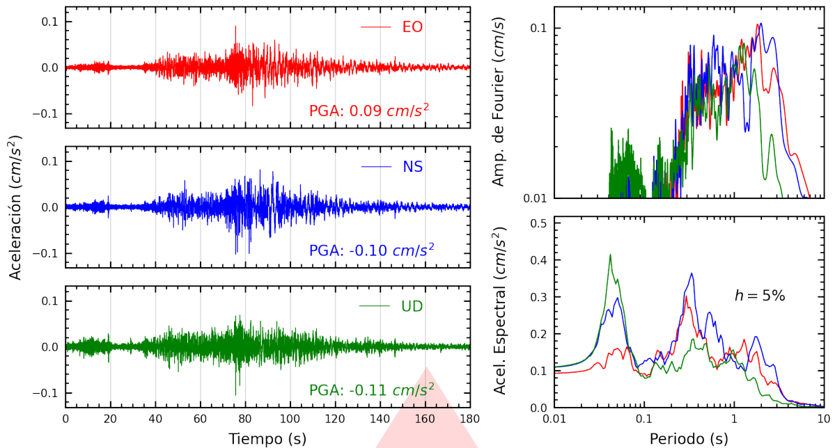
Figura A.47: Registros tiempo-historia, espectros de Fourier y de respuesta en las direcciones EO, NS y vertical de la estación SCHYO. Sismo de Pisco, Pisco - Ica del 2026-04-16, 03:09:02 (Hora local)
