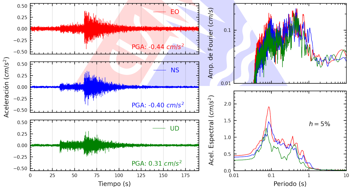
Figura A.38: Registros tiempo-historia, espectros de Fourier y de respuesta en las direcciones EO, NS y vertical de la estación INICT. Sismo de Pisco, Pisco - Ica del 2026-04-16, 03:09:02 (Hora local)
