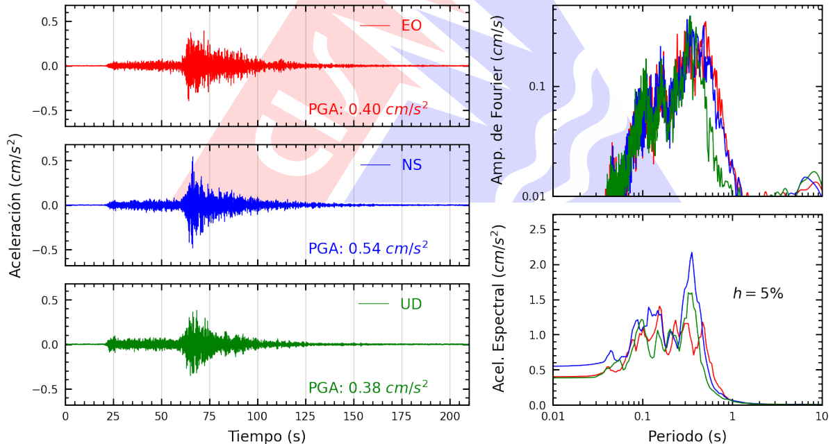
Figura A.34: Registros tiempo-historia, espectros de Fourier y de respuesta en las direcciones EO, NS y vertical de la estación CARAL. Sismo de Pisco, Pisco - Ica del 2026-04-16, 03:09:02 (Hora local)
