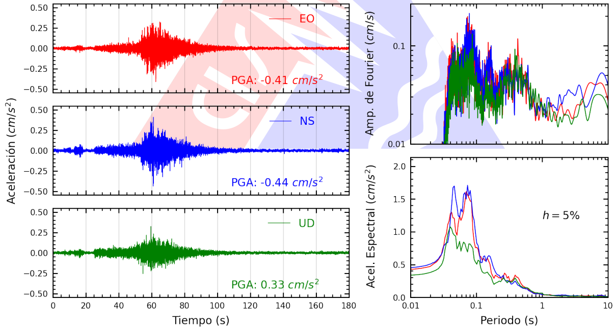
Figura A.40: Registros tiempo-historia, espectros de Fourier y de respuesta en las direcciones EO, NS y vertical de la estación SJLCE. Sismo de Pisco, Pisco - Ica del 2026-04-16, 03:09:02 (Hora local)
