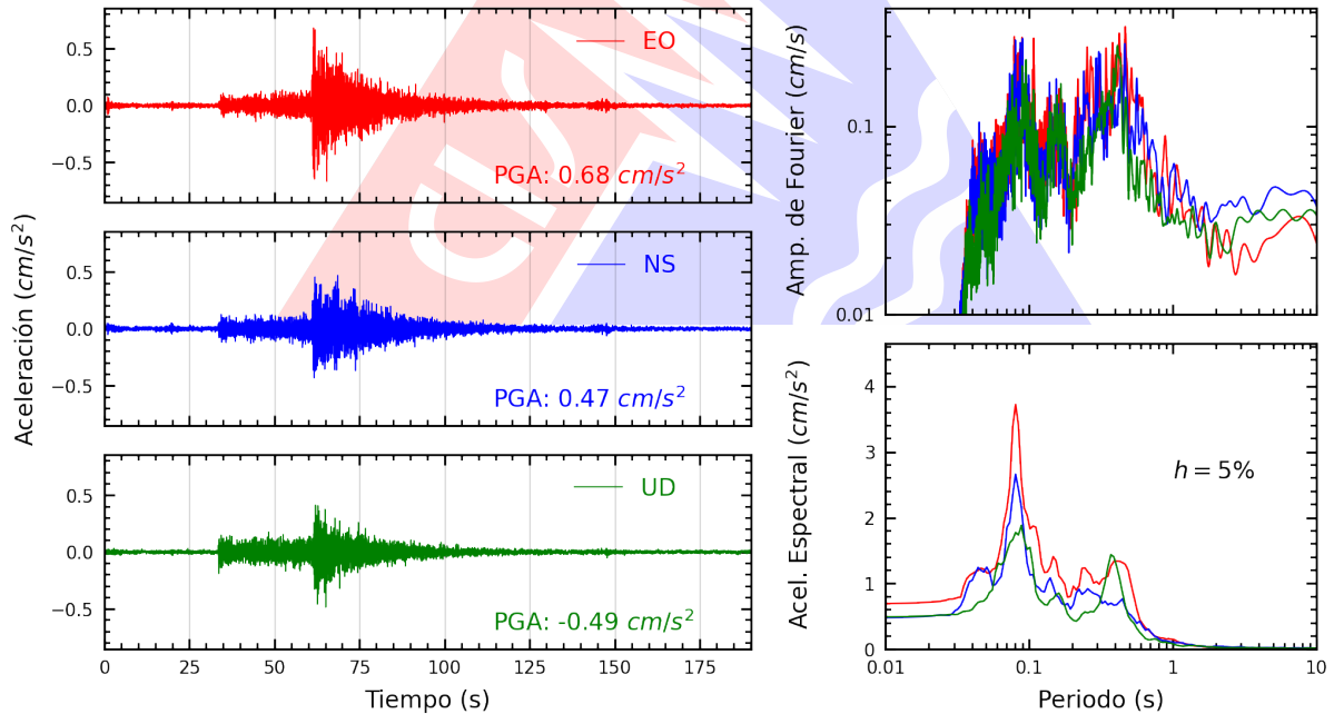
Figura A.26: Registros tiempo-historia, espectros de Fourier y de respuesta en las direcciones EO, NS y vertical de la estación CEPRE. Sismo de Pisco, Pisco - Ica del 2026-04-16, 03:09:02 (Hora local)
