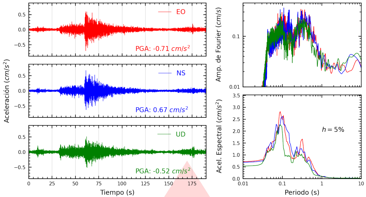
Figura A.25: Registros tiempo-historia, espectros de Fourier y de respuesta en las direcciones EO, NS y vertical de la estación URPE. Sismo de Pisco, Pisco - Ica del 2026-04-16, 03:09:02 (Hora local)
