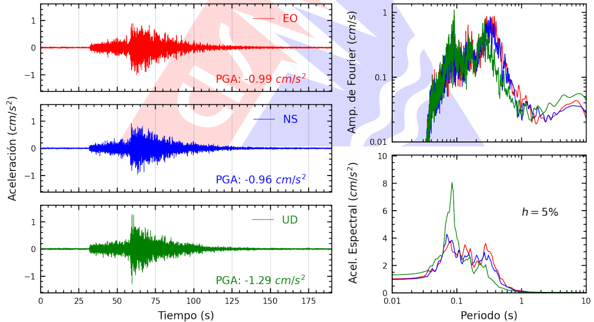
Figura A.12: Registros tiempo-historia, espectros de Fourier y de respuesta en las direcciones EO, NS y vertical de la estación SOVES. Sismo de Pisco, Pisco - Ica del 2026-04-16, 03:09:02 (Hora local)
