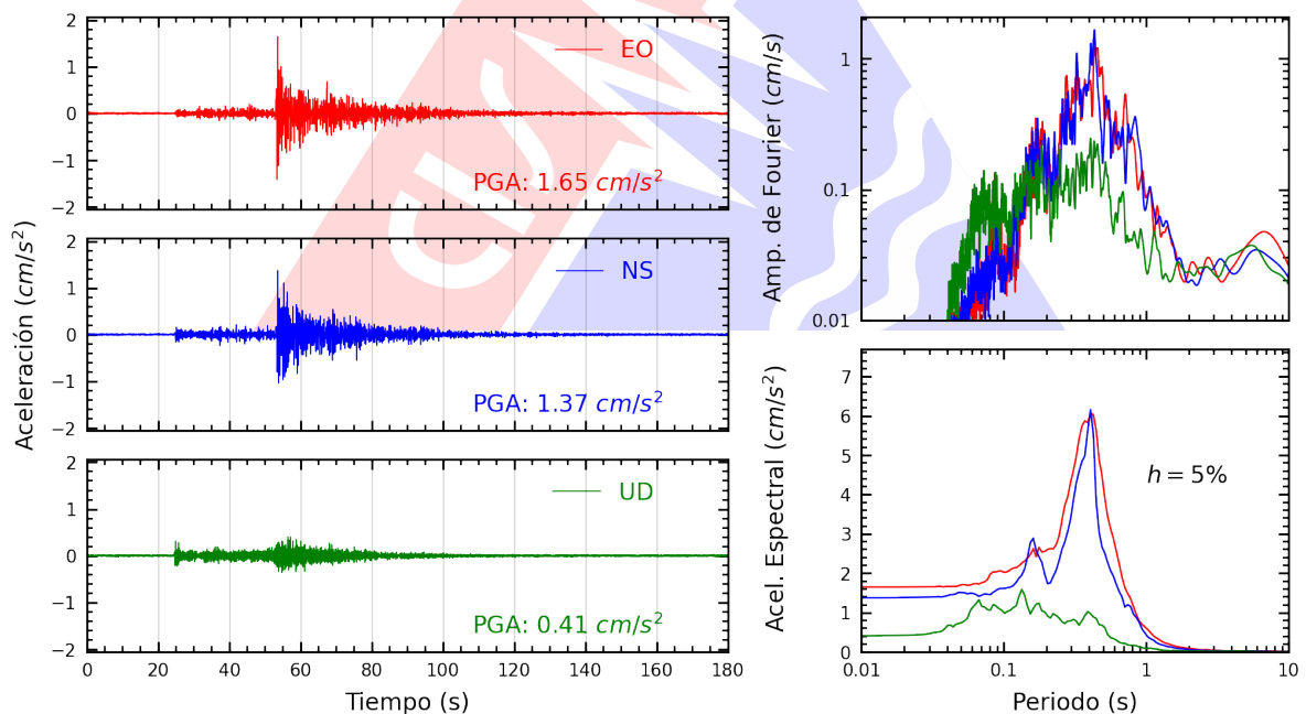
Figura A.6: Registros tiempo-historia, espectros de Fourier y de respuesta en las direcciones EO, NS y vertical de la estación ACAPU. Sismo de Pisco, Pisco - Ica del 2026-04-16, 03:09:02 (Hora local)
