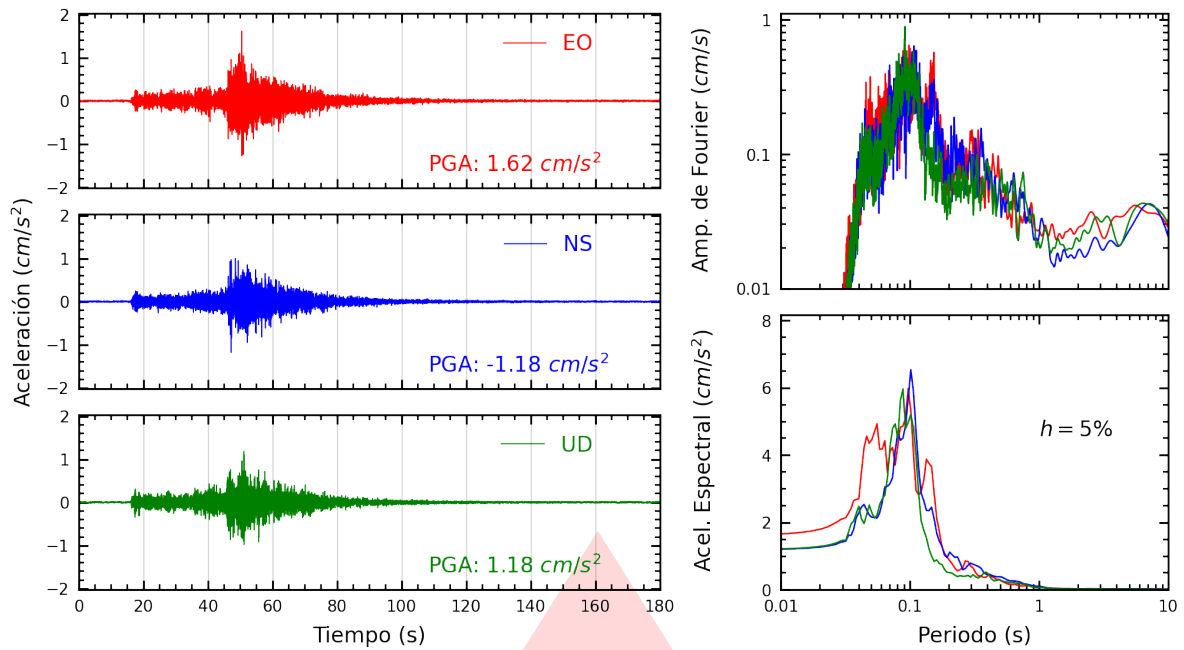
Figura A.7: Registros tiempo-historia, espectros de Fourier y de respuesta en las direcciones EO, NS y vertical de la estación AMORE. Sismo de Pisco, Pisco - Ica del 2026-04-16, 03:09:02 (Hora local)
