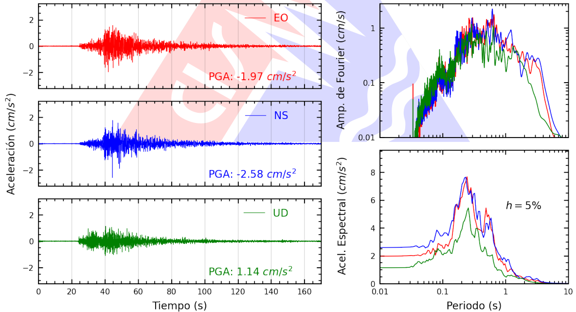
Figura A.2: Registros tiempo-historia, espectros de Fourier y de respuesta en las direcciones EO, NS y vertical de la estación SCICA. Sismo de Pisco, Pisco - Ica del 2026-04-16, 03:09:02 (Hora local)
