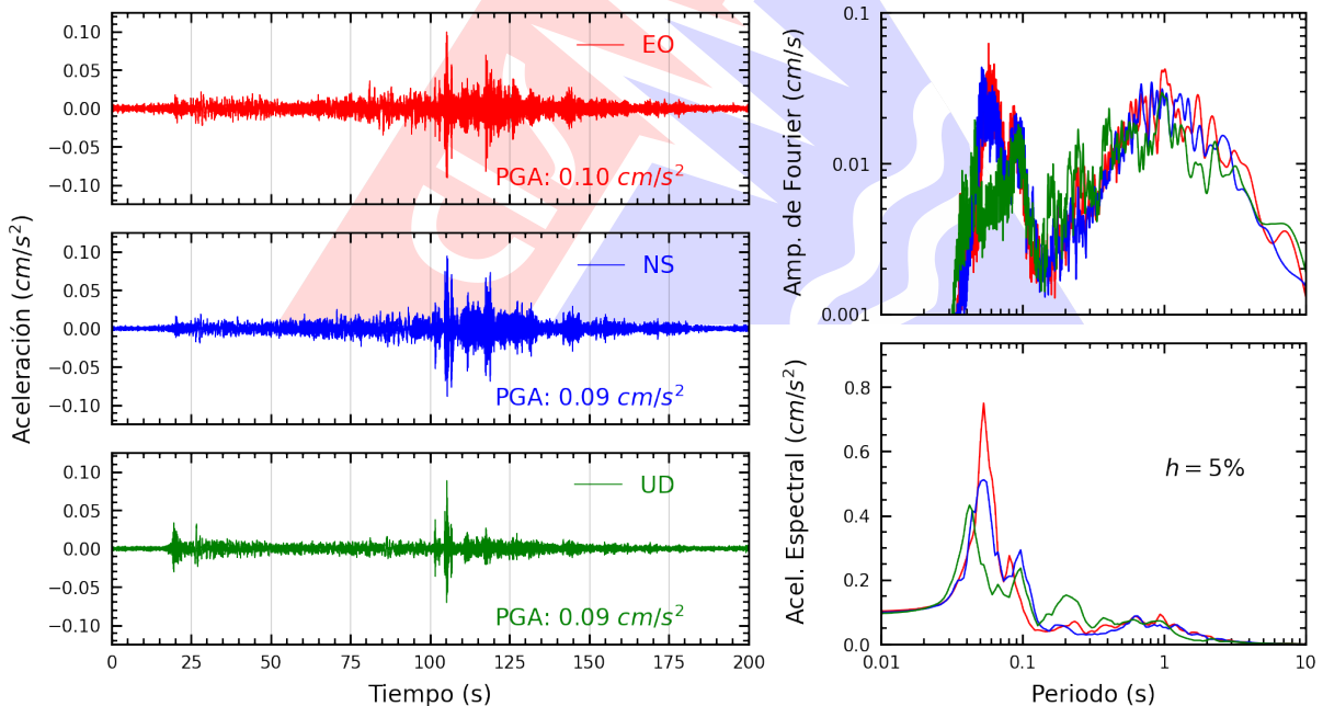
Figura A.48: Registros tiempo-historia, espectros de Fourier y de respuesta en las direcciones EO, NS y vertical de la estación UNMBA. Sismo de Pisco, Pisco - Ica del 2026-04-16, 03:09:02 (Hora local)
