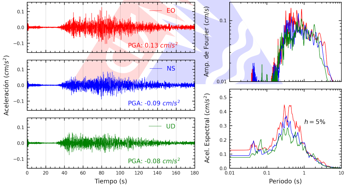
Figura A.46: Registros tiempo-historia, espectros de Fourier y de respuesta en las direcciones EO, NS y vertical de la estación SCAYA. Sismo de Pisco, Pisco - Ica del 2026-04-16, 03:09:02 (Hora local)
