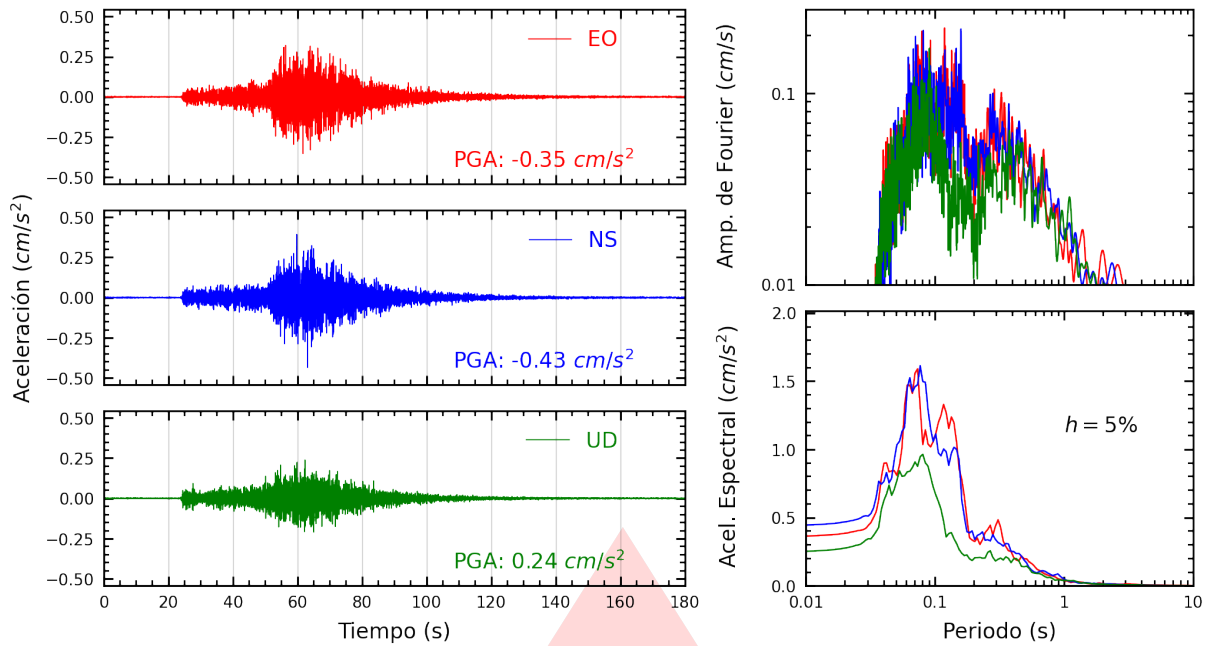
Figura A.41: Registros tiempo-historia, espectros de Fourier y de respuesta en las direcciones EO, NS y vertical de la estación ATARJ. Sismo de Pisco, Pisco - Ica del 2026-04-16, 03:09:02 (Hora local)
