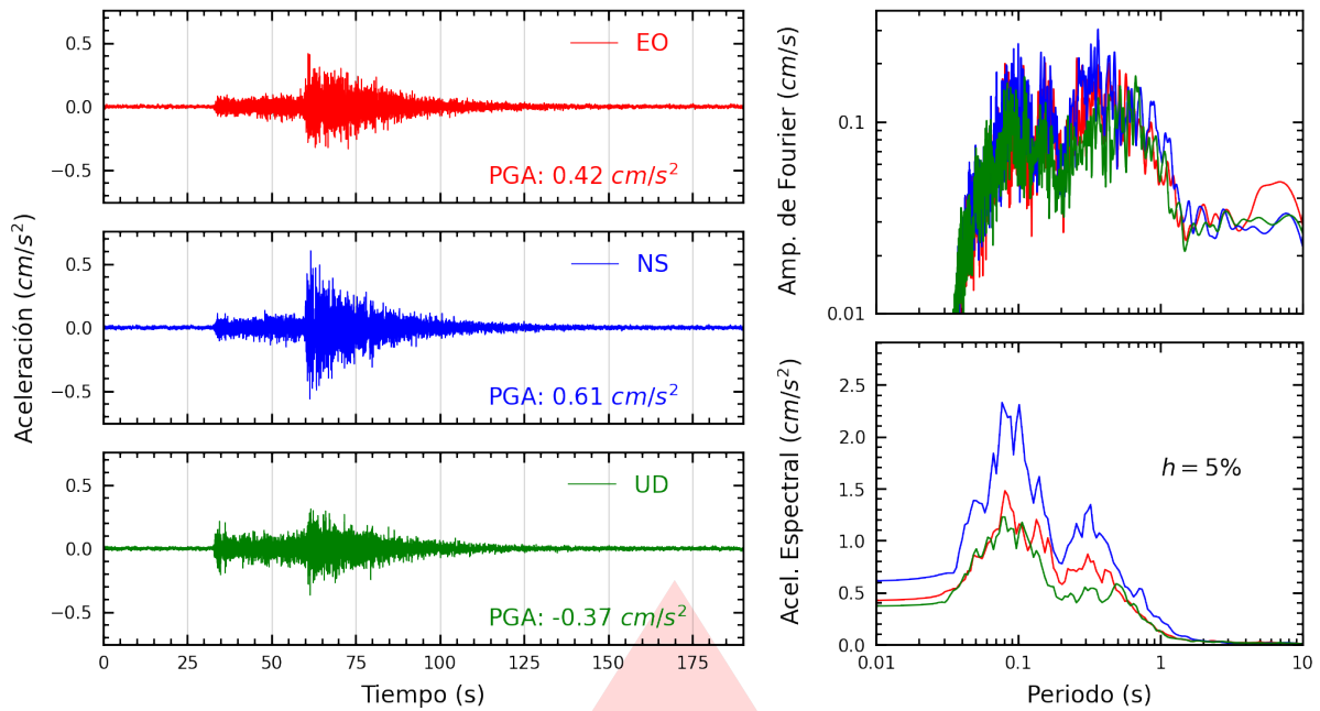
Figura A.31: Registros tiempo-historia, espectros de Fourier y de respuesta en las direcciones EO, NS y vertical de la estación SERVI. Sismo de Pisco, Pisco - Ica del 2026-04-16, 03:09:02 (Hora local)
