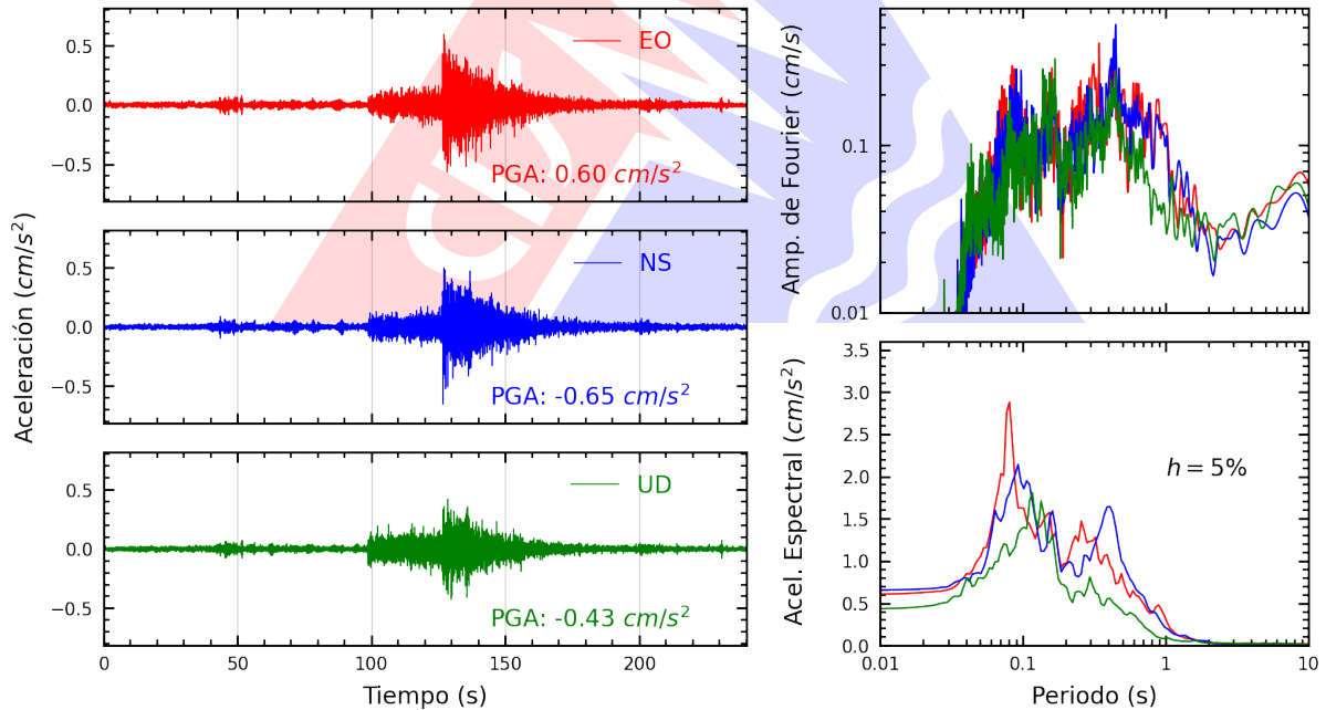
Figura A.28: Registros tiempo-historia, espectros de Fourier y de respuesta en las direcciones EO, NS y vertical de la estación UPCS. Sismo de Pisco, Pisco - Ica del 2026-04-16, 03:09:02 (Hora local)
