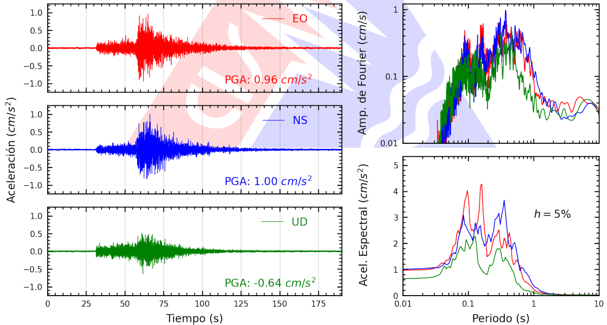
Figura A.20: Registros tiempo-historia, espectros de Fourier y de respuesta en las direcciones EO, NS y vertical de la estación USILP. Sismo de Pisco, Pisco - Ica del 2026-04-16, 03:09:02 (Hora local)
