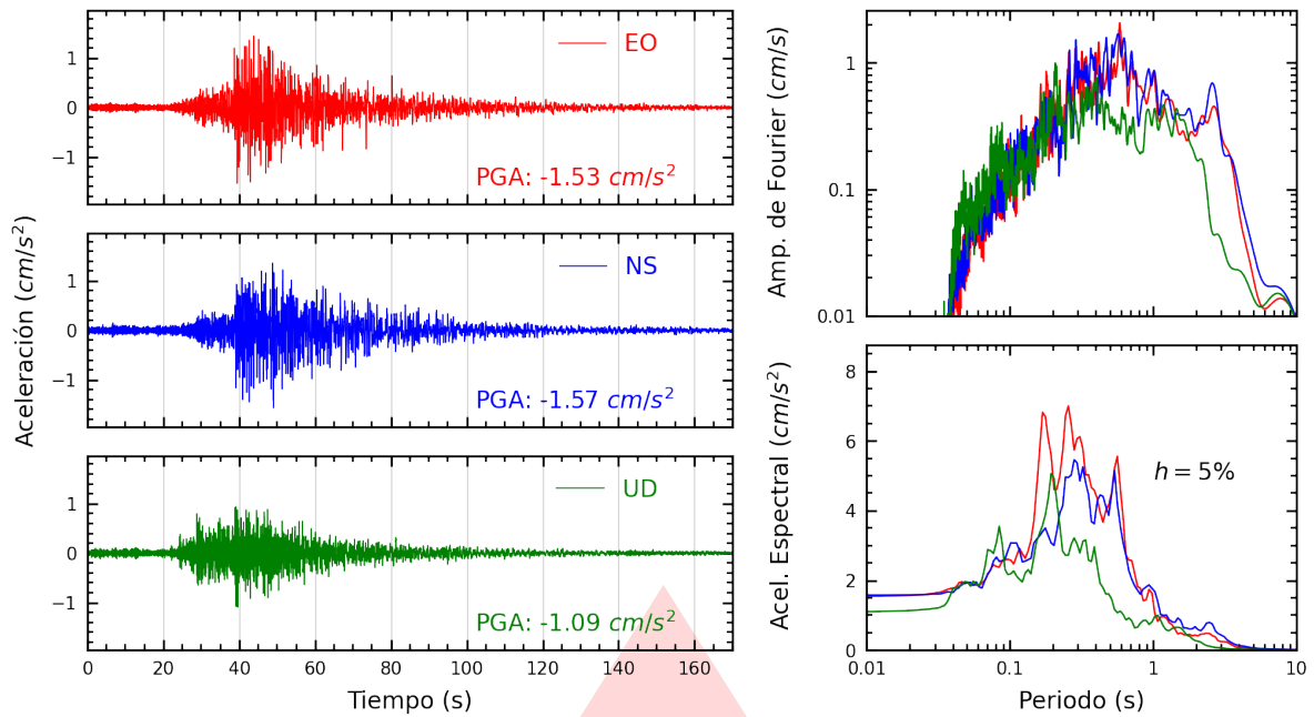
Figura A.9: Registros tiempo-historia, espectros de Fourier y de respuesta en las direcciones EO, NS y vertical de la estación UNICA. Sismo de Pisco, Pisco - Ica del 2026-04-16, 03:09:02 (Hora local)
