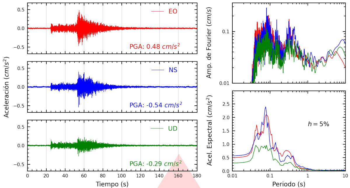
Figura A.33: Registros tiempo-historia, espectros de Fourier y de respuesta en las direcciones EO, NS y vertical de la estación UCSS. Sismo de Pisco, Pisco - Ica del 2026-04-16, 03:09:02 (Hora local)
