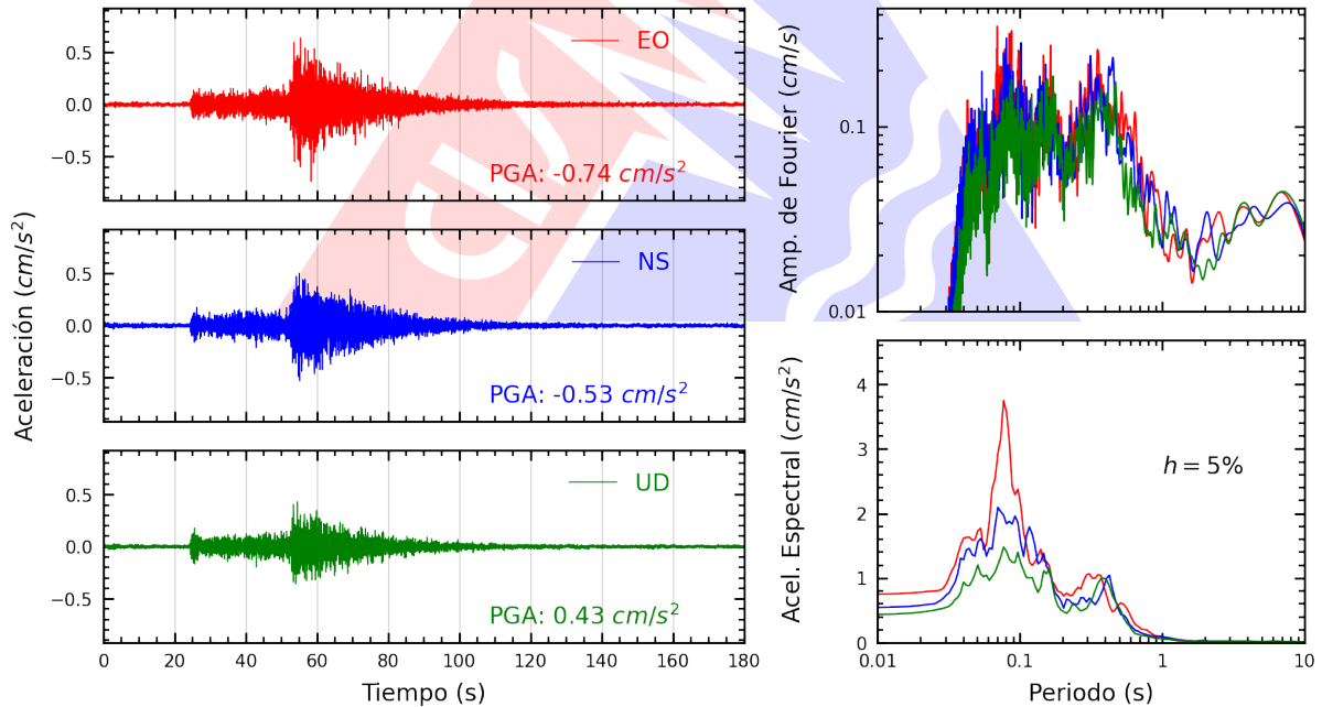
Figura A.24: Registros tiempo-historia, espectros de Fourier y de respuesta en las direcciones EO, NS y vertical de la estación FICPE. Sismo de Pisco, Pisco - Ica del 2026-04-16, 03:09:02 (Hora local)
