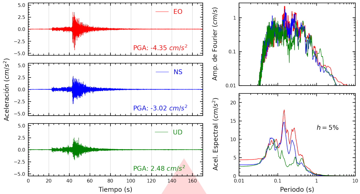
Figura A.1: Registros tiempo-historia, espectros de Fourier y de respuesta en las direcciones EO, NS y vertical de la estación ASIA. Sismo de Pisco, Pisco - Ica del 2026-04-16, 03:09:02 (Hora local)
