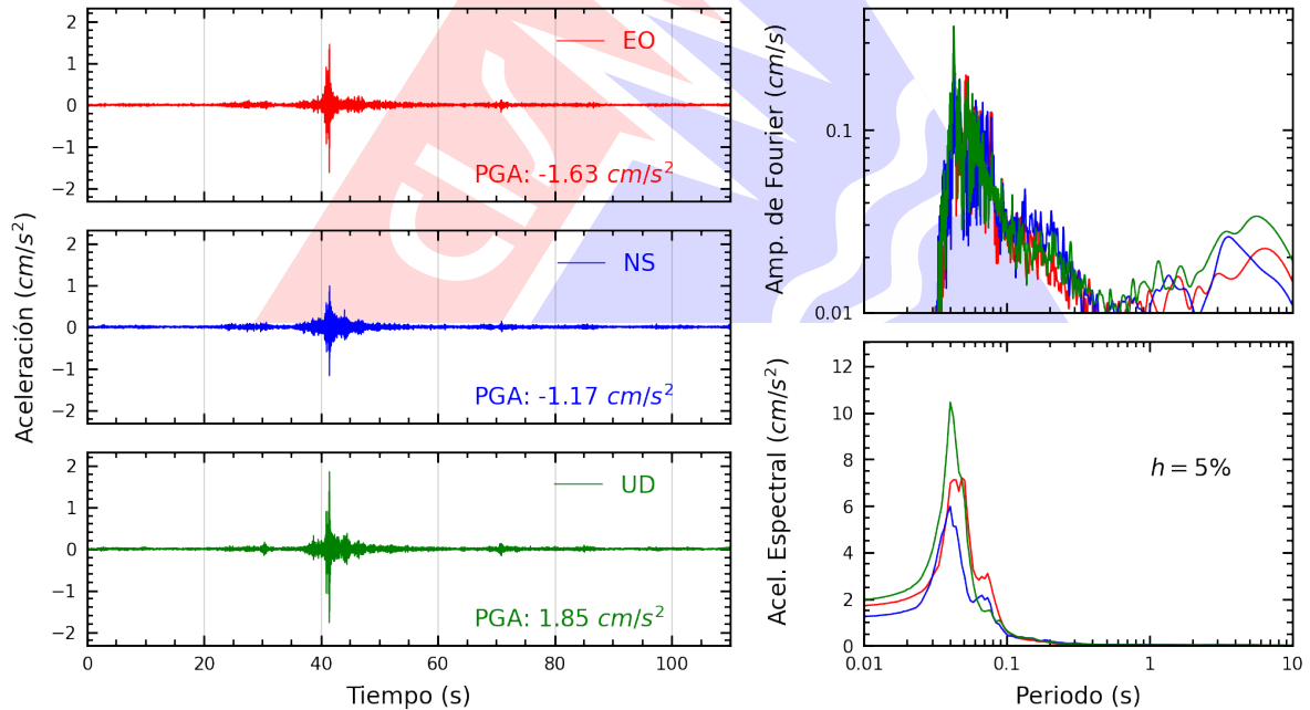
Figura A.4: Registros tiempo-historia, espectros de Fourier y de respuesta en las direcciones EO, NS y vertical de la estación PRADO. Sismo de Pisco, Pisco - Ica del 2026-04-16, 03:09:02 (Hora local)
