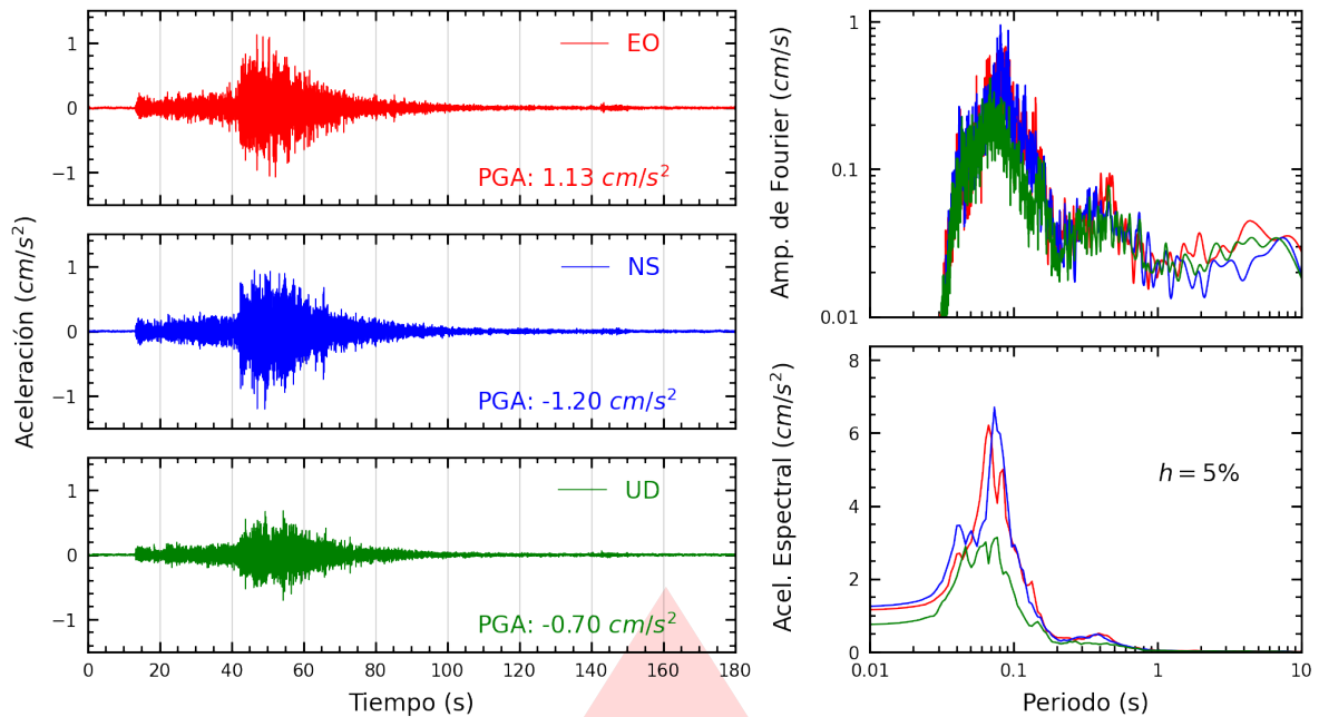
Figura A.13: Registros tiempo-historia, espectros de Fourier y de respuesta en las direcciones EO, NS y vertical de la estación JOSEO. Sismo de Pisco, Pisco - Ica del 2026-04-16, 03:09:02 (Hora local)
