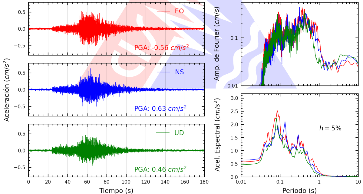
Figura A.30: Registros tiempo-historia, espectros de Fourier y de respuesta en las direcciones EO, NS y vertical de la estación UCVAT. Sismo de Pisco, Pisco - Ica del 2026-04-16, 03:09:02 (Hora local)
