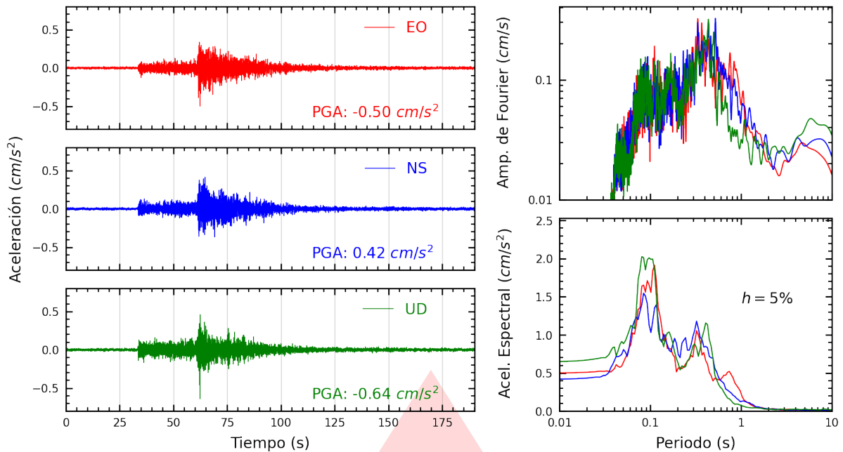
Figura A.29: Registros tiempo-historia, espectros de Fourier y de respuesta en las direcciones EO, NS y vertical de la estación UNFV. Sismo de Pisco, Pisco - Ica del 2026-04-16, 03:09:02 (Hora local)
