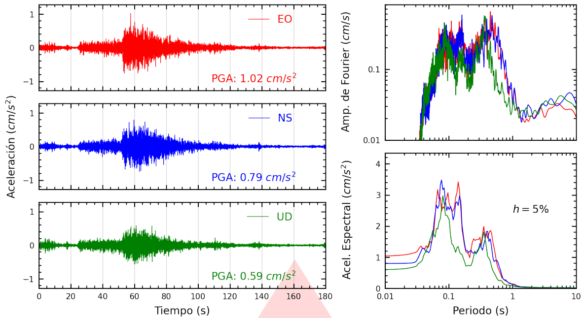
Figura A.19: Registros tiempo-historia, espectros de Fourier y de respuesta en las direcciones EO, NS y vertical de la estación SJLSV. Sismo de Pisco, Pisco - Ica del 2026-04-16, 03:09:02 (Hora local)
