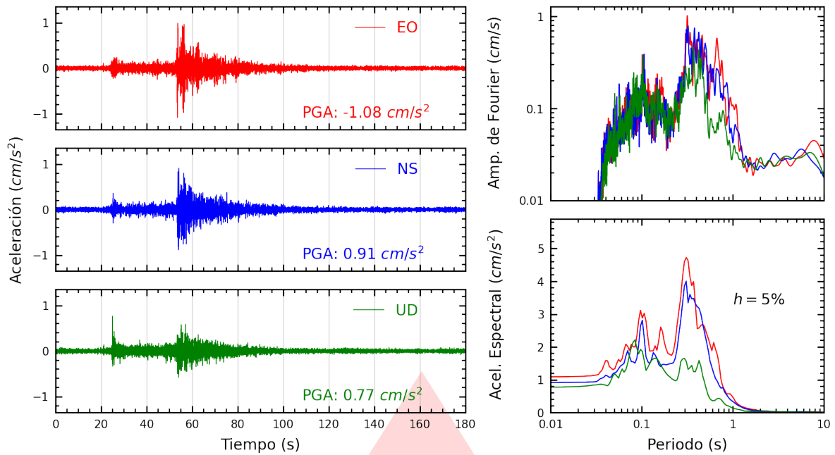
Figura A.17: Registros tiempo-historia, espectros de Fourier y de respuesta en las direcciones EO, NS y vertical de la estación MADRE. Sismo de Pisco, Pisco - Ica del 2026-04-16, 03:09:02 (Hora local)
