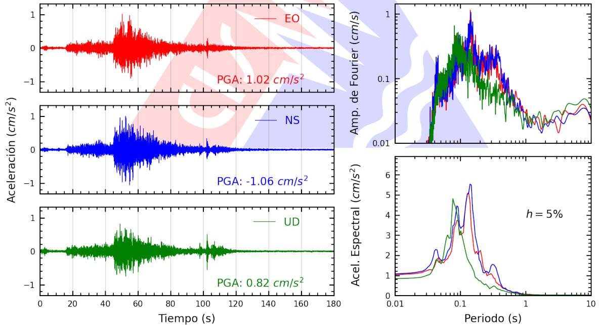
Figura A.18: Registros tiempo-historia, espectros de Fourier y de respuesta en las direcciones EO, NS y vertical de la estación CARAB. Sismo de Pisco, Pisco - Ica del 2026-04-16, 03:09:02 (Hora local)
