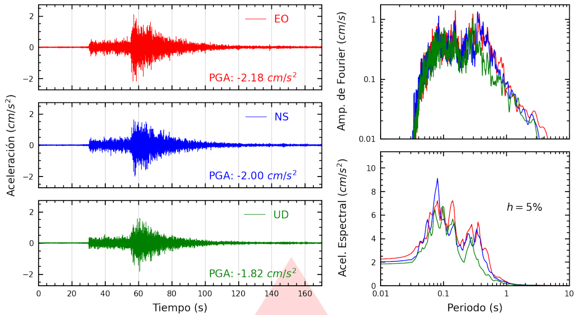
Figura A.3: Registros tiempo-historia, espectros de Fourier y de respuesta en las direcciones EO, NS y vertical de la estación PHERM. Sismo de Pisco, Pisco - Ica del 2026-04-16, 03:09:02 (Hora local)
