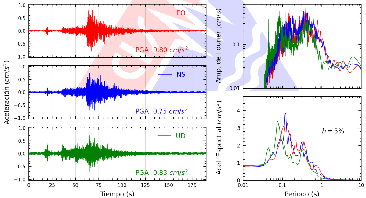
Figura A.22: Registros tiempo-historia, espectros de Fourier y de respuesta en las direcciones EO, NS y vertical de la estación SOCHO. Sismo de Pisco, Pisco - Ica del 2026-04-16, 03:09:02 (Hora local)
