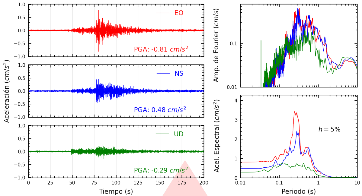
Figura A.23: Registros tiempo-historia, espectros de Fourier y de respuesta en las direcciones EO, NS y vertical de la estación DSMI. Sismo de Pisco, Pisco - Ica del 2026-04-16, 03:09:02 (Hora local)
