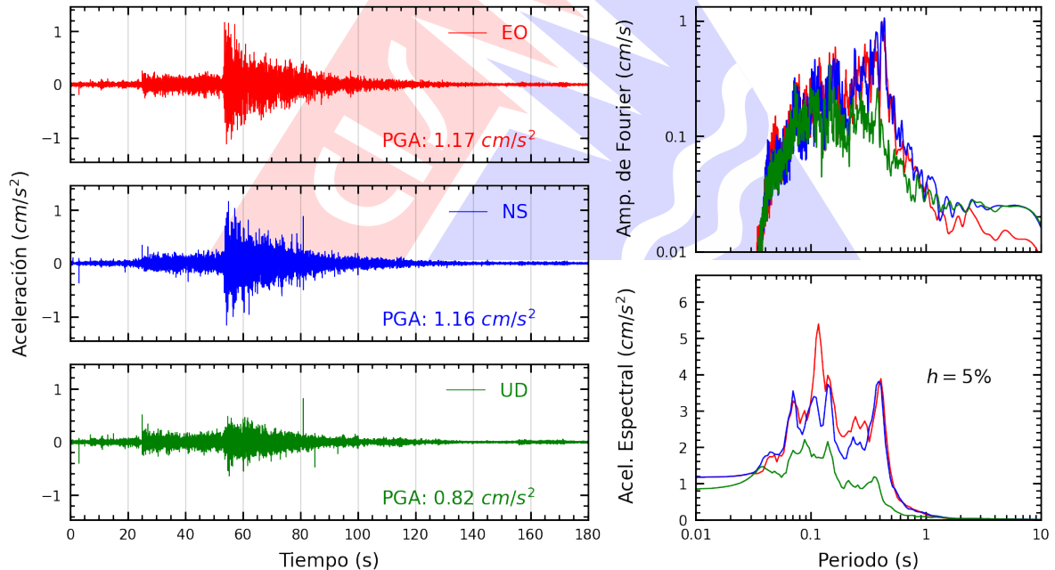
Figura A.14: Registros tiempo-historia, espectros de Fourier y de respuesta en las direcciones EO, NS y vertical de la estación SCOLI. Sismo de Pisco, Pisco - Ica del 2026-04-16, 03:09:02 (Hora local)
