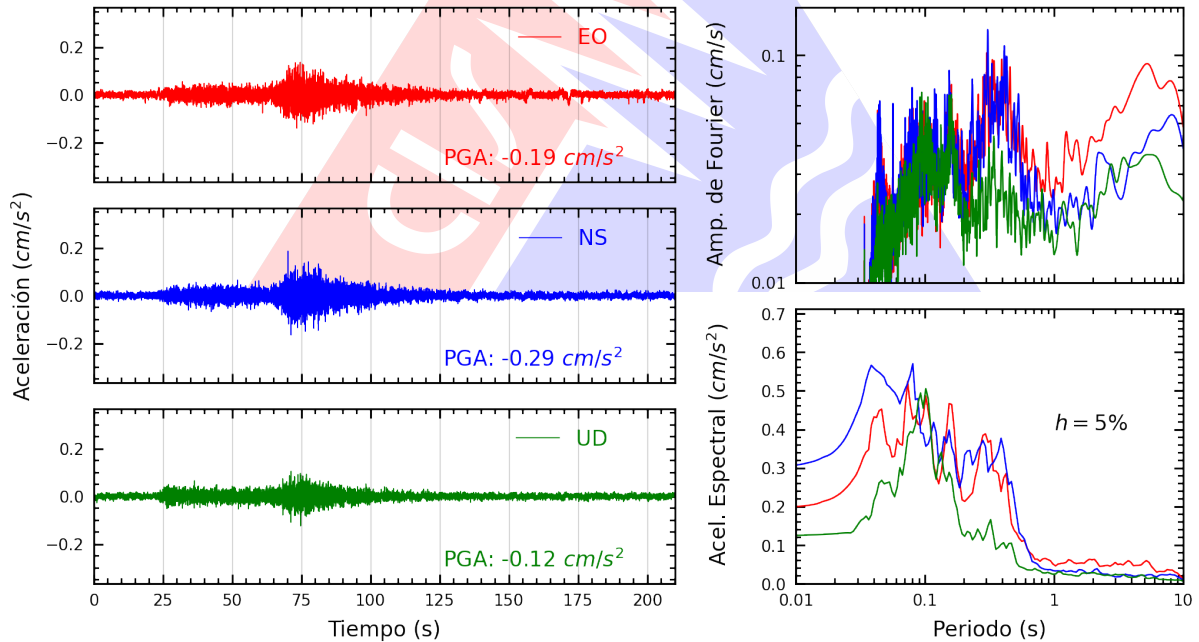
Figura A.44: Registros tiempo-historia, espectros de Fourier y de respuesta en las direcciones EO, NS y vertical de la estación UNAB. Sismo de Pisco, Pisco - Ica del 2026-04-16, 03:09:02 (Hora local)
