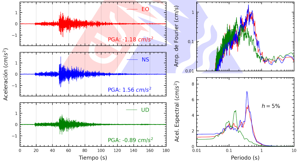
Figura A.10: Registros tiempo-historia, espectros de Fourier y de respuesta en las direcciones EO, NS y vertical de la estación MDPP. Sismo de Pisco, Pisco - Ica del 2026-04-16, 03:09:02 (Hora local)
