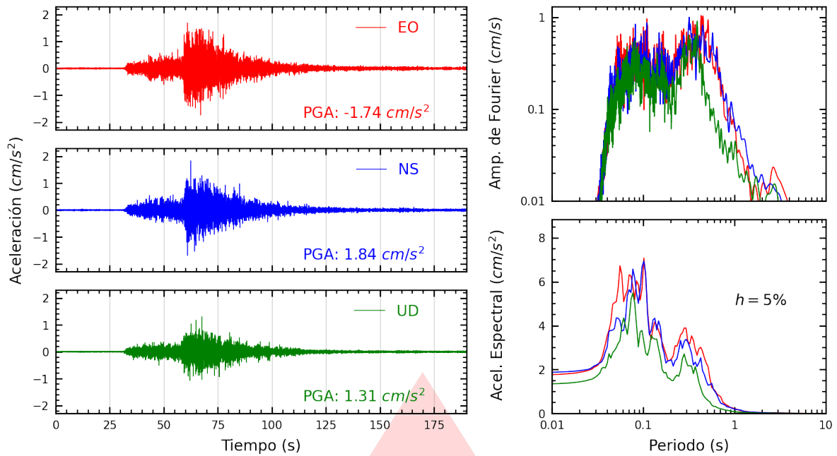
Figura A.5: Registros tiempo-historia, espectros de Fourier y de respuesta en las direcciones EO, NS y vertical de la estación UNTEL. Sismo de Pisco, Pisco - Ica del 2026-04-16, 03:09:02 (Hora local)
