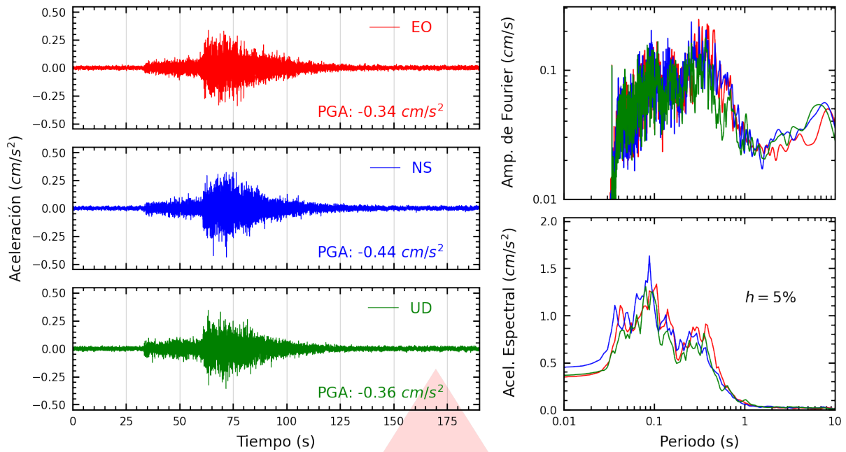
Figura A.39: Registros tiempo-historia, espectros de Fourier y de respuesta en las direcciones EO, NS y vertical de la estación USMP. Sismo de Pisco, Pisco - Ica del 2026-04-16, 03:09:02 (Hora local)
