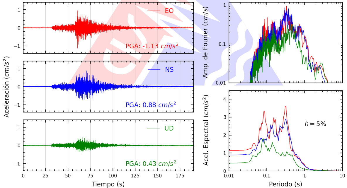
Figura A.16: Registros tiempo-historia, espectros de Fourier y de respuesta en las direcciones EO, NS y vertical de la estación BRISA. Sismo de Pisco, Pisco - Ica del 2026-04-16, 03:09:02 (Hora local)
