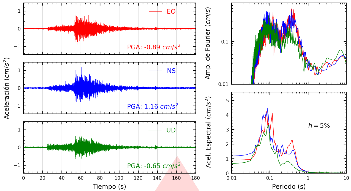
Figura A.15: Registros tiempo-historia, espectros de Fourier y de respuesta en las direcciones EO, NS y vertical de la estación SJLSC. Sismo de Pisco, Pisco - Ica del 2026-04-16, 03:09:02 (Hora local)
