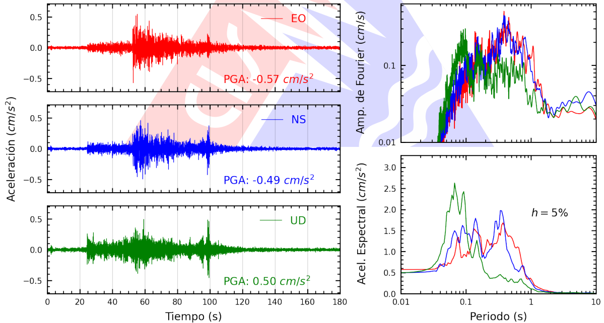
Figura A.32: Registros tiempo-historia, espectros de Fourier y de respuesta en las direcciones EO, NS y vertical de la estación RAMON. Sismo de Pisco, Pisco - Ica del 2026-04-16, 03:09:02 (Hora local)
