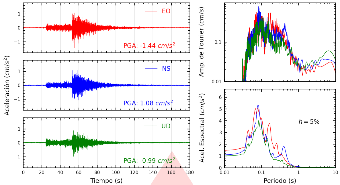
Figura A.11: Registros tiempo-historia, espectros de Fourier y de respuesta en las direcciones EO, NS y vertical de la estación INDEP. Sismo de Pisco, Pisco - Ica del 2026-04-16, 03:09:02 (Hora local)
