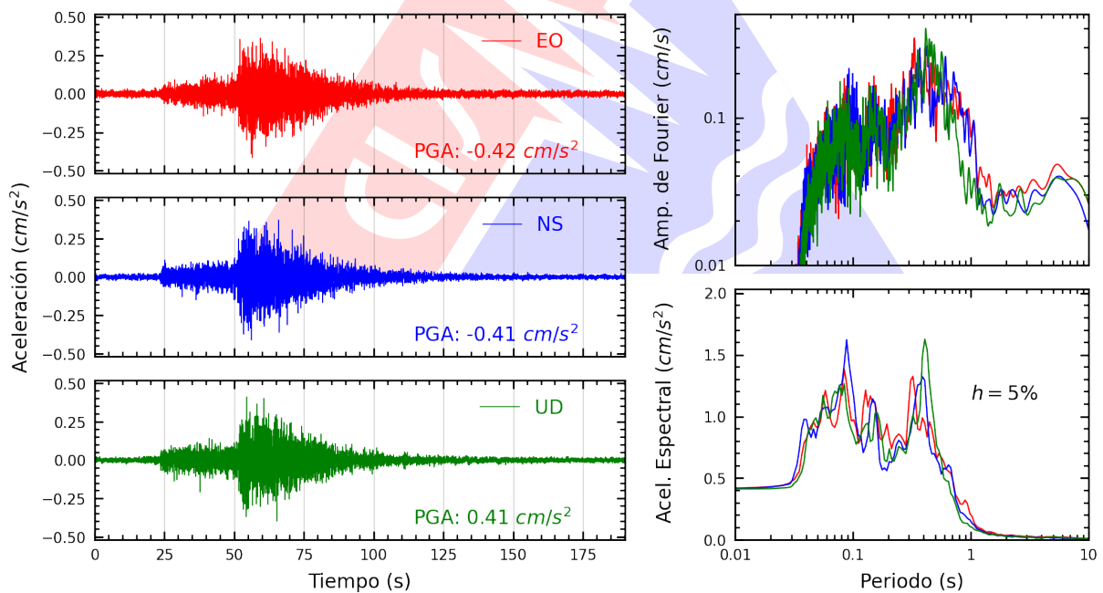
Figura A.42: Registros tiempo-historia, espectros de Fourier y de respuesta en las direcciones EO, NS y vertical de la estación IMCA. Sismo de Pisco, Pisco - Ica del 2026-04-16, 03:09:02 (Hora local)
