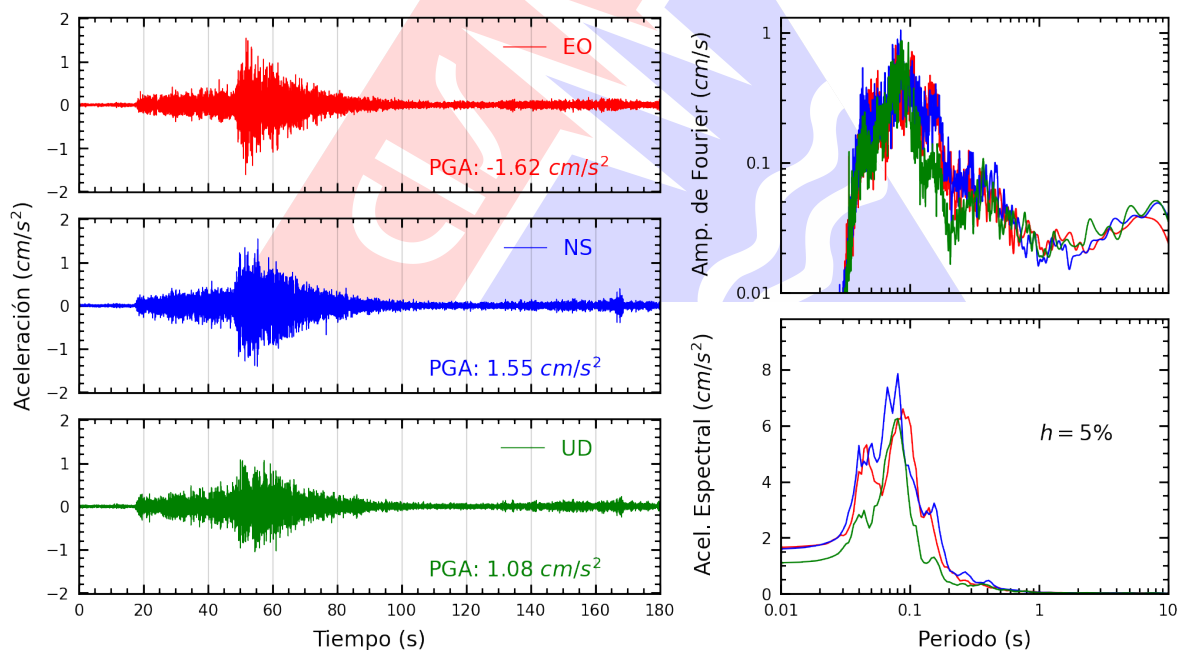
Figura A.8: Registros tiempo-historia, espectros de Fourier y de respuesta en las direcciones EO, NS y vertical de la estación SROSA. Sismo de Pisco, Pisco - Ica del 2026-04-16, 03:09:02 (Hora local)
