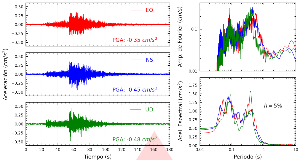
Figura A.37: Registros tiempo-historia, espectros de Fourier y de respuesta en las direcciones EO, NS y vertical de la estación COMAS. Sismo de Pisco, Pisco - Ica del 2026-04-16, 03:09:02 (Hora local)
