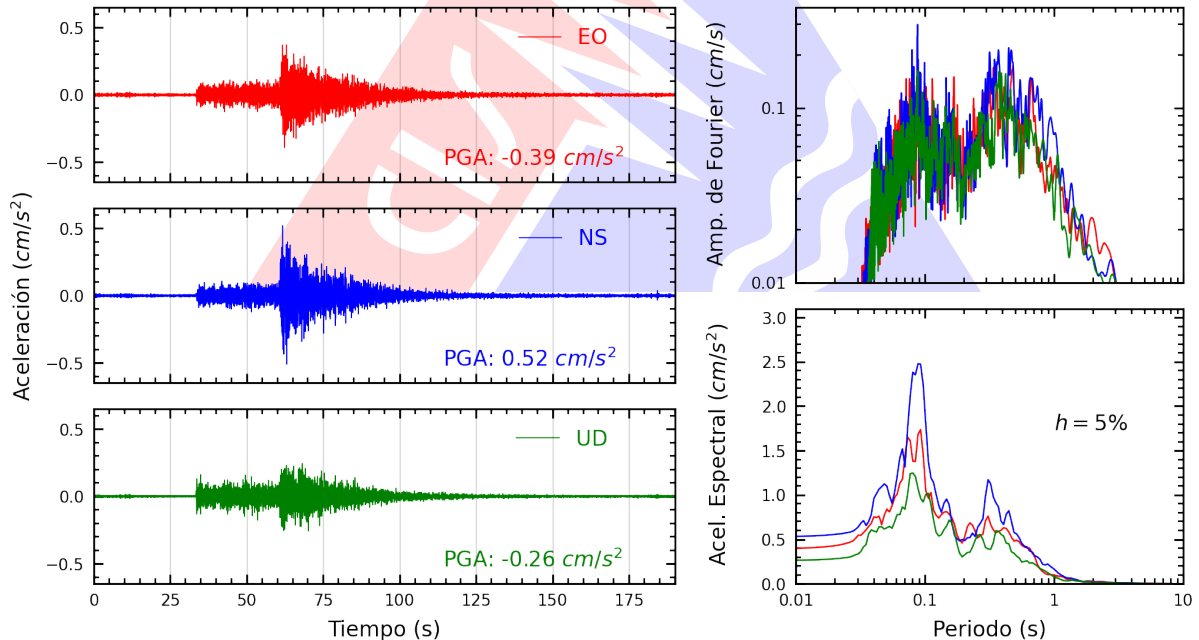
Figura A.36: Registros tiempo-historia, espectros de Fourier y de respuesta en las direcciones EO, NS y vertical de la estación BORJA. Sismo de Pisco, Pisco - Ica del 2026-04-16, 03:09:02 (Hora local)
