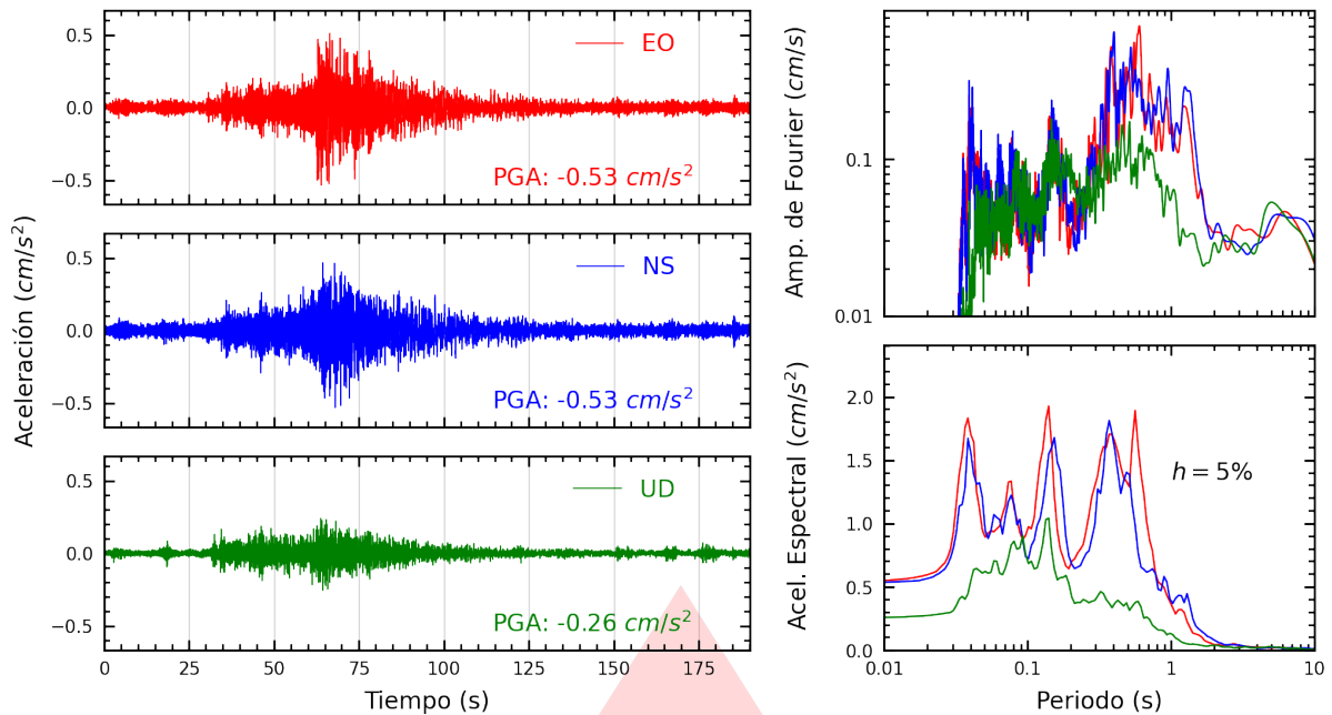
Figura A.35: Registros tiempo-historia, espectros de Fourier y de respuesta en las direcciones EO, NS y vertical de la estación DHNPE. Sismo de Pisco, Pisco - Ica del 2026-04-16, 03:09:02 (Hora local)
