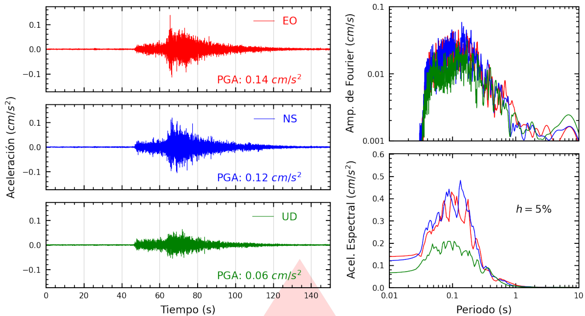
Figura A.45: Registros tiempo-historia, espectros de Fourier y de respuesta en las direcciones EO, NS y vertical de la estación UNSA2. Sismo de Pisco, Pisco - Ica del 2026-04-16, 03:09:02 (Hora local)
