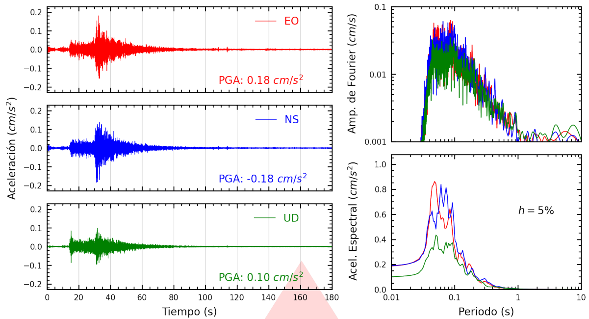
Figura A.1: Registros tiempo-historia, espectros de Fourier y de respuesta en las direcciones EO, NS y vertical de la estación UNSA2. Sismo de Ilo, Ilo - Moquegua del 2026-04-24, 11:18:19 (Hora local)
