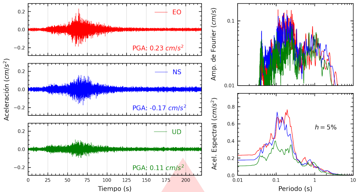
Figura A.23: Registros tiempo-historia, espectros de Fourier y de respuesta en las direcciones EO, NS y vertical de la estación ATARJ. Sismo de Ica, Ica - Ica del 2026-04-25, 15:14:40 (Hora local)
