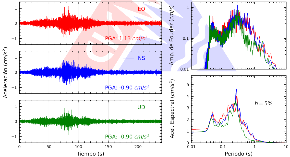
Figura A.6: Registros tiempo-historia, espectros de Fourier y de respuesta en las direcciones EO, NS y vertical de la estación UNTEL. Sismo de Ica, Ica - Ica del 2026-04-25, 15:14:40 (Hora local)
