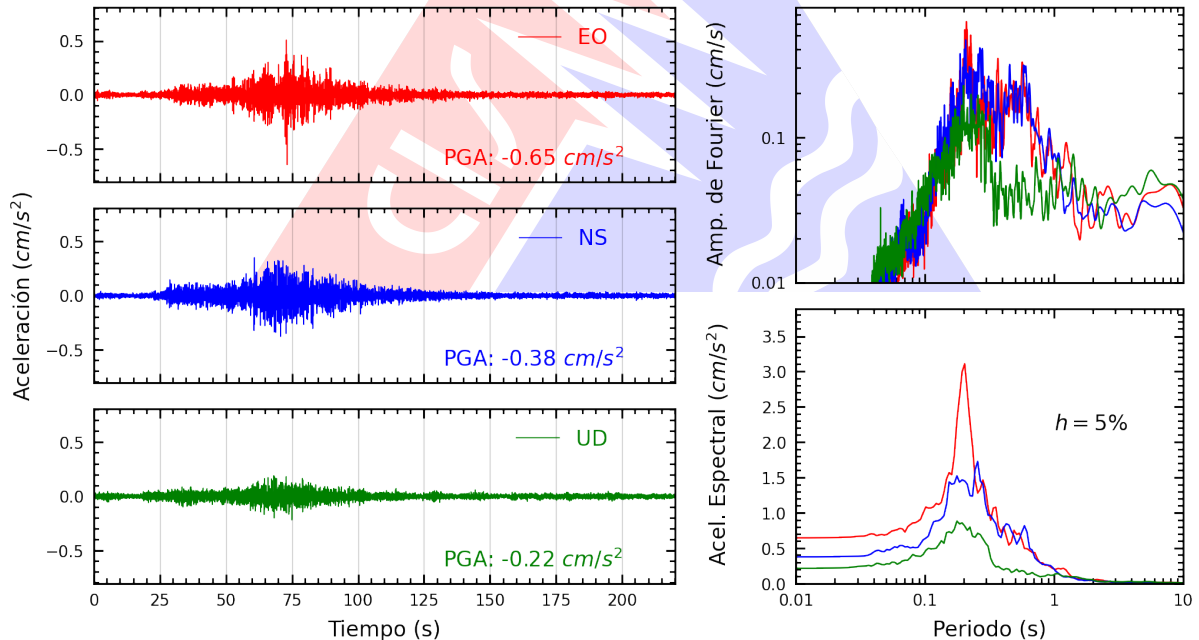
Figura A.12: Registros tiempo-historia, espectros de Fourier y de respuesta en las direcciones EO, NS y vertical de la estación VHAYA. Sismo de Ica, Ica - Ica del 2026-04-25, 15:14:40 (Hora local)
