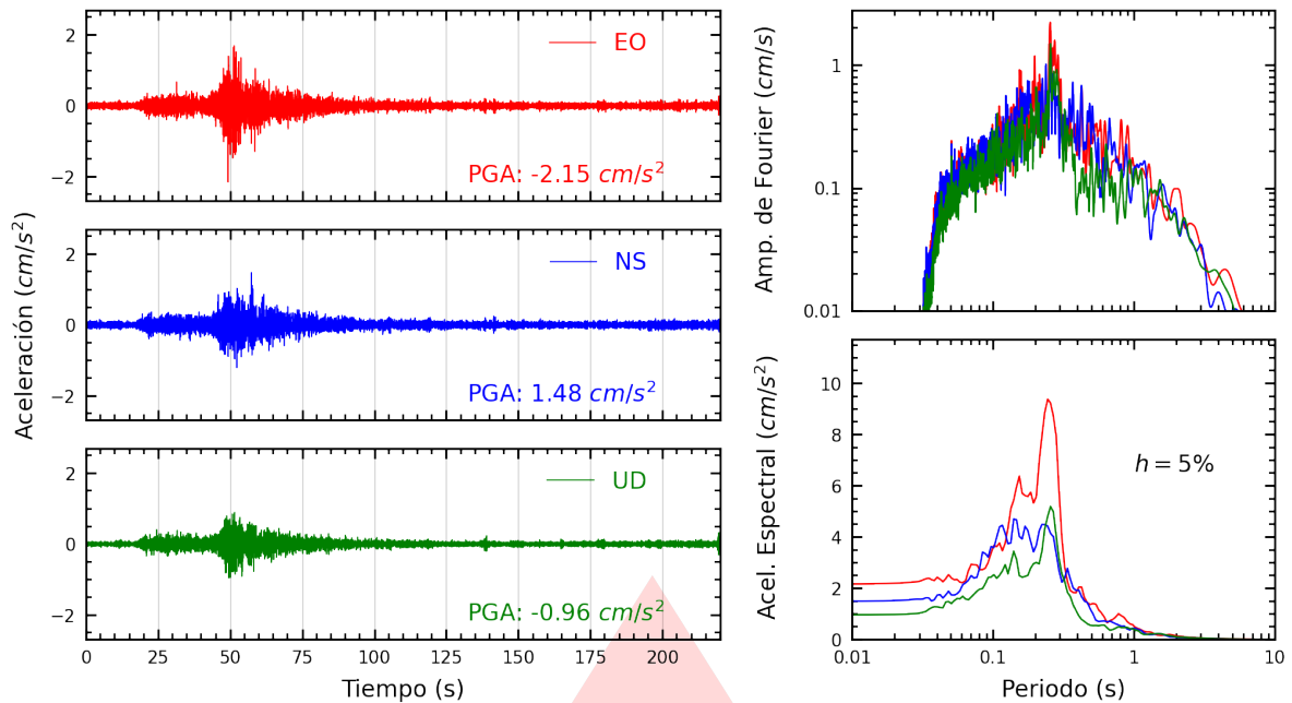
Figura A.3: Registros tiempo-historia, espectros de Fourier y de respuesta en las direcciones EO, NS y vertical de la estación PHERM. Sismo de Ica, Ica - Ica del 2026-04-25, 15:14:40 (Hora local)
