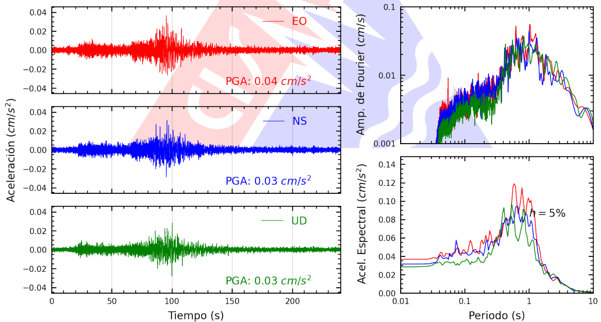
Figura A.26: Registros tiempo-historia, espectros de Fourier y de respuesta en las direcciones EO, NS y vertical de la estación UNSA2. Sismo de Ica, Ica - Ica del 2026-04-25, 15:14:40 (Hora local)
