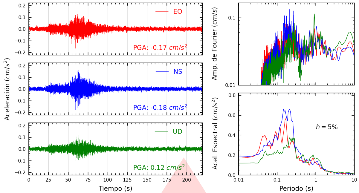
Figura A.25: Registros tiempo-historia, espectros de Fourier y de respuesta en las direcciones EO, NS y vertical de la estación UCSS. Sismo de Ica, Ica - Ica del 2026-04-25, 15:14:40 (Hora local)
