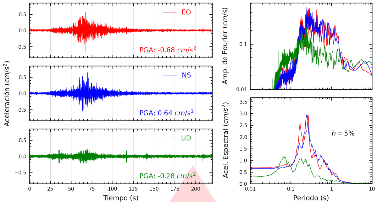
Figura A.11: Registros tiempo-historia, espectros de Fourier y de respuesta en las direcciones EO, NS y vertical de la estación ACAPU. Sismo de Ica, Ica - Ica del 2026-04-25, 15:14:40 (Hora local)
