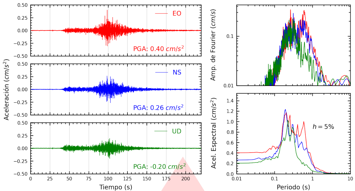
Figura A.17: Registros tiempo-historia, espectros de Fourier y de respuesta en las direcciones EO, NS y vertical de la estación CARAL. Sismo de Ica, Ica - Ica del 2026-04-25, 15:14:40 (Hora local)
