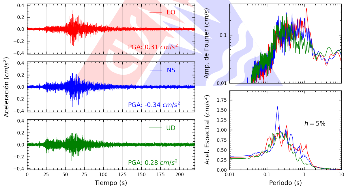
Figura A.20: Registros tiempo-historia, espectros de Fourier y de respuesta en las direcciones EO, NS y vertical de la estación UNFV. Sismo de Ica, Ica - Ica del 2026-04-25, 15:14:40 (Hora local)
