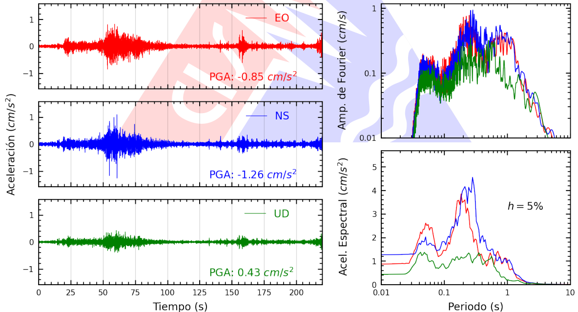
Figura A.4: Registros tiempo-historia, espectros de Fourier y de respuesta en las direcciones EO, NS y vertical de la estación BRIS2. Sismo de Ica, Ica - Ica del 2026-04-25, 15:14:40 (Hora local)
