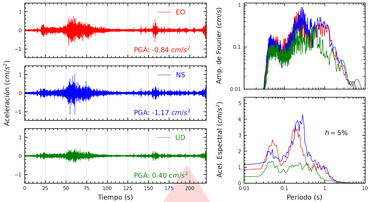
Figura A.5: Registros tiempo-historia, espectros de Fourier y de respuesta en las direcciones EO, NS y vertical de la estación BRISA. Sismo de Ica, Ica - Ica del 2026-04-25, 15:14:40 (Hora local)
