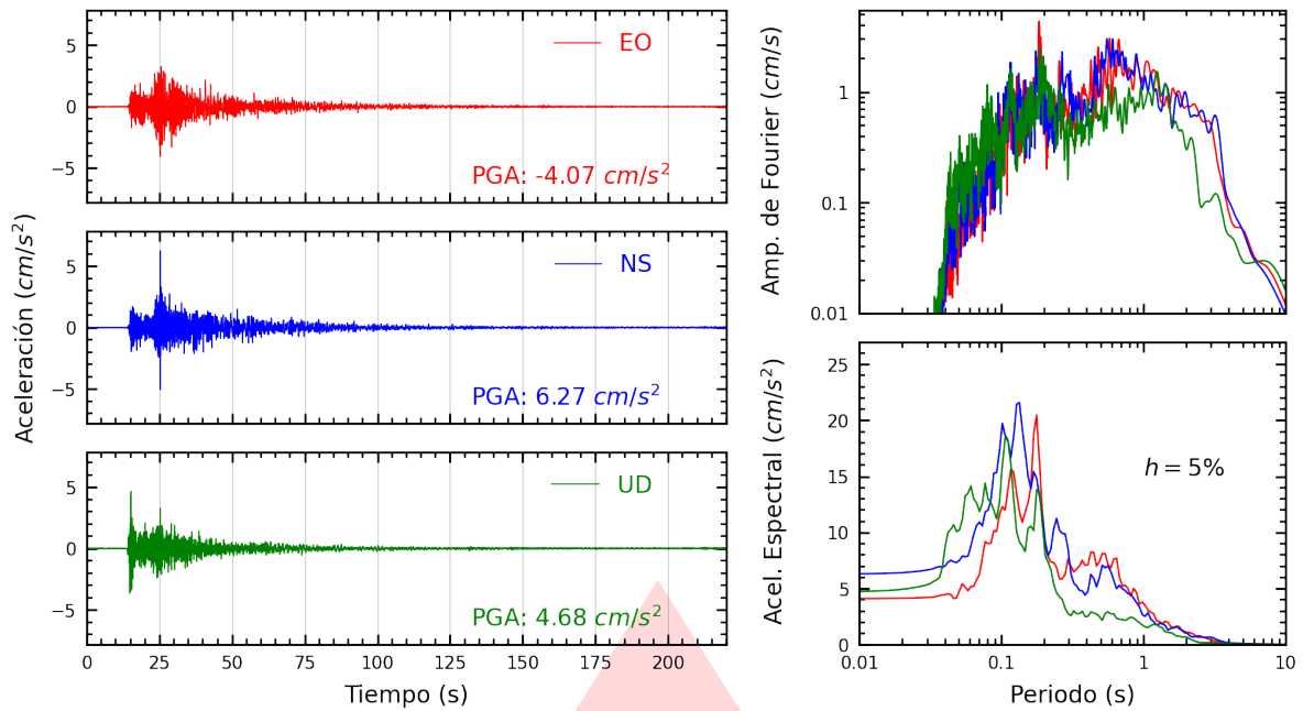
Figura A.1: Registros tiempo-historia, espectros de Fourier y de respuesta en las direcciones EO, NS y vertical de la estación UNICA. Sismo de Ica, Ica - Ica del 2026-04-25, 15:14:40 (Hora local)
