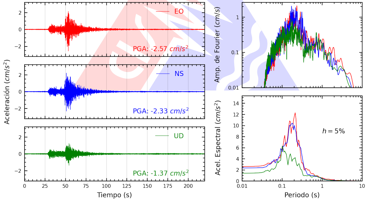
Figura A.2: Registros tiempo-historia, espectros de Fourier y de respuesta en las direcciones EO, NS y vertical de la estación ASIA. Sismo de Ica, Ica - Ica del 2026-04-25, 15:14:40 (Hora local)
