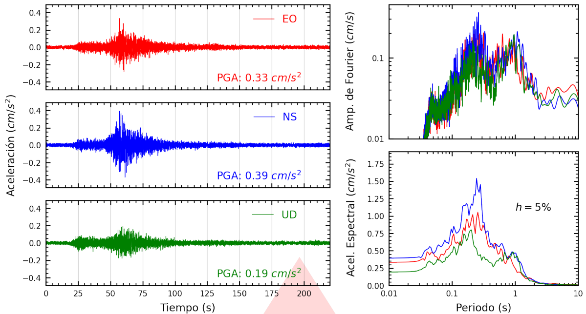
Figura A.19: Registros tiempo-historia, espectros de Fourier y de respuesta en las direcciones EO, NS y vertical de la estación SERVI. Sismo de Ica, Ica - Ica del 2026-04-25, 15:14:40 (Hora local)
