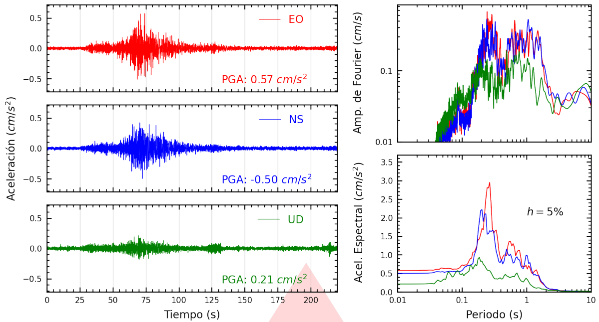
Figura A.13: Registros tiempo-historia, espectros de Fourier y de respuesta en las direcciones EO, NS y vertical de la estación DSMI. Sismo de Ica, Ica - Ica del 2026-04-25, 15:14:40 (Hora local)
