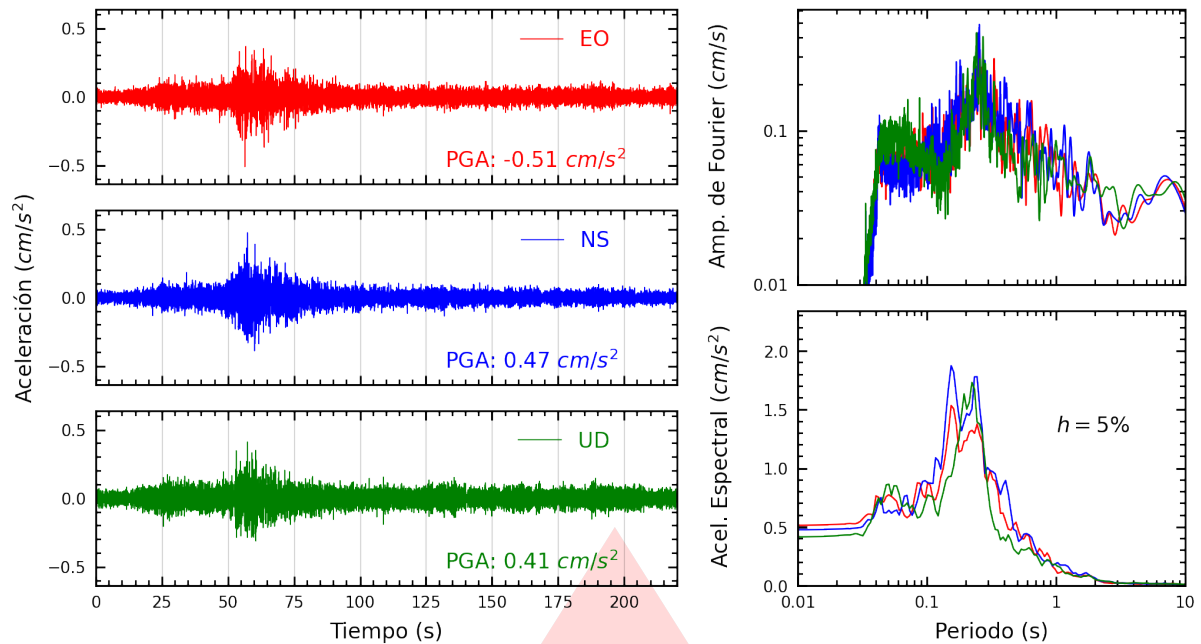
Figura A.15: Registros tiempo-historia, espectros de Fourier y de respuesta en las direcciones EO, NS y vertical de la estación URPE. Sismo de Ica, Ica - Ica del 2026-04-25, 15:14:40 (Hora local)
