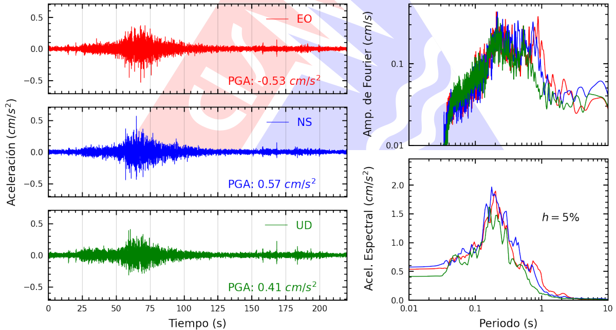
Figura A.14: Registros tiempo-historia, espectros de Fourier y de respuesta en las direcciones EO, NS y vertical de la estación UCVAT. Sismo de Ica, Ica - Ica del 2026-04-25, 15:14:40 (Hora local)
