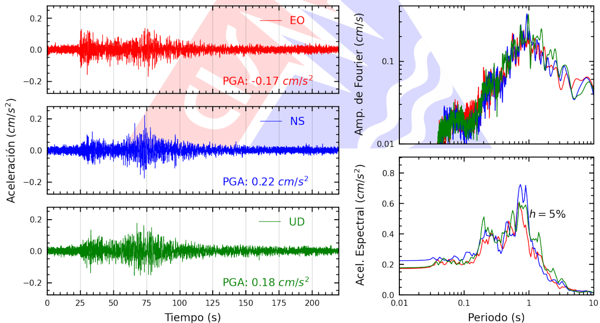
Figura A.24: Registros tiempo-historia, espectros de Fourier y de respuesta en las direcciones EO, NS y vertical de la estación UNSCH. Sismo de Ica, Ica - Ica del 2026-04-25, 15:14:40 (Hora local)
