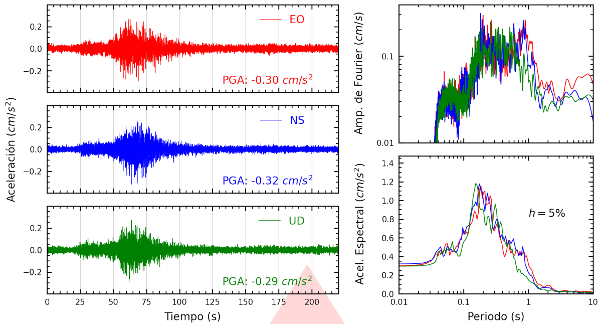
Figura A.21: Registros tiempo-historia, espectros de Fourier y de respuesta en las direcciones EO, NS y vertical de la estación IMCA. Sismo de Ica, Ica - Ica del 2026-04-25, 15:14:40 (Hora local)
