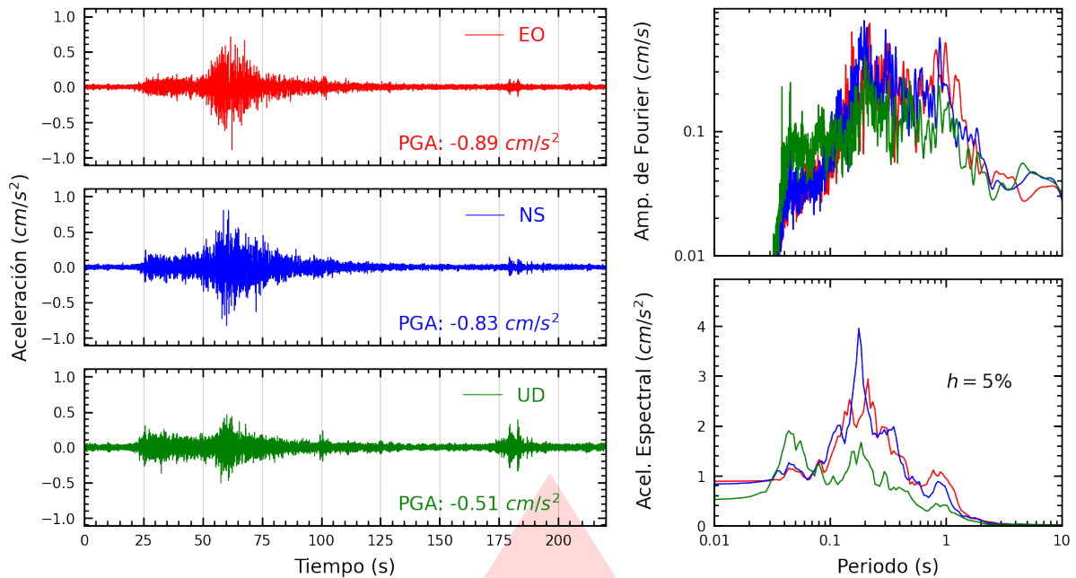
Figura A.9: Registros tiempo-historia, espectros de Fourier y de respuesta en las direcciones EO, NS y vertical de la estación SOCHO. Sismo de Ica, Ica - Ica del 2026-04-25, 15:14:40 (Hora local)
