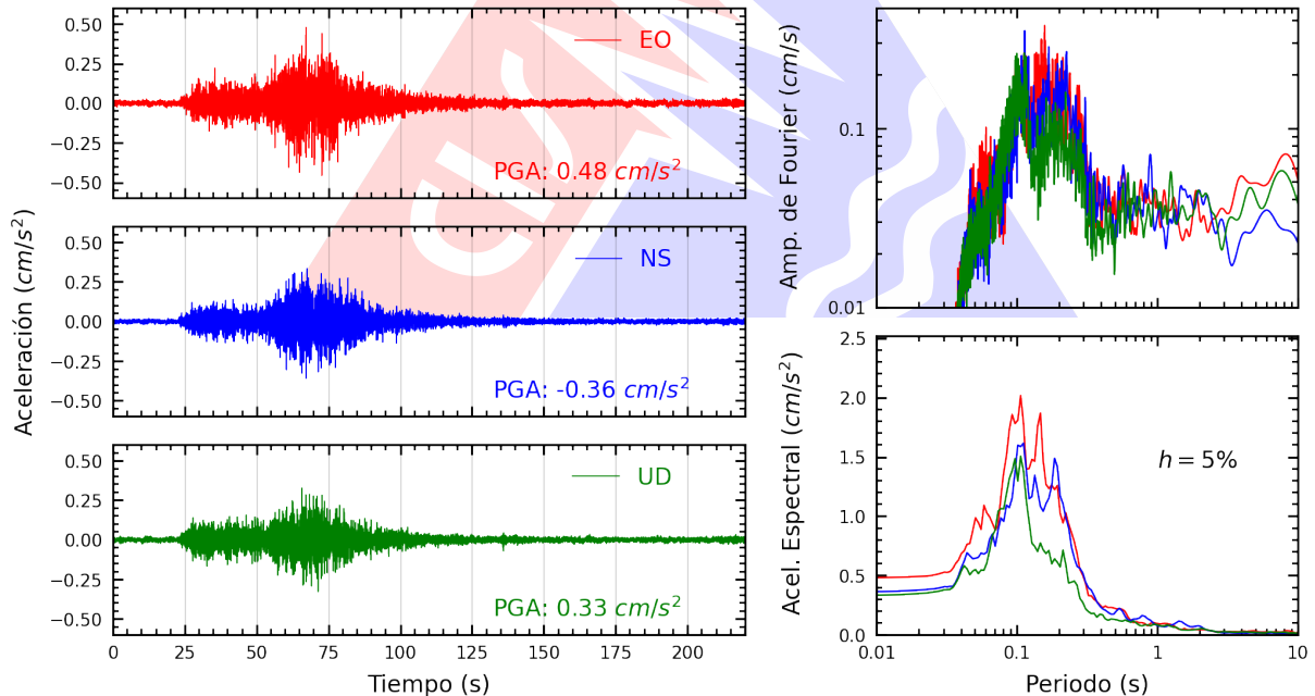
Figura A.16: Registros tiempo-historia, espectros de Fourier y de respuesta en las direcciones EO, NS y vertical de la estación AMORE. Sismo de Ica, Ica - Ica del 2026-04-25, 15:14:40 (Hora local)
