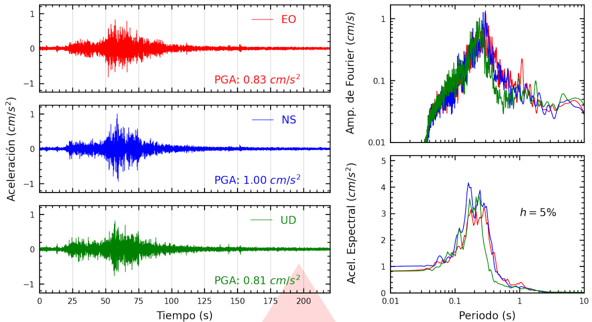
Figura A.7: Registros tiempo-historia, espectros de Fourier y de respuesta en las direcciones EO, NS y vertical de la estación SOVES. Sismo de Ica, Ica - Ica del 2026-04-25, 15:14:40 (Hora local)
