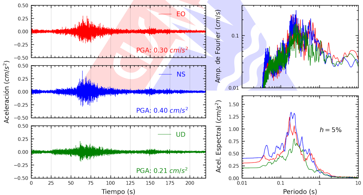
Figura A.18: Registros tiempo-historia, espectros de Fourier y de respuesta en las direcciones EO, NS y vertical de la estación COMAS. Sismo de Ica, Ica - Ica del 2026-04-25, 15:14:40 (Hora local)
