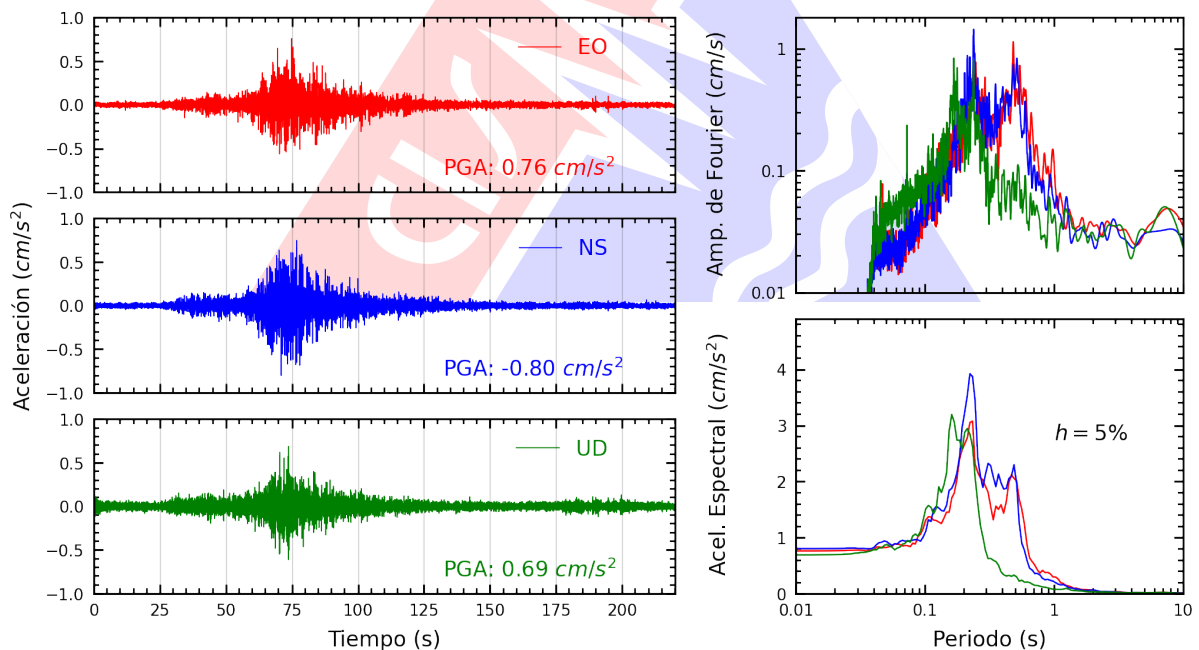
Figura A.10: Registros tiempo-historia, espectros de Fourier y de respuesta en las direcciones EO, NS y vertical de la estación MDPP. Sismo de Ica, Ica - Ica del 2026-04-25, 15:14:40 (Hora local)
