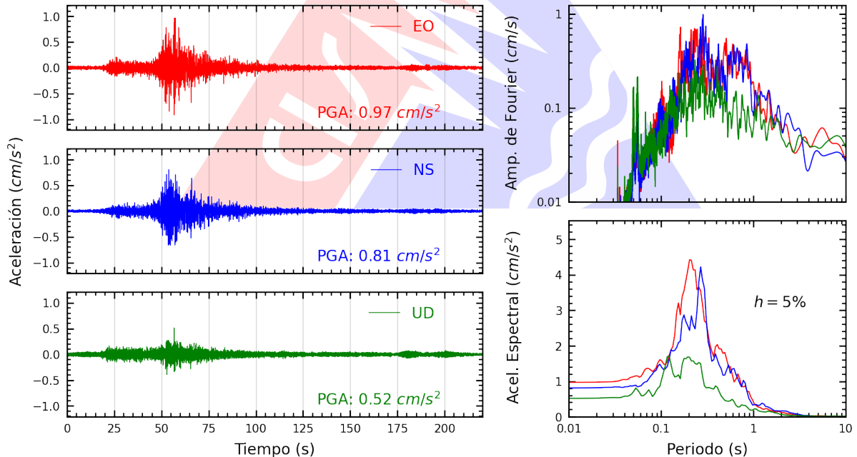
Figura A.8: Registros tiempo-historia, espectros de Fourier y de respuesta en las direcciones EO, NS y vertical de la estación USILP. Sismo de Ica, Ica - Ica del 2026-04-25, 15:14:40 (Hora local)
