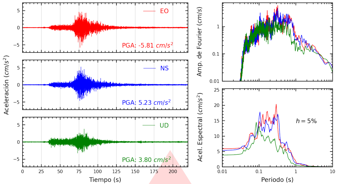
Figura A.27: Registros tiempo-historia, espectros de Fourier y de respuesta en las direcciones EO, NS y vertical de la estación MADRE. Sismo de Ica, Ica - Ica del 2026-05-19, 12:57:51 (Hora local)
