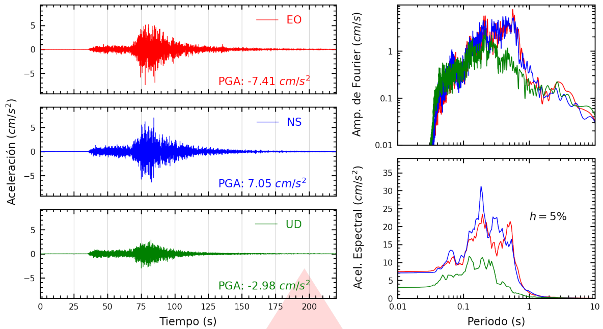
Figura A.23: Registros tiempo-historia, espectros de Fourier y de respuesta en las direcciones EO, NS y vertical de la estación VHAYA. Sismo de Ica, Ica - Ica del 2026-05-19, 12:57:51 (Hora local)
