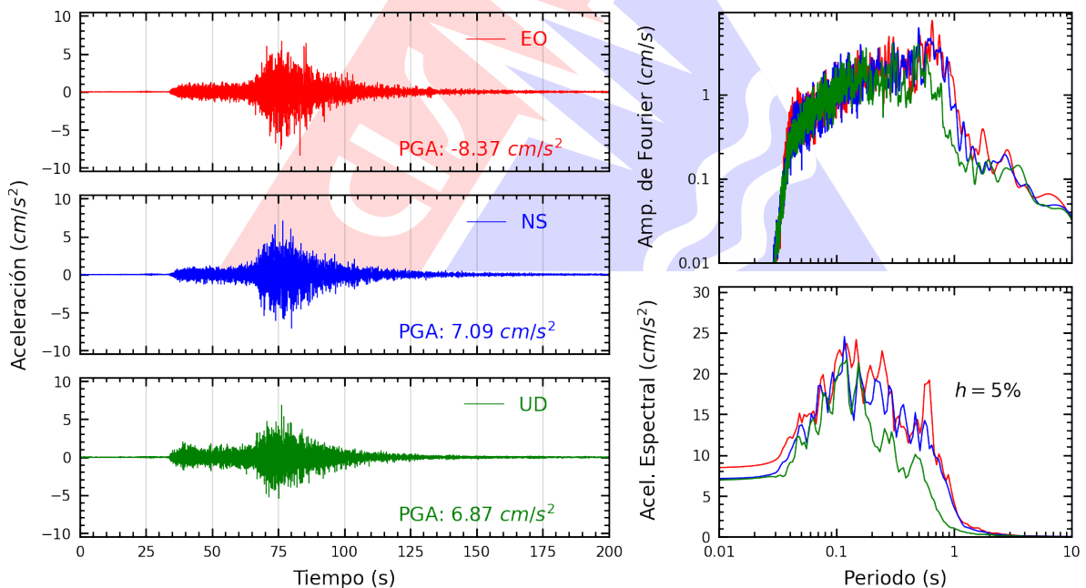
Figura A.22: Registros tiempo-historia, espectros de Fourier y de respuesta en las direcciones EO, NS y vertical de la estación UCVAT. Sismo de Ica, Ica - Ica del 2026-05-19, 12:57:51 (Hora local)
