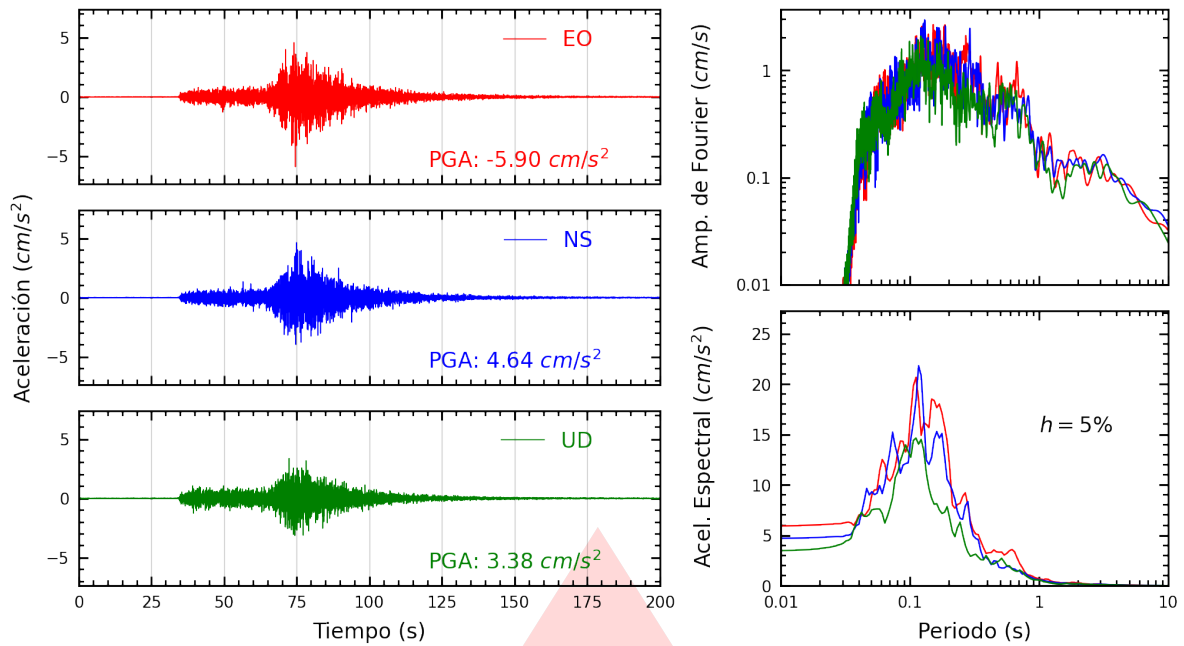
Figura A.25: Registros tiempo-historia, espectros de Fourier y de respuesta en las direcciones EO, NS y vertical de la estación JALVA. Sismo de Ica, Ica - Ica del 2026-05-19, 12:57:51 (Hora local)
