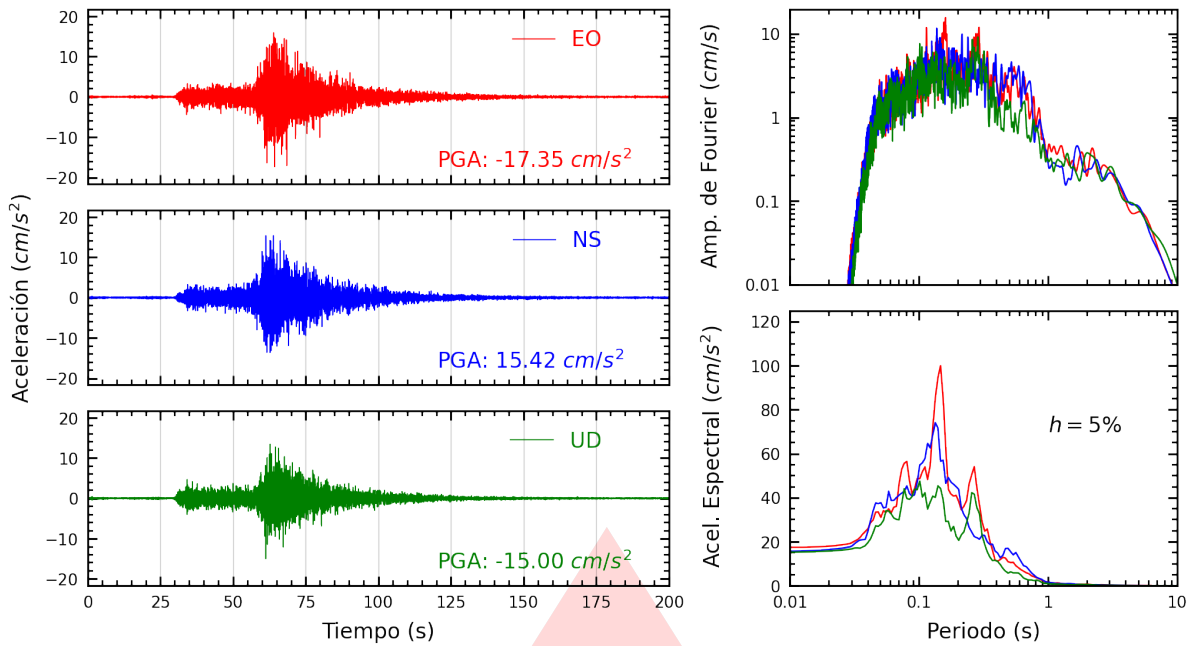
Figura A.5: Registros tiempo-historia, espectros de Fourier y de respuesta en las direcciones EO, NS y vertical de la estación PHERM. Sismo de Ica, Ica - Ica del 2026-05-19, 12:57:51 (Hora local)
