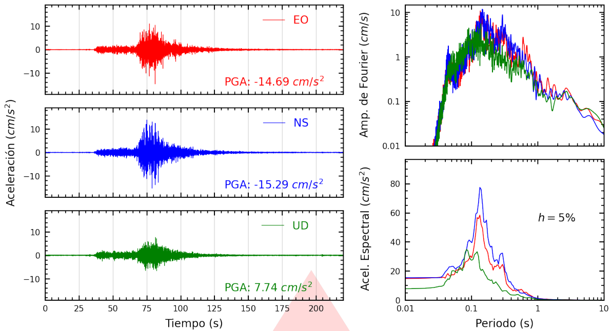
Figura A.7: Registros tiempo-historia, espectros de Fourier y de respuesta en las direcciones EO, NS y vertical de la estación CARAB. Sismo de Ica, Ica - Ica del 2026-05-19, 12:57:51 (Hora local)
