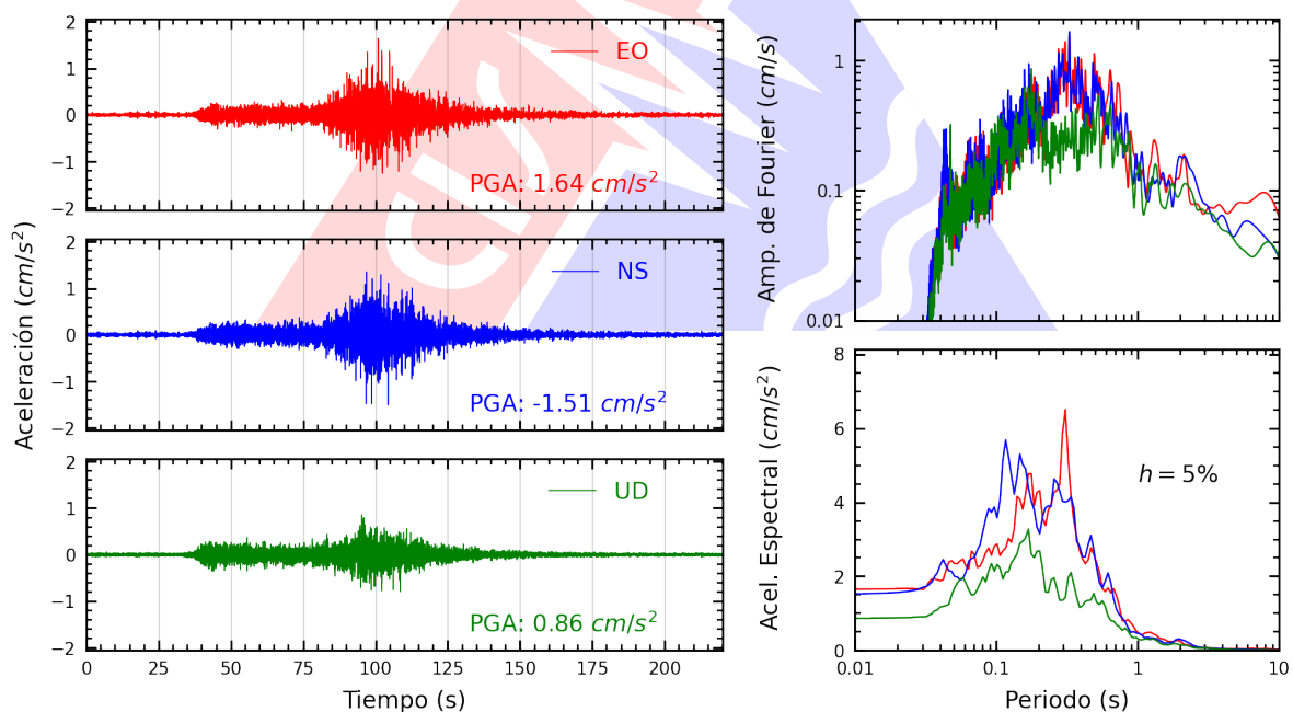
Figura A.44: Registros tiempo-historia, espectros de Fourier y de respuesta en las direcciones EO, NS y vertical de la estación UNAB. Sismo de Ica, Ica - Ica del 2026-05-19, 12:57:51 (Hora local)
