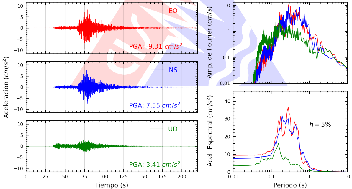
Figura A.18: Registros tiempo-historia, espectros de Fourier y de respuesta en las direcciones EO, NS y vertical de la estación ACAPU. Sismo de Ica, Ica - Ica del 2026-05-19, 12:57:51 (Hora local)
