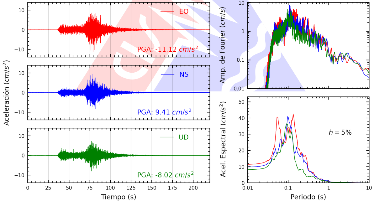
Figura A.16: Registros tiempo-historia, espectros de Fourier y de respuesta en las direcciones EO, NS y vertical de la estación AMORE. Sismo de Ica, Ica - Ica del 2026-05-19, 12:57:51 (Hora local)
