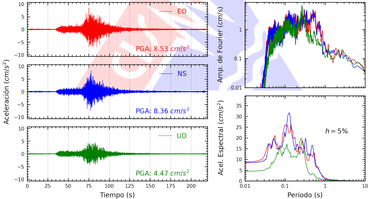
Figura A.20: Registros tiempo-historia, espectros de Fourier y de respuesta en las direcciones EO, NS y vertical de la estación OLIVO. Sismo de Ica, Ica - Ica del 2026-05-19, 12:57:51 (Hora local)
