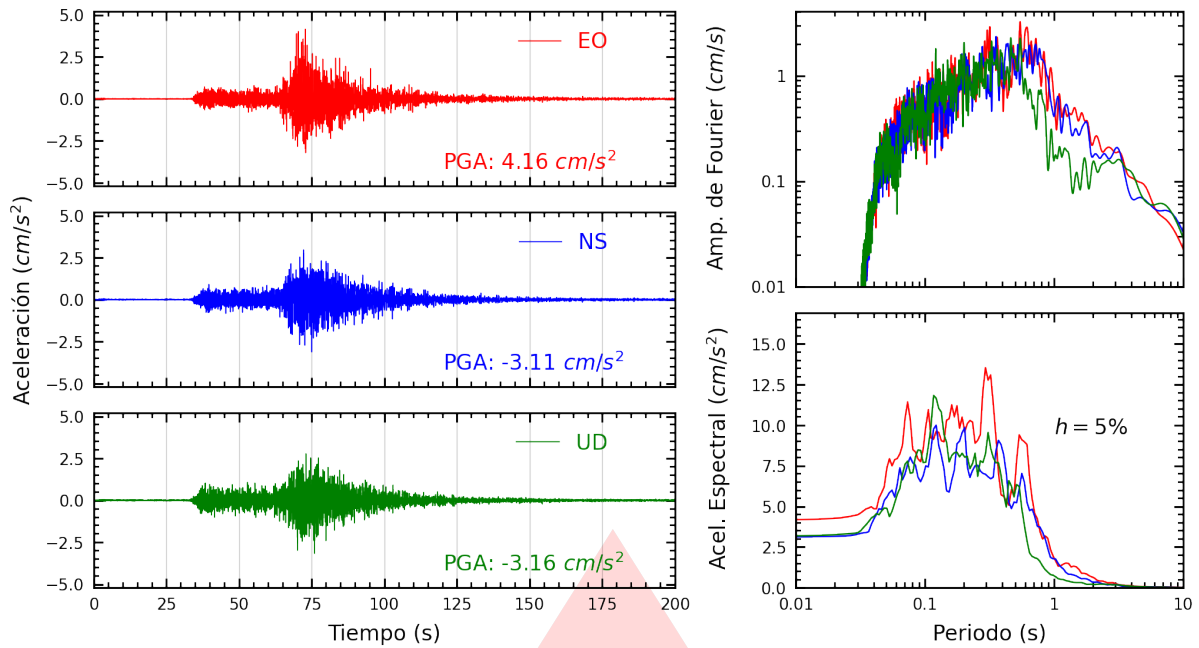
Figura A.37: Registros tiempo-historia, espectros de Fourier y de respuesta en las direcciones EO, NS y vertical de la estación UNFV. Sismo de Ica, Ica - Ica del 2026-05-19, 12:57:51 (Hora local)
