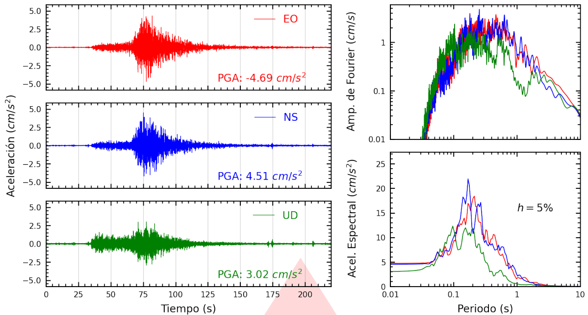
Figura A.35: Registros tiempo-historia, espectros de Fourier y de respuesta en las direcciones EO, NS y vertical de la estación RAMON. Sismo de Ica, Ica - Ica del 2026-05-19, 12:57:51 (Hora local)
