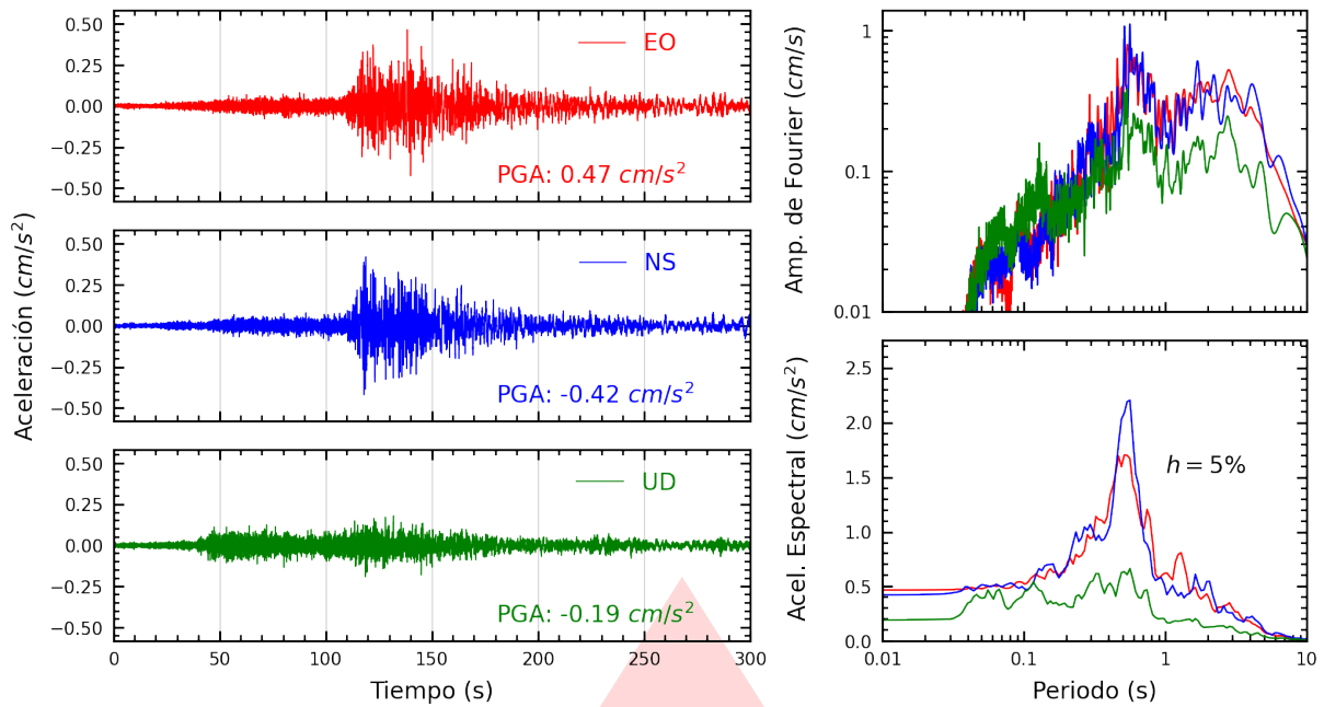
Figura A.51: Registros tiempo-historia, espectros de Fourier y de respuesta en las direcciones EO, NS y vertical de la estación UNIA. Sismo de Ica, Ica - Ica del 2026-05-19, 12:57:51 (Hora local)
