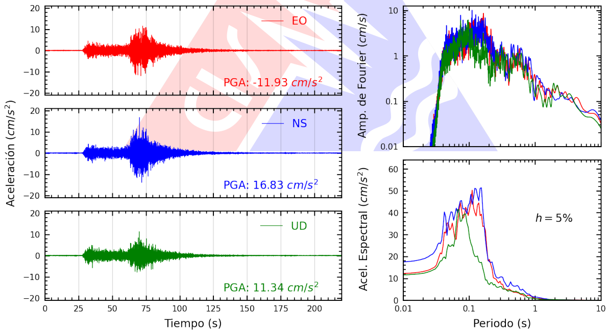
Figura A.6: Registros tiempo-historia, espectros de Fourier y de respuesta en las direcciones EO, NS y vertical de la estación SROSA. Sismo de Ica, Ica - Ica del 2026-05-19, 12:57:51 (Hora local)
