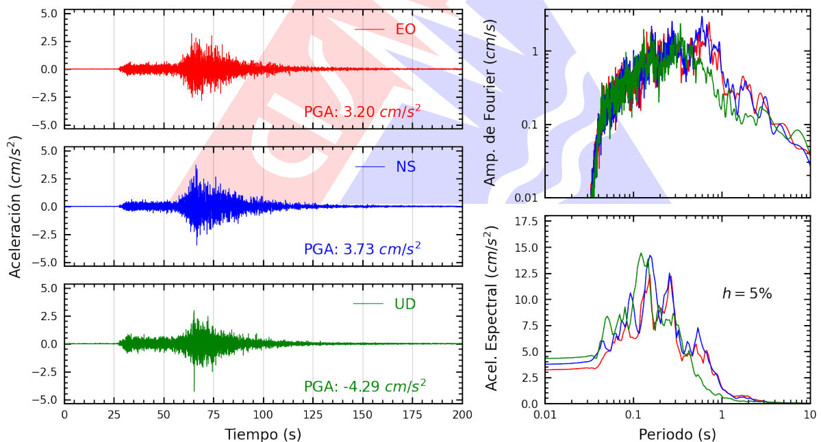
Figura A.36: Registros tiempo-historia, espectros de Fourier y de respuesta en las direcciones EO, NS y vertical de la estación UNMSM. Sismo de Ica, Ica - Ica del 2026-05-19, 12:57:51 (Hora local)
