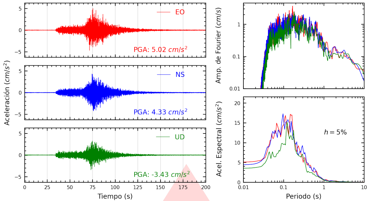
Figura A.33: Registros tiempo-historia, espectros de Fourier y de respuesta en las direcciones EO, NS y vertical de la estación FICPE. Sismo de Ica, Ica - Ica del 2026-05-19, 12:57:51 (Hora local)
