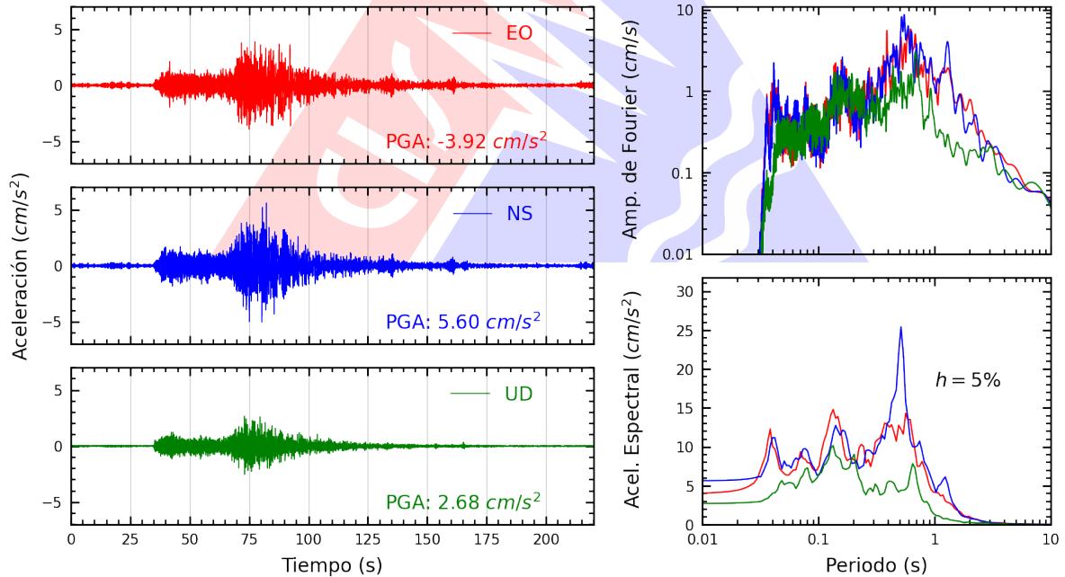
Figura A.28: Registros tiempo-historia, espectros de Fourier y de respuesta en las direcciones EO, NS y vertical de la estación DHNPE. Sismo de Ica, Ica - Ica del 2026-05-19, 12:57:51 (Hora local)
