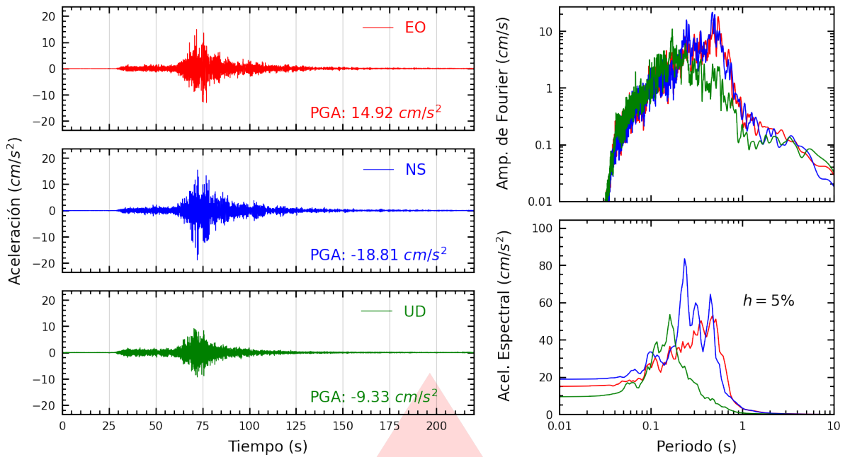
Figura A.3: Registros tiempo-historia, espectros de Fourier y de respuesta en las direcciones EO, NS y vertical de la estación MDPP. Sismo de Ica, Ica - Ica del 2026-05-19, 12:57:51 (Hora local)
