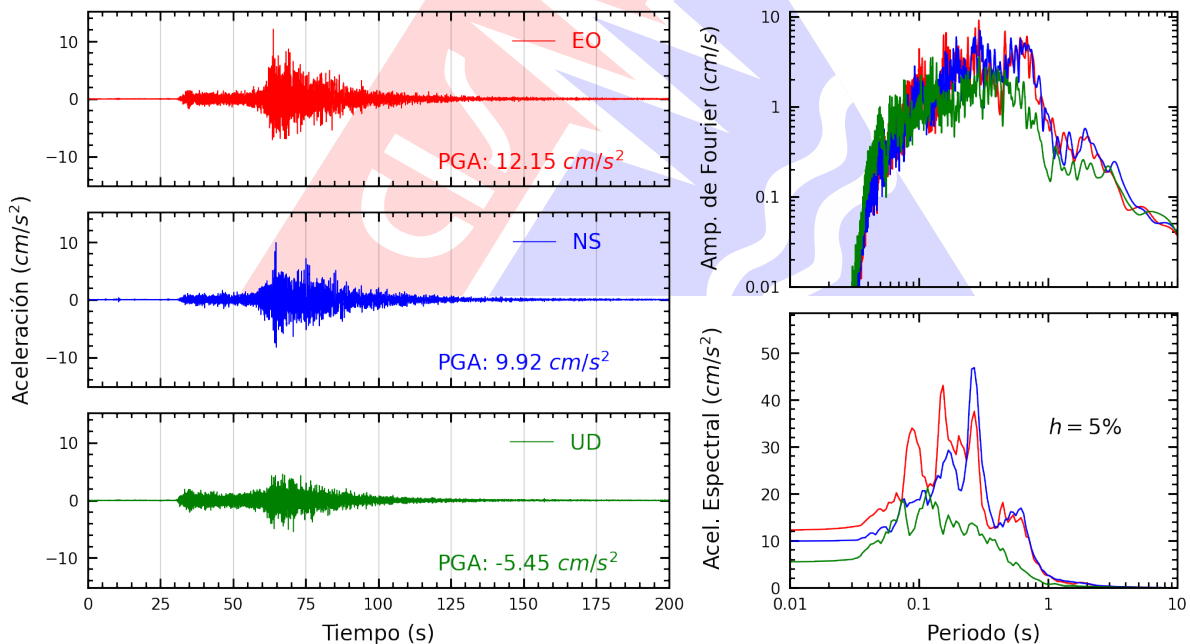
Figura A.12: Registros tiempo-historia, espectros de Fourier y de respuesta en las direcciones EO, NS y vertical de la estación USILP. Sismo de Ica, Ica - Ica del 2026-05-19, 12:57:51 (Hora local)
