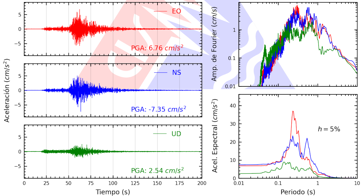
Figura A.24: Registros tiempo-historia, espectros de Fourier y de respuesta en las direcciones EO, NS y vertical de la estación DSMI. Sismo de Ica, Ica - Ica del 2026-05-19, 12:57:51 (Hora local)
