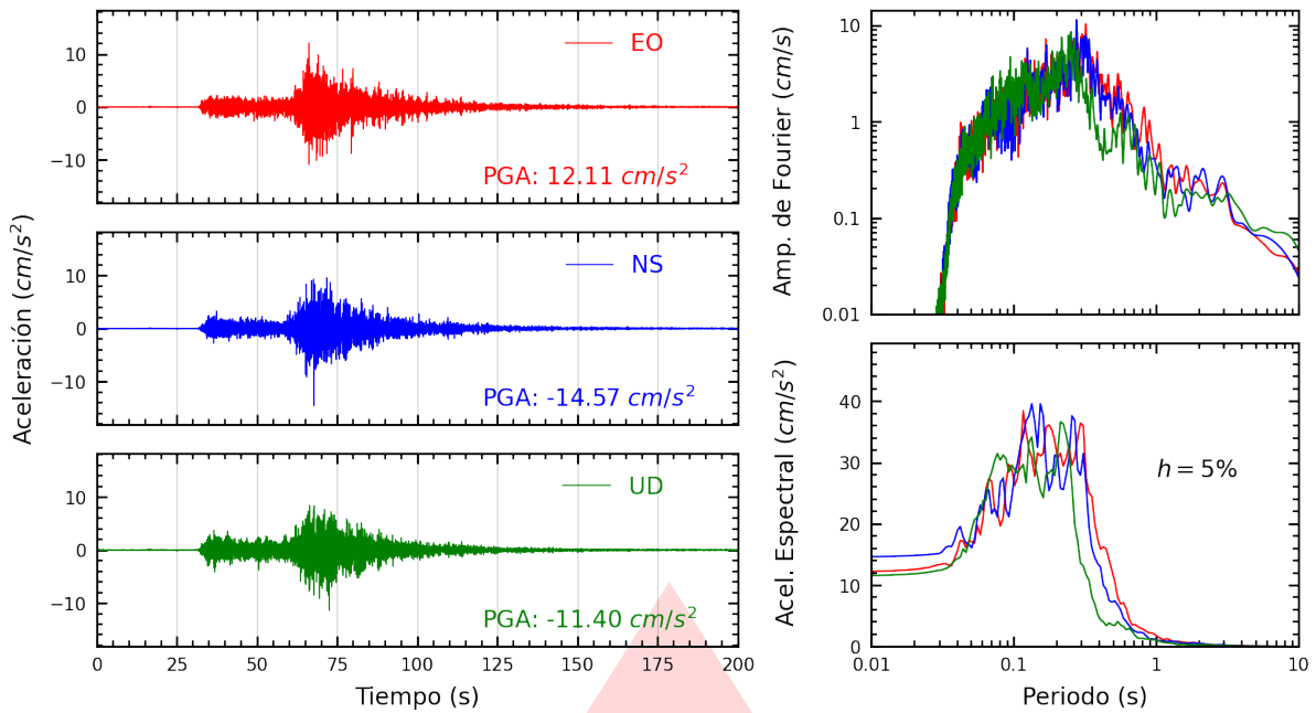
Figura A.9: Registros tiempo-historia, espectros de Fourier y de respuesta en las direcciones EO, NS y vertical de la estación SOVES. Sismo de Ica, Ica - Ica del 2026-05-19, 12:57:51 (Hora local)
