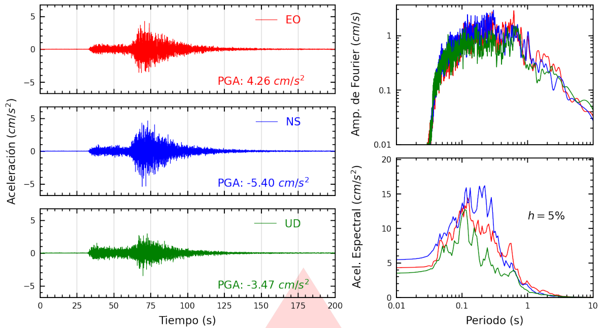
Figura A.31: Registros tiempo-historia, espectros de Fourier y de respuesta en las direcciones EO, NS y vertical de la estación SERVI. Sismo de Ica, Ica - Ica del 2026-05-19, 12:57:51 (Hora local)
