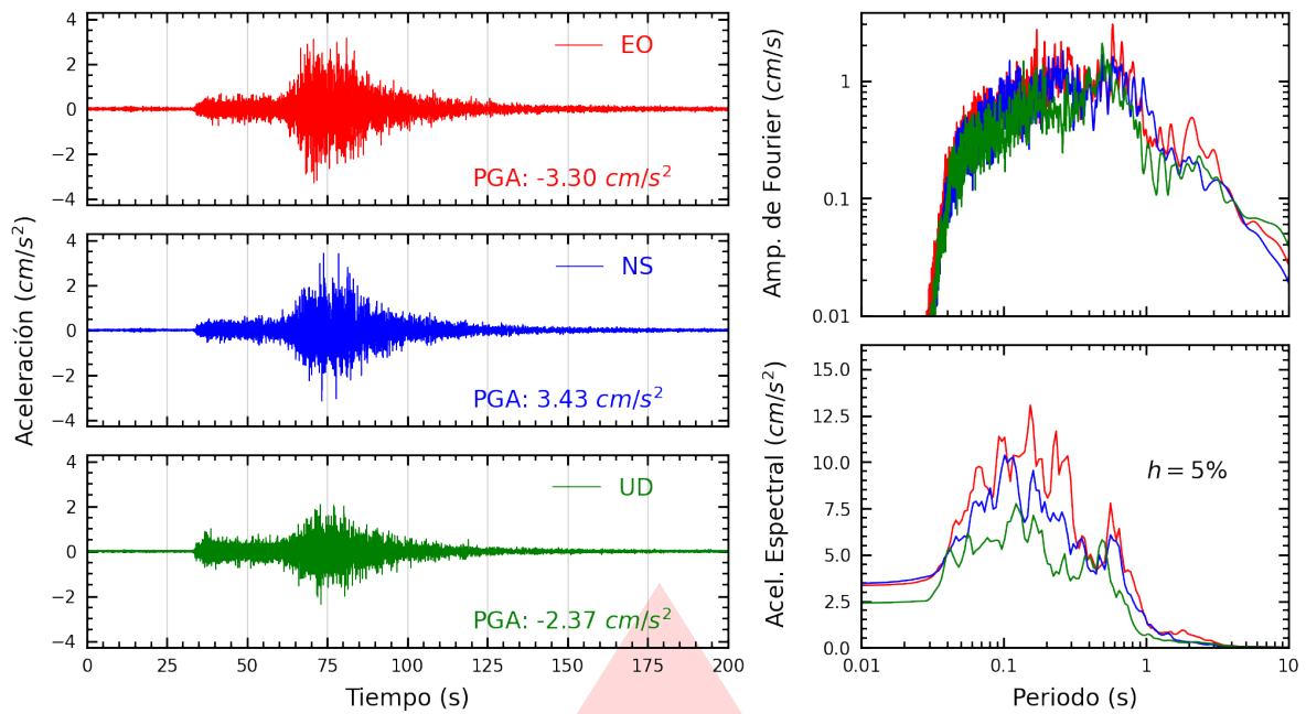
Figura A.41: Registros tiempo-historia, espectros de Fourier y de respuesta en las direcciones EO, NS y vertical de la estación INICT. Sismo de Ica, Ica - Ica del 2026-05-19, 12:57:51 (Hora local)
