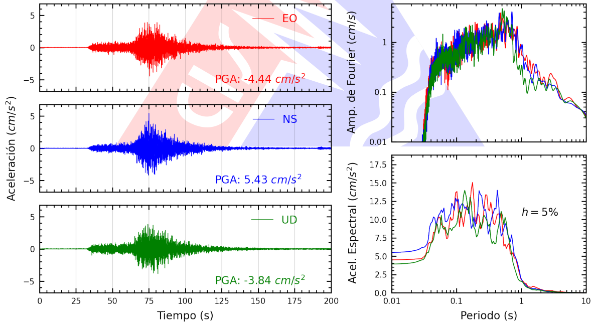
Figura A.30: Registros tiempo-historia, espectros de Fourier y de respuesta en las direcciones EO, NS y vertical de la estación IMCA. Sismo de Ica, Ica - Ica del 2026-05-19, 12:57:51 (Hora local)
