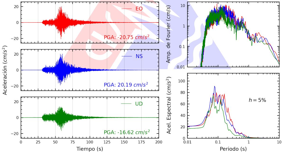
Figura A.2: Registros tiempo-historia, espectros de Fourier y de respuesta en las direcciones EO, NS y vertical de la estación ASIA. Sismo de Ica, Ica - Ica del 2026-05-19, 12:57:51 (Hora local)
