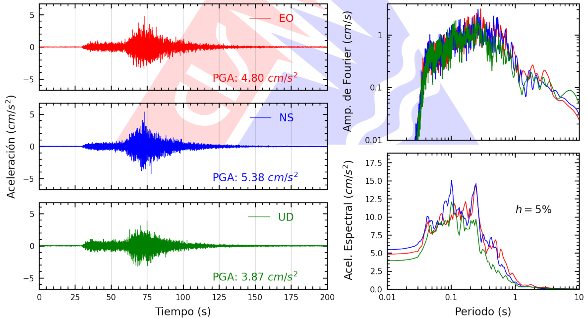
Figura A.32: Registros tiempo-historia, espectros de Fourier y de respuesta en las direcciones EO, NS y vertical de la estación USMP. Sismo de Ica, Ica - Ica del 2026-05-19, 12:57:51 (Hora local)
