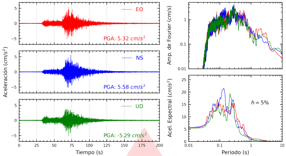
Figura A.29: Registros tiempo-historia, espectros de Fourier y de respuesta en las direcciones EO, NS y vertical de la estación URPE. Sismo de Ica, Ica - Ica del 2026-05-19, 12:57:51 (Hora local)
