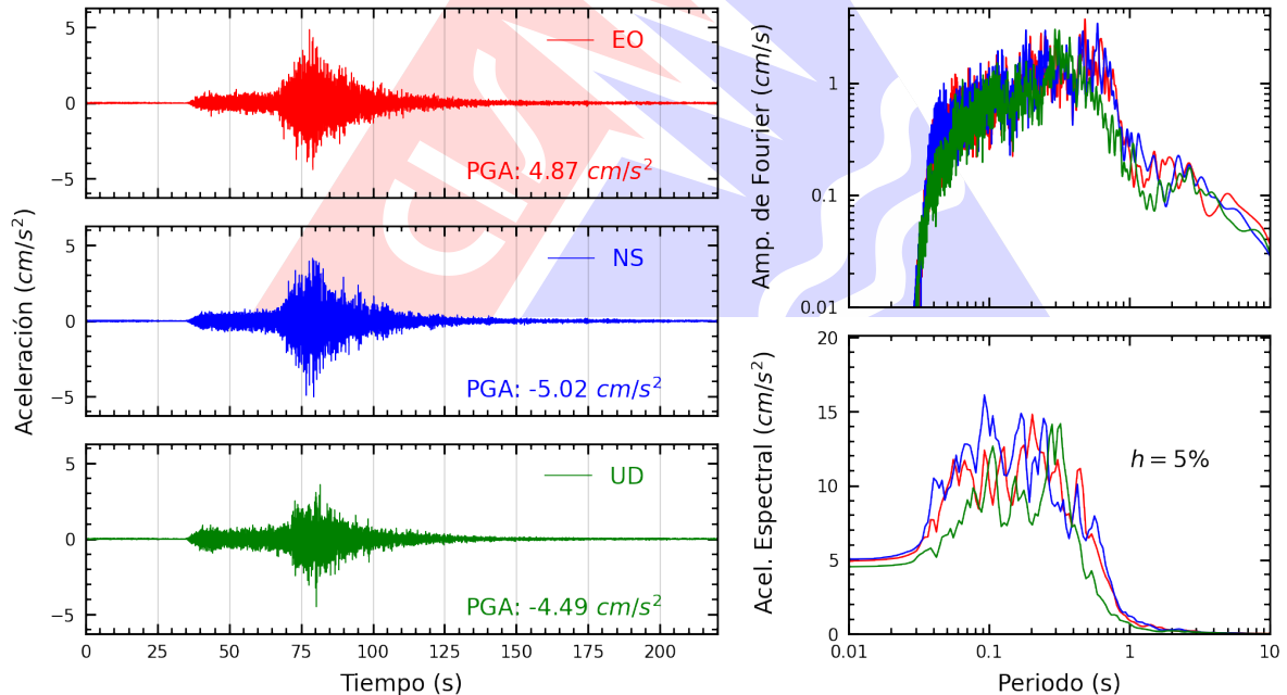
Figura A.34: Registros tiempo-historia, espectros de Fourier y de respuesta en las direcciones EO, NS y vertical de la estación COMAS. Sismo de Ica, Ica - Ica del 2026-05-19, 12:57:51 (Hora local)
