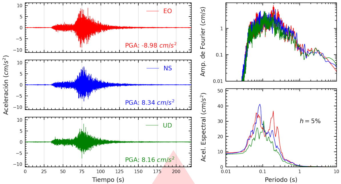
Figura A.19: Registros tiempo-historia, espectros de Fourier y de respuesta en las direcciones EO, NS y vertical de la estación INDEP. Sismo de Ica, Ica - Ica del 2026-05-19, 12:57:51 (Hora local)
