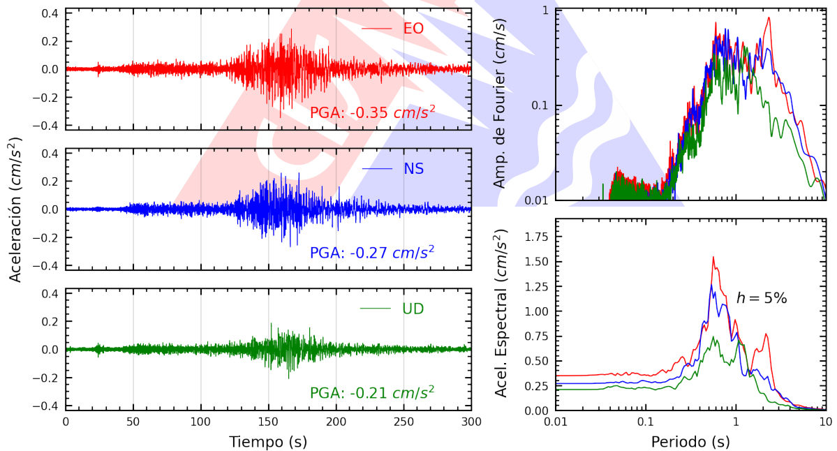
Figura A.52: Registros tiempo-historia, espectros de Fourier y de respuesta en las direcciones EO, NS y vertical de la estación UNC. Sismo de Ica, Ica - Ica del 2026-05-19, 12:57:51 (Hora local)
