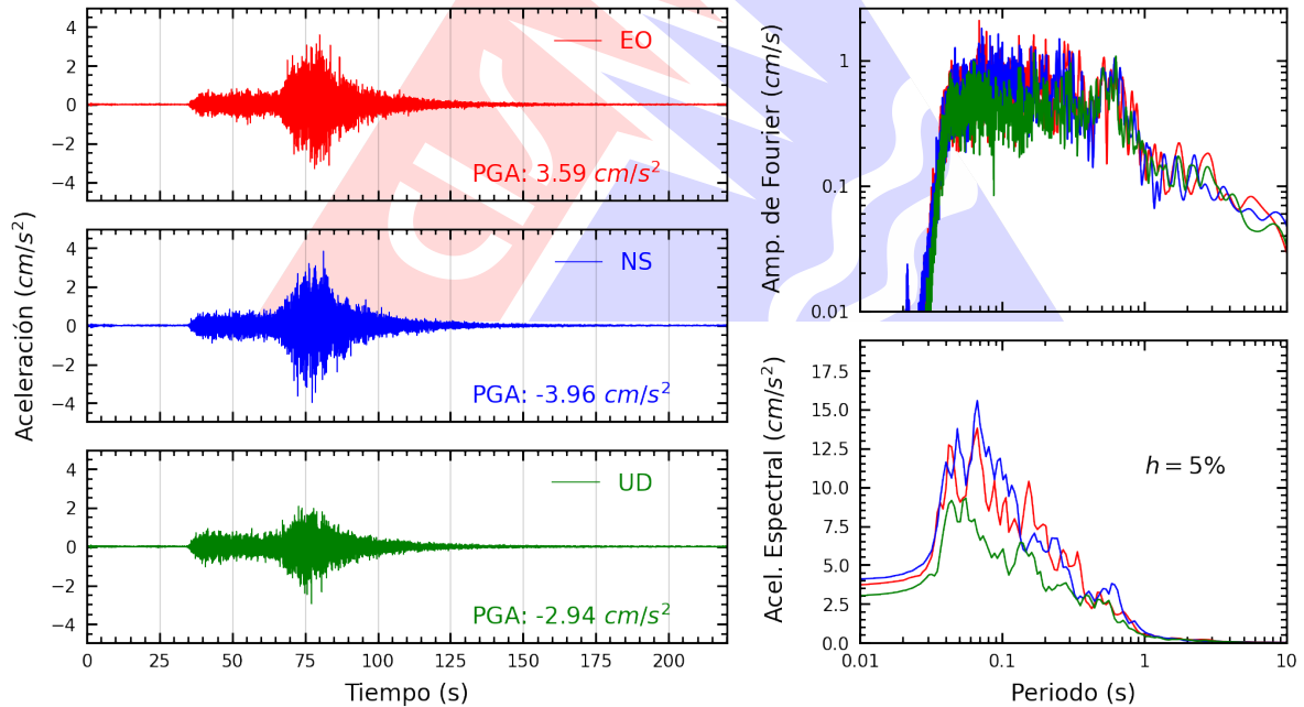
Figura A.38: Registros tiempo-historia, espectros de Fourier y de respuesta en las direcciones EO, NS y vertical de la estación SJLCE. Sismo de Ica, Ica - Ica del 2026-05-19, 12:57:51 (Hora local)
