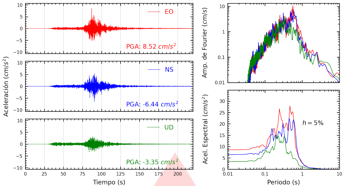
Figura A.21: Registros tiempo-historia, espectros de Fourier y de respuesta en las direcciones EO, NS y vertical de la estación CARAL. Sismo de Ica, Ica - Ica del 2026-05-19, 12:57:51 (Hora local)
