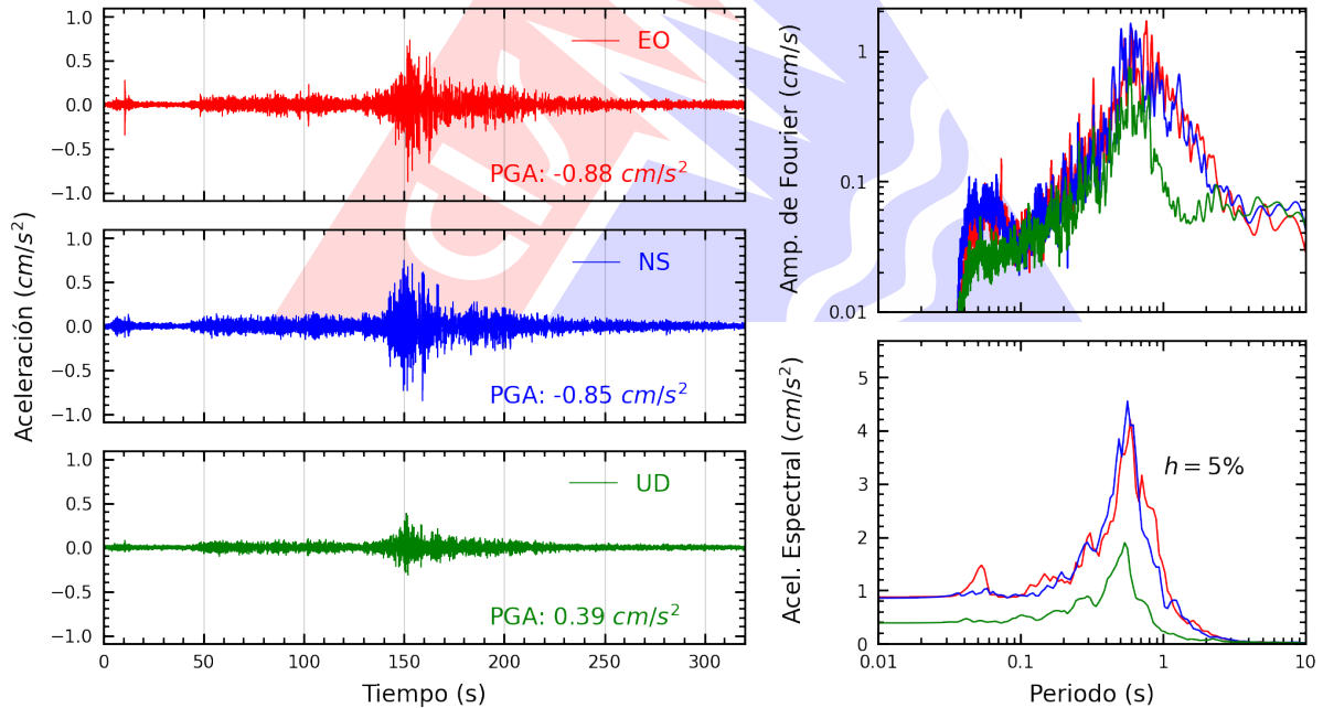
Figura A.46: Registros tiempo-historia, espectros de Fourier y de respuesta en las direcciones EO, NS y vertical de la estación UNTRM. Sismo de Ica, Ica - Ica del 2026-05-19, 12:57:51 (Hora local)
