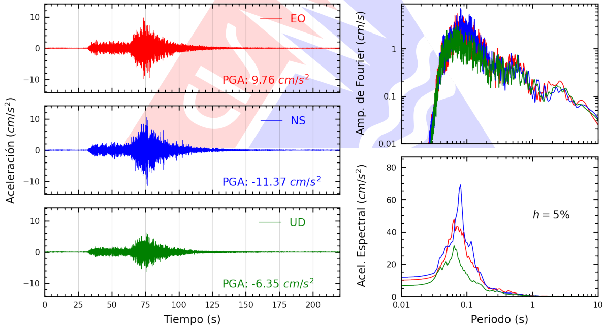
Figura A.14: Registros tiempo-historia, espectros de Fourier y de respuesta en las direcciones EO, NS y vertical de la estación JOSEO. Sismo de Ica, Ica - Ica del 2026-05-19, 12:57:51 (Hora local)
