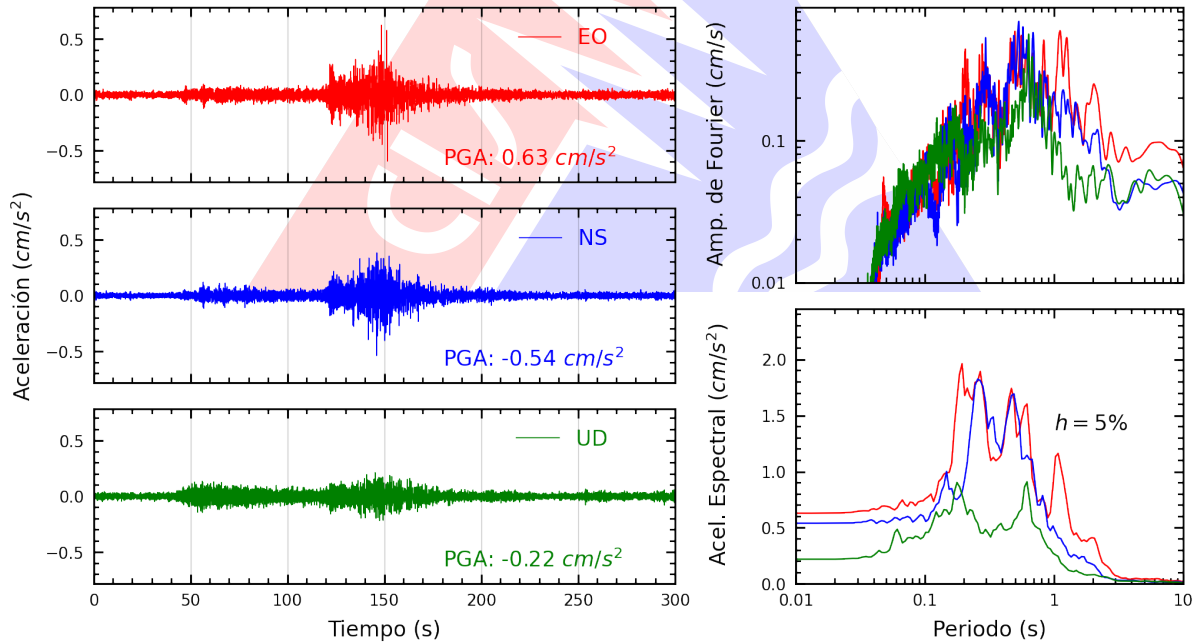
Figura A.48: Registros tiempo-historia, espectros de Fourier y de respuesta en las direcciones EO, NS y vertical de la estación UPAOT. Sismo de Ica, Ica - Ica del 2026-05-19, 12:57:51 (Hora local)
