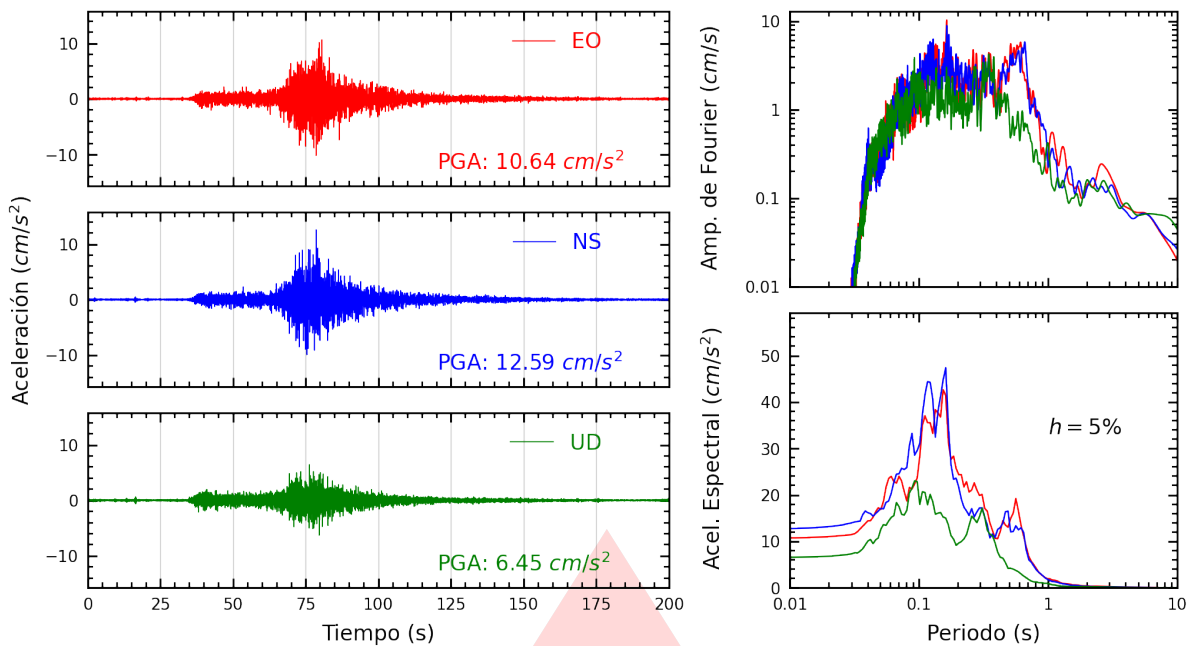
Figura A.11: Registros tiempo-historia, espectros de Fourier y de respuesta en las direcciones EO, NS y vertical de la estación SJLSV. Sismo de Ica, Ica - Ica del 2026-05-19, 12:57:51 (Hora local)
