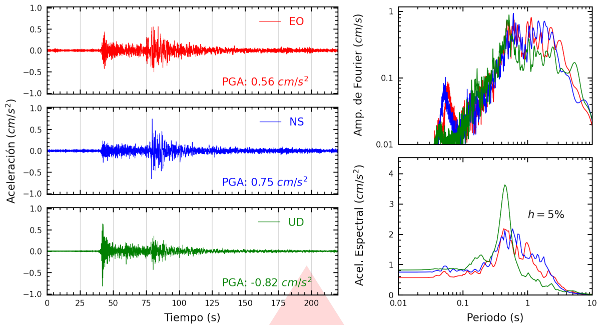
Figura A.47: Registros tiempo-historia, espectros de Fourier y de respuesta en las direcciones EO, NS y vertical de la estación UNMBA. Sismo de Ica, Ica - Ica del 2026-05-19, 12:57:51 (Hora local)
