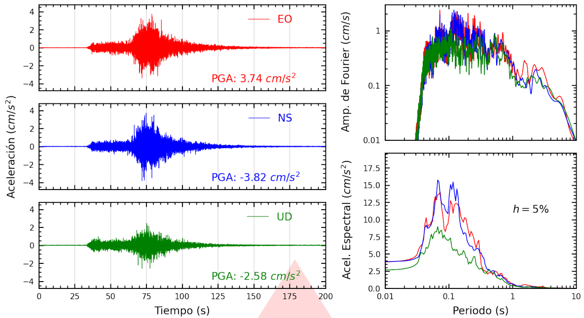
Figura A.39: Registros tiempo-historia, espectros de Fourier y de respuesta en las direcciones EO, NS y vertical de la estación ATARJ. Sismo de Ica, Ica - Ica del 2026-05-19, 12:57:51 (Hora local)
