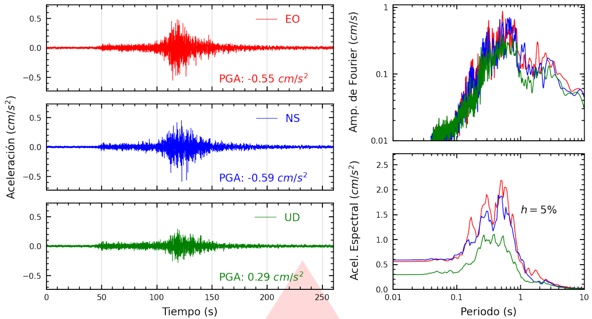
Figura A.49: Registros tiempo-historia, espectros de Fourier y de respuesta en las direcciones EO, NS y vertical de la estación UNASA. Sismo de Ica, Ica - Ica del 2026-05-19, 12:57:51 (Hora local)
