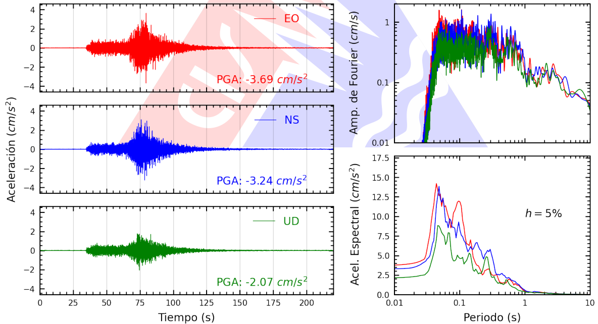
Figura A.40: Registros tiempo-historia, espectros de Fourier y de respuesta en las direcciones EO, NS y vertical de la estación UCSS. Sismo de Ica, Ica - Ica del 2026-05-19, 12:57:51 (Hora local)
