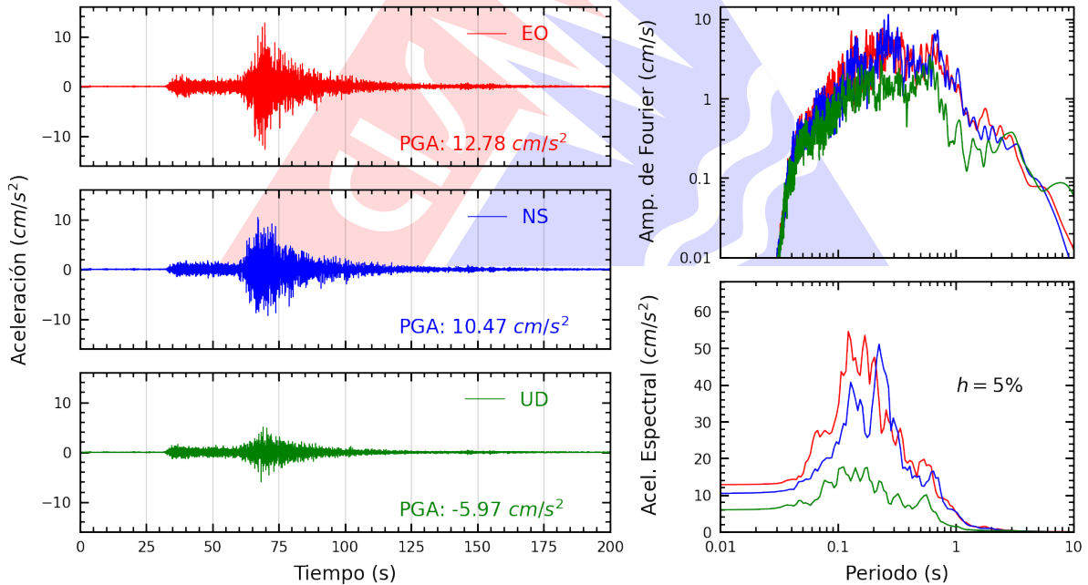
Figura A.10: Registros tiempo-historia, espectros de Fourier y de respuesta en las direcciones EO, NS y vertical de la estación BRISA. Sismo de Ica, Ica - Ica del 2026-05-19, 12:57:51 (Hora local)
