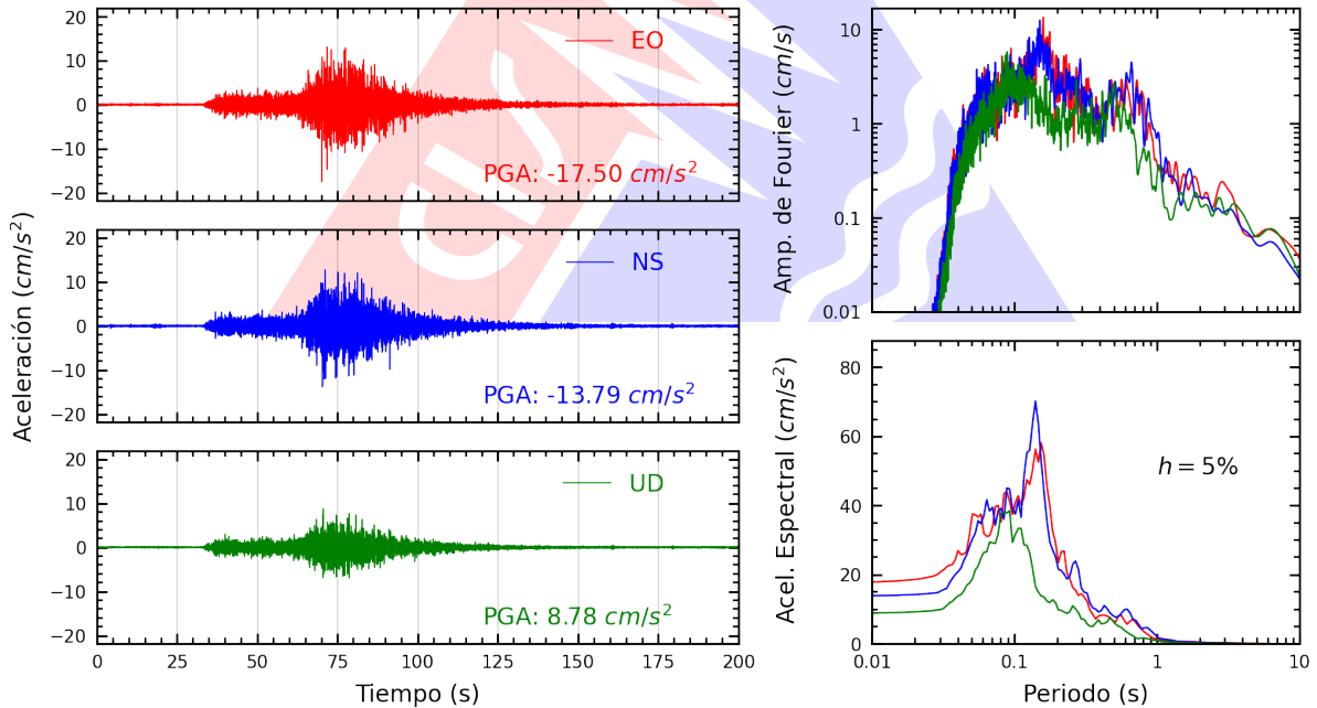
Figura A.4: Registros tiempo-historia, espectros de Fourier y de respuesta en las direcciones EO, NS y vertical de la estación USILM. Sismo de Ica, Ica - Ica del 2026-05-19, 12:57:51 (Hora local)
