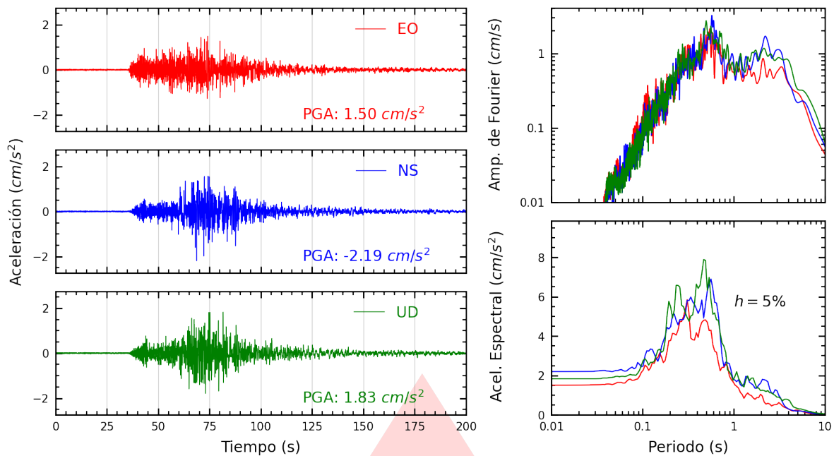
Figura A.43: Registros tiempo-historia, espectros de Fourier y de respuesta en las direcciones EO, NS y vertical de la estación UNSCH. Sismo de Ica, Ica - Ica del 2026-05-19, 12:57:51 (Hora local)
