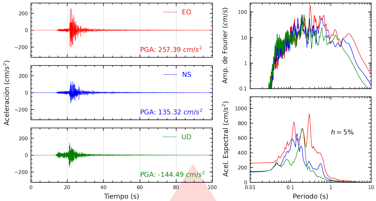
Figura A.1: Registros tiempo-historia, espectros de Fourier y de respuesta en las direcciones EO, NS y vertical de la estación UNICA. Sismo de Ica, Ica - Ica del 2026-05-19, 12:57:51 (Hora local)
