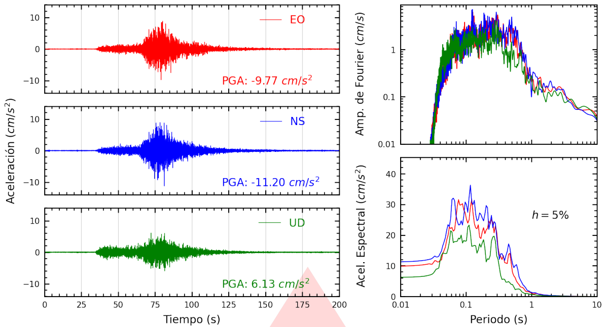
Figura A.15: Registros tiempo-historia, espectros de Fourier y de respuesta en las direcciones EO, NS y vertical de la estación SJLSC. Sismo de Ica, Ica - Ica del 2026-05-19, 12:57:51 (Hora local)
