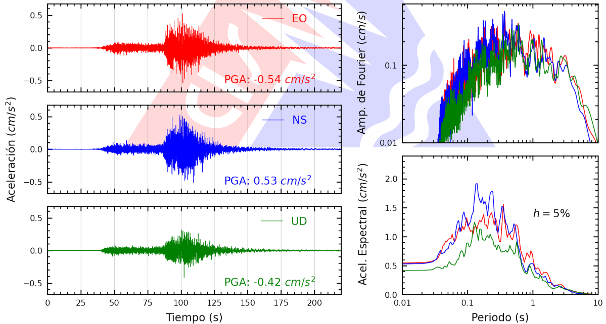
Figura A.50: Registros tiempo-historia, espectros de Fourier y de respuesta en las direcciones EO, NS y vertical de la estación UNSA2. Sismo de Ica, Ica - Ica del 2026-05-19, 12:57:51 (Hora local)
