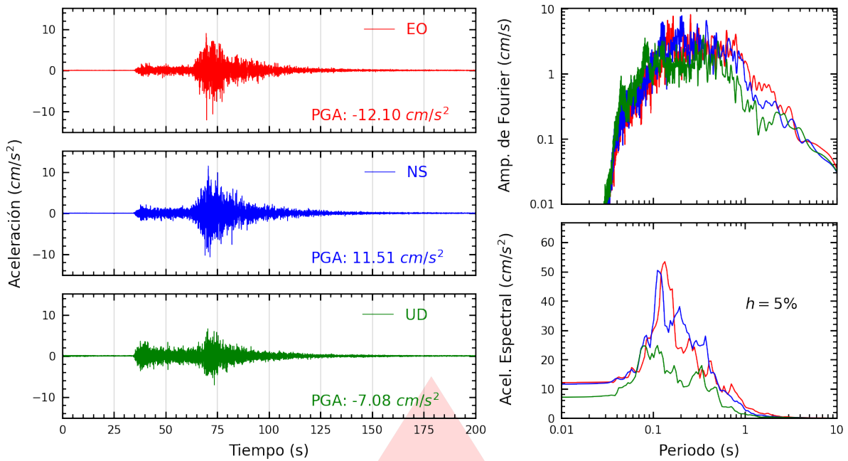
Figura A.13: Registros tiempo-historia, espectros de Fourier y de respuesta en las direcciones EO, NS y vertical de la estación SOCHO. Sismo de Ica, Ica - Ica del 2026-05-19, 12:57:51 (Hora local)
