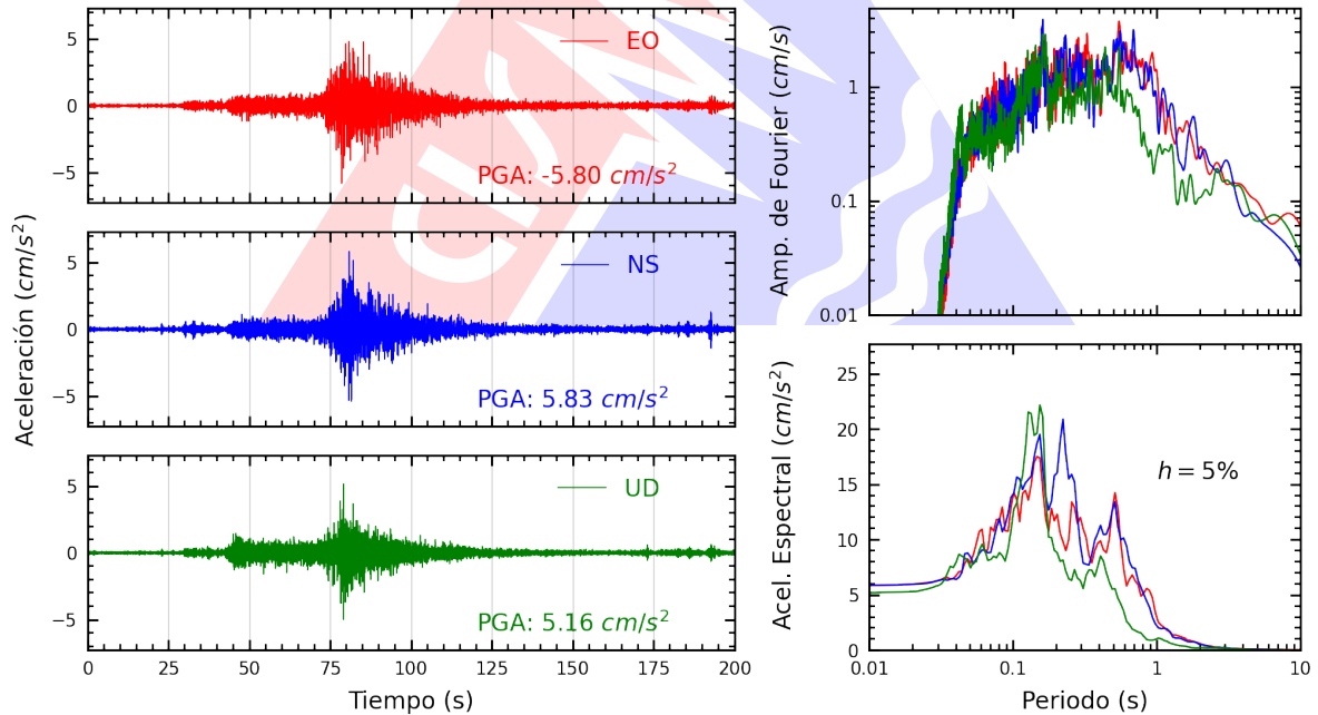
Figura A.26: Registros tiempo-historia, espectros de Fourier y de respuesta en las direcciones EO, NS y vertical de la estación UPCSM. Sismo de Ica, Ica - Ica del 2026-05-19, 12:57:51 (Hora local)
