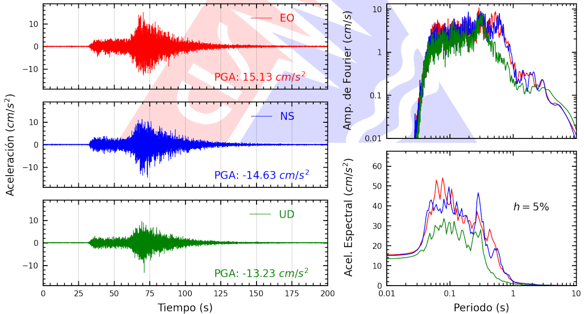
Figura A.8: Registros tiempo-historia, espectros de Fourier y de respuesta en las direcciones EO, NS y vertical de la estación UNTEL. Sismo de Ica, Ica - Ica del 2026-05-19, 12:57:51 (Hora local)
