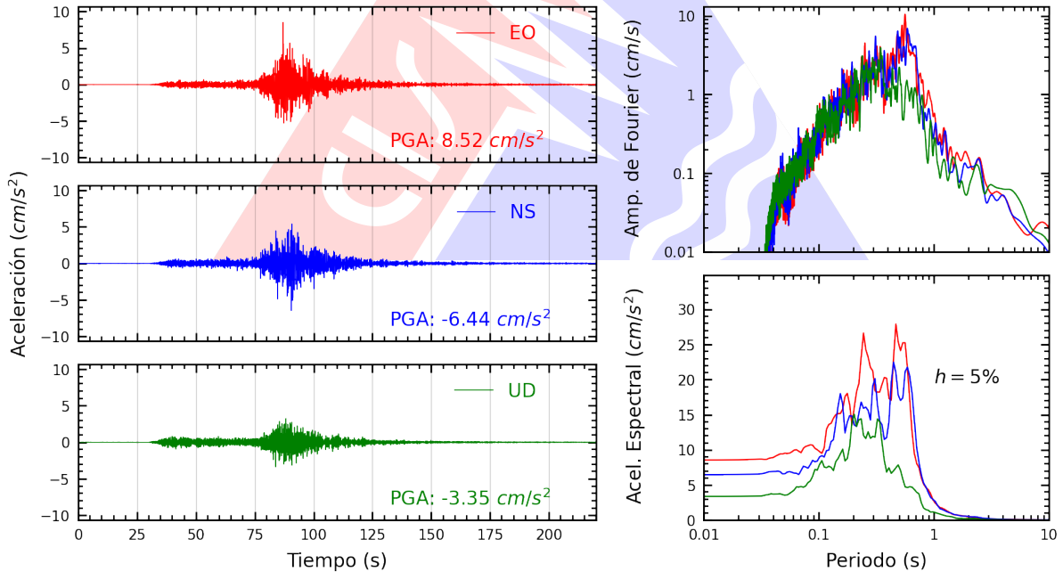
Figura A.20: Registros tiempo-historia, espectros de Fourier y de respuesta en las direcciones EO, NS y vertical de la estación CARAL. Sismo de Ica, Ica - Ica del 2026-05-19, 12:57:51 (Hora local)
