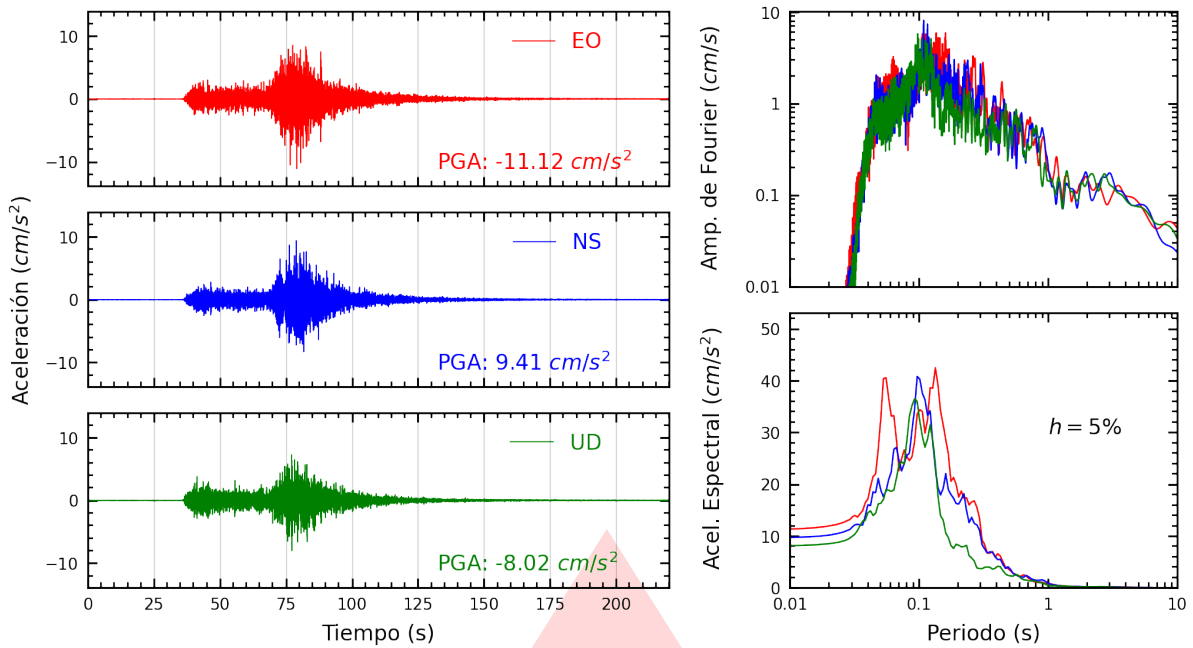
Figura A.15: Registros tiempo-historia, espectros de Fourier y de respuesta en las direcciones EO, NS y vertical de la estación AMORE. Sismo de Ica, Ica - Ica del 2026-05-19, 12:57:51 (Hora local)
