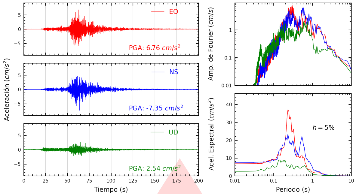
Figura A.23: Registros tiempo-historia, espectros de Fourier y de respuesta en las direcciones EO, NS y vertical de la estación DSMI. Sismo de Ica, Ica - Ica del 2026-05-19, 12:57:51 (Hora local)
