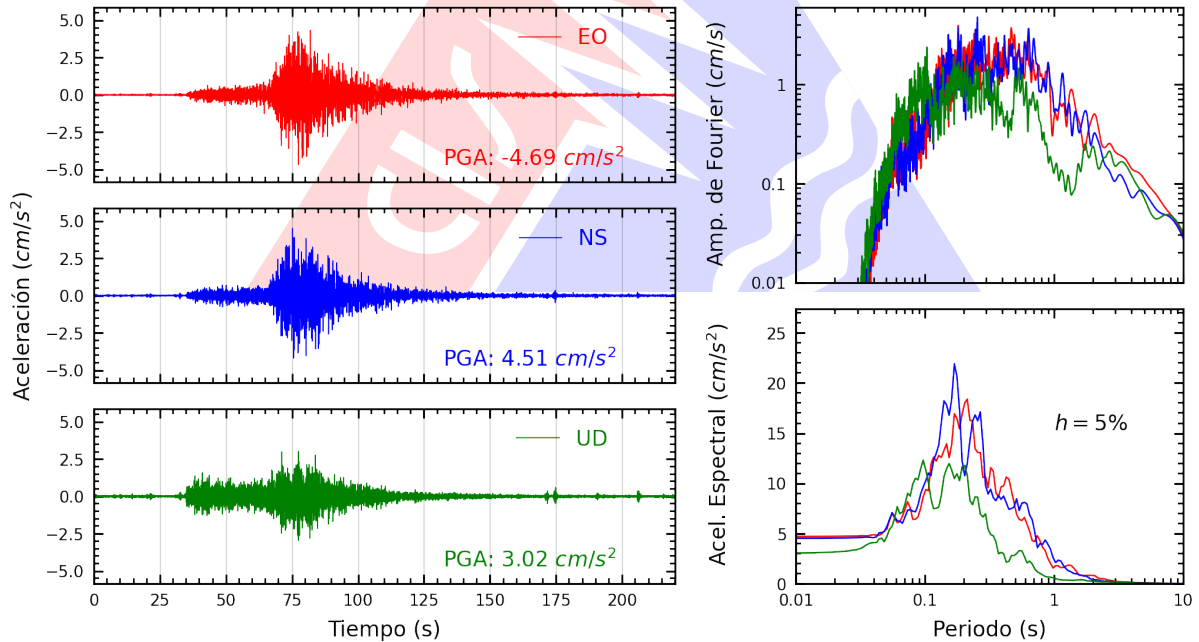
Figura A.34: Registros tiempo-historia, espectros de Fourier y de respuesta en las direcciones EO, NS y vertical de la estación RAMON. Sismo de Ica, Ica - Ica del 2026-05-19, 12:57:51 (Hora local)
