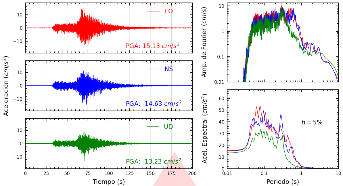
Figura A.7: Registros tiempo-historia, espectros de Fourier y de respuesta en las direcciones EO, NS y vertical de la estación UNTEL. Sismo de Ica, Ica - Ica del 2026-05-19, 12:57:51 (Hora local)
