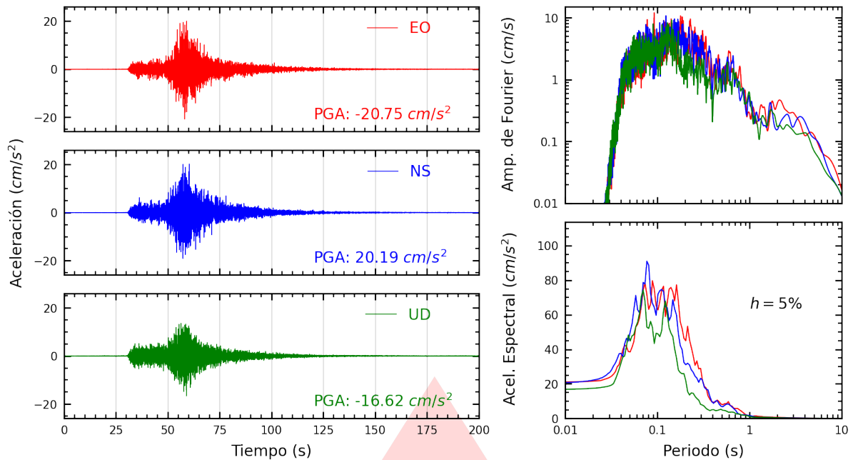
Figura A.1: Registros tiempo-historia, espectros de Fourier y de respuesta en las direcciones EO, NS y vertical de la estación ASIA. Sismo de Ica, Ica - Ica del 2026-05-19, 12:57:51 (Hora local)
