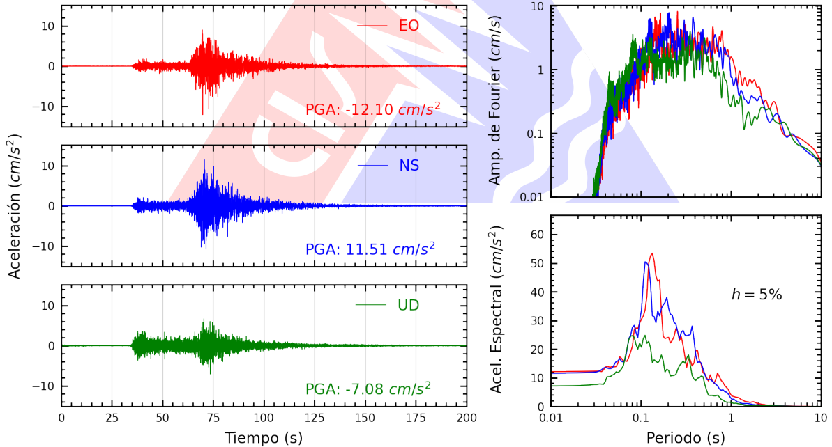
Figura A.12: Registros tiempo-historia, espectros de Fourier y de respuesta en las direcciones EO, NS y vertical de la estación SOCHO. Sismo de Ica, Ica - Ica del 2026-05-19, 12:57:51 (Hora local)
