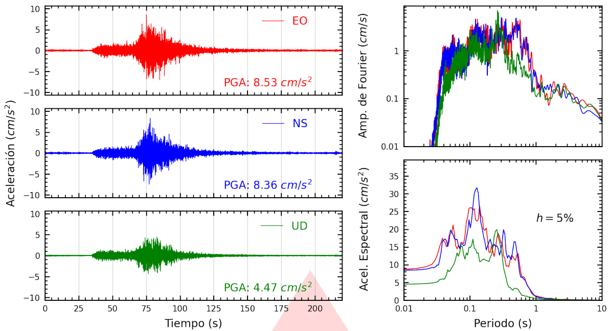
Figura A.19: Registros tiempo-historia, espectros de Fourier y de respuesta en las direcciones EO, NS y vertical de la estación OLIVO. Sismo de Ica, Ica - Ica del 2026-05-19, 12:57:51 (Hora local)
