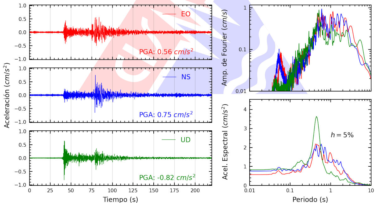
Figura A.46: Registros tiempo-historia, espectros de Fourier y de respuesta en las direcciones EO, NS y vertical de la estación UNMBA. Sismo de Ica, Ica - Ica del 2026-05-19, 12:57:51 (Hora local)
