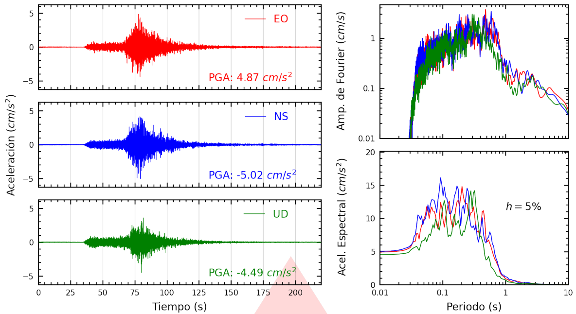
Figura A.33: Registros tiempo-historia, espectros de Fourier y de respuesta en las direcciones EO, NS y vertical de la estación COMAS. Sismo de Ica, Ica - Ica del 2026-05-19, 12:57:51 (Hora local)
