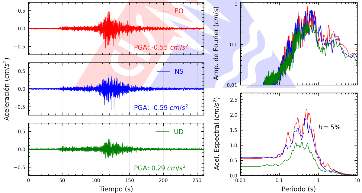
Figura A.48: Registros tiempo-historia, espectros de Fourier y de respuesta en las direcciones EO, NS y vertical de la estación UNASA. Sismo de Ica, Ica - Ica del 2026-05-19, 12:57:51 (Hora local)
