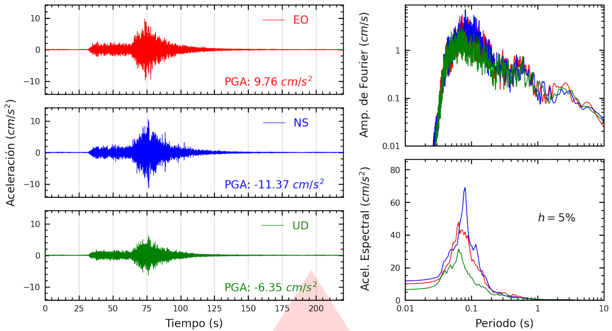
Figura A.13: Registros tiempo-historia, espectros de Fourier y de respuesta en las direcciones EO, NS y vertical de la estación JOSEO. Sismo de Ica, Ica - Ica del 2026-05-19, 12:57:51 (Hora local)
