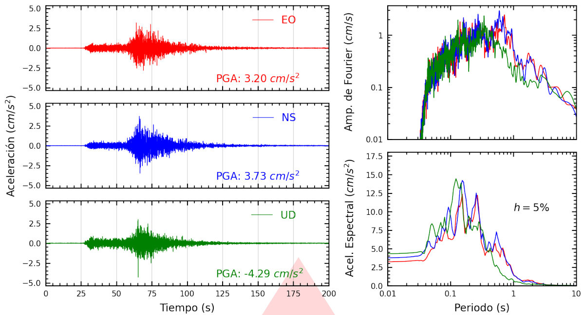
Figura A.35: Registros tiempo-historia, espectros de Fourier y de respuesta en las direcciones EO, NS y vertical de la estación UNMSM. Sismo de Ica, Ica - Ica del 2026-05-19, 12:57:51 (Hora local)
