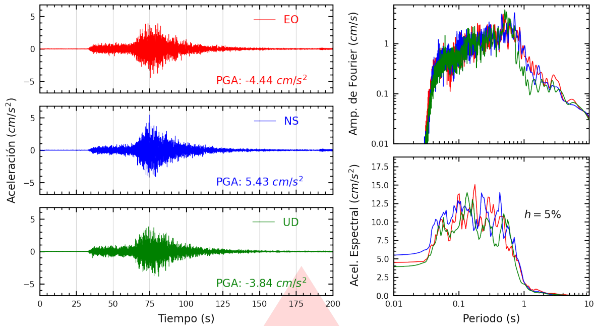
Figura A.29: Registros tiempo-historia, espectros de Fourier y de respuesta en las direcciones EO, NS y vertical de la estación IMCA. Sismo de Ica, Ica - Ica del 2026-05-19, 12:57:51 (Hora local)
