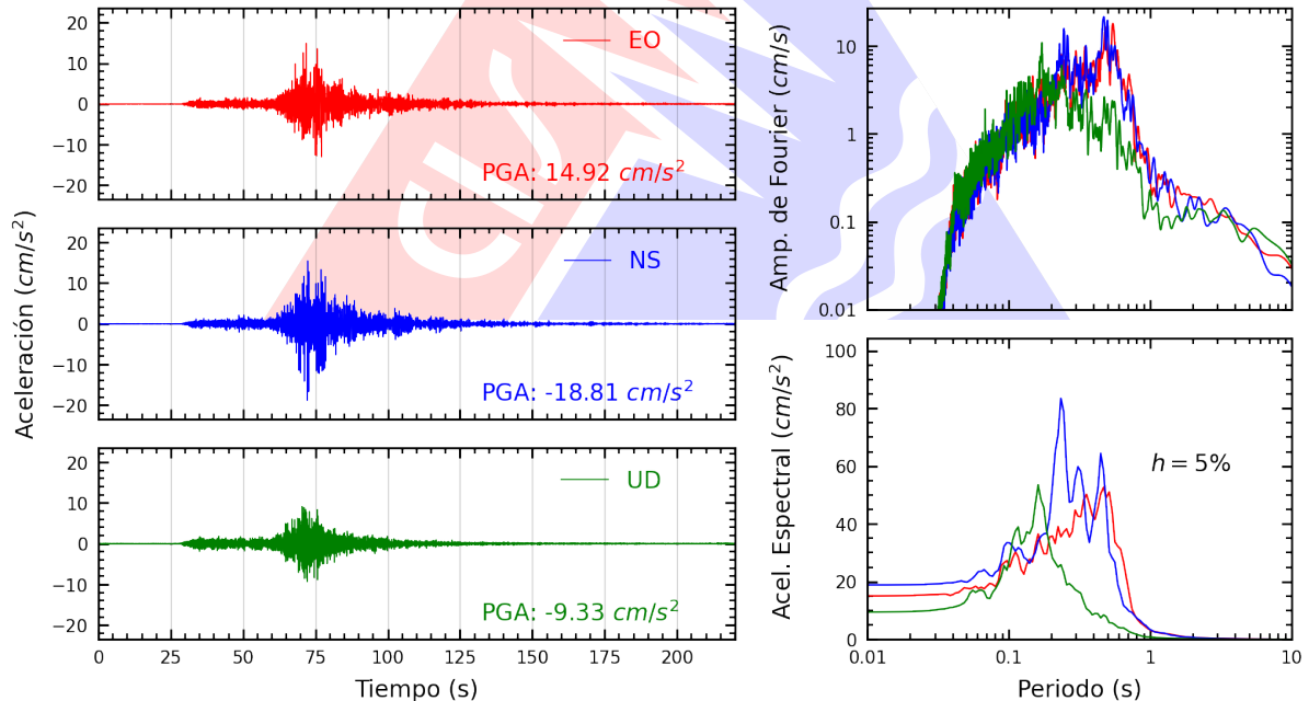
Figura A.2: Registros tiempo-historia, espectros de Fourier y de respuesta en las direcciones EO, NS y vertical de la estación MDPP. Sismo de Ica, Ica - Ica del 2026-05-19, 12:57:51 (Hora local)
