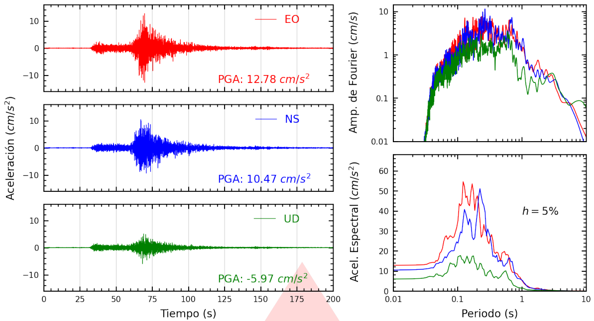
Figura A.9: Registros tiempo-historia, espectros de Fourier y de respuesta en las direcciones EO, NS y vertical de la estación BRISA. Sismo de Ica, Ica - Ica del 2026-05-19, 12:57:51 (Hora local)
