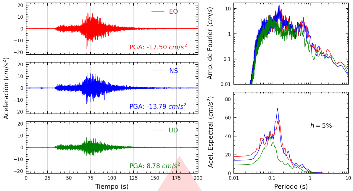
Figura A.3: Registros tiempo-historia, espectros de Fourier y de respuesta en las direcciones EO, NS y vertical de la estación USILM. Sismo de Ica, Ica - Ica del 2026-05-19, 12:57:51 (Hora local)
