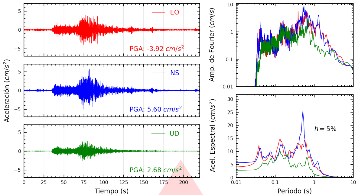
Figura A.27: Registros tiempo-historia, espectros de Fourier y de respuesta en las direcciones EO, NS y vertical de la estación DHPNE. Sismo de Ica, Ica - Ica del 2026-05-19, 12:57:51 (Hora local)
