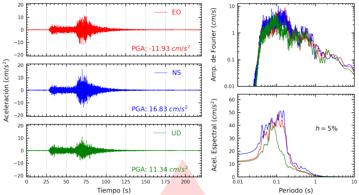
Figura A.5: Registros tiempo-historia, espectros de Fourier y de respuesta en las direcciones EO, NS y vertical de la estación SROSA. Sismo de Ica, Ica - Ica del 2026-05-19, 12:57:51 (Hora local)
