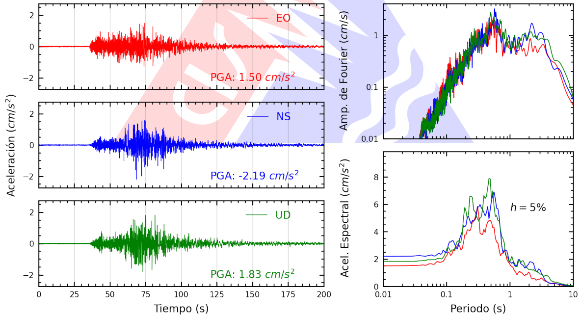
Figura A.42: Registros tiempo-historia, espectros de Fourier y de respuesta en las direcciones EO, NS y vertical de la estación UNSCH. Sismo de Ica, Ica - Ica del 2026-05-19, 12:57:51 (Hora local)
