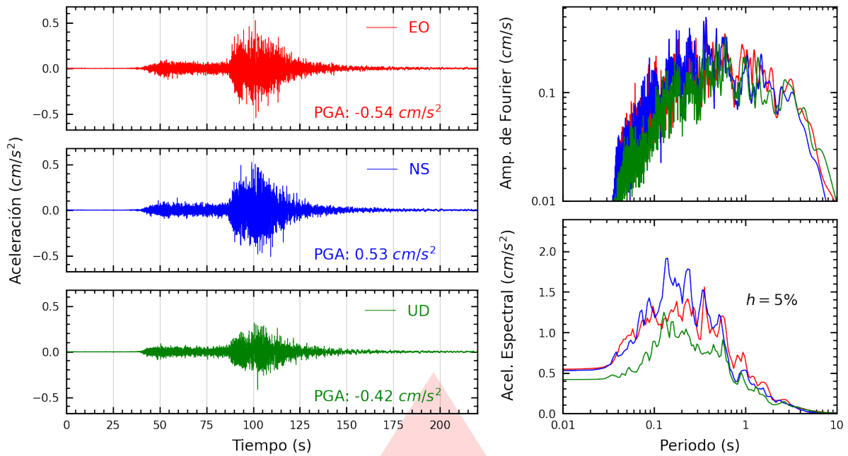
Figura A.49: Registros tiempo-historia, espectros de Fourier y de respuesta en las direcciones EO, NS y vertical de la estación UNSA2. Sismo de Ica, Ica - Ica del 2026-05-19, 12:57:51 (Hora local)
