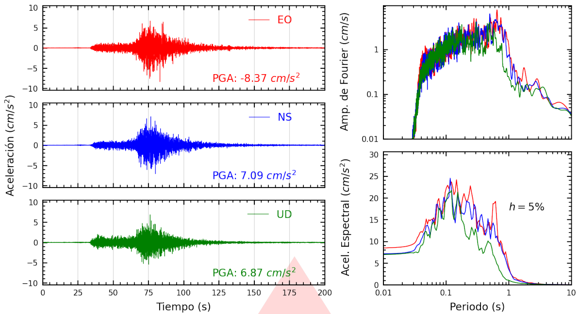
Figura A.21: Registros tiempo-historia, espectros de Fourier y de respuesta en las direcciones EO, NS y vertical de la estación UCVAT. Sismo de Ica, Ica - Ica del 2026-05-19, 12:57:51 (Hora local)
