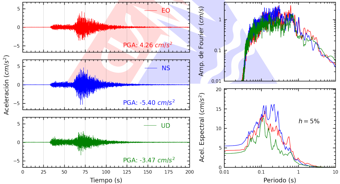
Figura A.30: Registros tiempo-historia, espectros de Fourier y de respuesta en las direcciones EO, NS y vertical de la estación SERVI. Sismo de Ica, Ica - Ica del 2026-05-19, 12:57:51 (Hora local)
