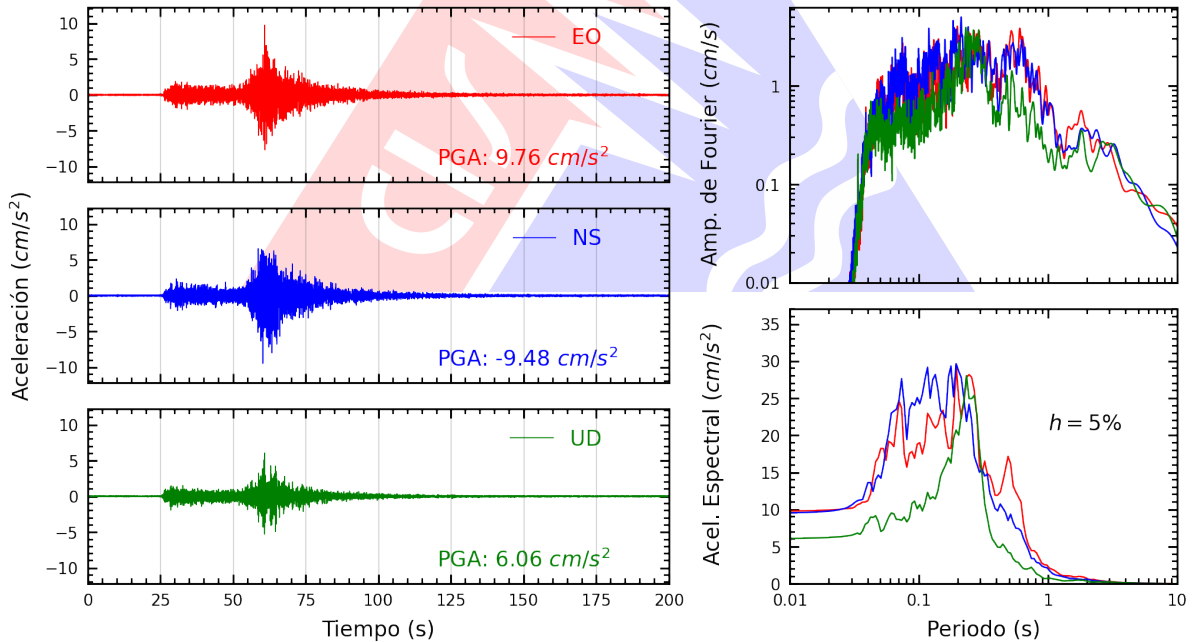
Figura A.16: Registros tiempo-historia, espectros de Fourier y de respuesta en las direcciones EO, NS y vertical de la estación UPCVI. Sismo de Ica, Ica - Ica del 2026-05-19, 12:57:51 (Hora local)
