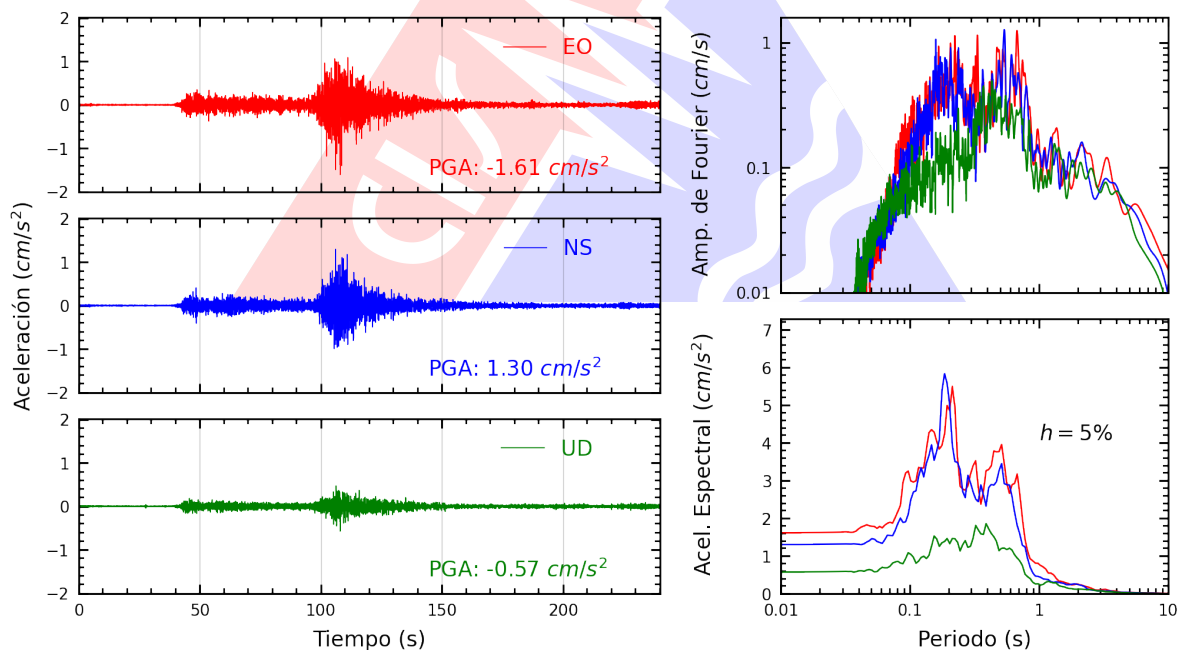
Figura A.44: Registros tiempo-historia, espectros de Fourier y de respuesta en las direcciones EO, NS y vertical de la estación UNAS. Sismo de Ica, Ica - Ica del 2026-05-19, 12:57:51 (Hora local)
