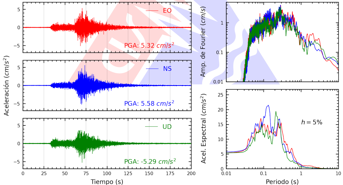
Figura A.28: Registros tiempo-historia, espectros de Fourier y de respuesta en las direcciones EO, NS y vertical de la estación URPE. Sismo de Ica, Ica - Ica del 2026-05-19, 12:57:51 (Hora local)
