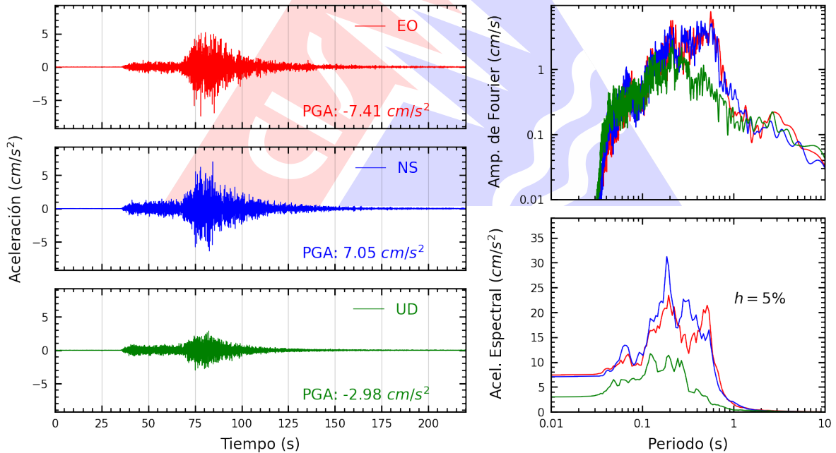
Figura A.22: Registros tiempo-historia, espectros de Fourier y de respuesta en las direcciones EO, NS y vertical de la estación VHAYA. Sismo de Ica, Ica - Ica del 2026-05-19, 12:57:51 (Hora local)
