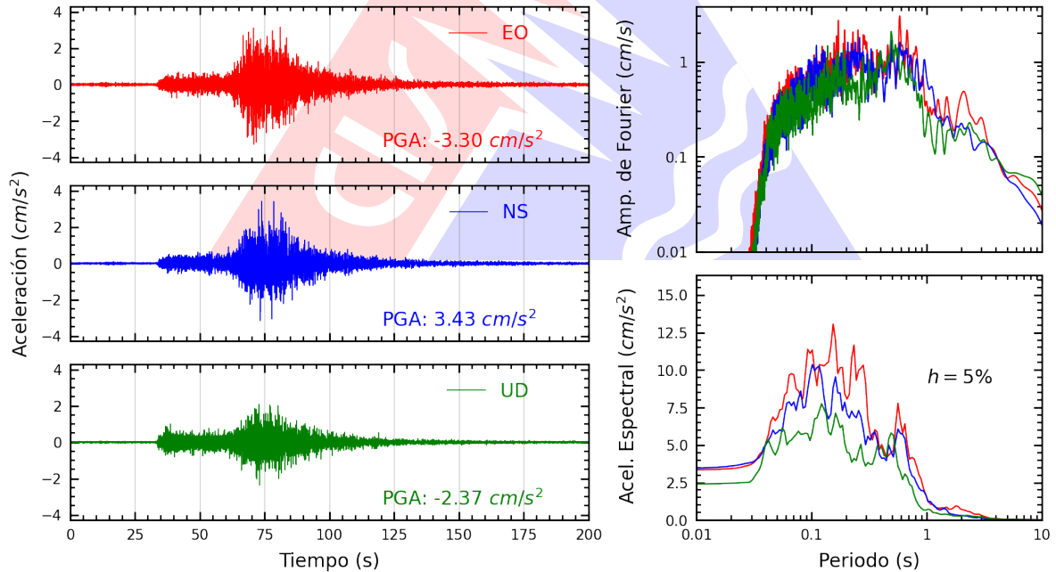
Figura A.40: Registros tiempo-historia, espectros de Fourier y de respuesta en las direcciones EO, NS y vertical de la estación INICT. Sismo de Ica, Ica - Ica del 2026-05-19, 12:57:51 (Hora local)
