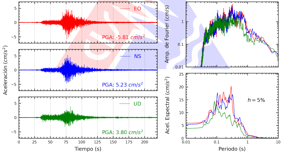
Figura A.26: Registros tiempo-historia, espectros de Fourier y de respuesta en las direcciones EO, NS y vertical de la estación MADRE. Sismo de Ica, Ica - Ica del 2026-05-19, 12:57:51 (Hora local)
