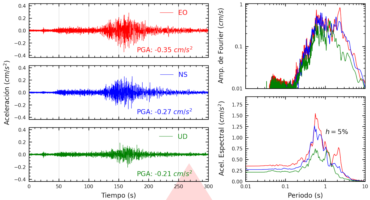
Figura A.51: Registros tiempo-historia, espectros de Fourier y de respuesta en las direcciones EO, NS y vertical de la estación UNC. Sismo de Ica, Ica - Ica del 2026-05-19, 12:57:51 (Hora local)
