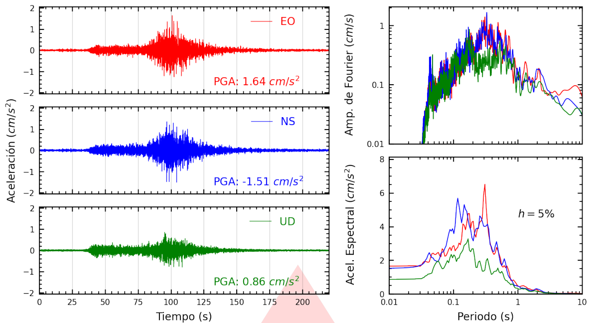
Figura A.43: Registros tiempo-historia, espectros de Fourier y de respuesta en las direcciones EO, NS y vertical de la estación UNAB. Sismo de Ica, Ica - Ica del 2026-05-19, 12:57:51 (Hora local)
