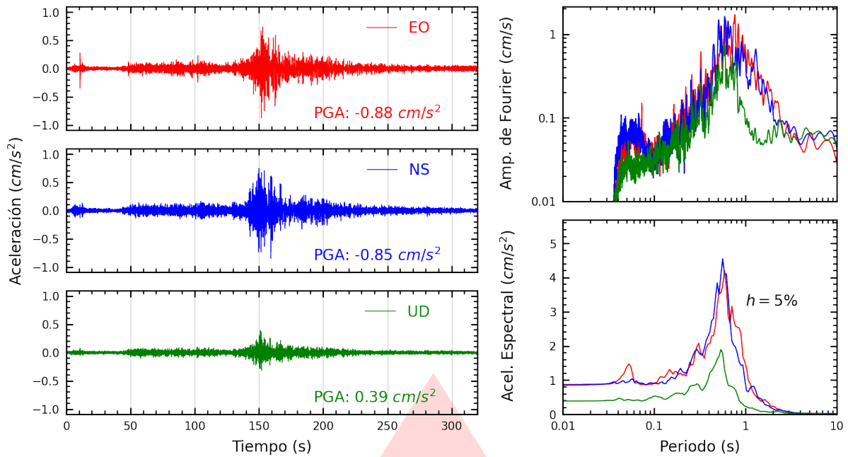
Figura A.45: Registros tiempo-historia, espectros de Fourier y de respuesta en las direcciones EO, NS y vertical de la estación UNTRM. Sismo de Ica, Ica - Ica del 2026-05-19, 12:57:51 (Hora local)
