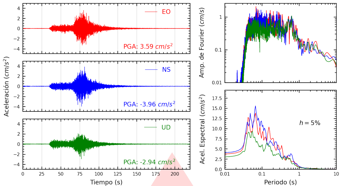
Figura A.37: Registros tiempo-historia, espectros de Fourier y de respuesta en las direcciones EO, NS y vertical de la estación SJLCE. Sismo de Ica, Ica - Ica del 2026-05-19, 12:57:51 (Hora local)
