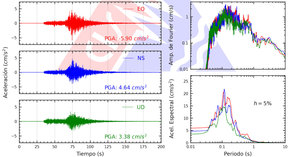
Figura A.24: Registros tiempo-historia, espectros de Fourier y de respuesta en las direcciones EO, NS y vertical de la estación JALVA. Sismo de Ica, Ica - Ica del 2026-05-19, 12:57:51 (Hora local)
