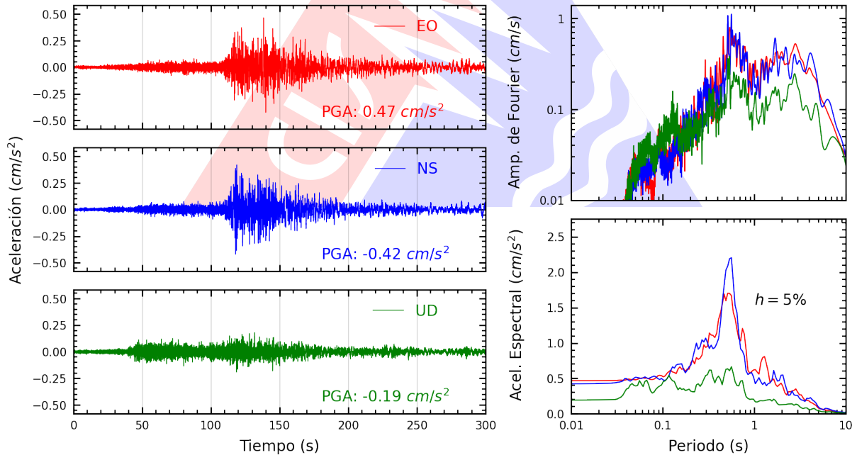
Figura A.50: Registros tiempo-historia, espectros de Fourier y de respuesta en las direcciones EO, NS y vertical de la estación UNIA. Sismo de Ica, Ica - Ica del 2026-05-19, 12:57:51 (Hora local)
