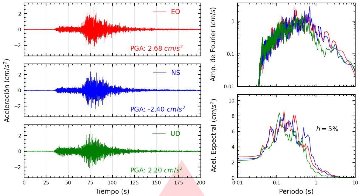
Figura A.41: Registros tiempo-historia, espectros de Fourier y de respuesta en las direcciones EO, NS y vertical de la estación BONDY. Sismo de Ica, Ica - Ica del 2026-05-19, 12:57:51 (Hora local)
