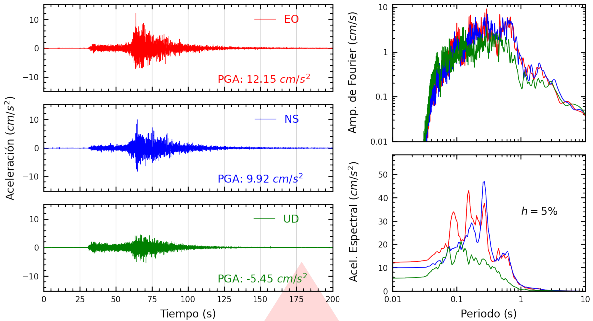
Figura A.11: Registros tiempo-historia, espectros de Fourier y de respuesta en las direcciones EO, NS y vertical de la estación USILP. Sismo de Ica, Ica - Ica del 2026-05-19, 12:57:51 (Hora local)
