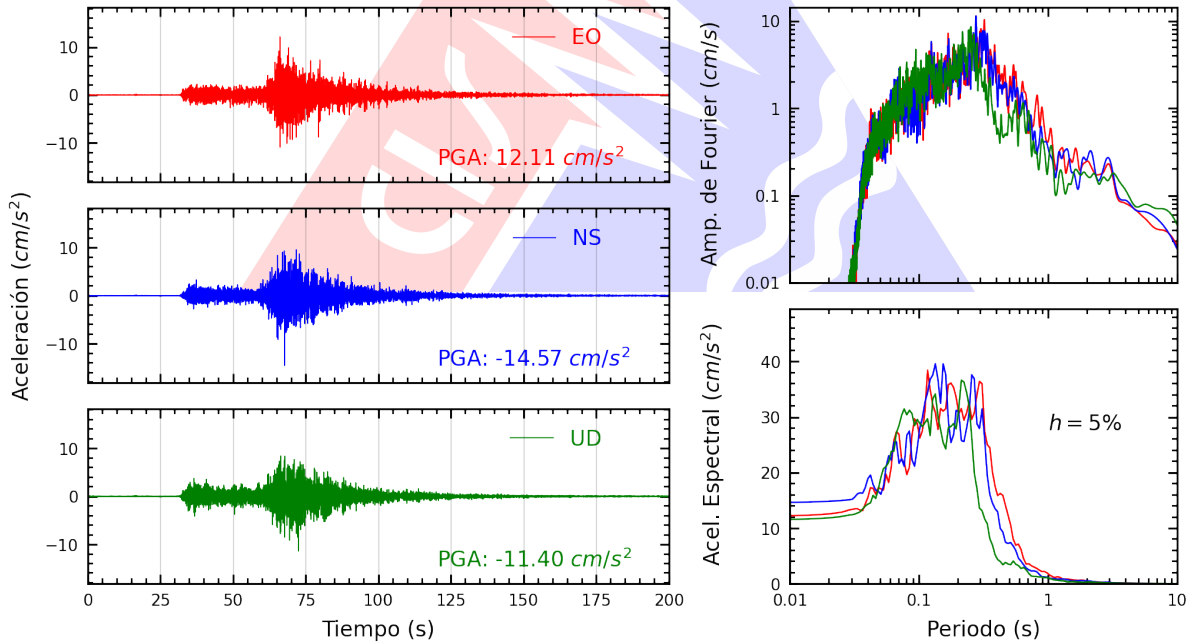
Figura A.8: Registros tiempo-historia, espectros de Fourier y de respuesta en las direcciones EO, NS y vertical de la estación SOVES. Sismo de Ica, Ica - Ica del 2026-05-19, 12:57:51 (Hora local)
