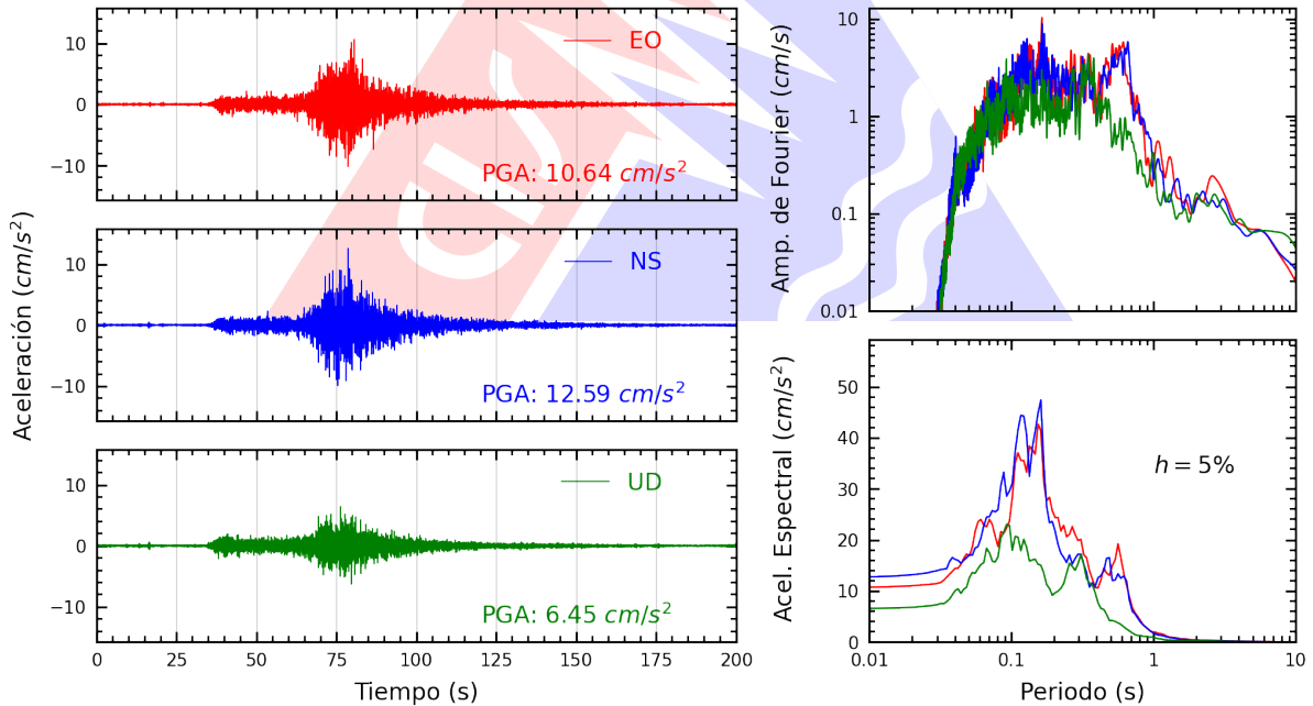
Figura A.10: Registros tiempo-historia, espectros de Fourier y de respuesta en las direcciones EO, NS y vertical de la estación SJLSV. Sismo de Ica, Ica - Ica del 2026-05-19, 12:57:51 (Hora local)
