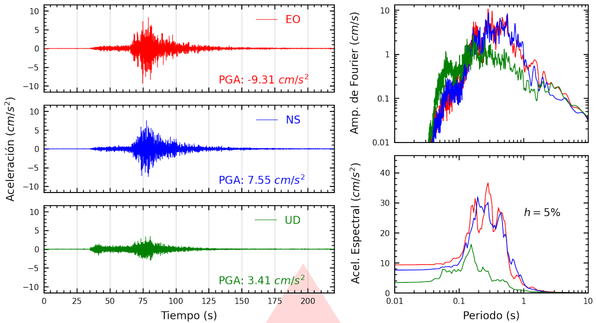
Figura A.17: Registros tiempo-historia, espectros de Fourier y de respuesta en las direcciones EO, NS y vertical de la estación ACAPU. Sismo de Ica, Ica - Ica del 2026-05-19, 12:57:51 (Hora local)
