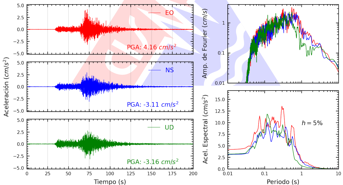
Figura A.36: Registros tiempo-historia, espectros de Fourier y de respuesta en las direcciones EO, NS y vertical de la estación UNFV. Sismo de Ica, Ica - Ica del 2026-05-19, 12:57:51 (Hora local)
