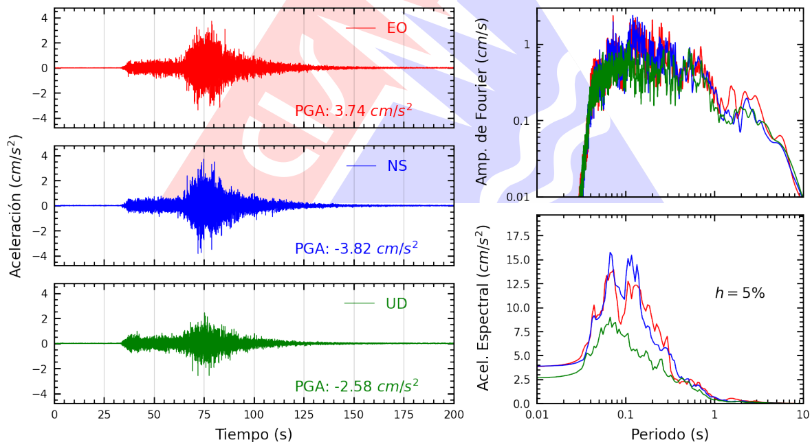
Figura A.38: Registros tiempo-historia, espectros de Fourier y de respuesta en las direcciones EO, NS y vertical de la estación ATARJ. Sismo de Ica, Ica - Ica del 2026-05-19, 12:57:51 (Hora local)
