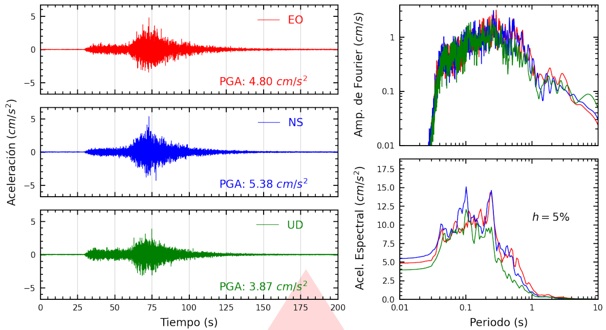
Figura A.31: Registros tiempo-historia, espectros de Fourier y de respuesta en las direcciones EO, NS y vertical de la estación USMP. Sismo de Ica, Ica - Ica del 2026-05-19, 12:57:51 (Hora local)
