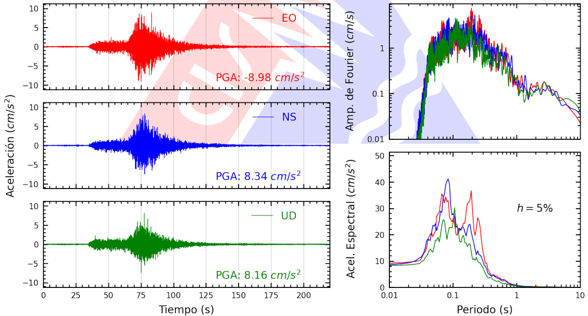
Figura A.18: Registros tiempo-historia, espectros de Fourier y de respuesta en las direcciones EO, NS y vertical de la estación INDEP. Sismo de Ica, Ica - Ica del 2026-05-19, 12:57:51 (Hora local)
