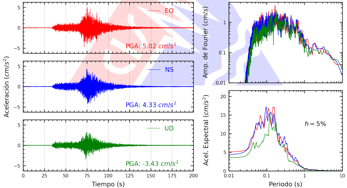
Figura A.32: Registros tiempo-historia, espectros de Fourier y de respuesta en las direcciones EO, NS y vertical de la estación FICPE. Sismo de Ica, Ica - Ica del 2026-05-19, 12:57:51 (Hora local)
