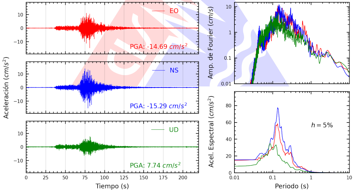
Figura A.6: Registros tiempo-historia, espectros de Fourier y de respuesta en las direcciones EO, NS y vertical de la estación CARAB. Sismo de Ica, Ica - Ica del 2026-05-19, 12:57:51 (Hora local)
