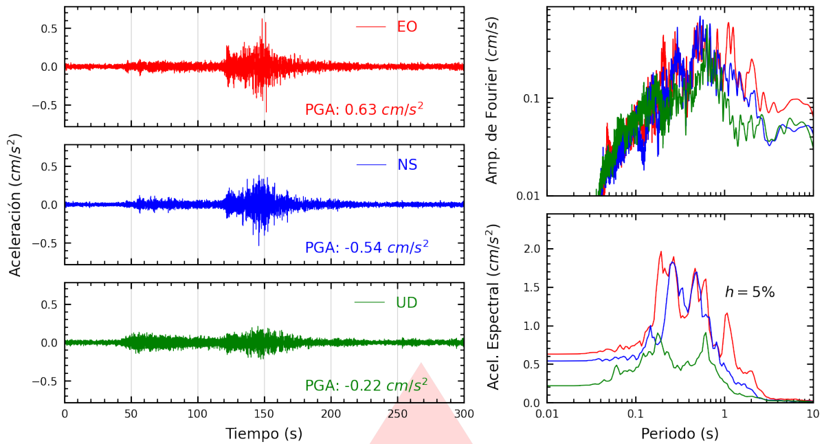
Figura A.47: Registros tiempo-historia, espectros de Fourier y de respuesta en las direcciones EO, NS y vertical de la estación UPAOT. Sismo de Ica, Ica - Ica del 2026-05-19, 12:57:51 (Hora local)
