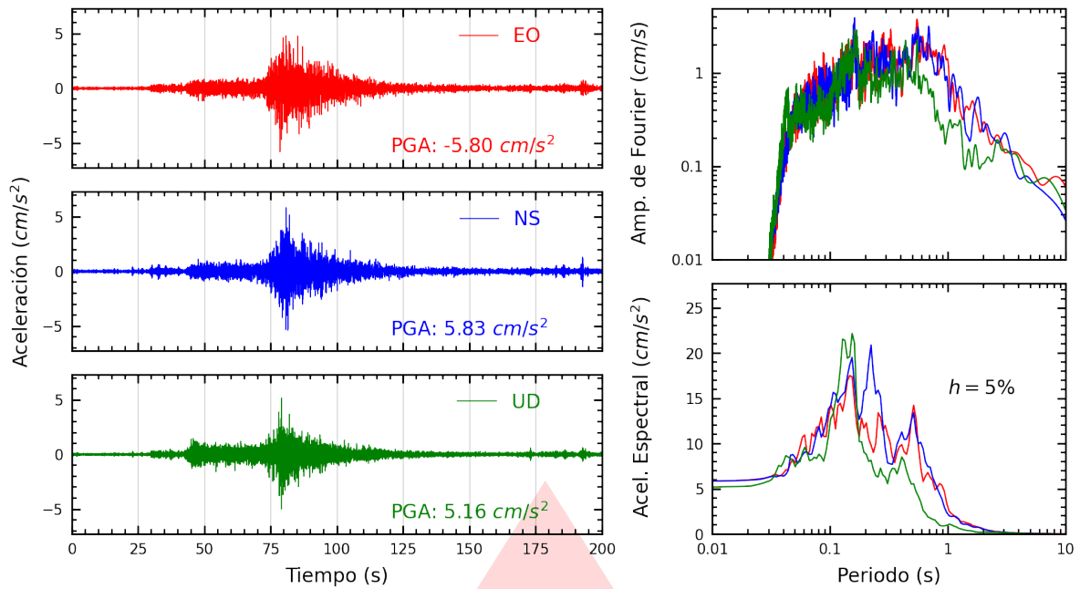
Figura A.25: Registros tiempo-historia, espectros de Fourier y de respuesta en las direcciones EO, NS y vertical de la estación UPCSM. Sismo de Ica, Ica - Ica del 2026-05-19, 12:57:51 (Hora local)
