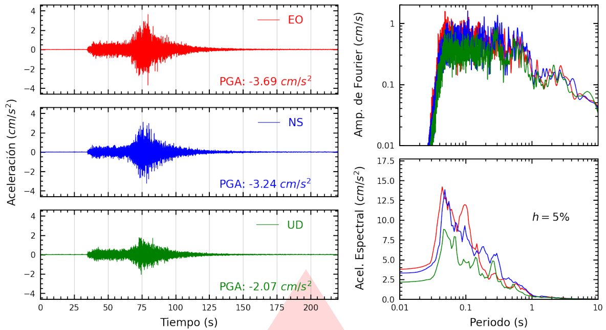
Figura A.39: Registros tiempo-historia, espectros de Fourier y de respuesta en las direcciones EO, NS y vertical de la estación UCSS. Sismo de Ica, Ica - Ica del 2026-05-19, 12:57:51 (Hora local)
