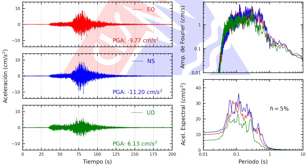
Figura A.14: Registros tiempo-historia, espectros de Fourier y de respuesta en las direcciones EO, NS y vertical de la estación SJLSC. Sismo de Ica, Ica - Ica del 2026-05-19, 12:57:51 (Hora local)
