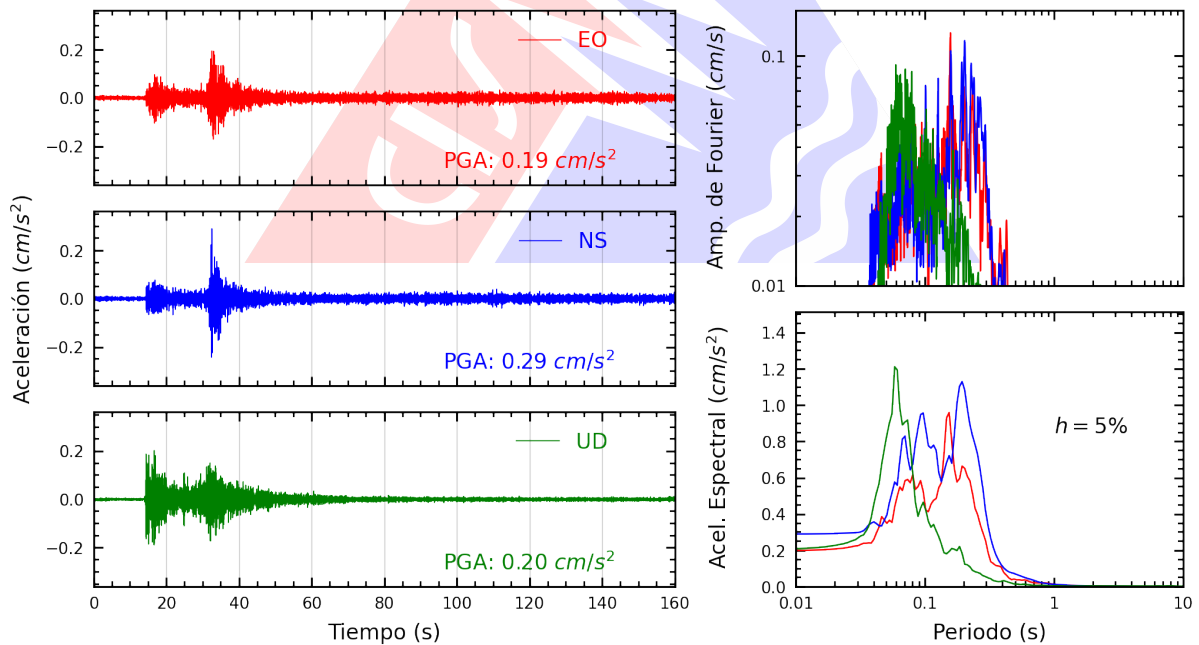
Figura A.2: Registros tiempo-historia, espectros de Fourier y de respuesta en las direcciones EO, NS y vertical de la estación UNAAA. Sismo de Nueva Cajamarca, Rioja - San Martín del 2026-06-17, 23:33:33 (Hora local)
