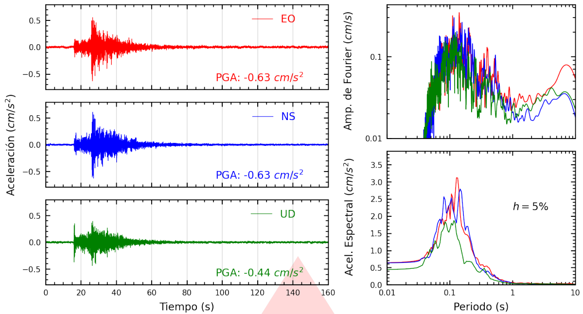
Figura A.1: Registros tiempo-historia, espectros de Fourier y de respuesta en las direcciones EO, NS y vertical de la estación UNTRM. Sismo de Nueva Cajamarca, Rioja - San Martín del 2026-06-17, 23:33:33 (Hora local)
