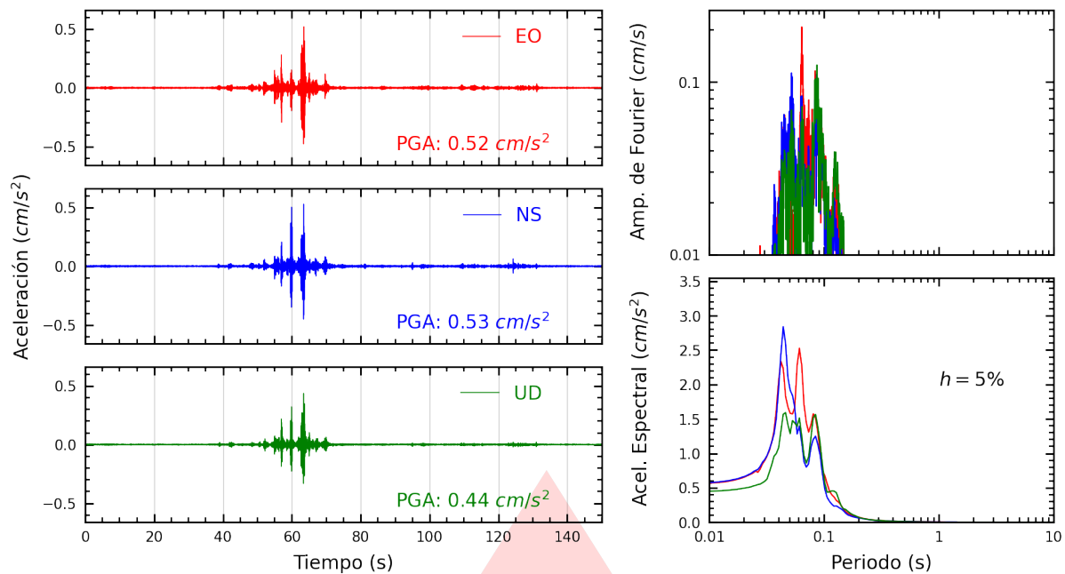
Figura A.1: Registros tiempo-historia, espectros de Fourier y de respuesta en las direcciones EO, NS y vertical de la estación UPAOP. Sismo de Jaén, Jaén - Cajamarca del 2026-06-19, 01:58:17 (Hora local)
