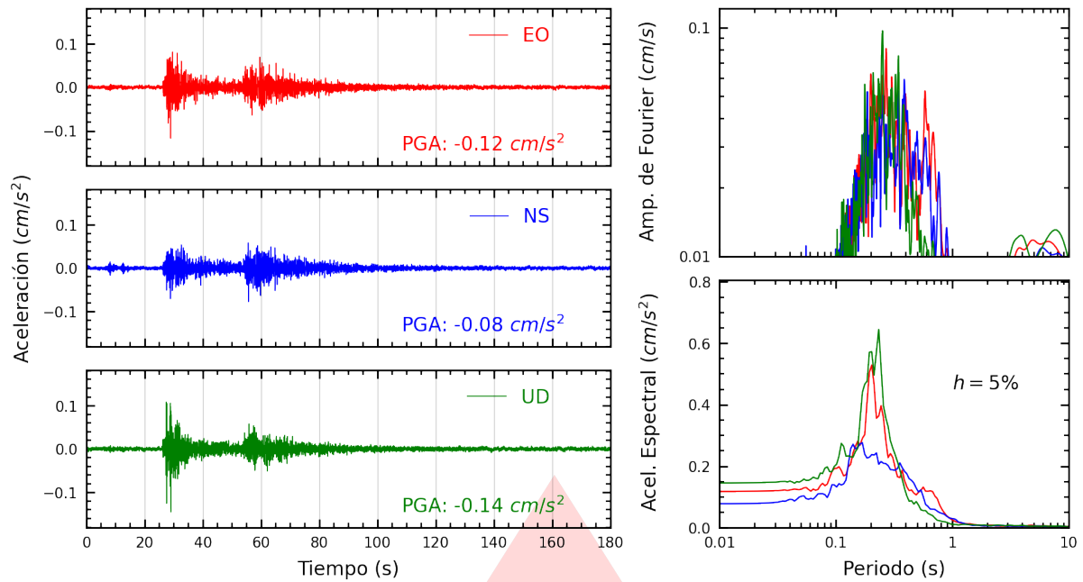
Figura A.3: Registros tiempo-historia, espectros de Fourier y de respuesta en las direcciones EO, NS y vertical de la estación CARAL. Sismo de Pozuzo, Oxapampa - Pasco del 2026-07-03, 16:24:06 (Hora local)
