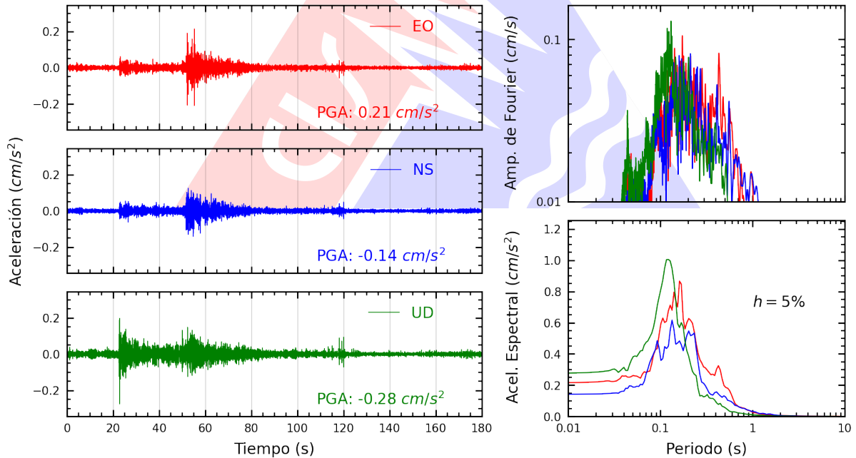
Figura A.2: Registros tiempo-historia, espectros de Fourier y de respuesta en las direcciones EO, NS y vertical de la estación UNIA. Sismo de Pozuzo, Oxapampa - Pasco del 2026-07-03, 16:24:06 (Hora local)
