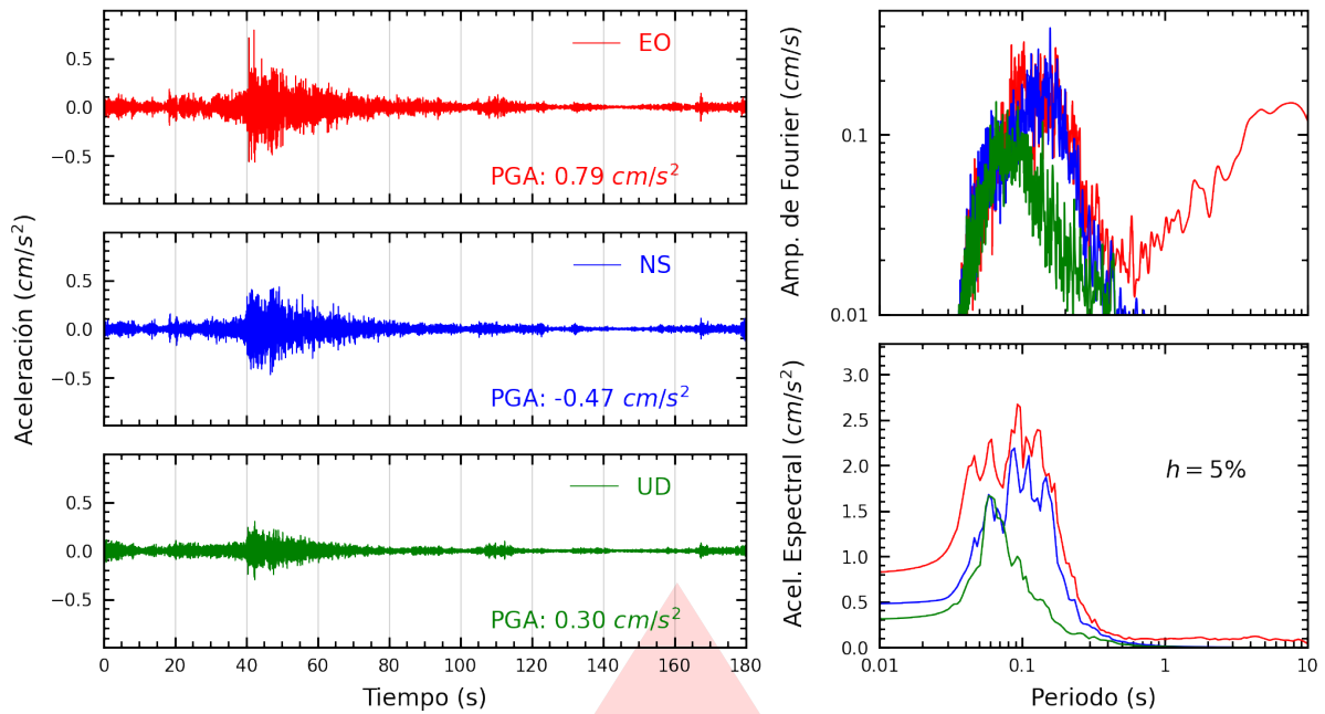
Figura A.1: Registros tiempo-historia, espectros de Fourier y de respuesta en las direcciones EO, NS y vertical de la estación UNAS. Sismo de Pozuzo, Oxapampa - Pasco del 2026-07-03, 16:24:06 (Hora local)
